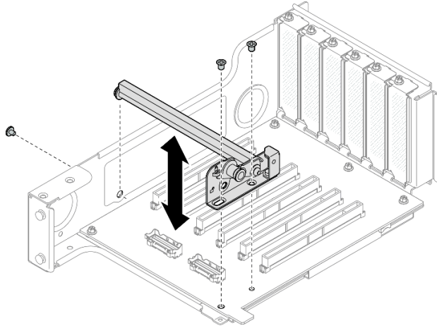
그림 167. 라이저에 PCIe 고정장치 설치
