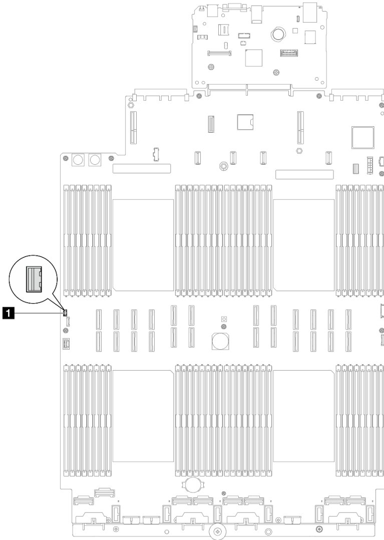
그림 100. 침입 스위치 분리
