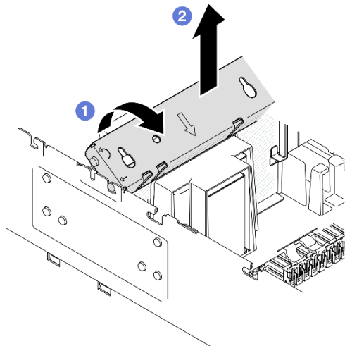
그림 67. 크로스바 제거
