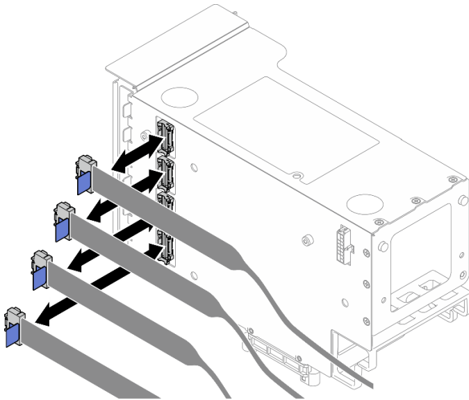
그림 143. 라이저 외부에서 PCIe 케이블 분리
