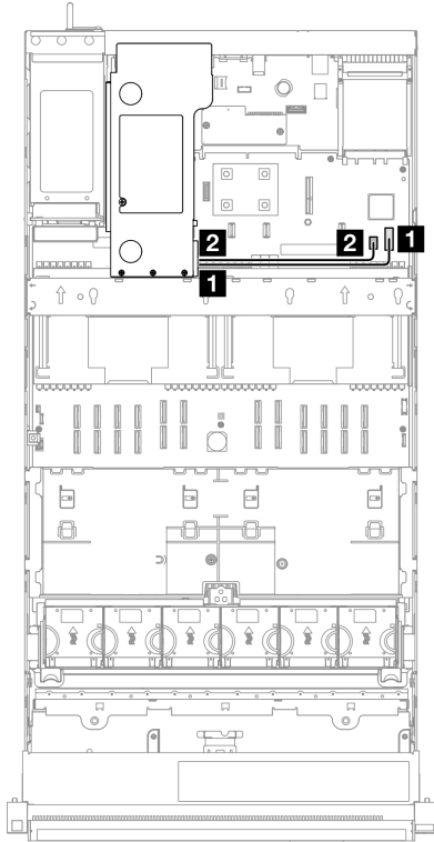
그림 227. 7mm 드라이브 백플레인의 케이블 배선
