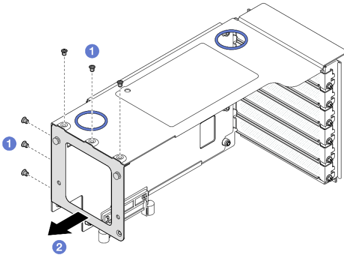
그림 174. FH PCIe 라이저에서 필터 제거
