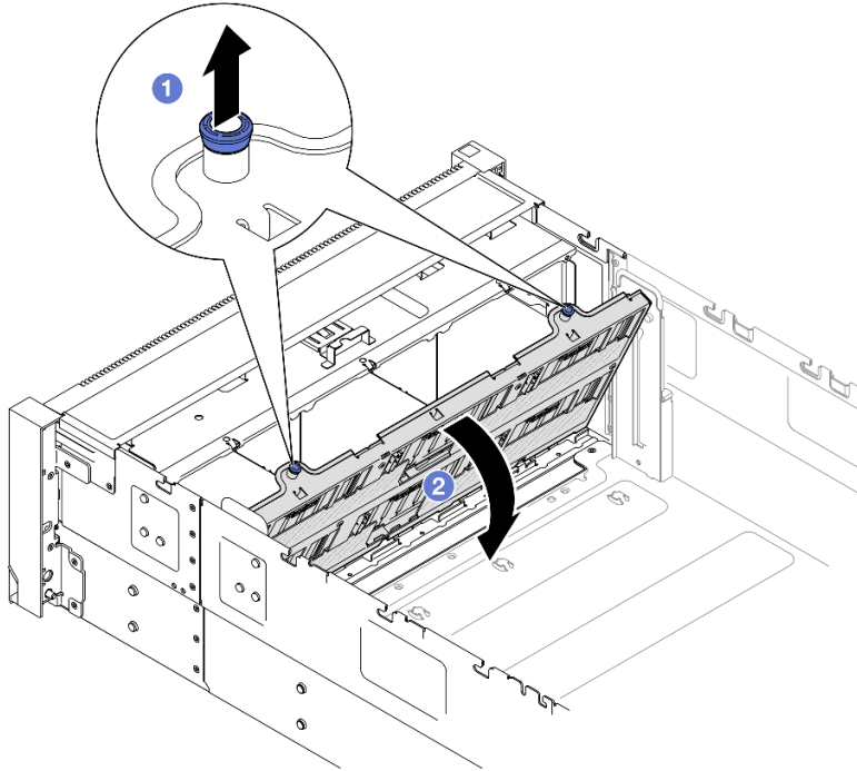
그림 73. 드라이브 백플레인 캐리어 어셈블리 제거
