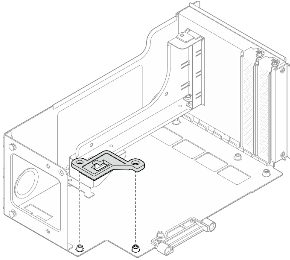
그림 141. 라이저에서 커넥터 가이드 제거
