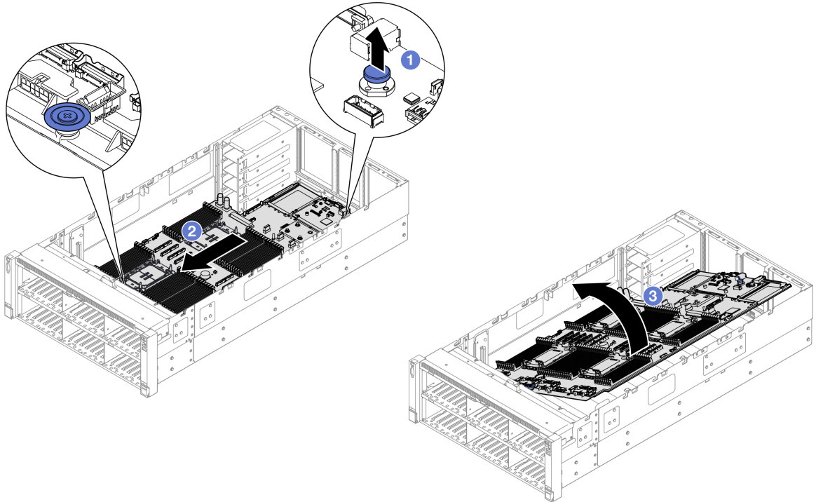
그림 213. 시스템 보드 어셈블리 제거
