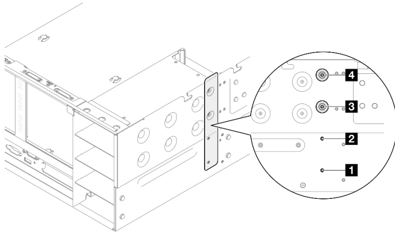
그림 187. 전원 공급 장치 키 나사 제거
