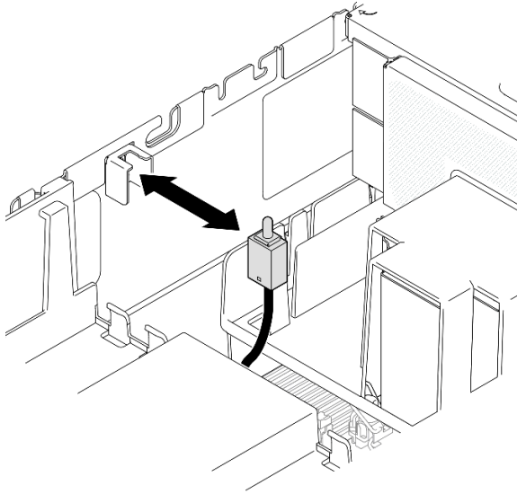
그림 102. 침입 스위치 설치
