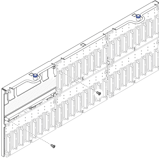
그림 75. 백플레인 캐리어의 예비 나사
