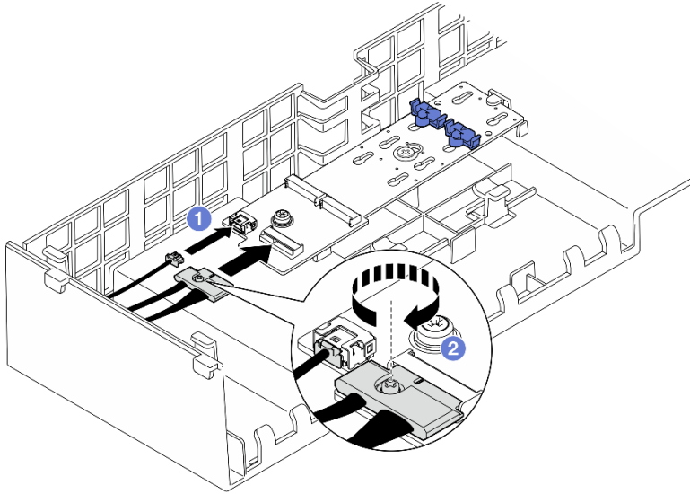
그림 46. SATA/NVMe 또는 NVMe M.2 부트 어댑터에 케이블 연결
