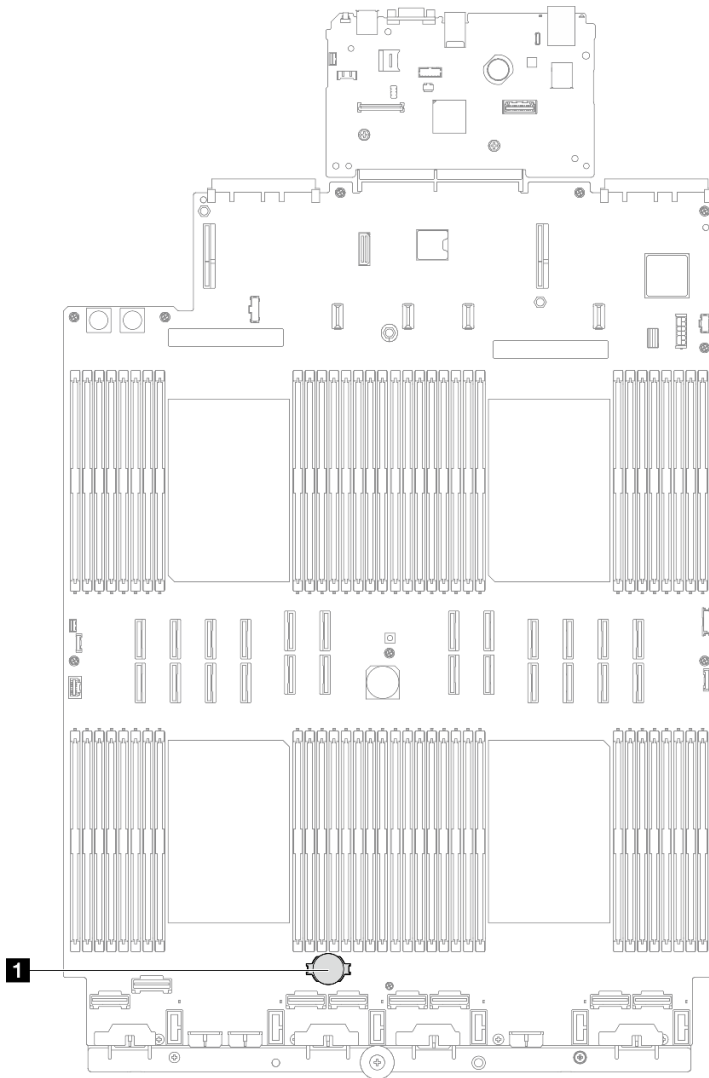
그림 60. CMOS 배터리 위치
