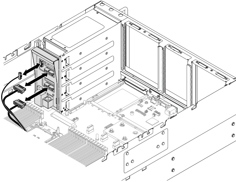
그림 182. 전원 분배 보드 케이블 연결
