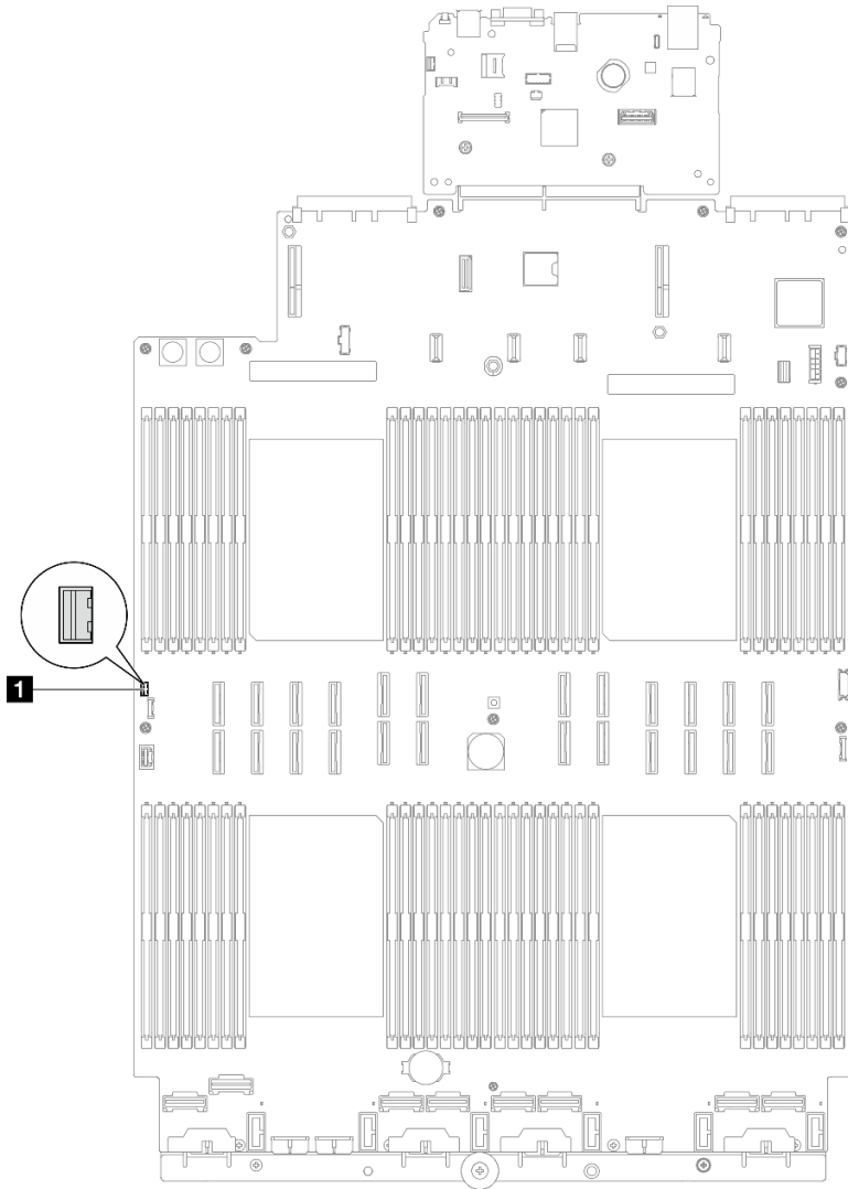
그림 103. 침입 스위치 연결
