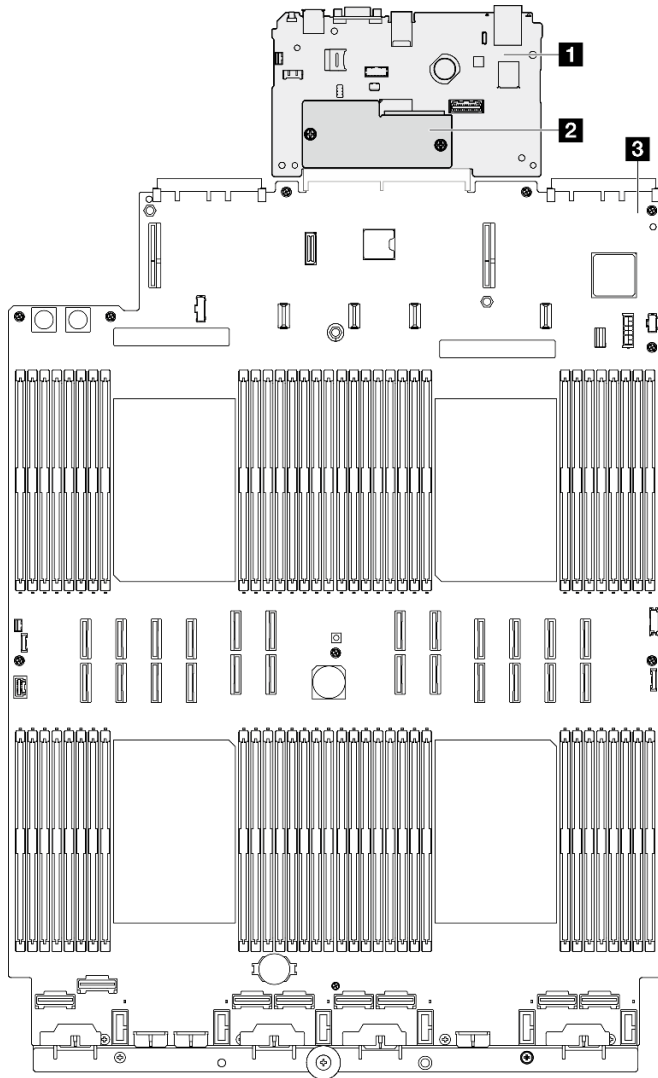
그림 210. 시스템 보드 어셈블리 레이아웃
