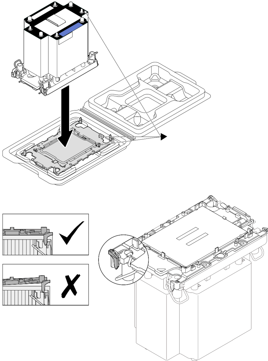
그림 201. 운송 트레이 내 프로세서로 PHM 조립
