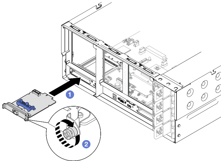
그림 115. 관리 NIC 어댑터 설치
