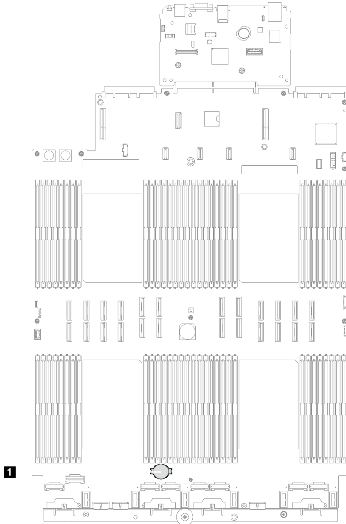
그림 63. CMOS 배터리 위치
