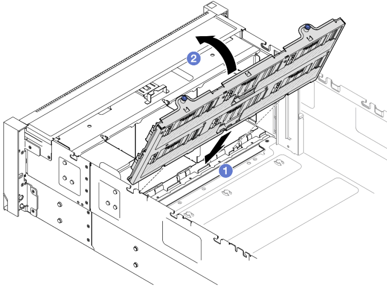
그림 79. 드라이브 백플레인 캐리어 어셈블리 설치
