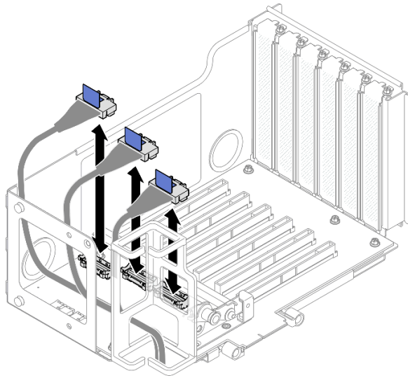
그림 144. 라이저 내부에서 PCIe 케이블 분리
