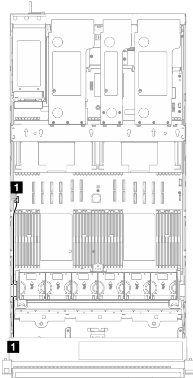
그림 230. 앞면 VGA 어셈블리의 케이블 배선
