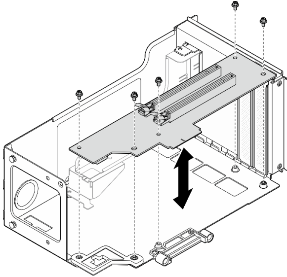
그림 154. 라이저에 PCIe 라이저 카드 설치
