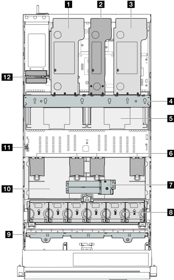
그림 8. 서버 평면도
