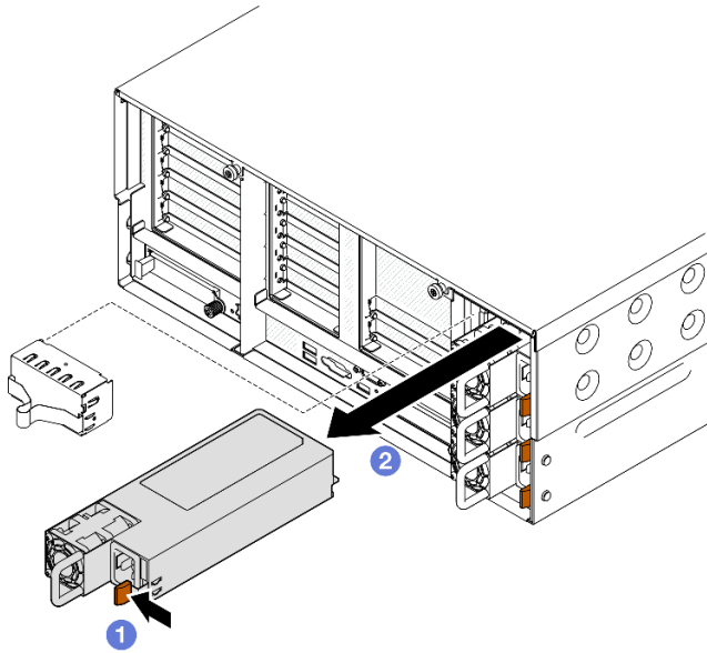
그림 191. 전원 공급 장치 제거
