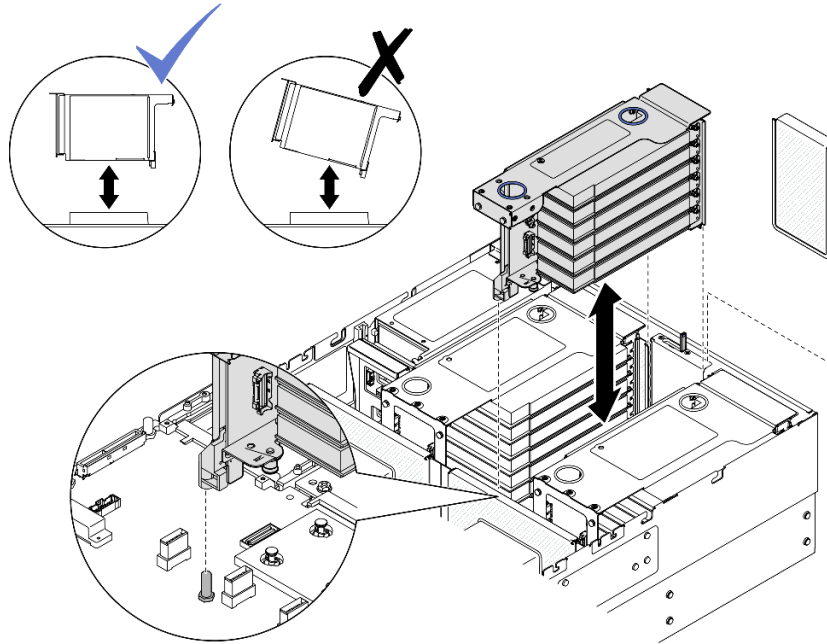
그림 123. PCIe 라이저 2 제거
