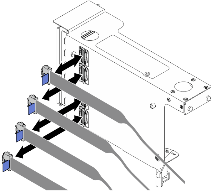
그림 149. 라이저 외부에서 PCIe 케이블 분리
