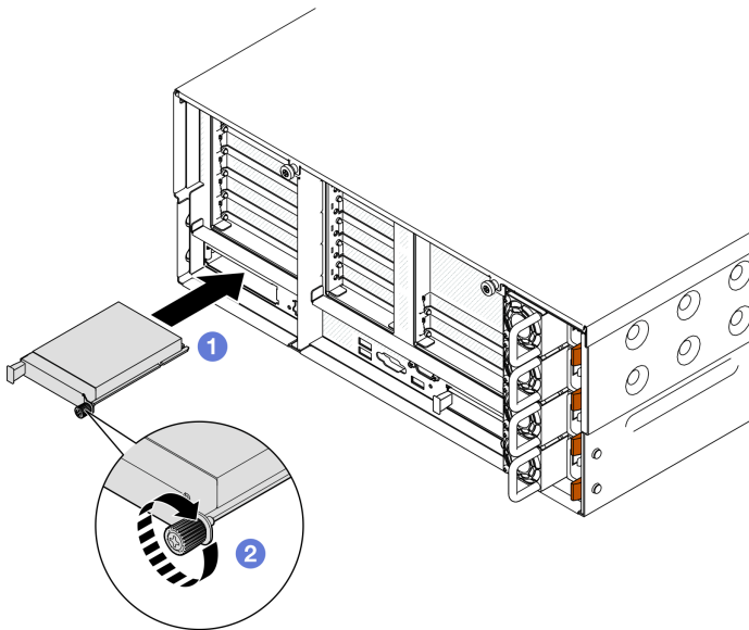
그림 121. OCP 모듈 설치
