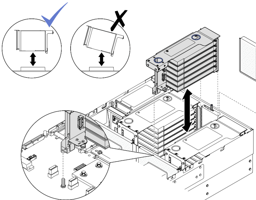
그림 136. PCIe 라이저 2 설치
