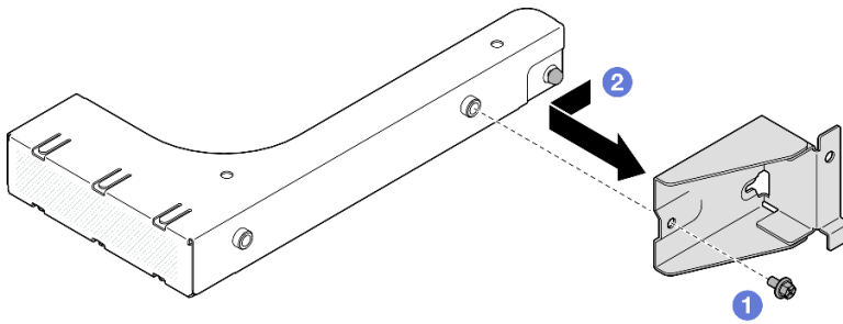
그림 30. 7mm 드라이브 케이스 브래킷 제거
