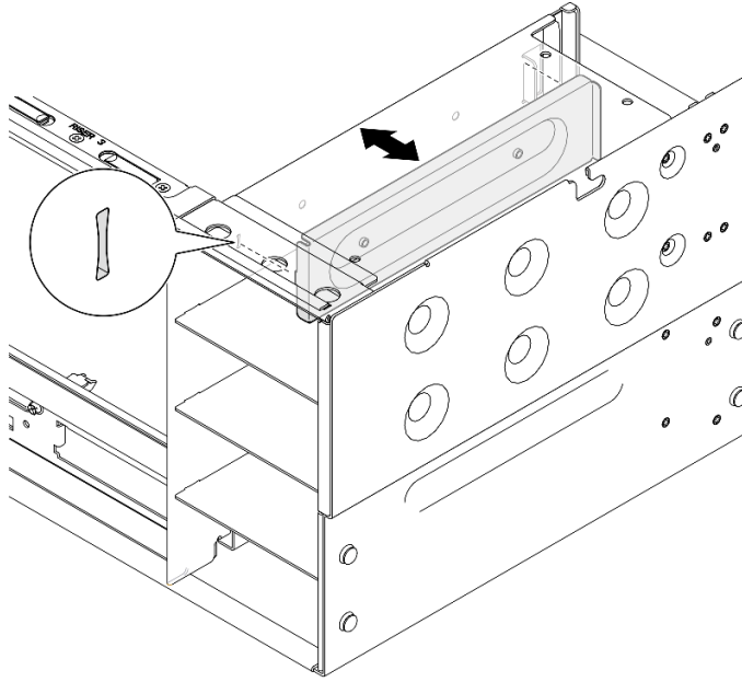
그림 185. 전원 공급 장치 브래킷 설치
