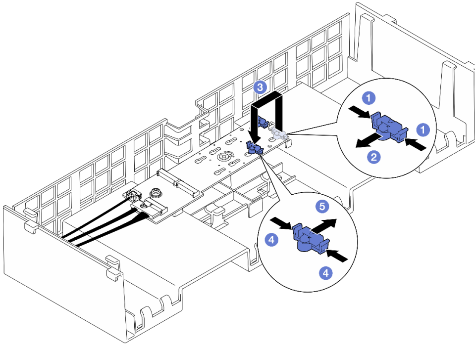
그림 111. M.2 고정장치 조정
