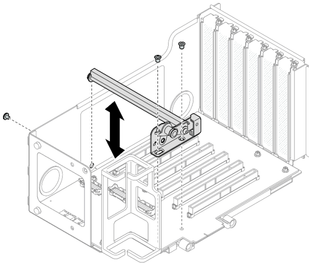
그림 159. 라이저에 PCIe 고정장치 설치
