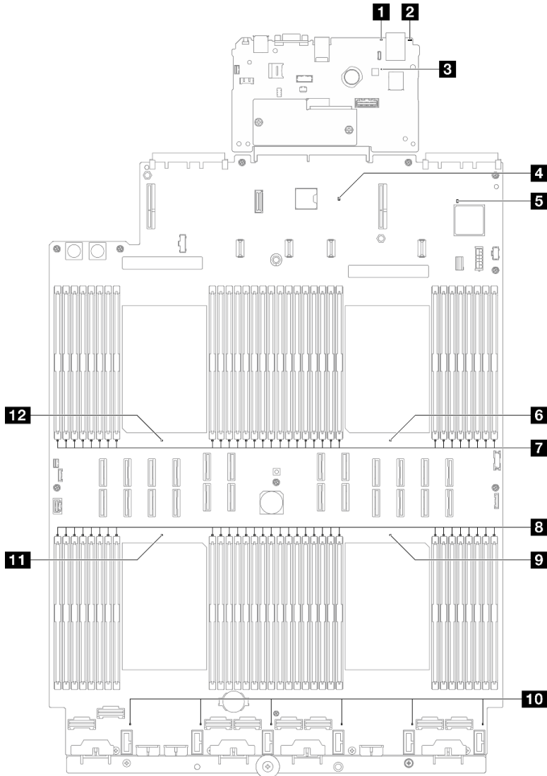
그림 244. 시스템 보드 어셈블리 LED
