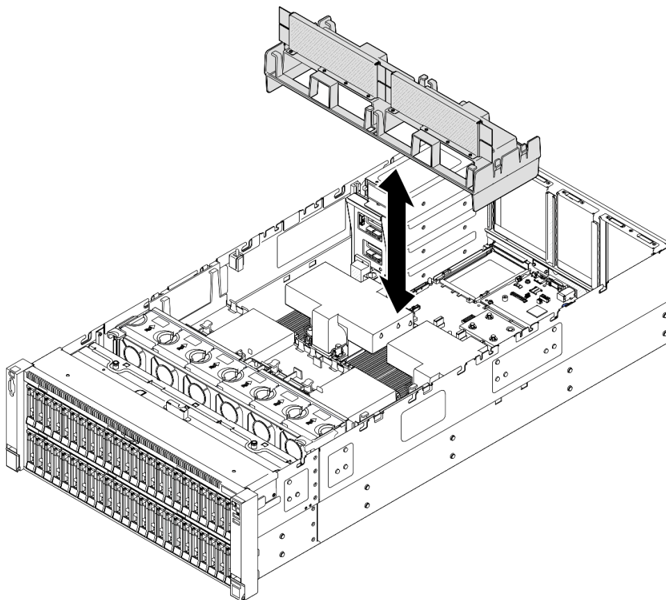
그림 53. 2U 성능 PHM용 뒷면 공기 조절 장치 제거
