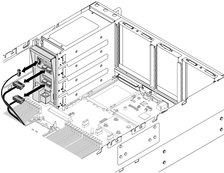
그림 178. 전원 분배 보드 케이블 분리
