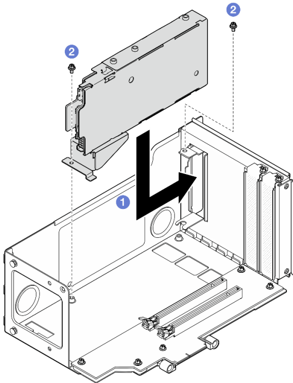
그림 32. 라이저에 7mm 드라이브 케이지 설치
