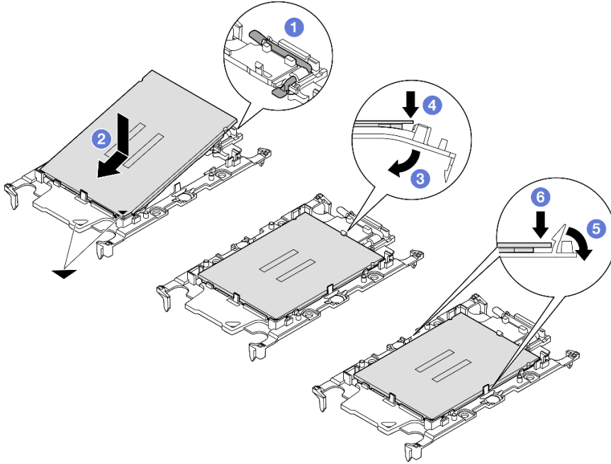
그림 199. 프로세서 캐리어 설치
