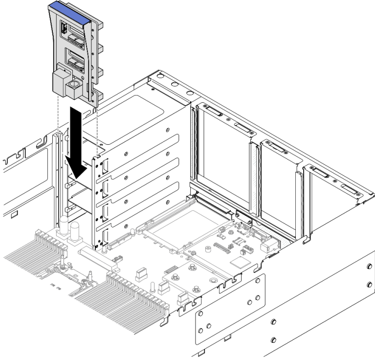
그림 181. 전원 분배 보드 설치
