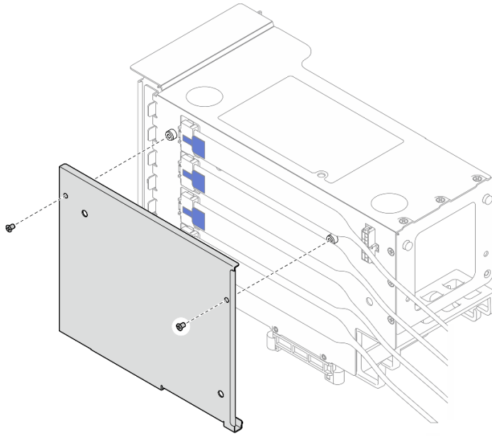
그림 163. 라이저에 덮개 설치
