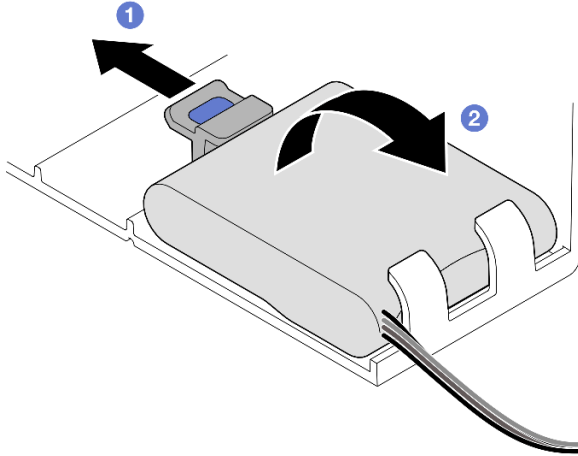
그림 85. 플래시 전원 모듈 제거
