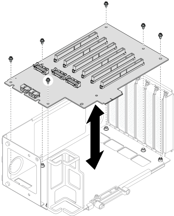
그림 146. 라이저에서 PCIe 라이저 카드 제거
