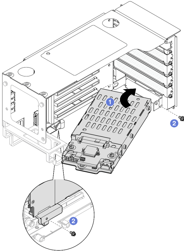
그림 35. 라이저에 7mm 드라이브 케이스 설치
