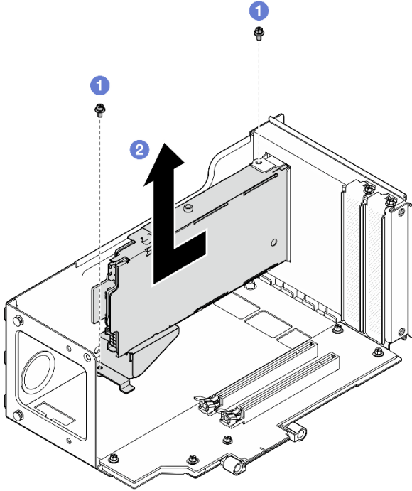
그림 20. 라이저에서 7mm 드라이브 케이스 제거
