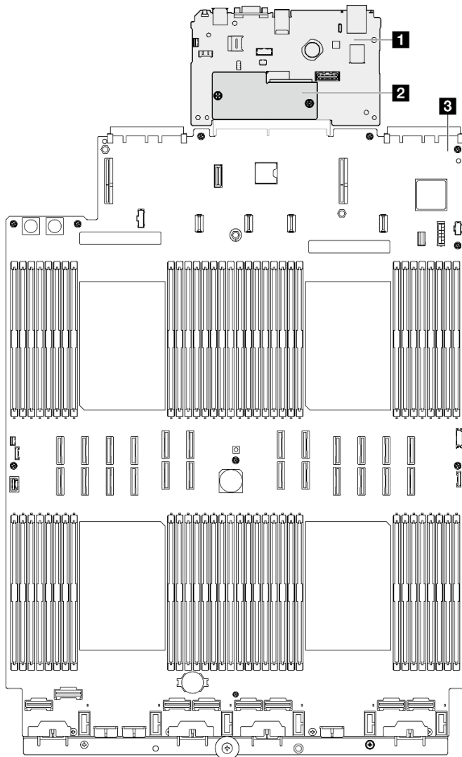
그림 10. 시스템 보드 어셈블리 레이아웃
