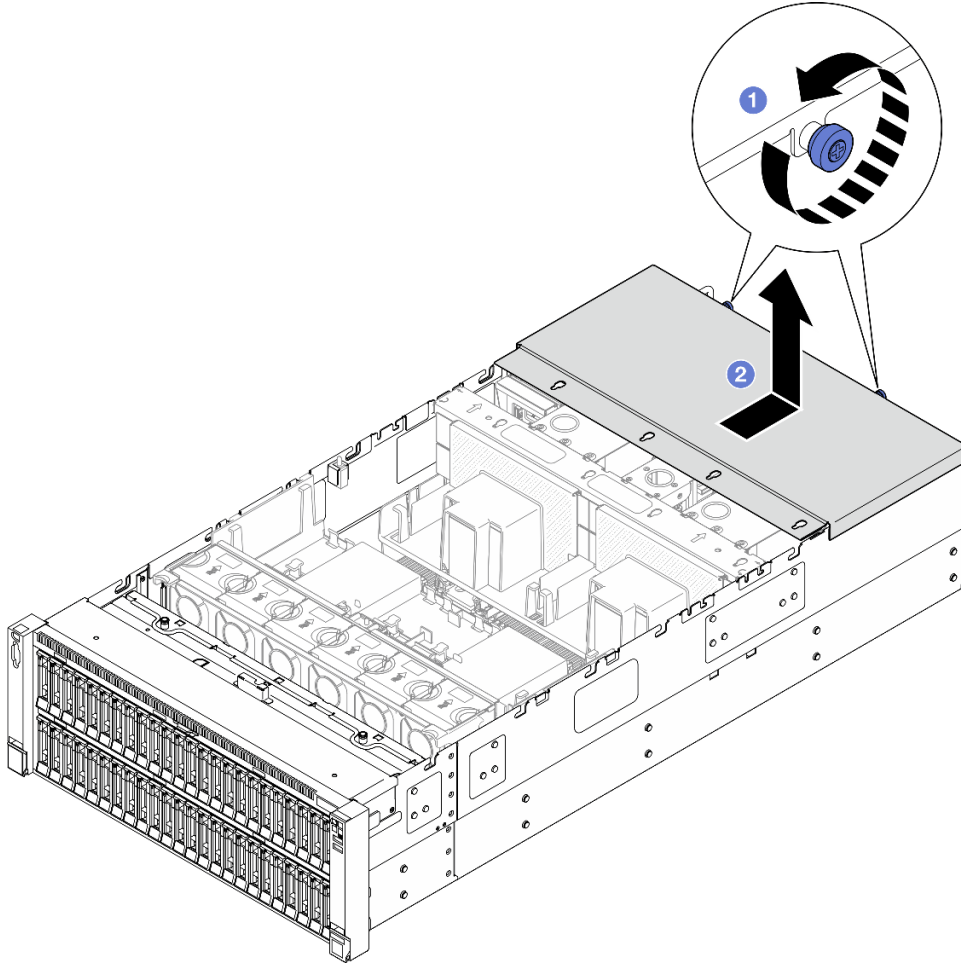
그림 219. 뒤쪽 윗면 덮개 제거
