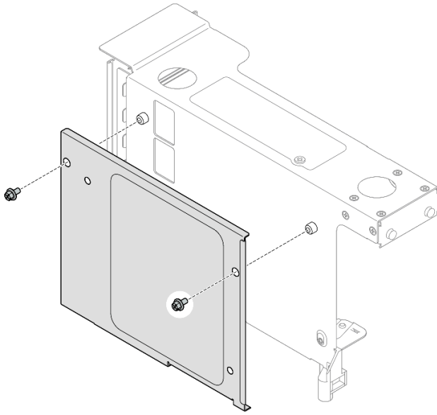
그림 169. 라이저에서 덮개 제거
