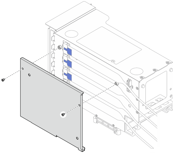
그림 142. 라이저에서 덮개 제거
