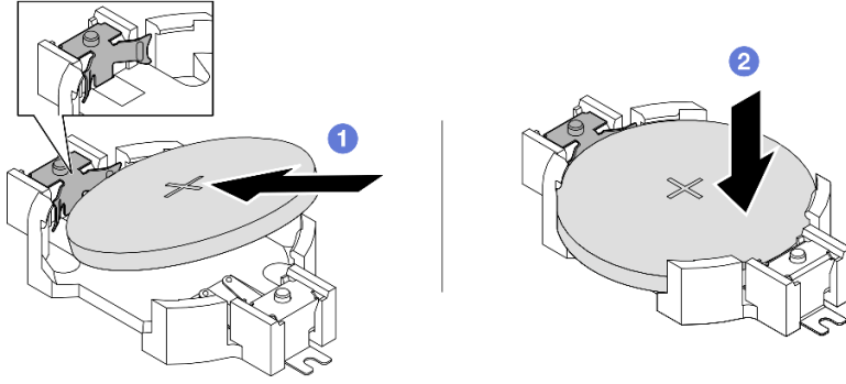
그림 64. CMOS 배터리 설치
