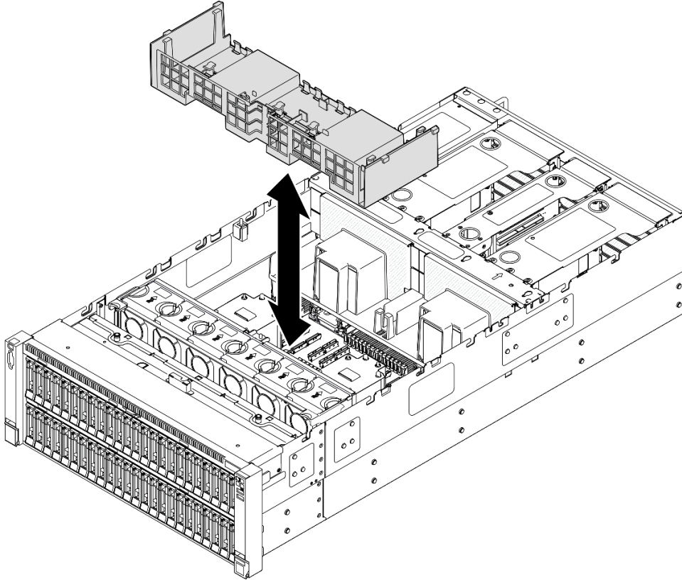
그림 42. 앞면 공기 조절 장치 제거
