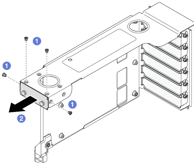
그림 176. FH PCIe 라이저에서 필터 제거
