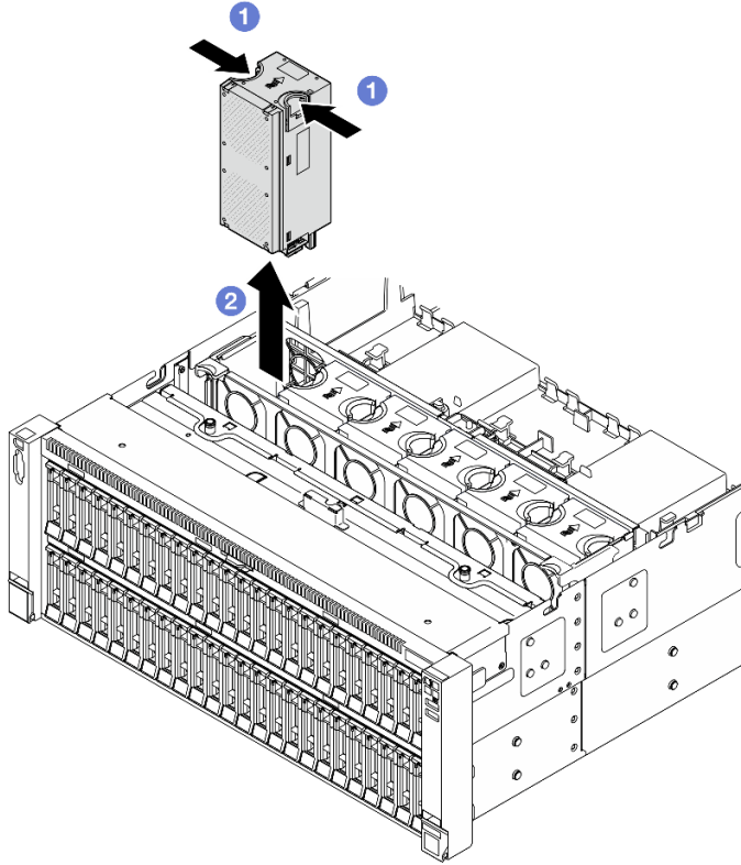
그림 80. 팬 모듈 제거
