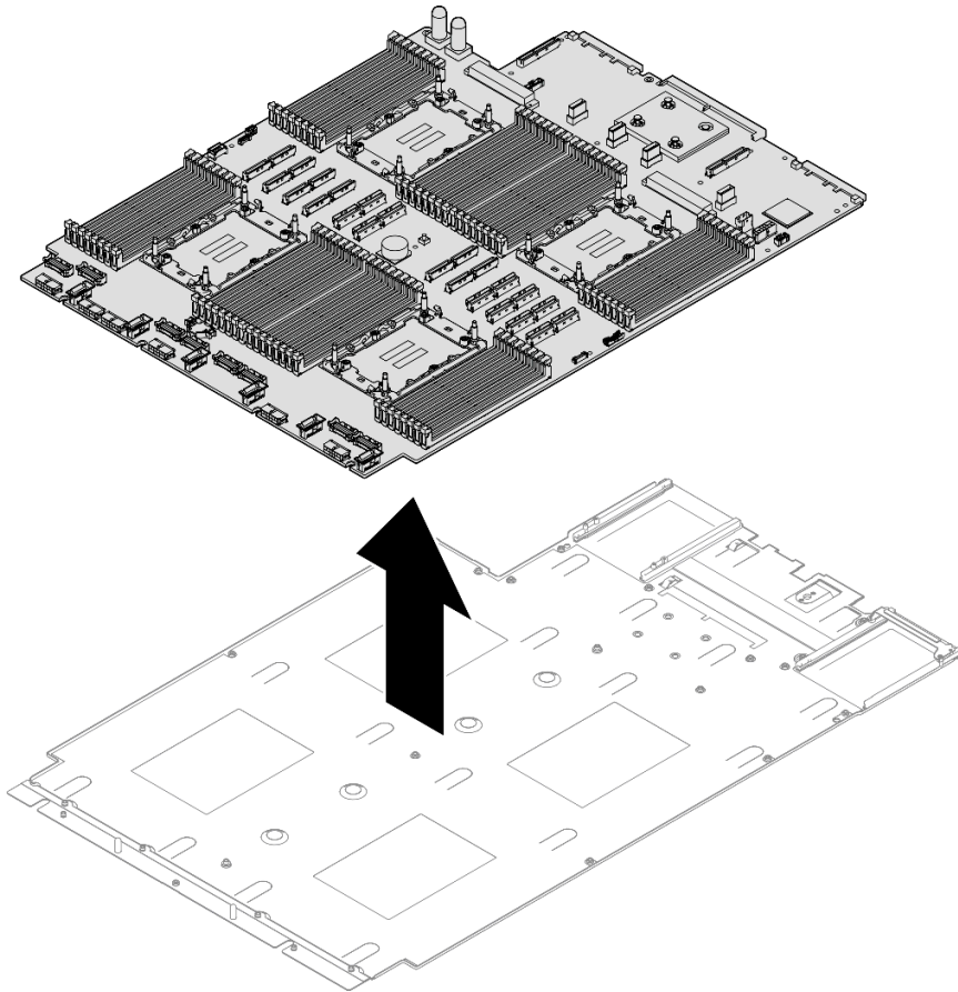
그림 250. 프로세서 보드 분해
