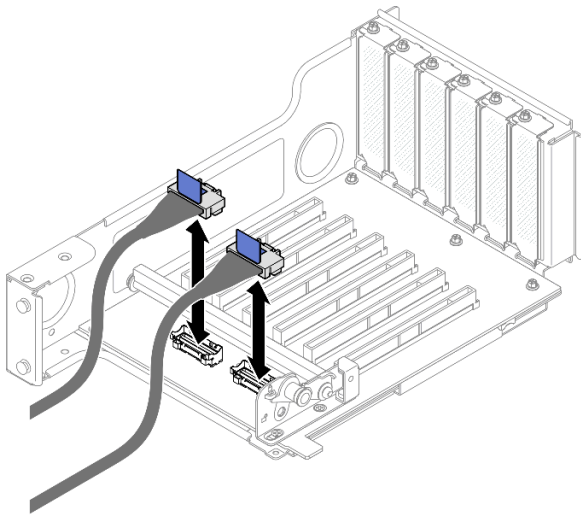
그림 150. 라이저 내부에서 PCIe 케이블 분리
