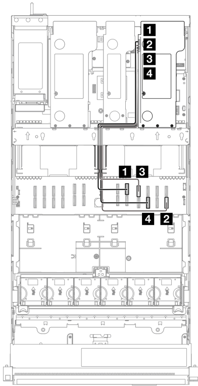
6슬롯 Gen 4 FH 라이저(PCle 라이저 1)의 케이블 배선
