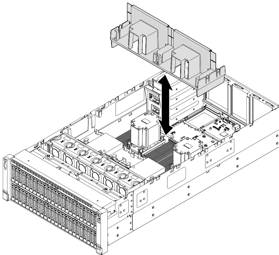
그림 52. 3U 표준 PHM용 뒷면 공기 조절 장치 제거
