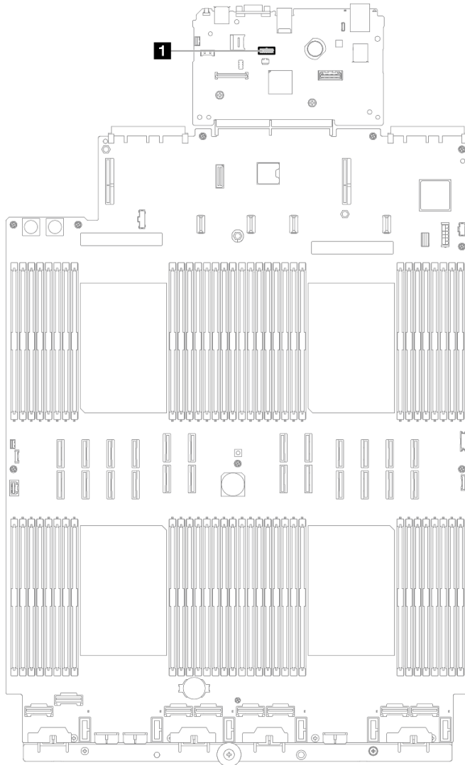
그림 209. 직렬 포트 모듈 연결
