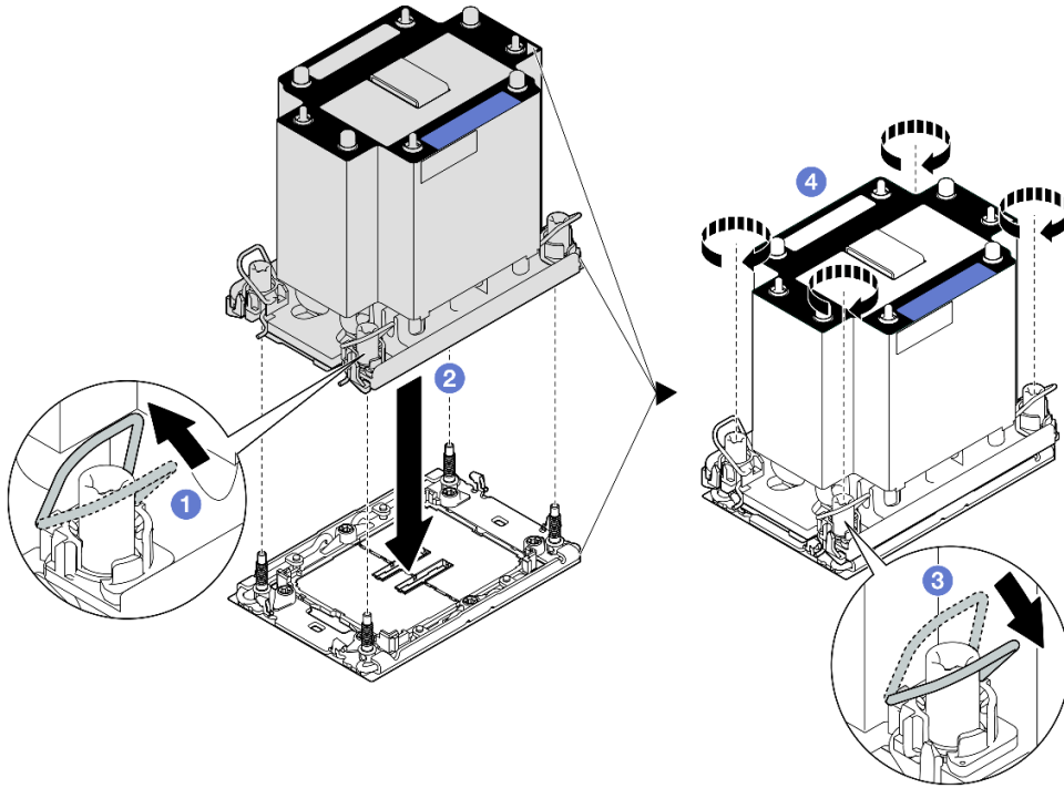
그림 202. 3U 표준 PHM 설치
