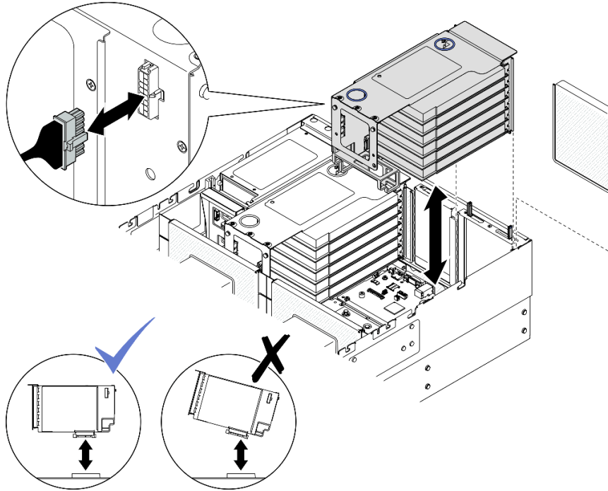
그림 124. PCIe 라이저 1 제거
