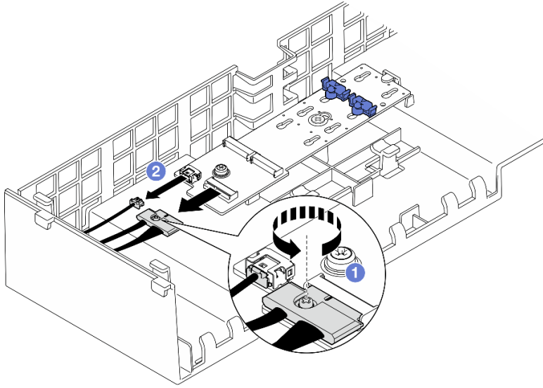
그림 40. SATA/NVMe 또는 NVMe M.2 부트 어댑터에서 케이블 분리
