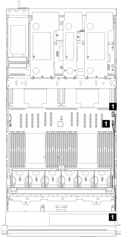
그림 229. 앞면 I/O 모듈의 케이블 배선
