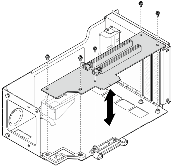
그림 140. 라이저에서 PCIe 라이저 카드 제거
