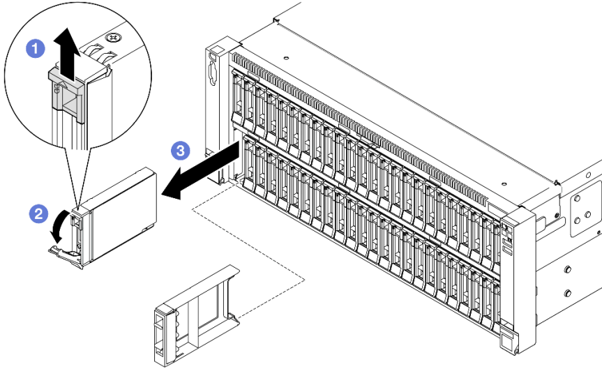
그림 71. 2.5인치 드라이브 제거
