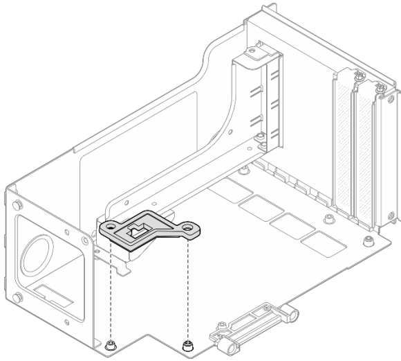
그림 153. 라이저에 커넥터 가이드 설치
