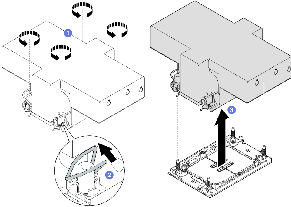
그림 195. 2U 성능 PHM 제거
