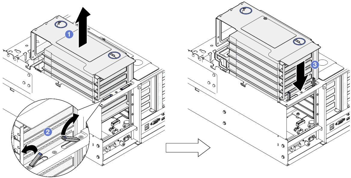
그림 66. PCIe 라이저 분리
