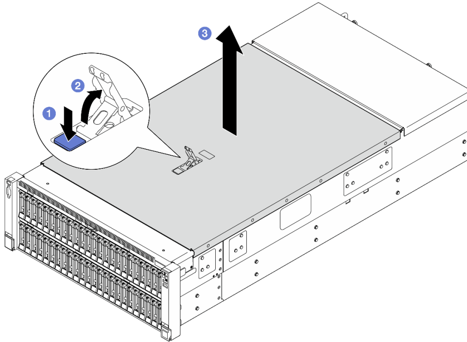
그림 218. 앞쪽 윗면 덮개 제거
