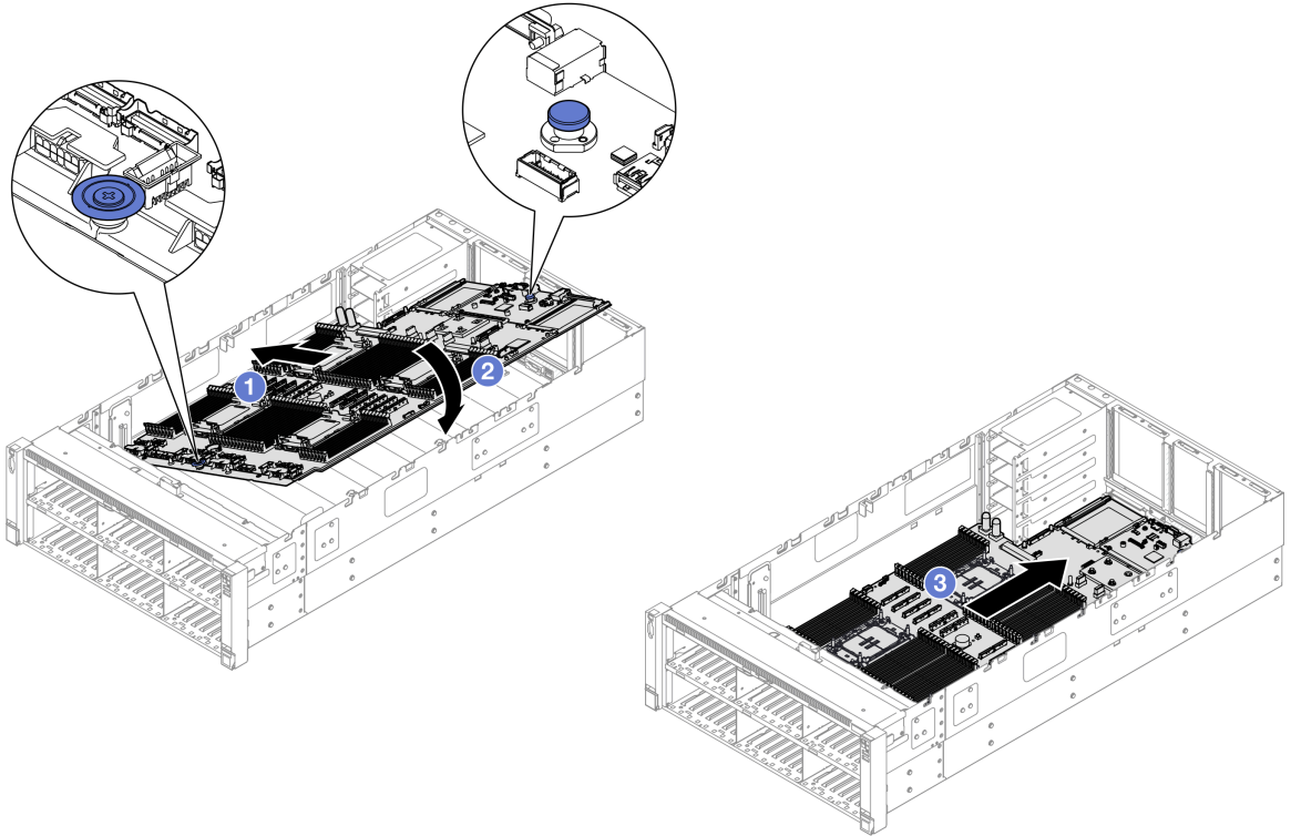
그림 216. 시스템 보드 어셈블리 설치
