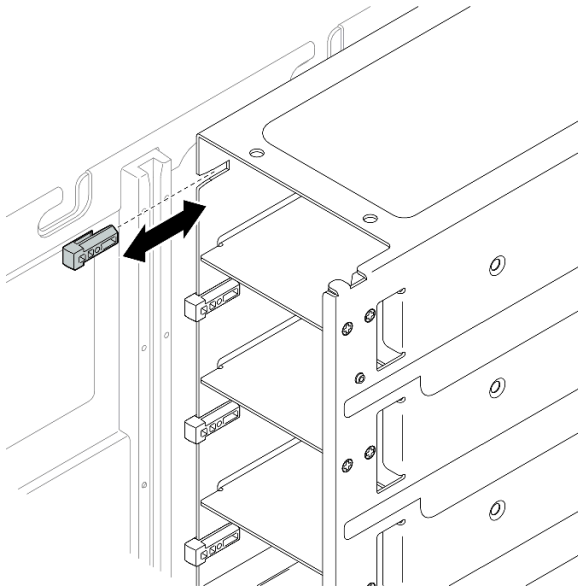
그림 189. 전원 공급 장치 키 설치
