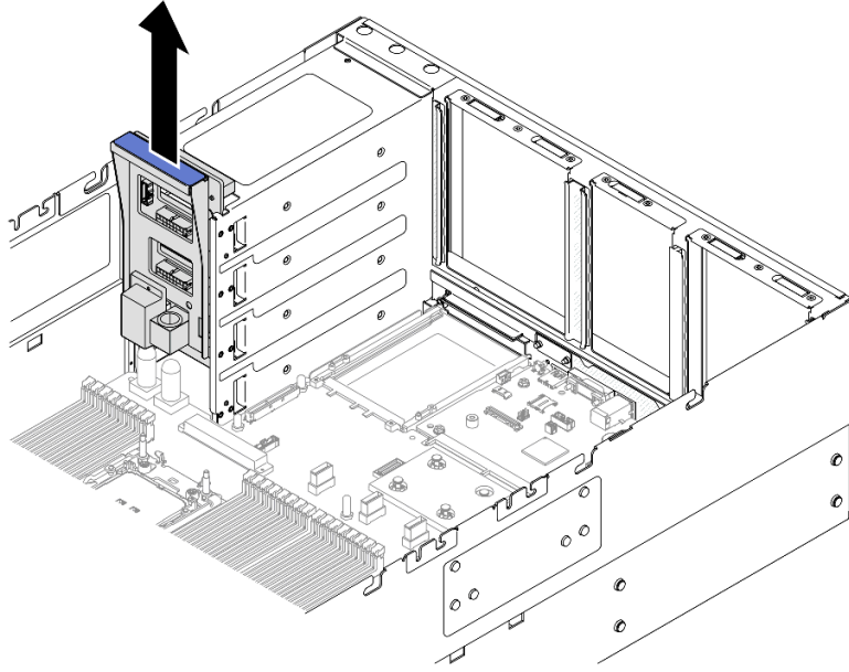
그림 179. 전원 분배 보드 제거
