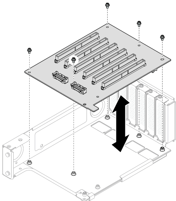
그림 152. 라이저에서 PCIe 라이저 카드 제거
