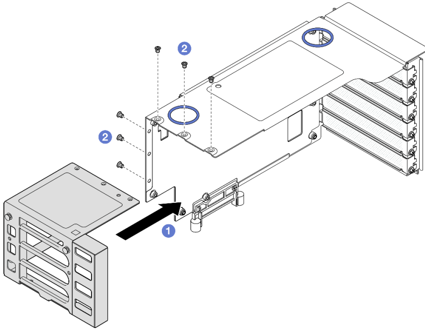
그림 175. FH PCIe 라이저에 PCIe 라이저 확장기 설치
