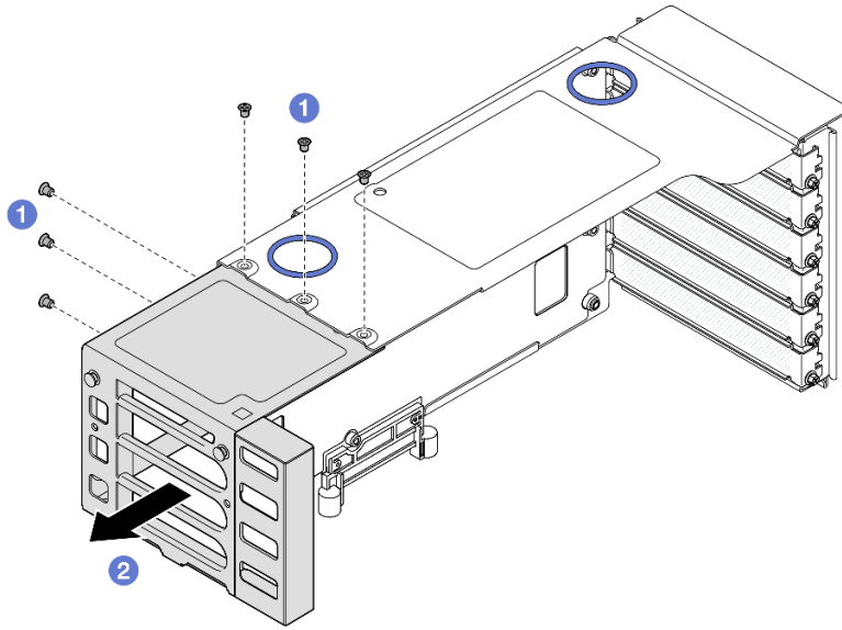
그림 172. FH PCIe 라이저에서 PCIe 라이저 확장기 제거
