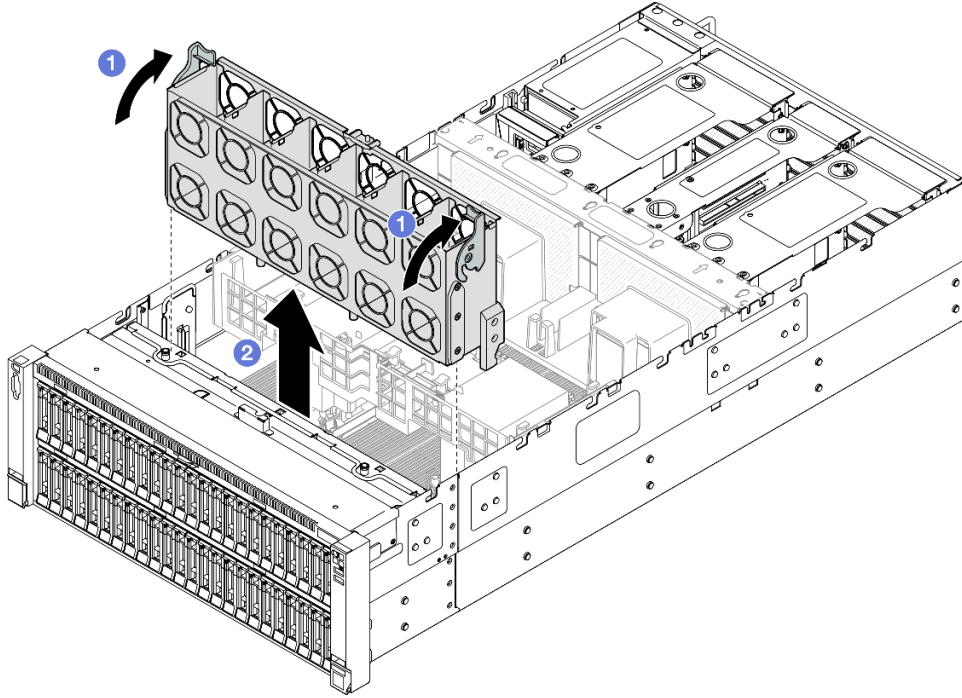
그림 81. 팬 케이지 제거
