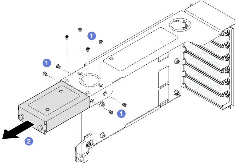
그림 173. HH PCIe 라이저에서 PCIe 라이저 확장기 제거
