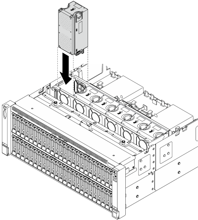
그림 83. 팬 모듈 설치
