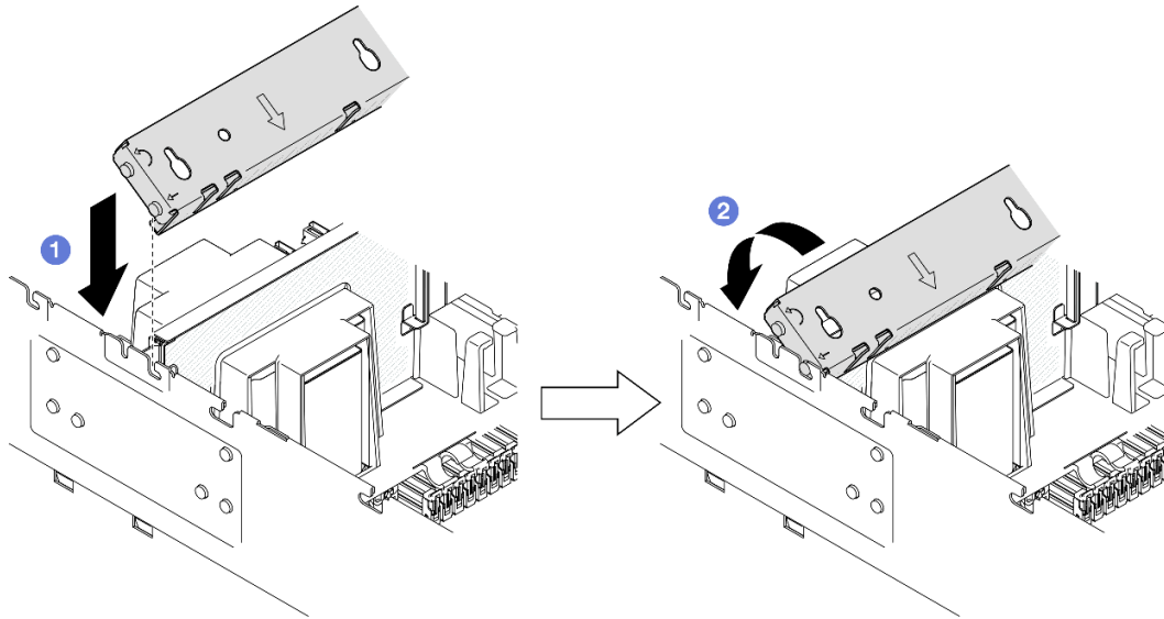
그림 69. 크로스바 설치
