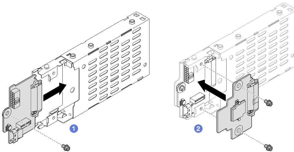
그림 28. 7mm 드라이브 백플레인 설치
