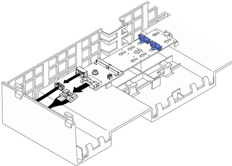
그림 39. SATA/x4 NVMe M.2 부트 어댑터에서 케이블 분리
