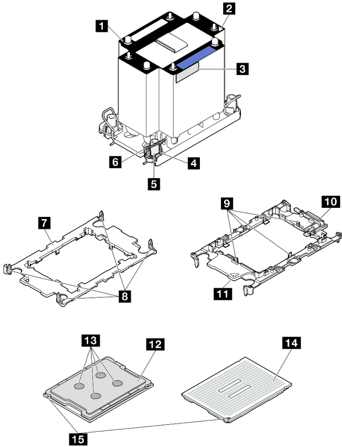
그림 193. PHM 구성 요소
