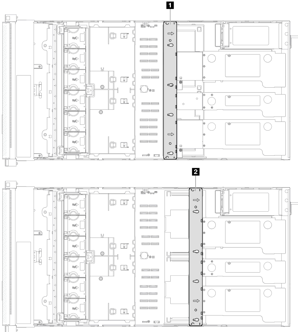
그림 65. 크로스바 위치
