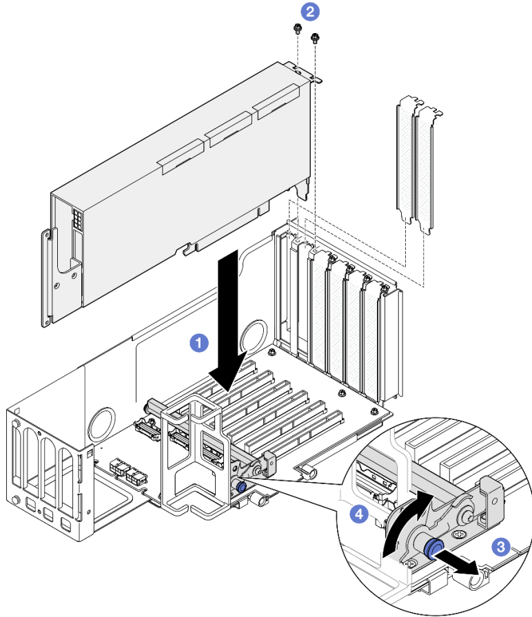
그림 95. PCIe 라이저에 GPU 어댑터 설치
