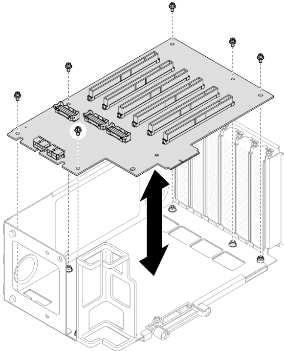
그림 158. 라이저에 PCIe 라이저 카드 설치
