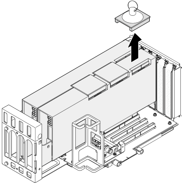
그림 88. GPU 어댑터 링크 브리지 제거
