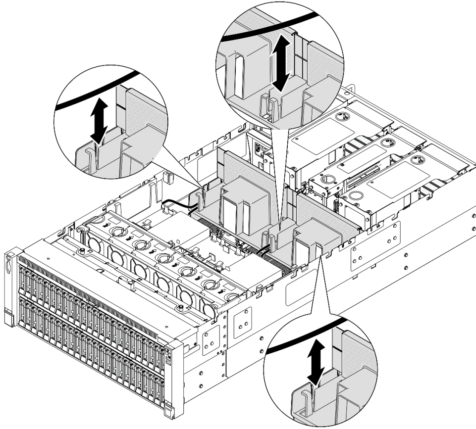
그림 51. 뒷면 공기 조절 장치에서 케이블 들어 올리기
