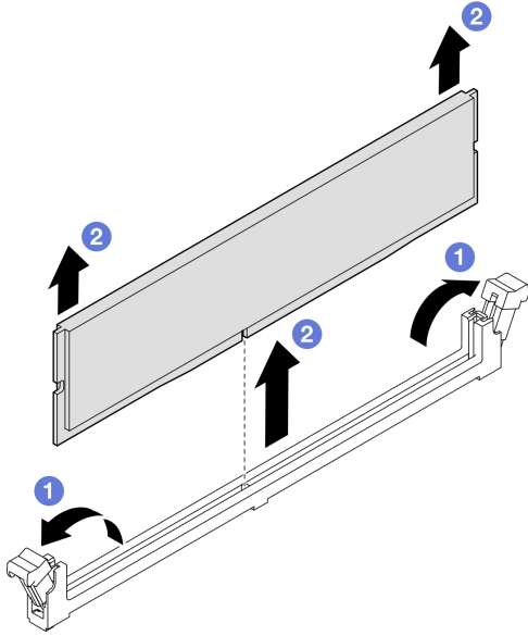
그림 116. 메모리 모듈 제거
