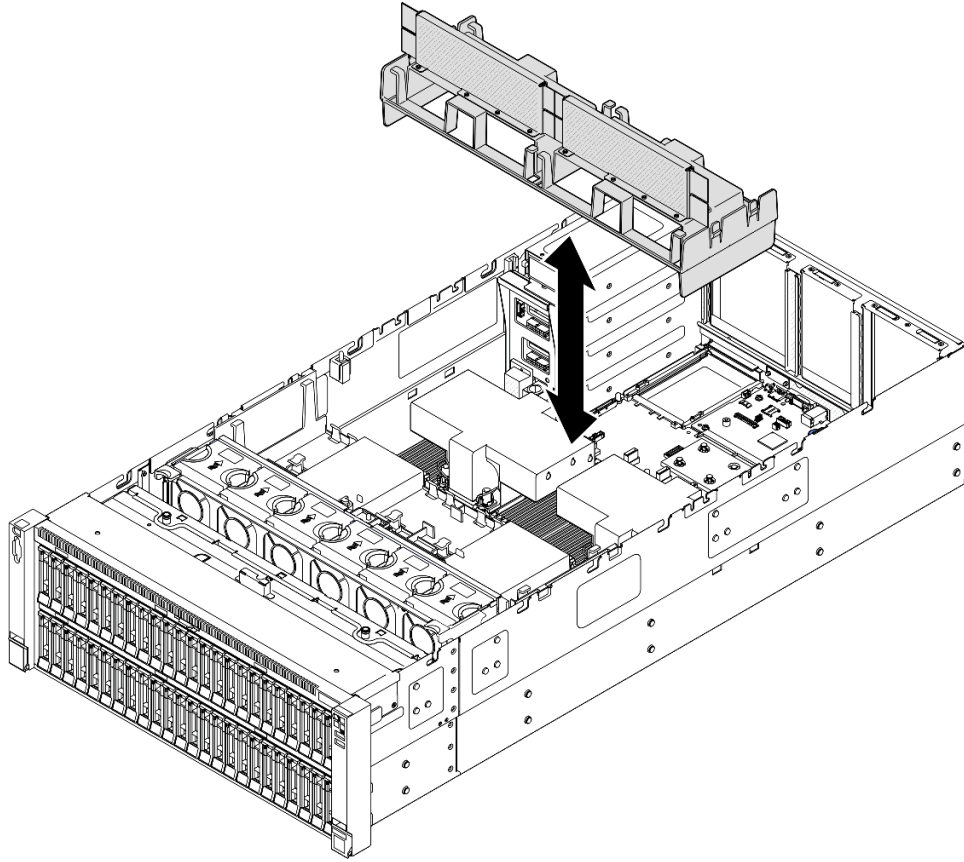
그림 55. 2U 성능 PHM용 뒷면 공기 조절 장치 설치
