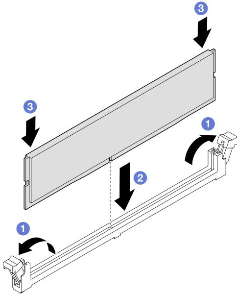
그림 117. 메모리 모듈 설치
