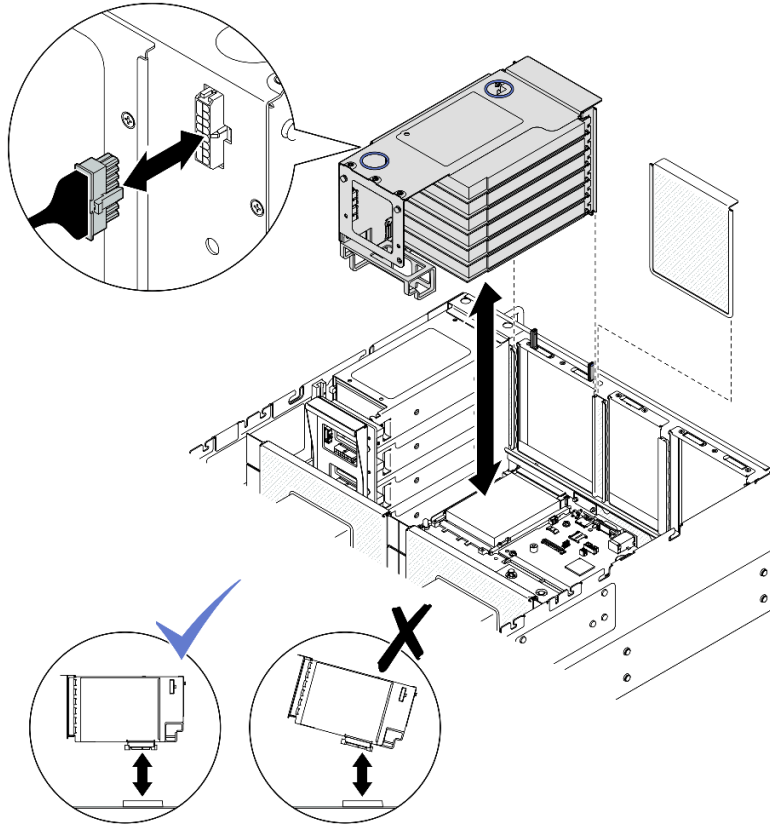
그림 127. PCIe 라이저 3 제거
