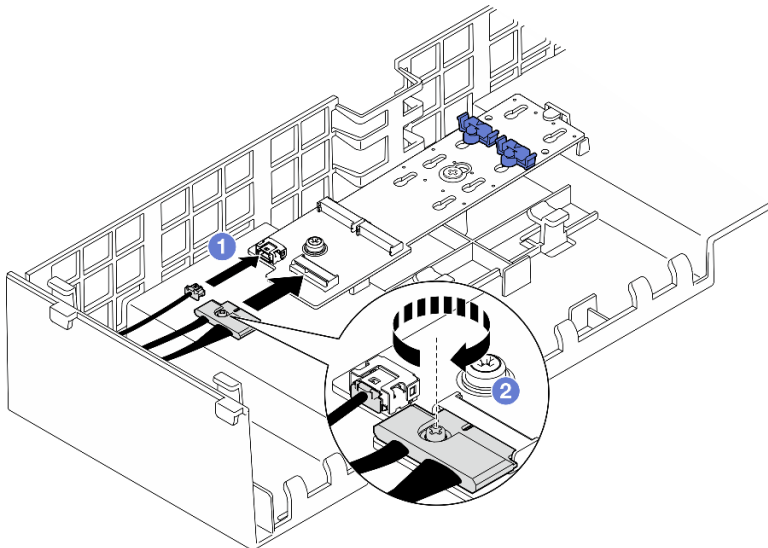
그림 109. SATA/NVMe 또는 NVMe M.2 부트 어댑터에 케이블 연결
