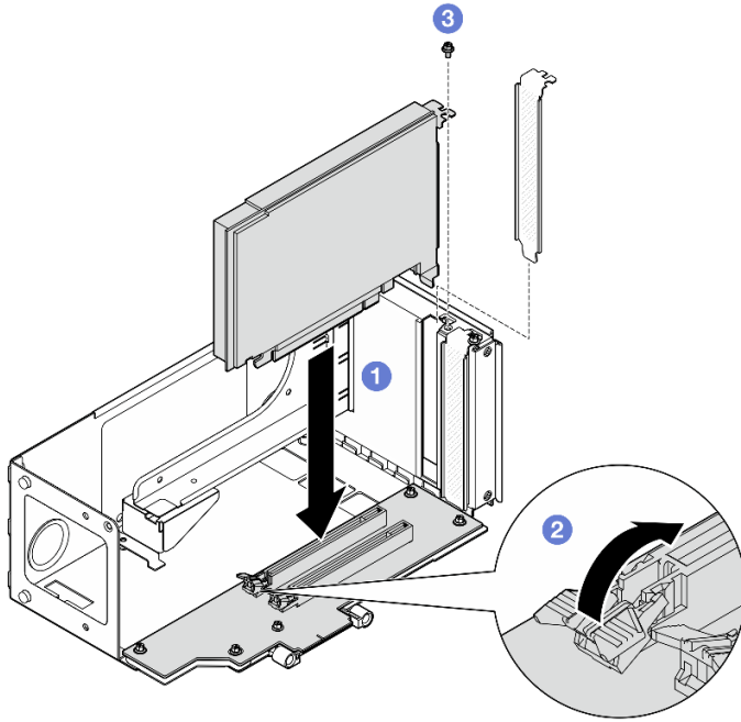
그림 131. 라이저에 PCIe 어댑터 설치
