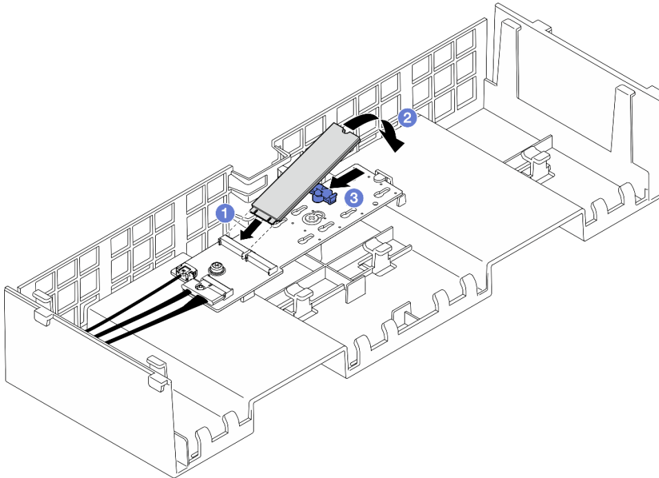
그림 113. M.2 드라이브 설치
