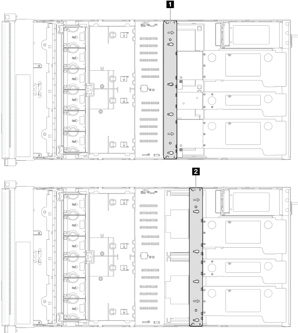
그림 68. 크로스바 위치
