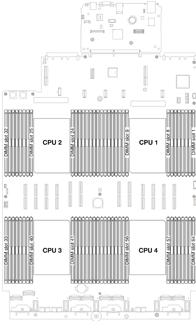
그림 17. 메모리 모듈 및 프로세서 레이아웃
