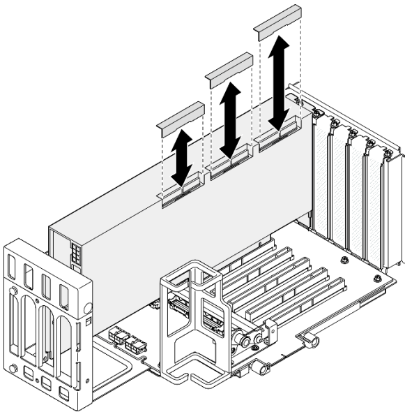
그림 89. GPU에 링크 커넥터 덮개 설치
