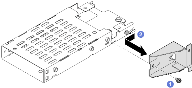
그림 21. 7mm 드라이브 케이스 브래킷 제거
