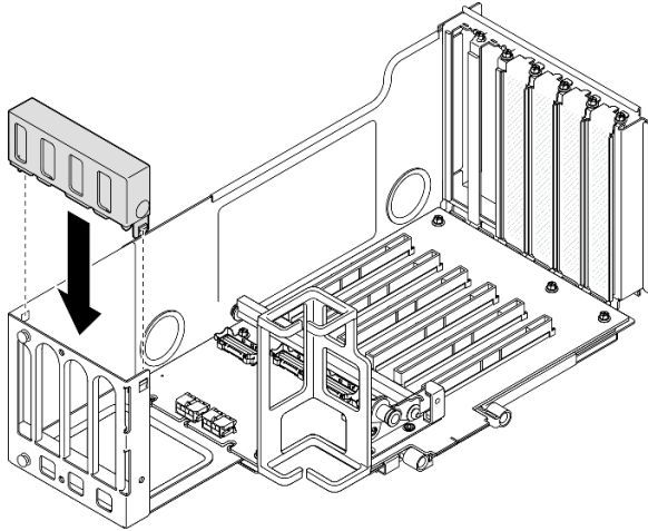
그림 93. 라이저 확장기 덮개 설치
