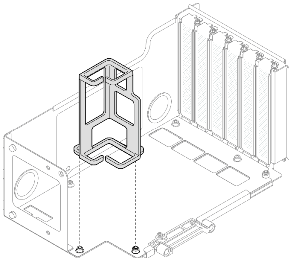
그림 157. 라이저에 케이블 고정장치 설치
