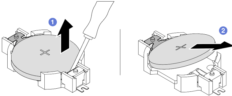
그림 62. CMOS 배터리 제거
