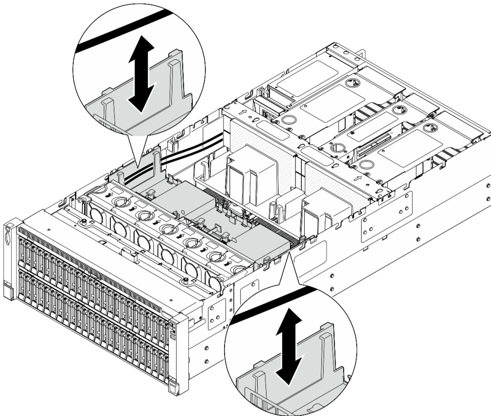
그림 41. 앞면 공기 조절 장치에서 케이블 들어 올리기
