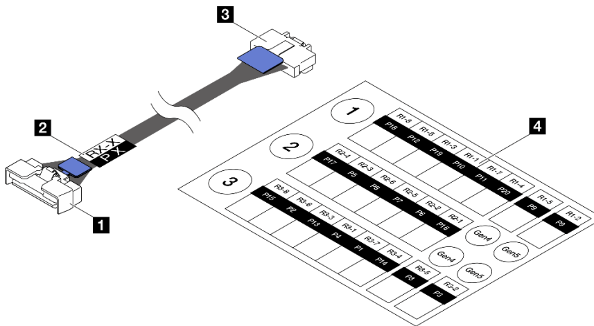
그림 155. PCIe 라이저 케이블
