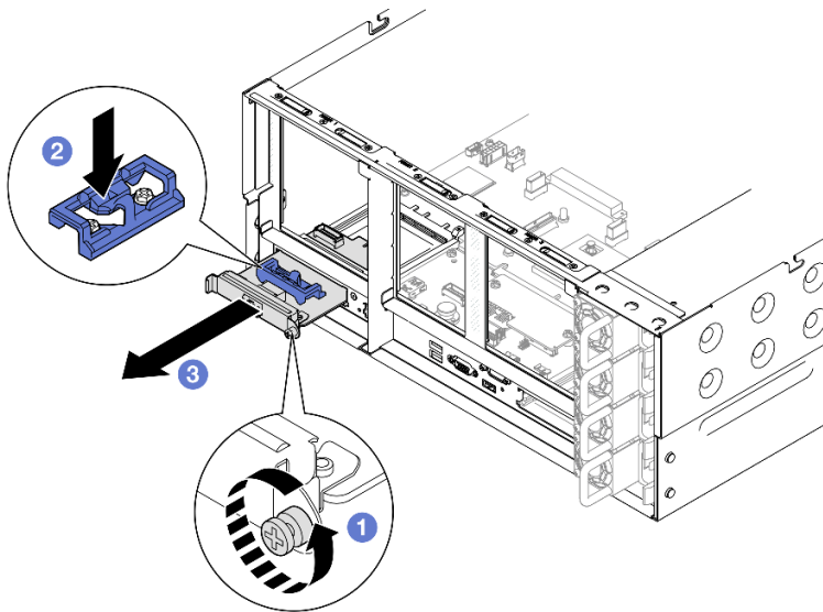
그림 114. 관리 NIC 어댑터 제거
