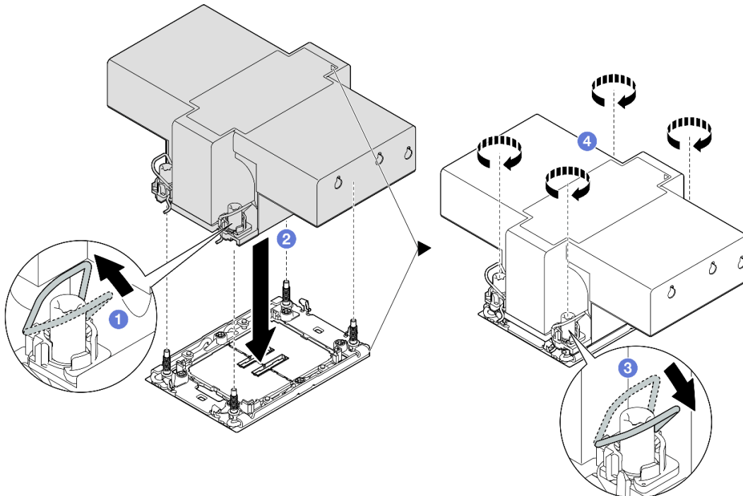
그림 203. 2U 성능 PHM 설치
