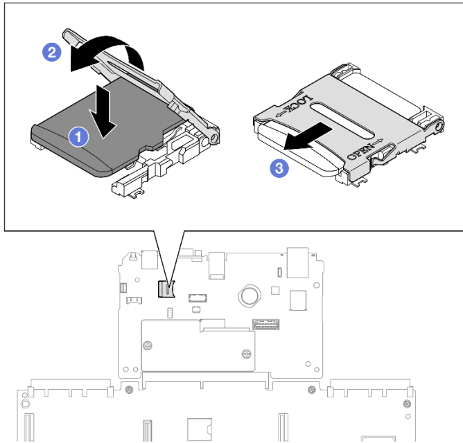
그림 119. MicroSD 카드 설치
