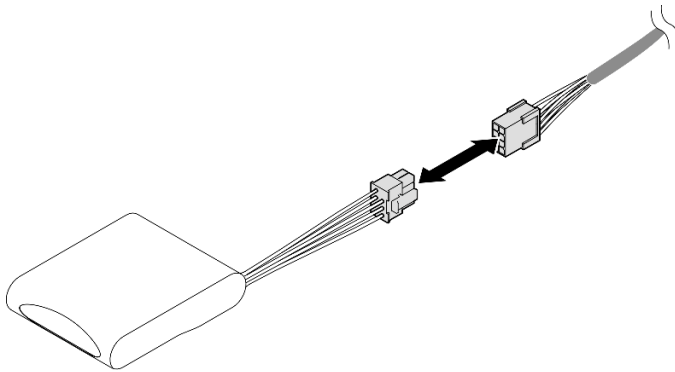
그림 84. 플래시 전원 모듈에서 케이블 분리
