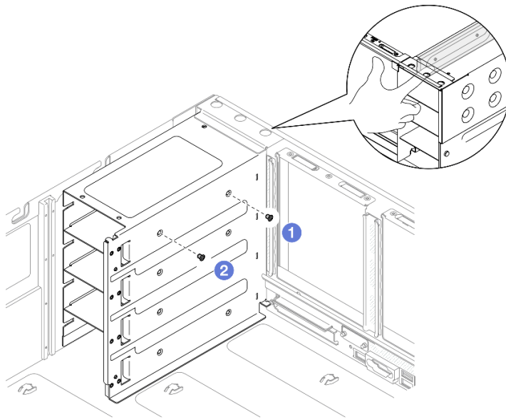
그림 186. 전원 공급 장치 브래킷 고정
