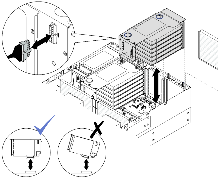
그림 137. PCIe 라이저 1 설치
