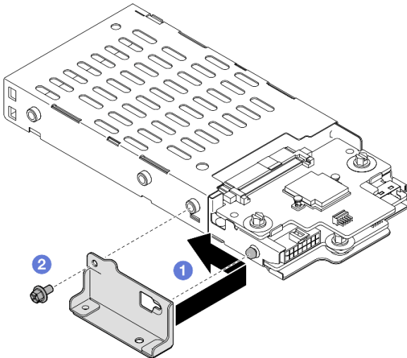
그림 34. 7mm 드라이브 케이지 브래킷 설치
