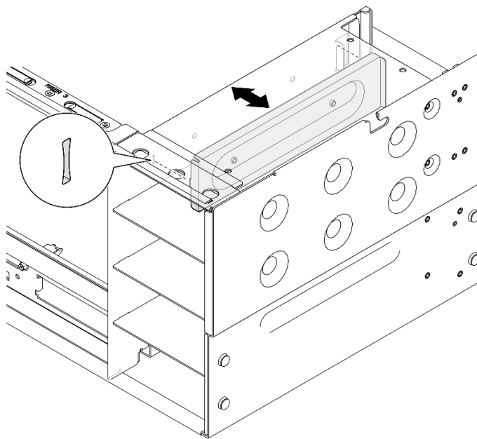
그림 184. 전원 공급 장치 브래킷 제거
