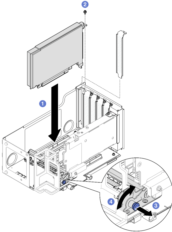
그림 132. 라이저에 PCIe 어댑터 설치
