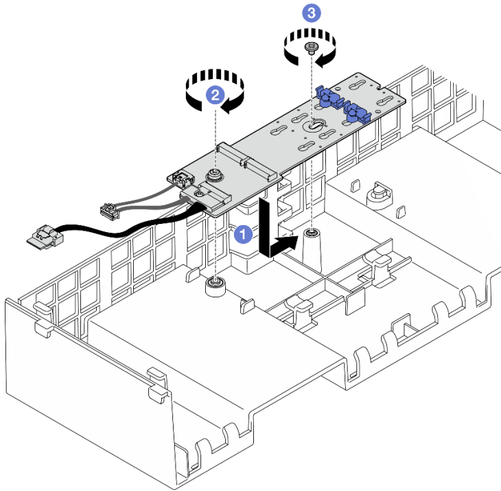
그림 110. M.2 부트 어댑터 설치
