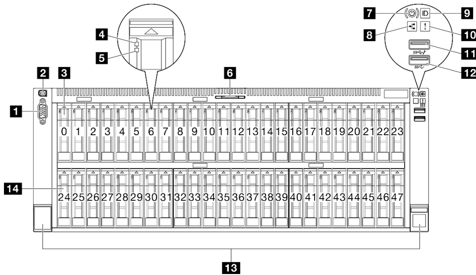
그림 2. 2.5인치 드라이브 구성의 앞면 보기
