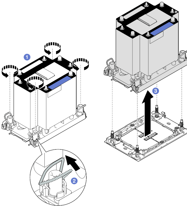
그림 194. 3U 표준 PHM 제거
