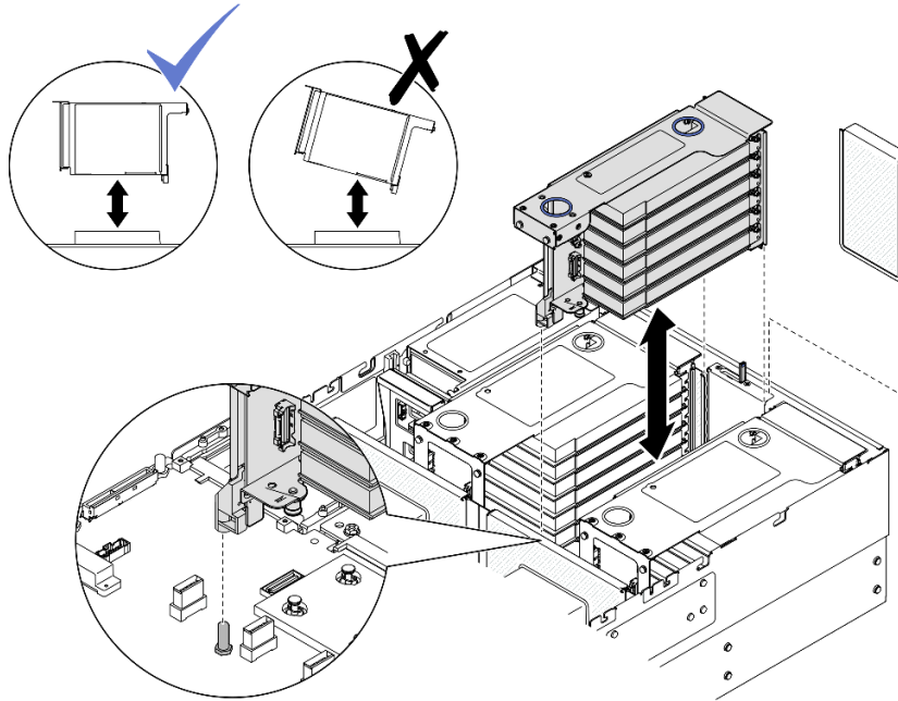
그림 122. PCIe 라이저 2 제거
