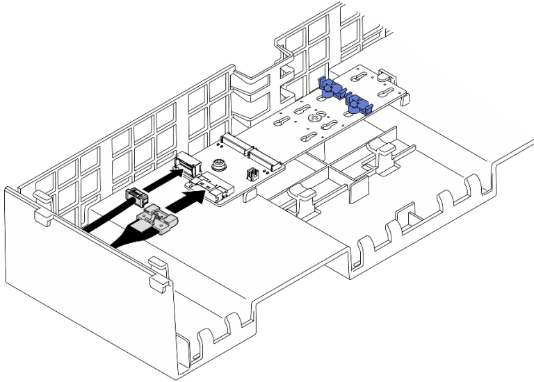
그림 108. SATA/x4 NVMe M.2 부트 어댑터에 케이블 연결
