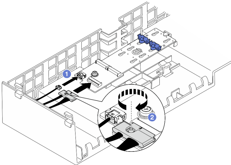
그림 58. SATA/NVMe 또는 NVMe M.2 부트 어댑터에 케이블 연결
