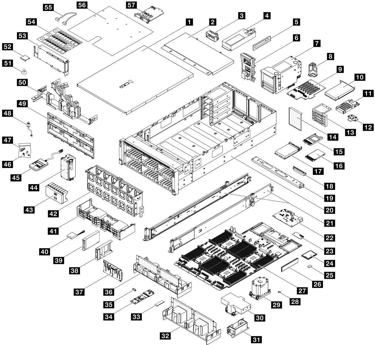
그림 13. 서버 구성 요소
