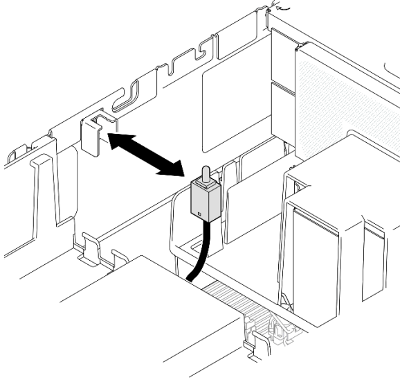
그림 101. 침입 스위치 제거
