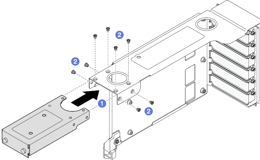
그림 177. FH PCIe 라이저에 PCIe 라이저 확장기 설치
