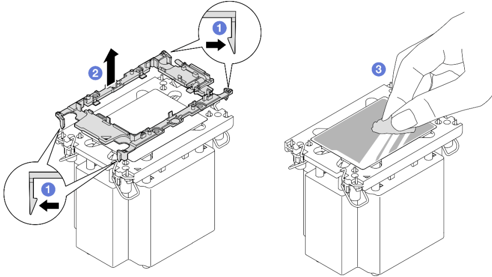
그림 197. 방열판에서 프로세서 캐리어 분리 중
