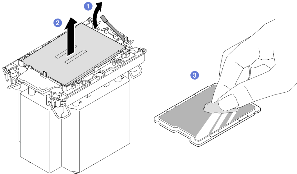
그림 196. 방열판 및 캐리어에서 프로세서 분리 중
