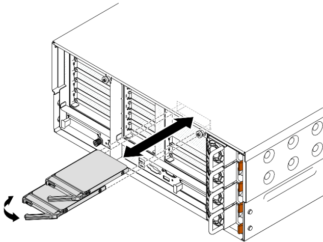
그림 19. 7mm 드라이브 제거
