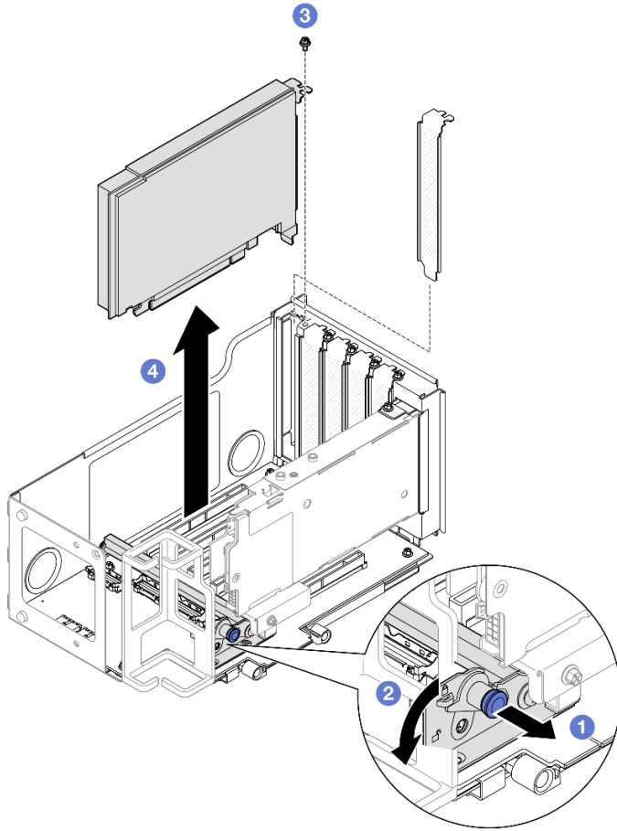
그림 129. 라이저에서 PCIe 어댑터 제거
