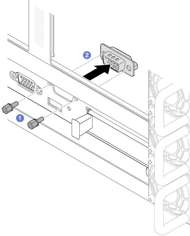
그림 205. 직렬 포트 모듈 제거
