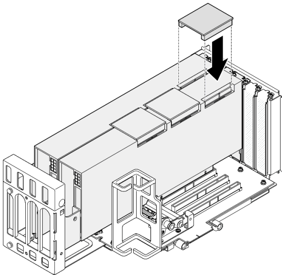
그림 99. GPU 어댑터 링크 브리지 설치
