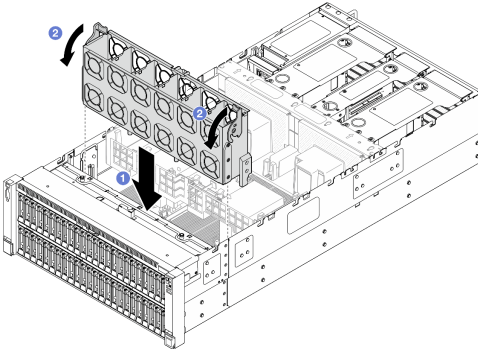
그림 82. 팬 케이스 설치
