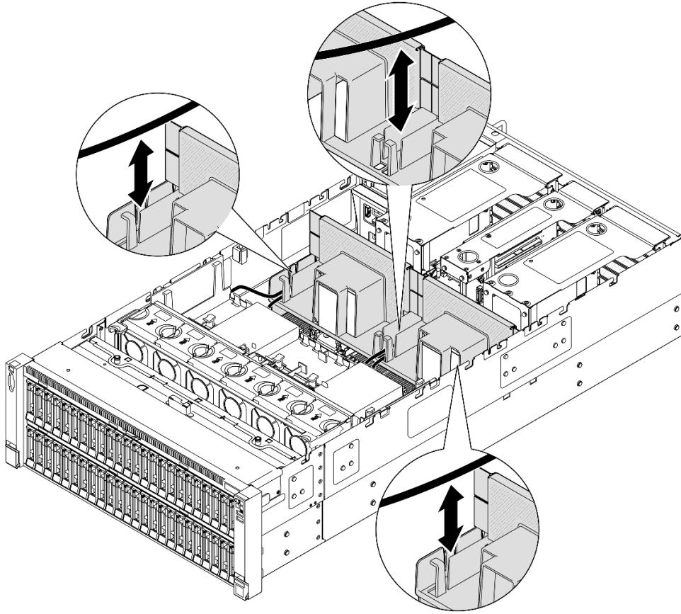
그림 56. 뒷면 공기 조절 장치를 통해 케이블 배선
