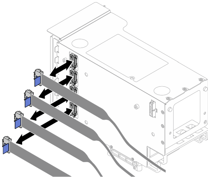
그림 162. 라이저 외부에 PCIe 라이저 케이블 연결
