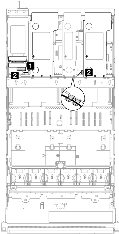
그림 235. 전원 분배 보드의 전원 케이블 배선
