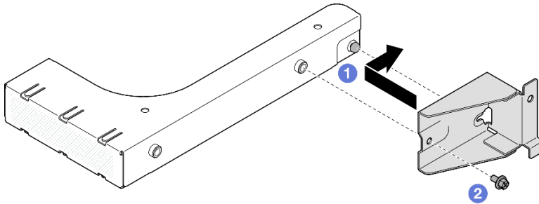
그림 23. 7mm 드라이브 케이지 브래킷 설치
