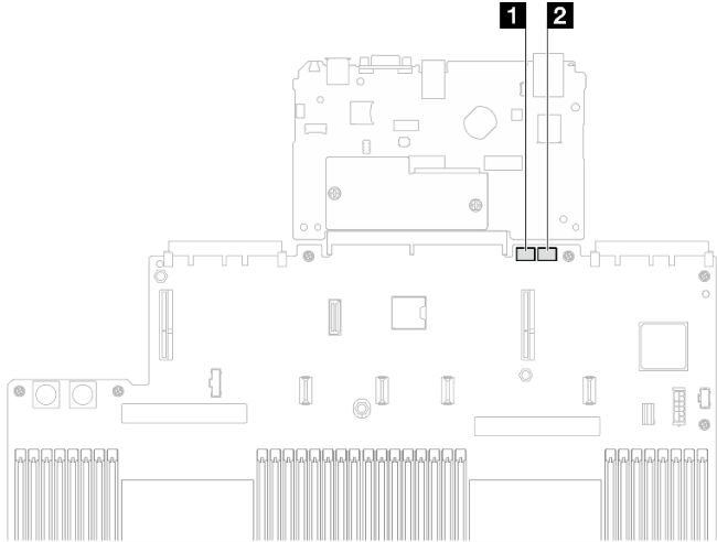
그림 12. 시스템 보드 어셈블리 스위치
