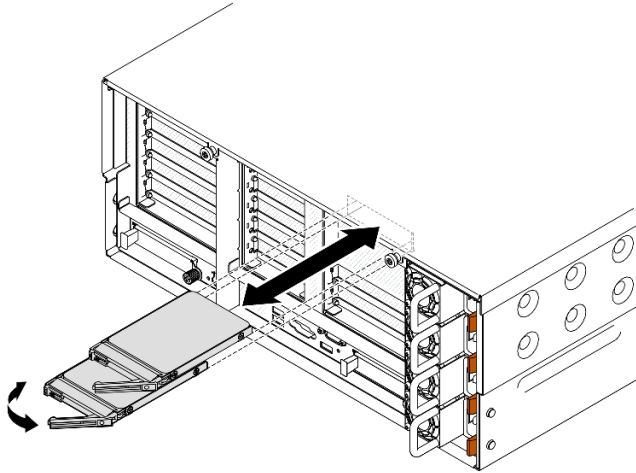
그림 37. 7mm 드라이브 설치
