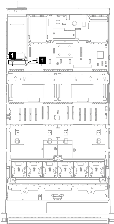
그림 236. 전원 분배 보드의 사이드밴드 케이블 배선
