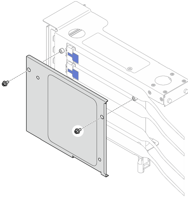
그림 148. 라이저에서 덮개 제거
