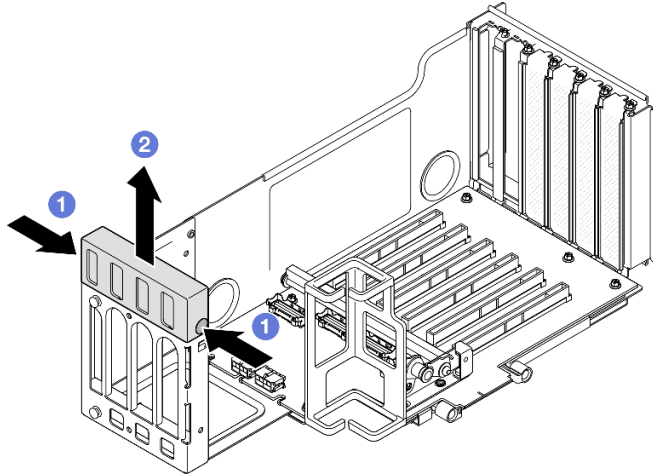
그림 94. 라이저 확장기 덮개 제거
