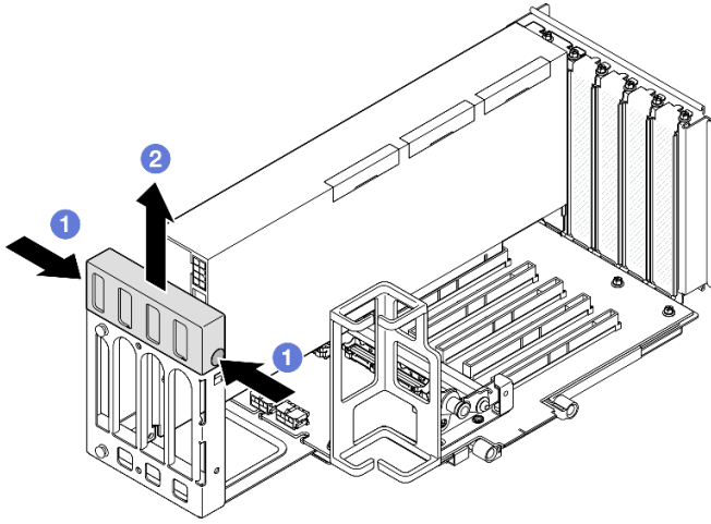
그림 90. 라이저 확장기 덮개 제거
