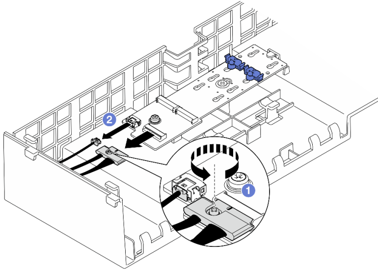
그림 107. SATA/NVMe 또는 NVMe M.2 부트 어댑터에서 케이블 분리
