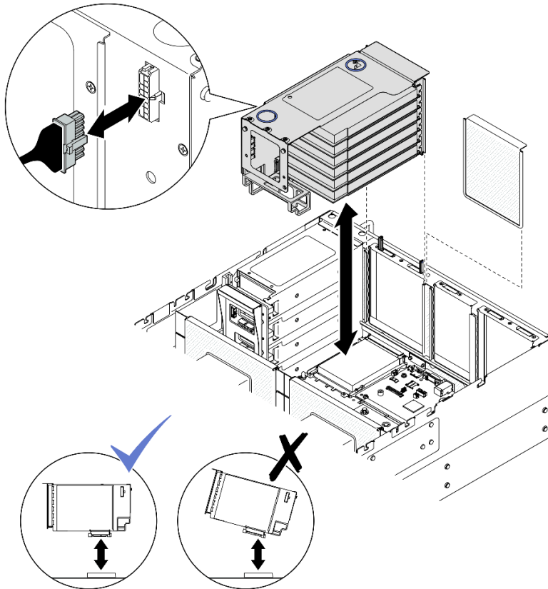
그림 134. PCIe 라이저 3 설치
