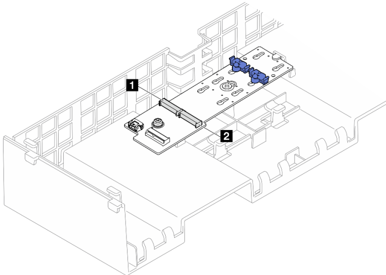
그림 112. M.2 드라이브 슬롯
