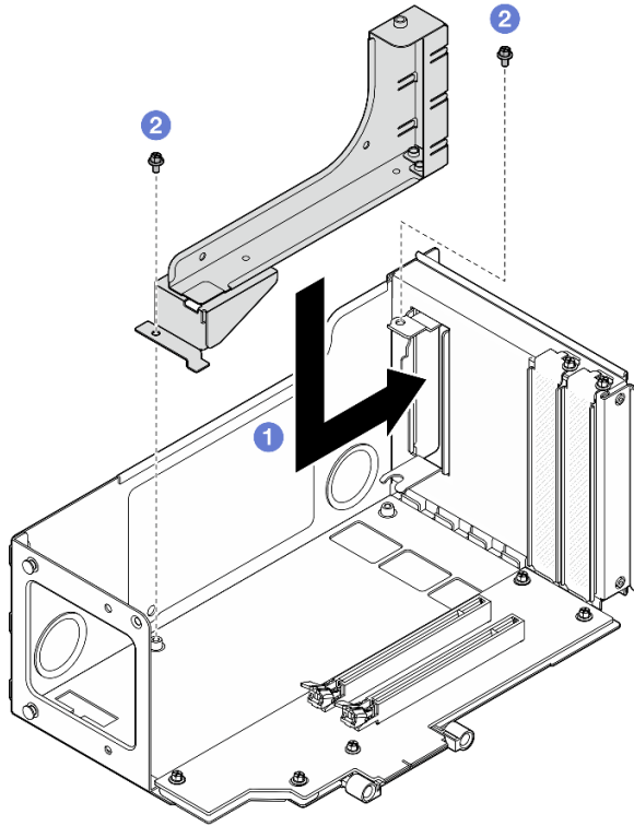
그림 24. 7mm 드라이브 케이스 필러 설치
