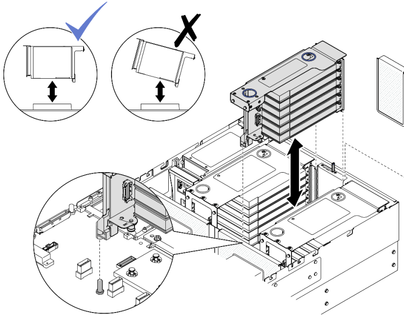
그림 125. PCIe 라이저 2 제거
