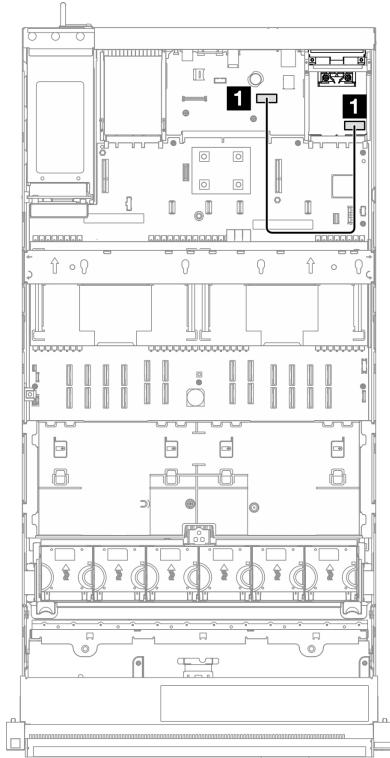
그림 234. 관리 NIC 어댑터의 케이블 배선
