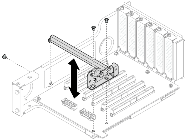
그림 151. 라이저에서 PCIe 고정장치 제거
