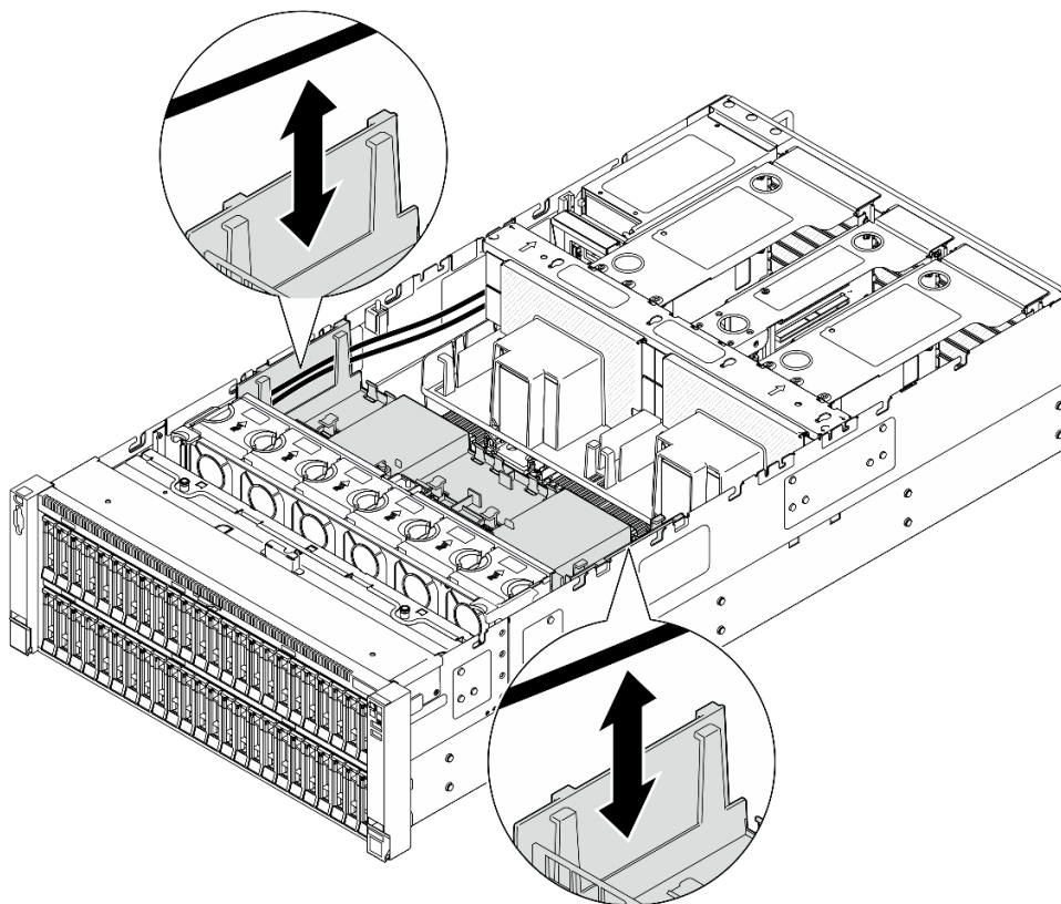
그림 44. 앞면 공기 조절 장치를 통해 케이블 배선
