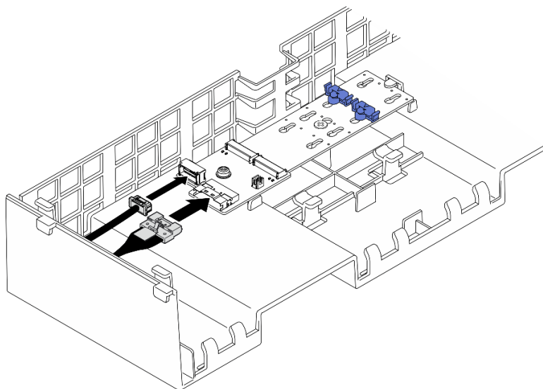
그림 45. SATA/x4 NVMe M.2 부트 어댑터에 케이블 연결
