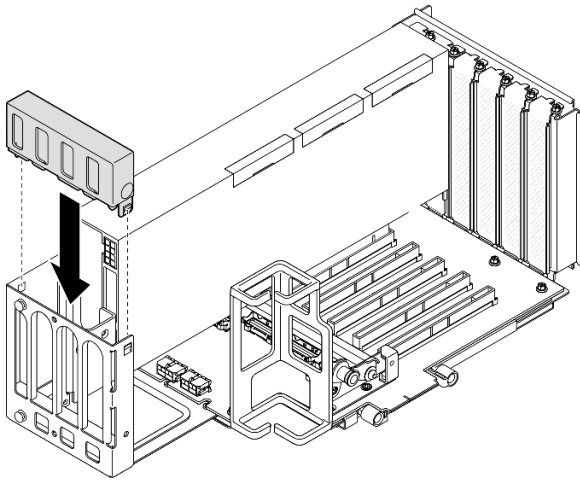
그림 97. 라이저 확장기 덮개 설치
