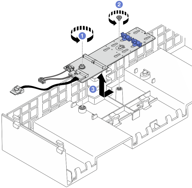
그림 105. M.2 부트 어댑터 제거
