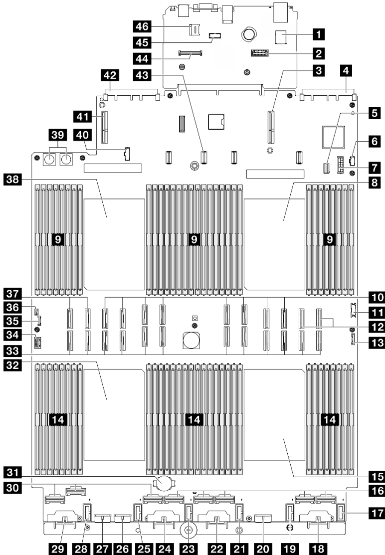
그림 11. 시스템 보드 어셈블리 커넥터
