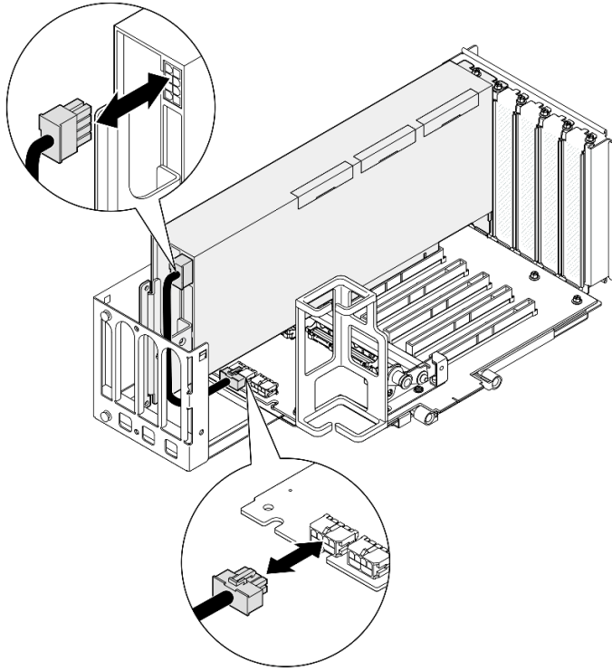
그림 96. GPU 어댑터에 전원 케이블 연결
