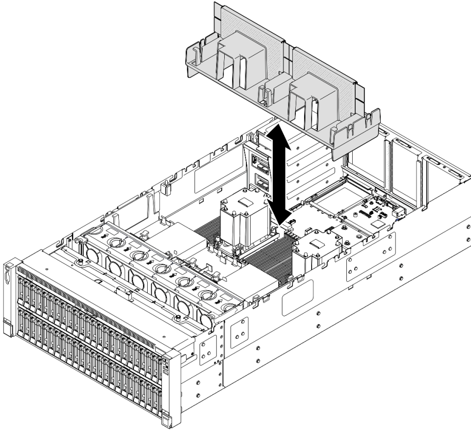
그림 54. 3U 표준 PHM용 뒷면 공기 조절 장치 설치
