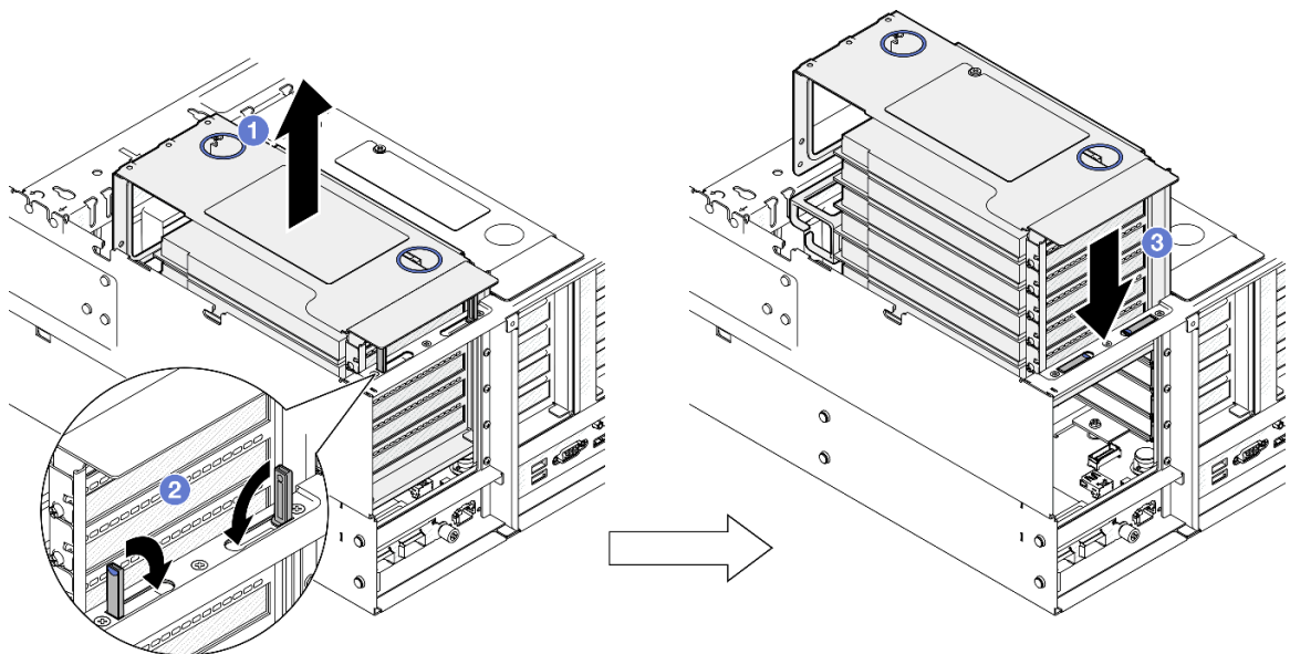
그림 70. PCIe 라이저 고정
