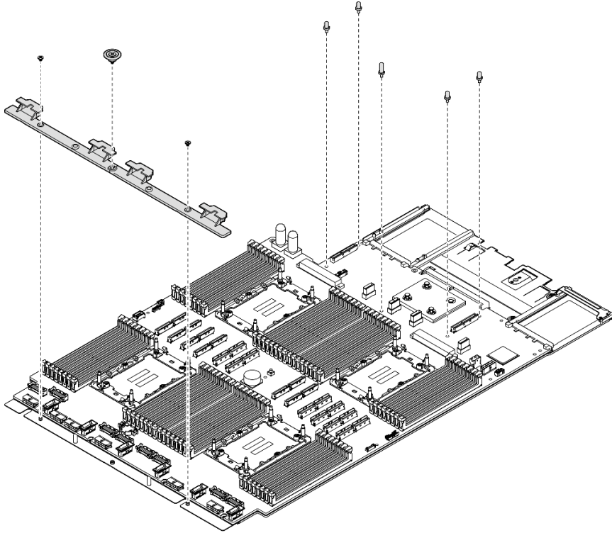
그림 248. 부품 제거
