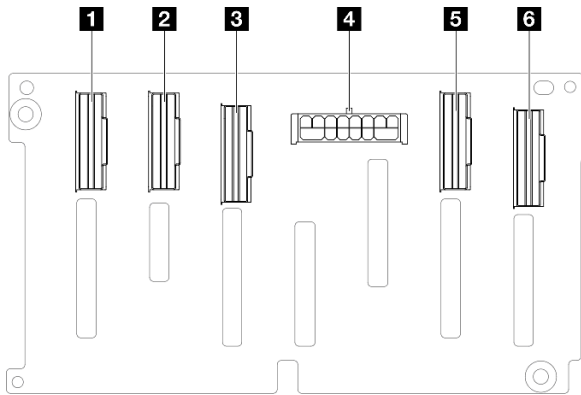
그림 223. 2.5인치 AnyBay 8베이 드라이브 백플레인 커넥터
