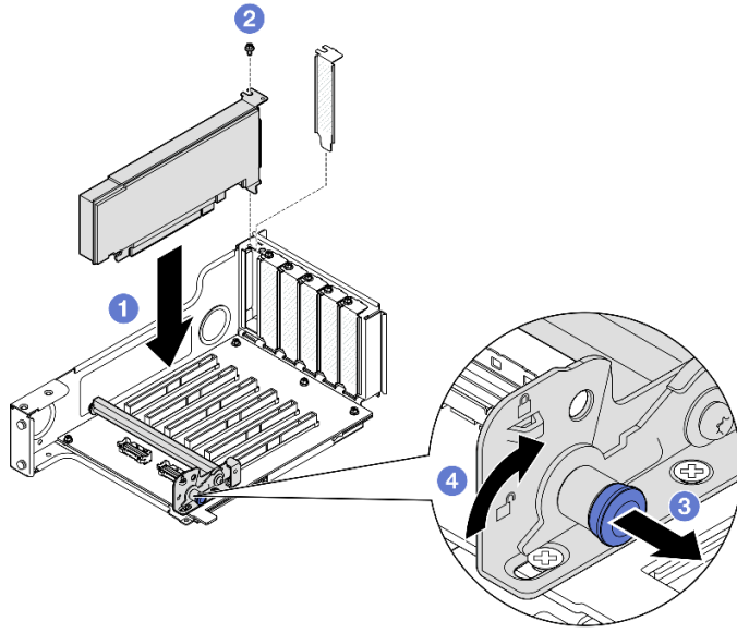
그림 133. 라이저에 PCIe 어댑터 설치
