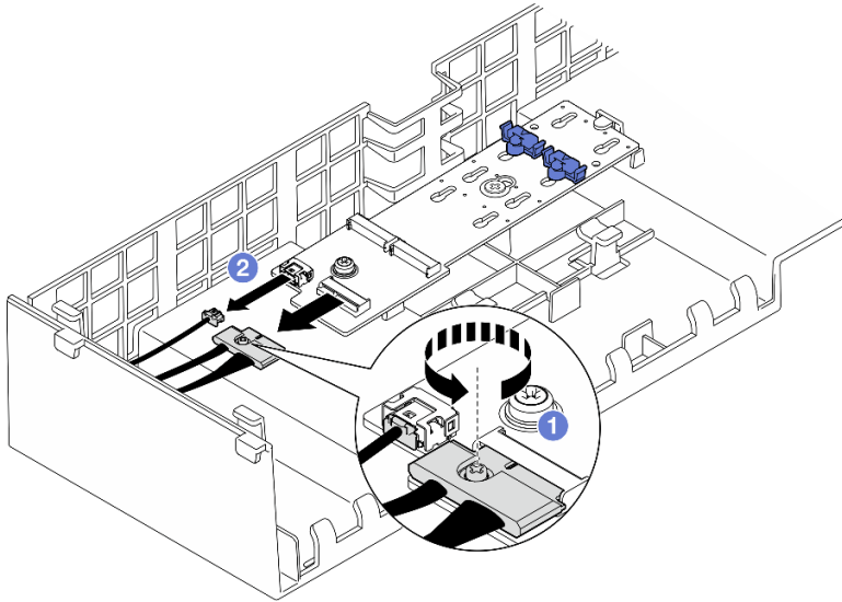
그림 50. SATA/NVMe 또는 NVMe M.2 부트 어댑터에서 케이블 분리
