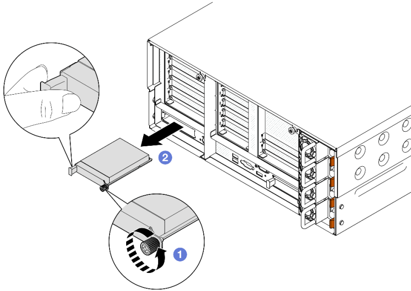
그림 120. OCP 모듈 제거
