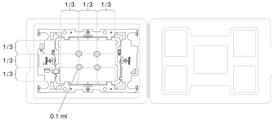
그림 200. 운송 트레이에 프로세서가 있는 열전도 그리스를 도포하십시오.
