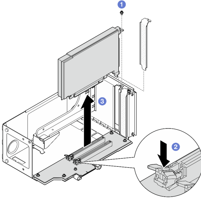
그림 128. 라이저에서 PCIe 어댑터 제거
