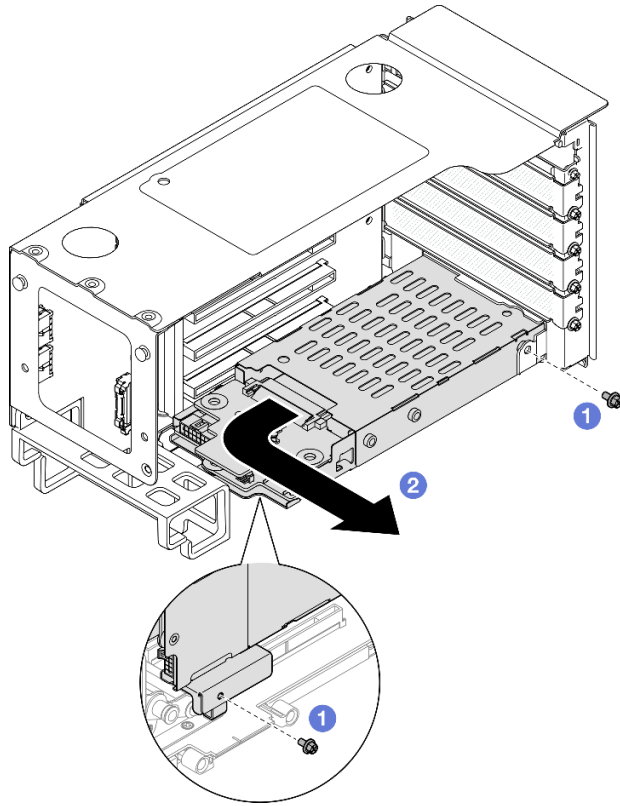
그림 25. 라이저에서 7mm 드라이브 케이지 제거
