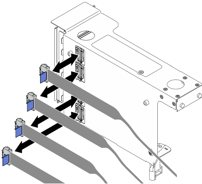
그림 170. 라이저 외부에 PCIe 라이저 케이블 연결
