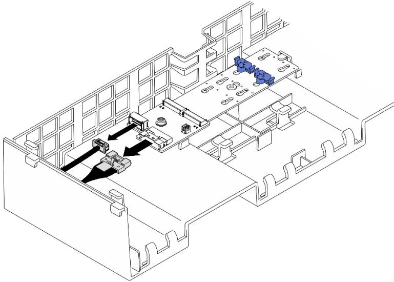
그림 49. SATA/x4 NVMe M.2 부트 어댑터에서 케이블 분리
