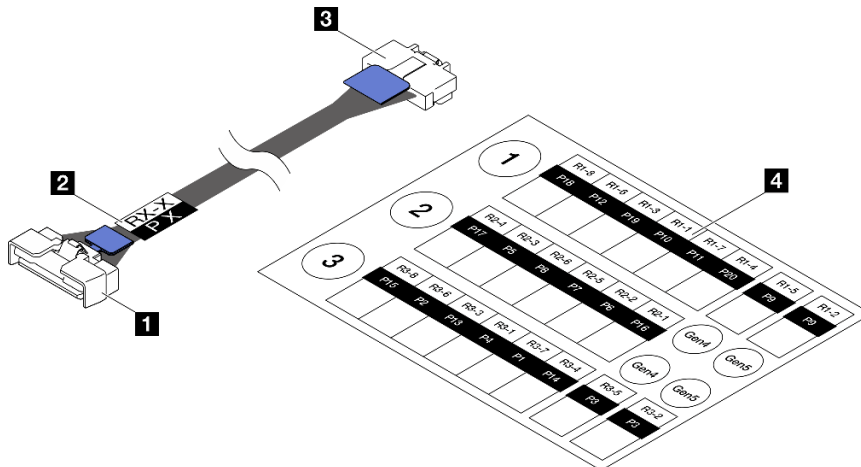
그림 164. PCIe 라이저 케이블
