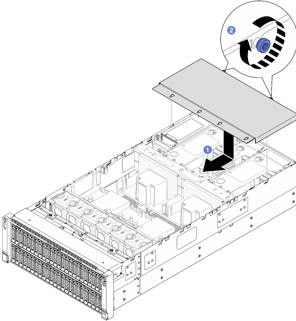
그림 220. 뒤쪽 윗면 덮개 설치
