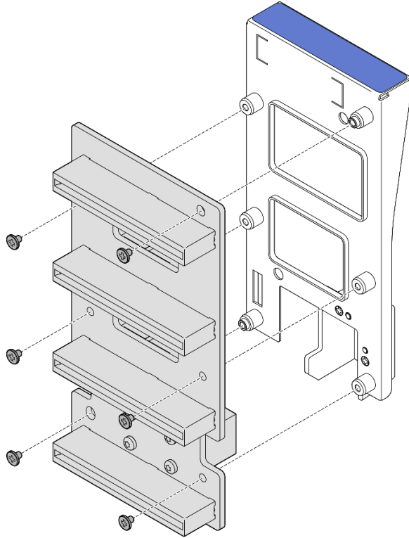
그림 180. 전원 분배 보드 분리
