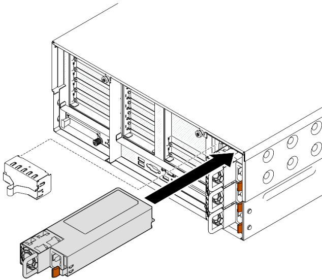
그림 192. 전원 공급 장치 설치
