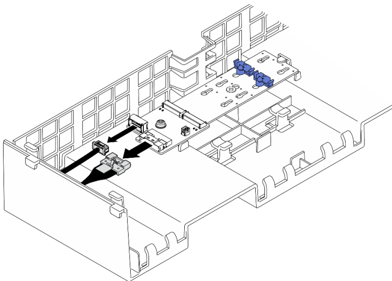
그림 106. SATA/x4 NVMe M.2 부트 어댑터에서 케이블 분리
