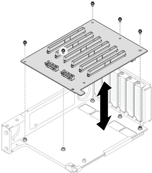
그림 166. 라이저에 PCIe 라이저 카드 설치
