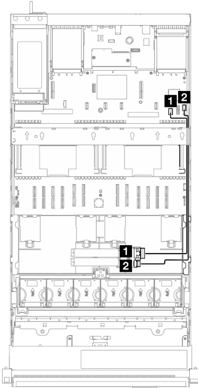
그림 232. PCH에 대한 SATA/x4 NVMe M.2 부트 어댑터의 케이블 배선
