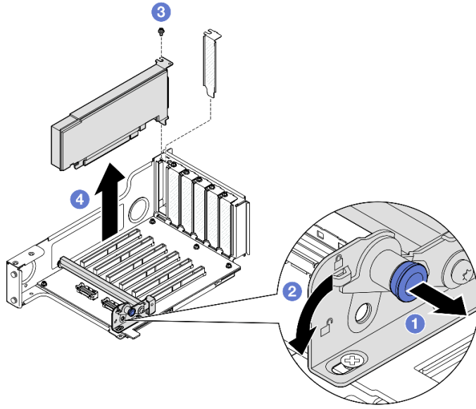
그림 130. 라이저에서 PCIe 어댑터 제거
