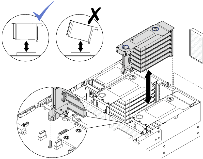
그림 139. PCIe 라이저 2 설치
