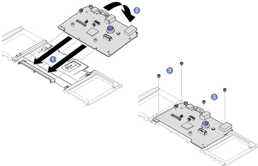
그림 215. 프로세서 보드에 시스템 I/O 보드 설치
