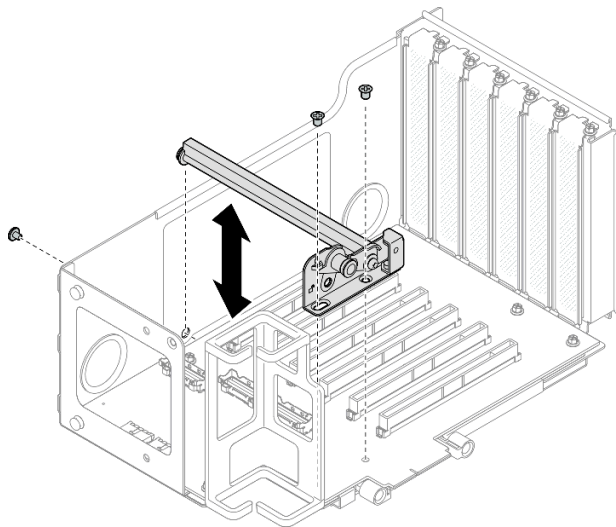
그림 145. 라이저에서 PCIe 고정장치 제거
