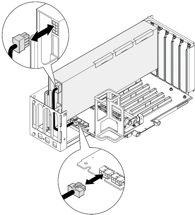
그림 91. GPU 어댑터에서 전원 케이블 분리
