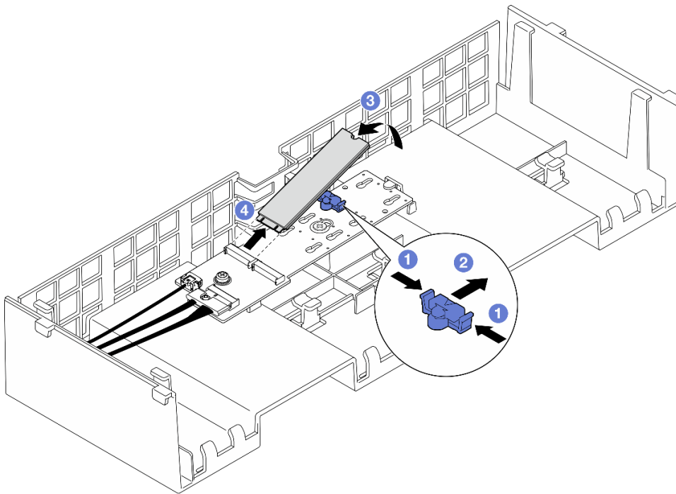
그림 104. M.2 드라이브 제거
