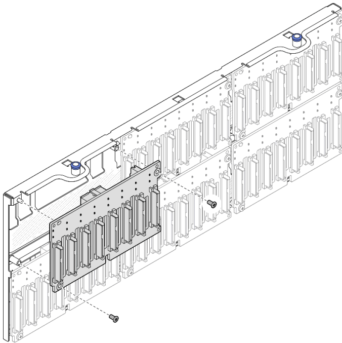
그림 74. 캐리어에서 백플레인 제거
