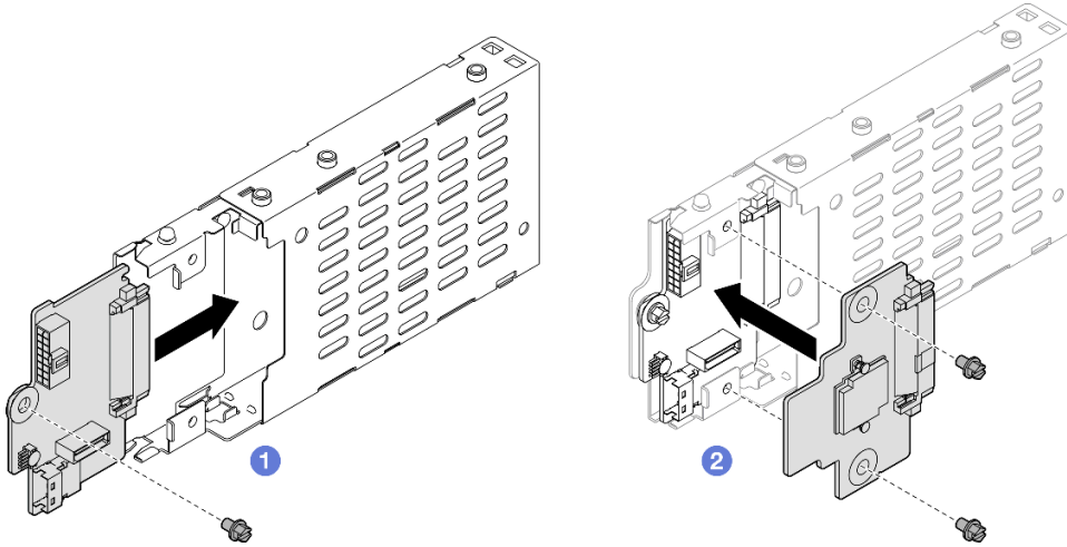
그림 33. 7mm 드라이브 백플레인 설치
