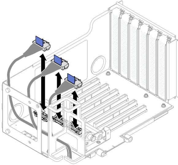
그림 160. 라이저 내부에 PCIe 라이저 케이블 연결
