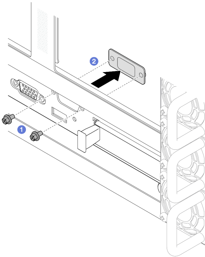
그림 207. 직렬 포트 필터 제거
