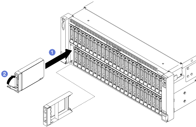
그림 72. 2.5인치 드라이브 설치
