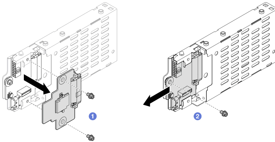
그림 27. 7mm 드라이브 케이스 분해
