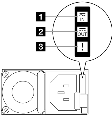
그림 242. 전원 공급 장치 LED
