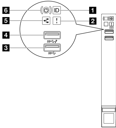
그림 9. 앞면 I/O 모듈
