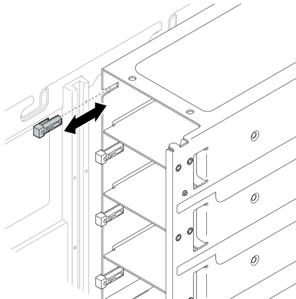
그림 188. 전원 공급 장치 키 제거
