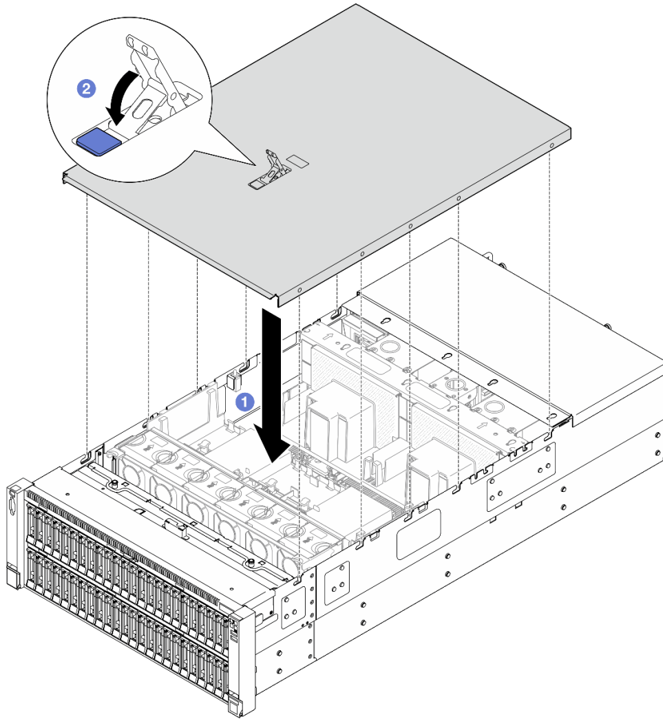
그림 221. 앞쪽 윗면 덮개 설치
