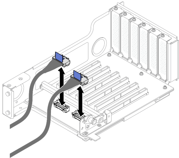
그림 168. 라이저 내부에 PCIe 라이저 케이블 연결
