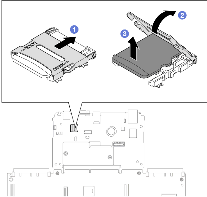
그림 118. MicroSD 카드 제거
