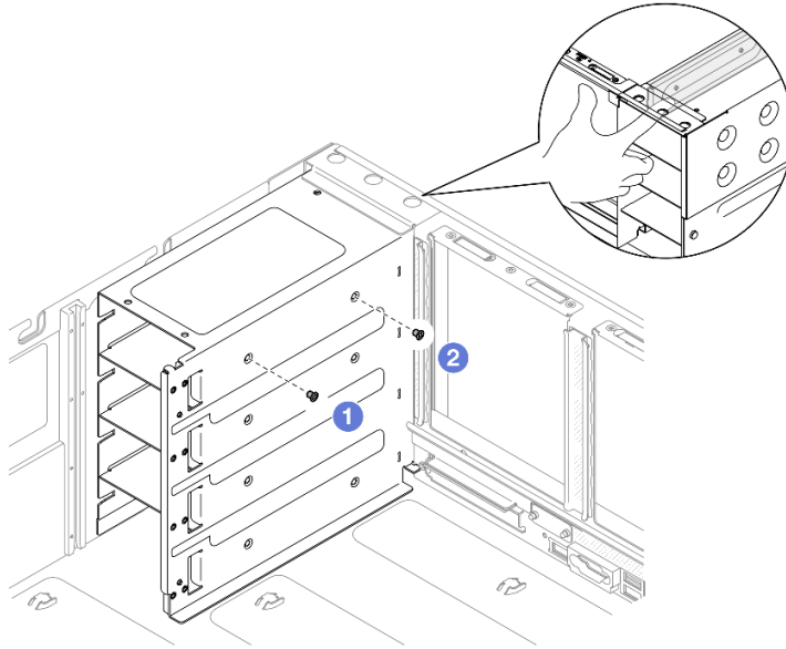
그림 183. 전원 공급 장치 브래킷 나사 제거
