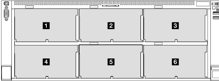
그림 76. 드라이브 백플레인 넘버링
