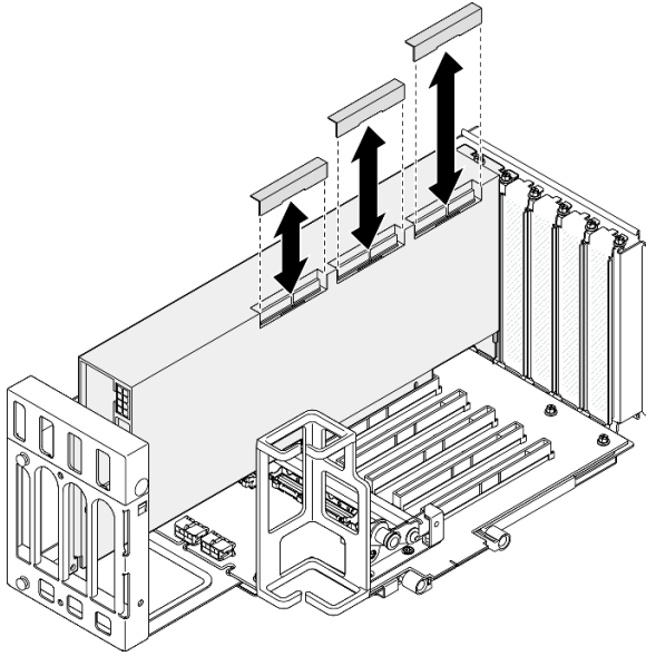
그림 98. GPU에서 링크 커넥터 덮개 제거
