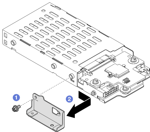
그림 26. 7mm 드라이브 케이지 브래킷 제거
