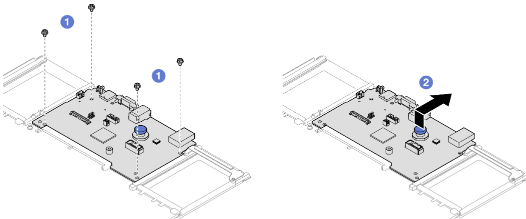
그림 247. 프로세서 보드에서 시스템 I/O 보드 분리
