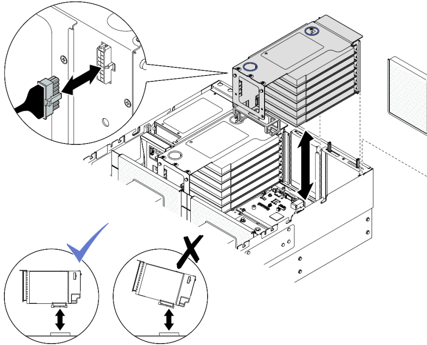
그림 126. PCIe 라이저 1 제거
