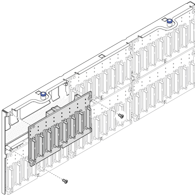
그림 78. 캐리어에 백플레인 설치
