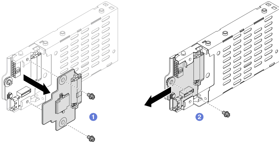
그림 22. 7mm 드라이브 케이지 분해
