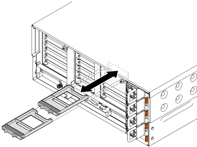
그림 36. 7mm 드라이버 필터 제거
