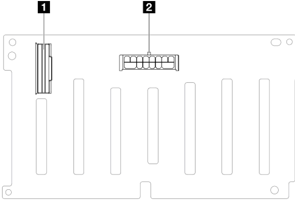
그림 224. 2.5인치 SAS/SATA 8베이 드라이브 백플레인 커넥터
