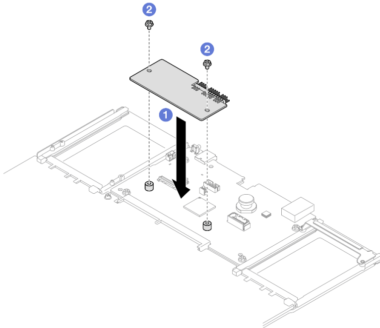
그림 212. 펌웨어 및 RoT 보안 모듈 설치
