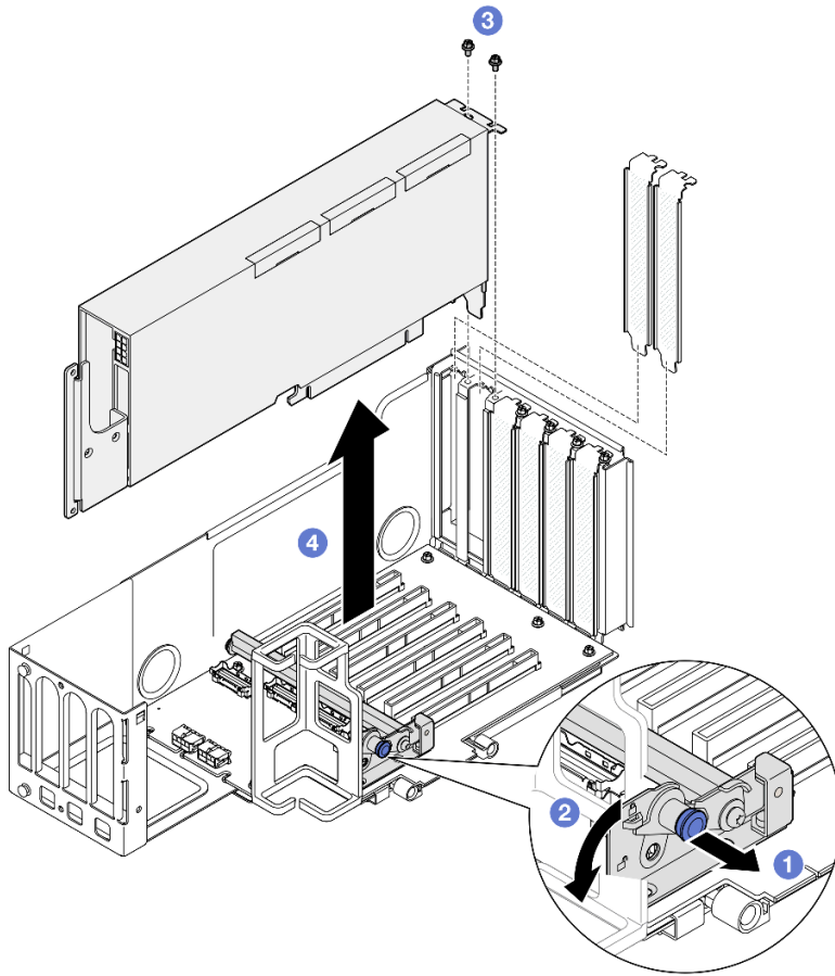
그림 92. PCIe 라이저에서 GPU 어댑터 제거
