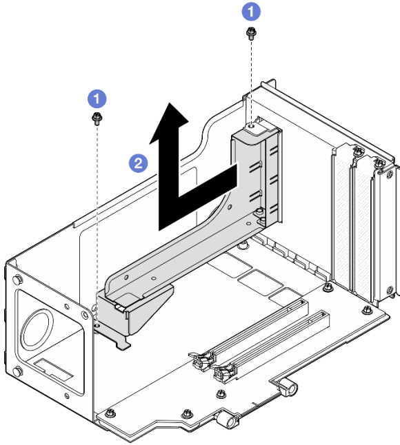
그림 29. 7mm 드라이브 케이스 필러 제거
