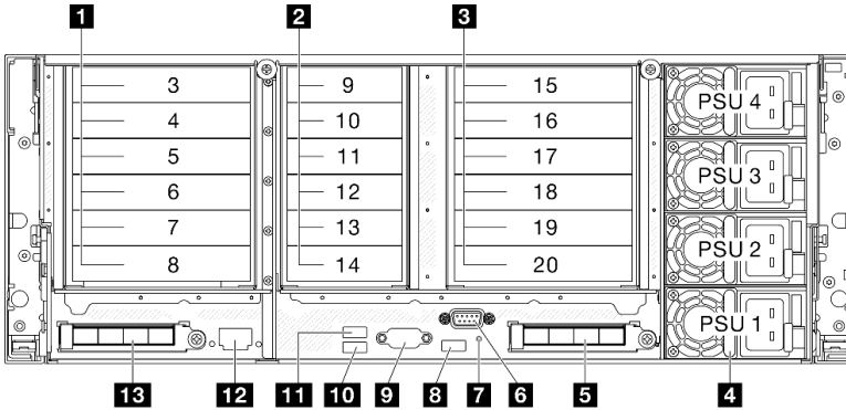
그림 3. 뒷면 보기
