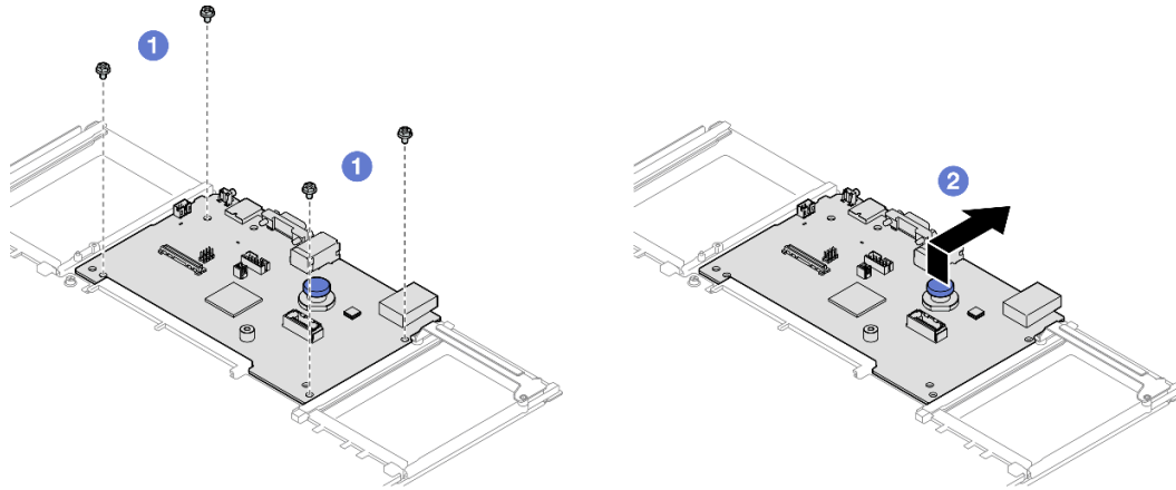
그림 214. 프로세서 보드에서 시스템 I/O 보드 분리
