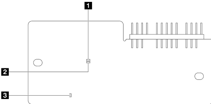
그림 245. 펌웨어 및 RoT 보안 모듈의 LED
