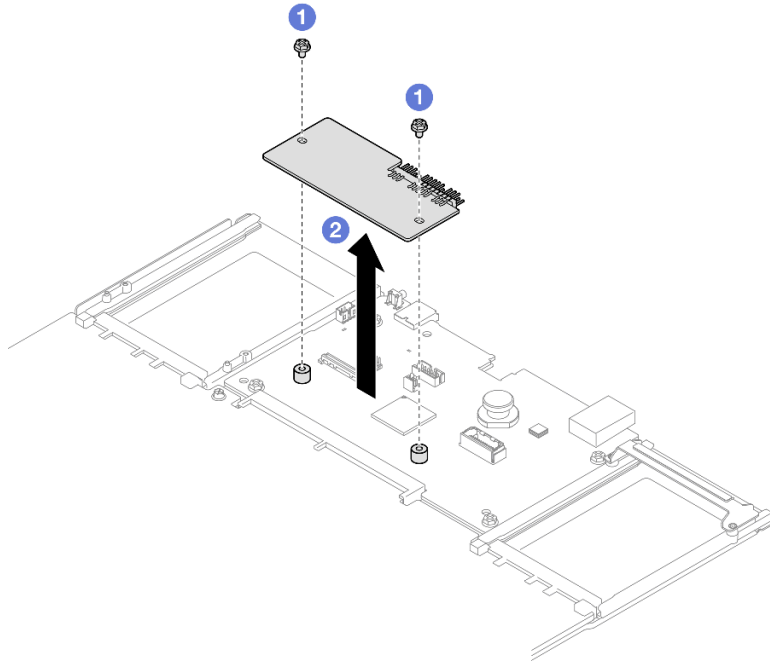
그림 211. 펌웨어 및 RoT 보안 모듈 제거
