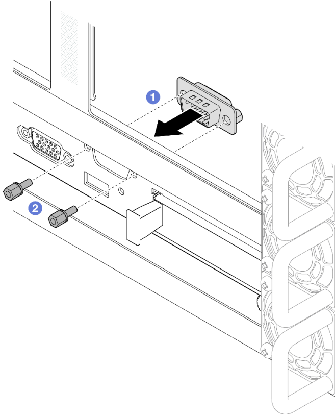
그림 208. 직렬 포트 모듈 설치
