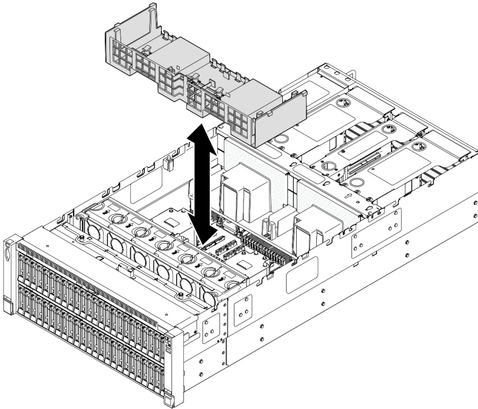
그림 43. 앞면 공기 조절 장치 설치
