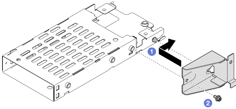
그림 31. 7mm 드라이브 케이지 브래킷 설치
