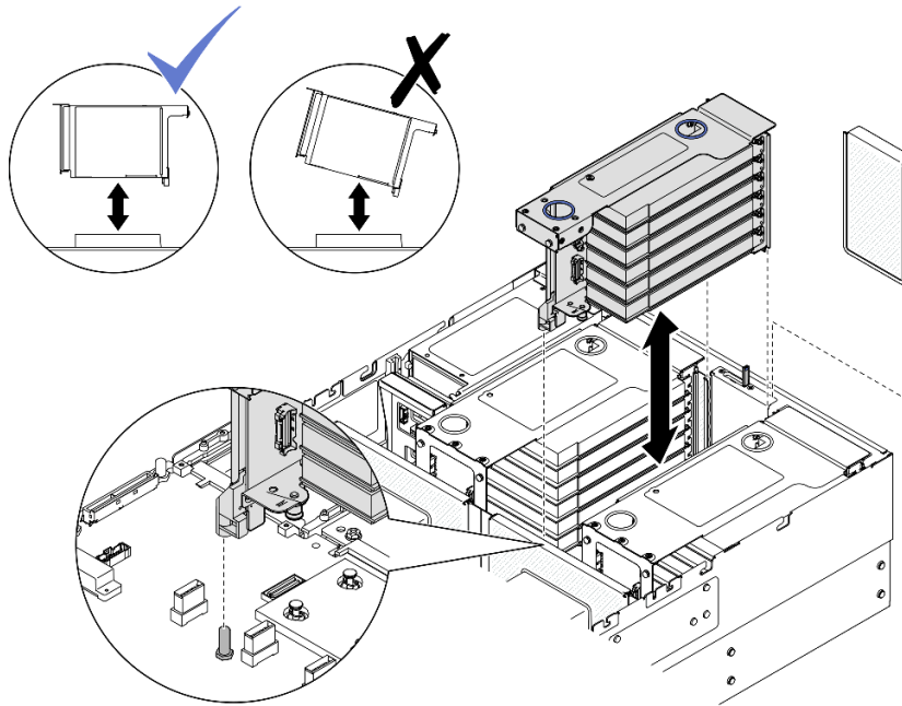
그림 138. PCIe 라이저 2 설치
