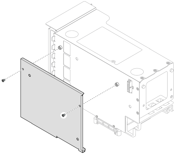
그림 161. 라이저에서 덮개 제거
