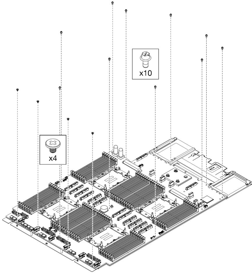
그림 249. 나사 제거
