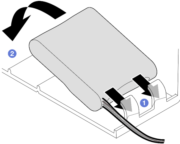
그림 86. 플래시 전원 모듈 설치
