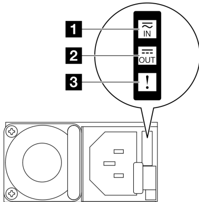
Рис. 16. Светодиодные индикаторы блока питания
