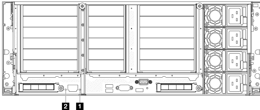
Рис. 15. Системные светодиодные индикаторы на задней панели
