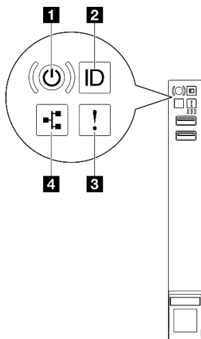
Рис. 14. Светодиодные индикаторы переднего модуля ввода-вывода
