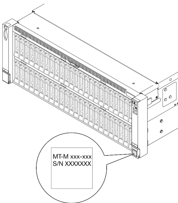
Рис. 22. Расположение идентификационной этикетки
