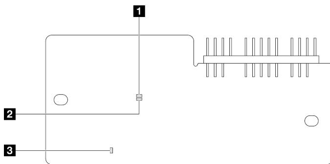
Рис. 19. Светодиодные индикаторы на компоненте «модуль безопасности микропрограммы и RoT»
