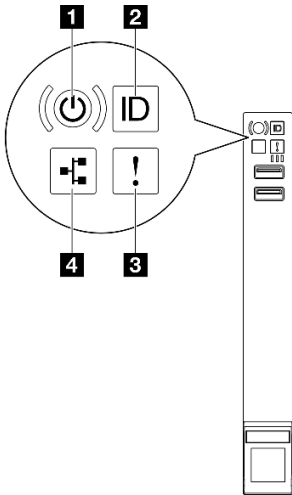
รูปภาพ 14. ไฟล์ LED โมดูล I/O ด้านหน้า
