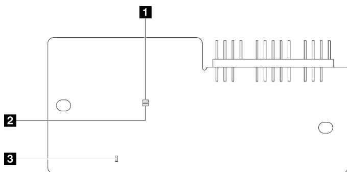
รูปภาพ 19. ไฟ LED บน โมดูลนิรภัยของเฟิร์มแวร์และ RoT
