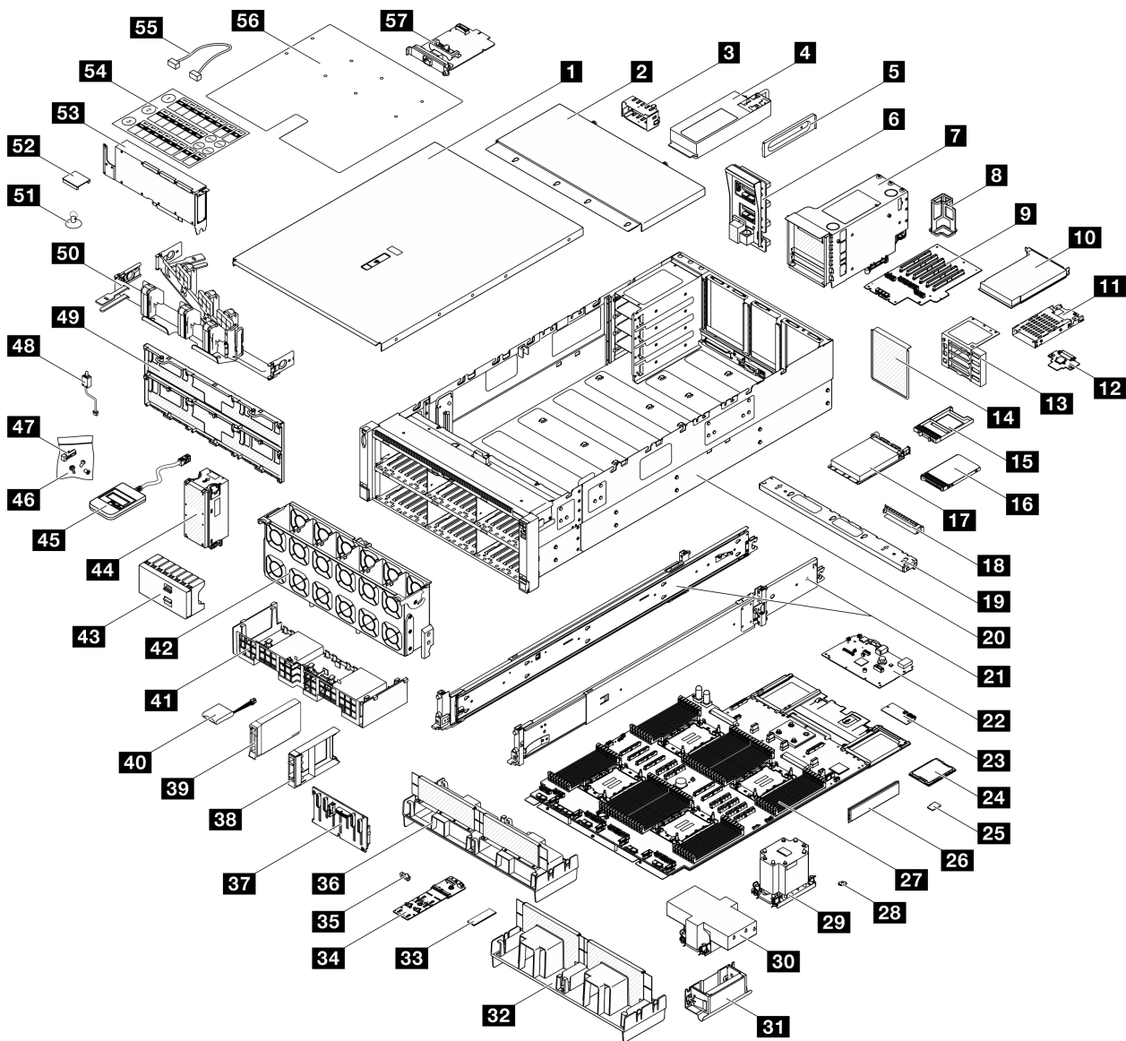
圖例 21. 伺服器元件
