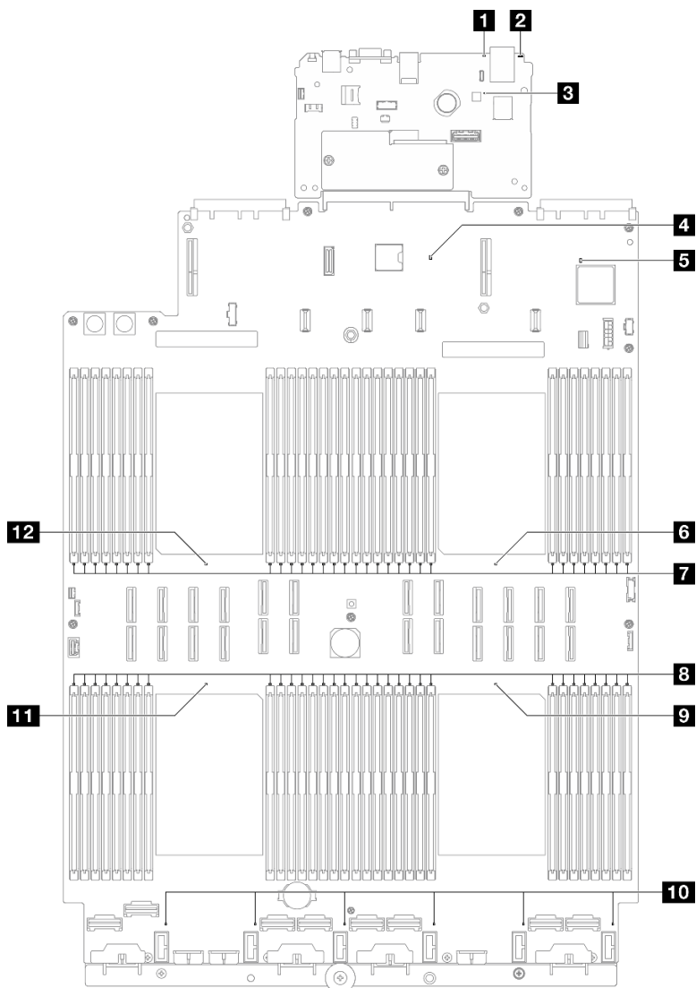
圖例 18. 主機板組件 LED
