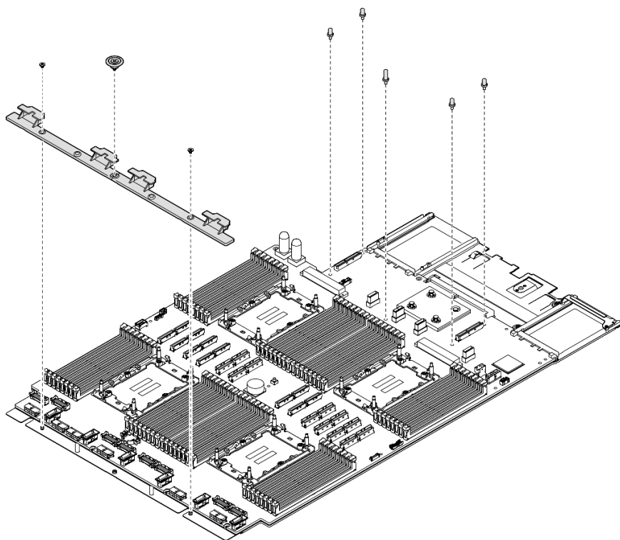
圖例 248. 卸下元件
