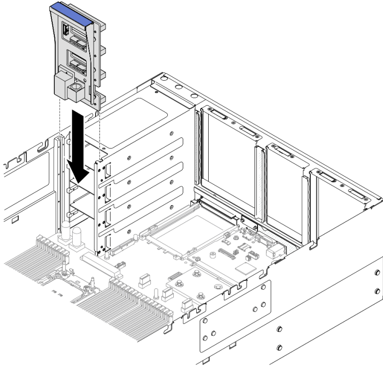
圖例 181. 安裝電源配送板
