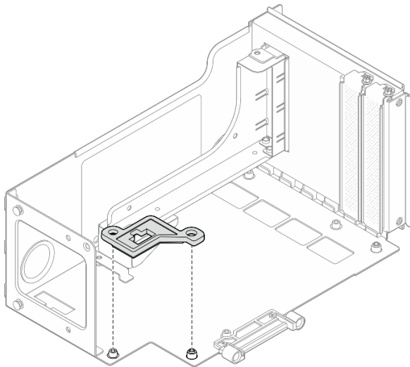
圖例 141. 從擴充卡卸下接頭導件
