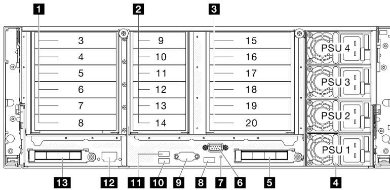
圖例 3. 背面圖
