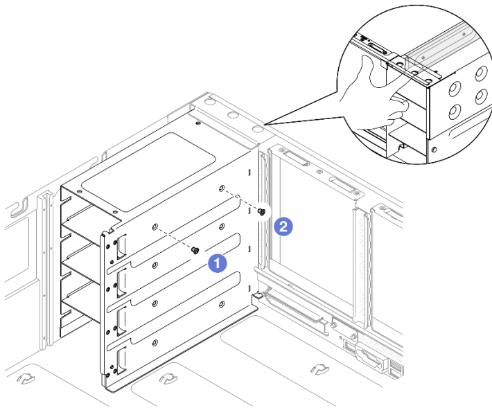
圖例 183. 卸下電源供應器托架螺絲
