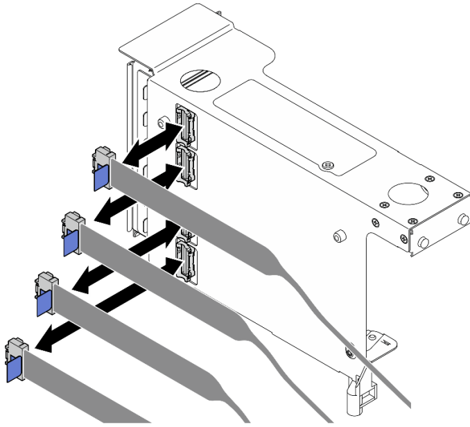
圖例 170. 將 PCIe 擴充卡纜線連接到擴充卡外部
