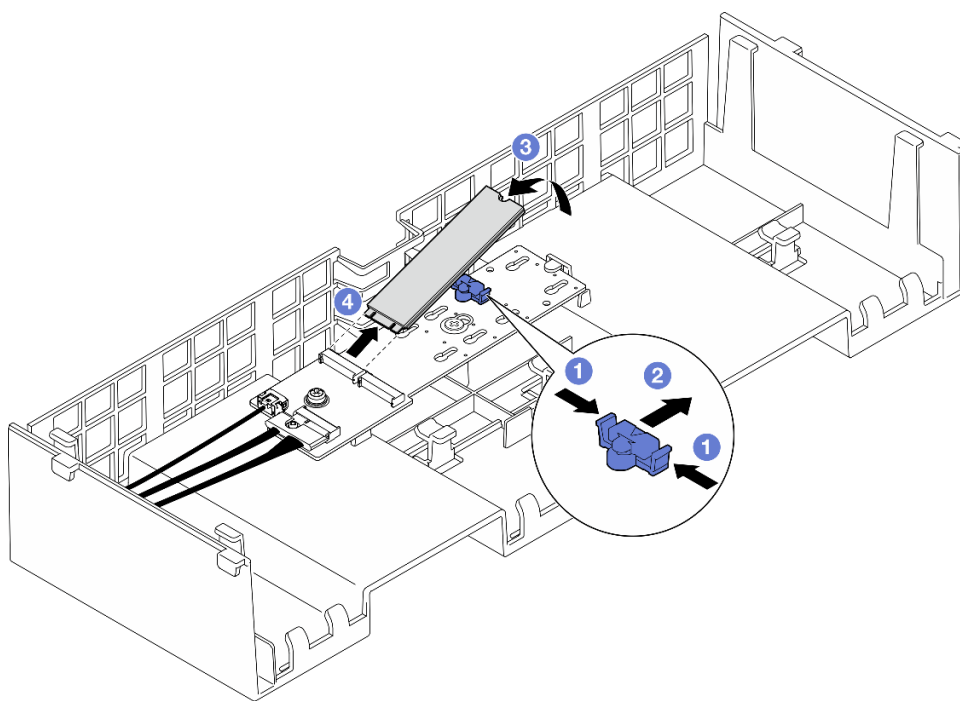
圖例 104. 卸下 M.2 硬碟
