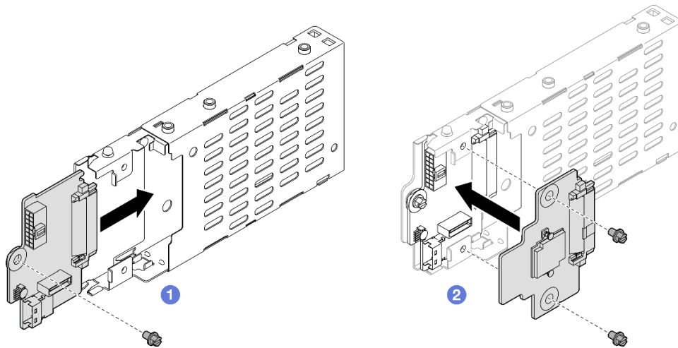
圖例 33. 安裝 7 公釐硬碟背板
