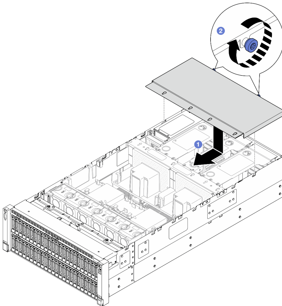
圖例 220. 安裝後方上蓋
