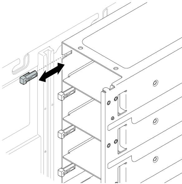
圖例 189. 安裝電源供應器鑰匙
