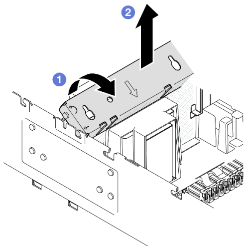
圖例 67. 卸下橫槓
