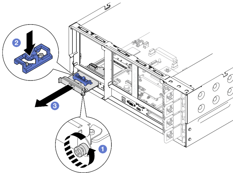
圖例 114. 卸下管理 NIC 配接卡
