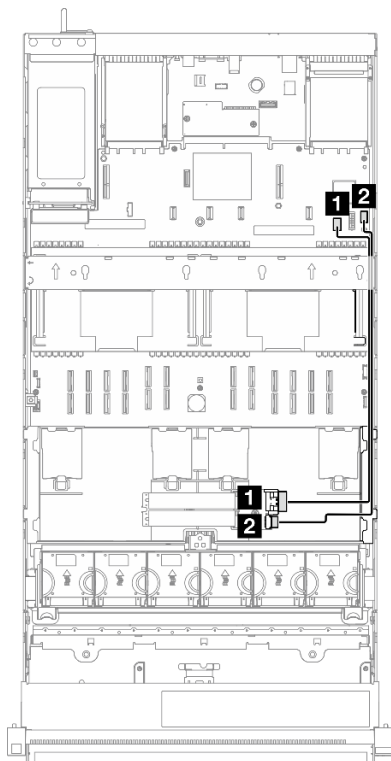
圖例 231. SATA/NVMe 或 NVMe M.2 開機配接卡的纜線佈線
