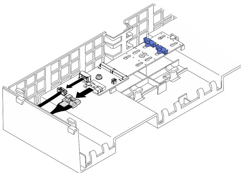
圖例 106. 從 SATA/x4 NVMe M.2 開機配接卡 拔下纜線
