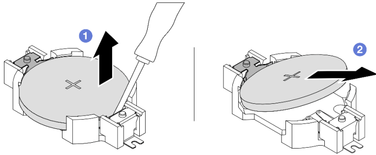
圖例 62. 卸下 CMOS 電池
