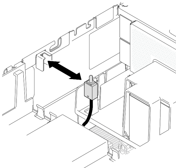
圖例 101. 卸下入侵開關
