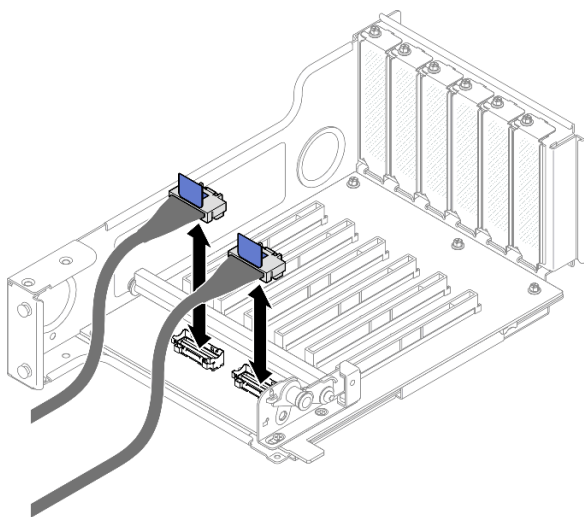
圖例 150. 從擴充卡內部拔下 PCIe 纜線
