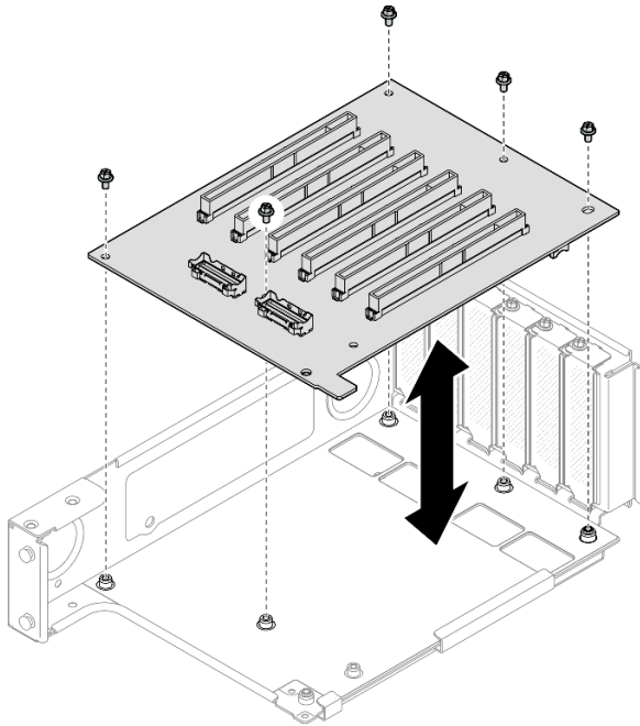
圖例 166. 將 PCIe 擴充卡安裝到擴充卡
