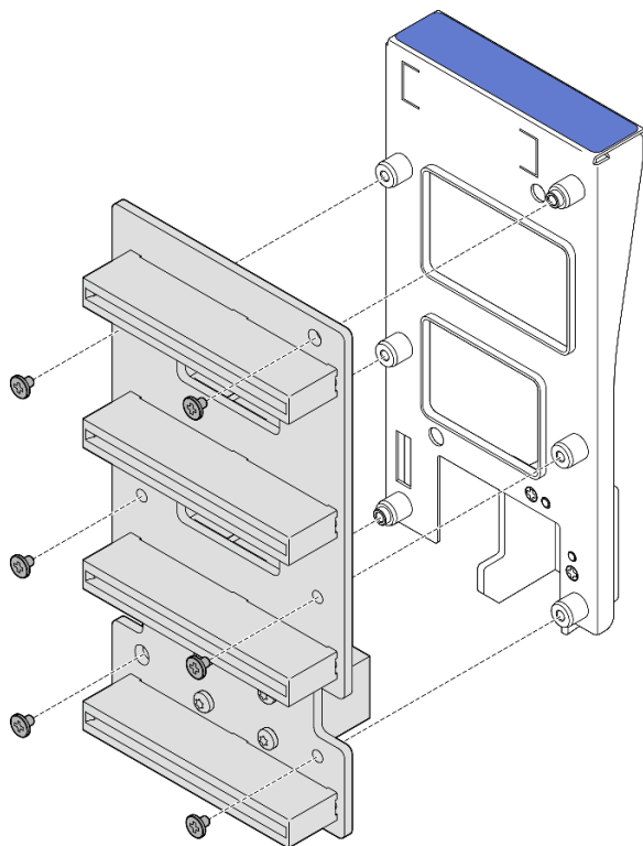
圖例 180. 拆卸電源配送板
