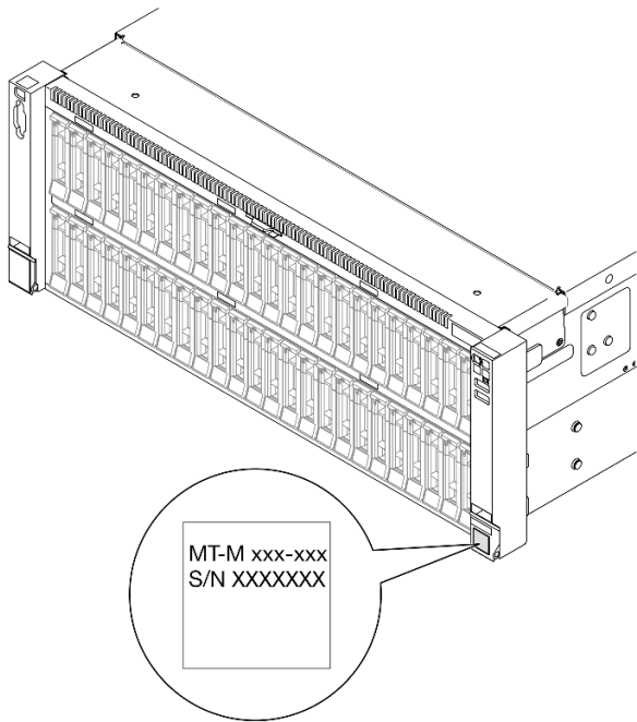
圖例 14. ID 標籤的位置
