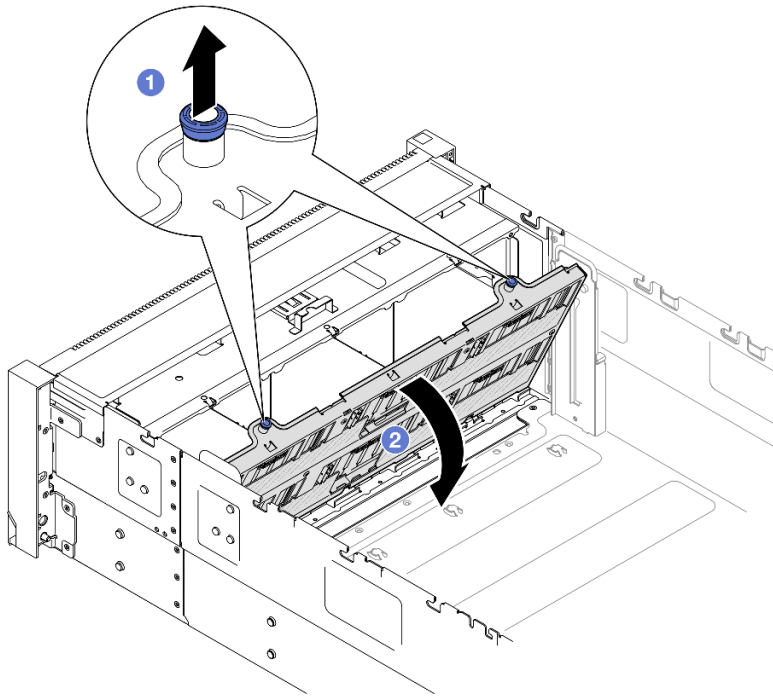
圖例 73. 卸下硬碟背板支架組件
