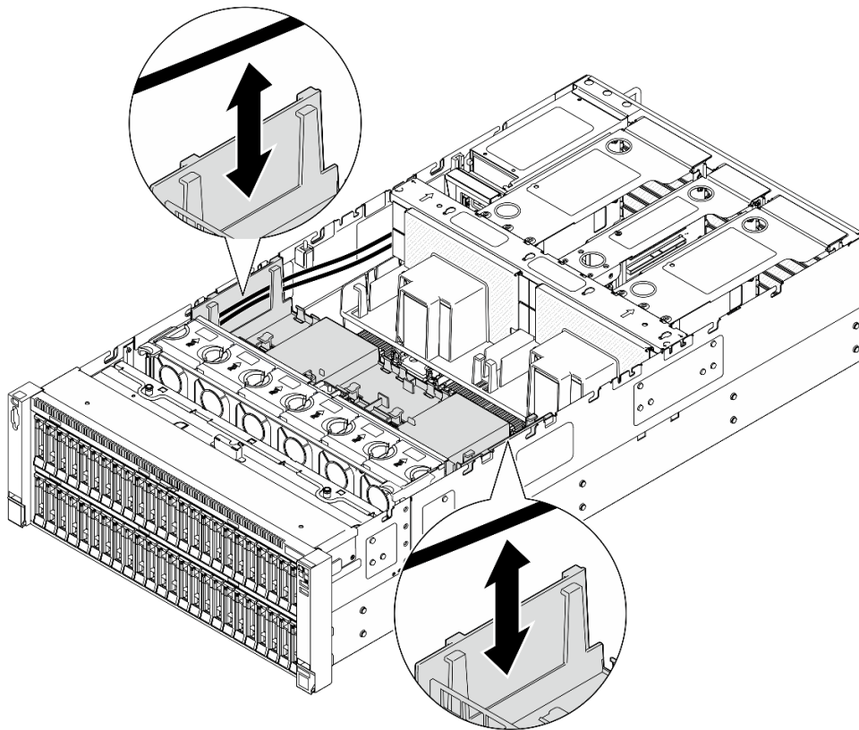
圖例 44. 將纜線穿過前方空氣擋板
