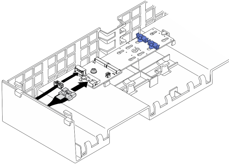
圖例 57. 將纜線連接到 SATA/x4 NVMe M.2 開機配接卡
