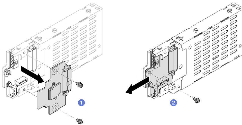
圖例 22. 拆卸 7 公釐框架
