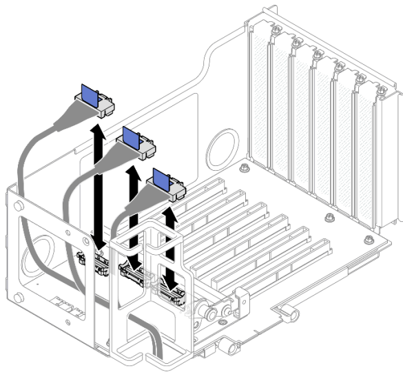
圖例 144. 從擴充卡內部拔下 PCIe 纜線
