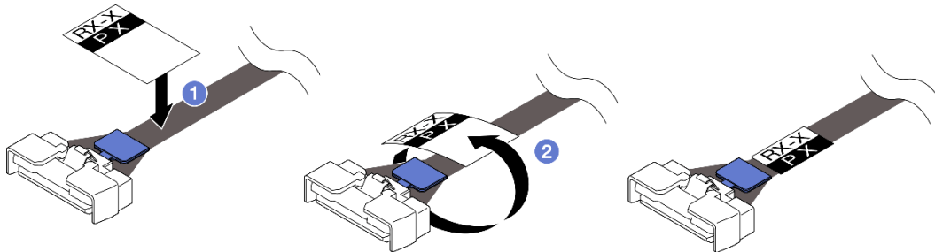
圖例 156. 將標籤貼在纜線上
