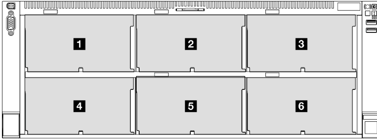
圖例 76. 硬碟背板編號
