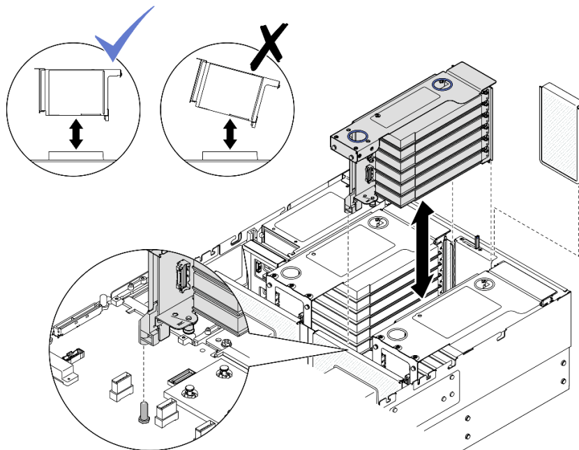
圖例 122. 卸下 PCIe 擴充卡 2
