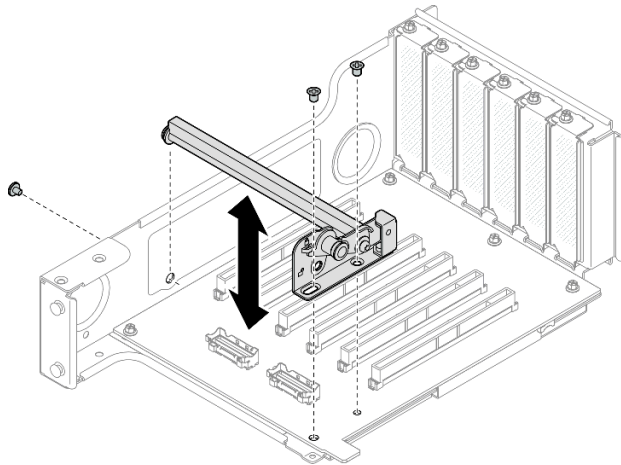
圖例 151. 從擴充卡卸下 PCIe 固定器
