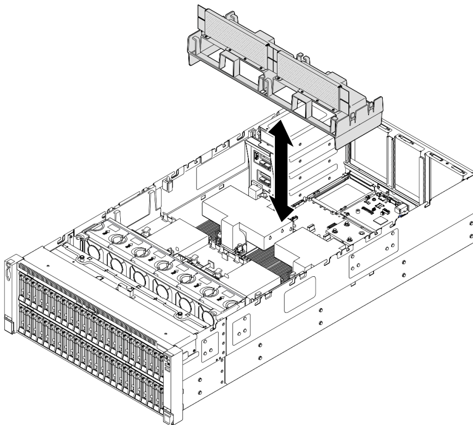
圖例 53. 為 2U 效能 PHM 卸下後方空氣擋板
