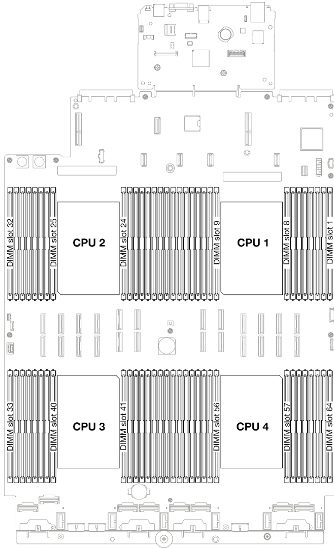
圖例 17. 記憶體模組和處理器佈置
