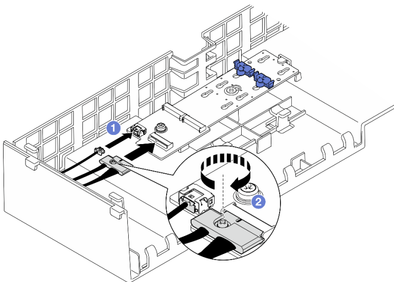
圖例 109. 將纜線連接到 SATA/NVMe 或 NVMe M.2 開機配接卡
