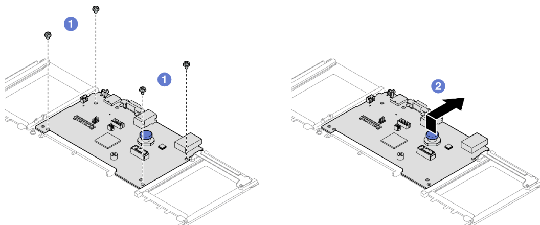
圖例 214. 將系統 I/O 板與處理器板分開
