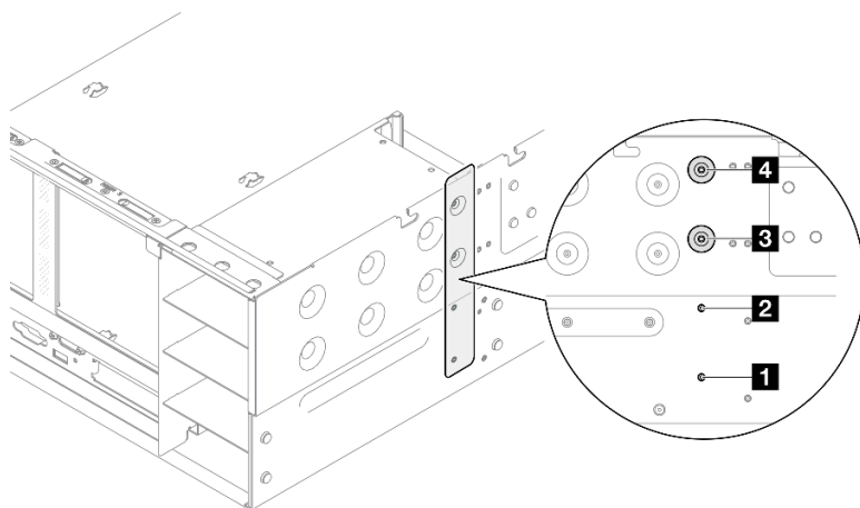
圖例 187. 卸下電源供應器鑰匙螺絲
