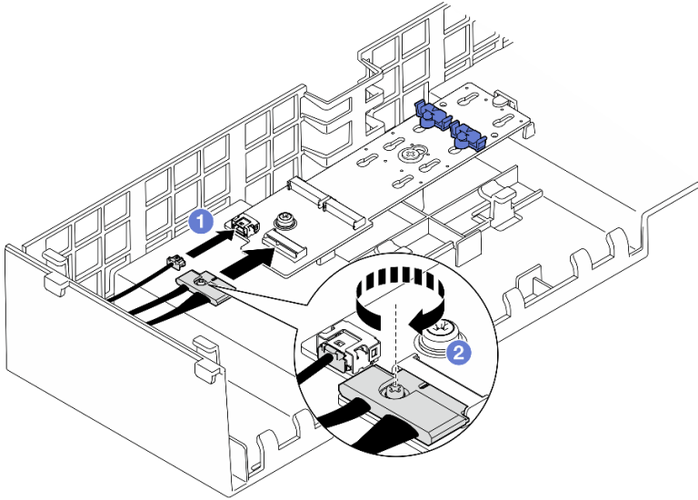
圖例 46. 將纜線連接到 SATA/NVMe 或 NVMe M.2 開機配接卡
