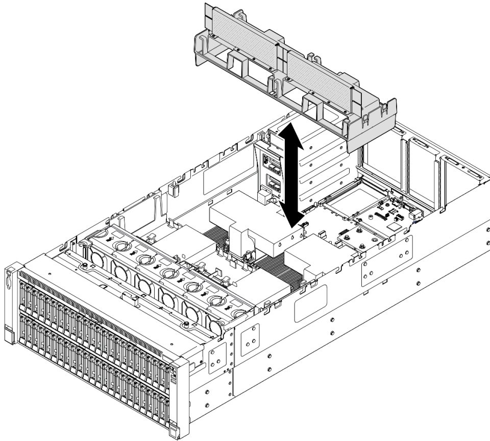
圖例 55. 為 2U 效能 PHM 安裝後方空氣擋板
