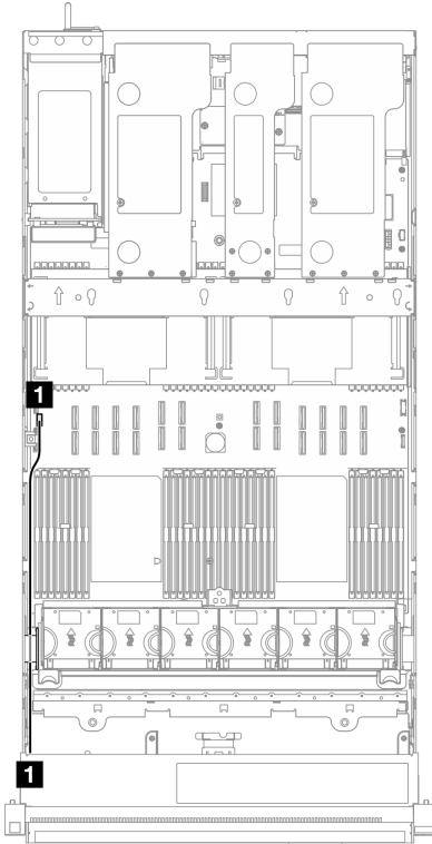
圖例 228. 外部診斷手持裝置接頭的纜線佈線
