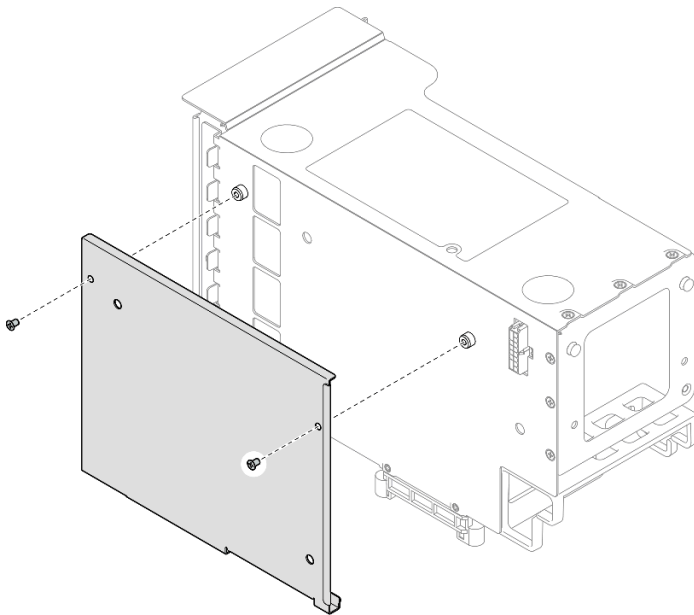
圖例 161. 從擴充卡卸下蓋板
