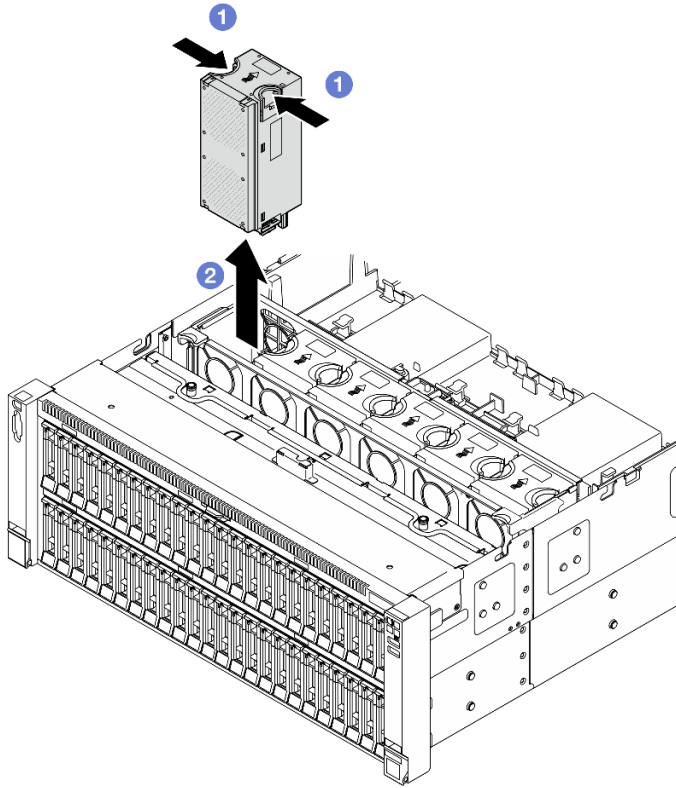
圖例 80. 卸下風扇模組
