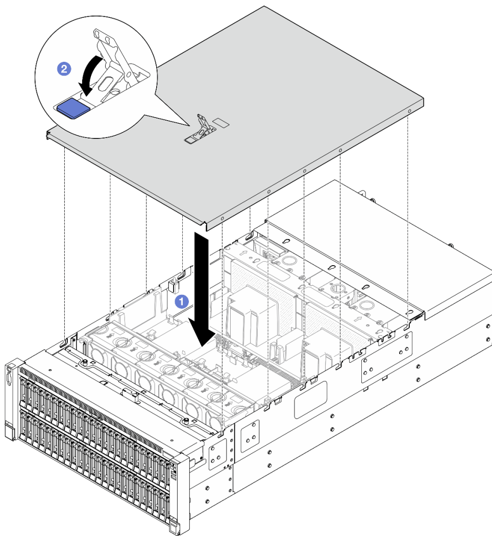
圖例 221. 安裝前方上蓋
