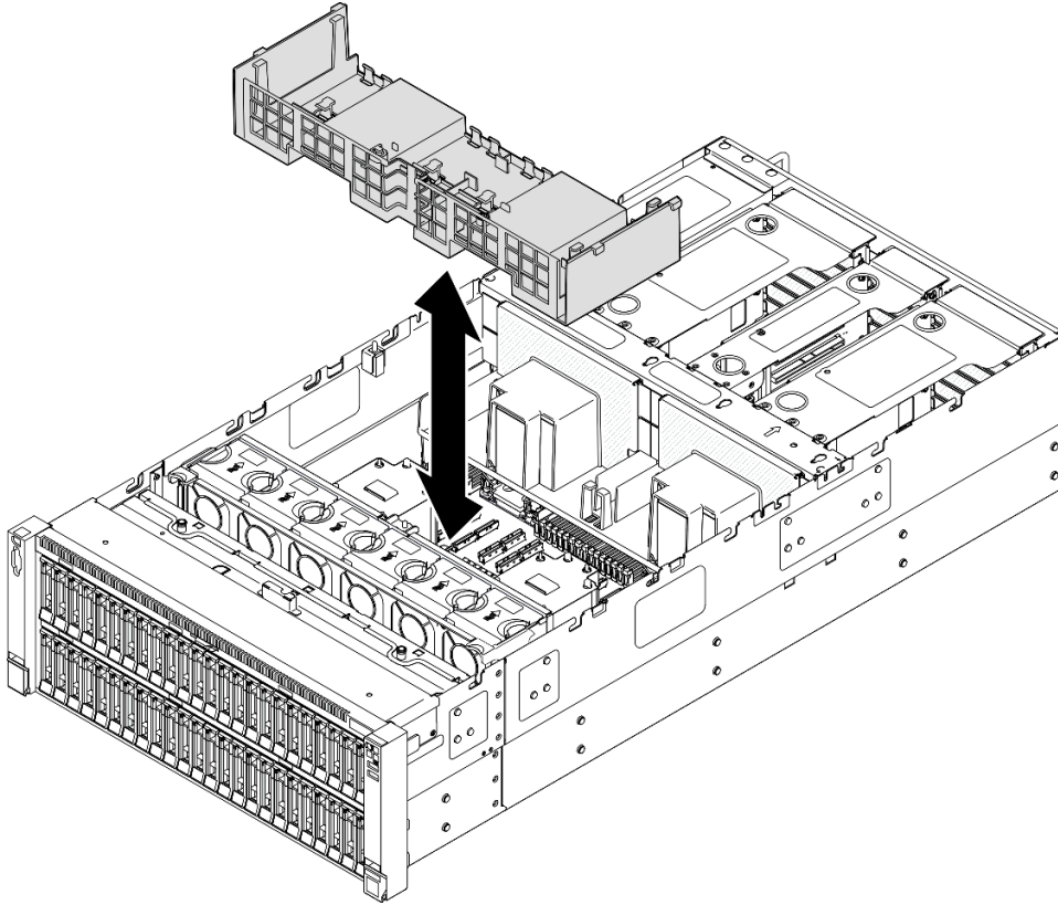
圖例 42. 卸下前方空氣擋板
