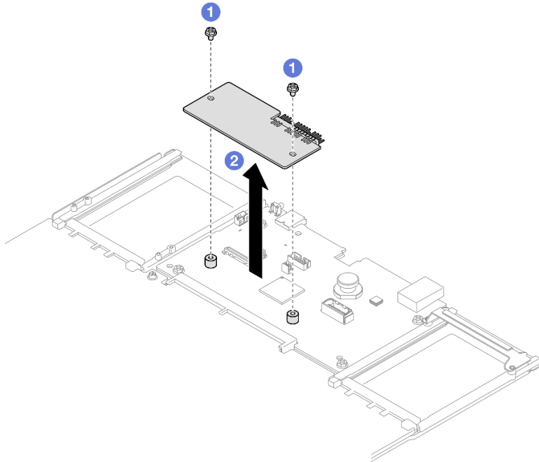
圖例 211. 卸下韌體和 RoT 安全模組
