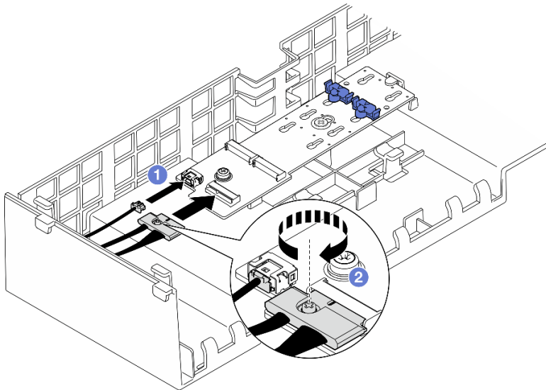
圖例 58. 將纜線連接到 SATA/NVMe 或 NVMe M.2 開機配接卡
