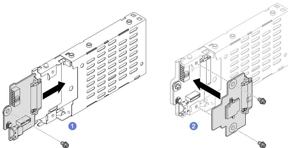
圖例 28. 安裝 7 公釐硬碟背板
