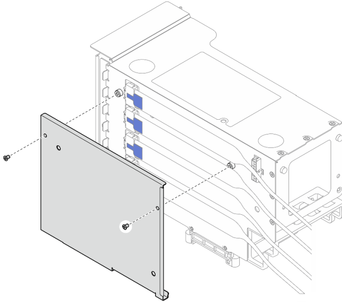
圖例 142. 從擴充卡卸下蓋板
