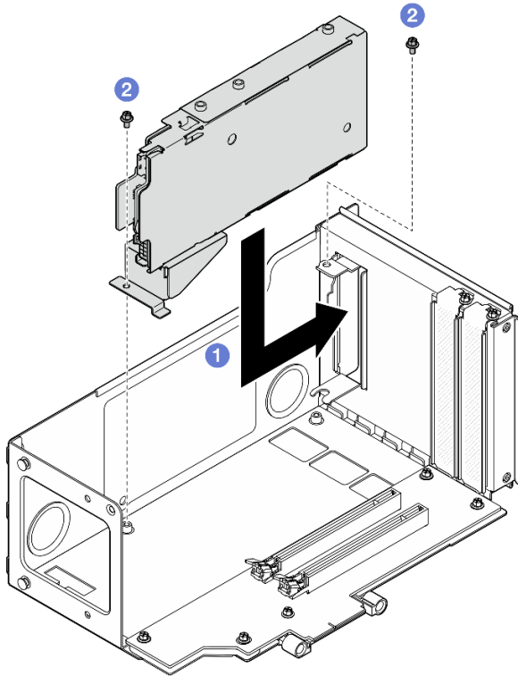
圖例 32. 將 7 公釐框架安裝到擴充卡
