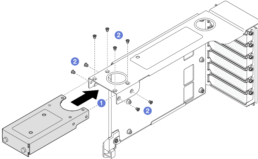
圖例 177. 將 PCIe 擴充卡延伸器安裝到 FH PCIe 擴充卡
