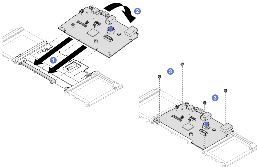
圖例 215. 將系統 I/O 板安裝在處理器板上
