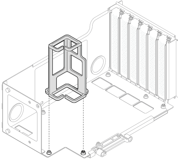
圖例 157. 將纜線固定夾安裝到擴充卡
