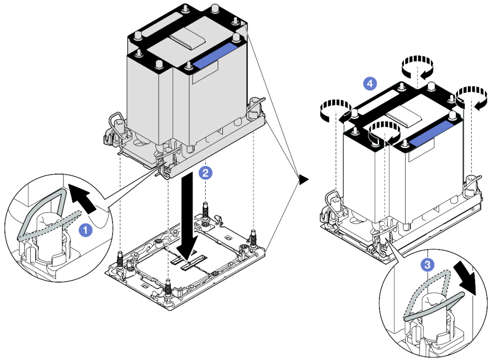
圖例 202. 安裝 3U 標準 PHM
