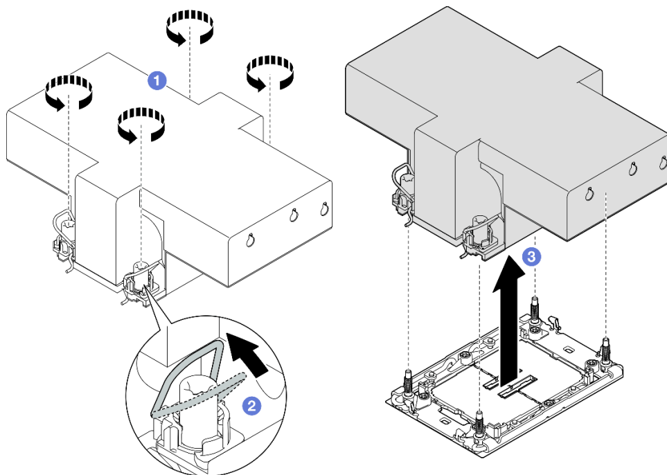
圖例 195. 卸下 2U 效能 PHM
