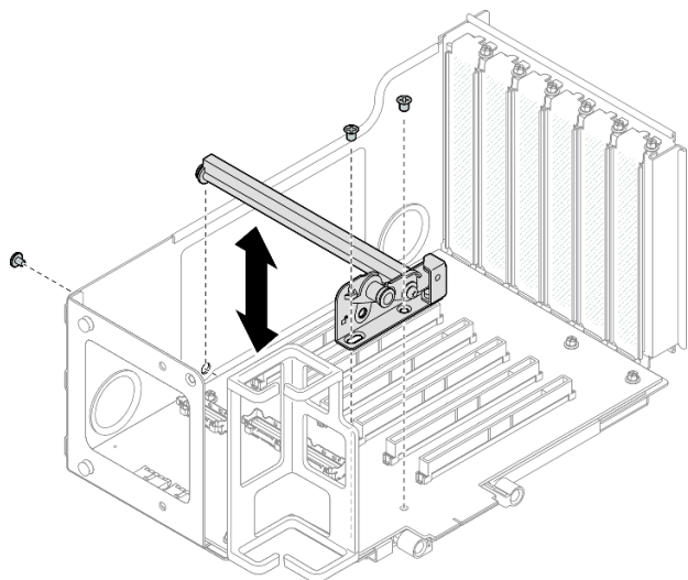
圖例 159. 將 PCIe 固定器安裝到擴充卡
