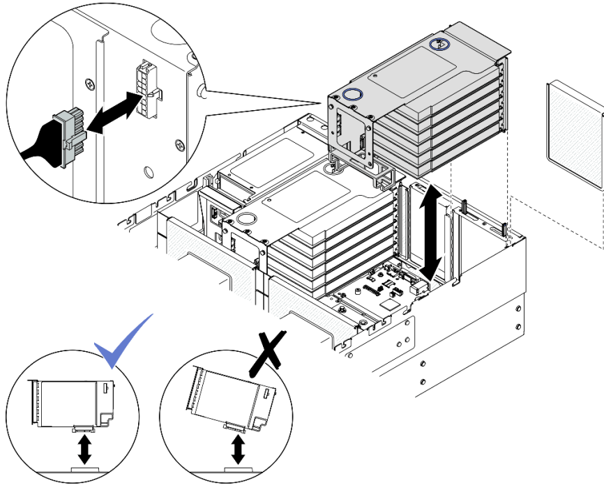
圖例 137. 安裝 PCIe 擴充卡 1
