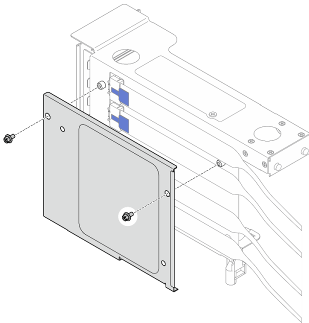
圖例 171. 將蓋板安裝到擴充卡
