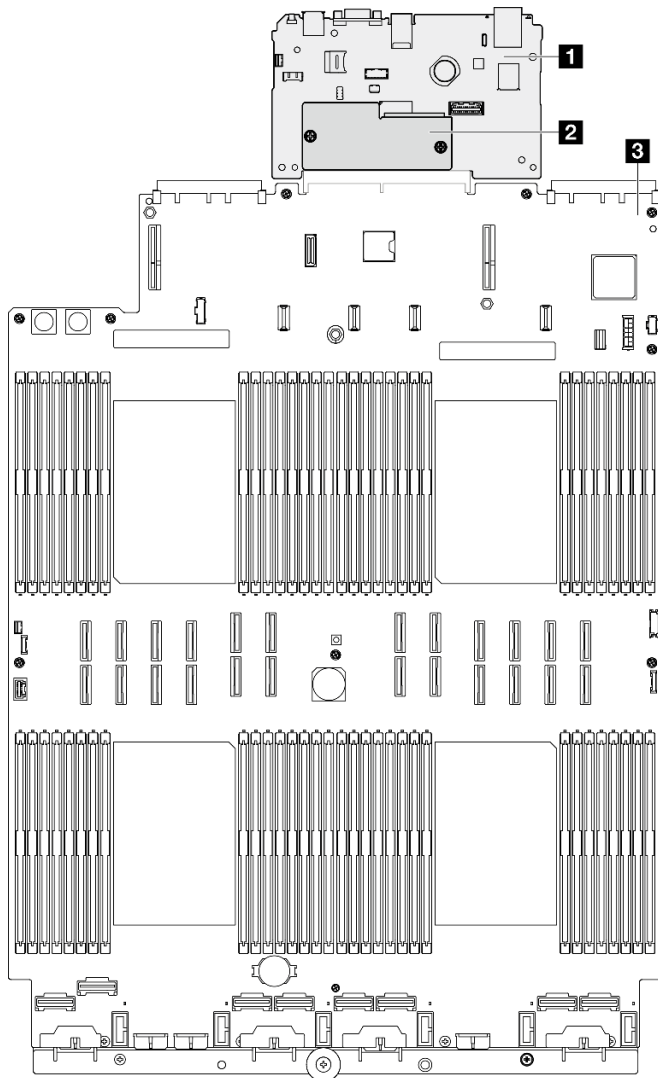
圖例 210. 主機板組件佈置
