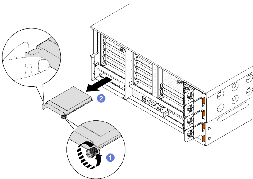
圖例 120. 卸下 OCP 模組
