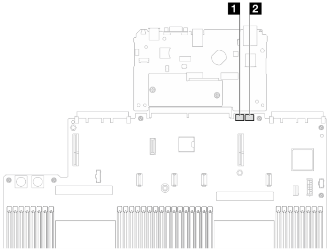
圖例 12. 主機板組件開關
