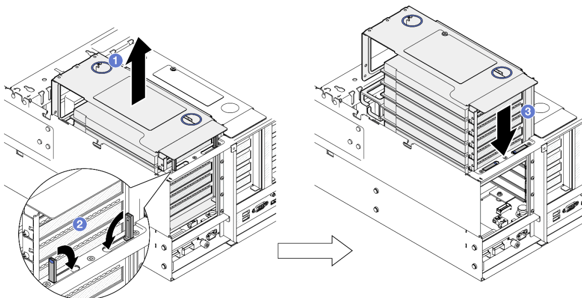
圖例 70. 固定 PCIe 擴充卡
