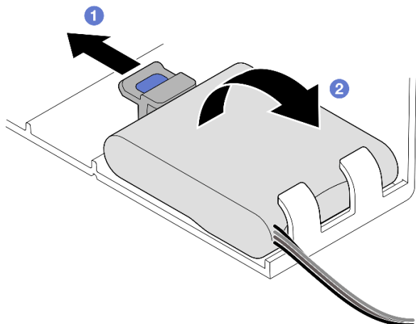
圖例 85. 卸下快閃記憶體電源模組
