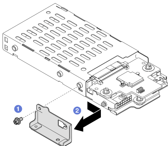
圖例 26. 卸下 7 公釐框架托架
