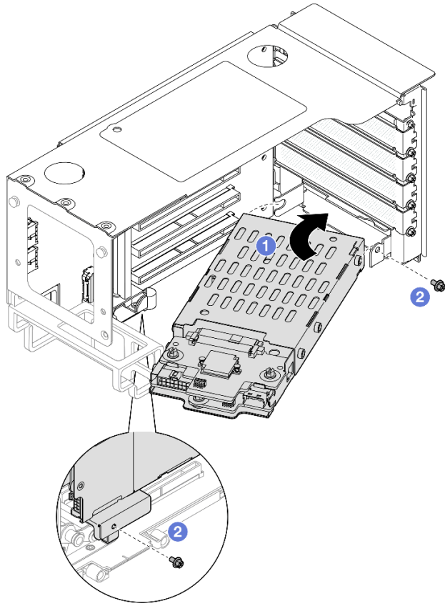
圖例 35. 將 7 公釐框架安裝到擴充卡
