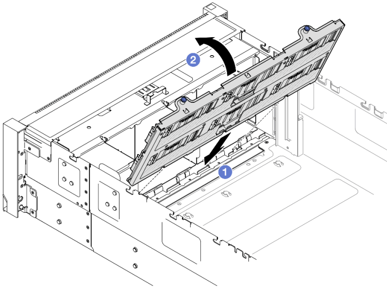
圖例 79. 安裝硬碟背板支架組件
