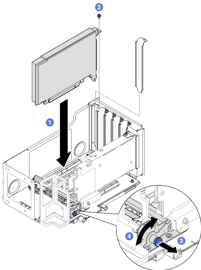
圖例 132. 將 PCIe 配接卡安裝到擴充卡
