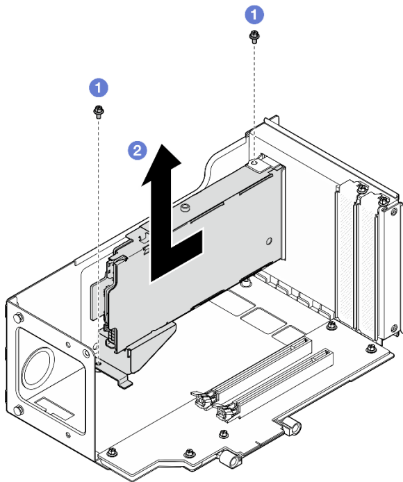
圖例 20. 從擴充卡卸下 7 公釐框架
