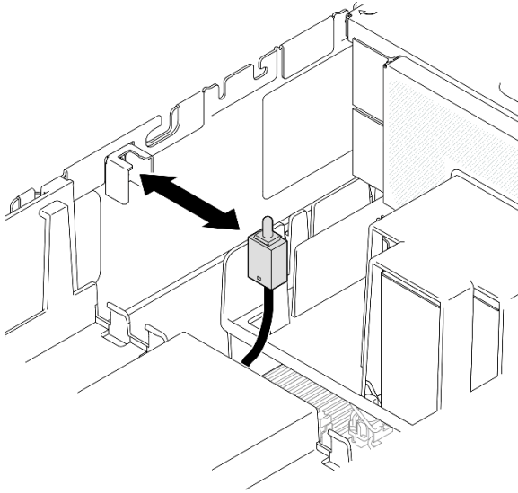
圖例 102. 安裝入侵開關
