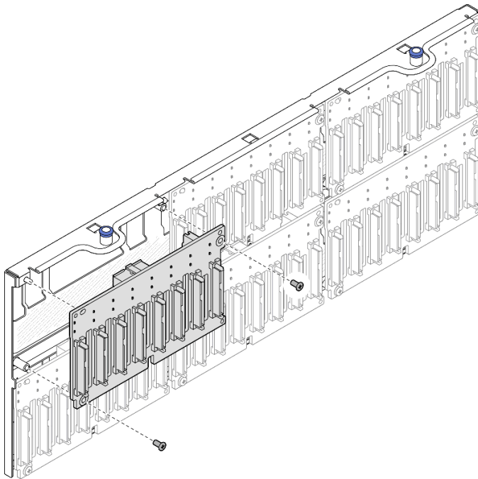
圖例 74. 從支架上卸下背板
