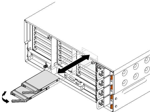
圖例 37. 安裝 7 公釐硬碟
