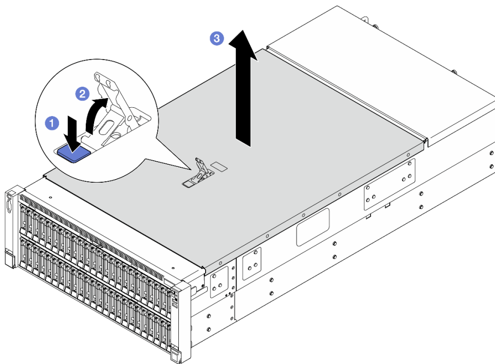
圖例 218. 卸下前方上蓋
