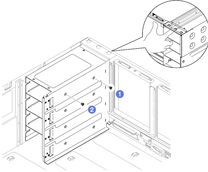
圖例 186. 固定電源供應器托架
