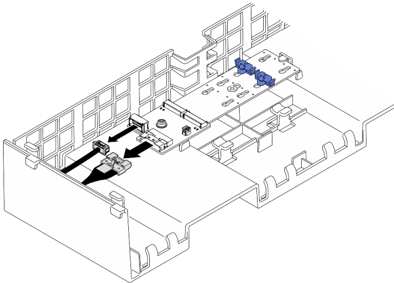
圖例 39. 從 SATA/x4 NVMe M.2 開機配接卡 拔下纜線
