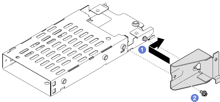
圖例 31. 安裝 7 公釐框架托架
