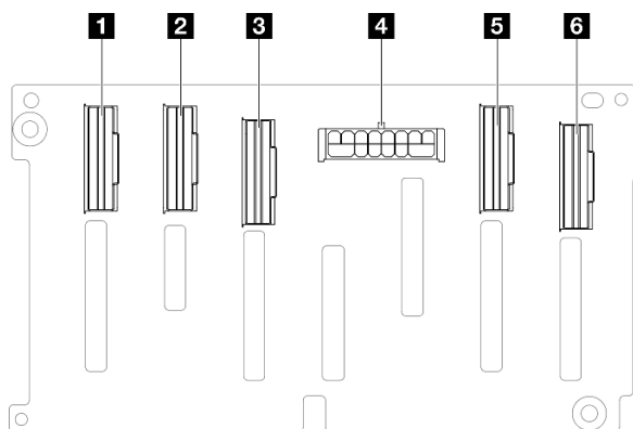
圖例 223. 2.5 吋 AnyBay 8 機槽硬碟背板接頭
