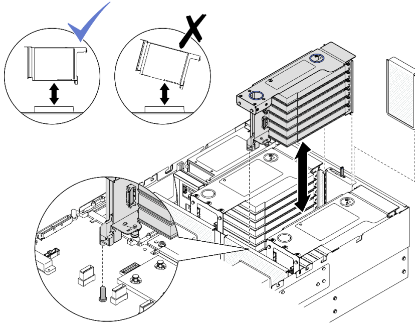
圖例 125. 卸下 PCIe 擴充卡 2
