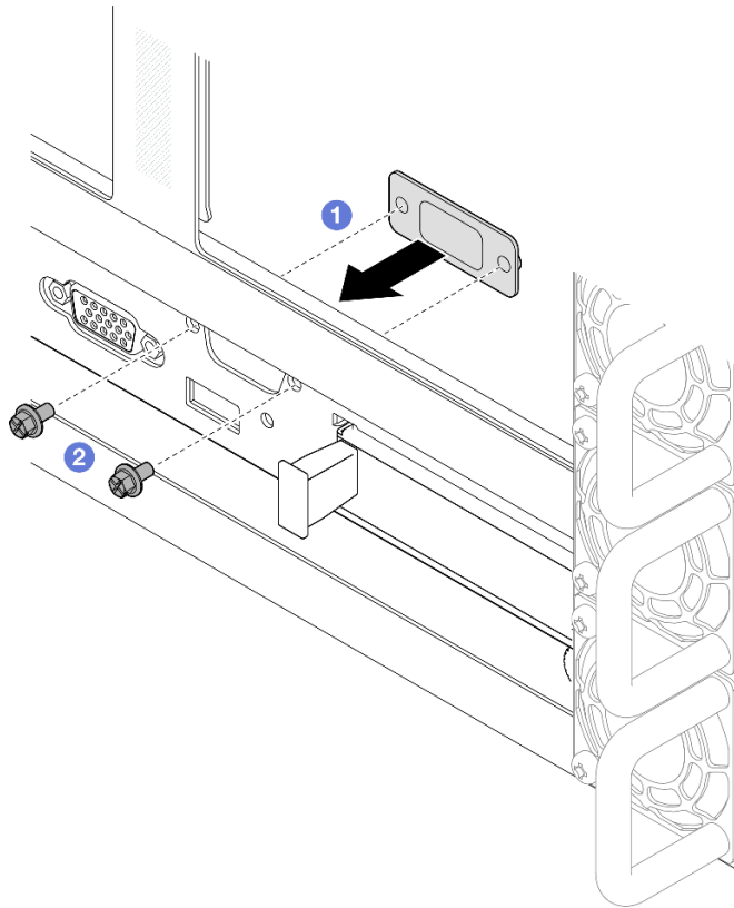
圖例 206. 安裝序列埠填充板
