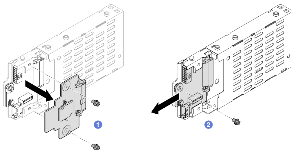
圖例 27. 拆卸 7 公釐框架
