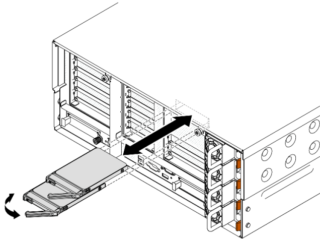
圖例 19. 卸下 7 公釐硬碟
