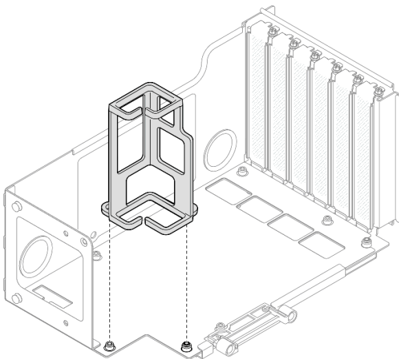
圖例 147. 從擴充卡卸下纜線固定夾
