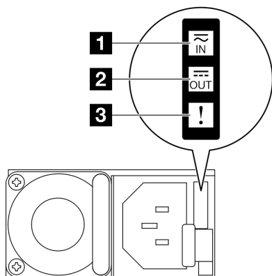
圖例 242. 電源供應器 LED
