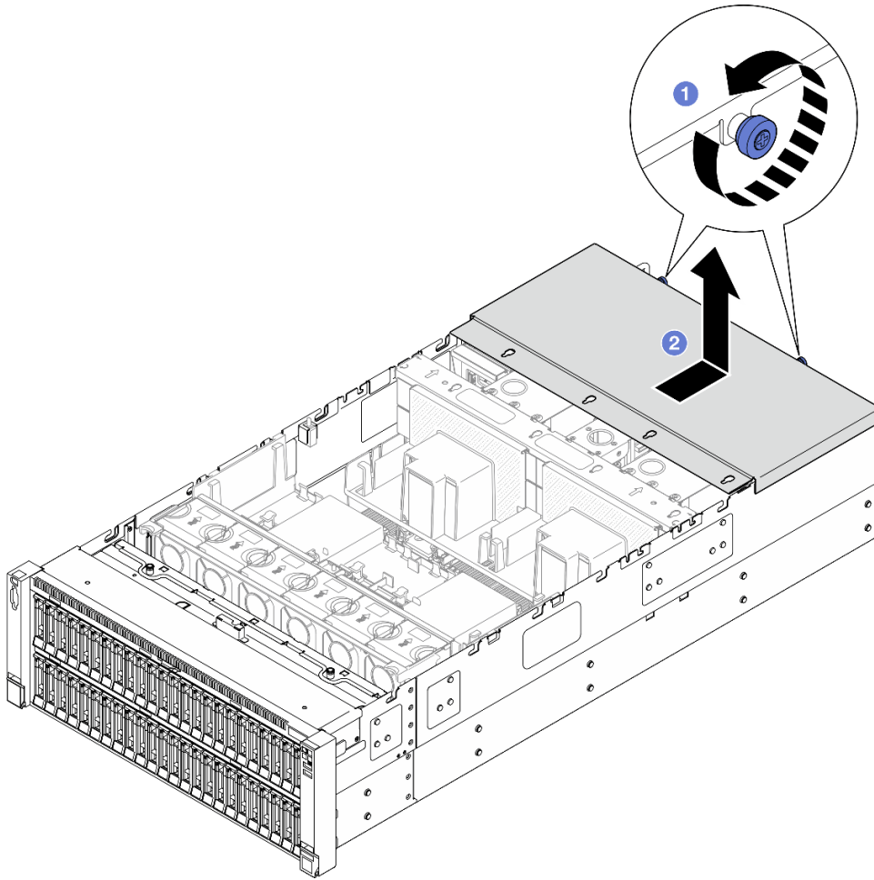
圖例 219. 卸下後方上蓋
