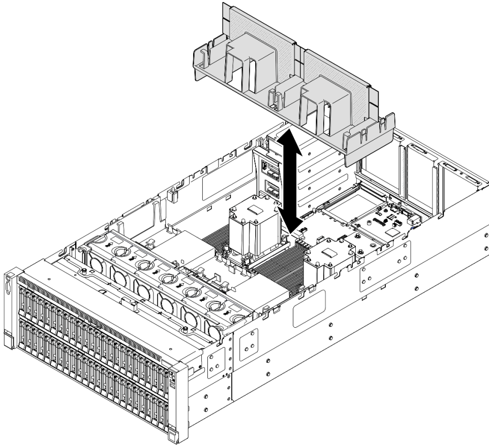
圖例 54. 為 3U 標準 PHM 安裝後方空氣擋板
