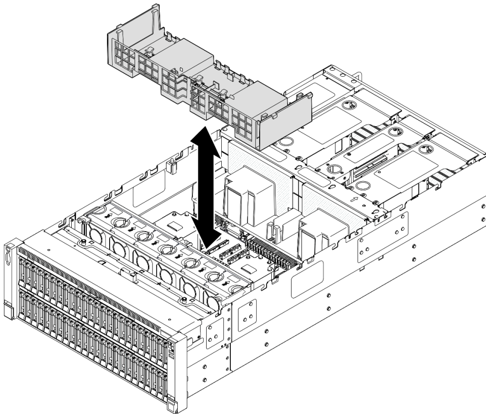
圖例 43. 安裝前方空氣擋板
