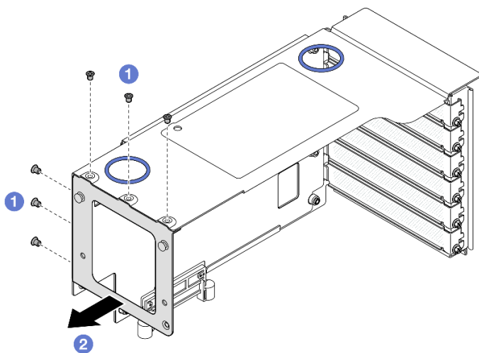
圖例 174. 從 FH PCIe 擴充卡卸下填充板
