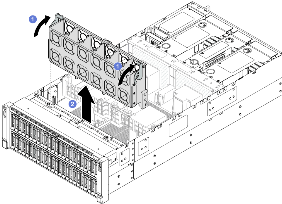
圖例 81. 卸下風扇機盒
