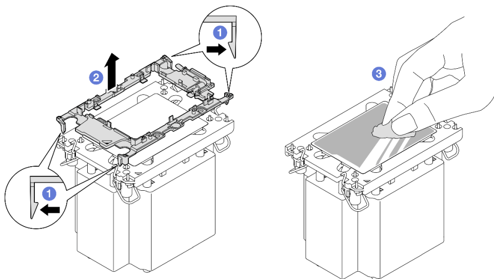
圖例 197. 將處理器支架與散熱槽分開
