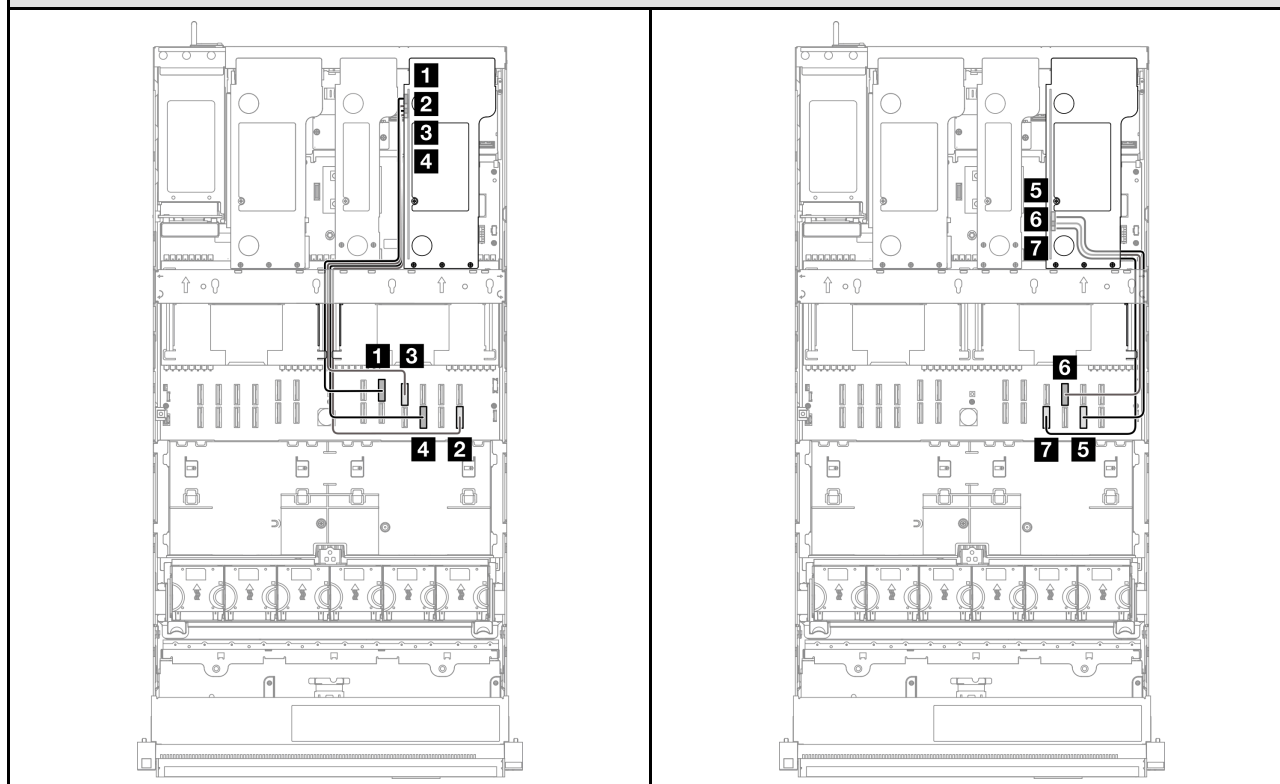
六插槽 Gen 5 FH 擴充卡 (PCIe 擴充卡 1) 的纜線佈線
