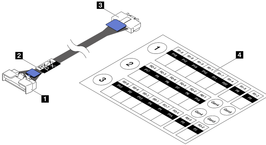
圖例 155. PCIe 擴充卡纜線
