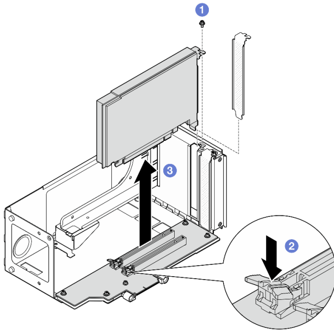
圖例 128. 從擴充卡卸下 PCIe 配接卡
