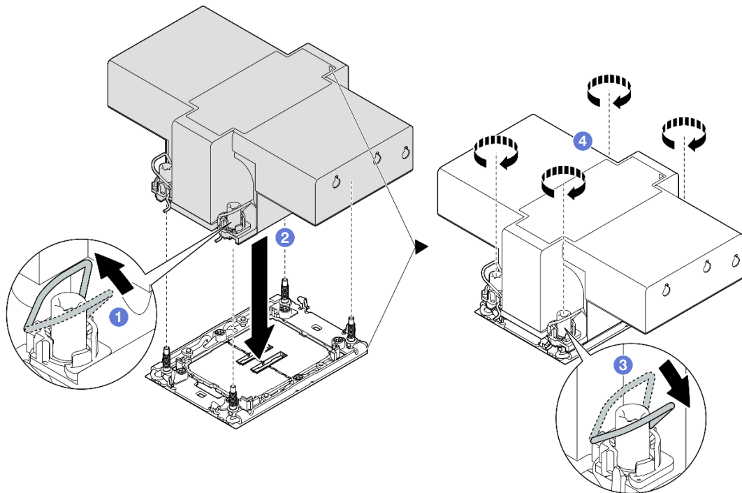
圖例 203. 安裝 2U 效能 PHM
