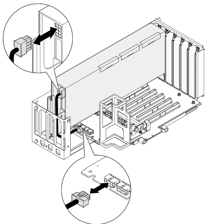
圖例 91. 從 GPU 配接卡拔下電源線
