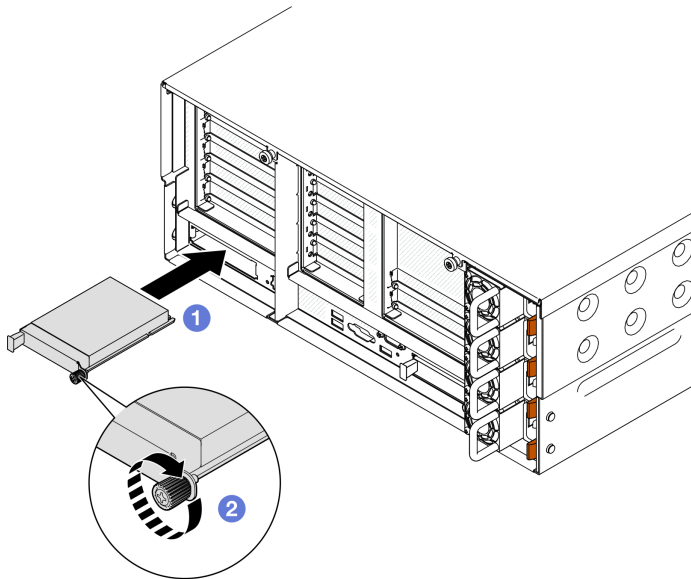
圖例 121. 安裝 OCP 模組
