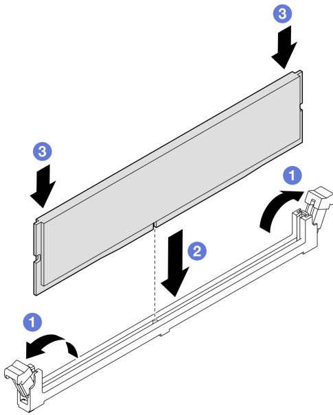
圖例 117. 安裝記憶體模組
