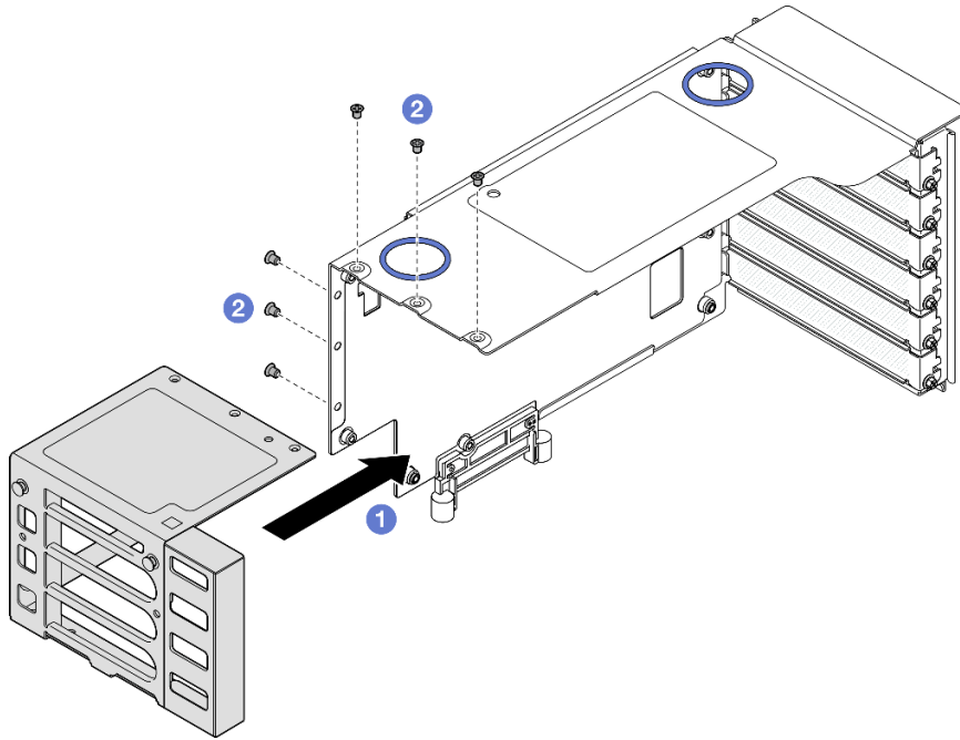
圖例 175. 將 PCIe 擴充卡延伸器安裝到 FH PCIe 擴充卡
