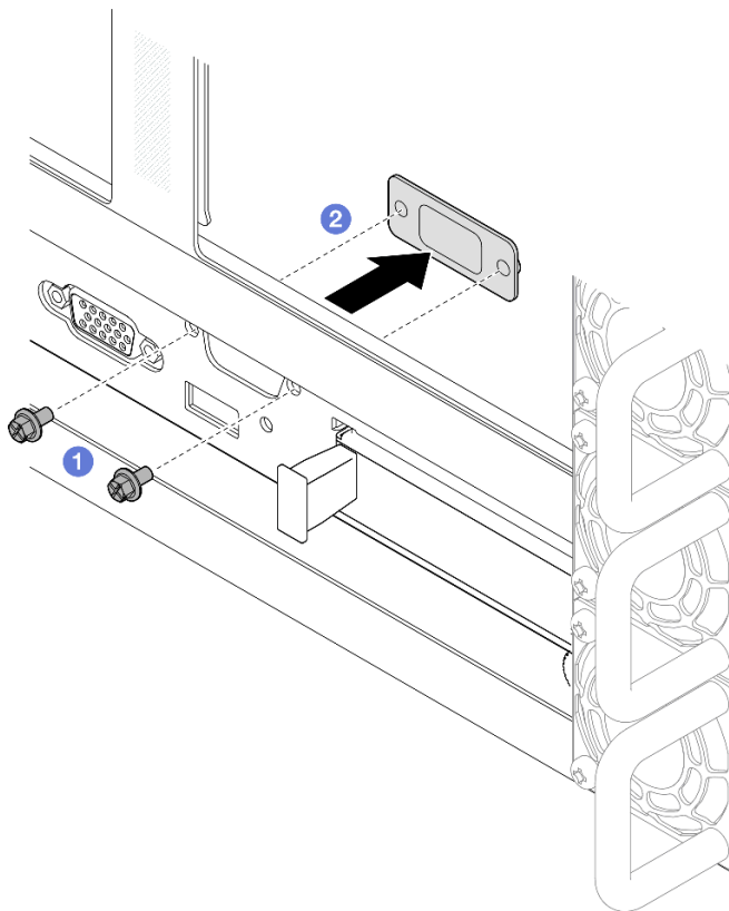
圖例 207. 卸下序列埠填充板
