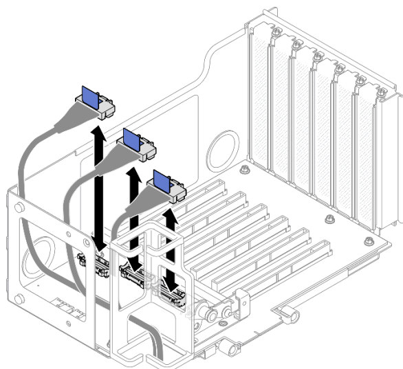
圖例 160. 將 PCIe 擴充卡纜線連接到擴充卡內部
