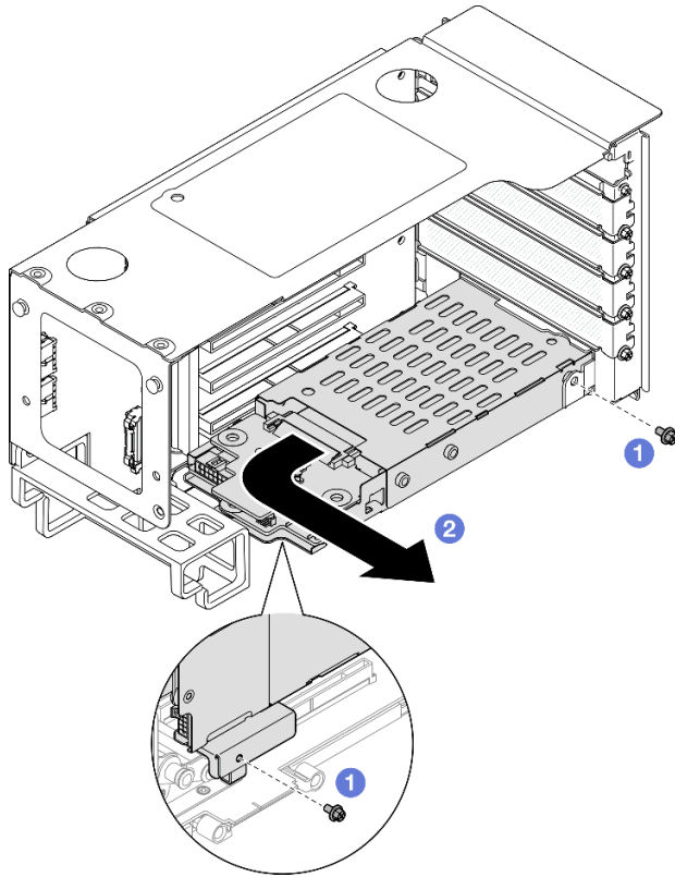
圖例 25. 從擴充卡卸下 7 公釐框架
