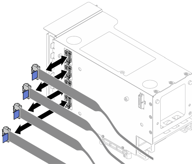
圖例 143. 從擴充卡外部拔下 PCIe 纜線
