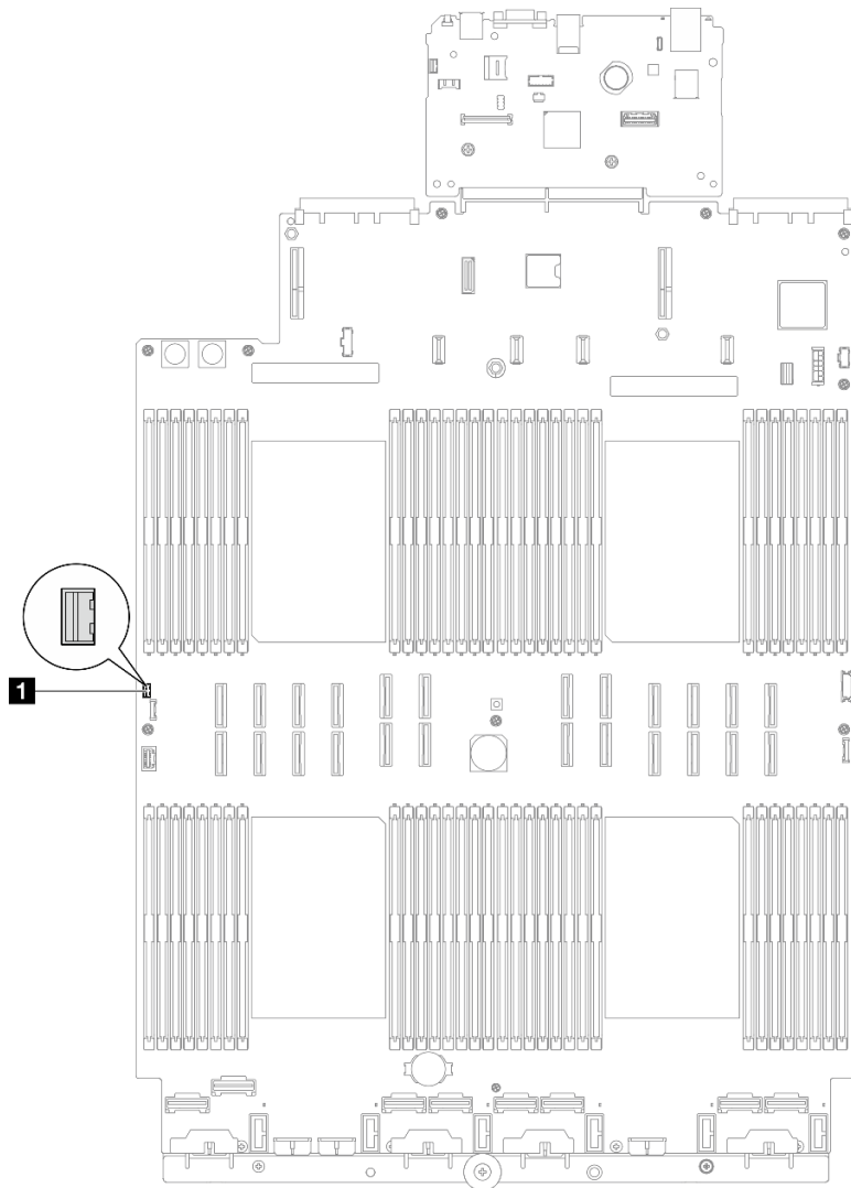
圖例 100. 中斷入侵開關的纜線連接
