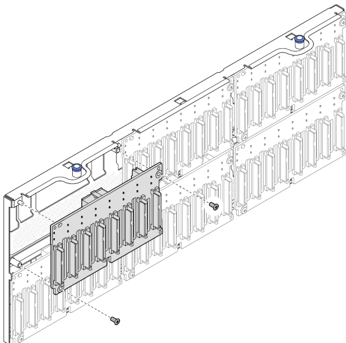
圖例 78. 將背板安裝到支架
