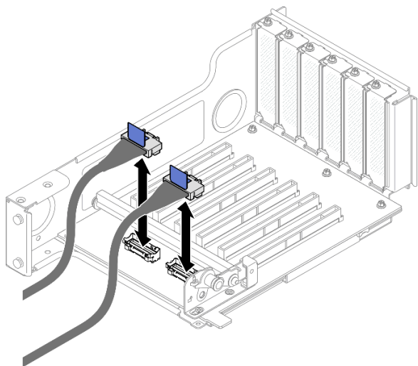
圖例 168. 將 PCIe 擴充卡纜線連接到擴充卡內部
