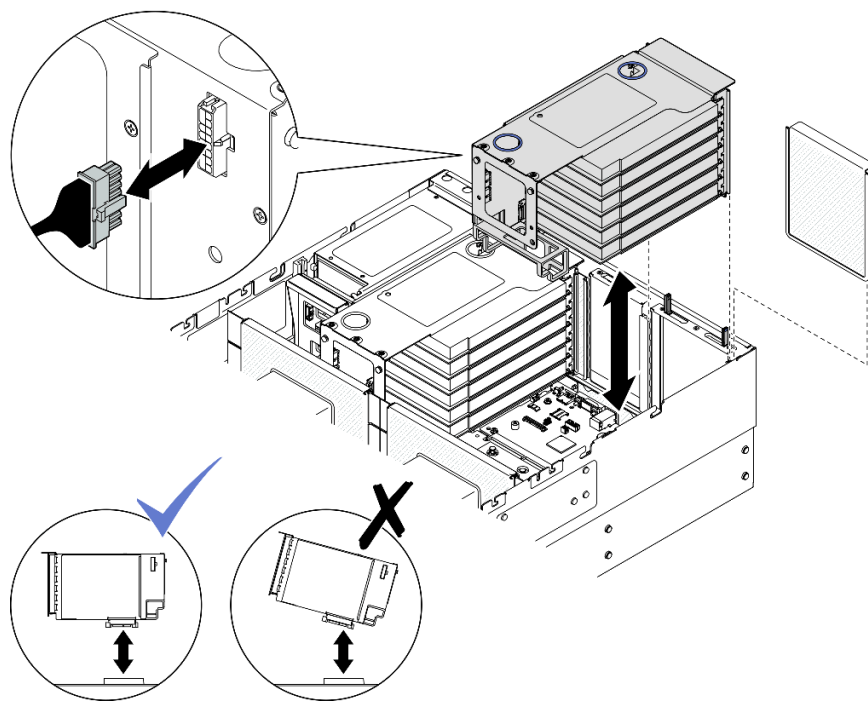
圖例 135. 安裝 PCIe 擴充卡 1
