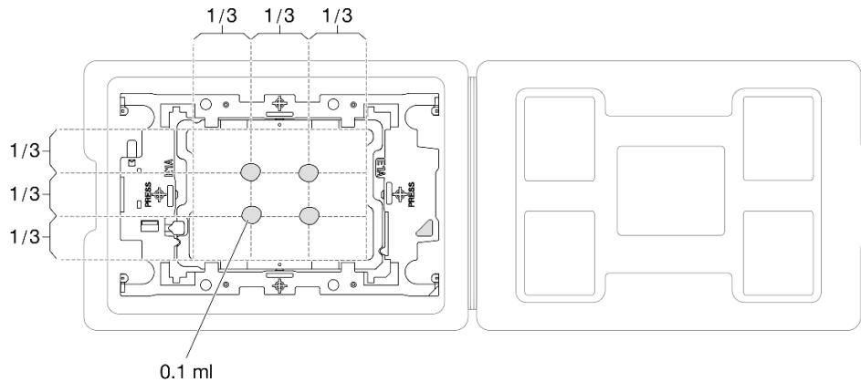
圖例 200. 運送匣中的處理器塗上散熱膏
