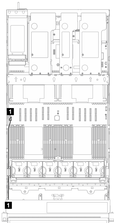
圖例 230. 正面 VGA 組件的纜線佈線
