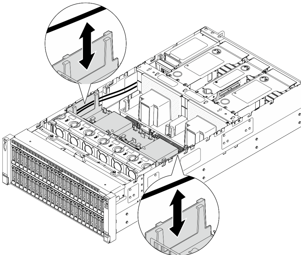
圖例 41. 將纜線從前方空氣擋板中取出
