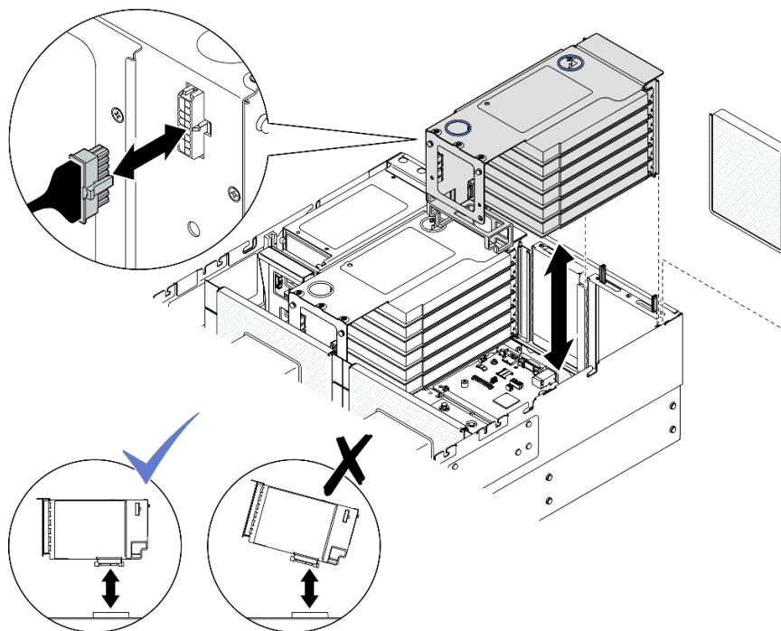
圖例 126. 卸下 PCIe 擴充卡 1
