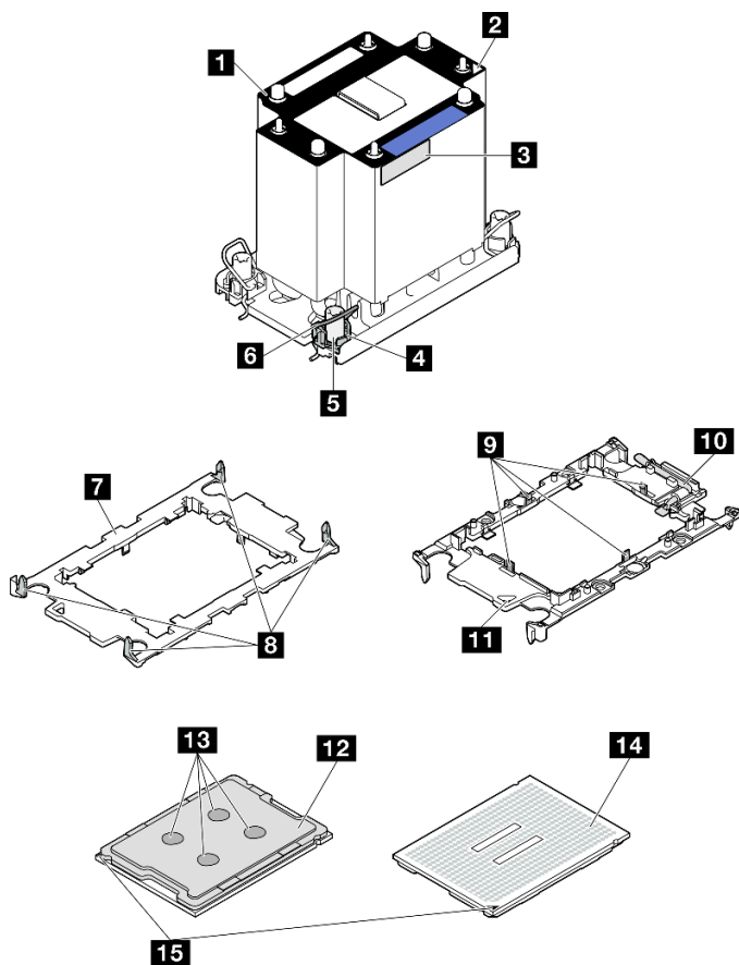
圖例 193. PHM 元件
