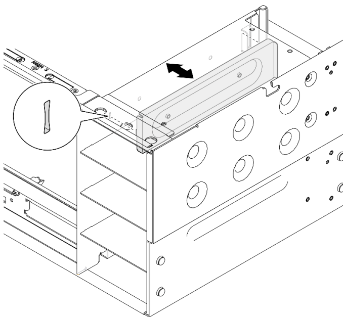
圖例 184. 卸下電源供應器托架
