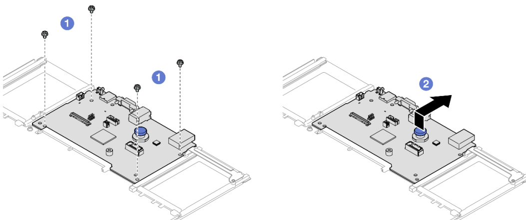
圖例 247. 將系統 I/O 板與處理器板分開
