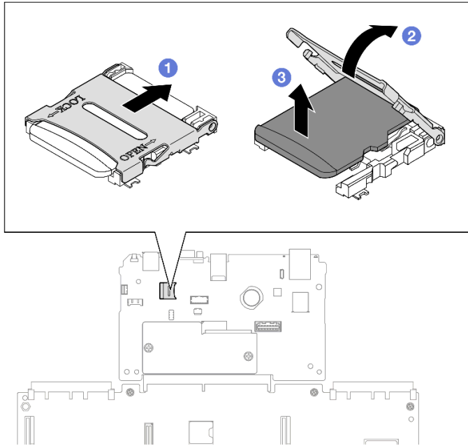
圖例 118. 卸下 MicroSD 卡
