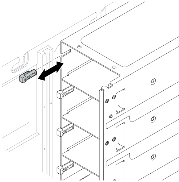
圖例 188. 卸下電源供應器鑰匙
