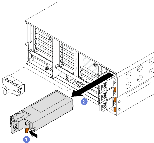
圖例 191. 卸下電源供應器
