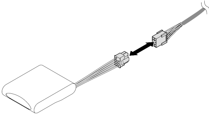
圖例 38. 從快閃記憶體電源模組拔掉纜線
