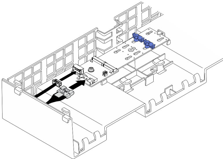
圖例 108. 將纜線連接到 SATA/x4 NVMe M.2 開機配接卡
