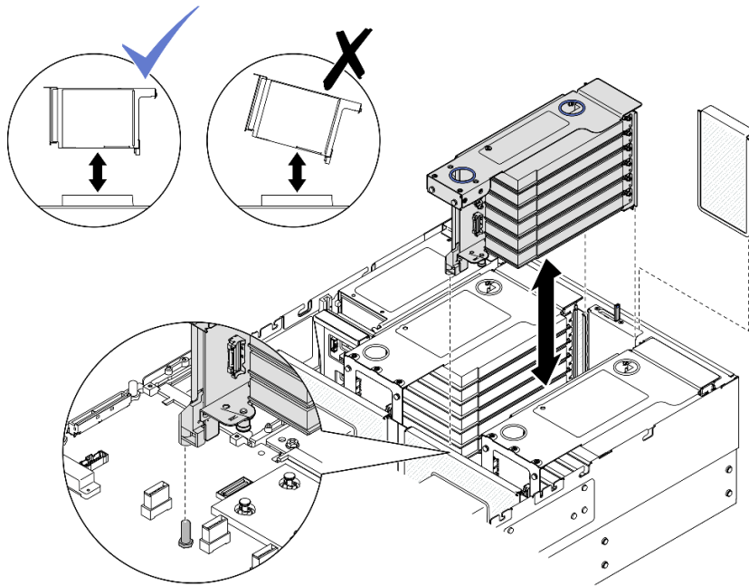
圖例 123. 卸下 PCIe 擴充卡 2
