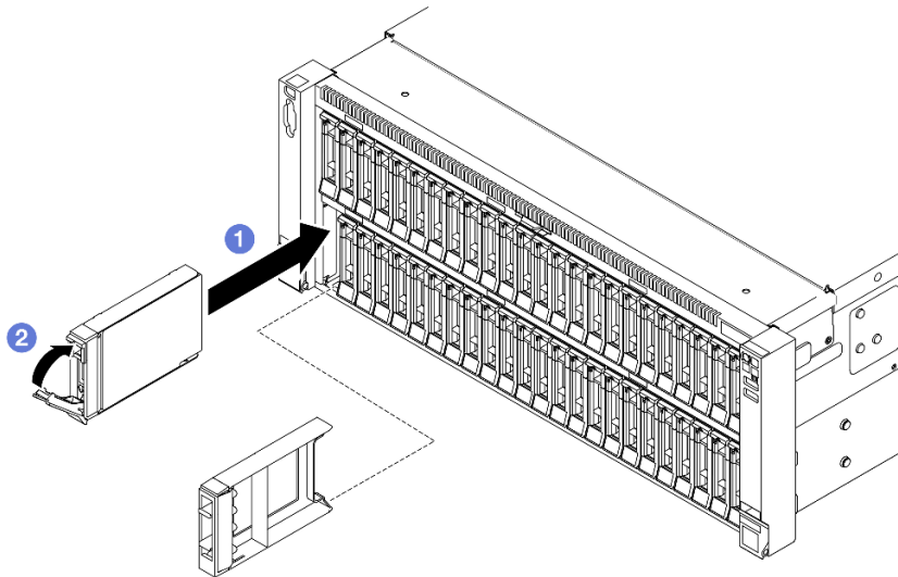
圖例 72. 安裝 2.5 吋硬碟
