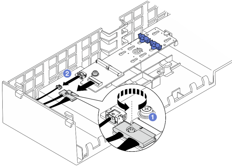
圖例 107. 從 SATA/NVMe 或 NVMe M.2 開機配接卡拔下纜線
