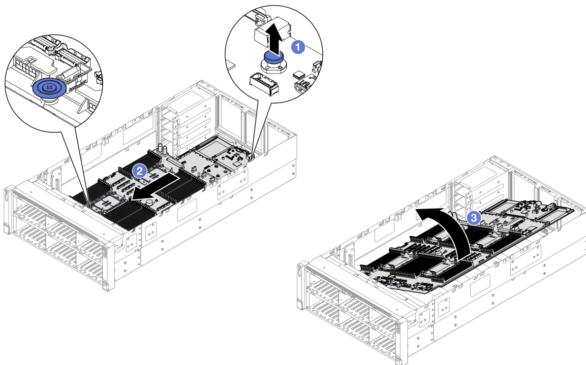
圖例 213. 卸下主機板組件
