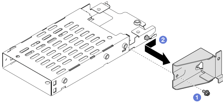
圖例 21. 卸下 7 公釐框架托架
