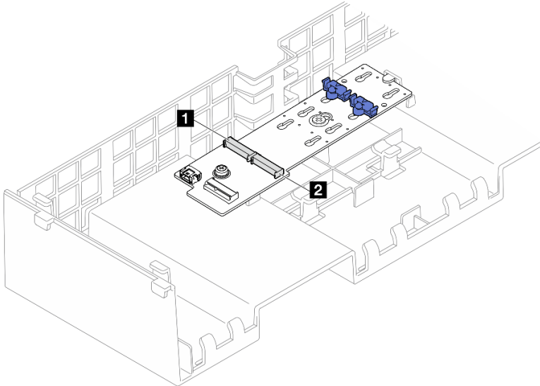
圖例 112. M.2 硬碟插槽
