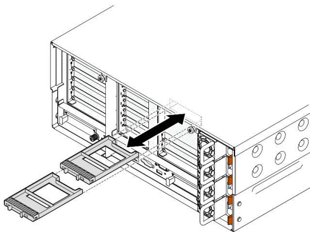
圖例 36. 卸下 7 公釐硬碟填充板
