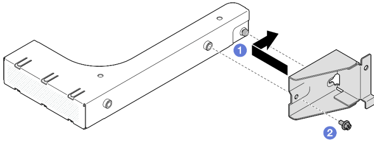
圖例 23. 安裝 7 公釐框架托架
