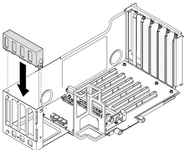
圖例 93. 安裝擴充卡延伸器蓋板
