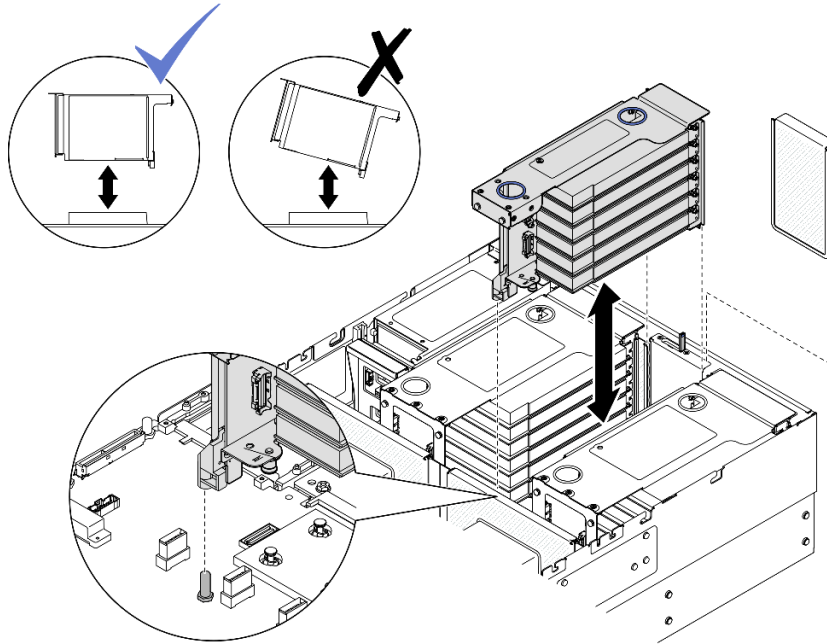
圖例 139. 安裝 PCIe 擴充卡 2
