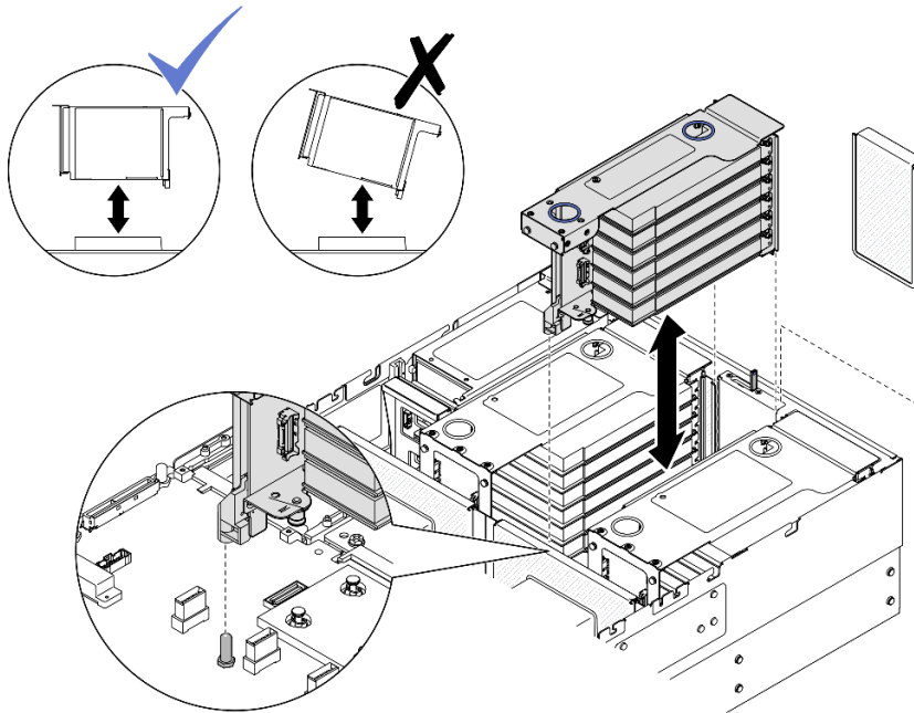
圖例 136. 安裝 PCIe 擴充卡 2
