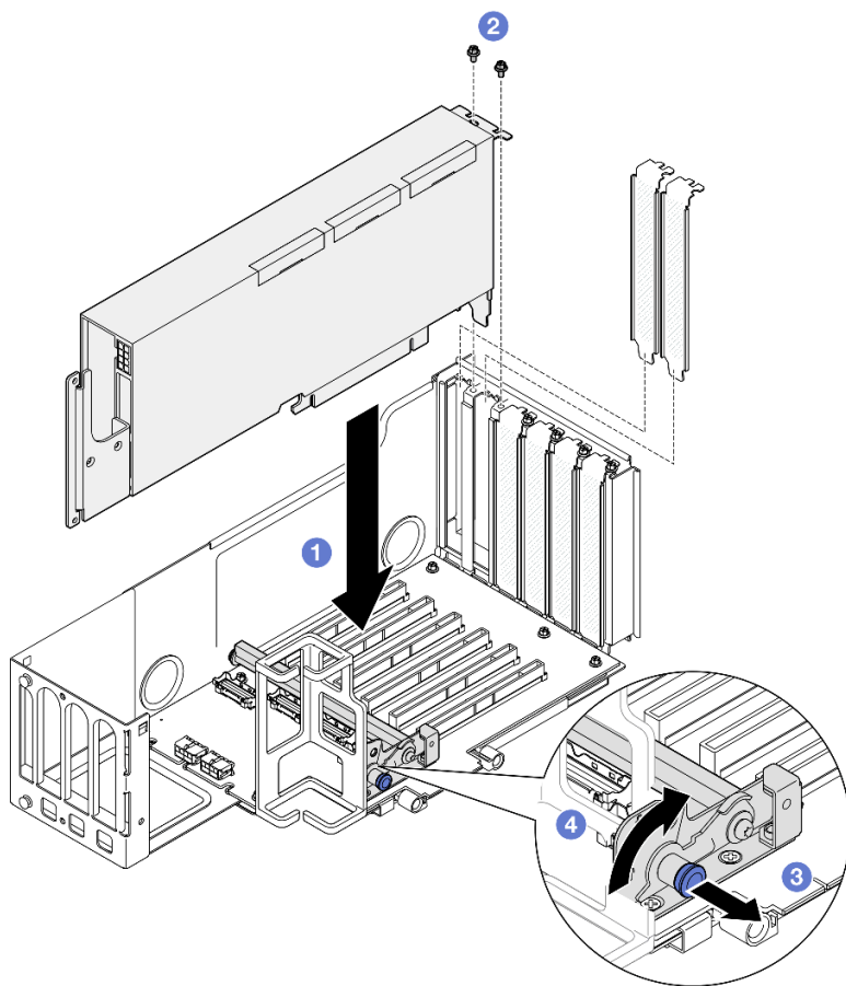
圖例 95. 將 GPU 配接卡安裝到 PCIe 擴充卡
