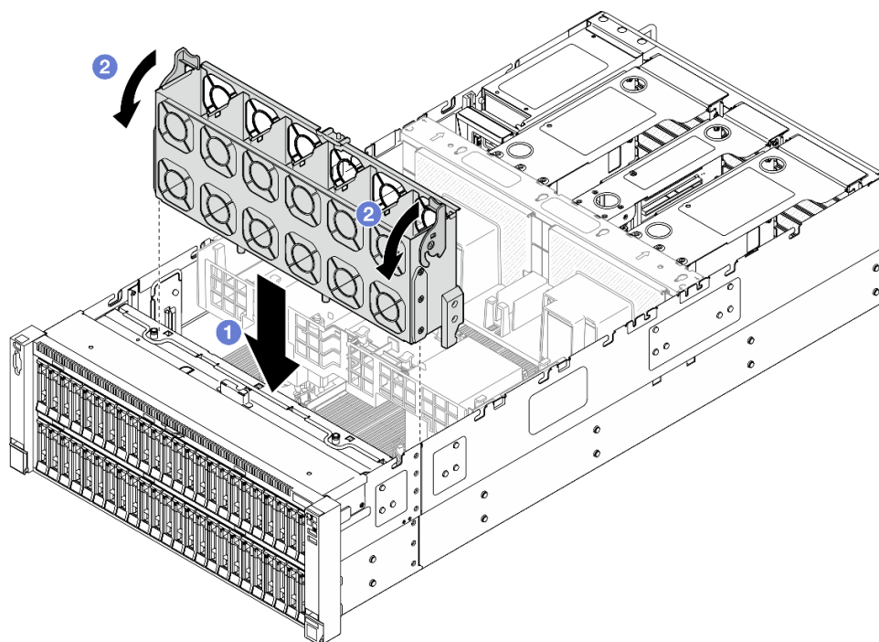
圖例 82. 安裝風扇機盒
