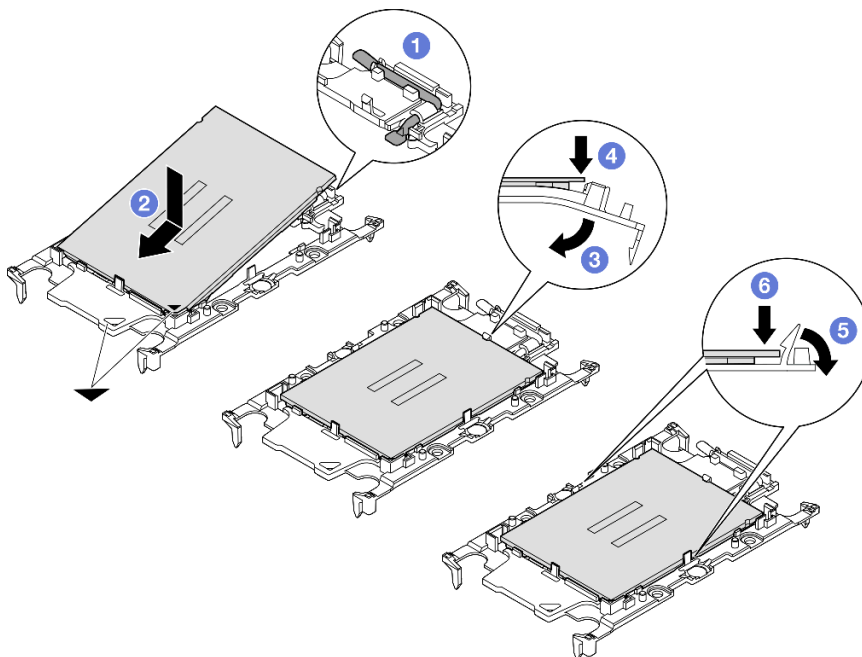
圖例 199. 安裝處理器支架
