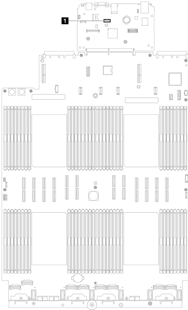
圖例 204. 拔下序列埠模組
