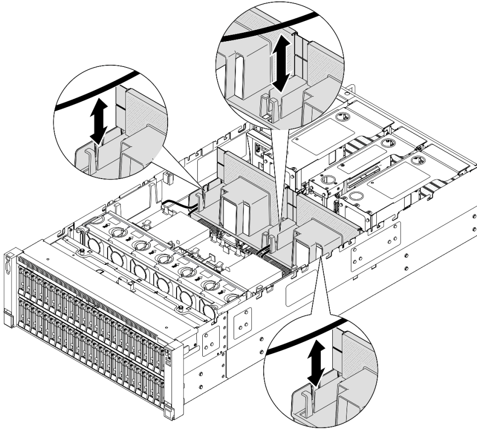
圖例 56. 將纜線穿過後方空氣擋板
