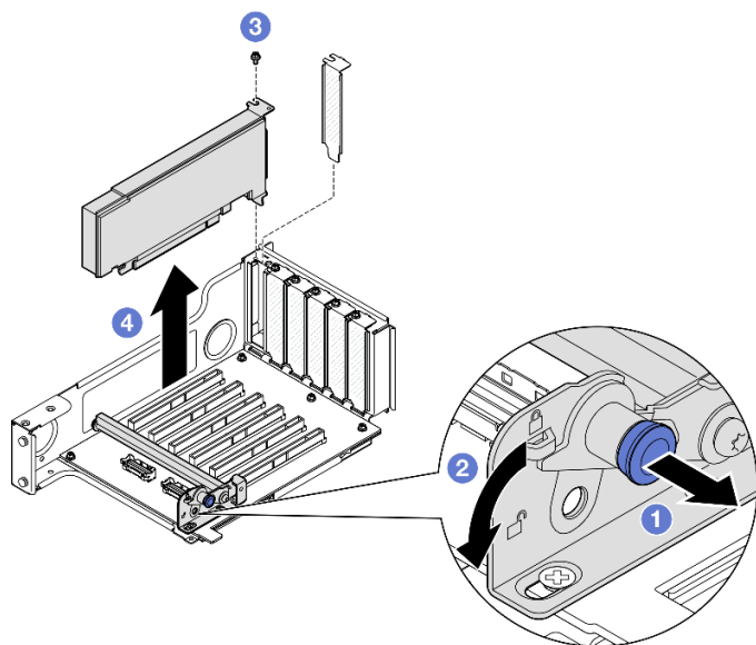
圖例 130. 從擴充卡卸下 PCIe 配接卡
