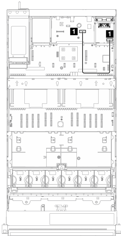
圖例 234. 管理 NIC 配接卡的纜線佈線
