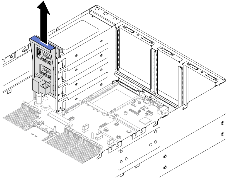
圖例 179. 卸下電源配送板
