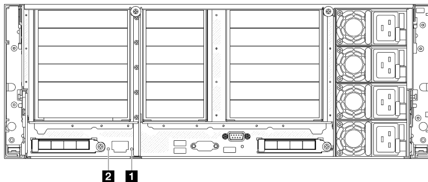
圖例 241. 背面系統 LED
