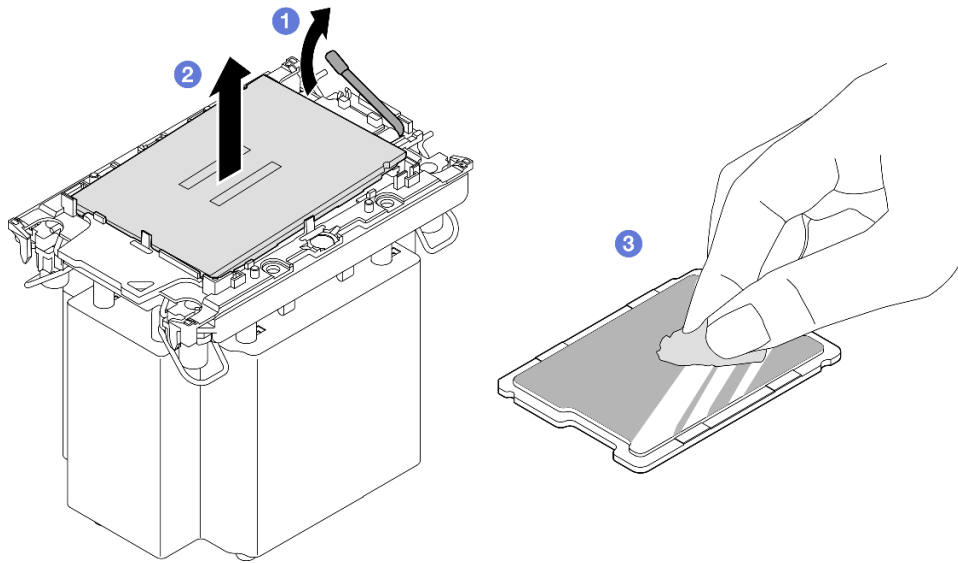
圖例 196. 將處理器與散熱槽和支架分開
