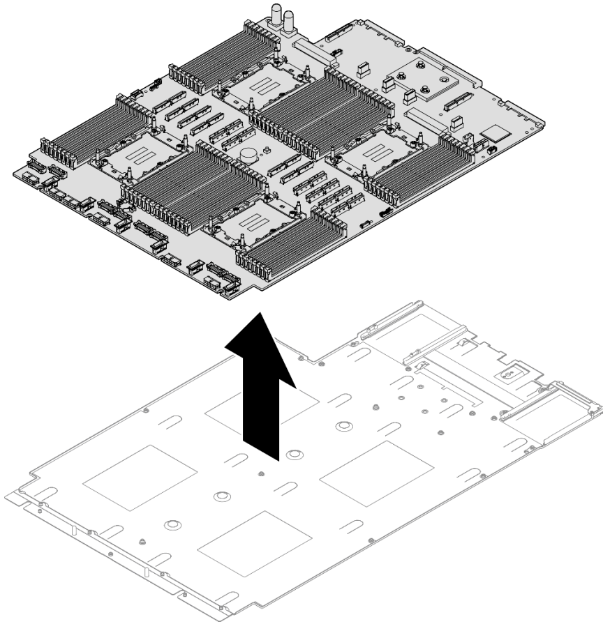
圖例 250. 拆卸處理器板
