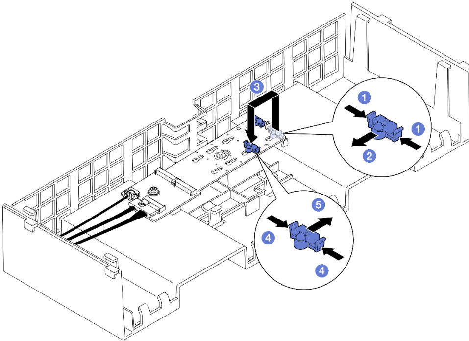
圖例 111. 調整 M.2 固定器
