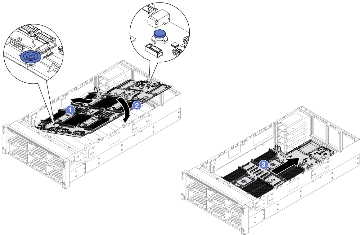
圖例 216. 安裝主機板組件
