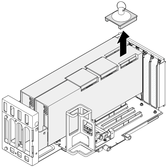
圖例 88. 卸下 GPU 配接卡鏈結橋接器
