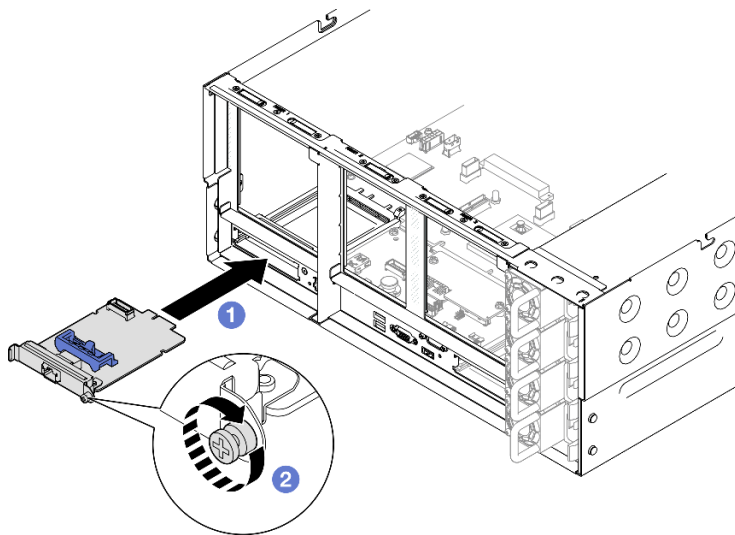
圖例 115. 安裝管理 NIC 配接卡
