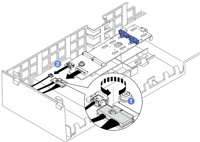
圖例 40. 從 SATA/NVMe 或 NVMe M.2 開機配接卡拔下纜線
