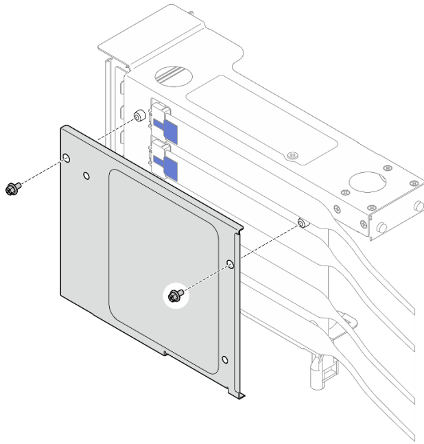
圖例 148. 從擴充卡卸下蓋板
