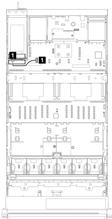
圖例 236. 電源配送板的側頻纜線佈線
