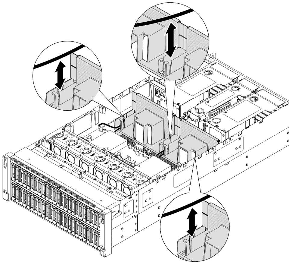
圖例 51. 將纜線從後方空氣擋板中取出
