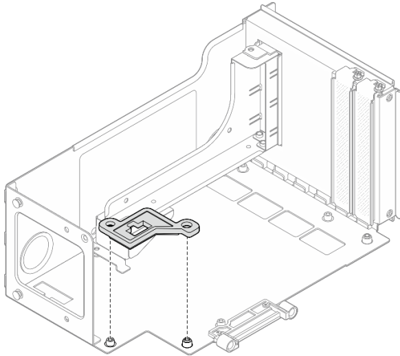
圖例 153. 將接頭導件安裝到擴充卡
