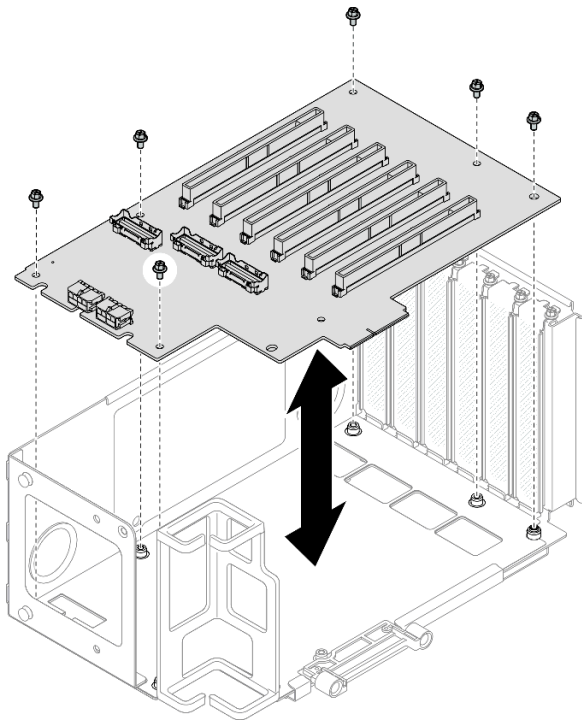
圖例 158. 將 PCIe 擴充卡安裝到擴充卡
