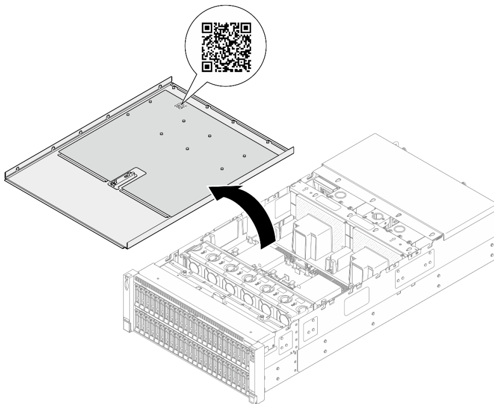
圖例 16. 服務標籤和 QR 代碼
