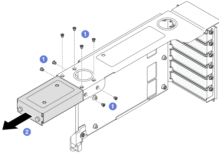
圖例 173. 從 HH PCIe 擴充卡卸下 PCIe 擴充卡延伸器
