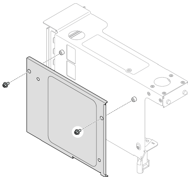
圖例 169. 從擴充卡卸下蓋板
