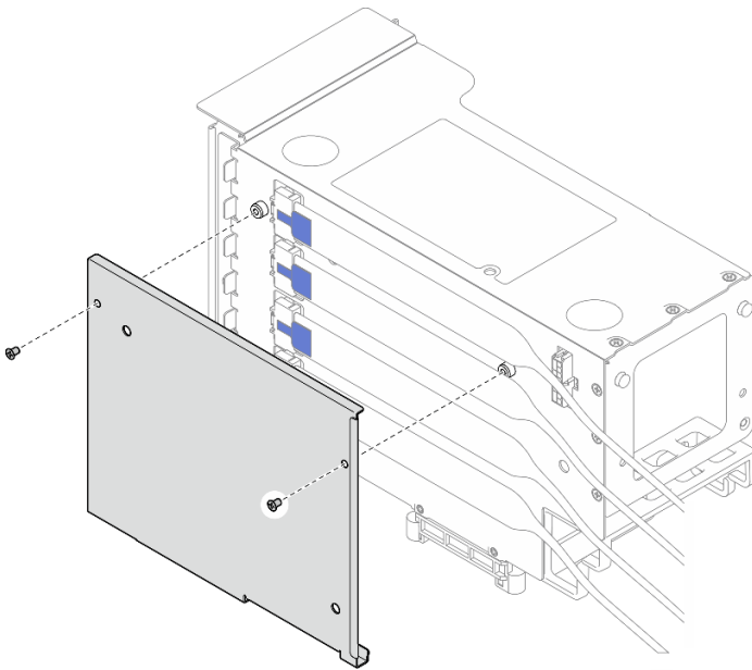
圖例 163. 將蓋板安裝到擴充卡
