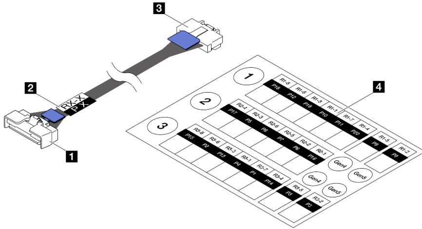
圖例 164. PCIe 擴充卡纜線
