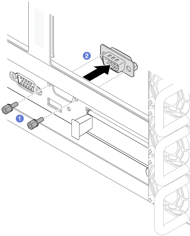
圖例 205. 卸下序列埠模組
