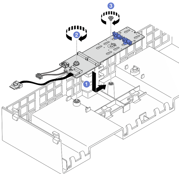
圖例 110. 安裝 M.2 開機配接卡
