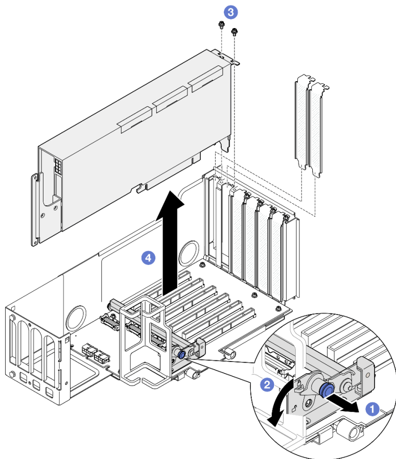
圖例 92. 從 PCIe 擴充卡卸下 GPU 配接卡
