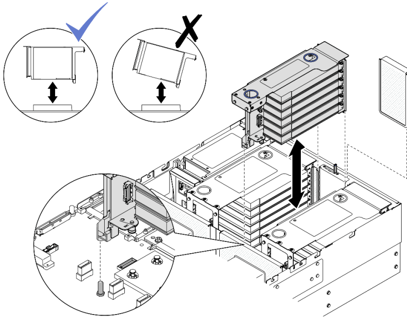
圖例 138. 安裝 PCIe 擴充卡 2
