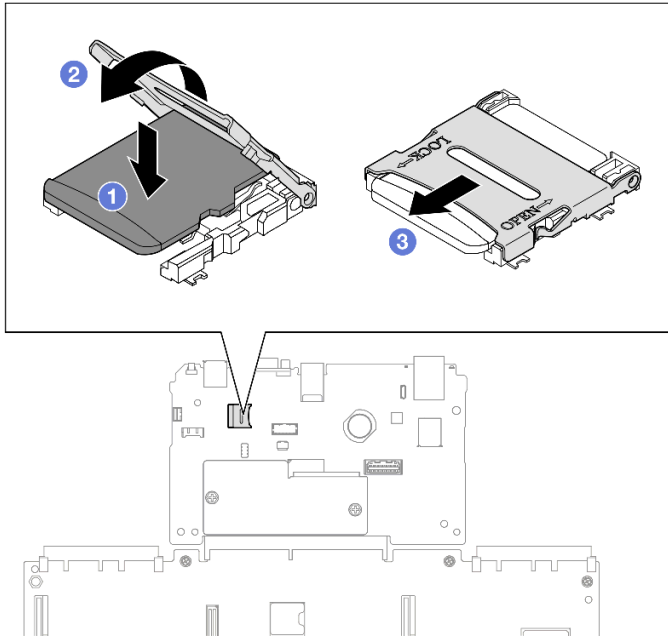
圖例 119. 安裝 MicroSD 卡
