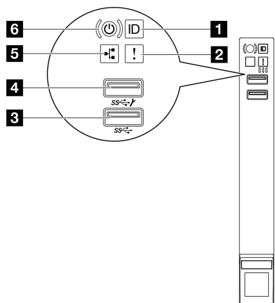
圖例 9. 正面 I/O 模組
