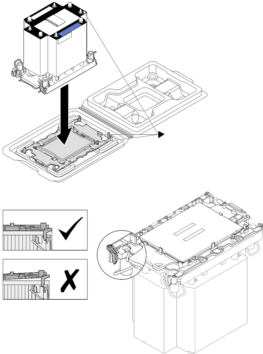
圖例 201. 將 PHM 和處理器裝到運送匣中
