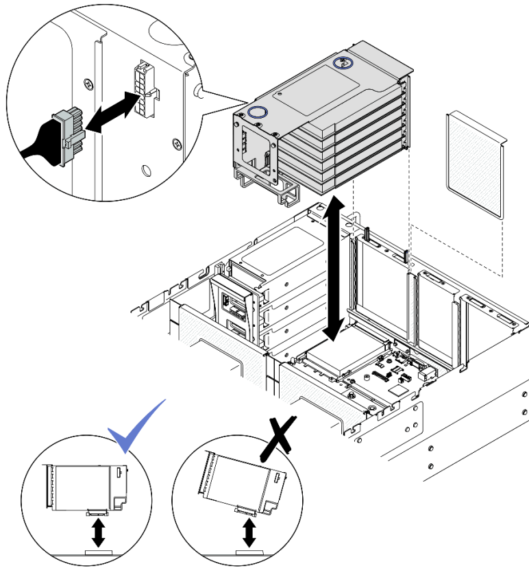
圖例 127. 卸下 PCIe 擴充卡 3
