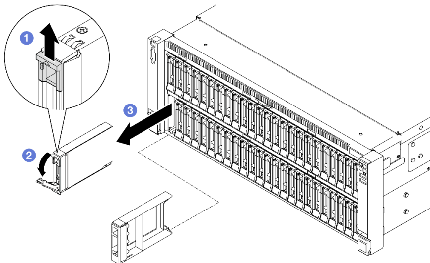
圖例 71. 卸下 2.5 吋硬碟
