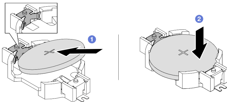
圖例 64. CMOS 電池安裝
