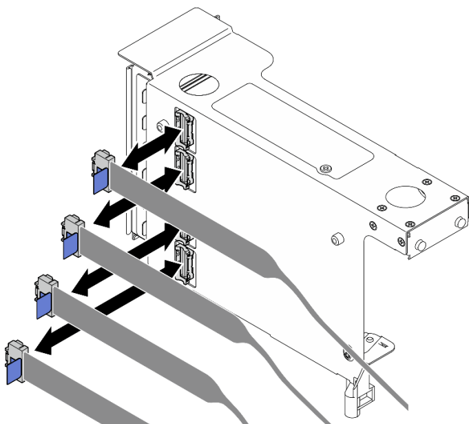
圖例 149. 從擴充卡外部拔下 PCIe 纜線
