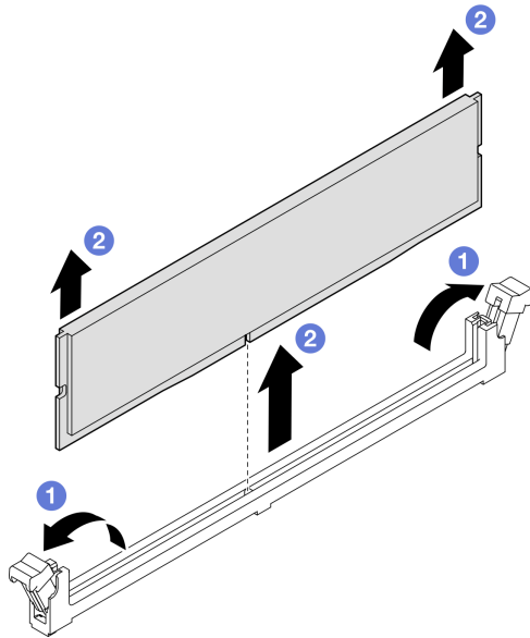
圖例 116. 卸下記憶體模組
