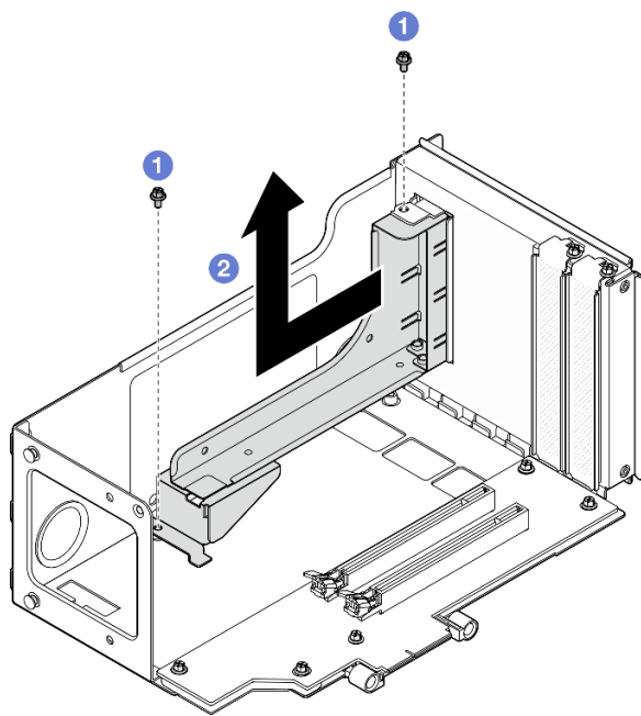
圖例 29. 卸下 7 公釐框架填充板
