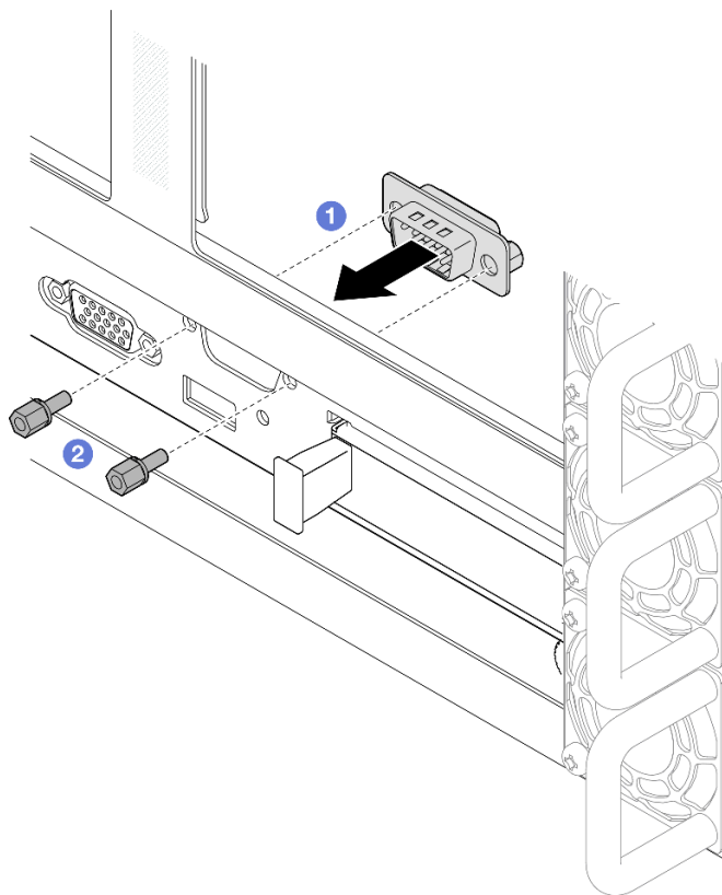
圖例 208. 安裝序列埠模組
