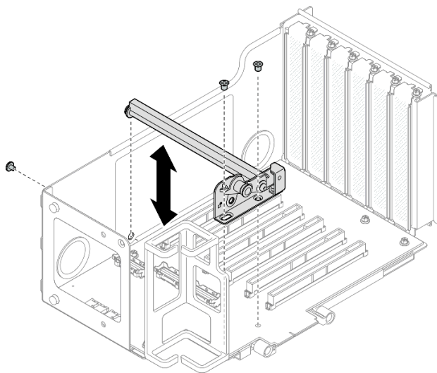
圖例 145. 從擴充卡卸下 PCIe 固定器
