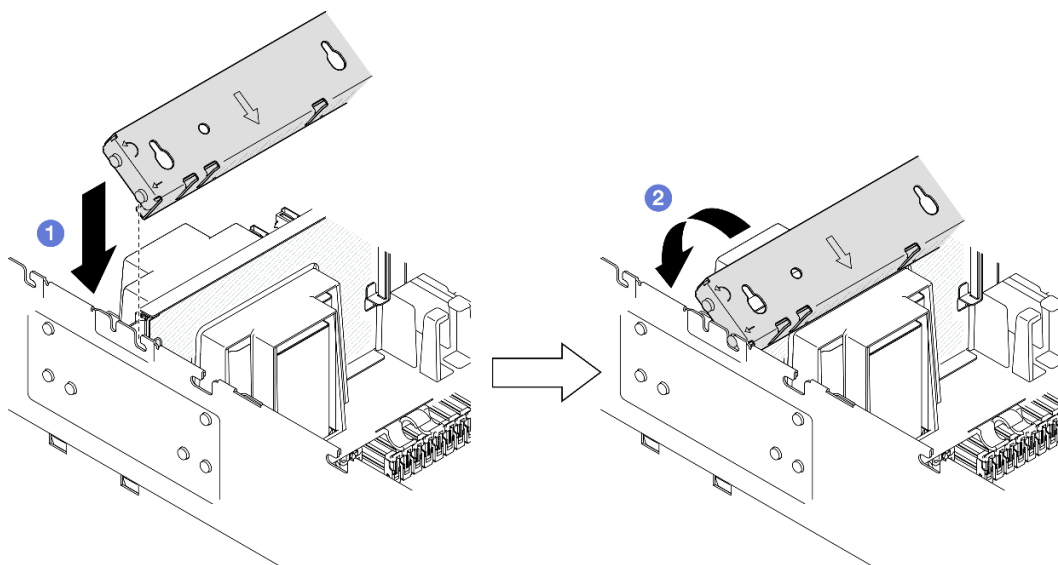
圖例 69. 安裝橫槓
