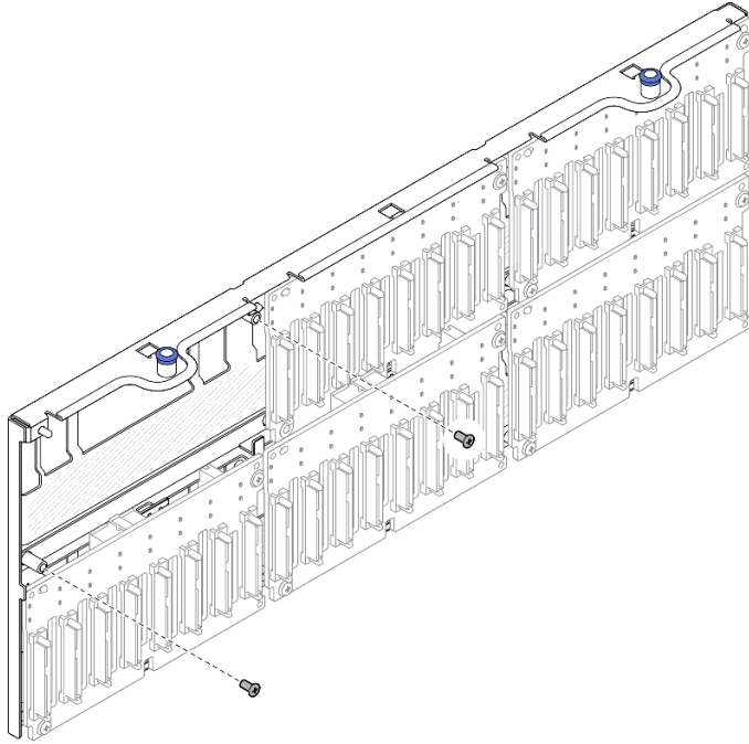
圖例 75. 背板支架上的備用螺絲
