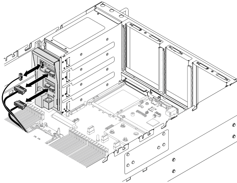
圖例 178. 拔掉電源配送板纜線
