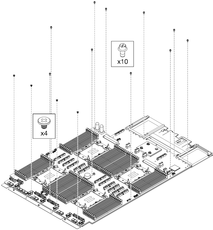
圖例 249. 卸下螺絲
