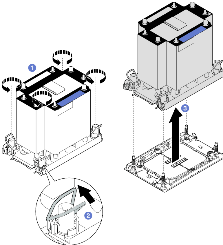
圖例 194. 卸下 3U 標準 PHM
