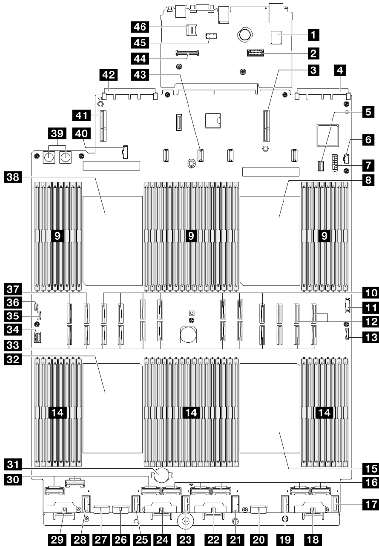
圖例 11. 主機板組件接頭
