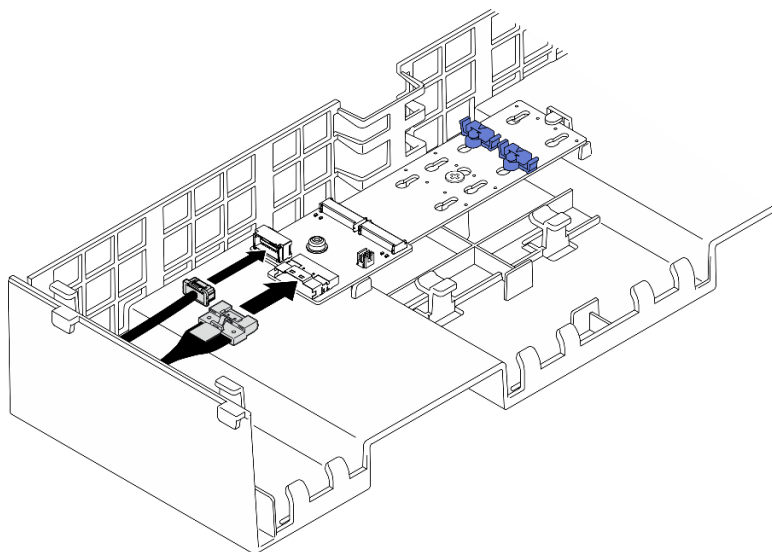
圖例 45. 將纜線連接到 SATA/x4 NVMe M.2 開機配接卡
