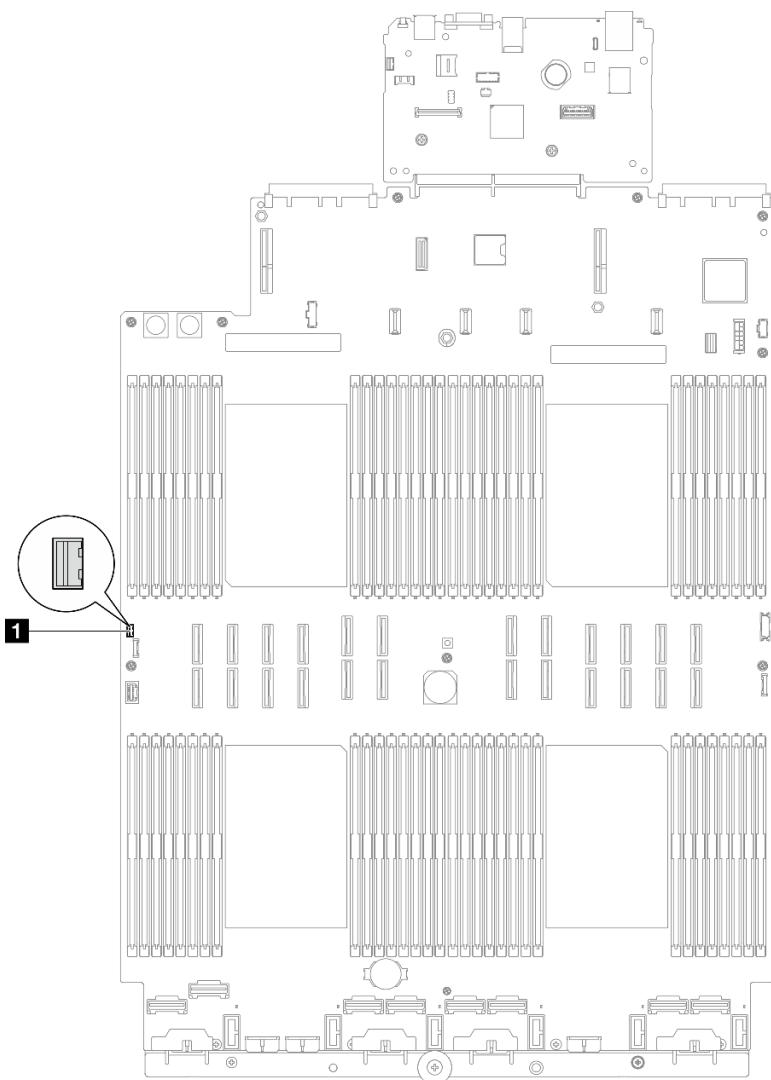
圖例 103. 連接入侵開關
