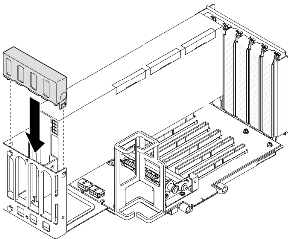
圖例 97. 安裝擴充卡延伸器蓋板
