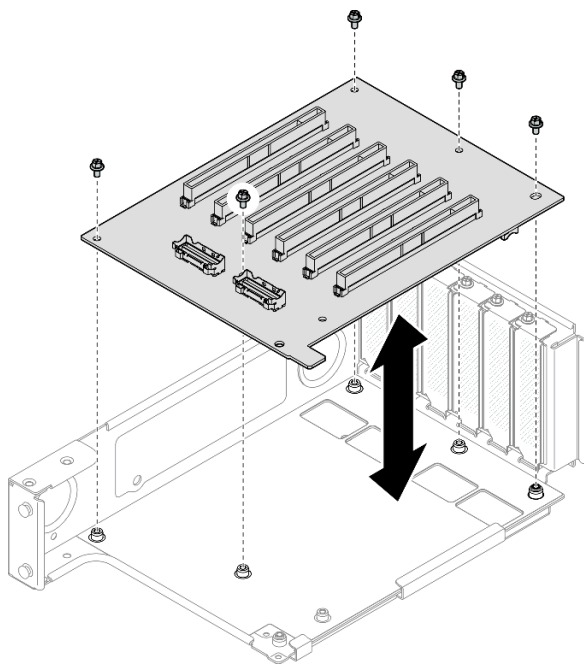
圖例 152. 從擴充卡卸下 PCIe 擴充卡
