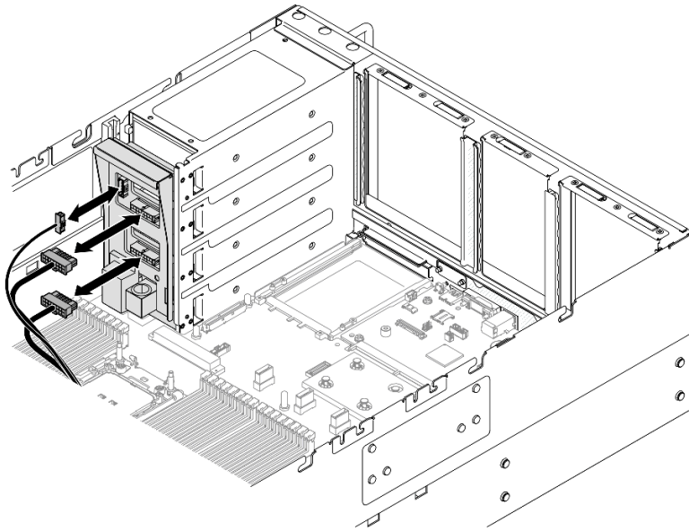
圖例 182. 連接電源配送板纜線
