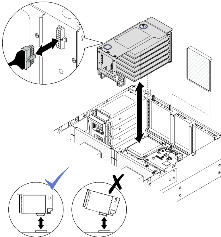
圖例 134. 安裝 PCIe 擴充卡 3
