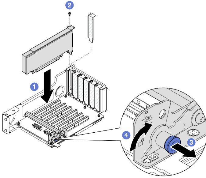
圖例 133. 將 PCIe 配接卡安裝到擴充卡
