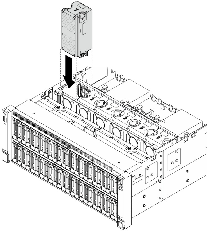
圖例 83. 安裝風扇模組
