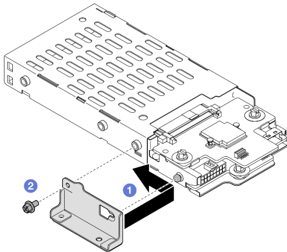
圖例 34. 安裝 7 公釐框架托架
