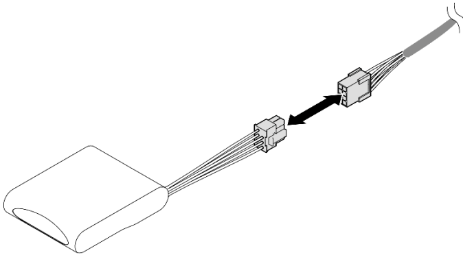
圖例 84. 從快閃記憶體電源模組拔掉纜線
