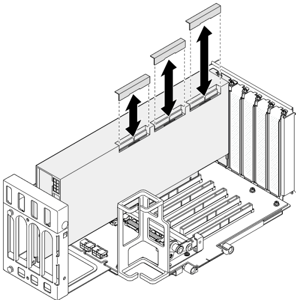
圖例 89. 將鏈結接頭蓋板安裝到 GPU 上
