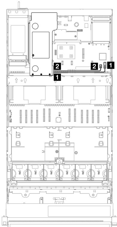
圖例 227. 7 公釐硬碟背板的纜線佈線
