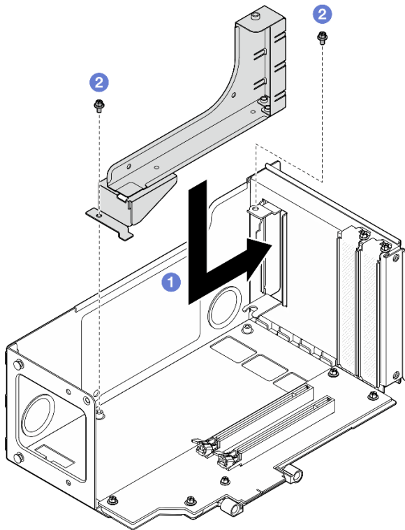
圖例 24. 安裝 7 公釐框架填充板
