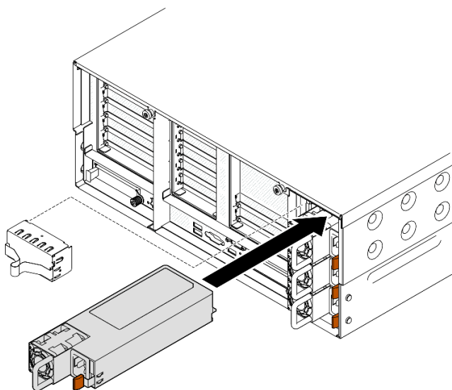
圖例 192. 安裝電源供應器
