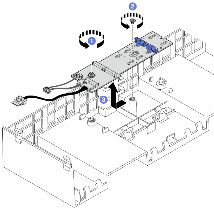
圖例 105. 卸下 M.2 開機配接卡
