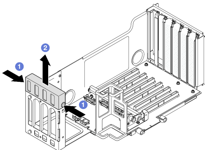
圖例 94. 卸下擴充卡延伸器蓋板
