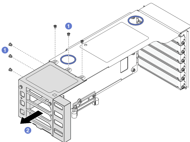
圖例 172. 從 FH PCIe 擴充卡卸下 PCIe 擴充卡延伸器
