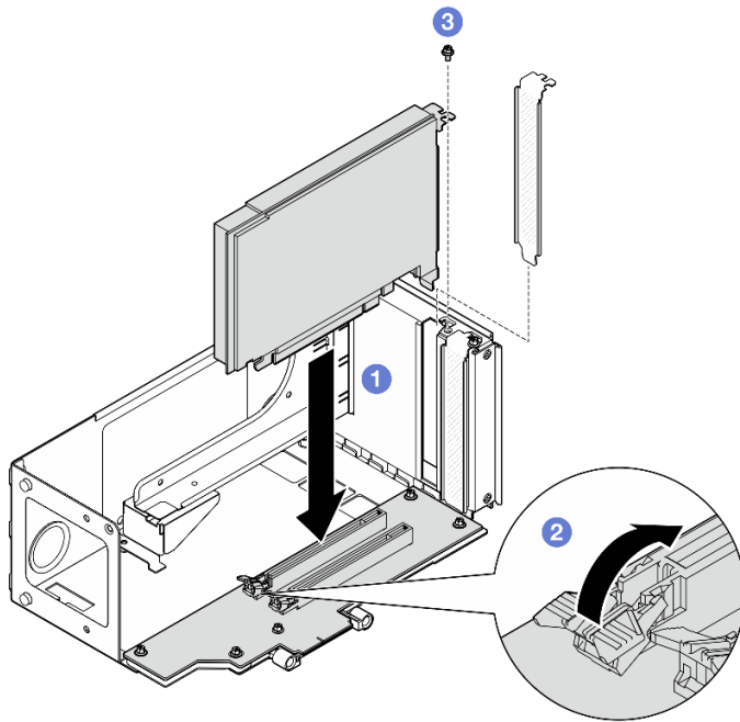
圖例 131. 將 PCIe 配接卡安裝到擴充卡
