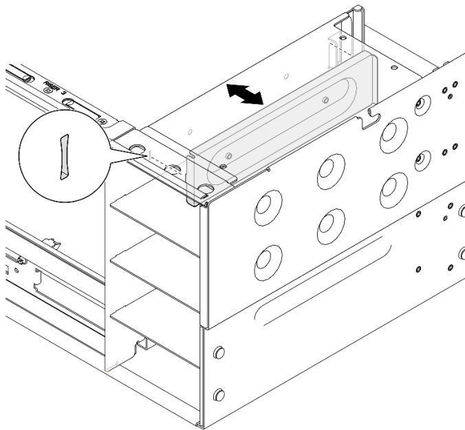
圖例 185. 安裝電源供應器托架
