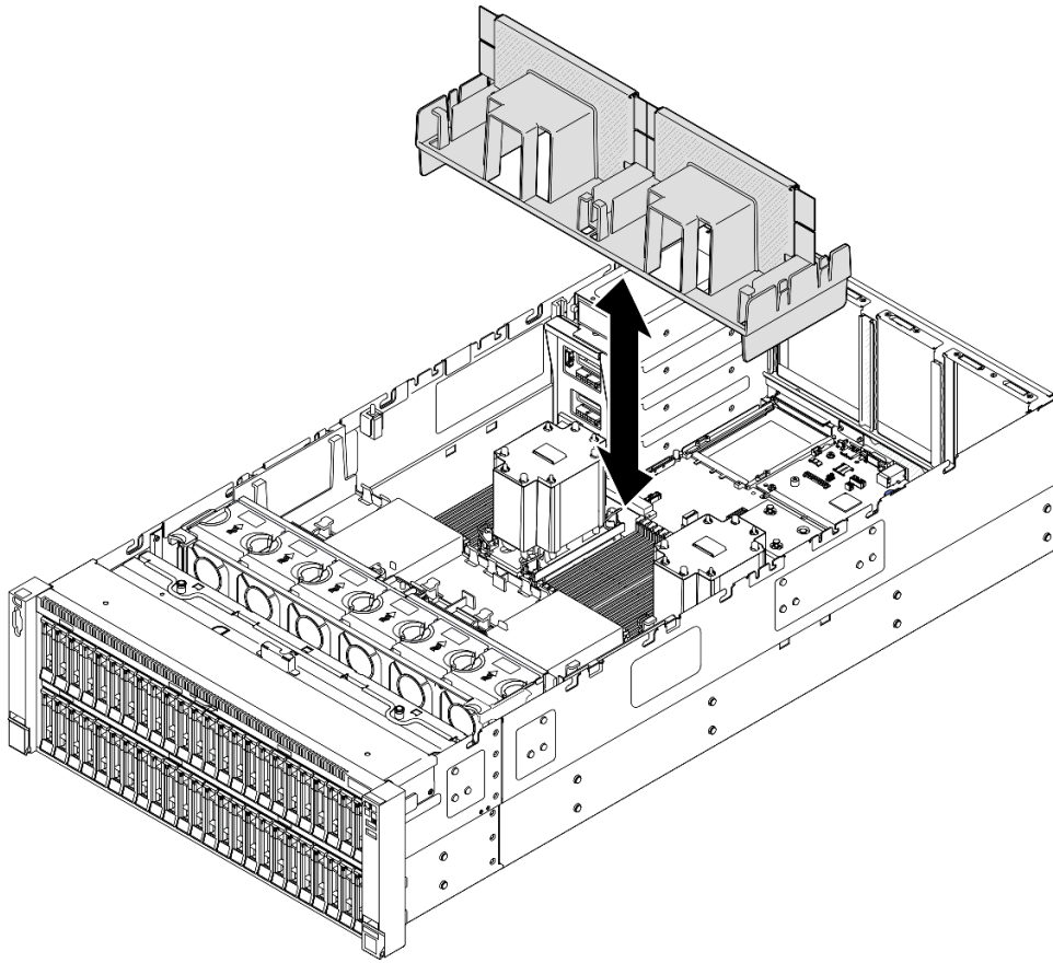
圖例 52. 為 3U 標準 PHM 卸下後方空氣擋板
