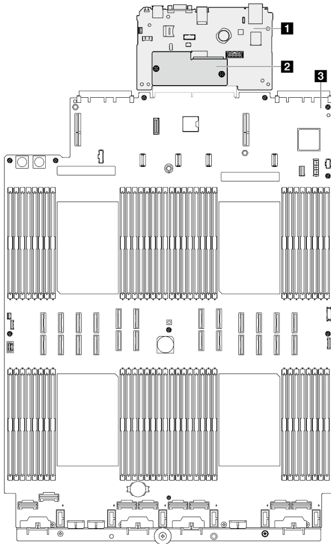
圖例 10. 主機板組件佈置
