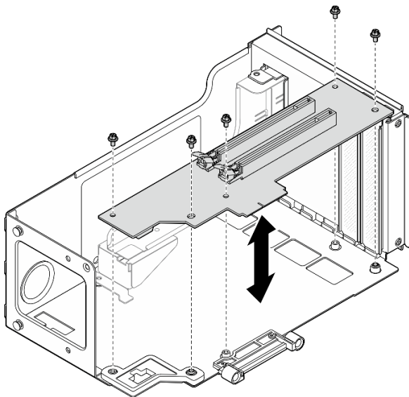
圖例 154. 將 PCIe 擴充卡安裝到擴充卡
