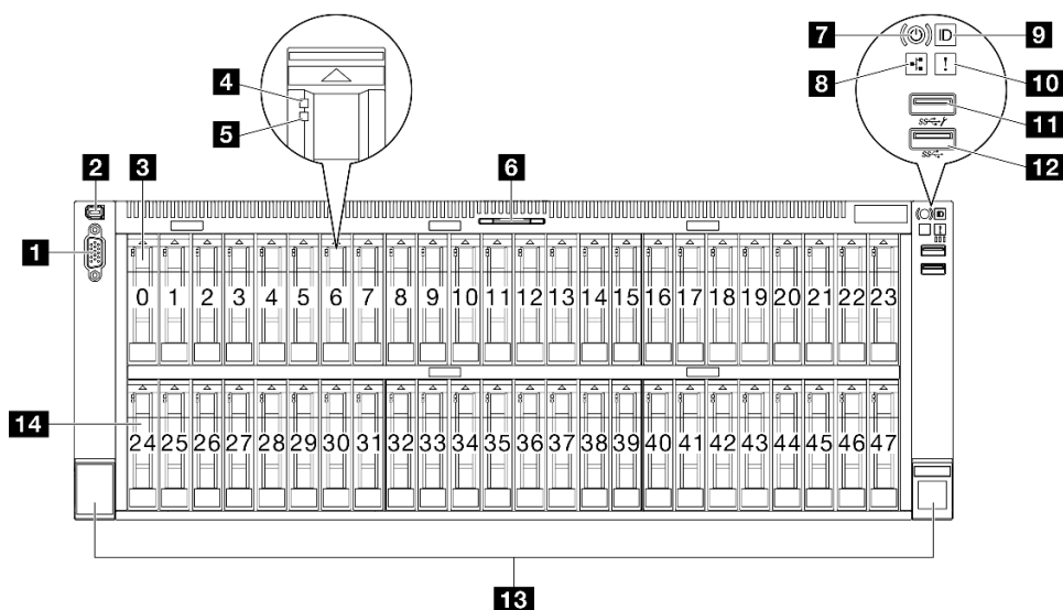
圖例 2. 2.5 吋硬碟配置的正面圖
