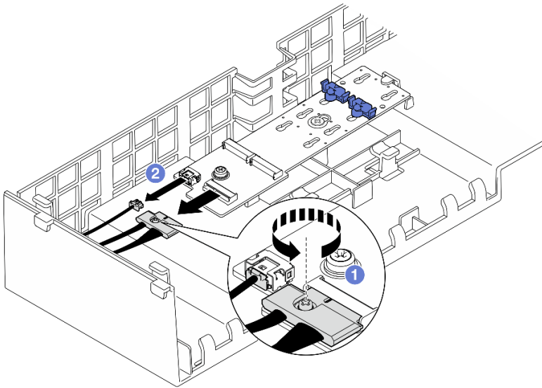
圖例 50. 從 SATA/NVMe 或 NVMe M.2 開機配接卡 拔下纜線
