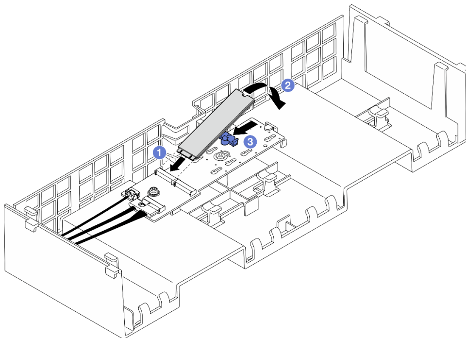
圖例 113. 安裝 M.2 硬碟
