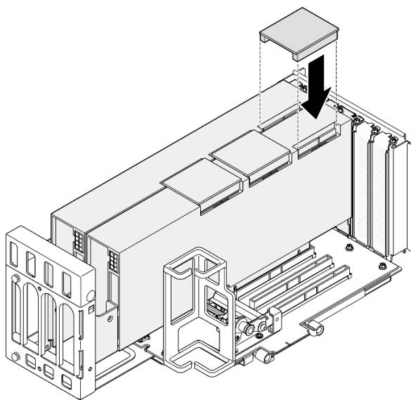
圖例 99. 安裝 GPU 配接卡鏈結橋接器
