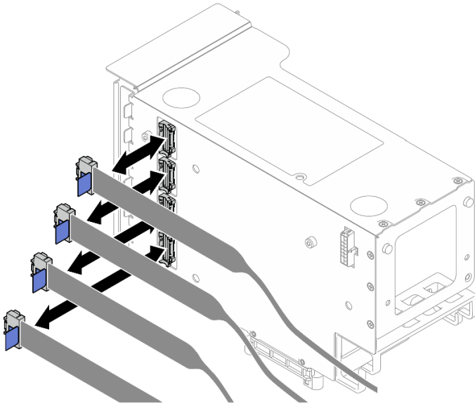
圖例 162. 將 PCIe 擴充卡纜線連接到擴充卡外部
