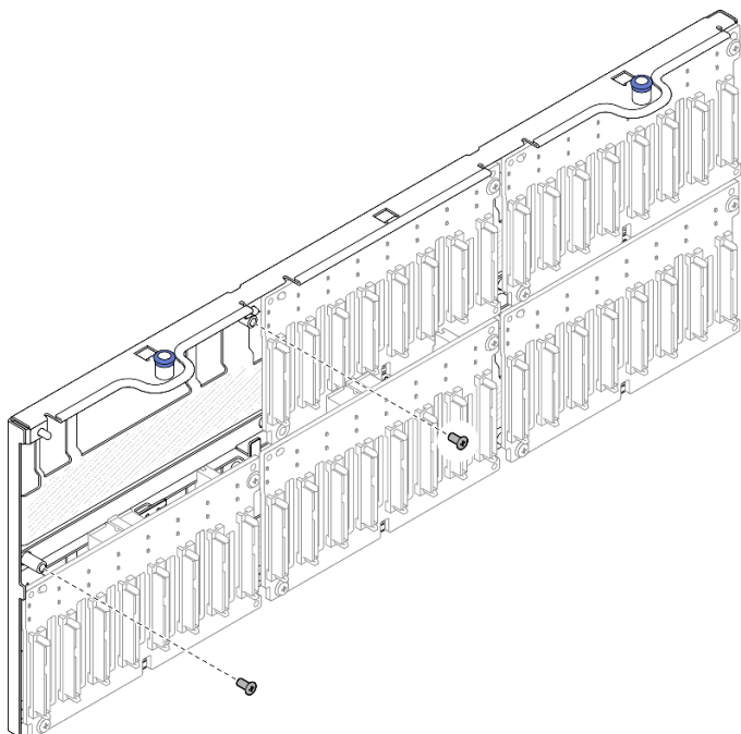
圖例 77. 背板支架上的備用螺絲
