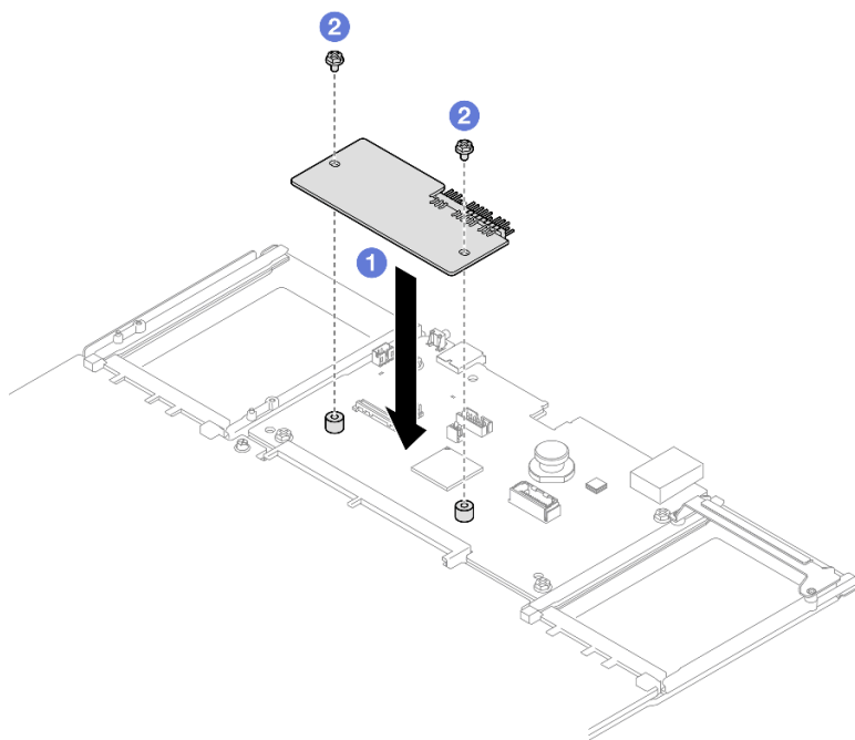
圖例 212. 安裝韌體和 RoT 安全模組
