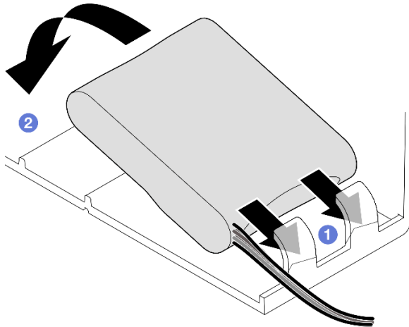
圖例 86. 快閃記憶體電源模組安裝
