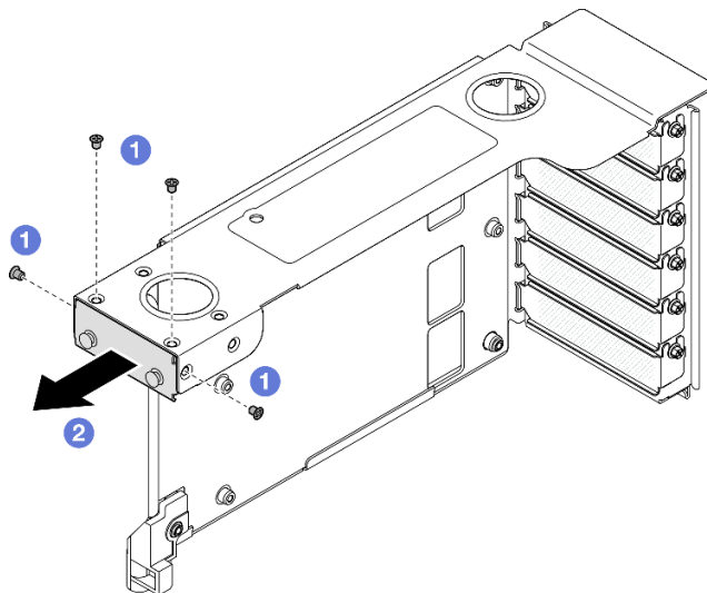
圖例 176. 從 FH PCIe 擴充卡卸下填充板
