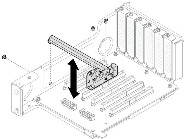
圖例 167. 將 PCIe 固定器安裝到擴充卡
