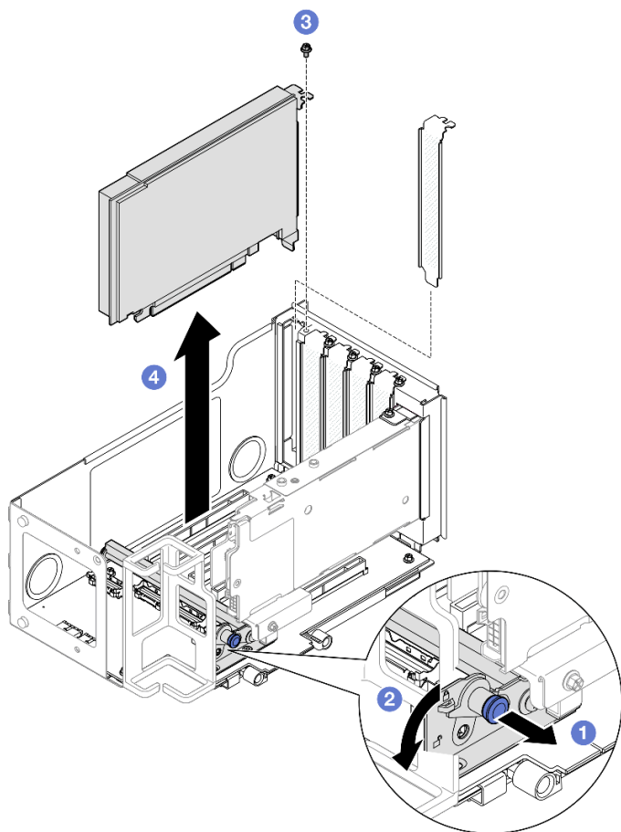
圖例 129. 從擴充卡卸下 PCIe 配接卡
