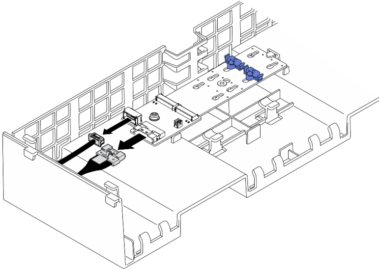
圖例 49. 從 SATA/x4 NVMe M.2 開機配接卡 拔下纜線
