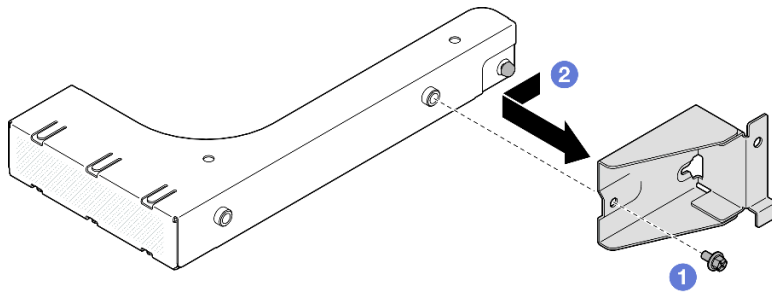
圖例 30. 卸下 7 公釐框架托架
