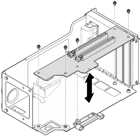
圖例 140. 從擴充卡卸下 PCIe 擴充卡
