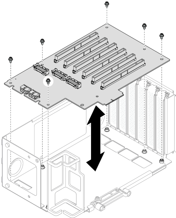
圖例 146. 從擴充卡卸下 PCIe 擴充卡
