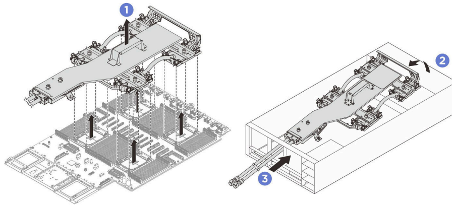
図 102. コールド・プレート・アセンブリの取り外し
