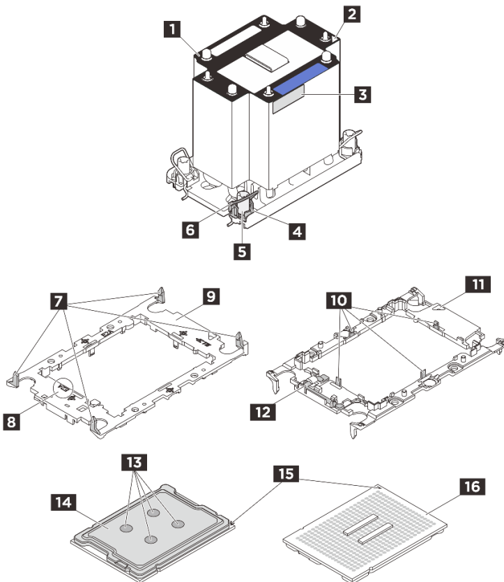
図 238. PHM コンポーネント
