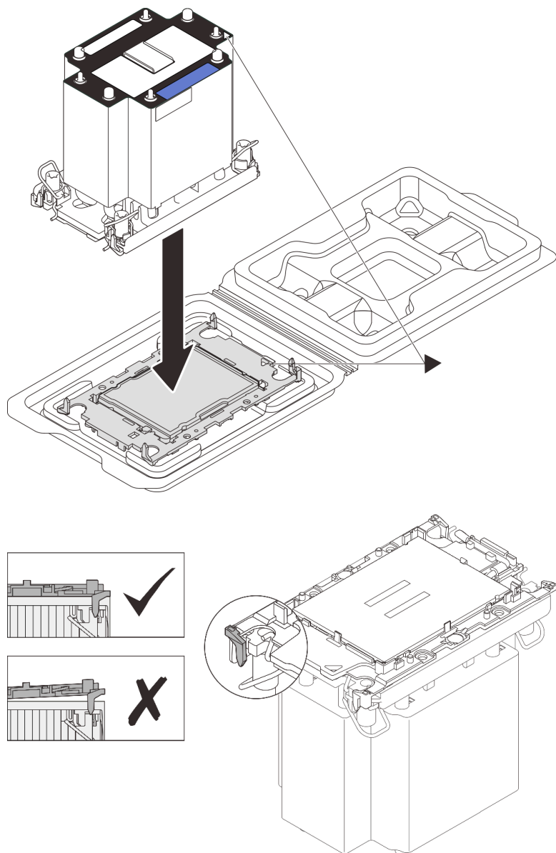
図 241. 配送用トレイのプロセッサーで PHM を取り付けます。
