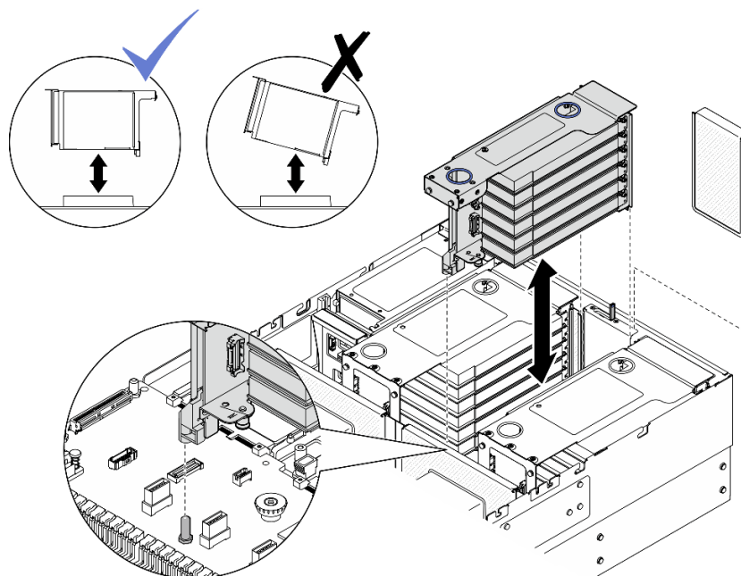
図 185. PCIe ライザー 2 の取り付け
