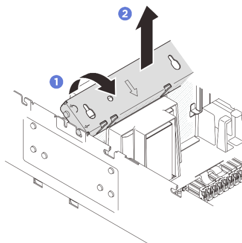
図 37. クロス・バーの取り外し
