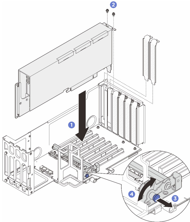
図 80. GPU アダプターの PCIe ライザーへの取り付け
