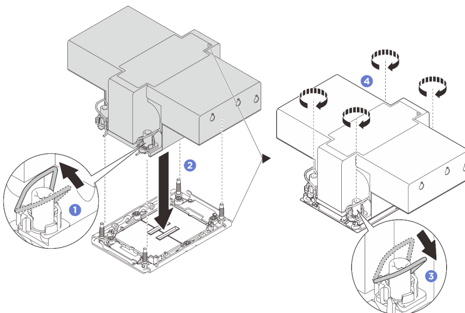
図 243. 2U パフォーマンス PHM の取り付け
