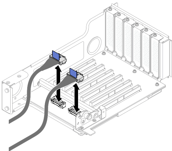
図 210. ライザーの内側への PCIe ライザー・ケーブルの接続
