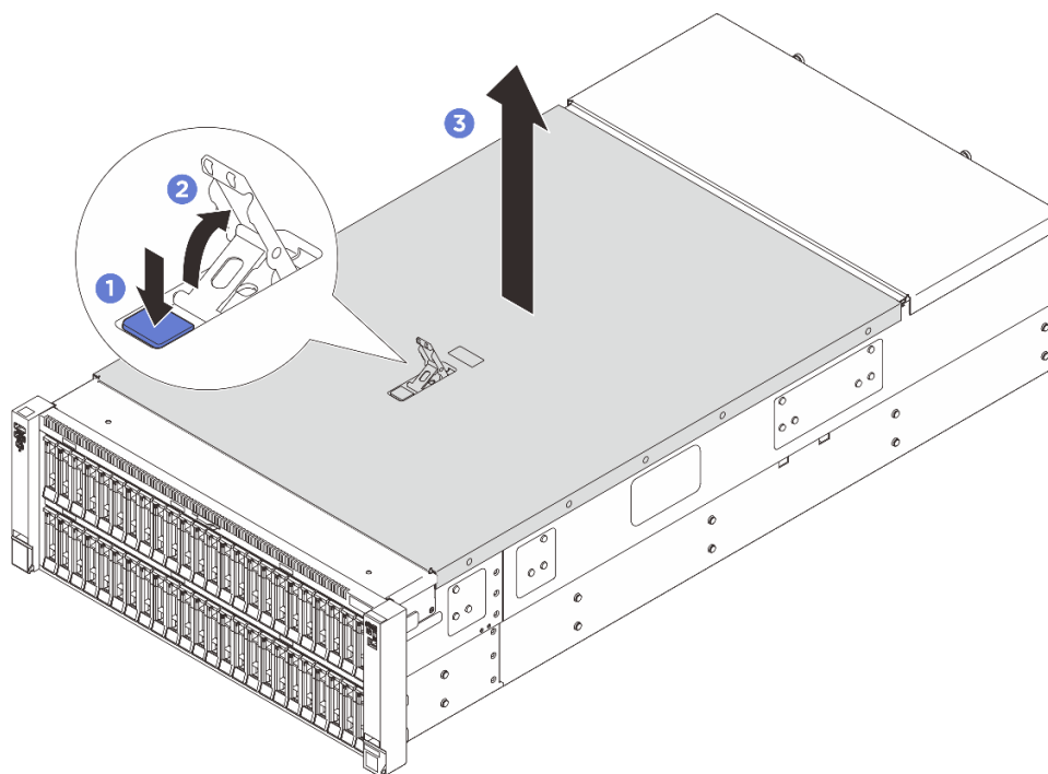
図295. 前面トップ・カバーの取り外し
