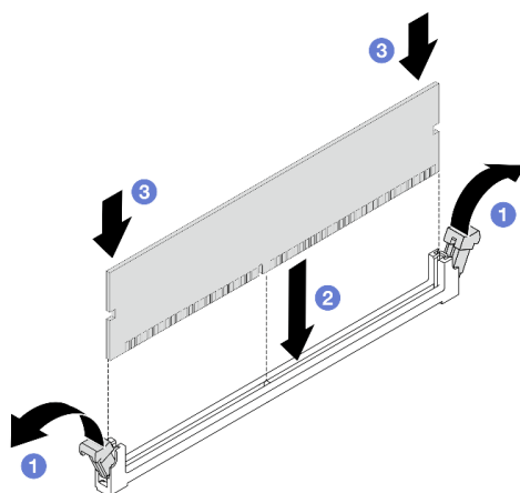
図 165. メモリー・モジュールの取り付け
