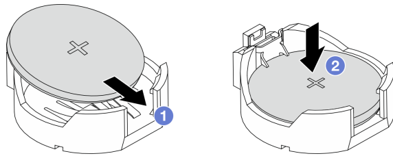
図 34. CMOS バッテリーの取り付け
