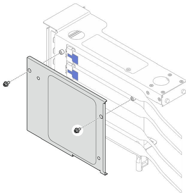
図 213. ライザー・ケージへのカバーの取り付け
