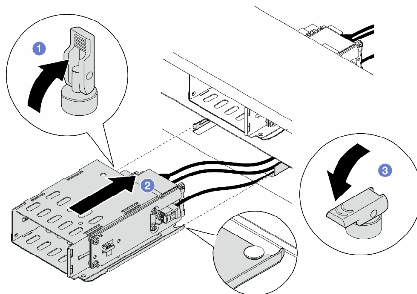
図 65. E3.S 2T ケージの取り付け
