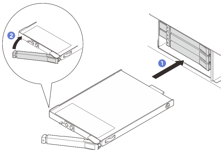
図45. E3.S ホット・スワップ・ドライブの取り付け
