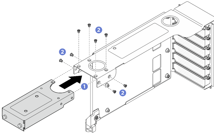
図 219. FH PCIe ライザーへの PCIe ライザー・エクステンダーの取り付け
