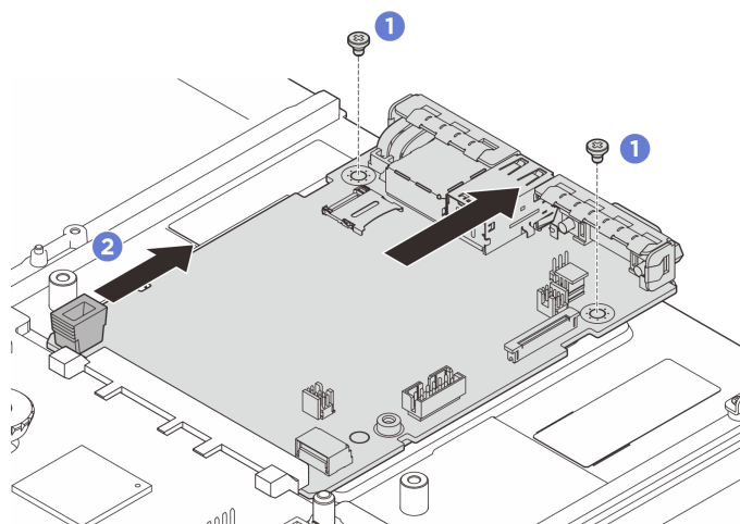
図 291. システム I/O ボードの取り外し
