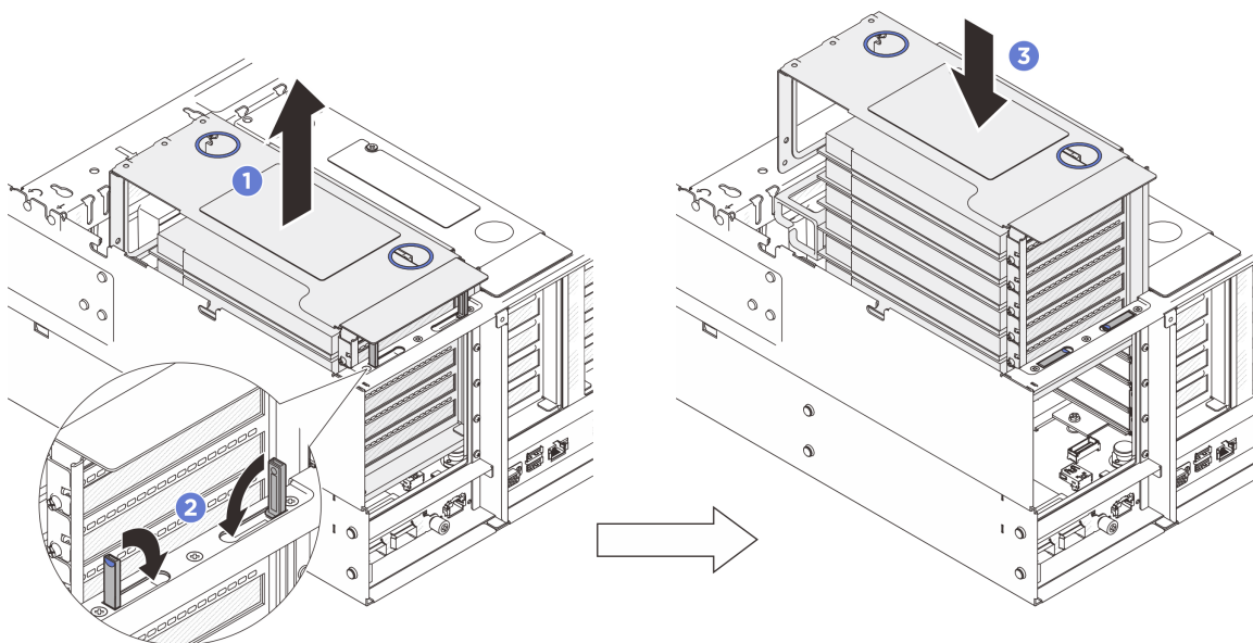
図 40. PCIe ライザーの固定
