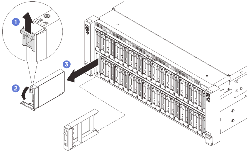
図5. 2.5 インチ ドライブの取り外し
