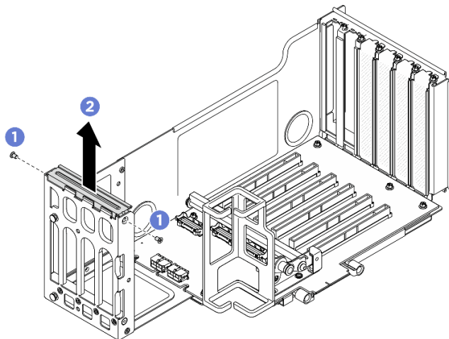
図 79. ライザー・エクステンダー・カバーの取り外し
