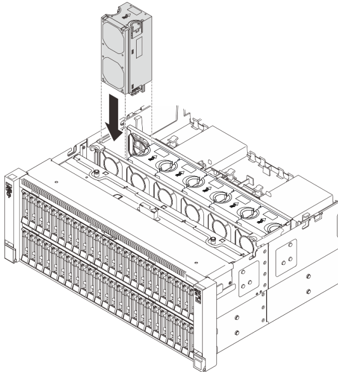
図 69. ファンの取り付け
