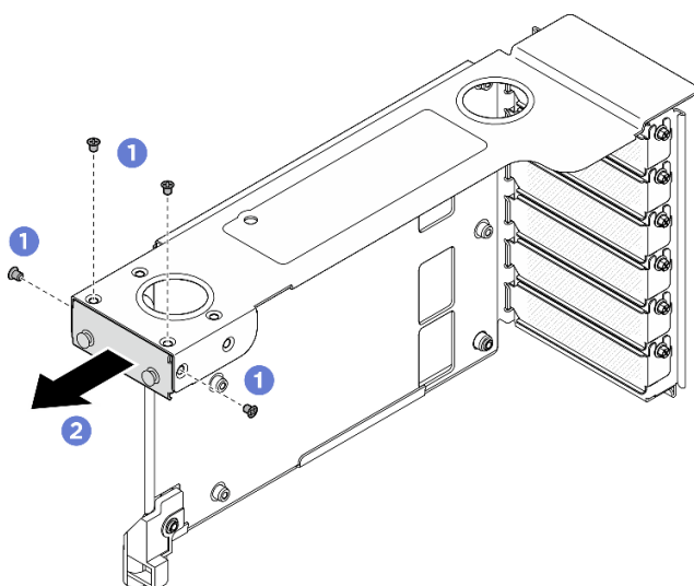
図 218. FH PCIe ライザーからのフィラーの取り外し
