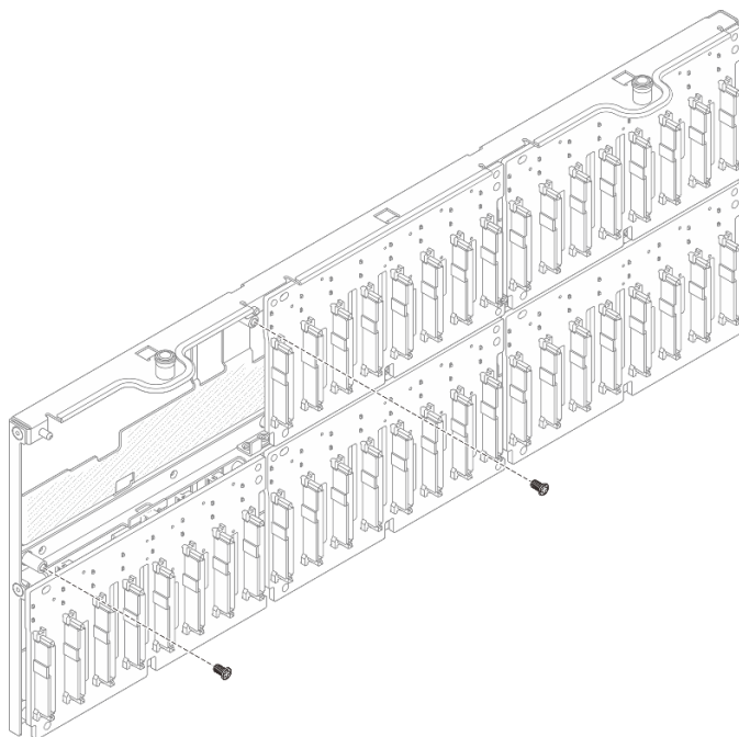
図 11. バックプレーン・キャリアのスペアねじ (2.5 インチ ベイ・シャーシ)
