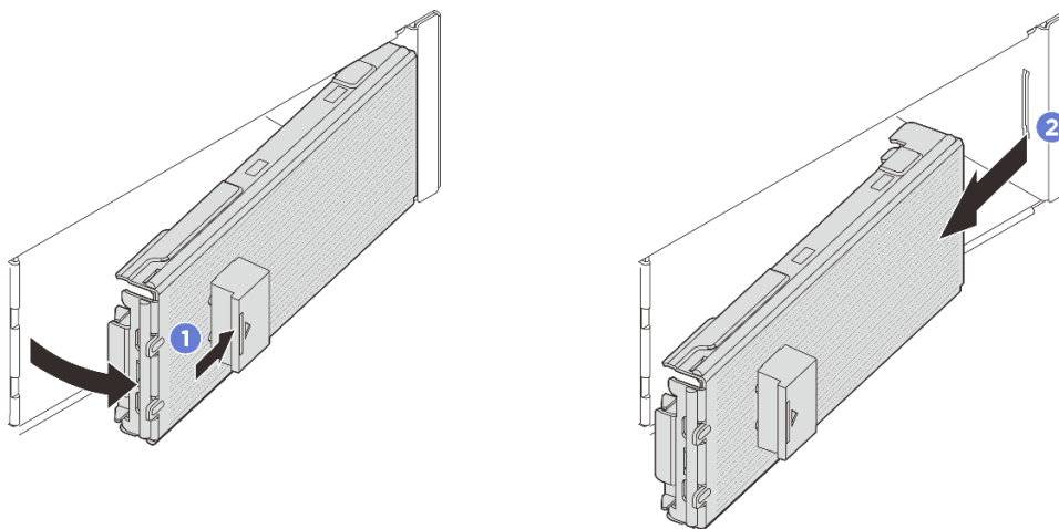
図 41. E3.S ベゼルの取り外し
