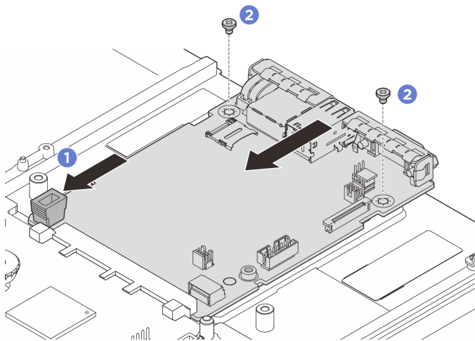
図 292. システム I/O ボードの取り付け
