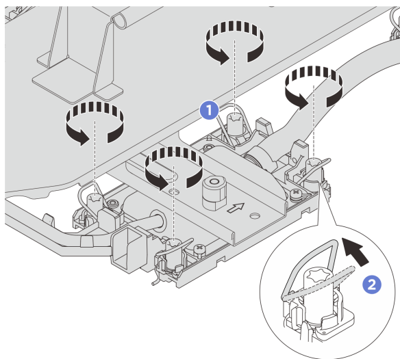
図 100. Torx T30 ナットを緩める
