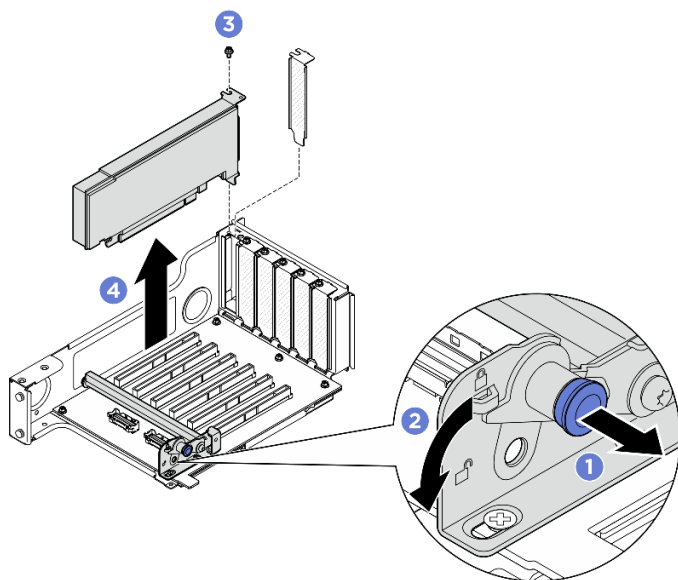
図 179. ライザーからの PCIe アダプターの取り外し
