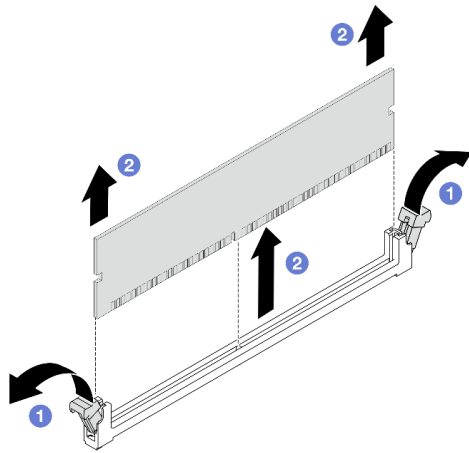
図 163. メモリー・モジュールの取り外し
