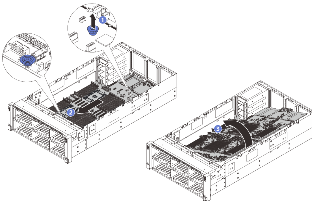
図 290. システム・ボード・アセンブリーの取り外し
