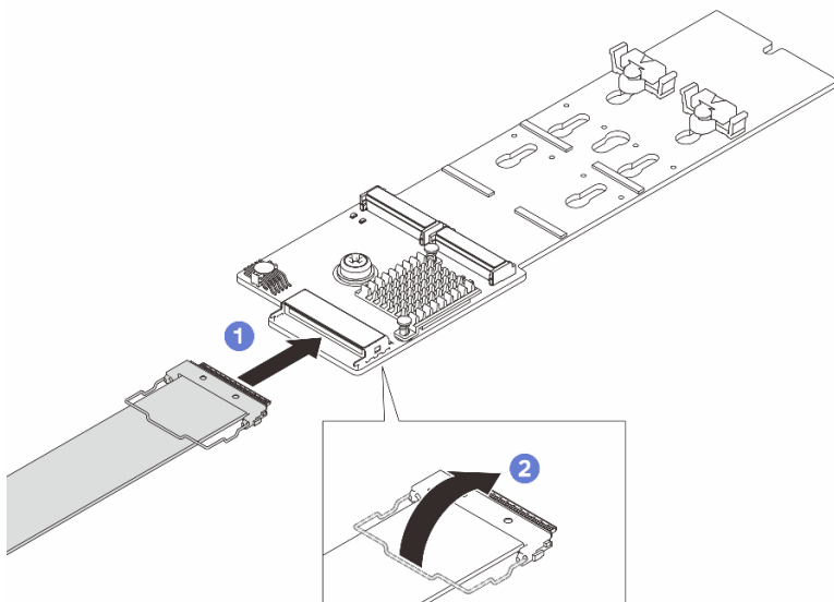
図 90. M.2 バックプレーン・ケーブルの接続
