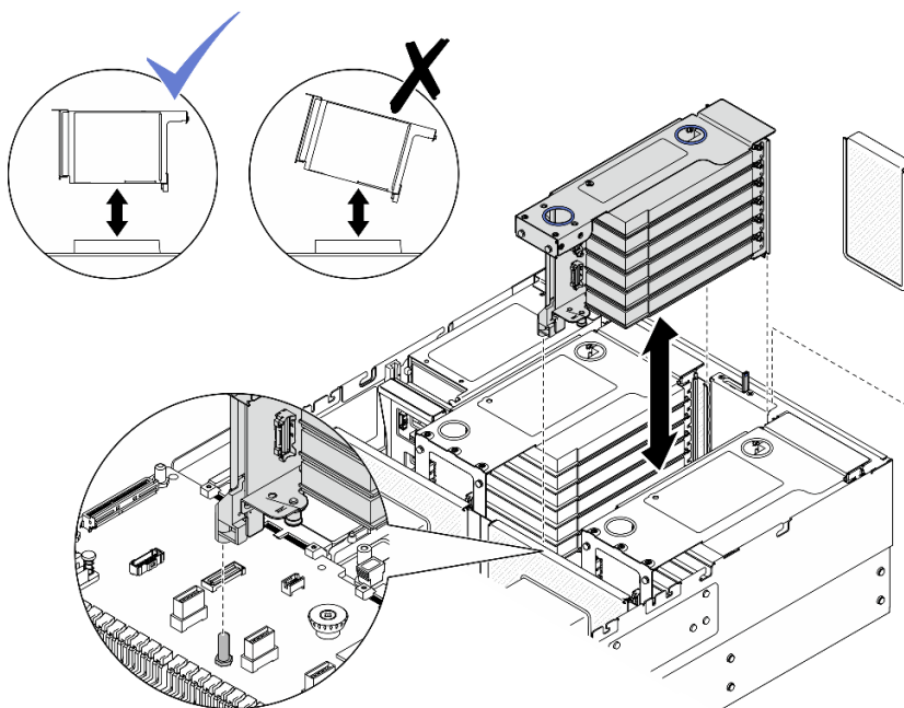
図 173. PCIe ライザー 2 の取り外し
