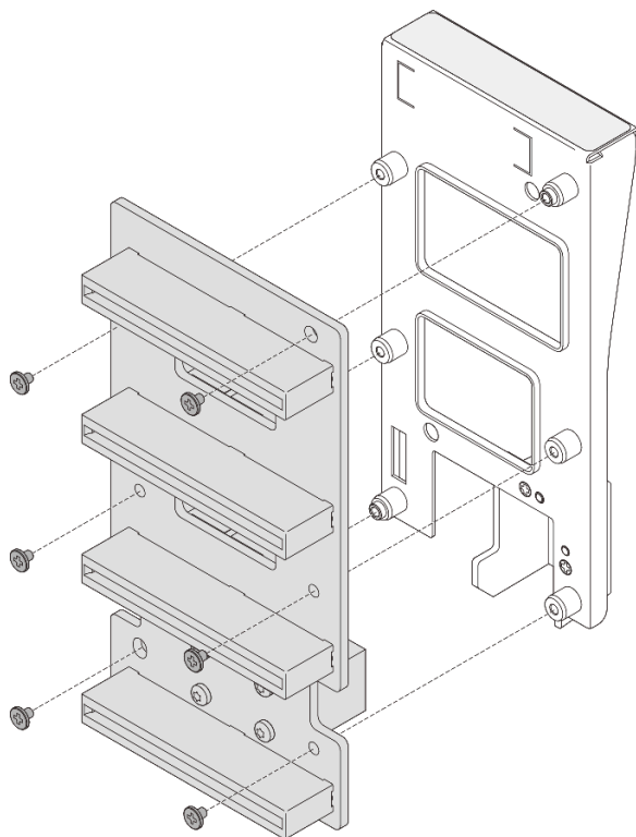
図 222. 分電盤の切り離し
