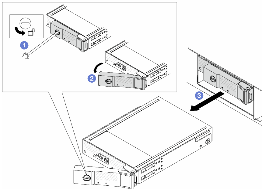
図 54. CMM の取り外し
