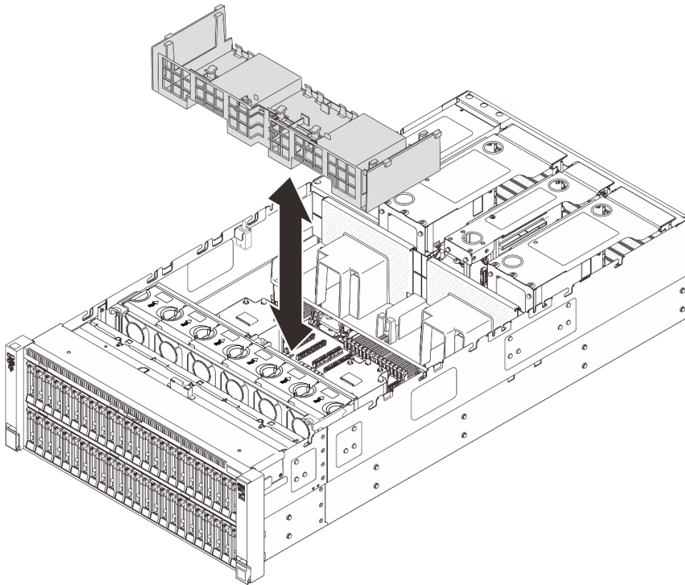
図 21. 前面エアー・バッフルの取り付け
