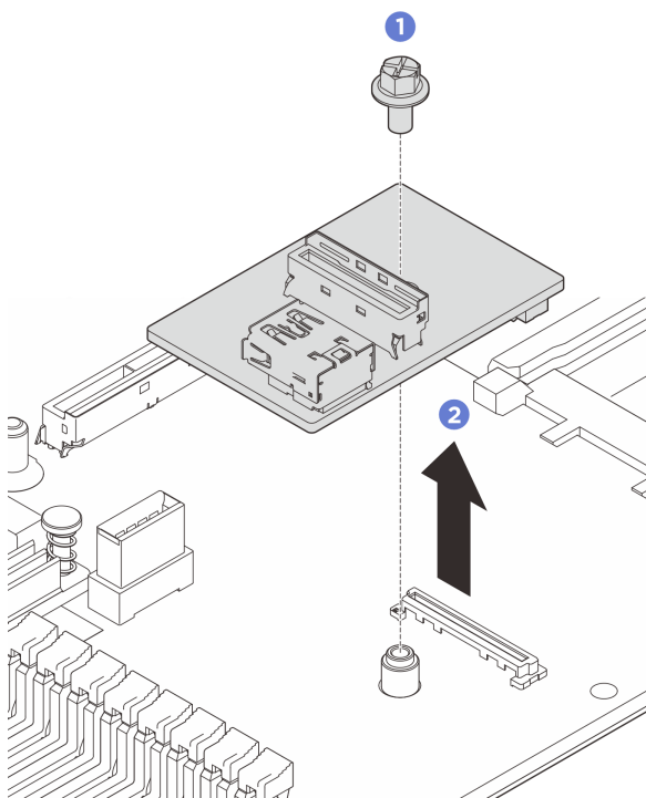
図 300. USB I/O ボードの取り外し
