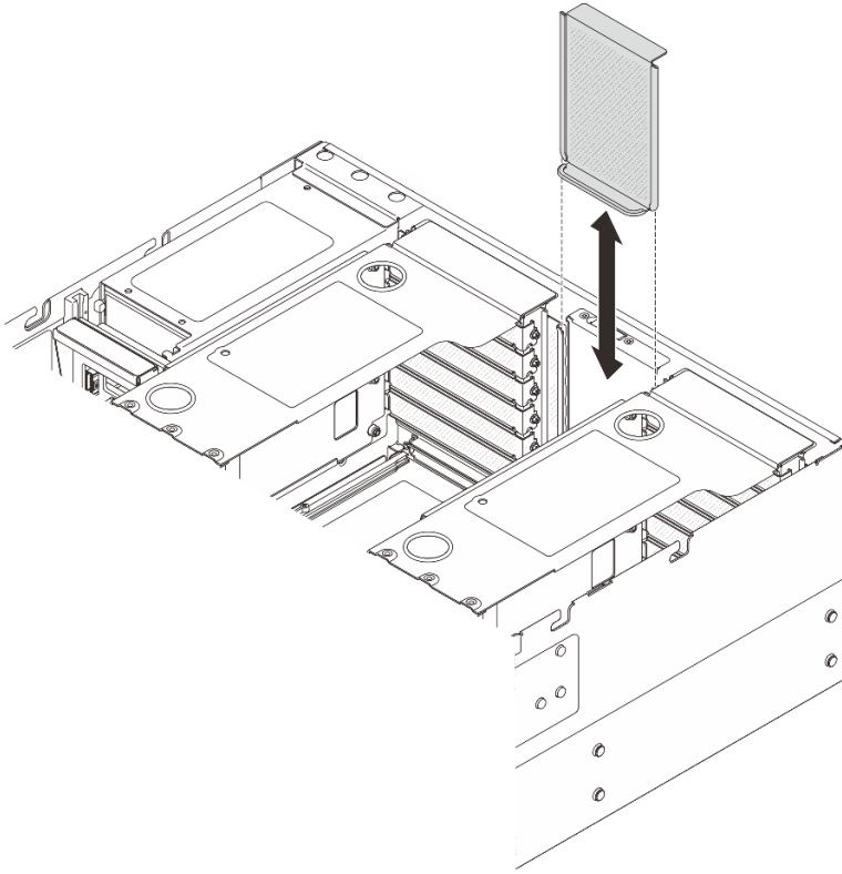
図 112. ライザー・フィルターの取り付け
