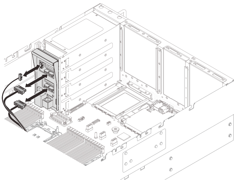
図 224. 分電盤のケーブルの接続
