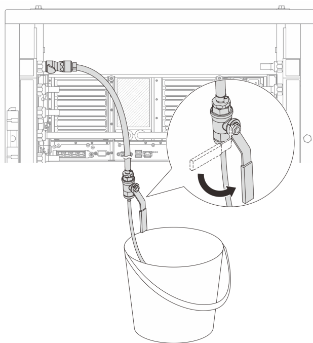
図 156. 供給側のブリーダーのバルブを開く
