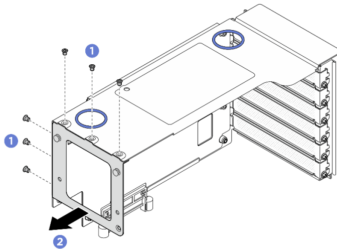
図 216. FH PCIe ライザー・ケージからのフィラーの取り外し
