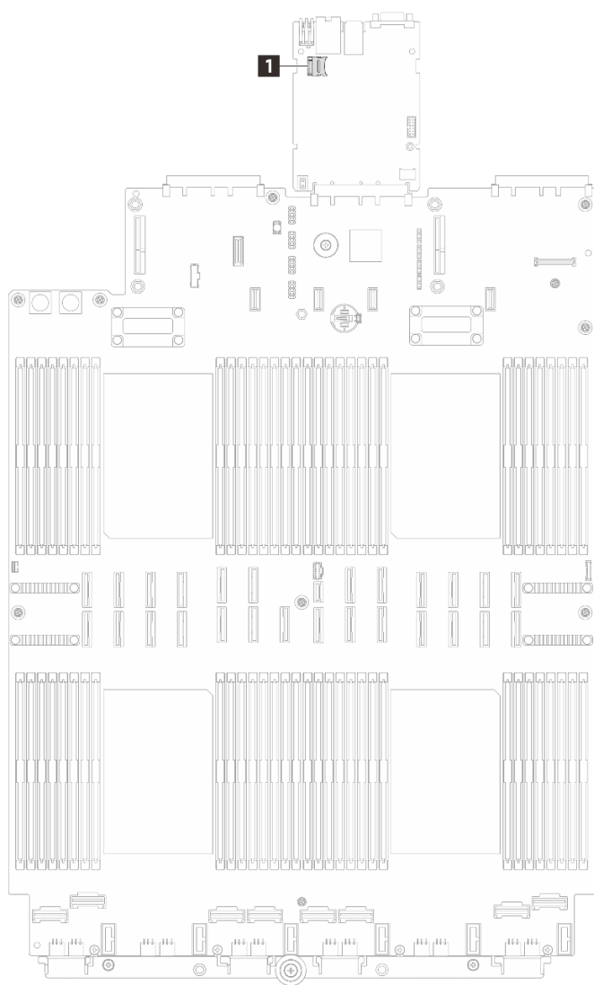
図 168. MicroSD カードの位置
