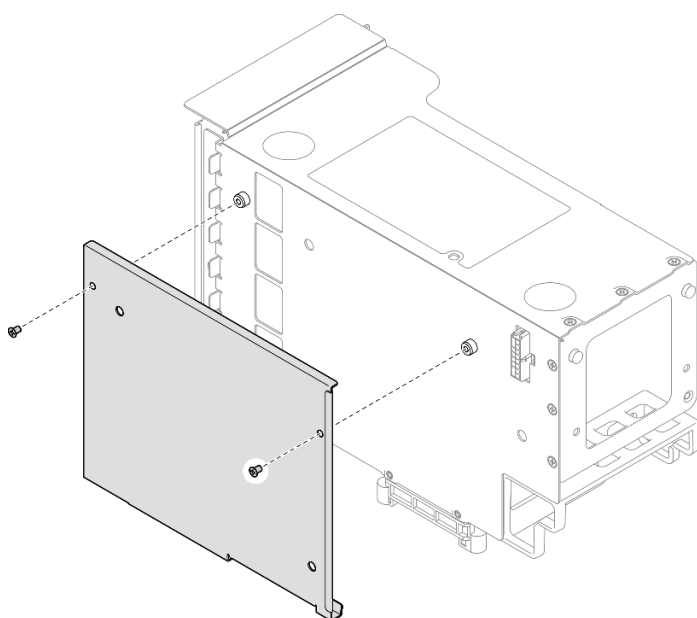
図 205. ライザー・ケージからのカバーの取り外し
