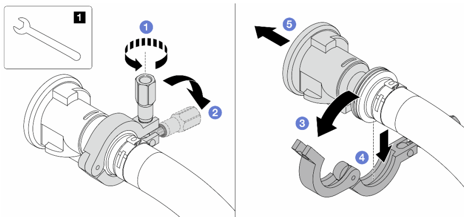
図 130. ボール・バルブの取り外し
