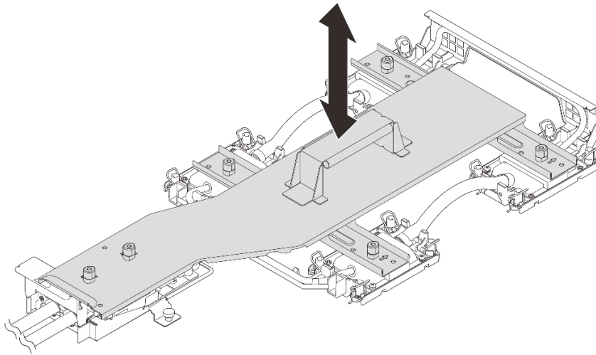
図98. コールド・プレート・キャリアの取り付け
