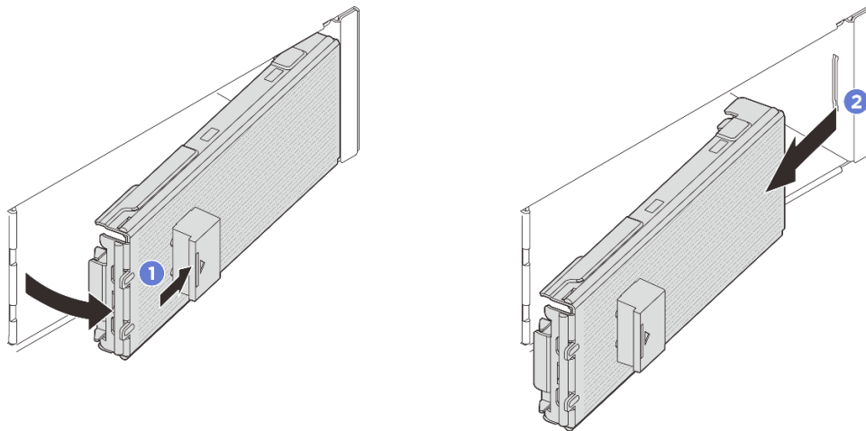
図 53. E3.S ベゼルの取り外し
