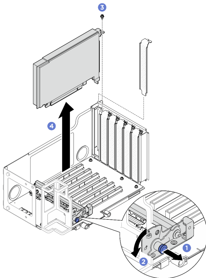
図 178. ライザーからの PCIe アダプターの取り外し
