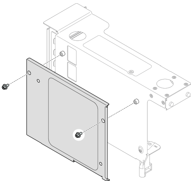
図 211. ライザー・ケージからのカバーの取り外し
