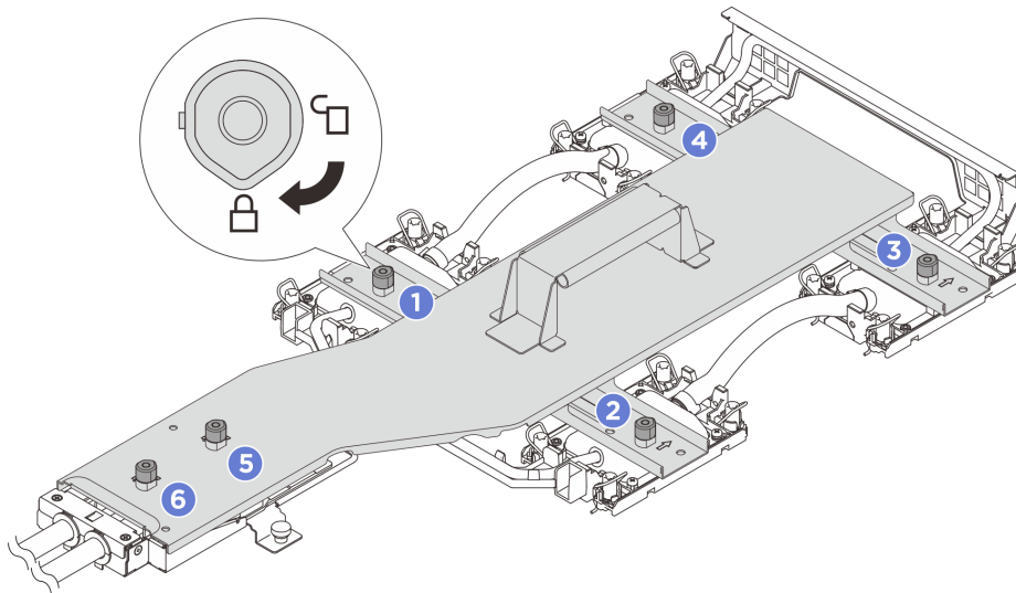
図99. コールド・プレート・キャリアの固定
