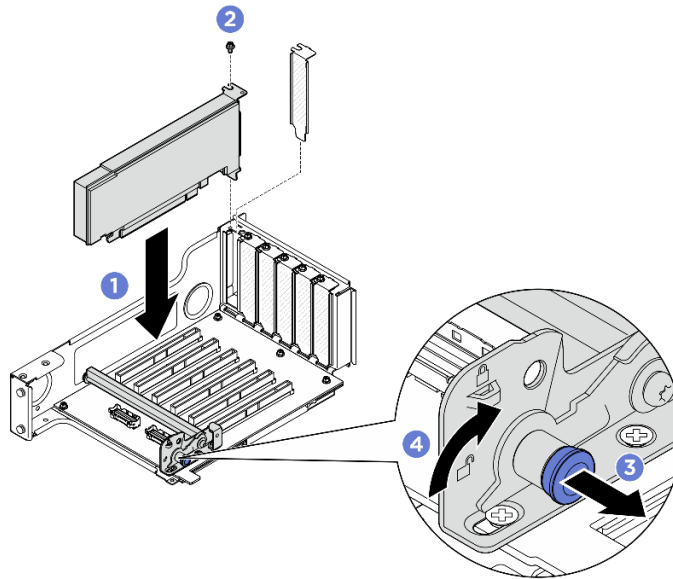
図 182. PCIe アダプターの PCIe ライザーへの取り付け
