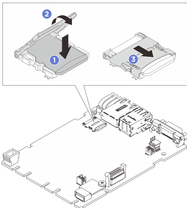
図 169. microSD カードの取り付け
