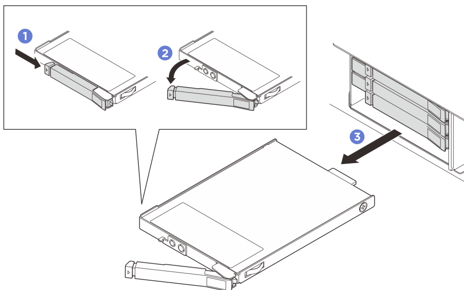
図 42. E3.S ホット・スワップ・ドライブの取り外し
