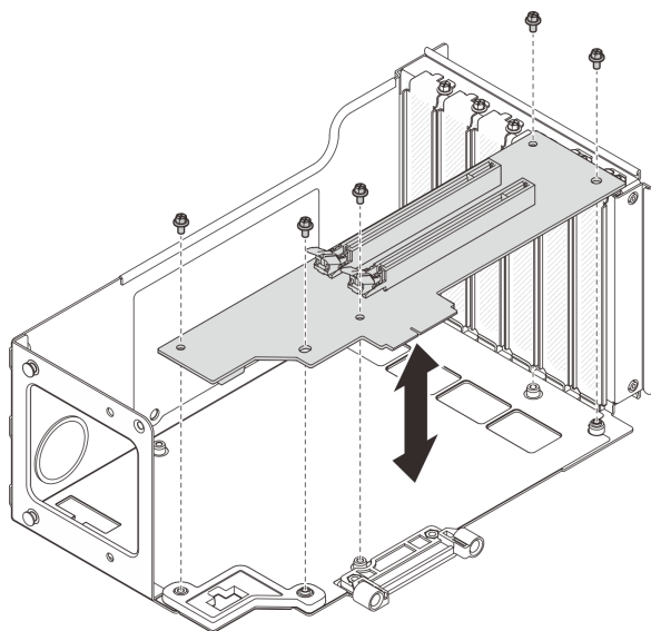
図 186. ライザー・ケージからの PCIe ライザー・カードの取り外し
