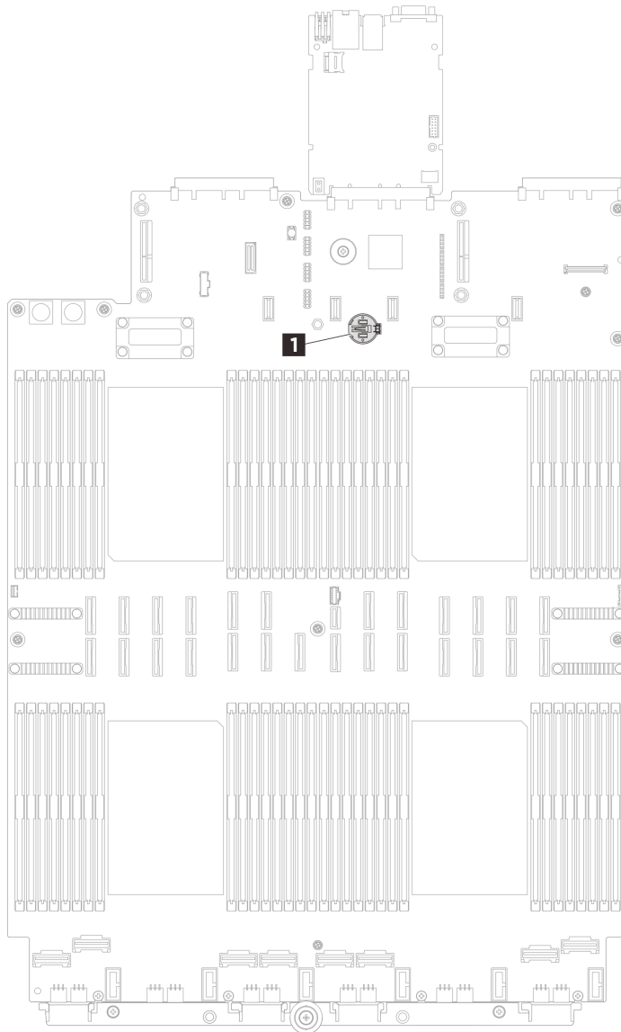
図 33. CMOS バッテリーの位置
