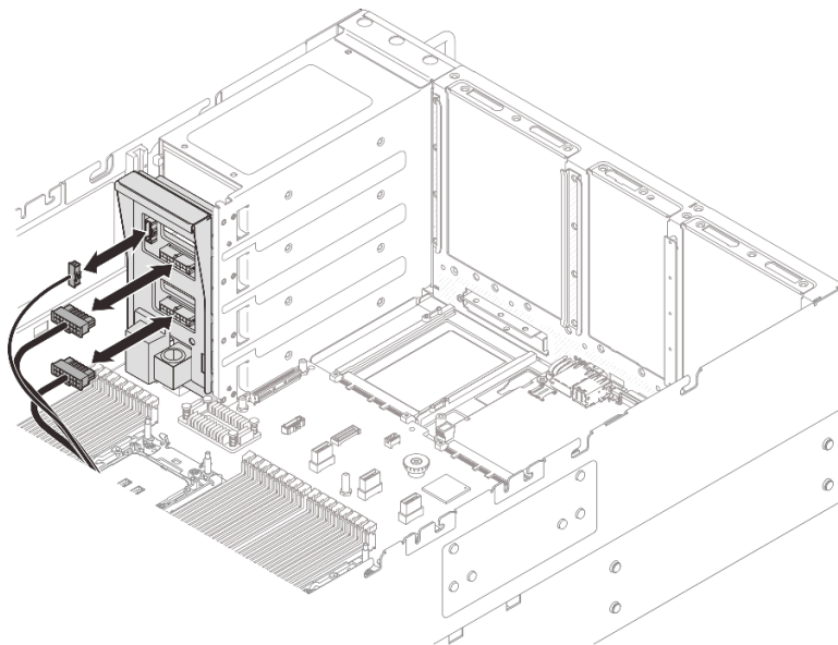
図 220. 分電盤のケーブルの取り外し
