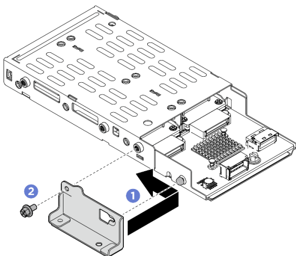
図 272. M.2 ドライブ・ケージ・ブラケットを取り付ける
