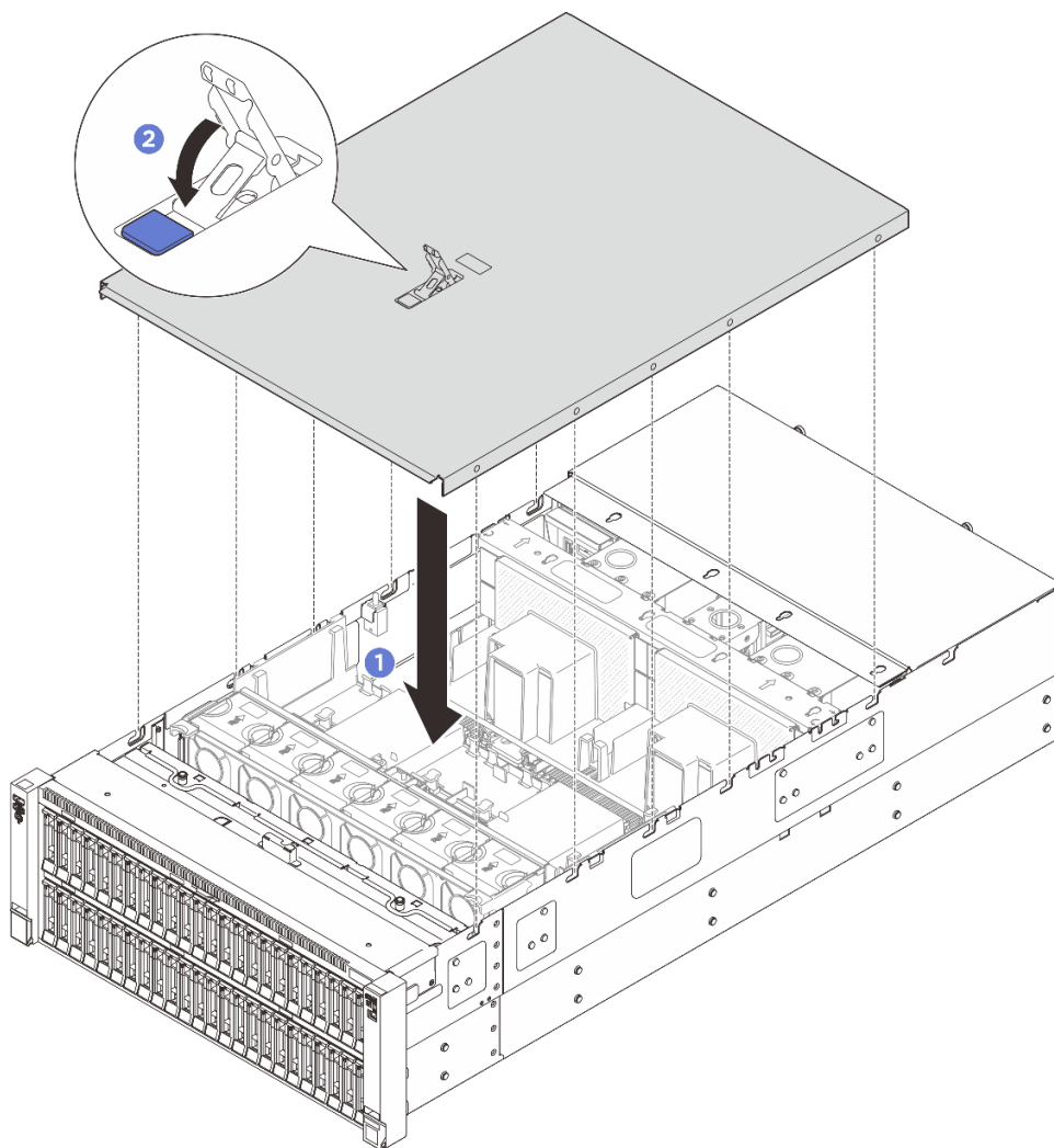
図298. 前面トップ・カバーの取り付け
