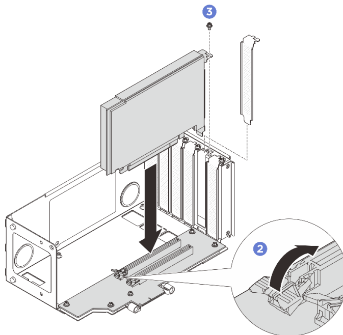
図 180. PCIe アダプターの PCIe ライザーへの取り付け
