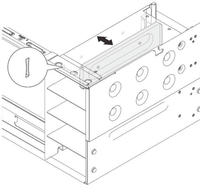
図 227. パワー・サプライ・ブラケットの取り付け
