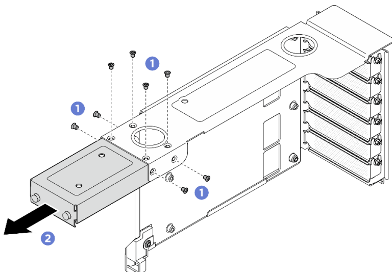
図 215. HH PCIe ライザー・ケージからのライザー・エクステンダーの取り外し
