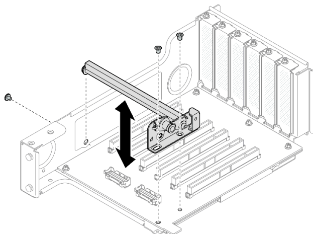
図 197. ライザー・ケージからの PCIe 保持具の取り外し
