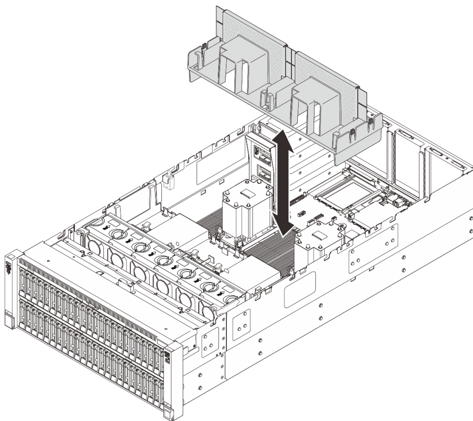
図 26. 3U 標準 PHM 用背面エアー・バッフルの取り外し
