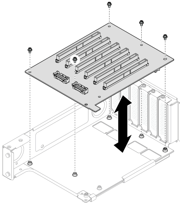
図 208. ライザー・ケージへの PCIe ライザー・カードの取り付け
