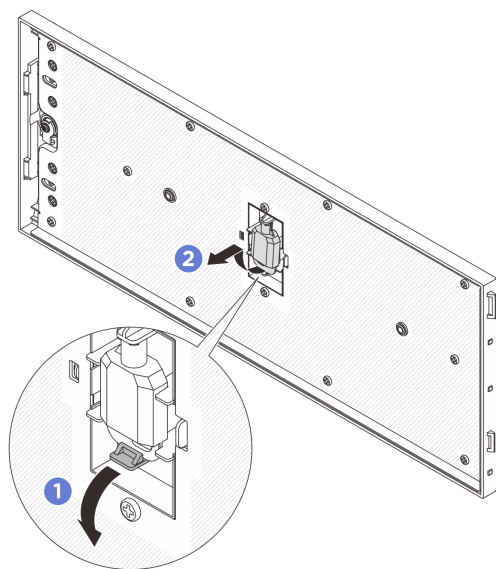
図 276. キーの取り外し
