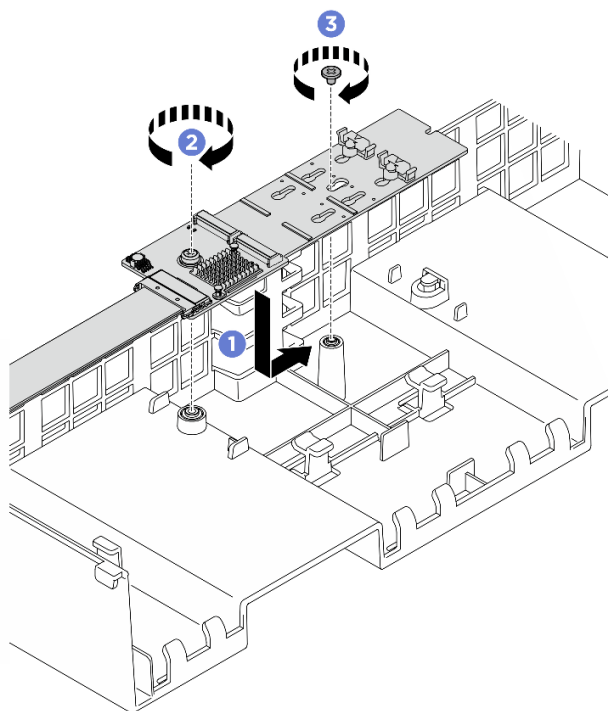
図 91. M.2 バックプレーンの取り付け
