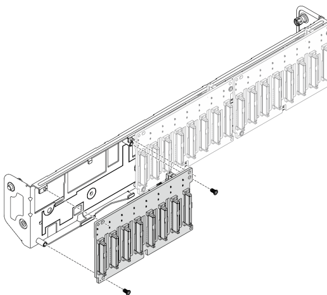
図10. キャリアからのバックプレーンの取り外し (E3.5 ベイ・シャーシ)
