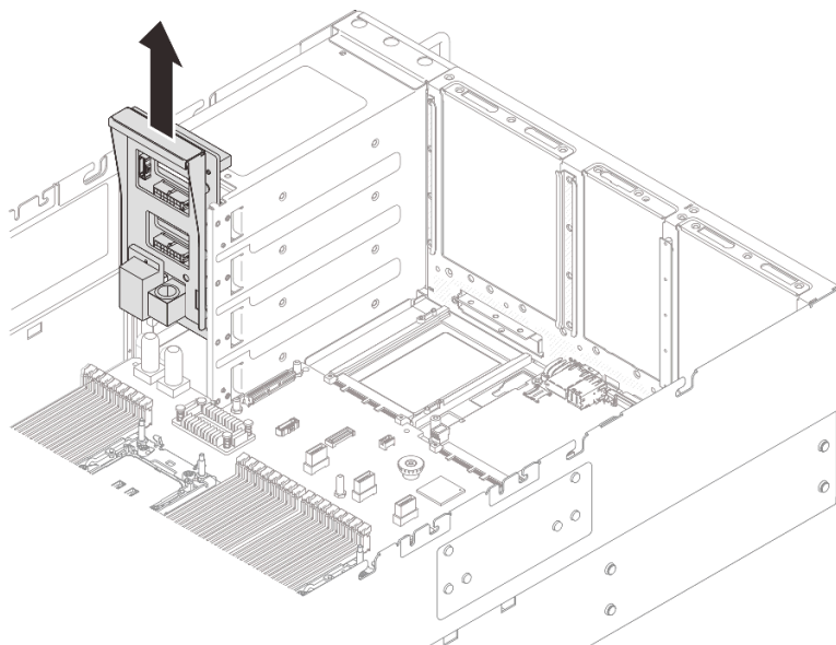
図 221. 分電盤の取り外し
