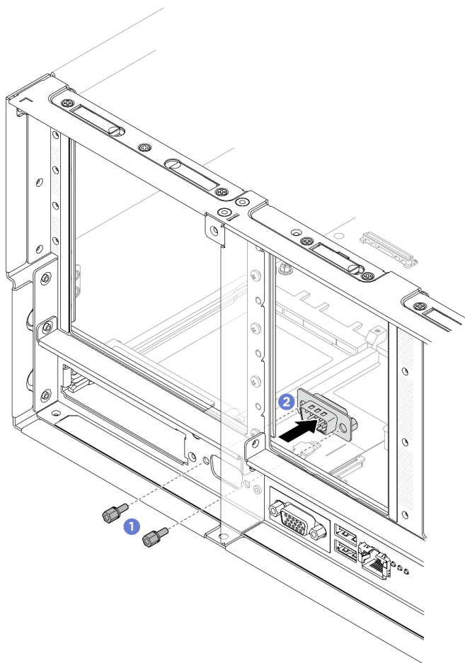
図 280. シリアル・ポート・モジュールの取り外し
