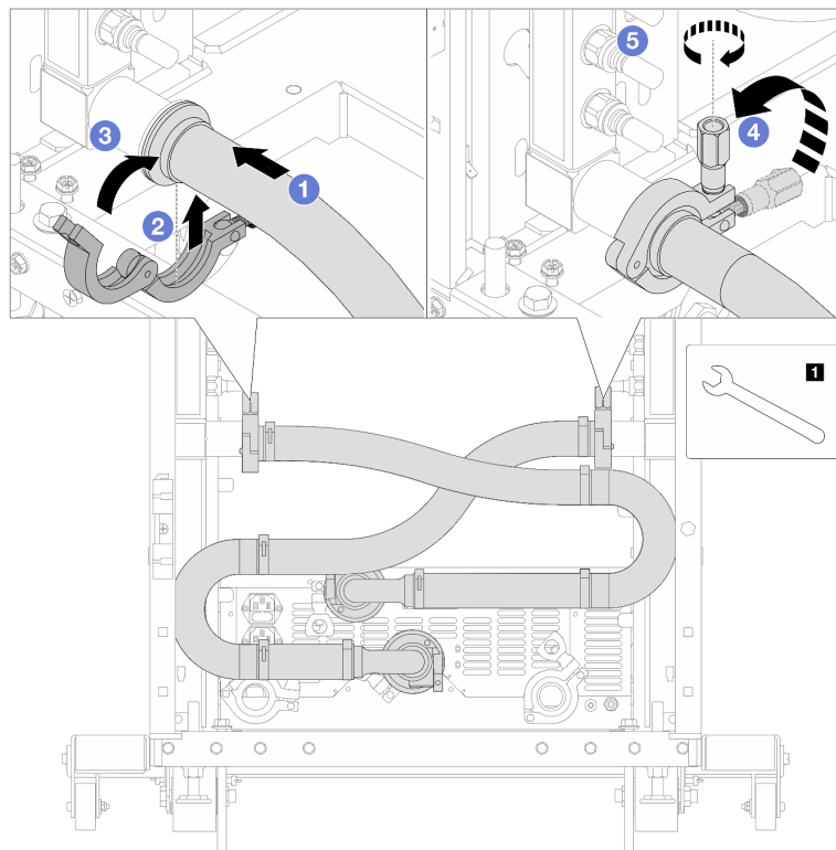
図 132. 接続セットの取り付け
