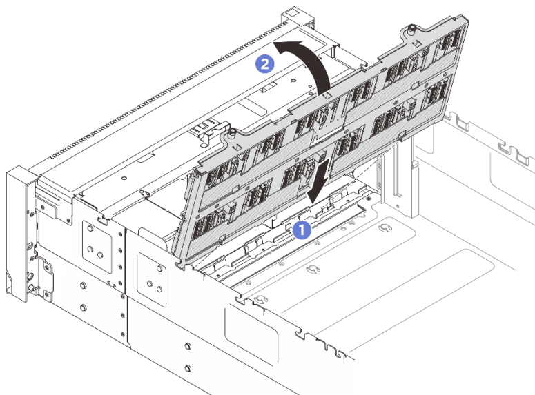
図 15. ドライブ・バックプレーン・キャリア・アセンブリーの取り付け (2.5 インチ ベイ・シャーシ)
