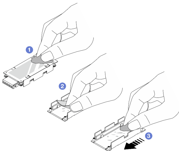
図 257. ヒートシンクと底板のクリーニング
