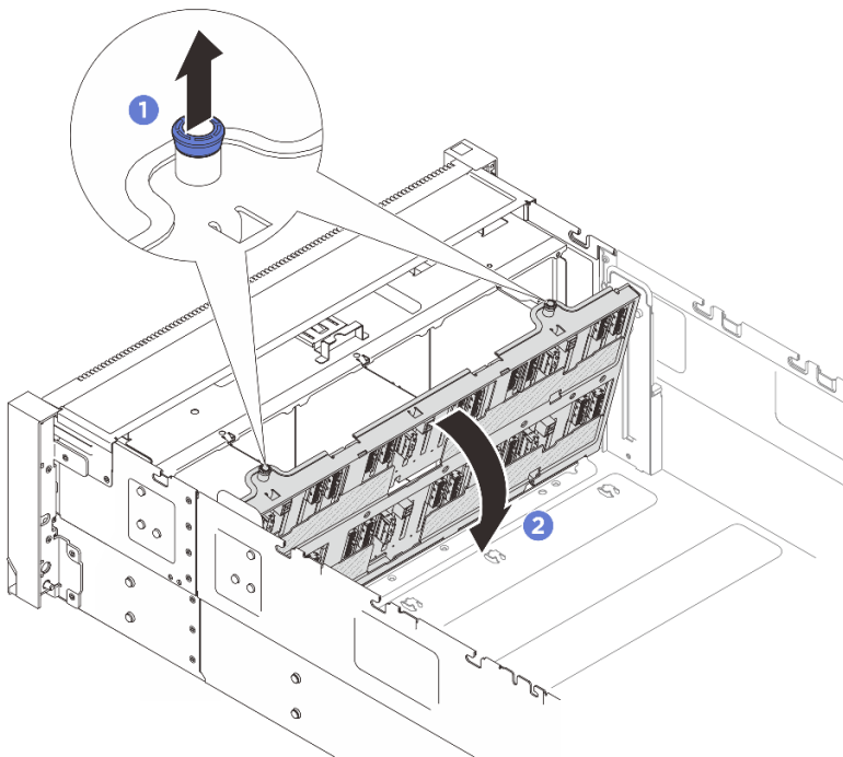
図7. ドライブ・バックプレーン・キャリア・アセンブリーの取り外し (2.5 インチ ベイ・シャーシ)
