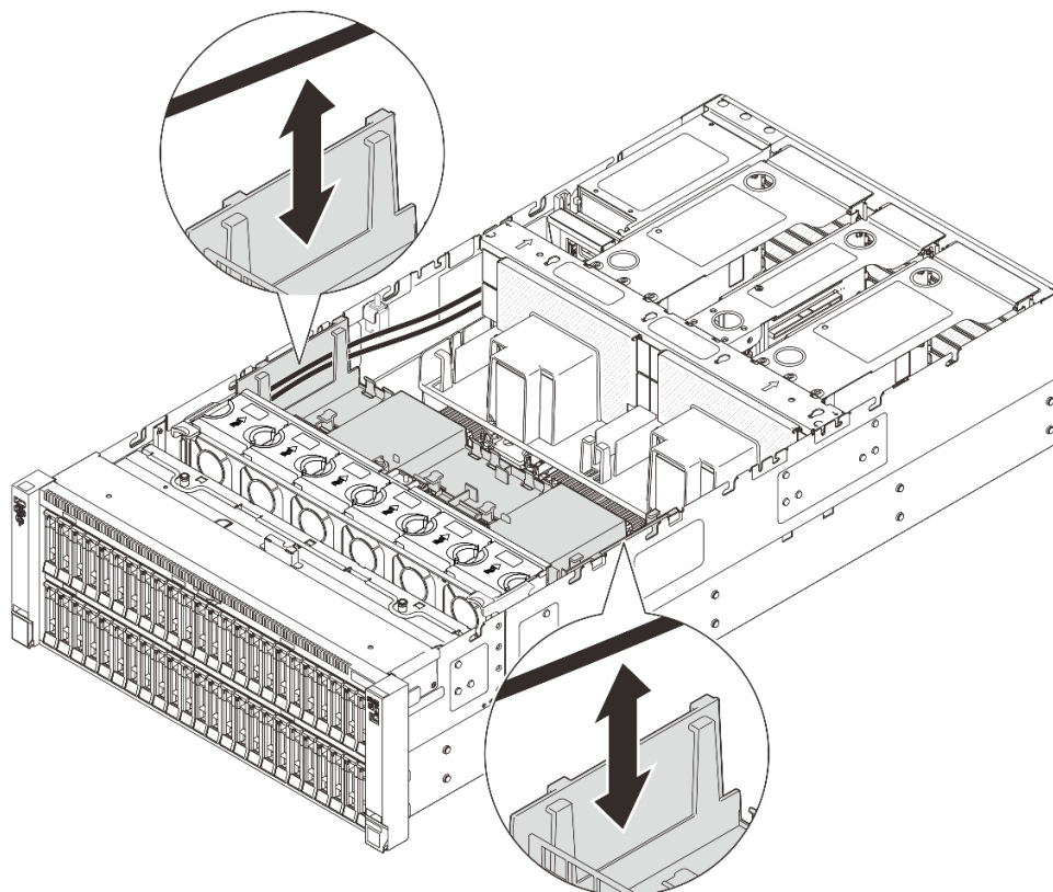
図 22. 前面エアー・バッフルのケーブル配線
