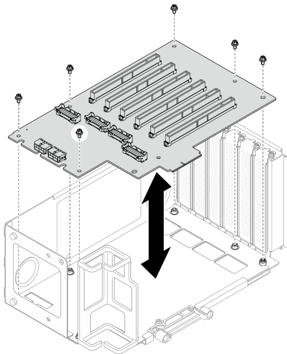
図 192. ライザー・ケージからの PCIe ライザー・カードの取り外し
