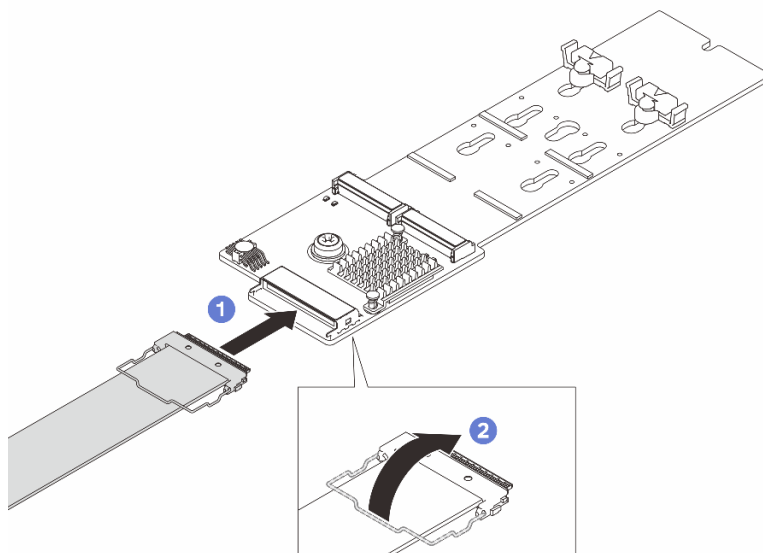
図 23. M.2 バックプレーン・ケーブルの接続
