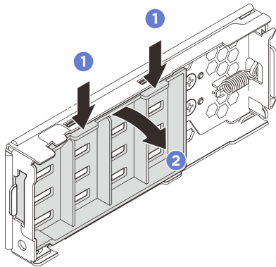
図 47. 内板の取り外し
