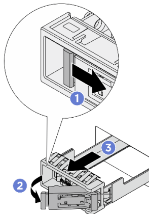
図 252. M.2 ドライブ・トレイの取り外し
