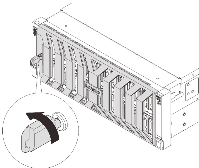
図 278. セキュリティー・ベゼルのロック
