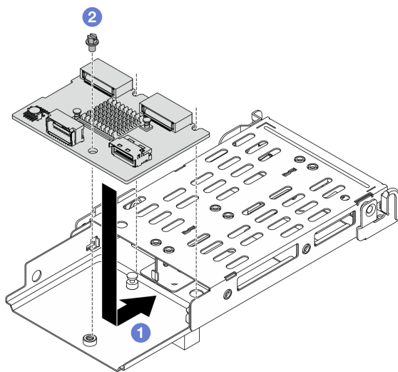
図 271. M.2 バックプレーンの取り付け
