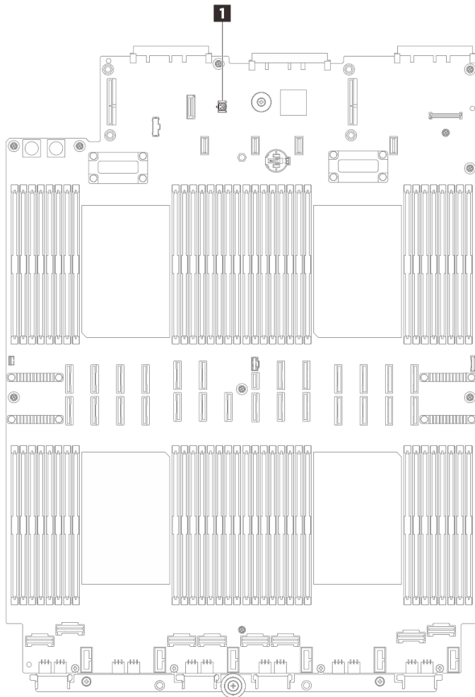
図 95. 漏水検知センサー・モジュールの取り外し
