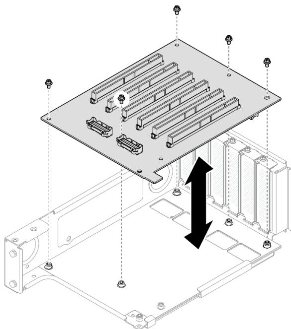
図 198. ライザー・ケージからの PCIe ライザー・カードの取り外し
