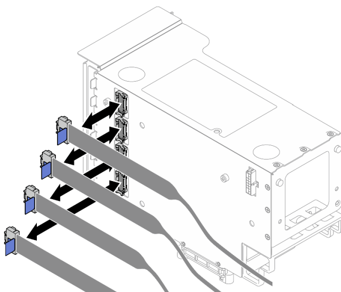
図 189. ライザーの外側からの PCIe ライザー・ケーブルの切り離し
