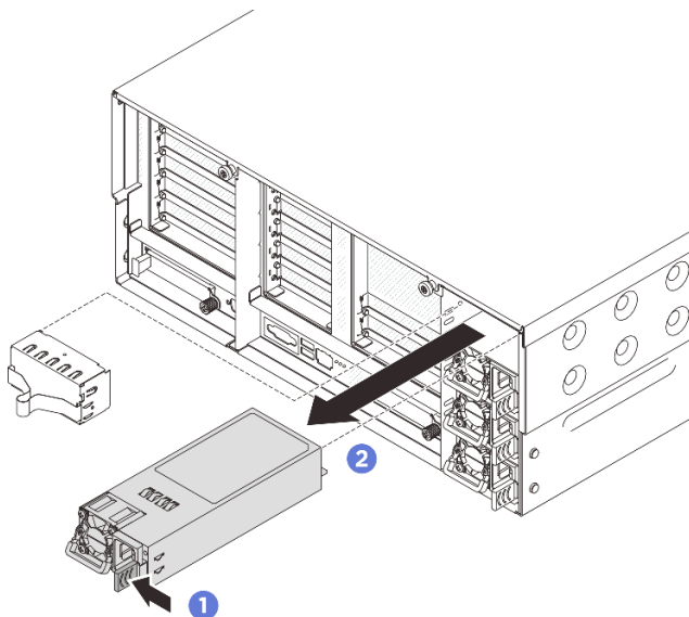
図 229. パワー・サプライ・ユニットの取り外し
