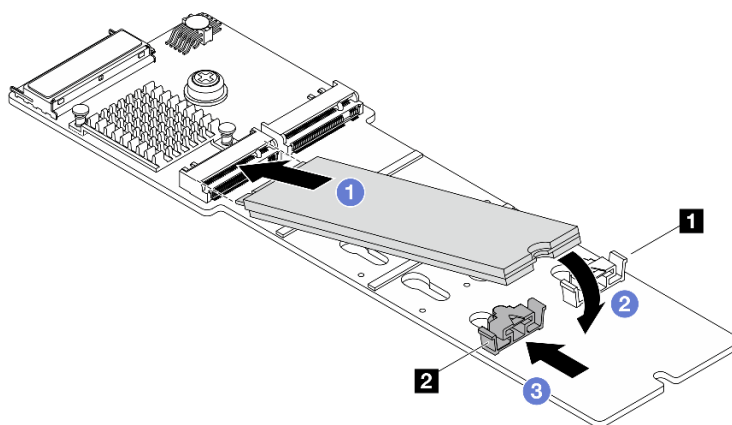
図 94. M.2 ドライブの取り付け
