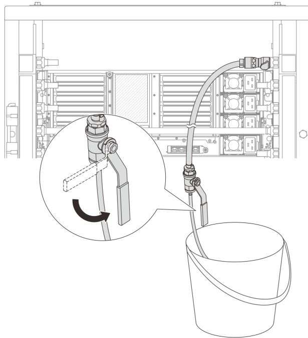
図 141. リターン側のブリーダー・バルブを開く
