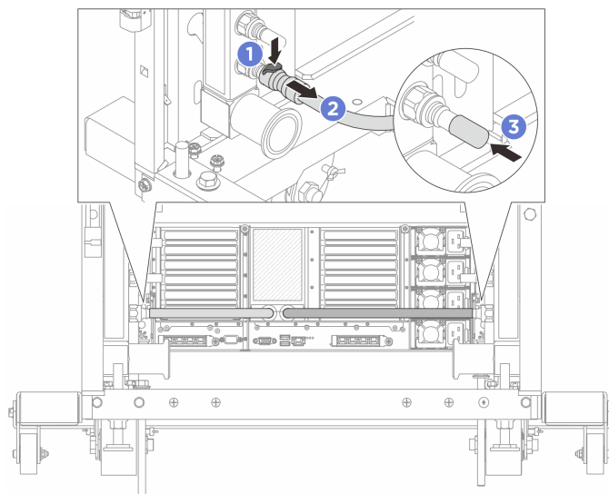
図 121. クイック・コネクト・プラグの取り外し
