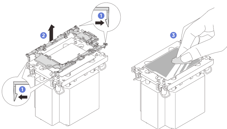
図 237. ヒートシンクからプロセッサ・キャリアを取り外す
