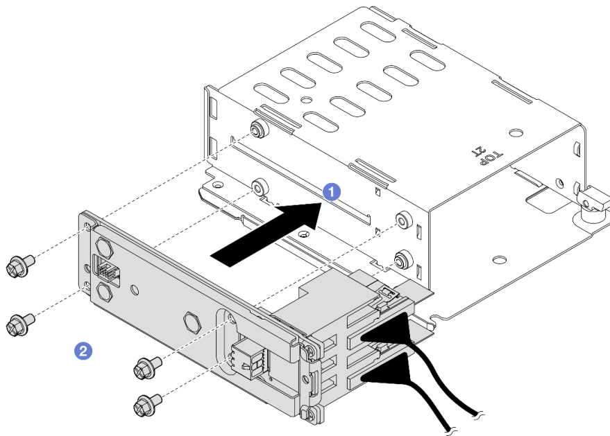
図 64. バックプレーンの取り付け
