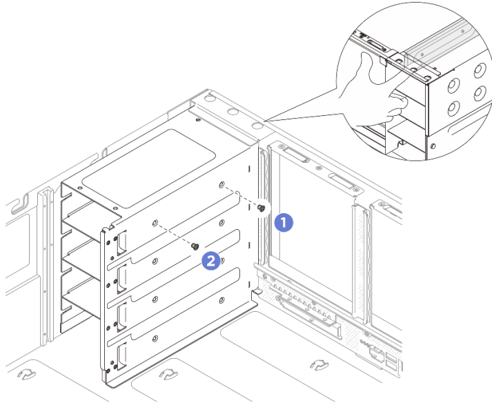
図 228. パワー・サプライ・ブラケットの固定
