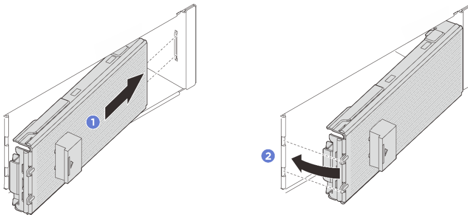
図 48. E3.S ベゼルの取り付け
