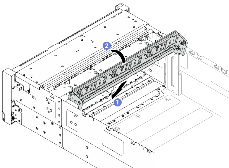
図 16. ドライブ・バックプレーン・キャリア・アセンブリーの取り付け (E3.5 ベイ・シャーシ)
