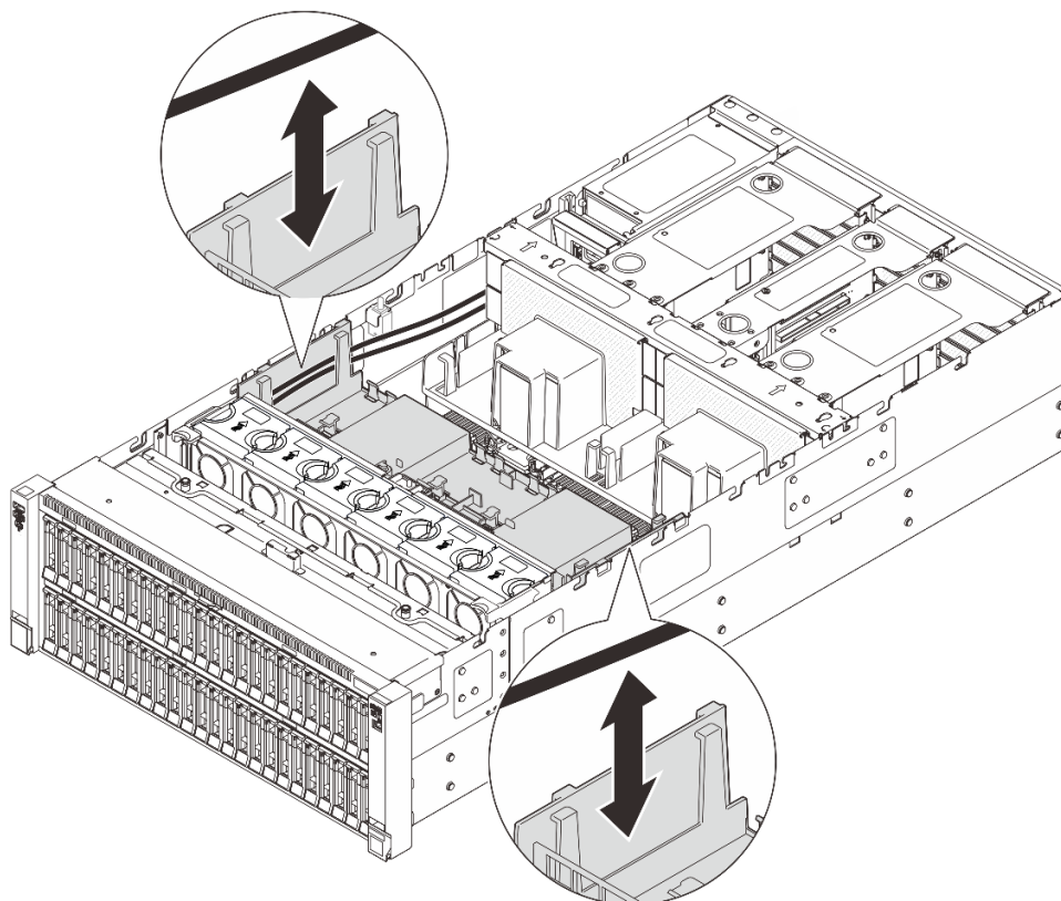
図 19. 前面エア・バッフルからケーブルを持ち上げる
