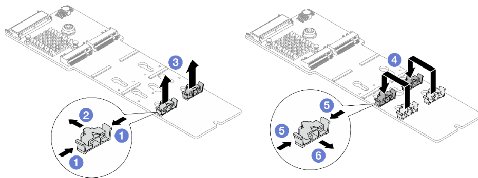
図 93. M.2 保持器具の調整
