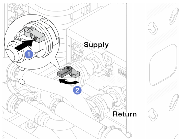
図 138. ボール・バルブを開く
