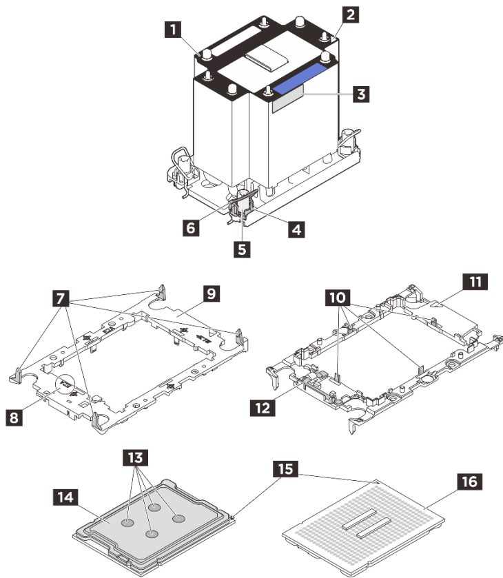
図 233. PHM コンポーネント
