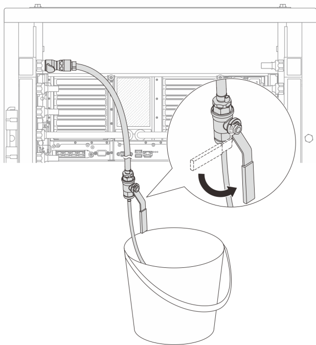
図 160. 供給側のブリーダーのバルブを開く
