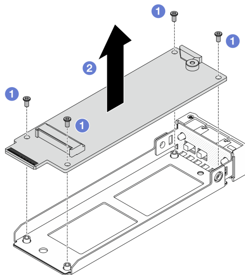
図 255. M.2 変換コネクタの取り外し
