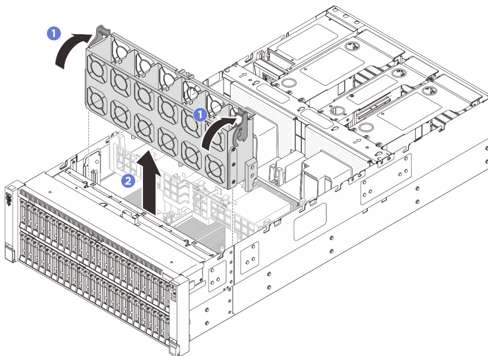
図 67. ファン・ケージの取り外し
