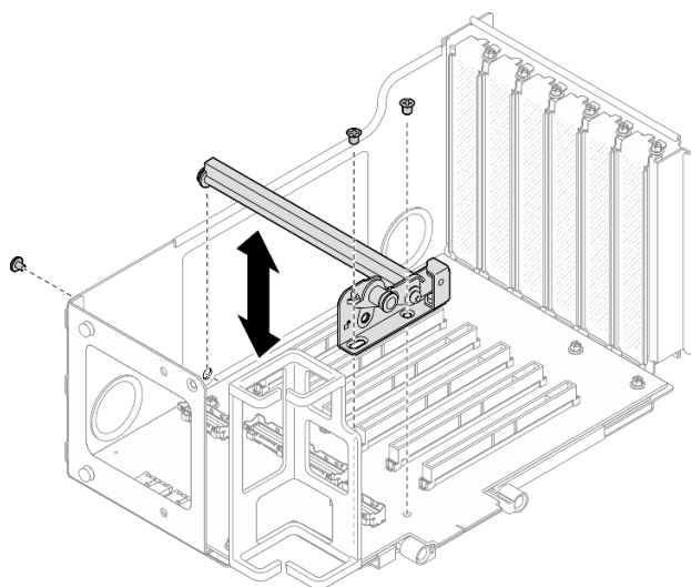
図 191. ライザー・ケージからの PCIe 保持具の取り外し
