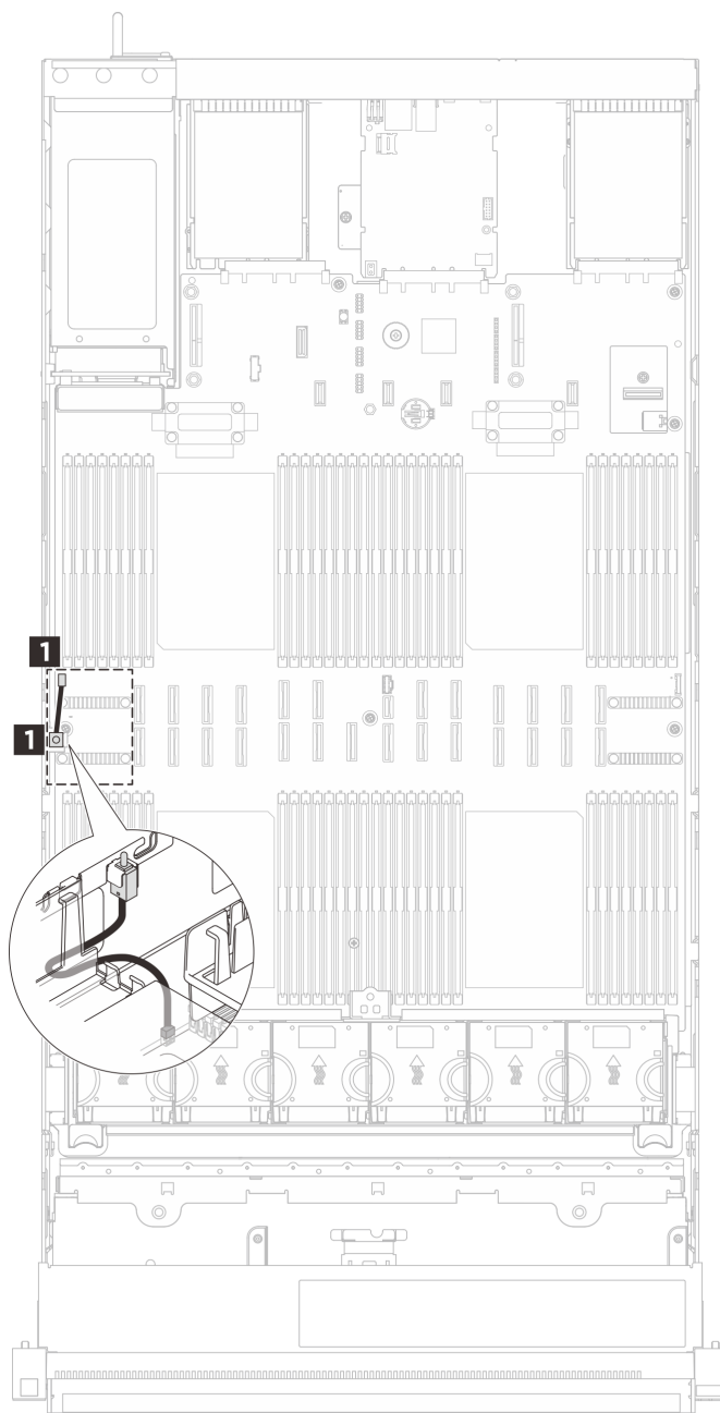
図 86. 侵入検出スイッチの接続
