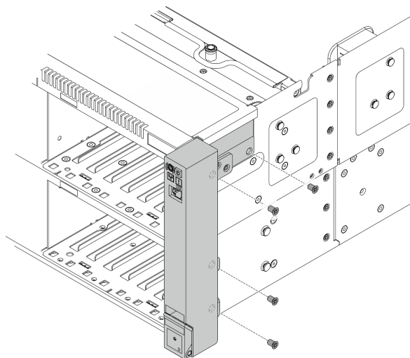
図245. ねじの取り外し
