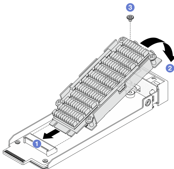
図 261. ヒートシンクが付いた M.2 ドライブの取り付け
