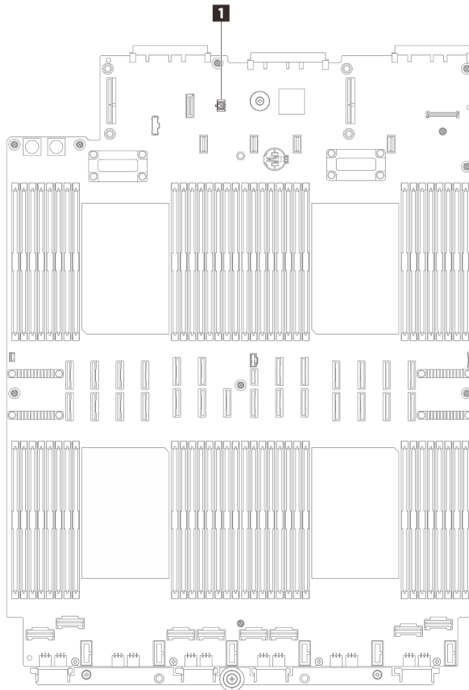
図 113. 漏水検知センサー・モジュールの接続
