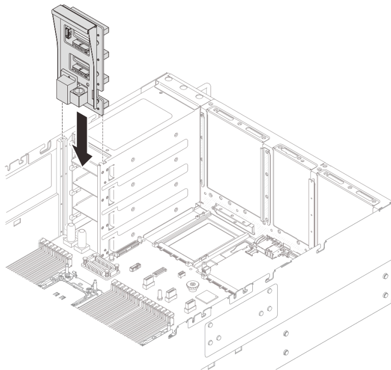
図 223. 分電盤の取り付け
