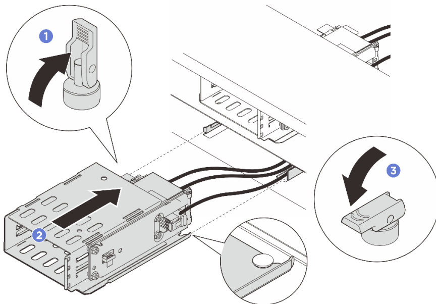
図 52. E3.S 1T ケージの取り付け
