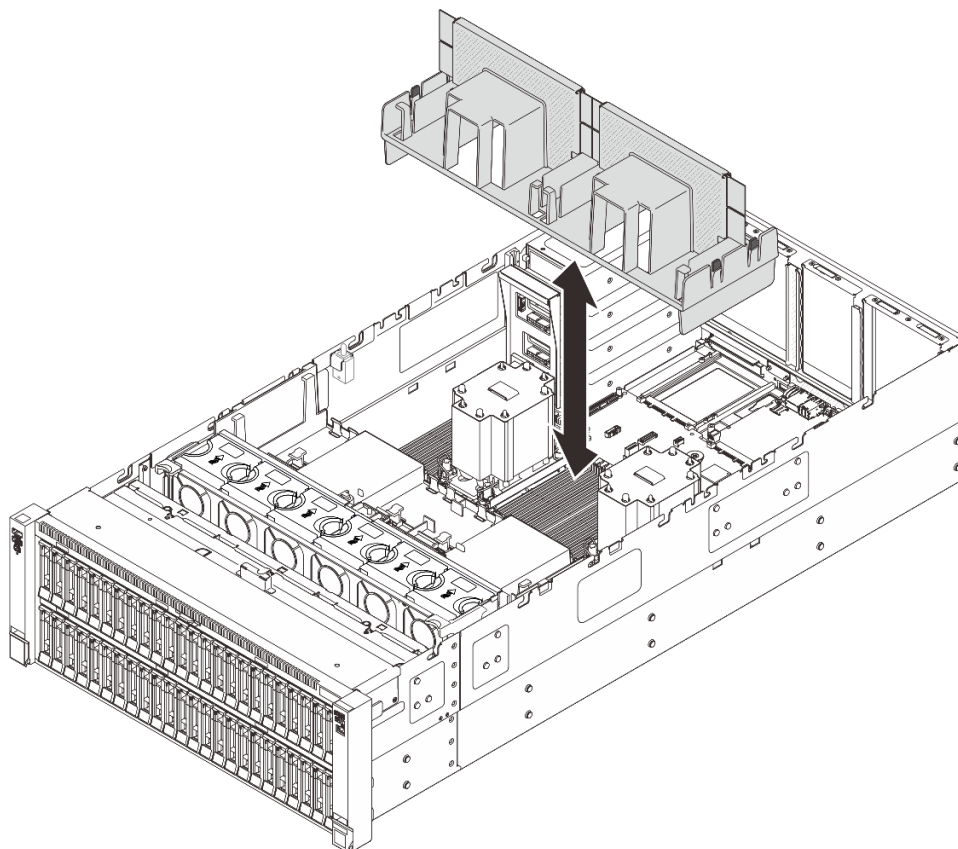
図 28. 3U 標準 PHM 用背面エア・バッフルの取り付け
