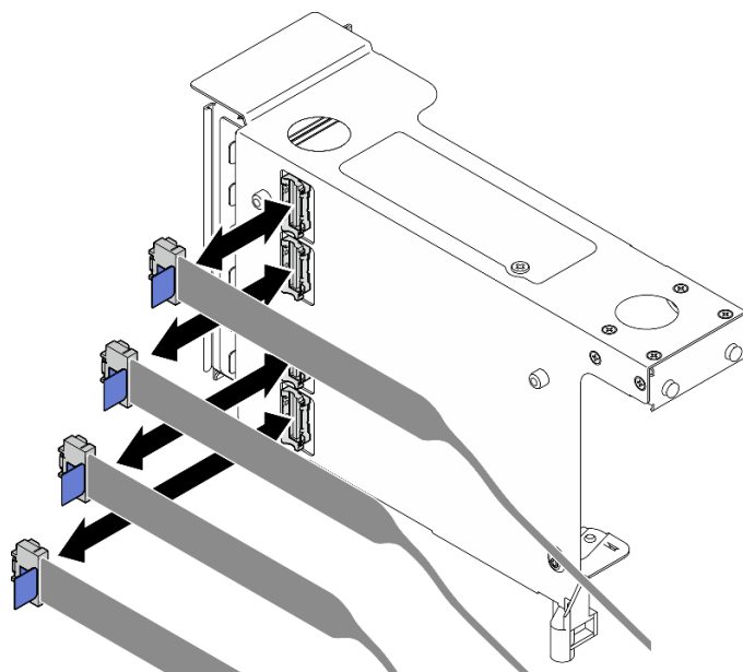
図 212. ライザーの外側への PCIe ライザー・ケーブルの接続
