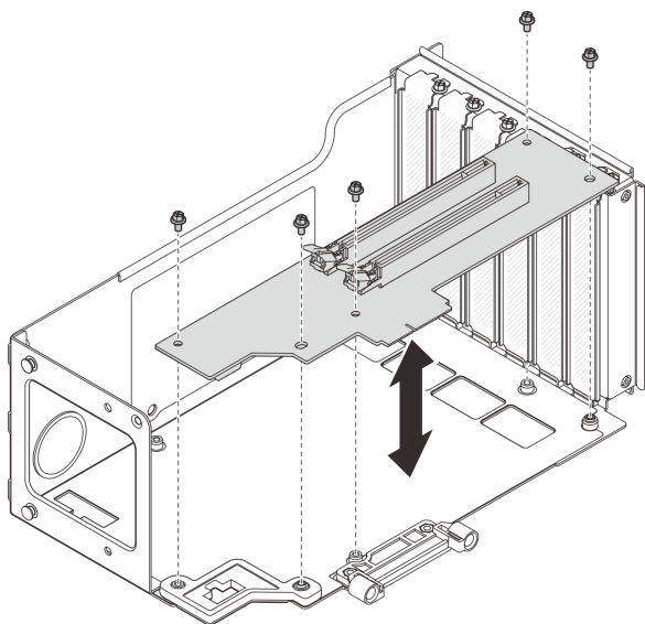
図200. ライザー・ケージへの PCIe ライザー・カードの取り付け
