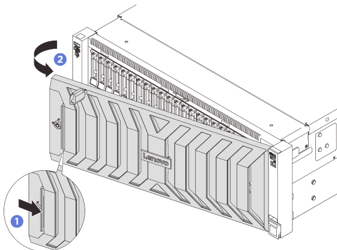
図 275. セキュリティー・ベゼルの取り外し
