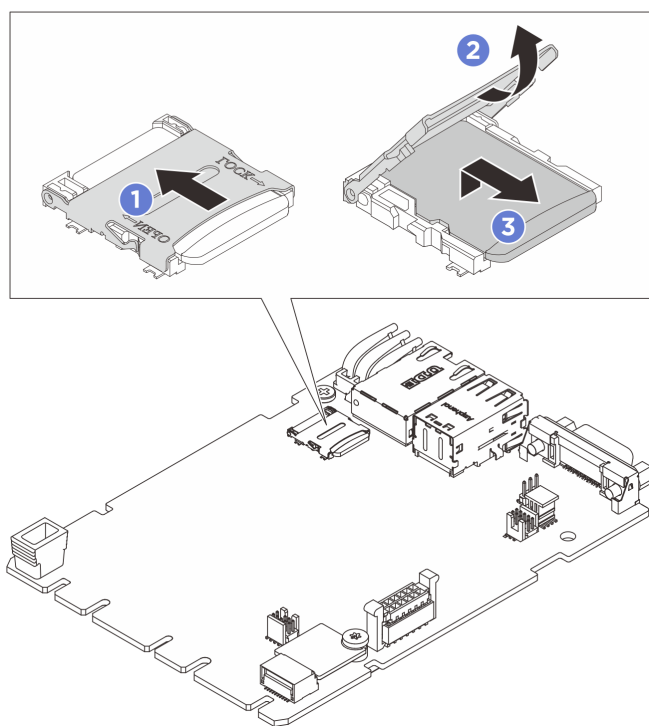
図 167. microSD カードの取り外し
