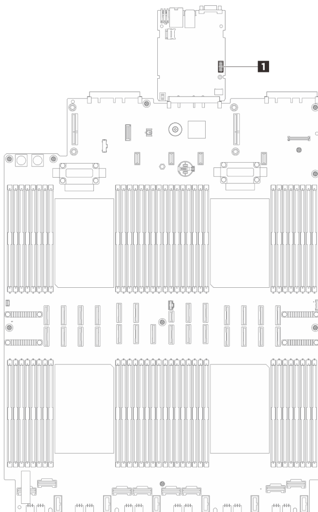
図284. シリアル・ポート・モジュールの接続
