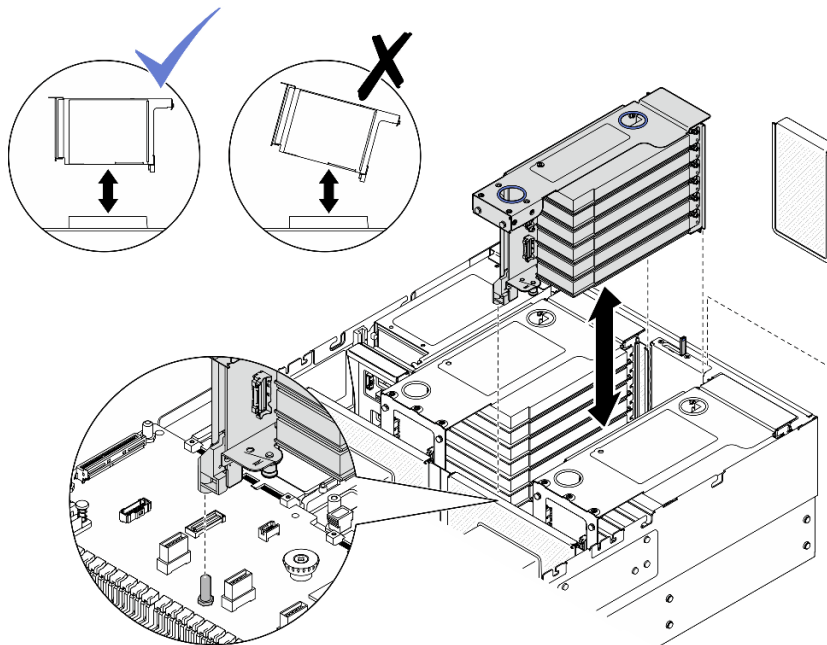
図 175. PCIe ライザー 2 の取り外し
