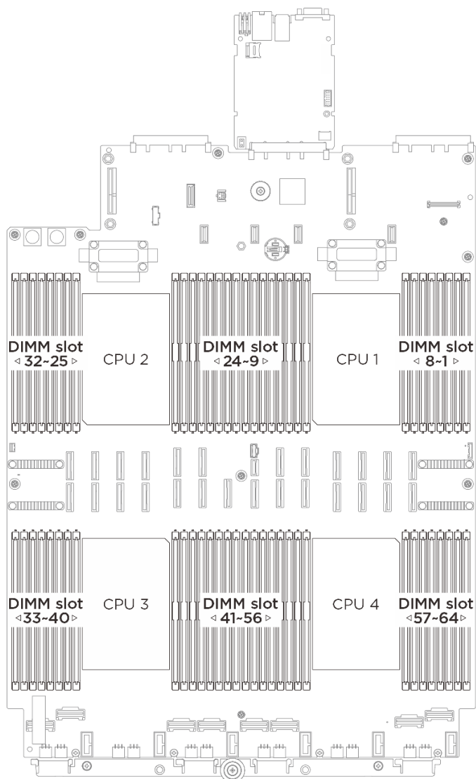
図 164. メモリー・モジュールおよびプロセッサのレイアウト
