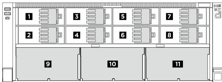
図 3. バックプレーン番号
