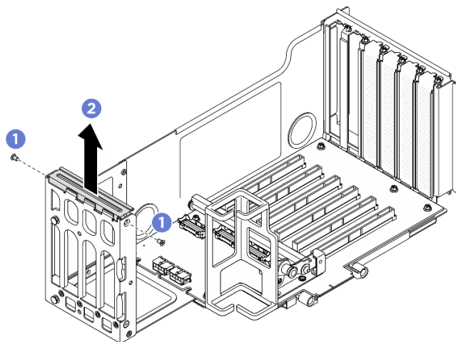
図 75. ライザー・エクステンダー・カバーの取り外し
