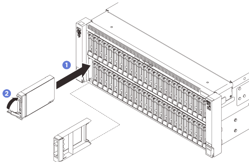
図 6. 2.5 インチ ドライブの取り付け
