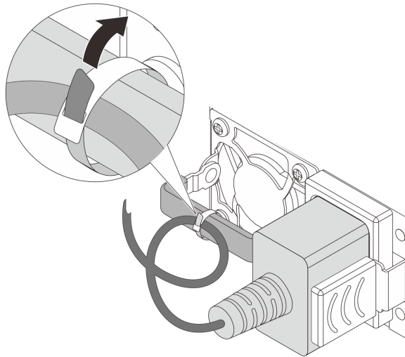
図 232. 電源コードの配線と結び付け
