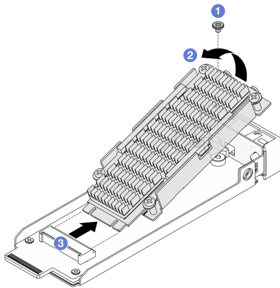
図 254. ヒートシンク付き M.2 ドライブを取り外す
