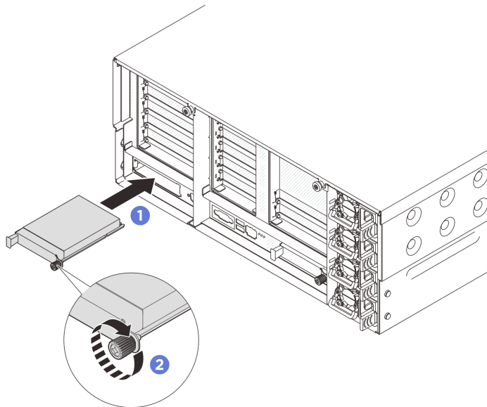
図 171. OCP モジュールの取り付け
