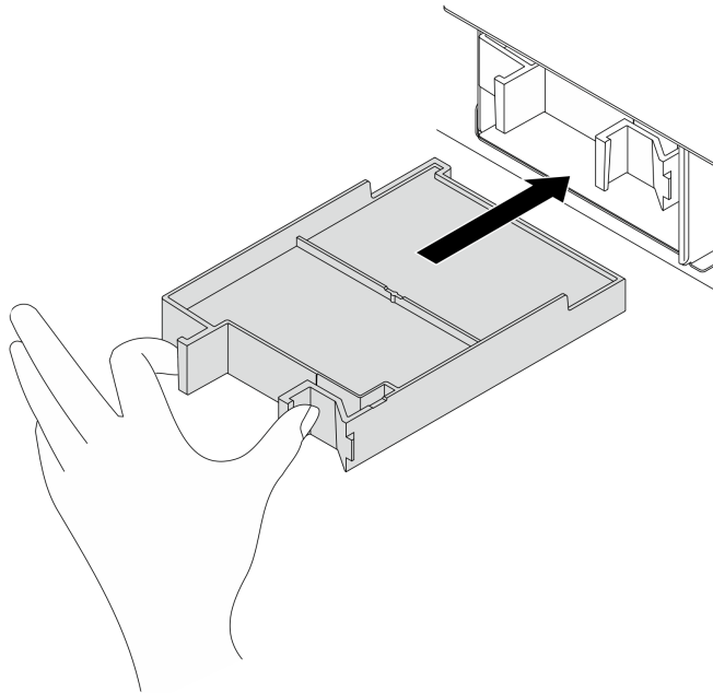
図 55. CMM ベイ・フィラーの取り付け
