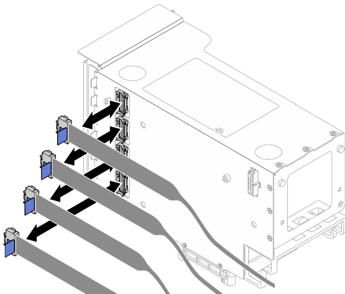
図 206. ライザーの外側への PCIe ライザー・ケーブルの接続
