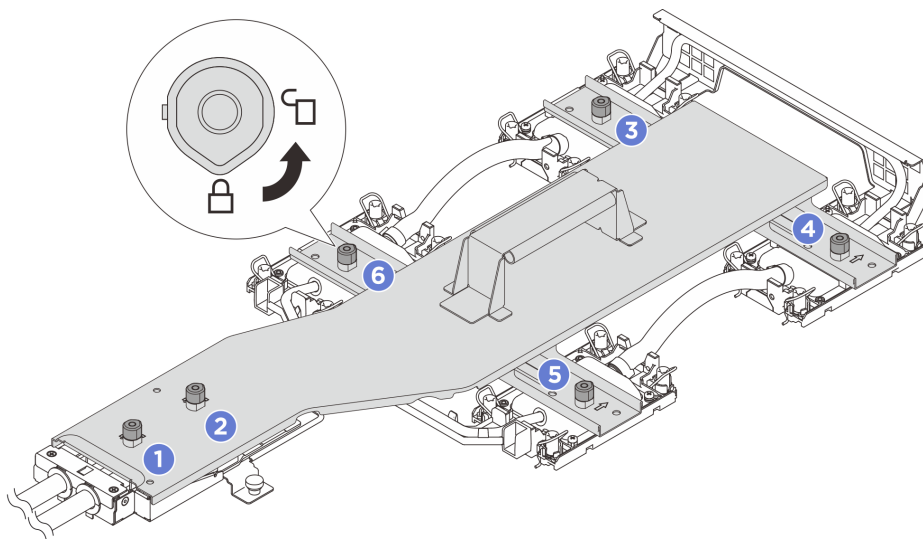
図 109. コールド・プレート・キャリアを緩める
