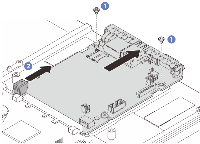
図 287. システム I/O ボードの取り外し
