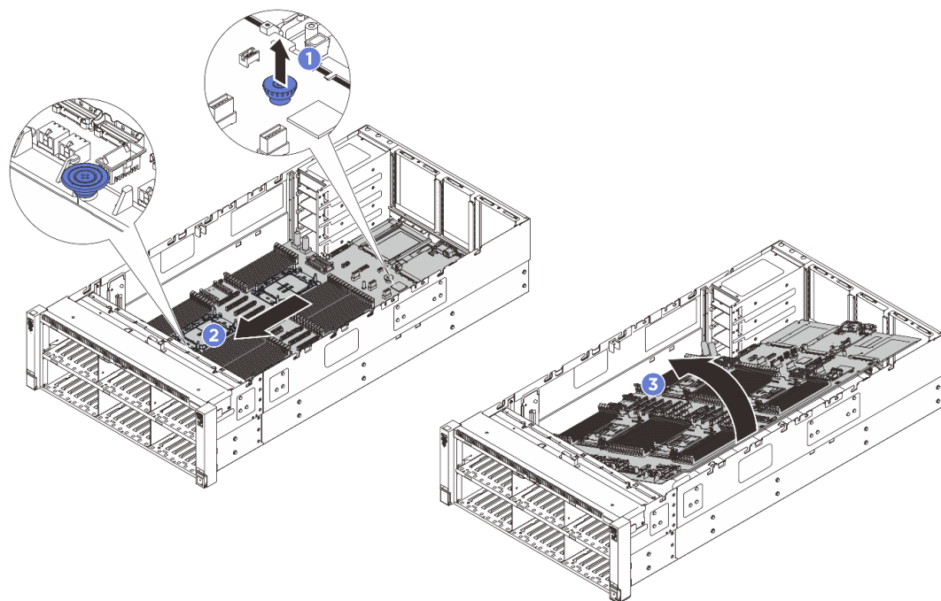
図 286. システム・ボード・アセンブリーの取り外し
