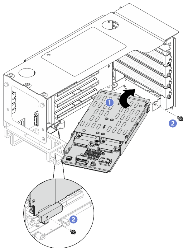
図 273. ライザーへの M.2 ドライブ・ケージの取り付け
