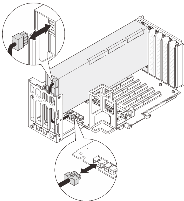
図 76. GPU アダプターからの電源ケーブルの切り離し
