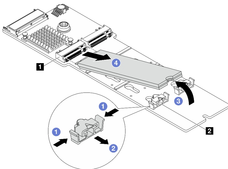
図 87. M.2 ドライブの取り外し
