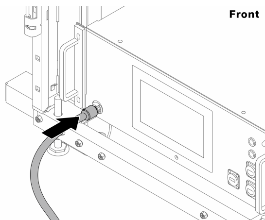
図 134. CDU の正面
