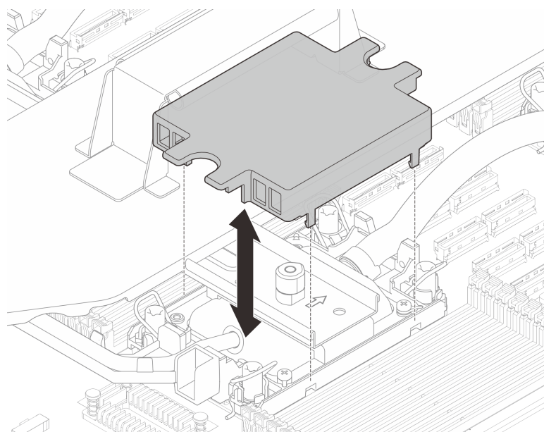
図111. コールド・プレート・カバーの取り付け
