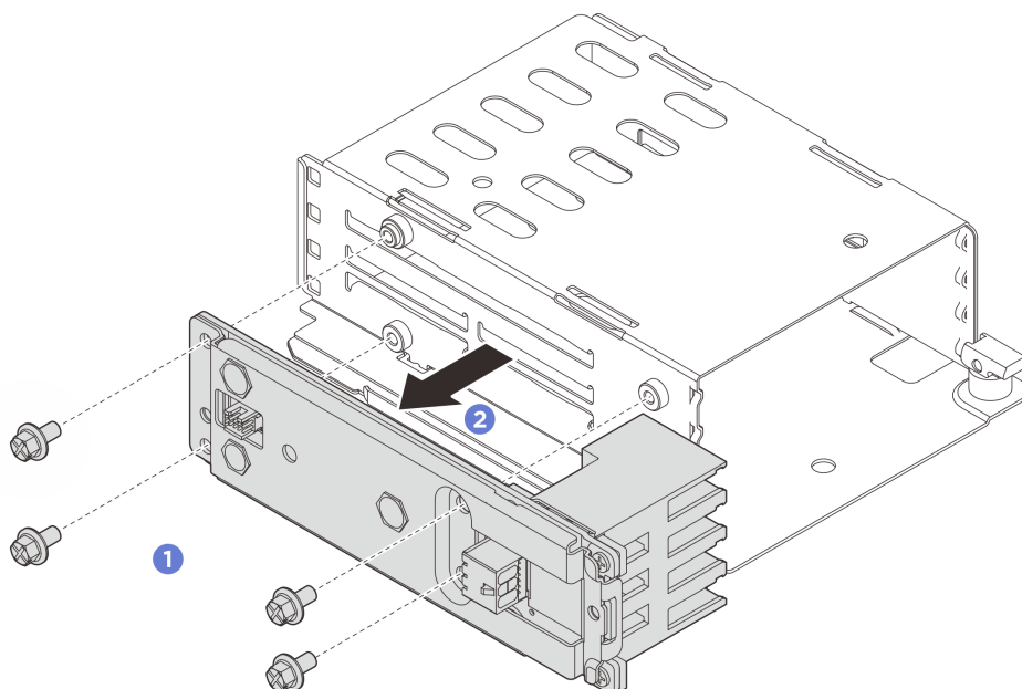
図 50. バックプレーン・アセンブリーの取り外し
