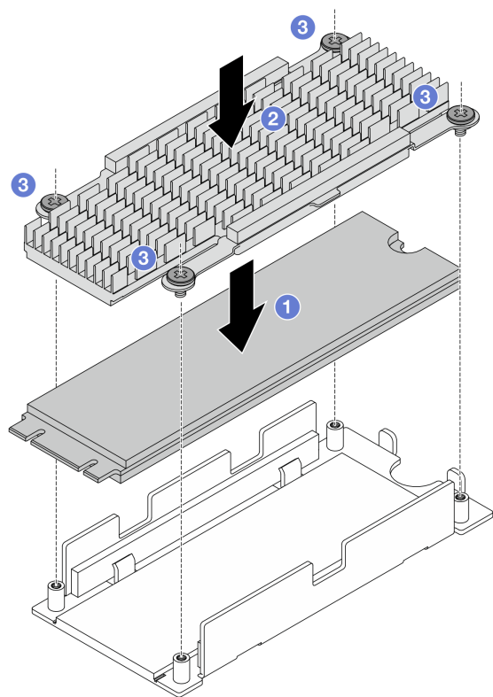
図 259. ヒートシンクと M.2 ドライブの組み立て
