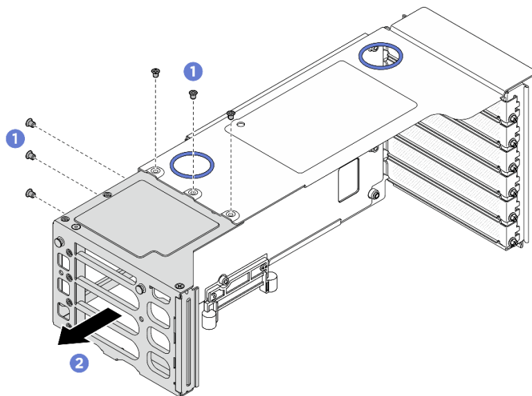
図 214. FH PCIe ライザー・ケージからのライザー・エクステンダーの取り外し
