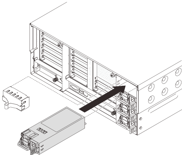
図 231. パワー・サプライ・ユニットの取り付け
