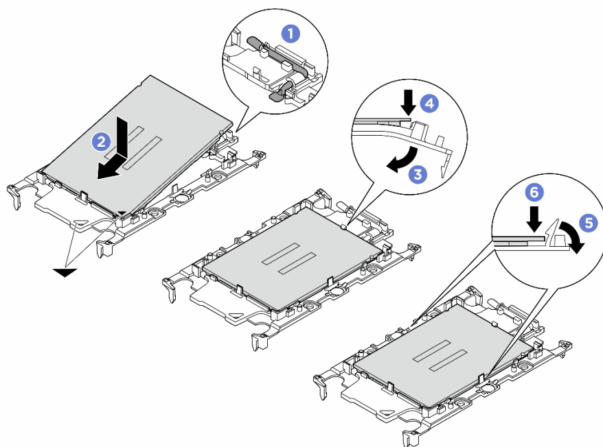
図 239. プロセッサ・キャリアの取り付け
