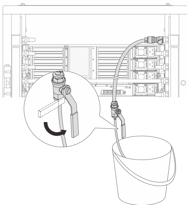
図 159. リターン側のブリーダー・バルブを開く
