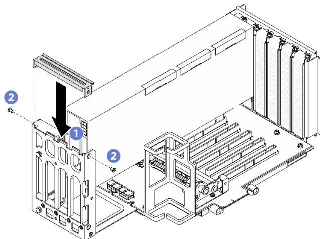
図 78. ライザー・エクステンダー・カバーの取り付け
