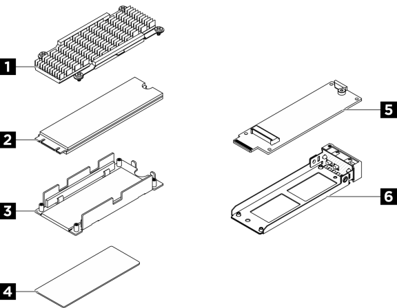
図 249. ホット・スワップ M.2 ドライブ・アセンブリーの部品
