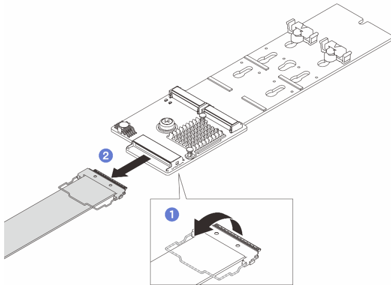
図 89. M.2 バックプレーン・ケーブルの取り外し
