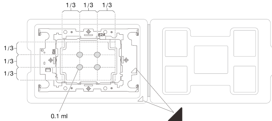
図 240. 配送トレイのプロセッサで熱伝導グリースを塗布する
