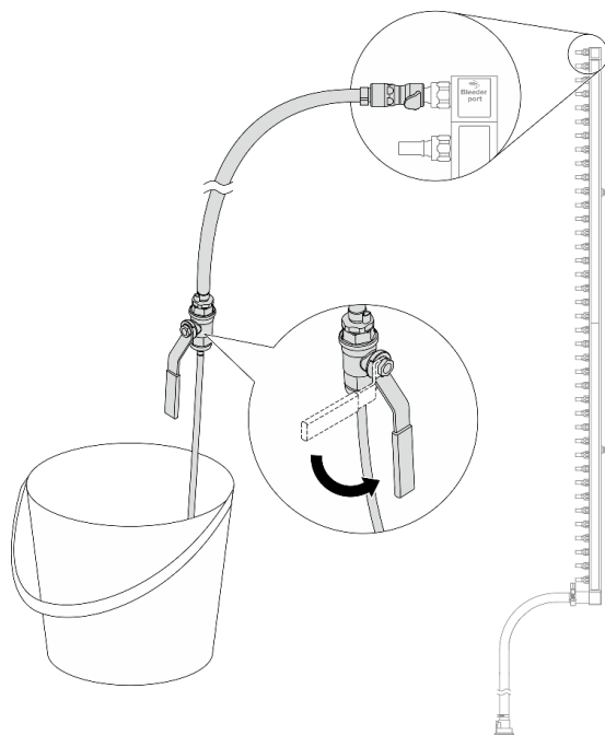
図 149. ブリーダー・バルブを開く
