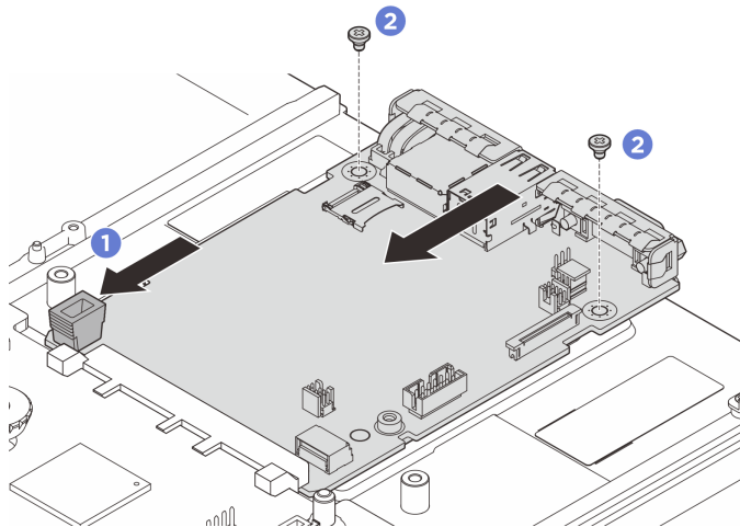
図 288. システム I/O ボードの取り付け
