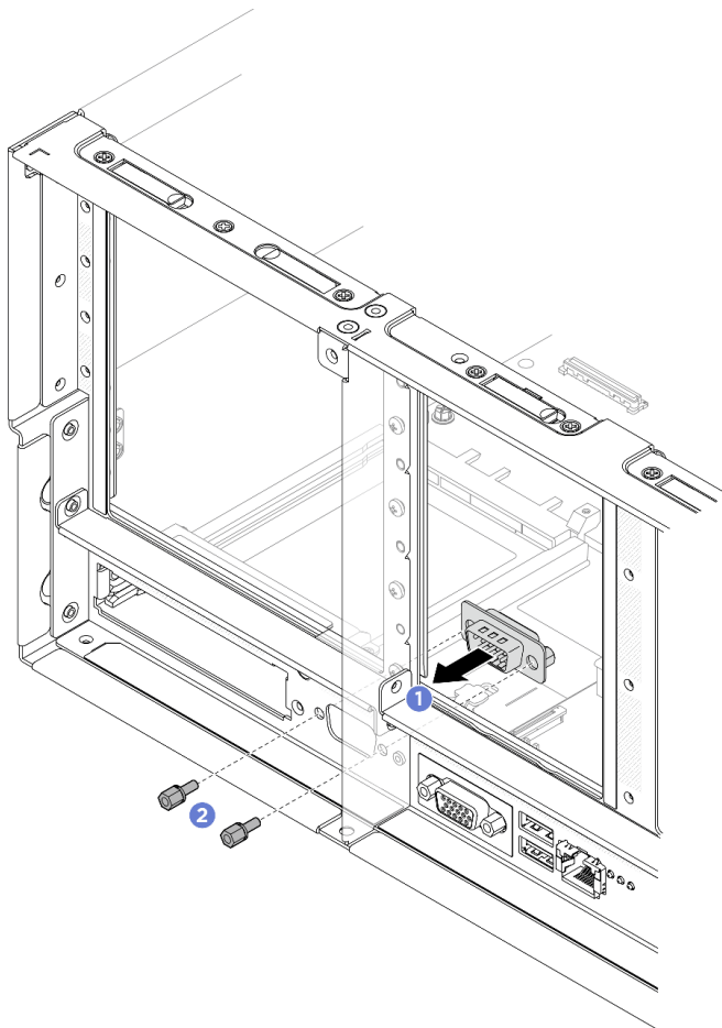
図 283. シリアル・ポート・モジュールの取り付け
