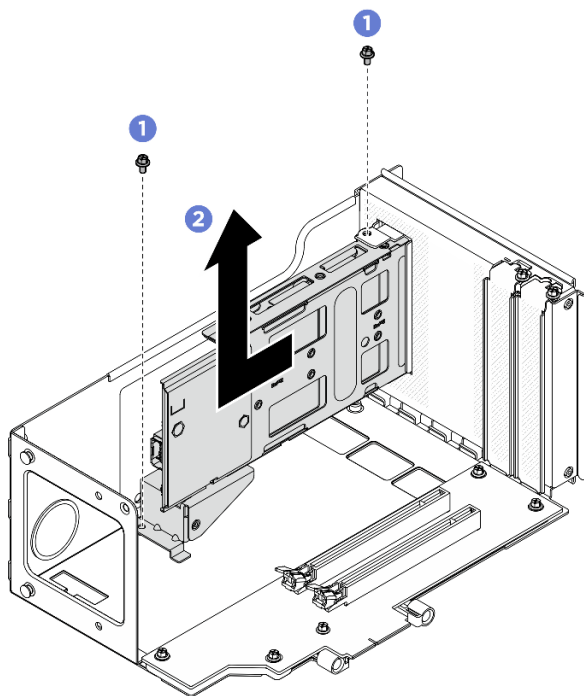
図 262. ライザーからの M.2 ドライブ・ケージの取り外し
