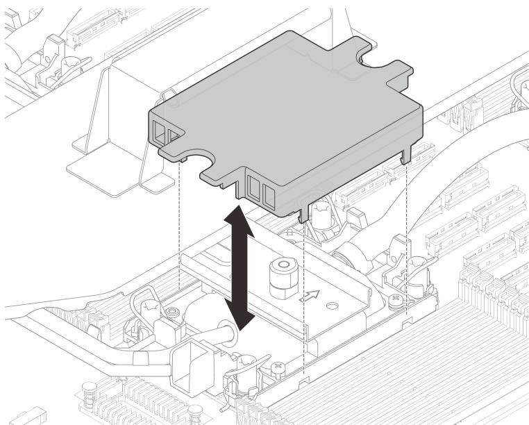
図97. コールド・プレート・カバーの取り外し
