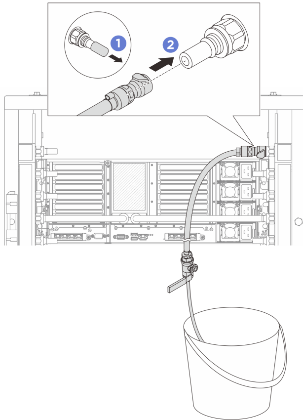
図 157. リターン側へのブリーダー・キットの取り付け
