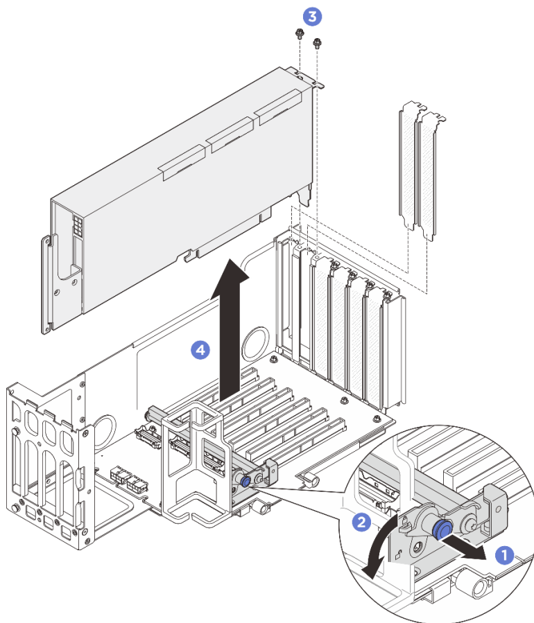
図 77. PCIe ライザーからの GPU アダプターの取り外し
