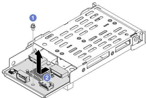
図 263. M.2 バックプレーンの取り外し
