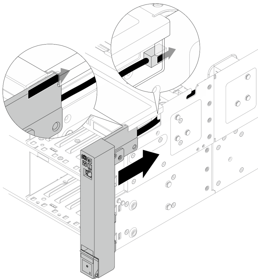
図 247. ラック・ラッチの取り付け
