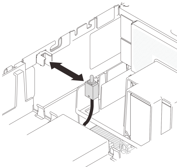
図 85. 侵入検出スイッチの取り付け
