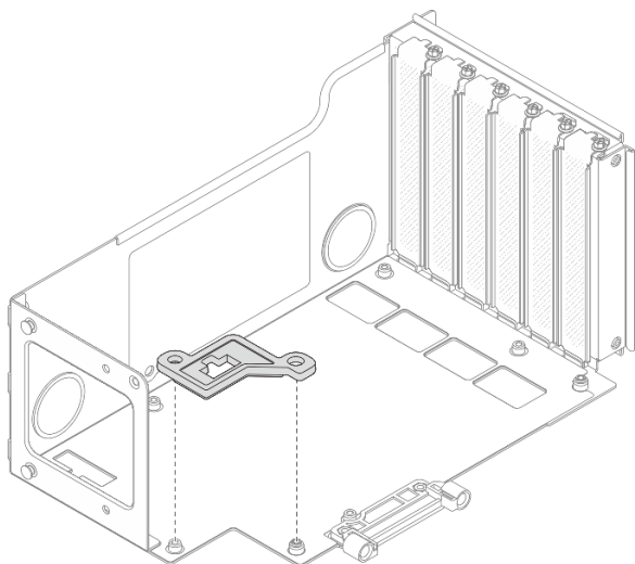
図199. ライザー・ケージへのコネクタ・ガイドの取り付け
