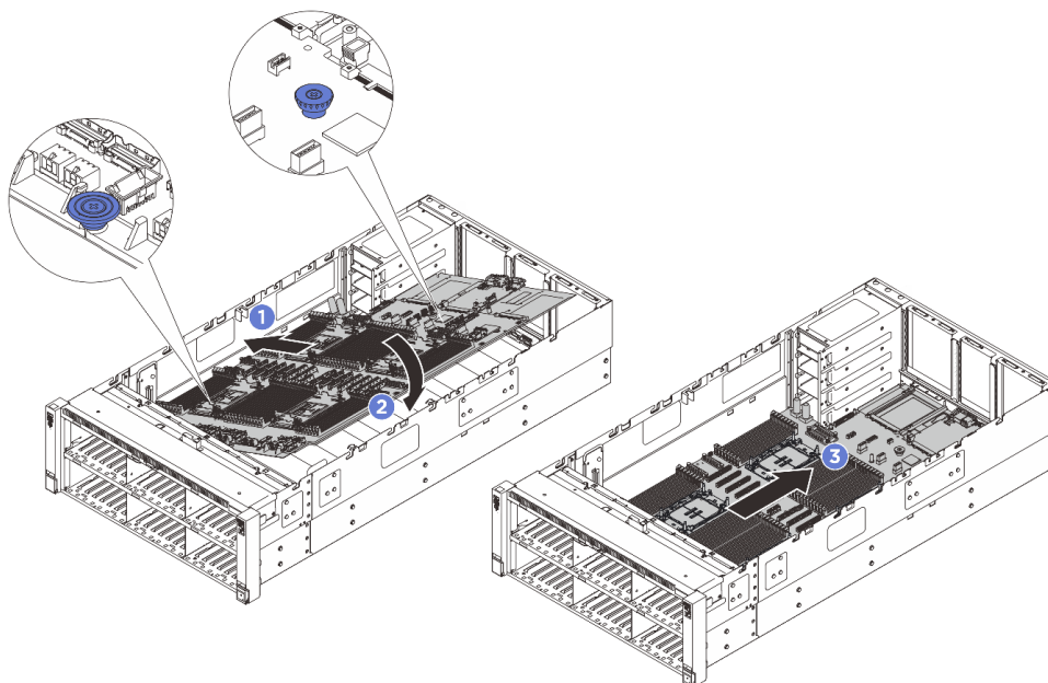
図 289. システム・ボード・アセンブリーの取り付け
