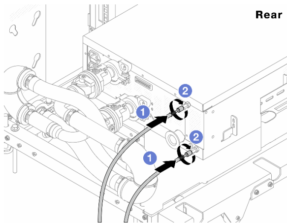
図 135. CDU の背面
