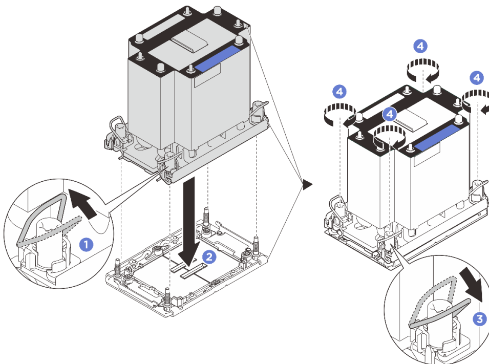
図 242. 2U 標準 PHM の取り付け
