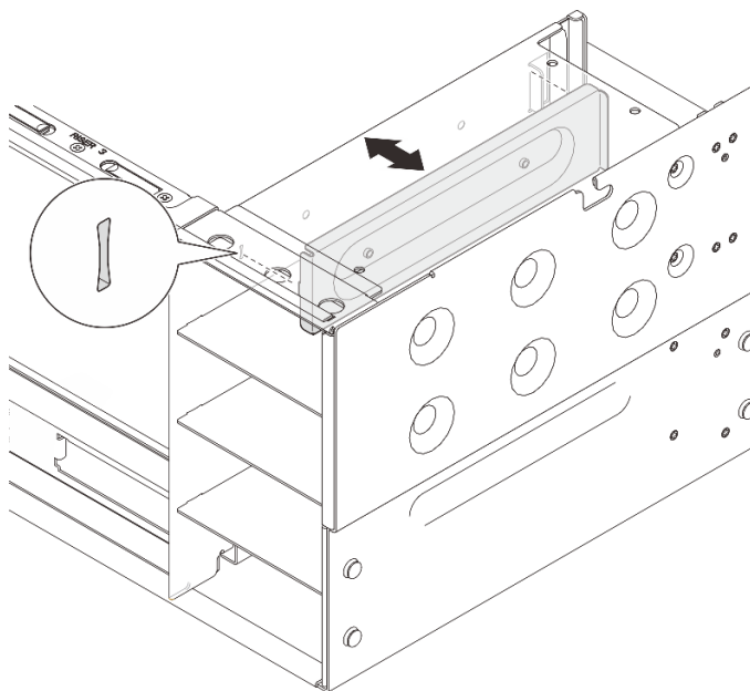
図 226. パワー・サプライ・ブラケットの取り外し
