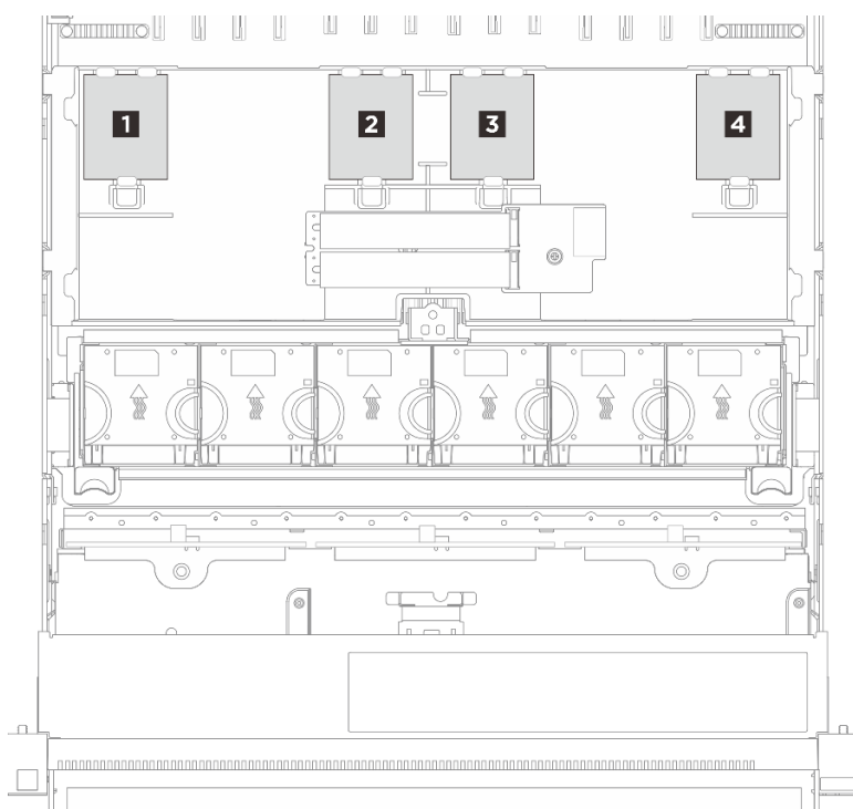
図 72. フラッシュ電源モジュールの位置
