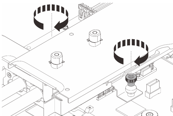
図 107. コールド・プレート・アセンブリーの取り付け
