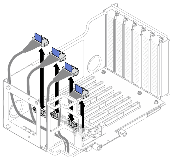
図 204. ライザーの内側への PCIe ライザー・ケーブルの接続
