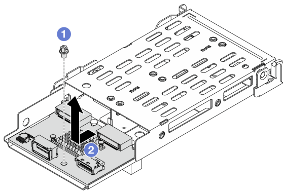
図 266. M.2 バックプレーンの取り外し
