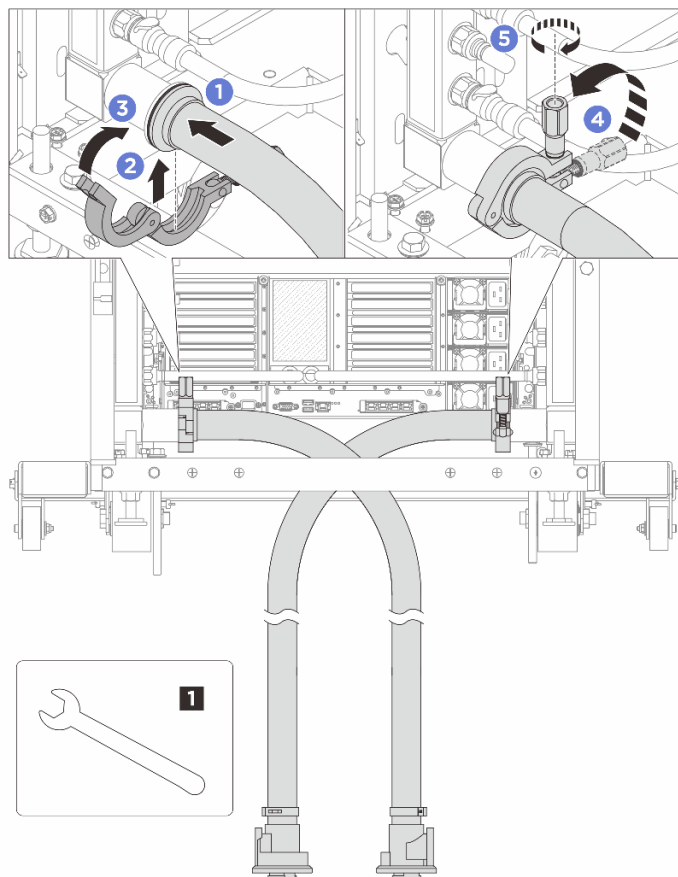
図 153. ホース・キットの取り付け
