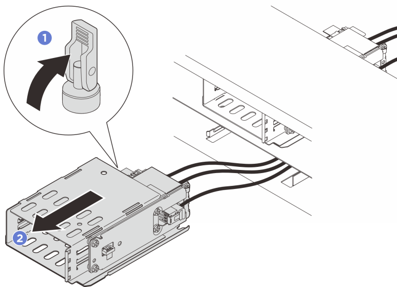
図 49. E3.S 1T ケージの取り外し
