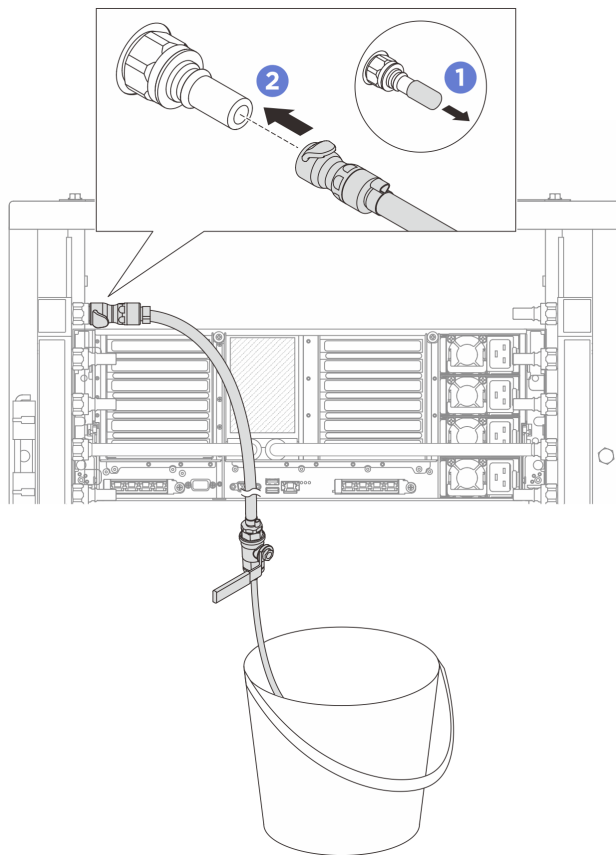
図 137. 供給側へのブリーダー・キットの取り付け
