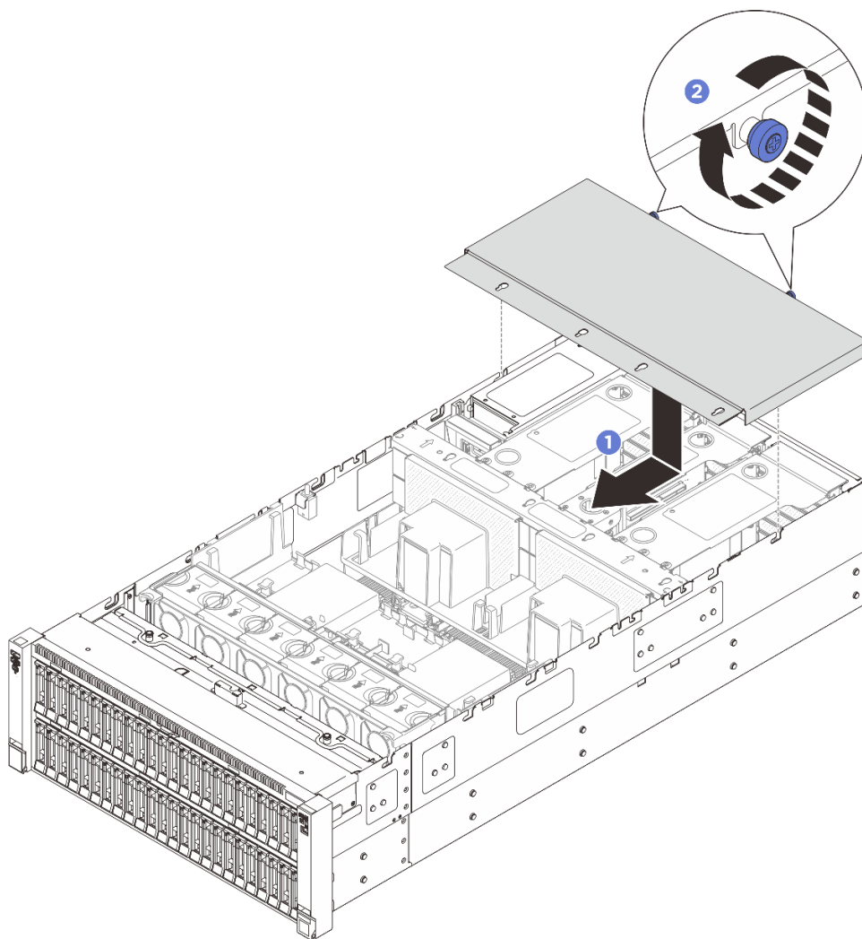
図 297. 背面トップ・カバーの取り付け
