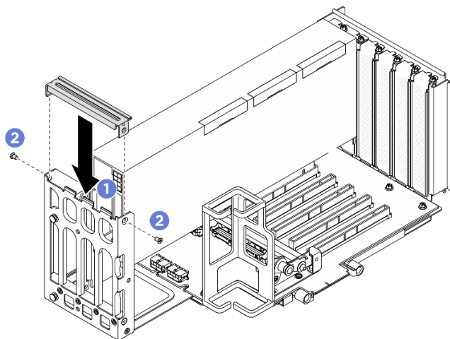
図 82. ライザー・エクステンダー・カバーの取り付け
