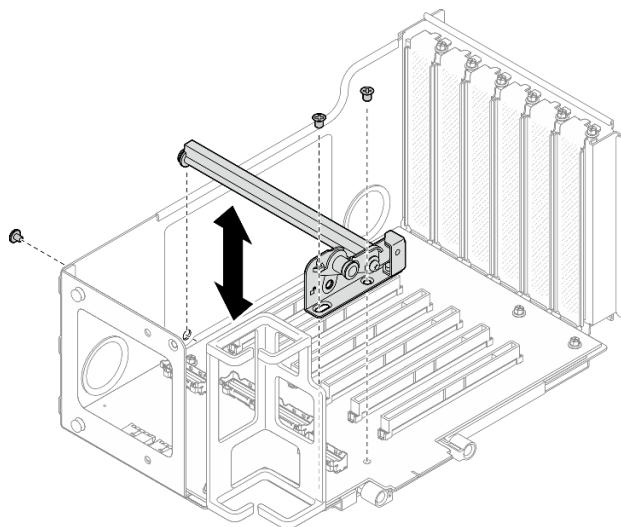
図 203. ライザー・ケージへの PCIe 保持具の取り付け
