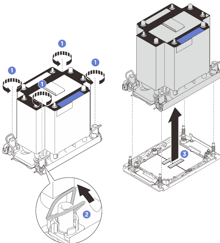
図 234. 3U 標準 PHM の取り外し
