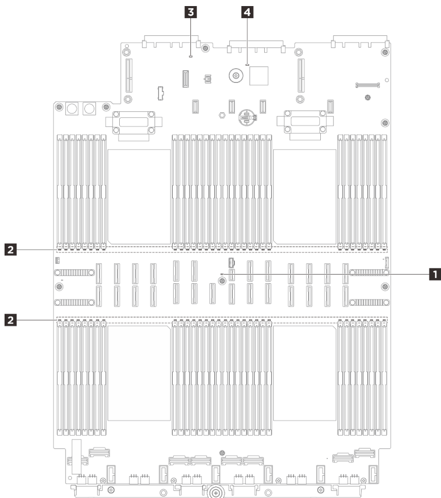
図 310. プロセッサ・ボード LED
