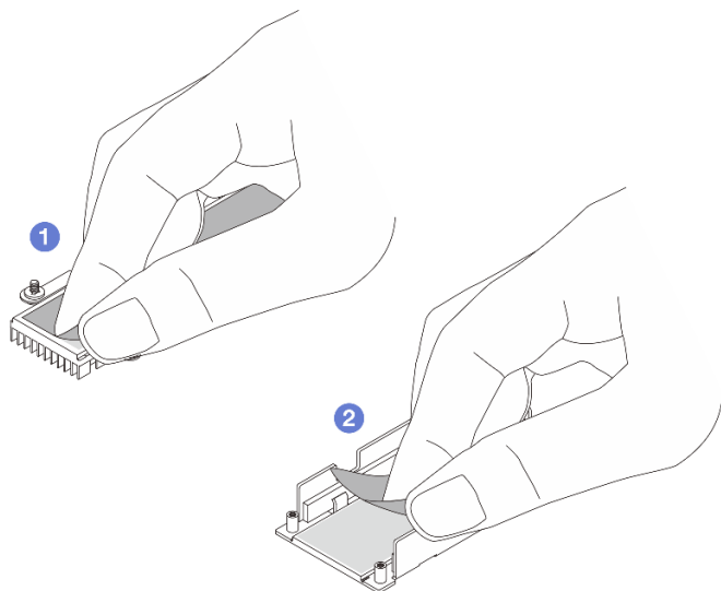
図 258. フィルムをはがす
