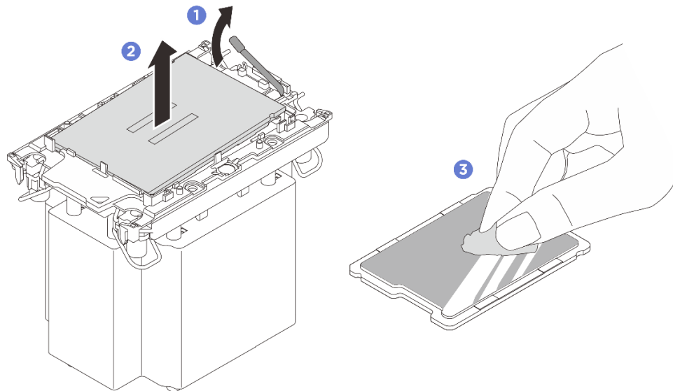
図 236. プロセッサをキャリアとヒートシンクから取り外す
