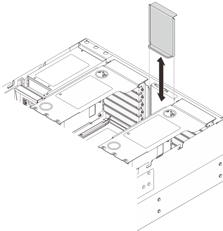
図96. ライザー・フィルターの取り外し
