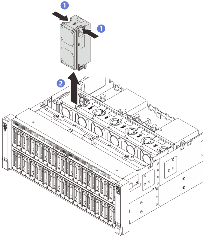
図 66. ファンの取り外し
