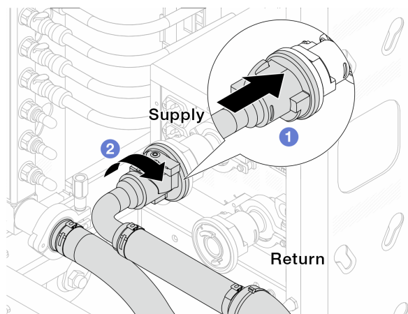
図 133. ボール・バルブの接続
