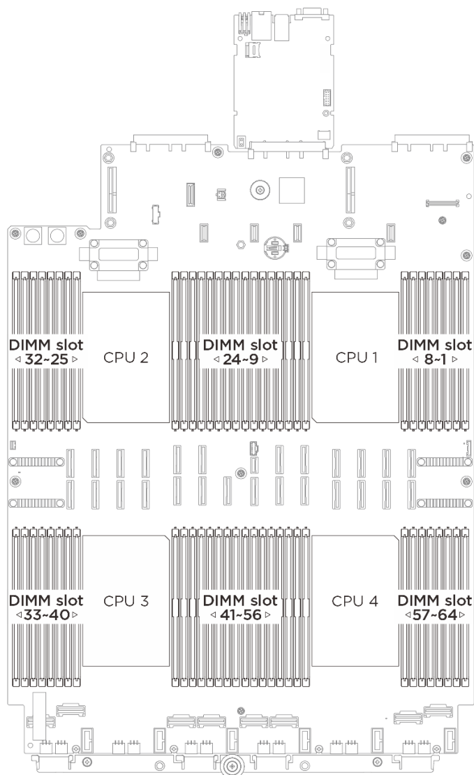
図 162. メモリー・モジュールおよびプロセッサのレイアウト
