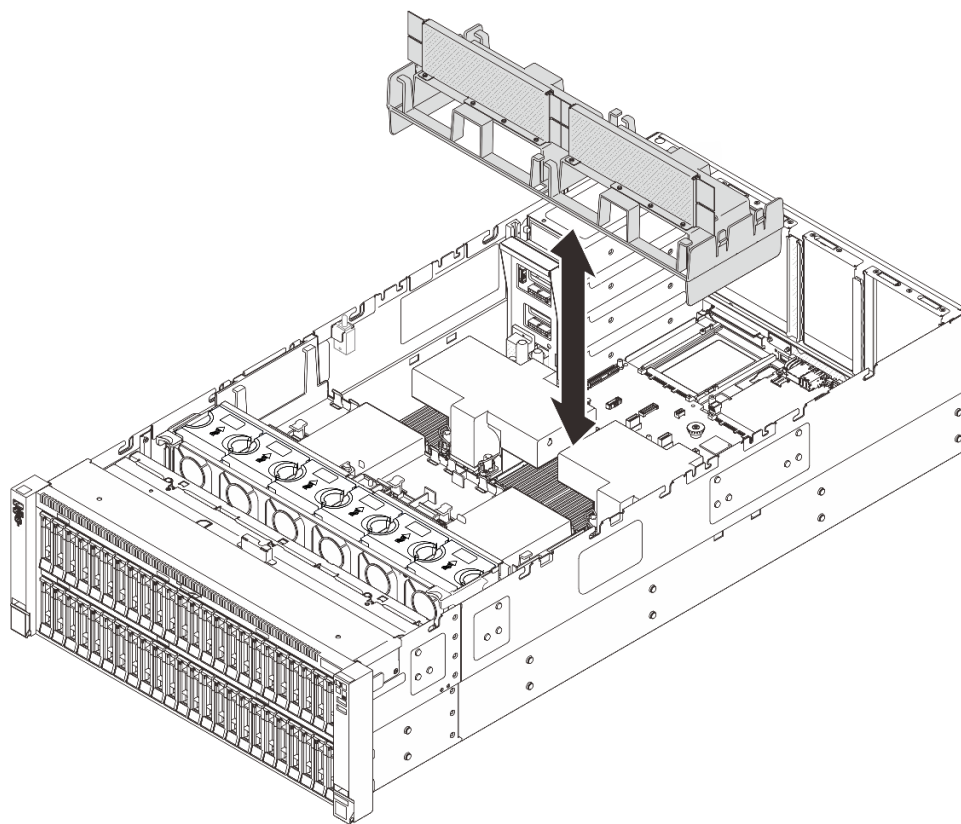
図 27. 2U パフォーマンス PHM 用背面エアー・バッフルの取り外し
