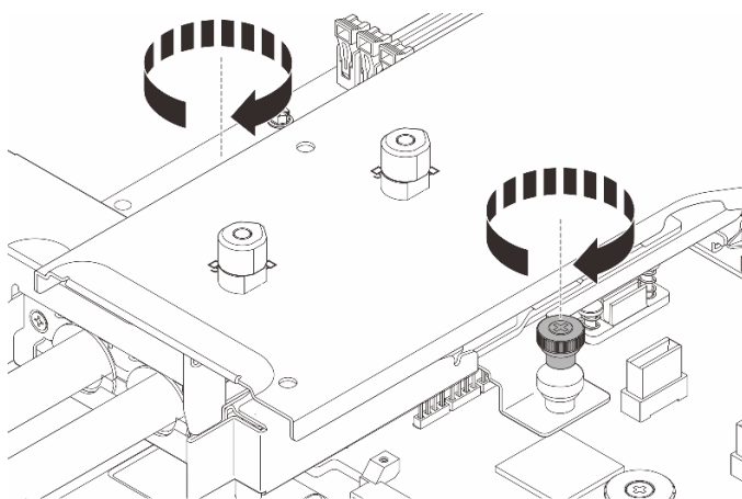
図 101. コールド・プレート・アセンブリーの取り外し
