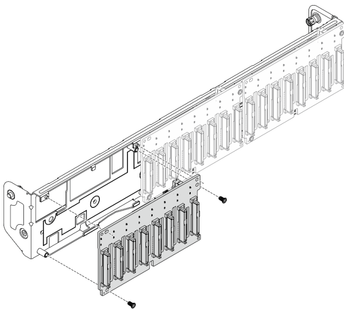
図 14. バックプレーンのキャリアへの取り付け (E3.S ベイ・シャーシ)
