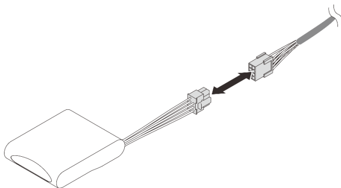
図 17. フラッシュ電源モジュールからのケーブルの切り離し
