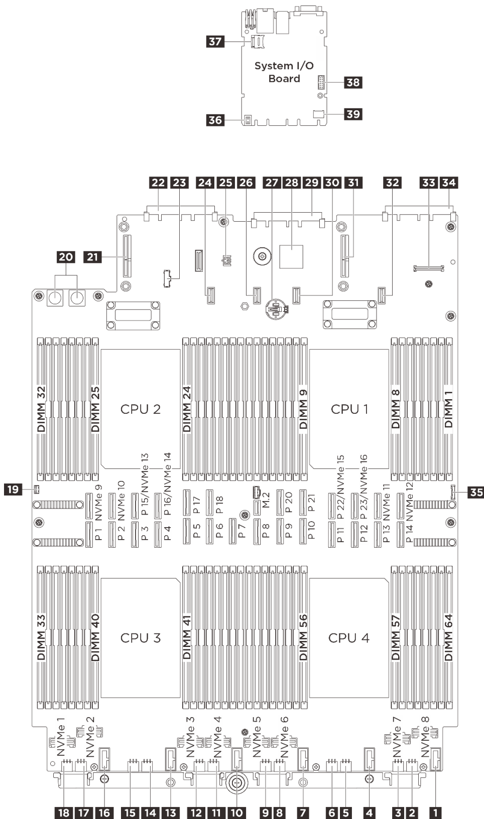
図 304. システム・ボード・アセンブリー・コネクタ
