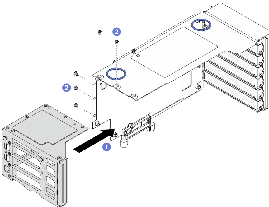
図 217. FH PCIe ライザーへの PCIe ライザー・エクステンダーの取り付け
