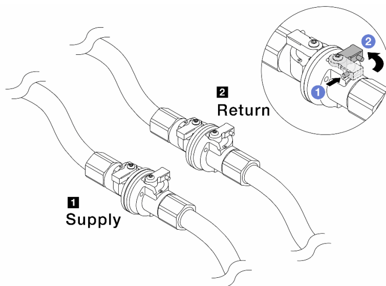
図 143. ボール・バルブを閉じる
