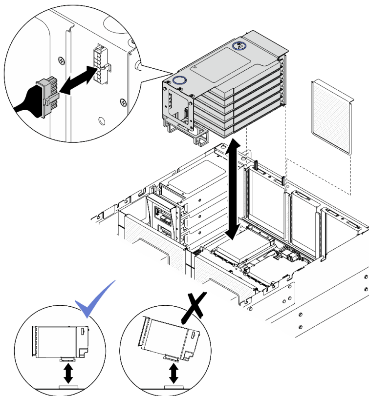
図 176. PCIe ライザー 3 の取り外し
