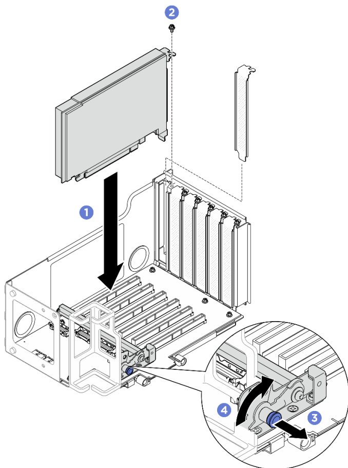
図 181. PCIe アダプターの PCIe ライザーへの取り付け
