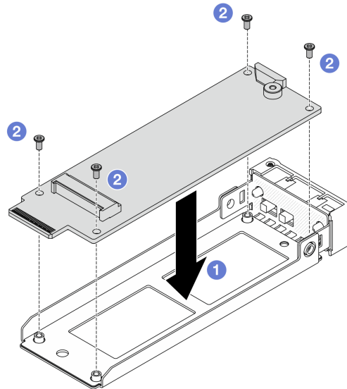
図 260. M.2 変換コネクタの取り付け
