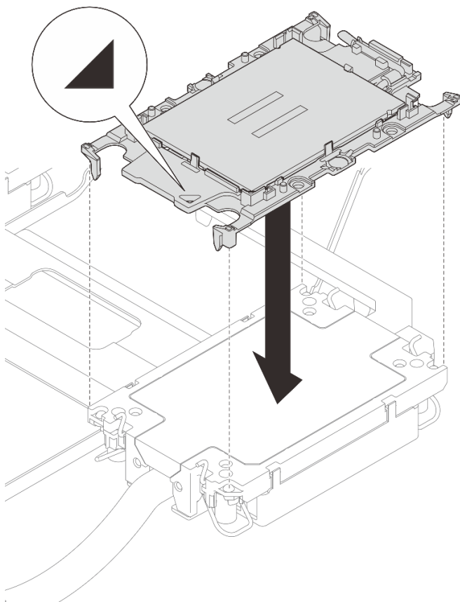
図 105. コールド・プレートへのプロセッサの取り付け
