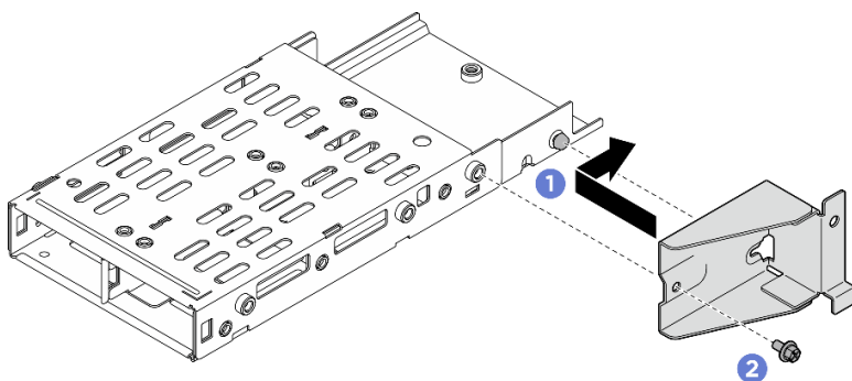
図 269. M.2 ドライブ・ケージ・ブラケットを取り付ける
