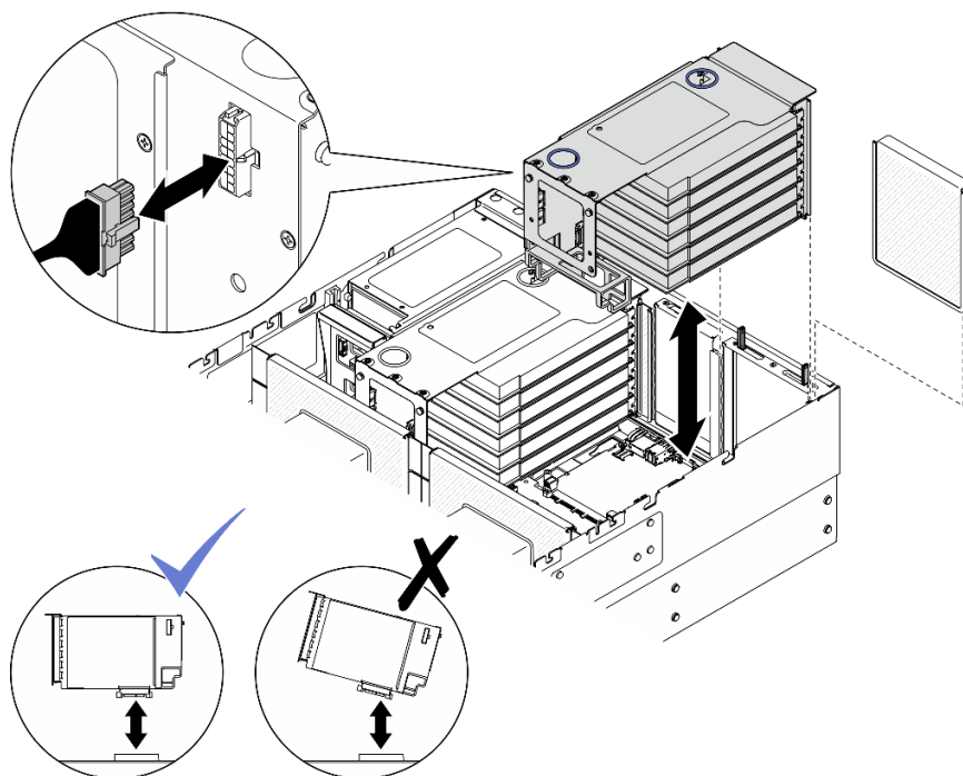
図 184. PCIe ライザー 1 の取り付け
