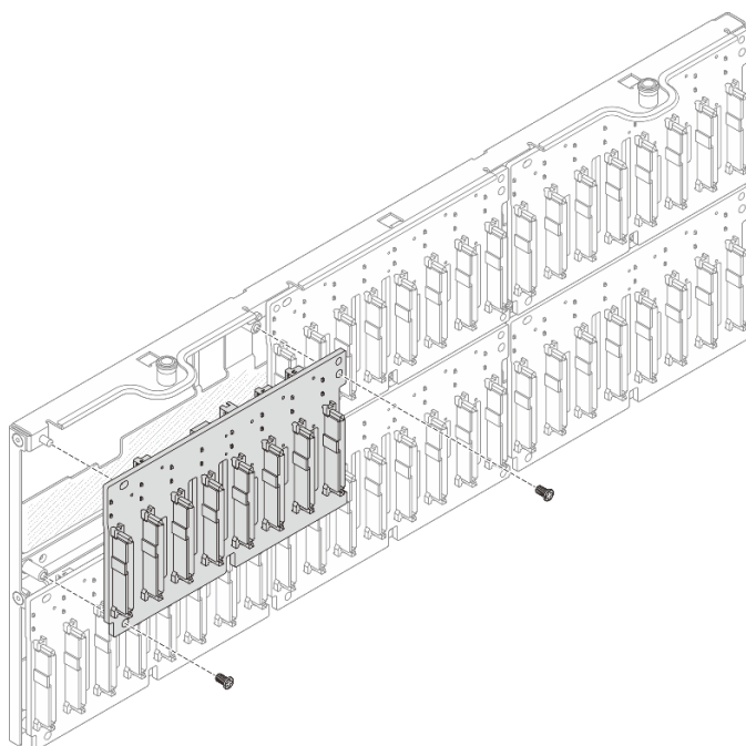
図9. キャリアからのバックプレーンの取り外し (2.5 インチ ベイ・シャーシ)
