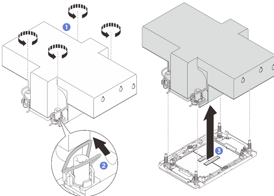
図 235. 2U パフォーマンス PHM の取り外し
