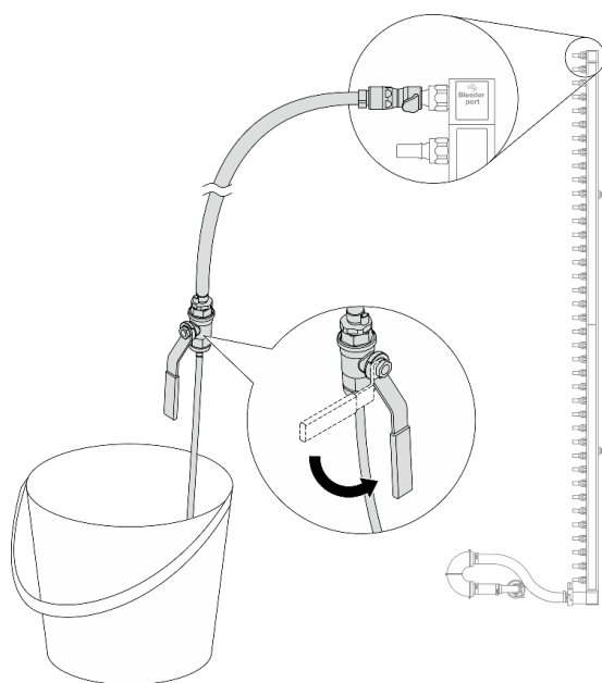
図 127. ブリーダー・バルブを開く
