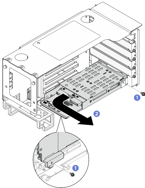
図 265. 6 スロット FH ライザーからの M.2 ドライブ・ケージの取り外し
