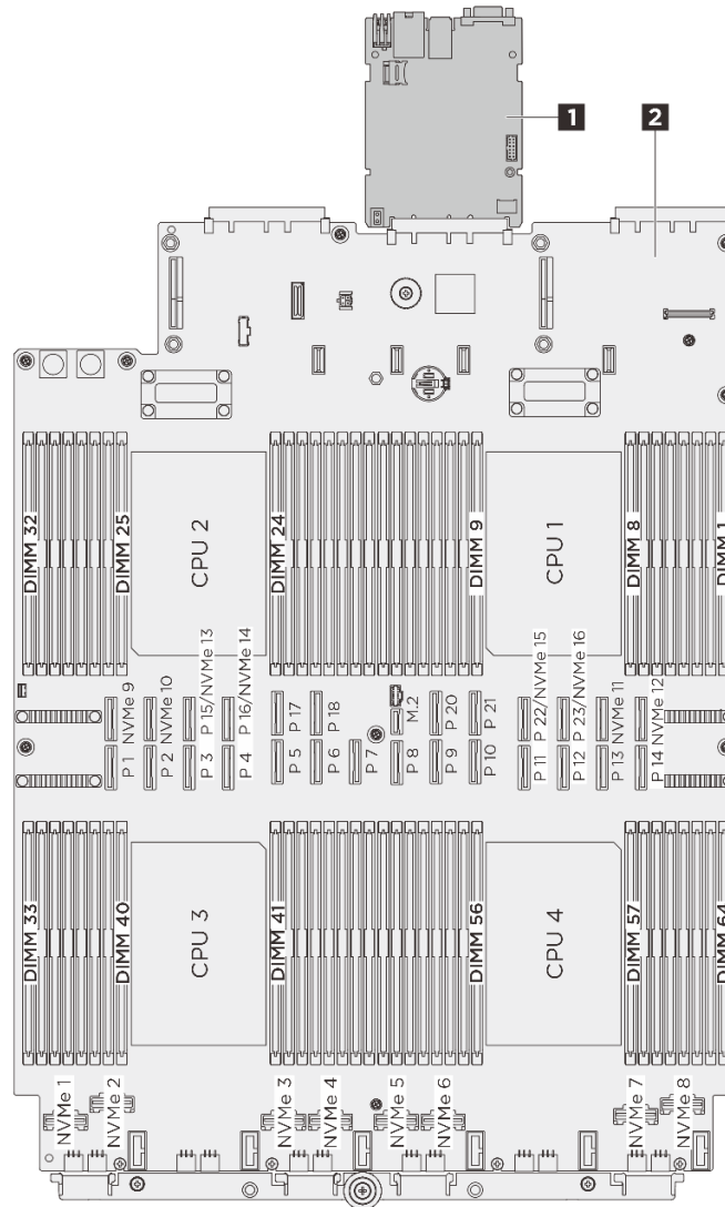
図 285. システム・ボード・アセンブリーのレイアウト
