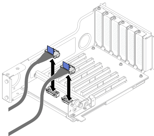
図 196. ライザーの内側からの PCIe ライザー・ケーブルの切り離し
