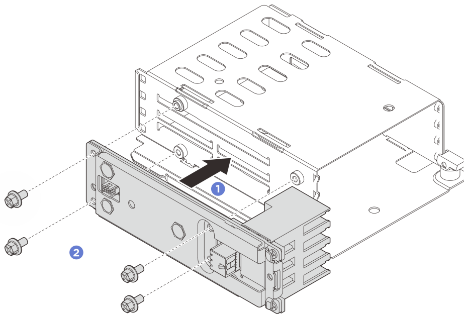
図 51. バックプレーン・アセンブリーの取り付け
