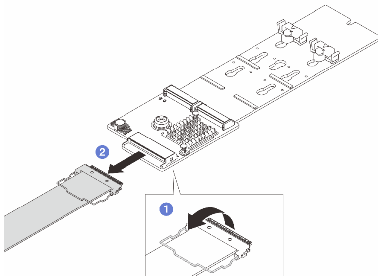
図 18. M.2 バックプレーン・ケーブルの取り外し
