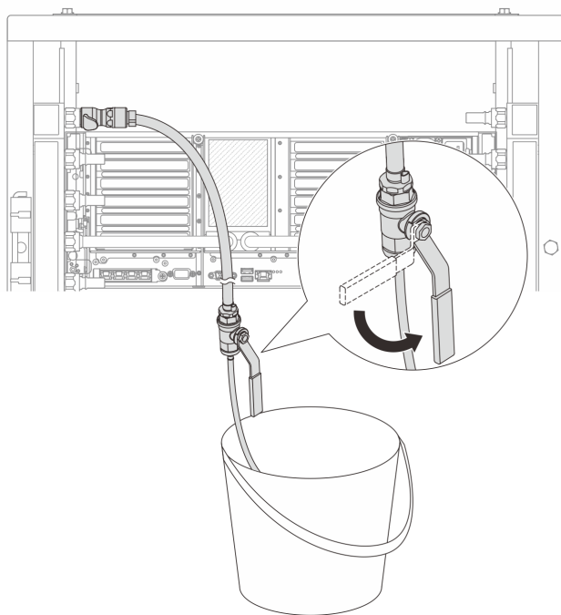
図 142. 供給側のブリーダーのバルブを開く
