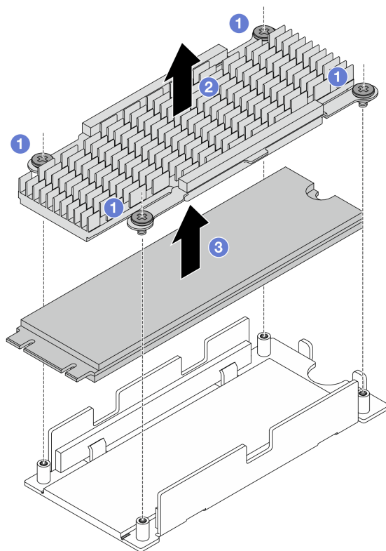
図 256. M.2 ドライブとヒートシンクの分離
