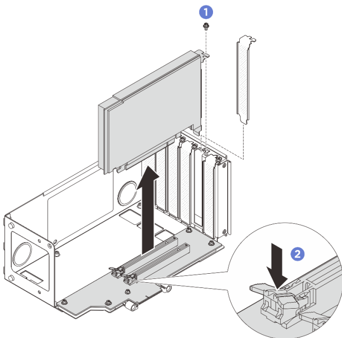
図 177. ライザーからの PCIe アダプターの取り外し
