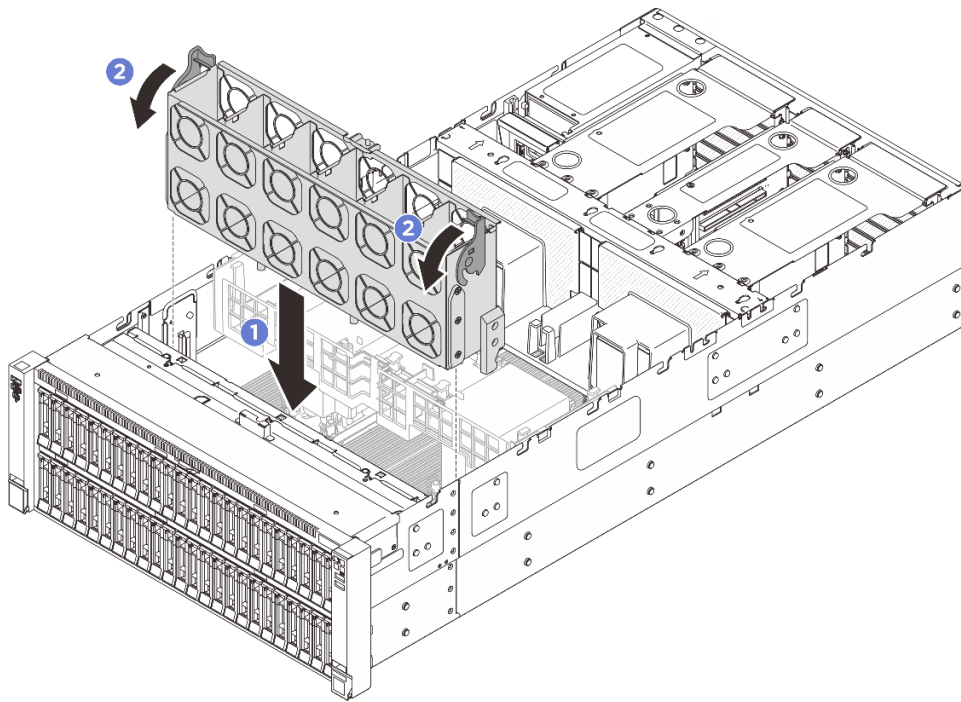
図 68. ファン・ケージの取り付け
