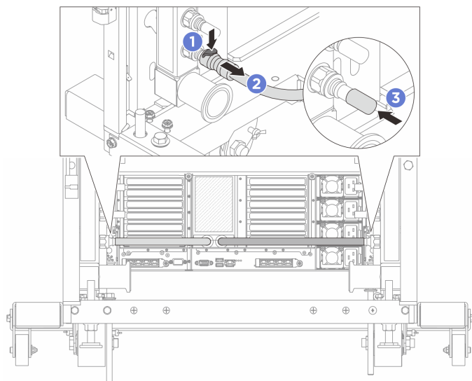
図 144. クイック・コネクト・プラグの取り外し
