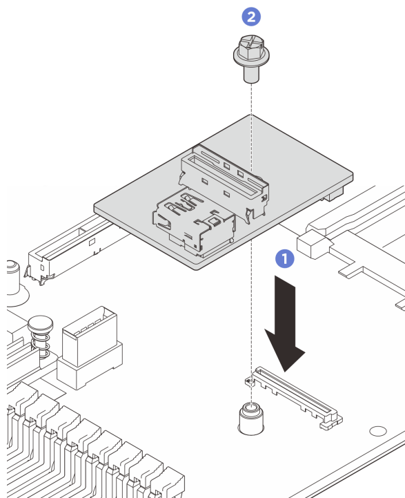
図 301. USB I/O ボードの取り付け
