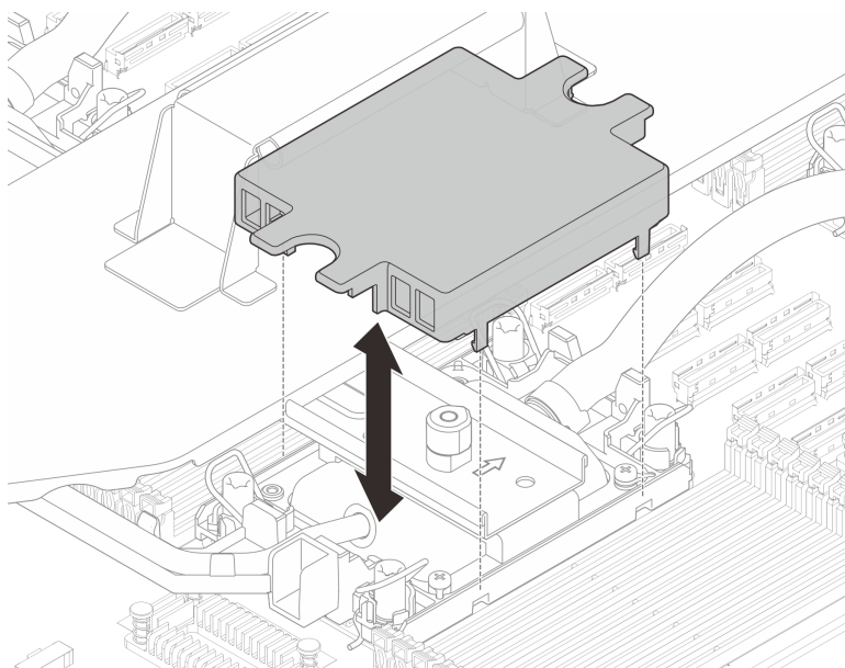
図319. コールド・プレート・カバーの取り外し
