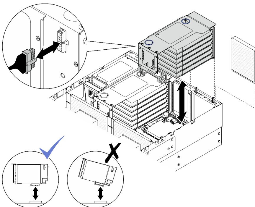
図 174. PCIe ライザー 1 の取り外し
