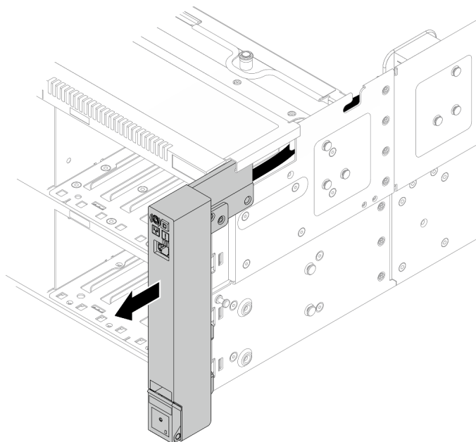
図246. ラック・ラッチの取り外し
