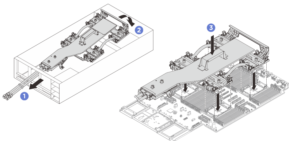
図 106. コールド・プレート・アセンブリーの取り付け
