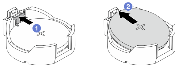
図 32. CMOS バッテリーの取り外し
