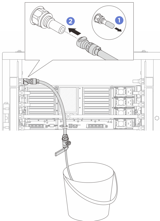
図 154. 供給側へのブリーダー・キットの取り付け
