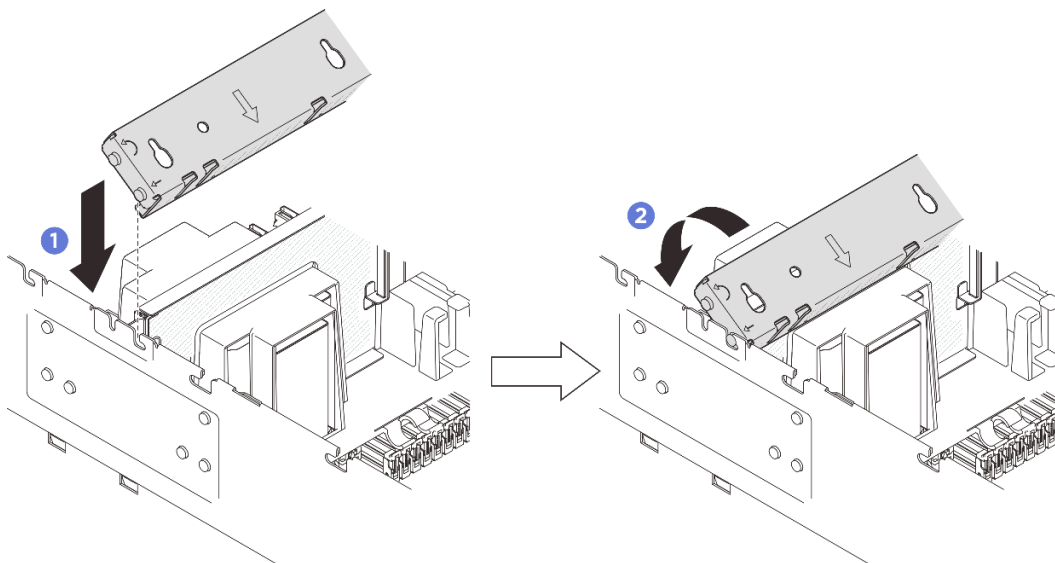
図 39. クロス・バーの取り付け
