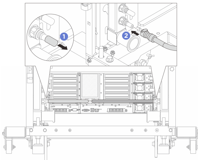
図 152. クイック・コネクト・プラグの取り付け
