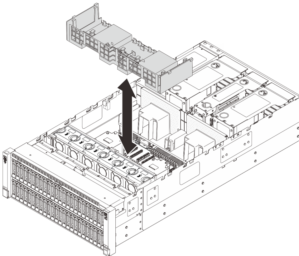
図 20. 前面エアー・バッフルの取り外し
