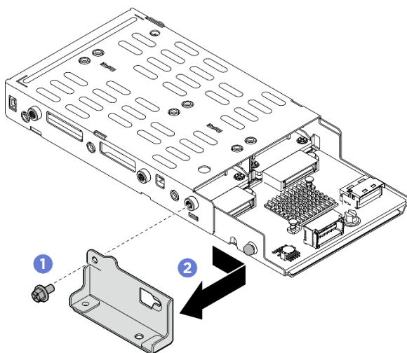
図 267. M.2 ドライブ・ケーシング・ブラケットの取り外し
