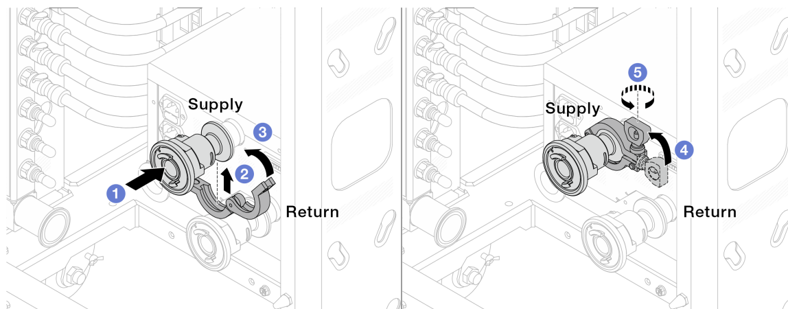
図 131. ボール・バルブの取り付け
