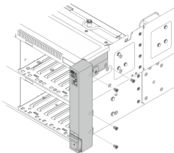
図 248. ねじの取り付け
