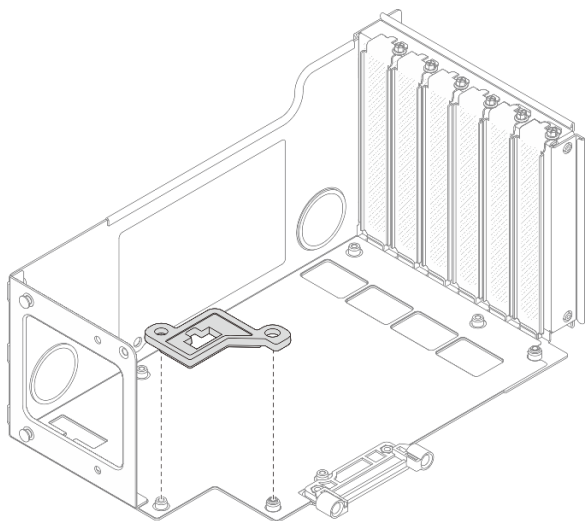
図 187. ライザー・ケージからのコネクタ・ガイドの取り外し
