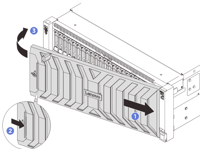
図 277. セキュリティー・ベゼルの取り付け
