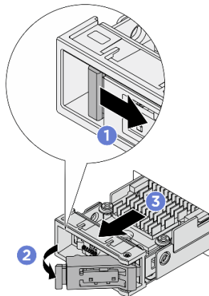
図 250. ホット・スワップ M.2 ドライブ・アセンブリーの取り外し
