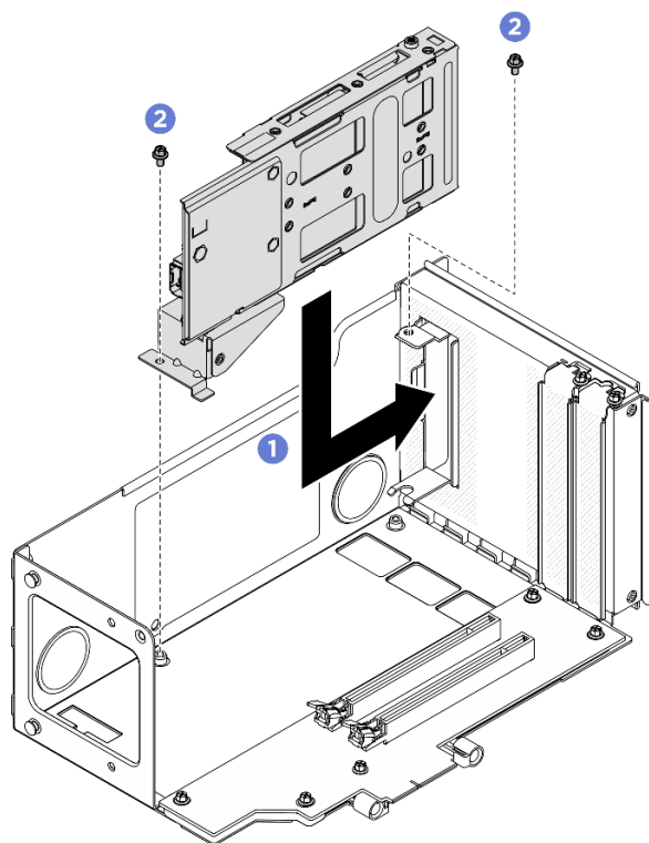
図 270. ライザーへの M.2 ドライブ・ケージの取り付け
