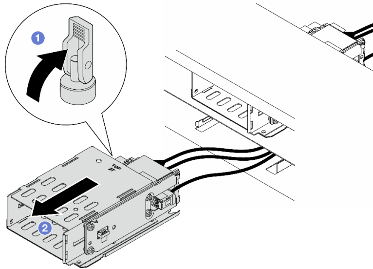
図 62. E3.S 2T ケージの取り外し
