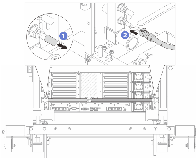
図 136. クイック・コネクト・プラグの取り付け
