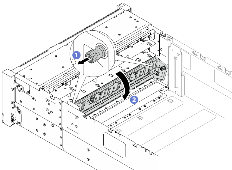
図8. ドライブ・バックプレーン・キャリア・アセンブリーの取り外し (E3.S ベイ・シャーシ)
