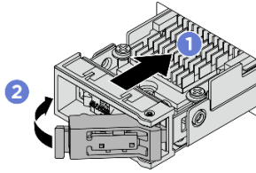
図 253. M.2 ドライブ・アセンブリーの取り付け
