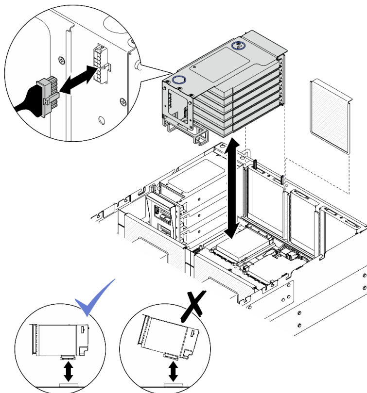
図 183. PCIe ライザー 3 の取り付け
