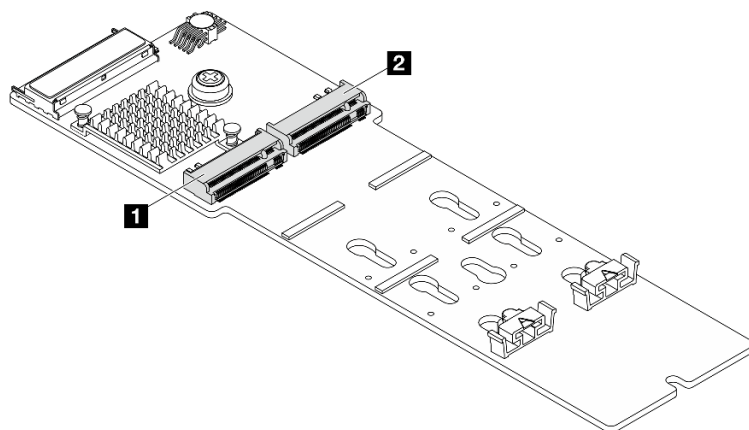
図 92. M.2 ドライブ・スロット
