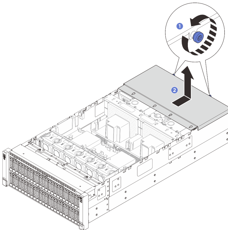
図 296. 背面トップ・カバーの取り外し
