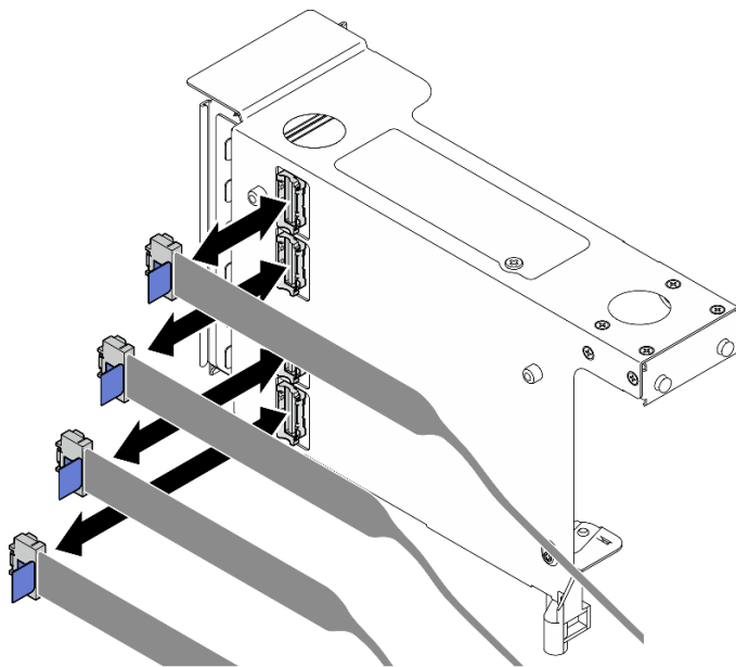
図 195. ライザーの外側からの PCIe ライザー・ケーブルの切り離し
