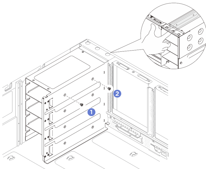
図 225. パワー・サプライ・ブラケットねじの取り外し
