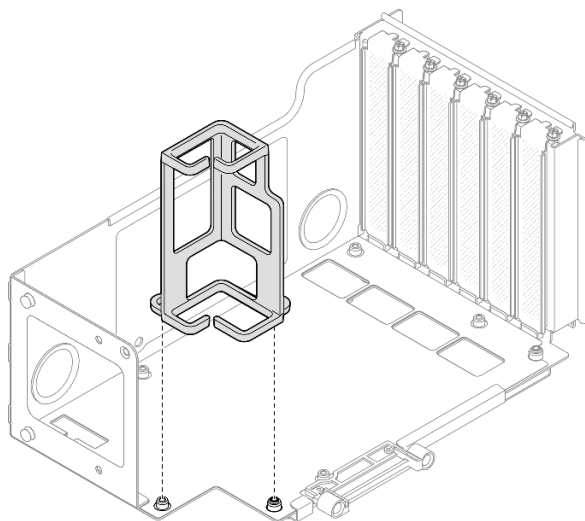
図 201. ライザー・ケージへのケーブル保持具の取り付け
