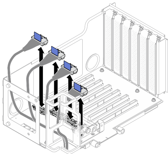
図 190. ライザーの内側からの PCIe ライザー・ケーブルの切り離し
