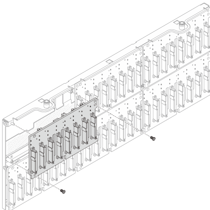
図 13. バックプレーンのキャリアへの取り付け (2.5 インチ ベイ・シャーシ)
