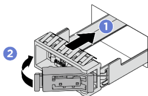
図 251. M.2 ドライブ・トレイの取り付け
