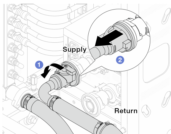
図 122. 接続セットの取り外し
