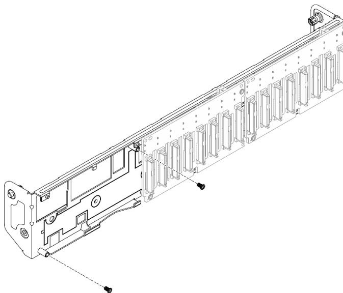
図 12. バックプレーン・キャリアのスペアねじ (E3.5 ベイ・シャーシ)
