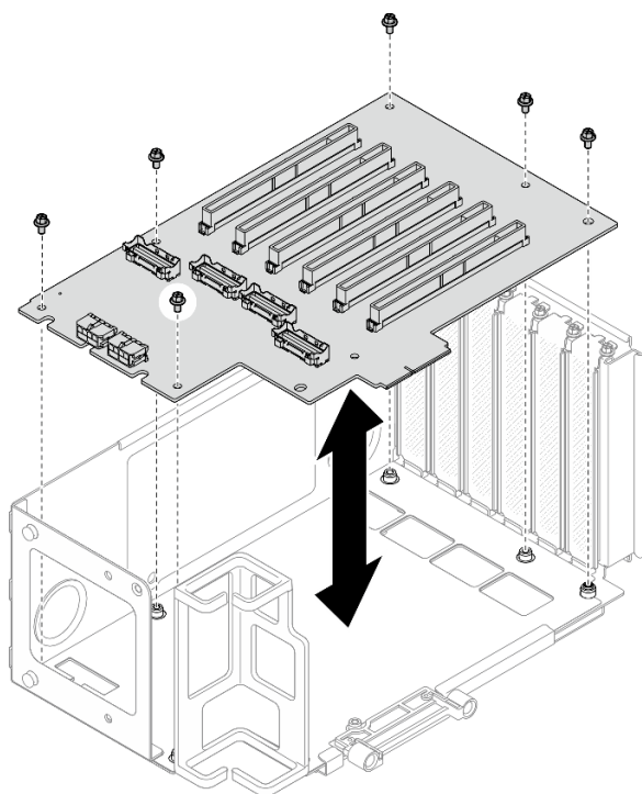
図 202. ライザー・ケージへの PCIe ライザー・カードの取り付け
