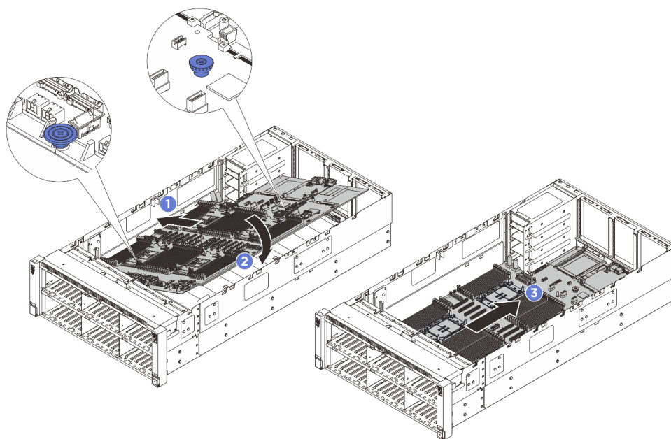
図 293. システム・ボード・アセンブリーの取り付け
