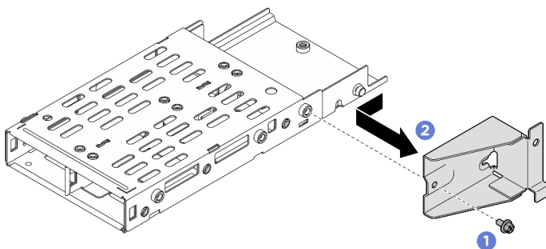
図 264. M.2 ドライブ・ケージ・ブラケットの取り外し
