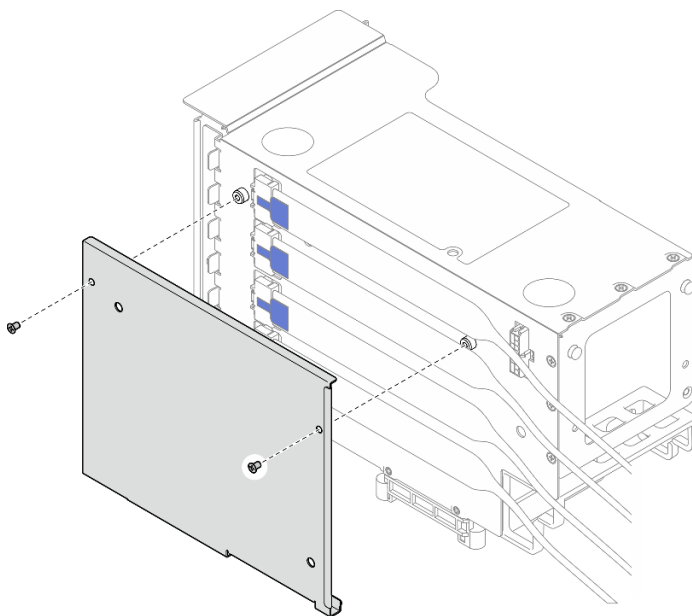
図 207. ライザー・ケージへのカバーの取り付け
