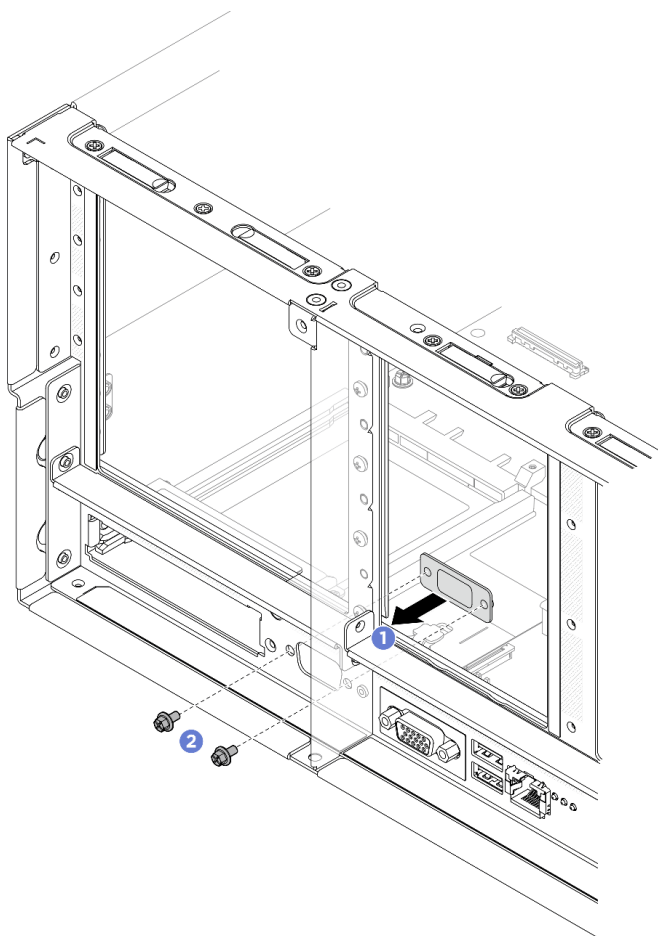
図 281. シリアル・ポート・フィラーの取り付け
