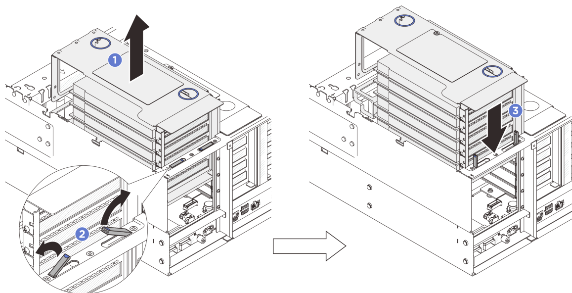
図 36. PCIe ライザーの取り外し
