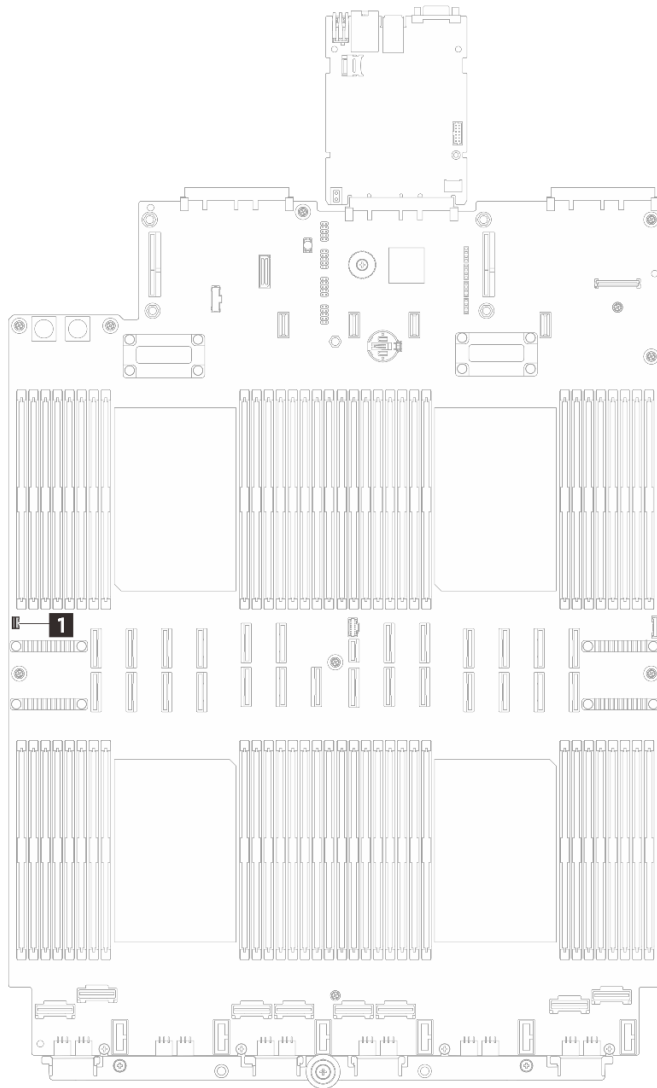
図 83. 侵入検出スイッチの切り離し
