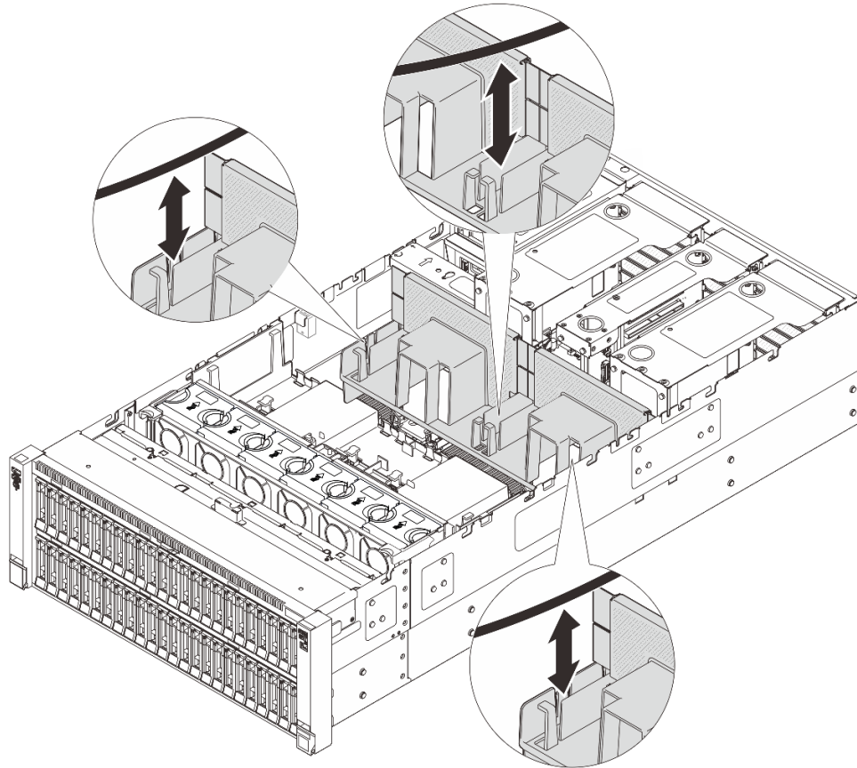
図 25. 背面エア・バッフルからケーブルを持ち上げる
