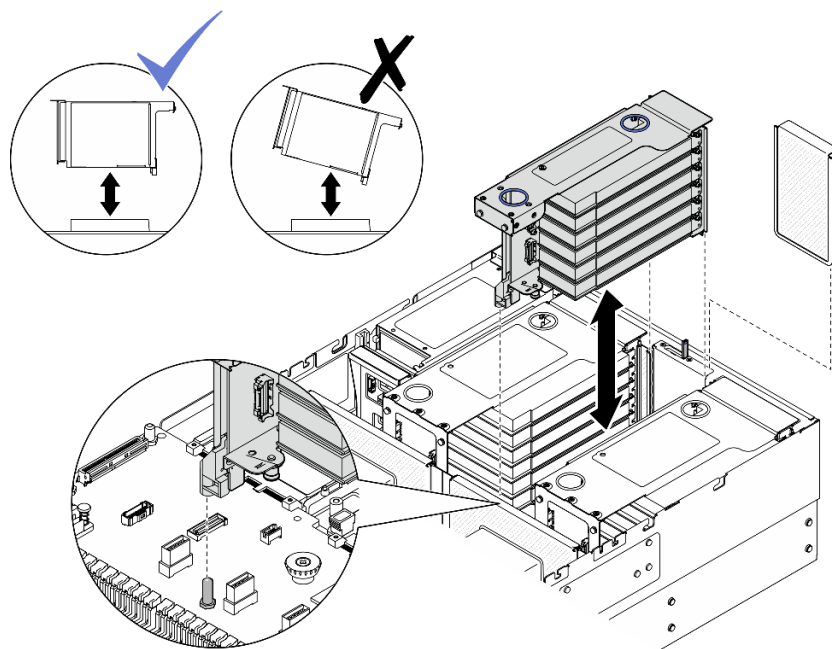
図 172. PCIe ライザー 2 の取り外し
