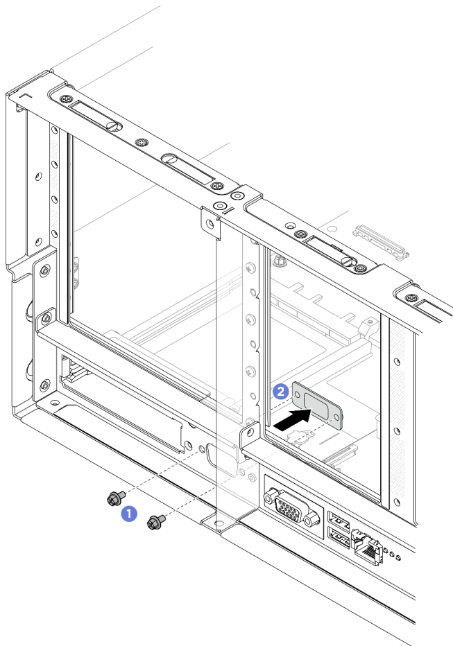
図 282. シリアル・ポート・フィラーの取り外し
