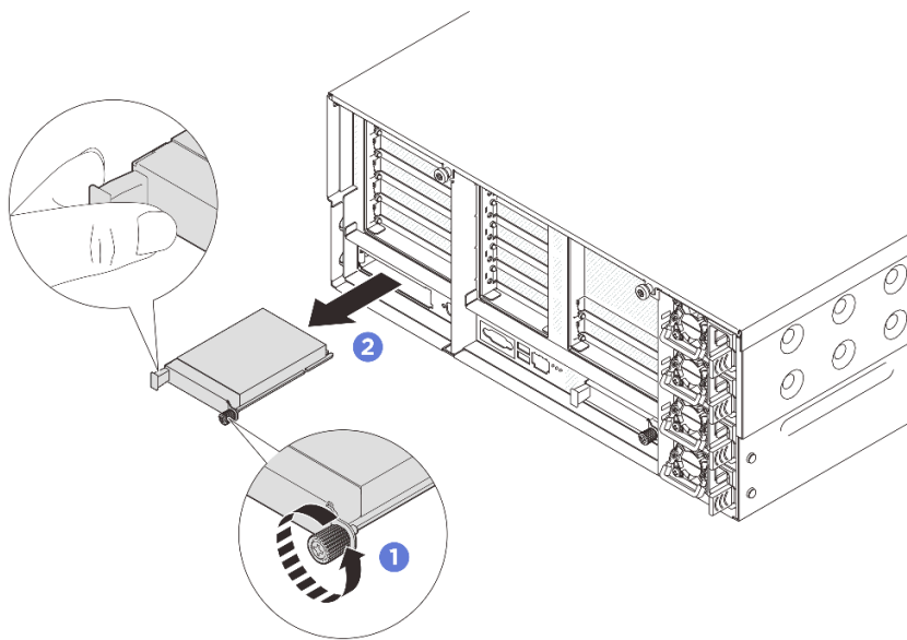
図 170. OCF モジュールの取り外し
