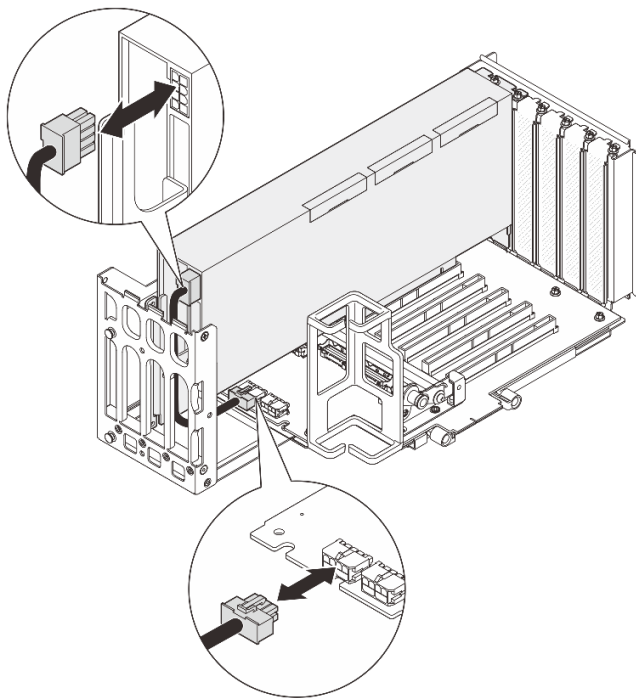
図 81. 電源ケーブルを GPU アダプターに接続する
