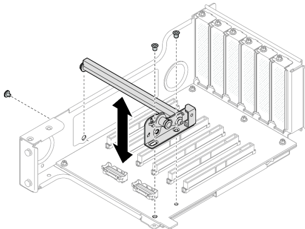
図 209. ライザー・ケージへの PCIe 保持具の取り付け
