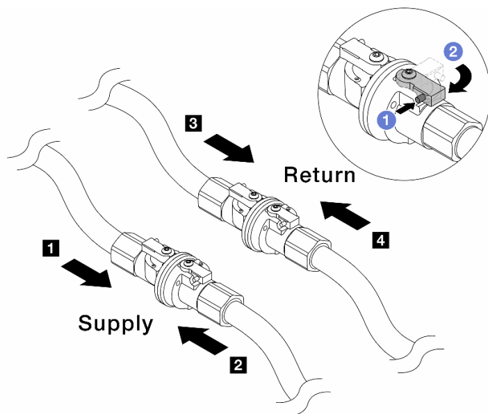
図 161. ボール・バルブを開く
