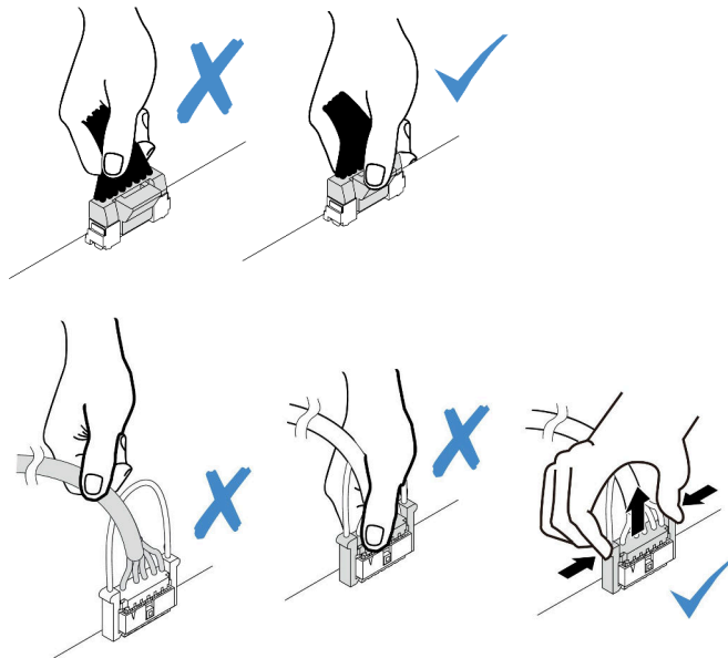
図 244. ケーブルのシステム・ボード・アセンブリーからの切り離し
