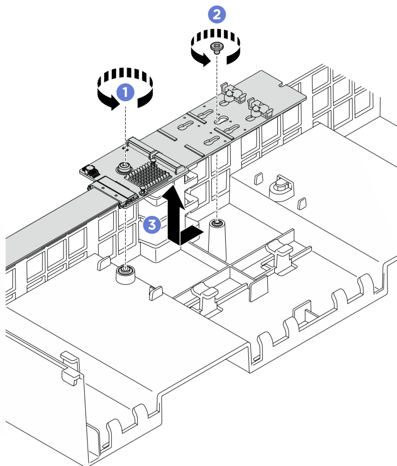
図 88. M.2 バックプレーンの取り外し
