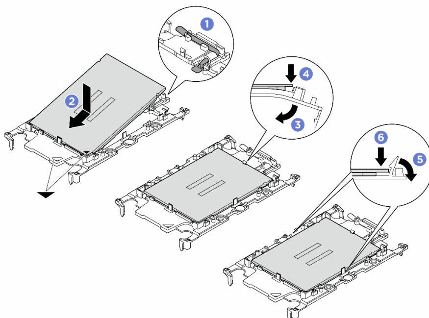
図 103. プロセッサ・キャリアの取り付け
