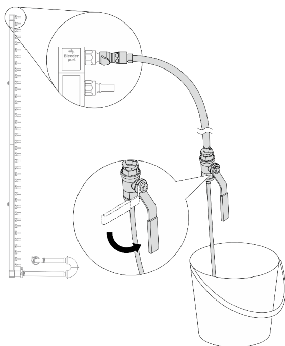
図 125. ブリーダー・バルブを開く
