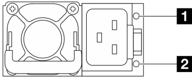
図 312. CRPS Premium パワー・サプライ上の LED
