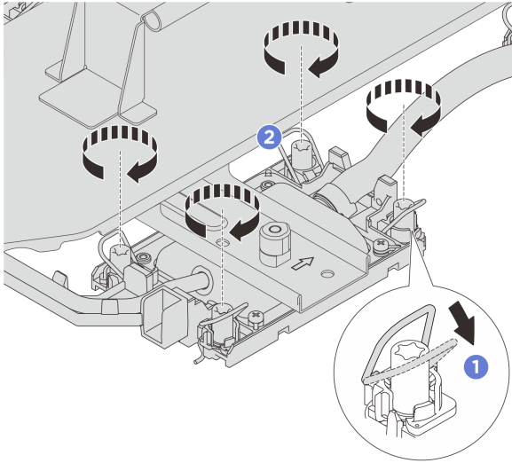
図 108. Torx T30 ナットの締め付け
