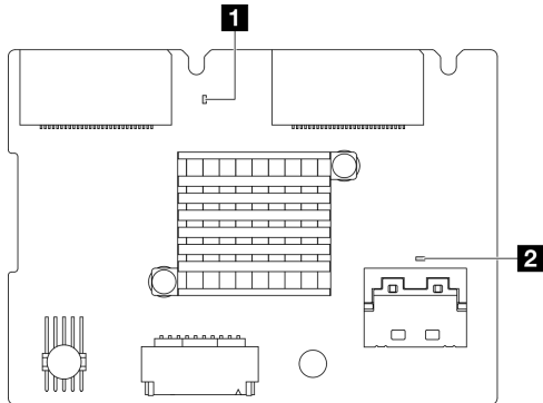
그림 27. 뒷면 M.2 백플레인 LED
