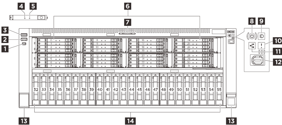
그림 4. E3.S 1T 베이이 있는 서버 모델의 앞면 보기
