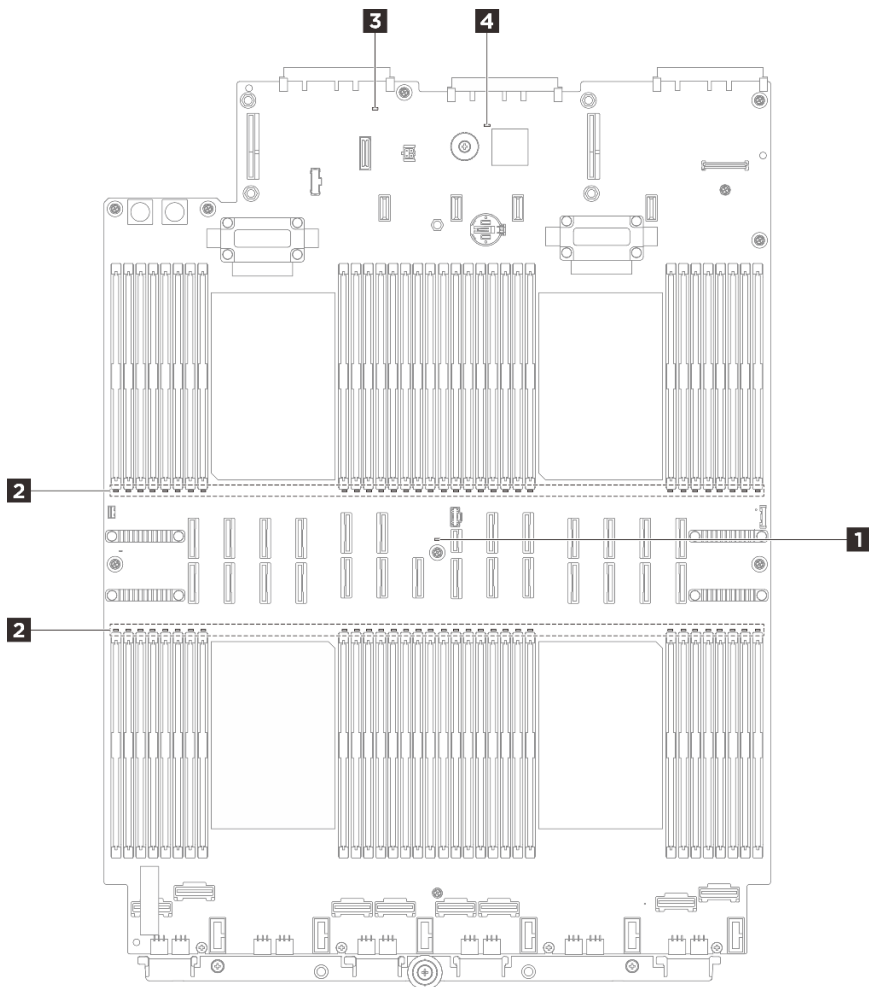
그림 21. 프로세서 보드 LED
