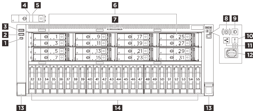
그림 6. E3.S 2T 베이가 있는 서버 모델의 앞면 보기
