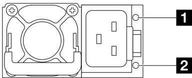
그림 23. CRPS Premium 전원 공급 장치의 LED
