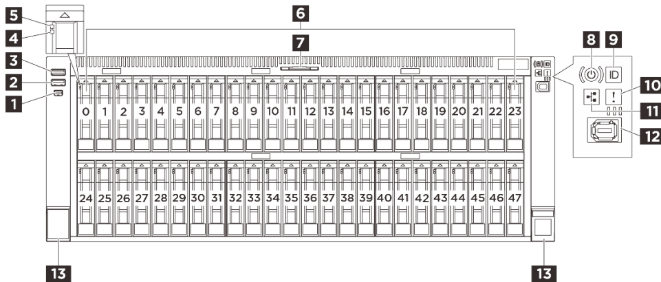
그림 2. 2.5인치 베이가 지원되는 서버 모델의 앞면 보기
