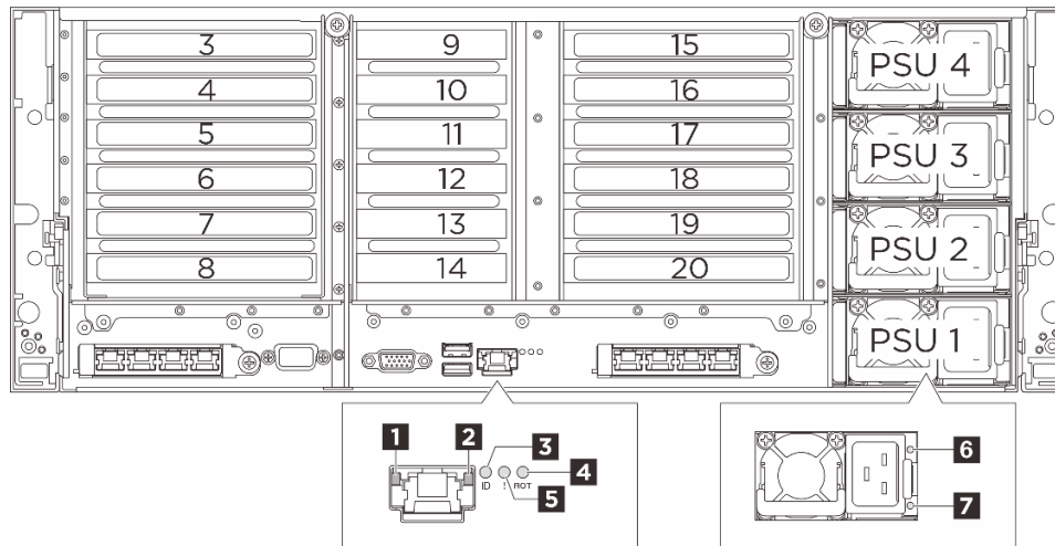
그림 11. 뒷면 LED
