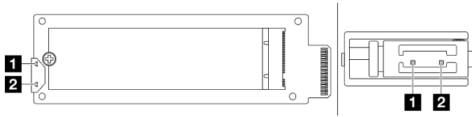
그림 26. 뒷면 M.2 인터포저 LED
