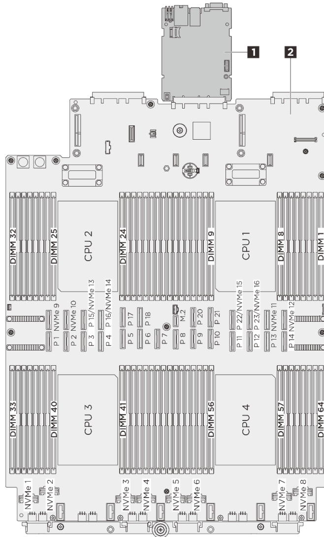
그림 13. 시스템 보드 어셈블리 레이아웃
