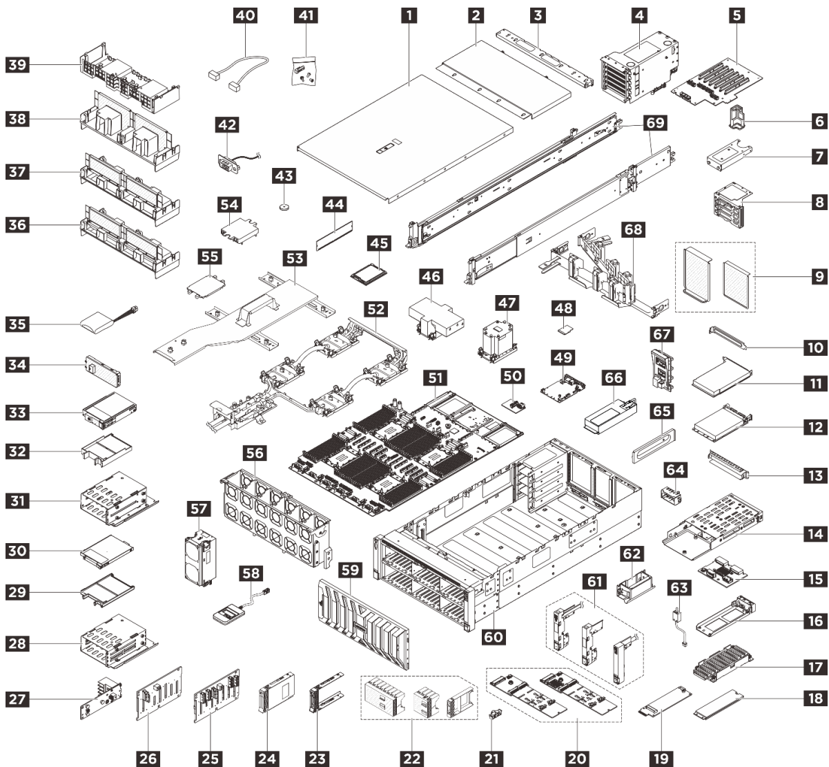
그림 29. 서버 구성 요소
