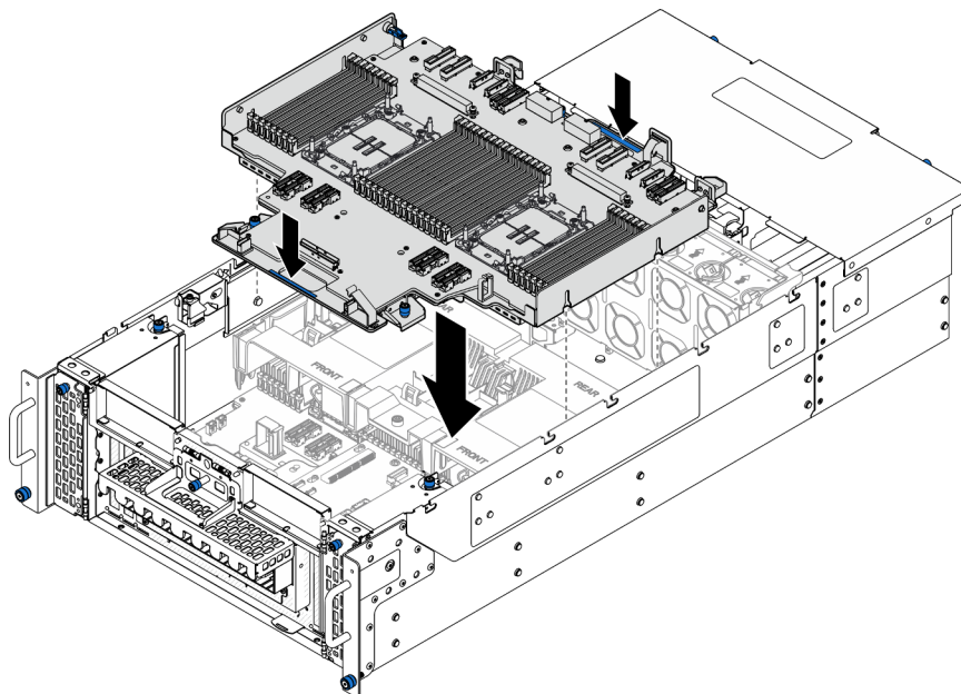
Figura 183. Instalación de la placa del procesador superior (CPU BD)
