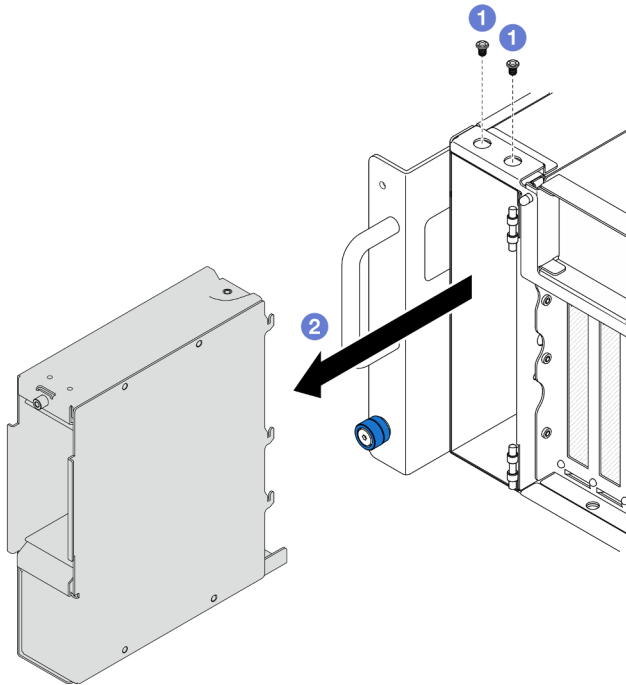
Figura 32. Extracción del compartimiento de la unidad E3.S
