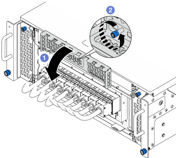
Figura 7. Cierre de la cubierta de UPI
