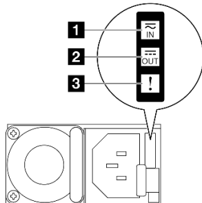
Figura 207. LED del suministro de alimentación
