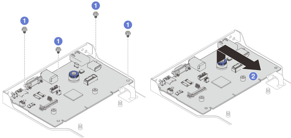
Figura 159. Extracción de la placa de E/S de la abrazadera
