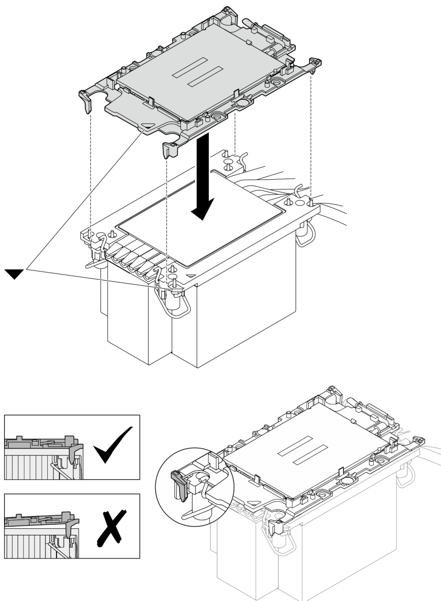
Figura 136. Ensamblaje del PHM con el procesador en la bandeja de envío
