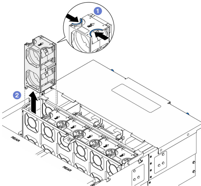
Figura 43. Extracción de un módulo de ventilador
