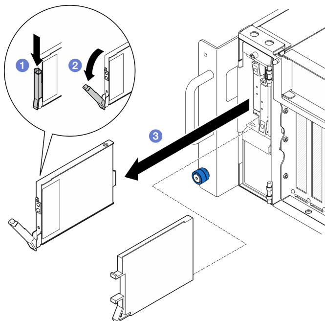
Figura 22. Extracción de una unidad E3.S
