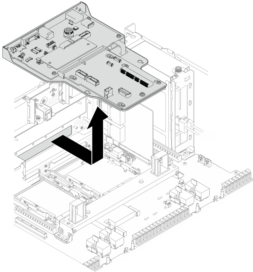
Figura 157. Extracción del conjunto de la placa de E/S y de interposición del sistema
