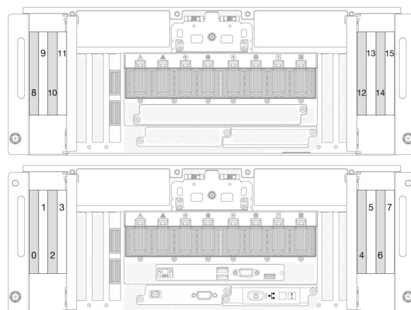
Figura 24. Numeración de la bahía de unidad E3.S
