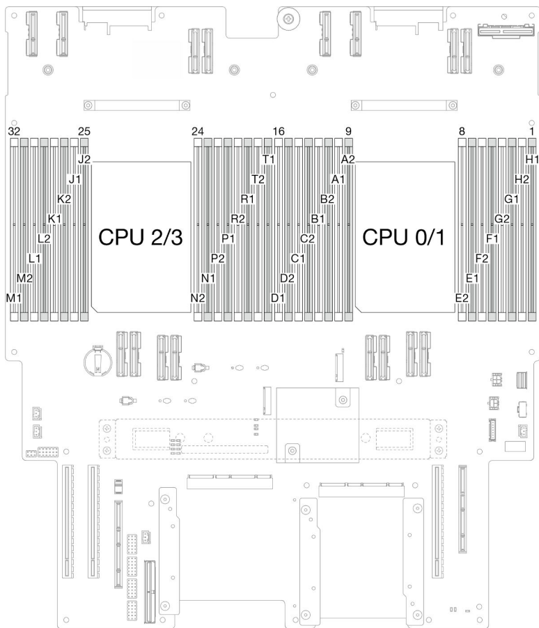
Figura 2. Diseño de los módulos de memoria y procesadores (placa del procesador inferior (MB))
