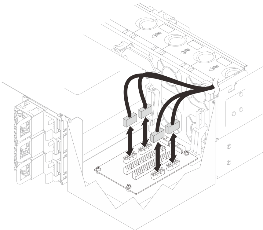
Figura 113. Conexión de los cables de expansión PCIe
