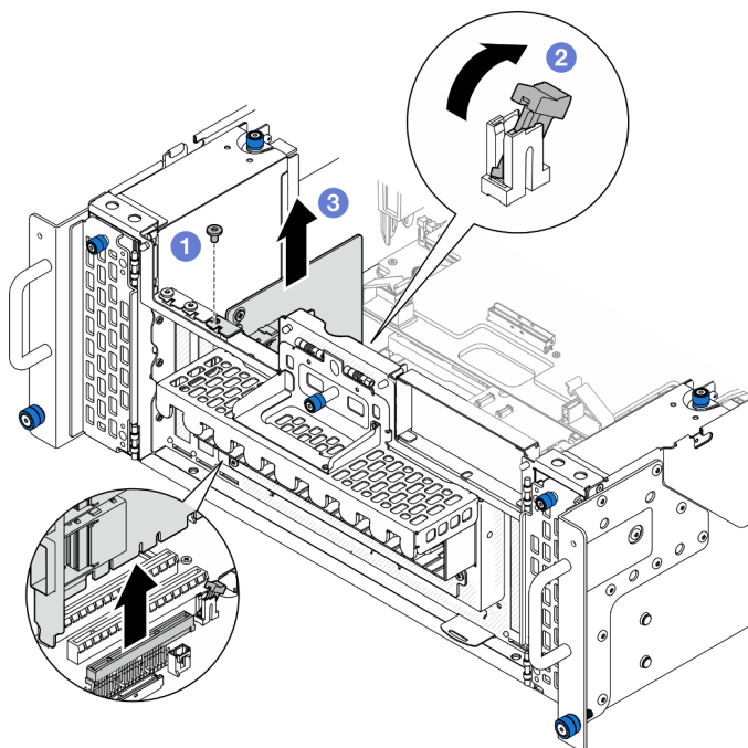
Figura 146. Extracción de la tarjeta de banda lateral
