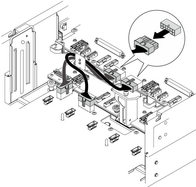
Figura 180. Desconexión de los cables de alimentación de la placa del procesador superior (CPU BD)
