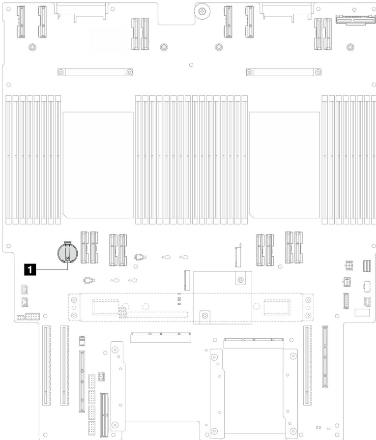
Figura 15. Ubicación de batería CMOS
