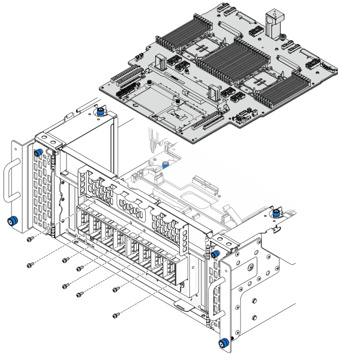
Figura 172. Retirada de los tornillos del módulo UPI
