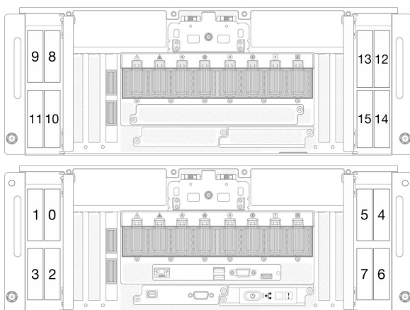
Figura 23. Numeración de la bahía de unidad de 2,5 pulgadas
