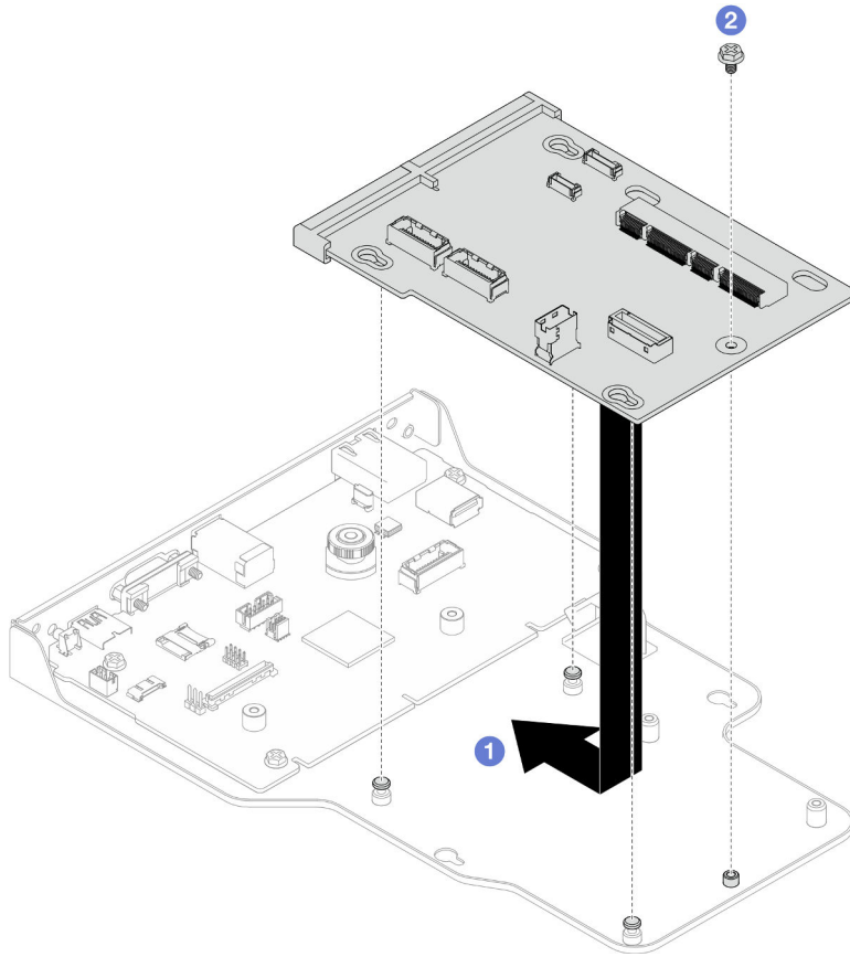
Figura 161. Instalación de la placa de interposición
