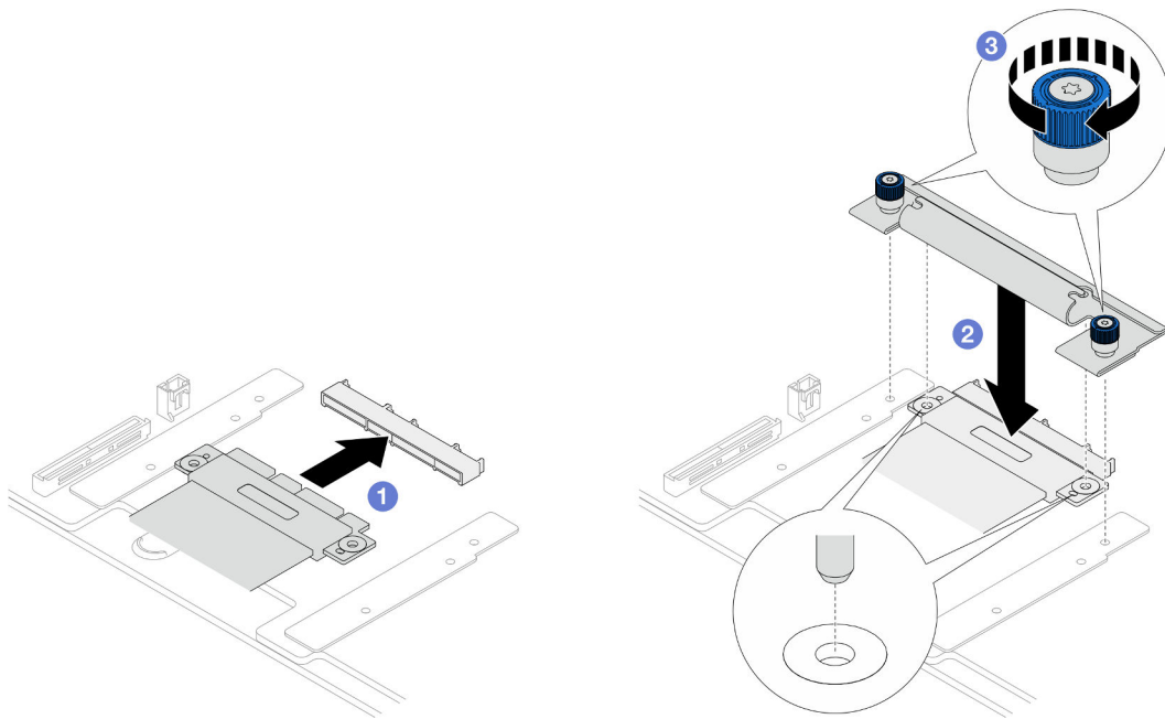
Figura 74. Conexión del cable SCM
