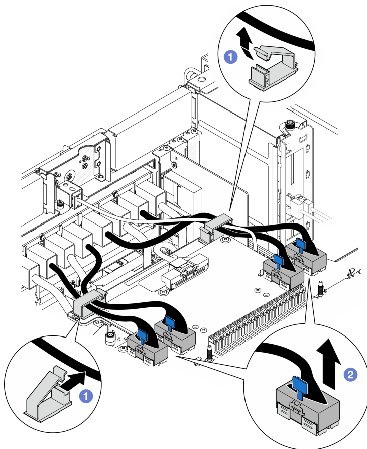
Figura 177. Desconexión de los cables del módulo UPI
