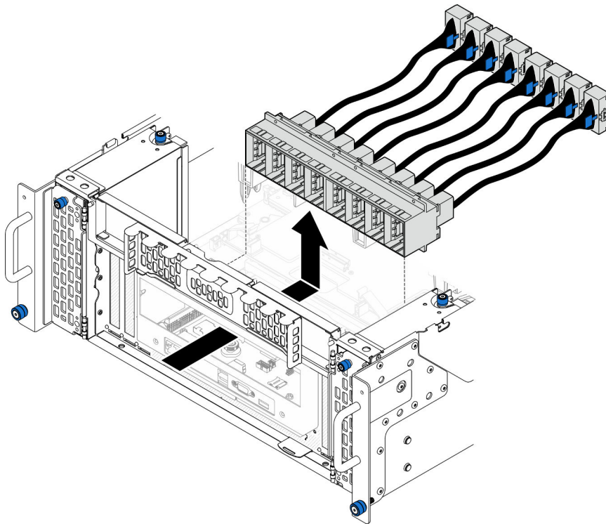
Figura 173. Extracción del módulo UPI
