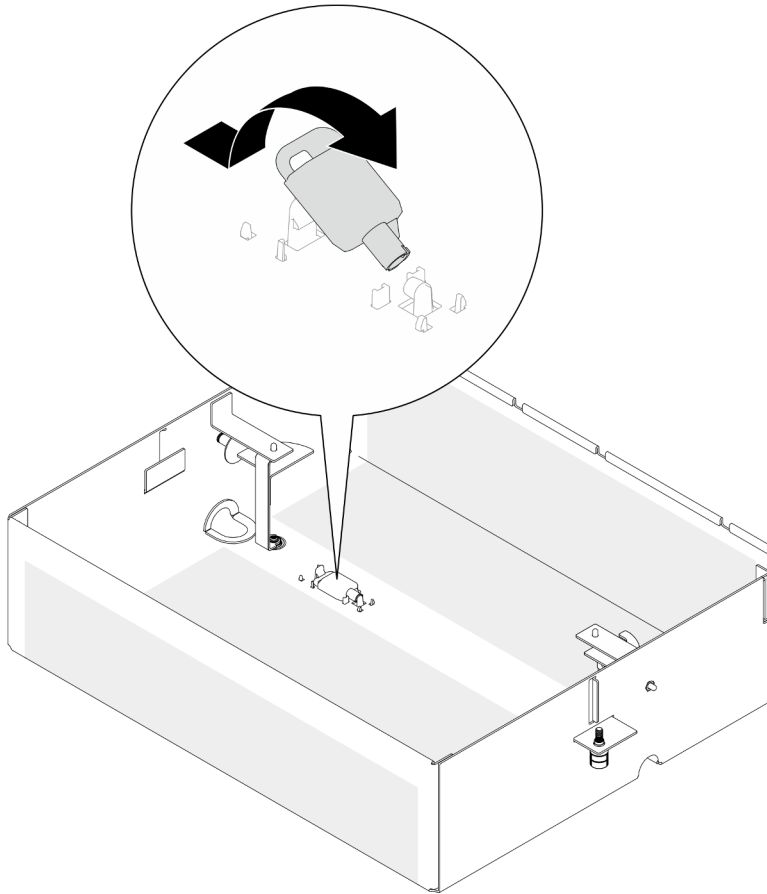
Figura 140. Extracción de la llave
