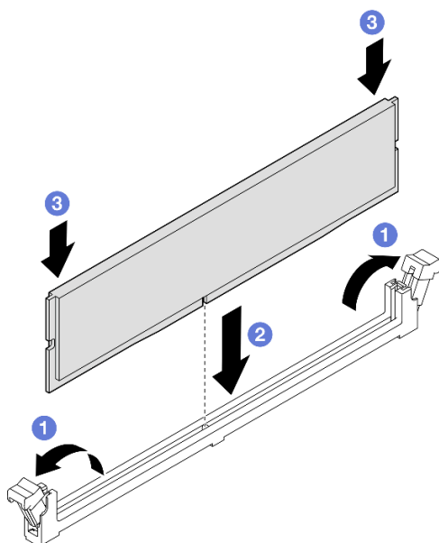
Figura 91. Instalación de un módulo de memoria
