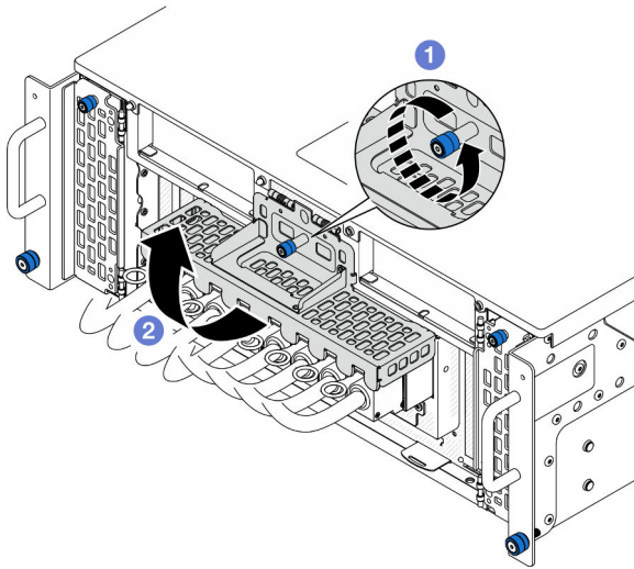
Figura 4. Apertura de la cubierta de UPI
