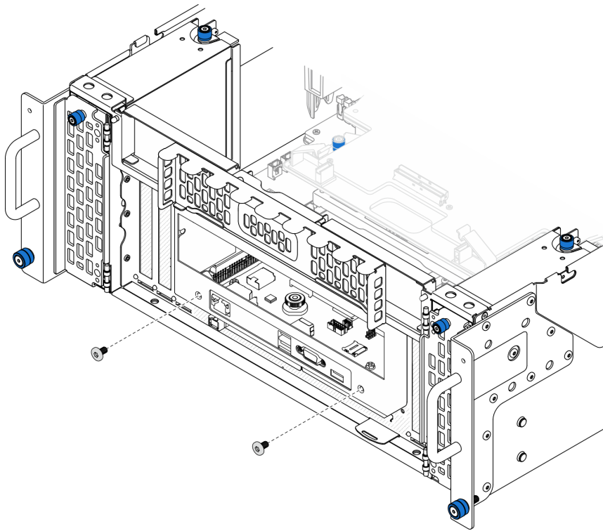
Figura 156. Aflojado del conjunto de la placa de E/S y de interposición del sistema
