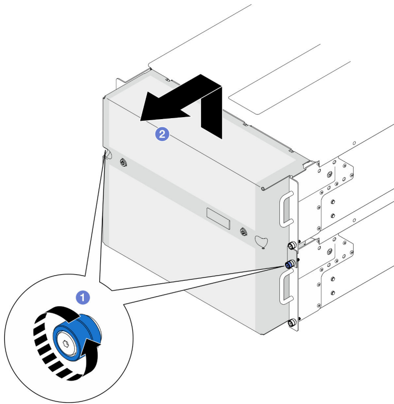
Figura 139. Extracción del marco biselado de seguridad
