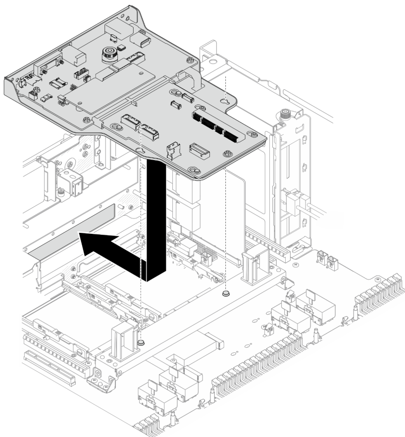
Figura 162. Instalación del conjunto de la placa de E/S y de interposición del sistema
