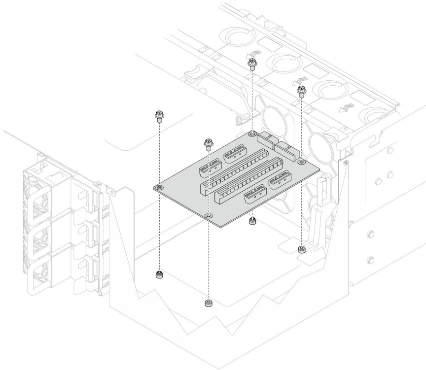
Figura 110. Extracción de la tarjeta de expansión PCIe
