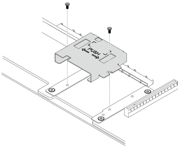
Figura 56. Instalación del compartimiento del panel frontal del operador
