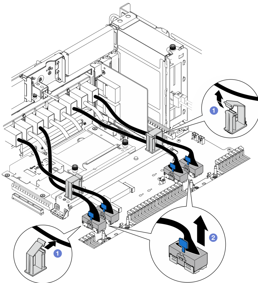
Figura 68. Desconexión de los cables del módulo UPI
