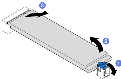
Figura 78. Extracción de la unidad M.2
