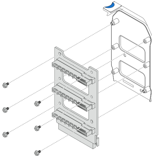
Figura 123. Desensamblaje de la placa de interposición de alimentación
