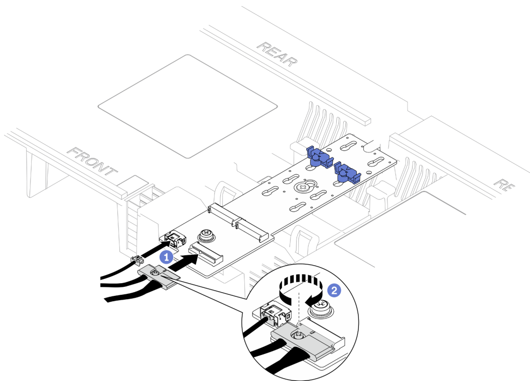
Figura 12. Conexión del cable al adaptador de arranque M.2
