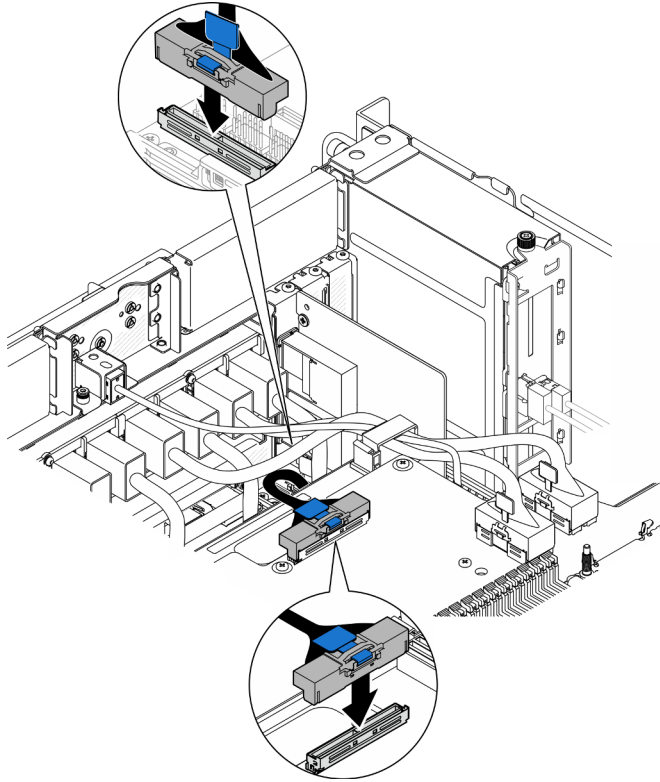
Figura 187. Conexión del cable de banda lateral interno
