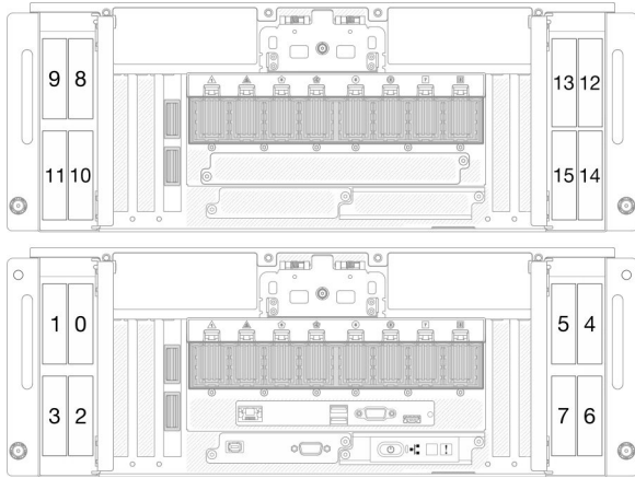
Figura 18. Numeración de la bahía de unidad de 2,5 pulgadas
