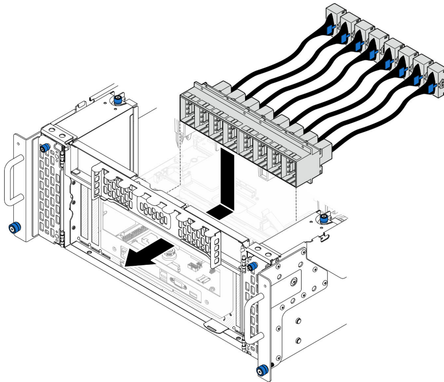
Figura 174. Instalación del módulo UPI
