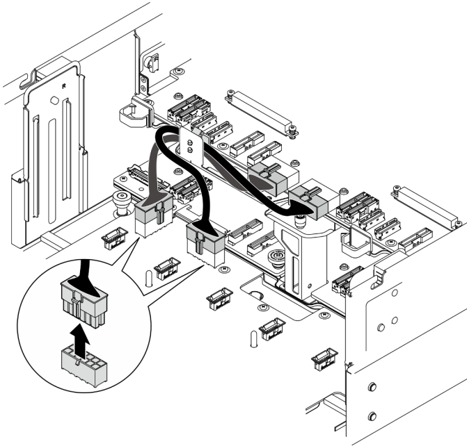
Figura 115. Desconexión de los cables de la placa de la distribución de alimentación
