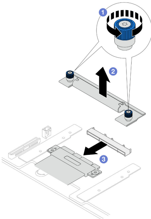
Figura 70. Desconexión del cable SCM
