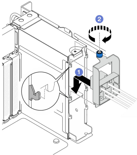
Figura 36. Instalación de un conjunto de cables E3.S
