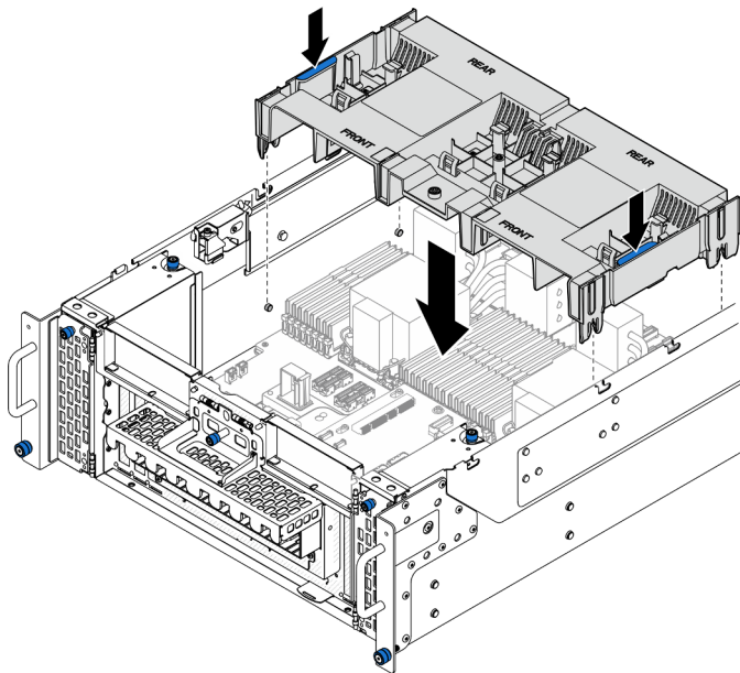
Figura 14. Instalación del deflector de aire de la placa del procesador inferior (MB)
