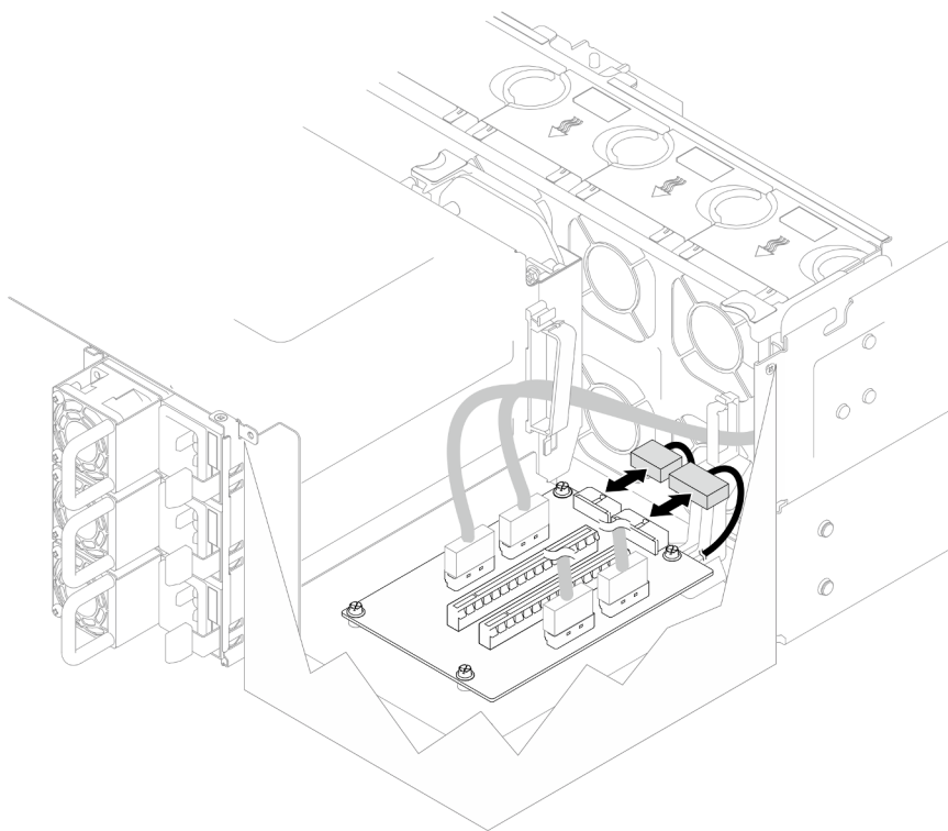
Figura 108. Desconexión de los cables de alimentación
