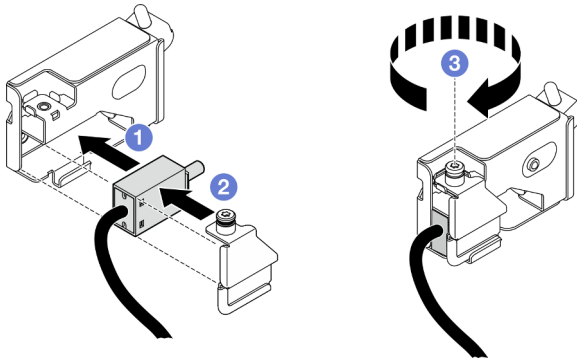
Figura 60. Instalación del conmutador de intrusión de la cubierta superior
