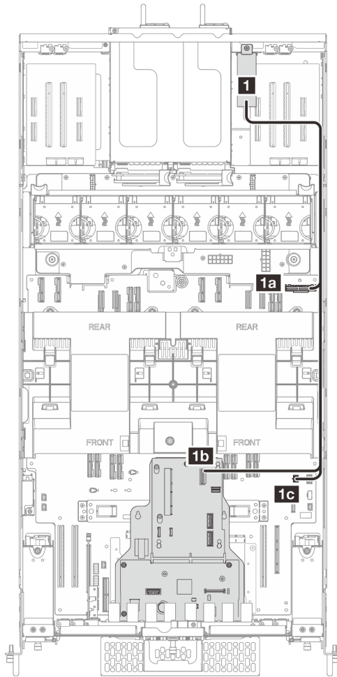
Figura 199. Disposición de los cables de OCP
