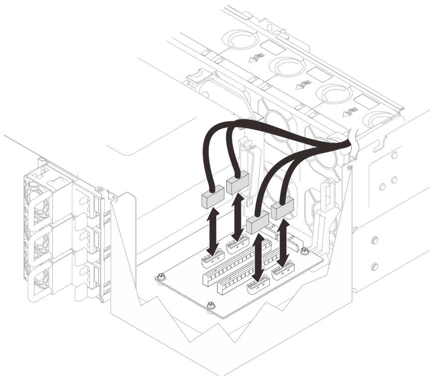
Figura 109. Desconexión de los cables de expansión PCIe
