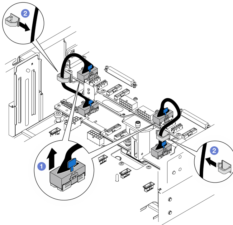
Figura 179. Desconexión de los cables de UPI internos
