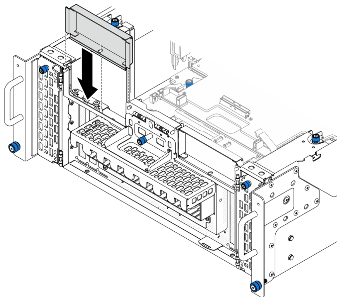
Figura 147. Instalación del relleno de PCIe izquierdo
