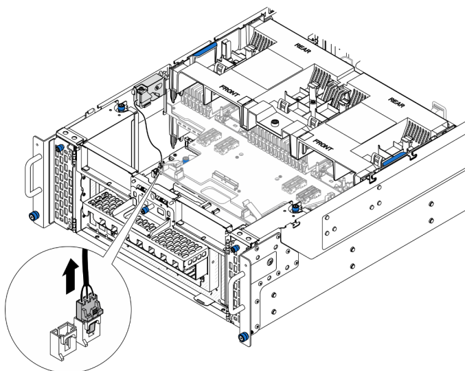
Figura 58. Desconexión del conmutador de intrusión
