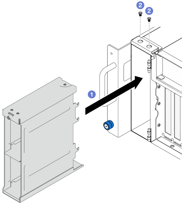
Figura 33. Instalación de un compartimiento de la unidad de 2,5 pulgadas
