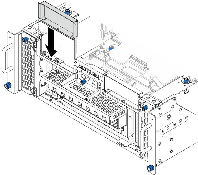
Figura 106. Instalación del relleno de PCIe izquierdo
