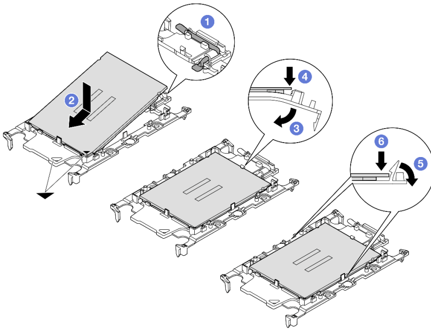
Figura 134. Instalación de un transportador de procesador
