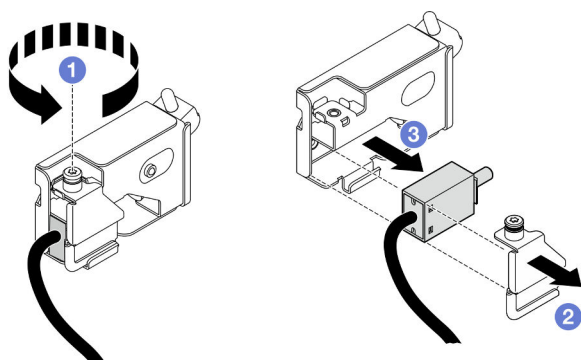
Figura 59. Extracción del conmutador de intrusión de la cubierta superior
