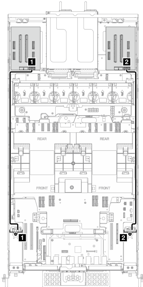
Figura 194. Disposición de los cables de alimentación para las posteriores de la unidad de 2,5"
