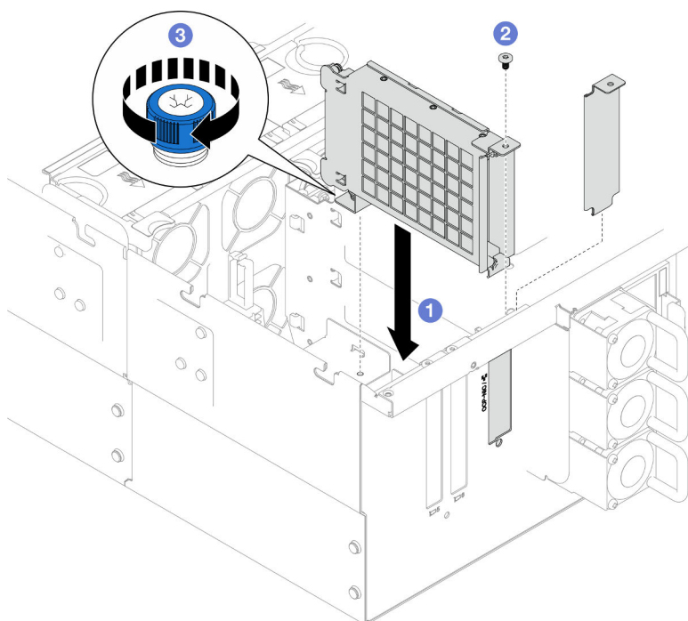
Figura 98. Instalación del compartimiento del módulo OCP
