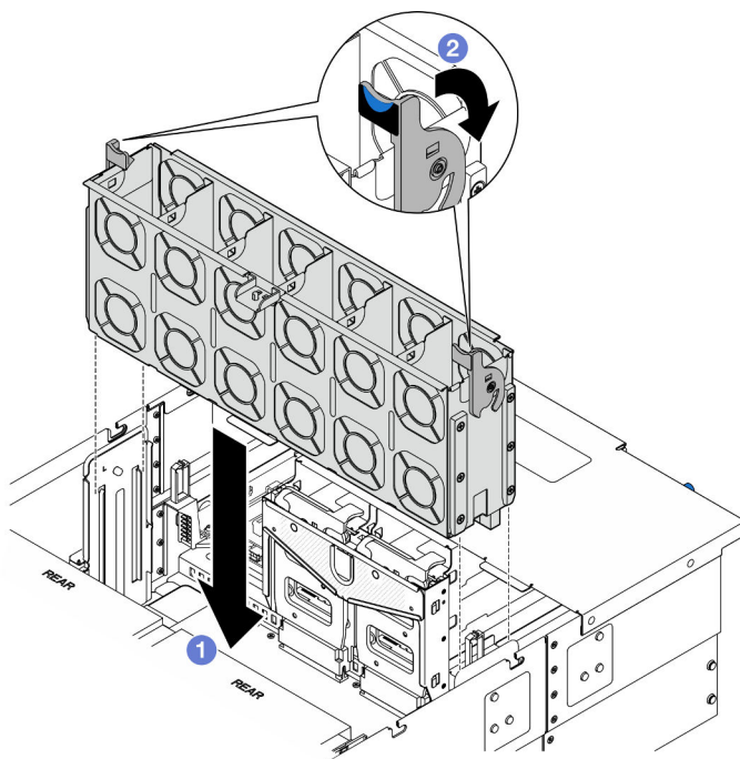
Figura 45. Instalación del compartimiento del ventilador
