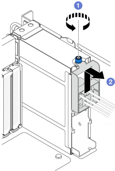
Figura 35. Extracción del conjunto de cables E3.S
