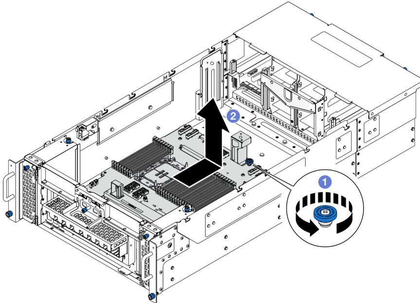
Figura 71. Extracción de la placa del procesador inferior (MB)
