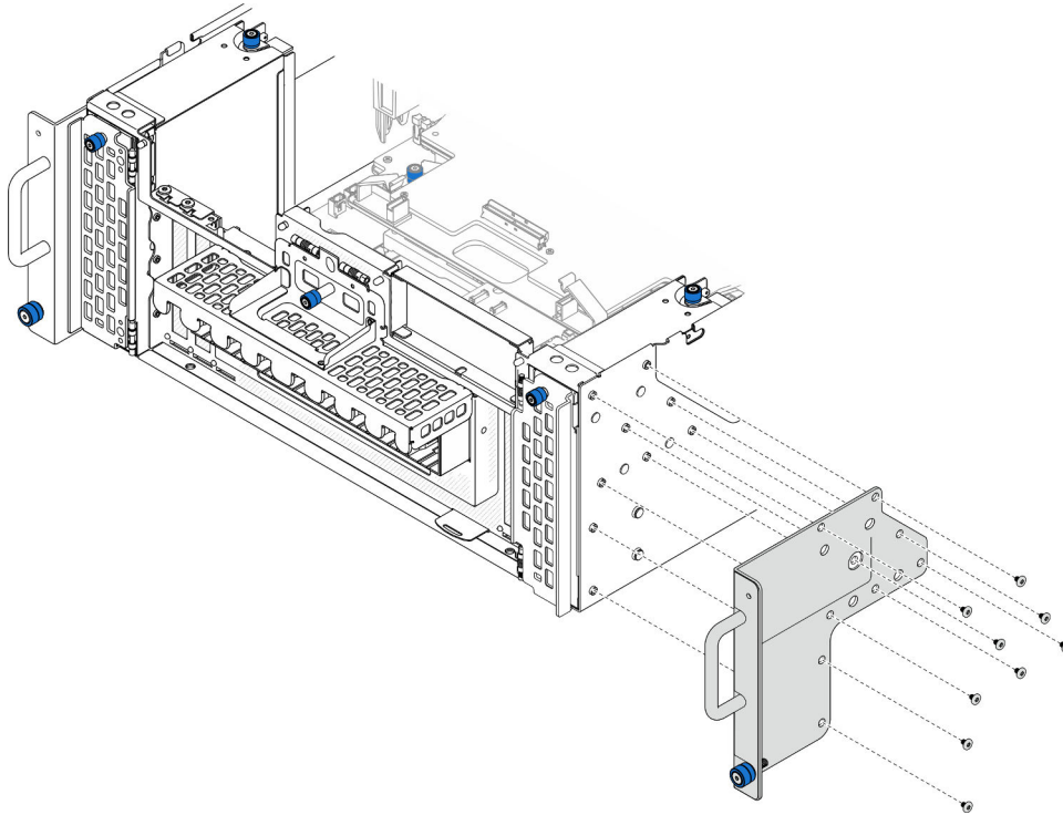
Figura 37. Extracción de la brida EIA
