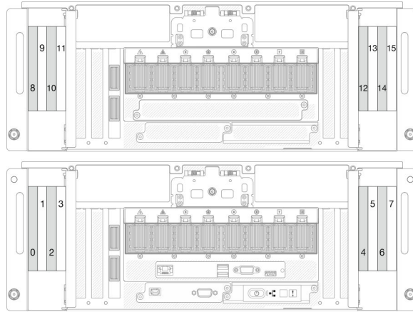
Figura 19. Numeración de la bahía de unidad E3.S
