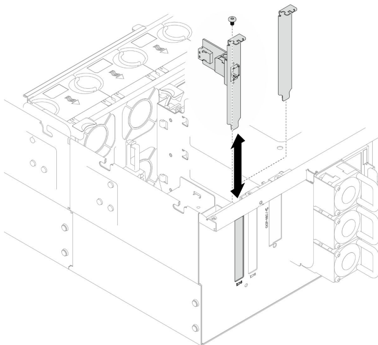
Figura 42. Instalación del conjunto de puertos Ethernet
