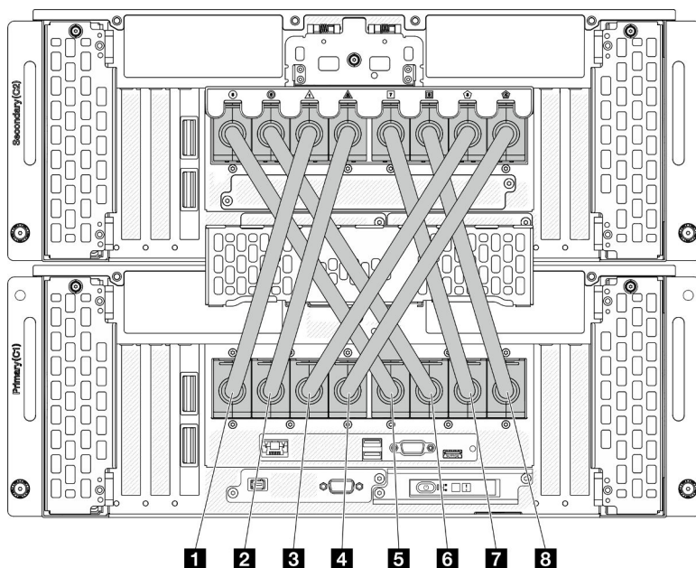
Figura 5. Desconexión de los cables de UPI externos
