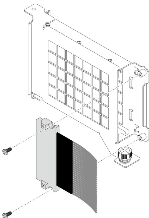
Figura 96. Extracción del cable de OCP
