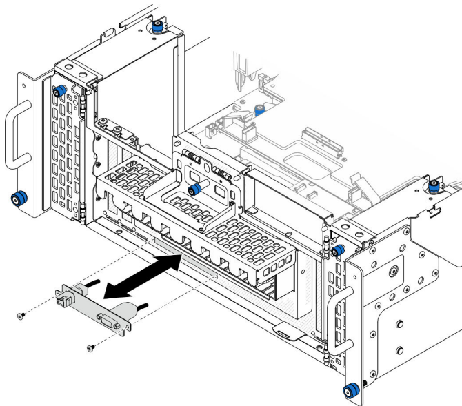
Figura 144. Instalación del conjunto de puertos serie
