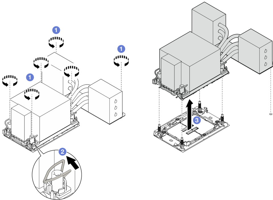
Figura 130. Extracción de un PHM 3U
