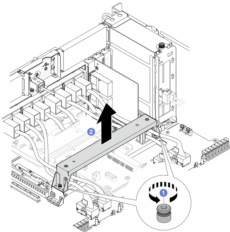
Figura 151. Extracción de la abrazadera de soporte
