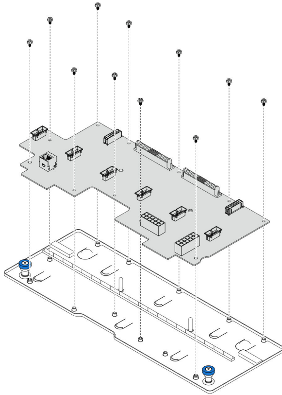
Figura 118. Desensamblaje de la placa de distribución de alimentación
