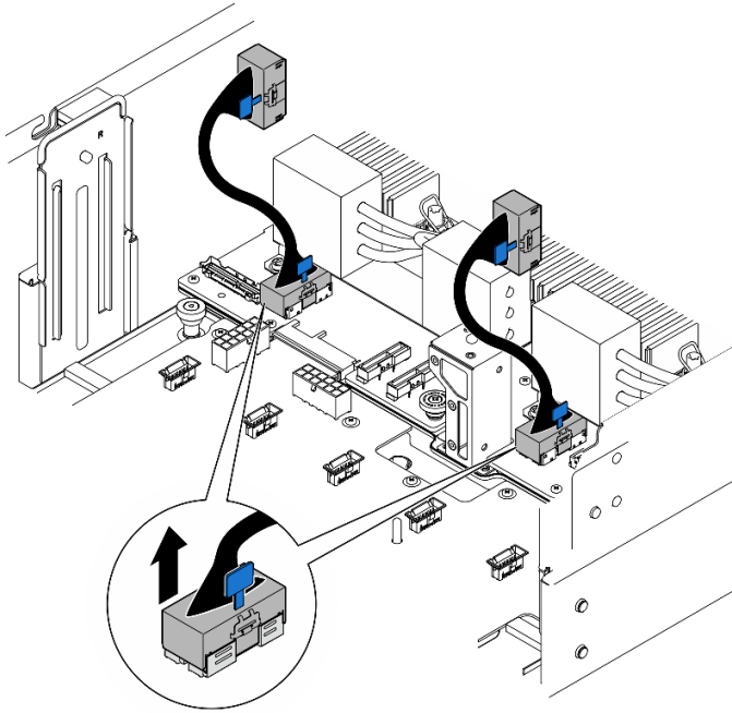
Figura 69. Desconexión de los cables de UPI internos
