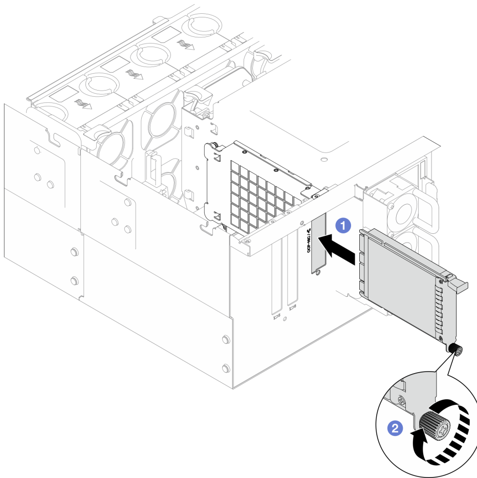
Figura 99. Instalación del módulo OCP
