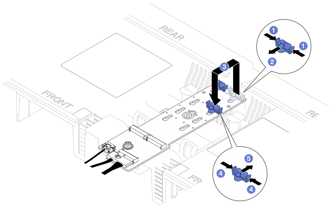
Figura 83. Ajuste del elemento de sujeción M.2
