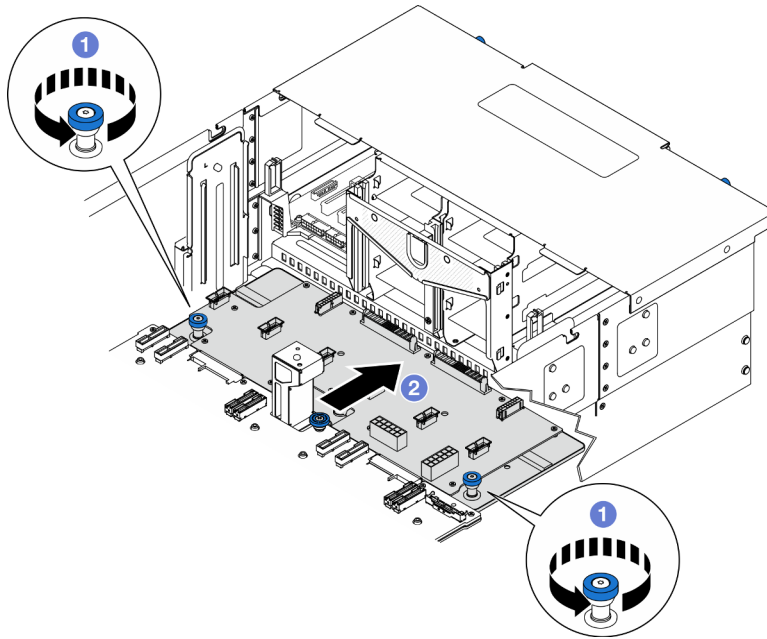
Figura 116. Desenganche de la placa de distribución de alimentación
