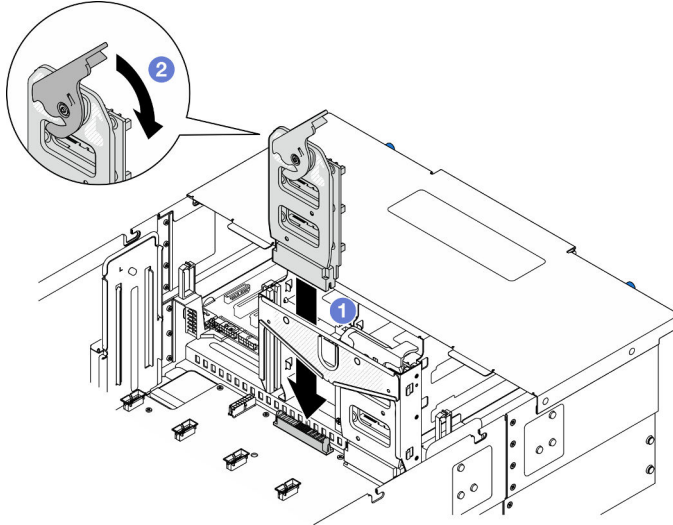
Figura 124. Instalación de la placa de interposición de alimentación
