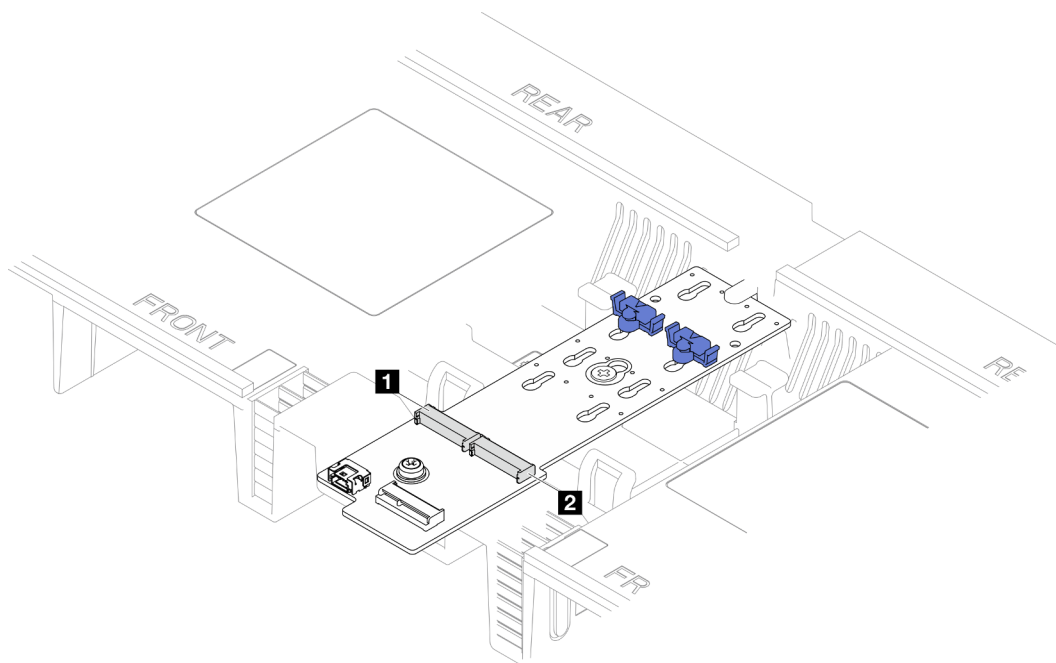
Figura 86. Ranuras de unidad M.2
