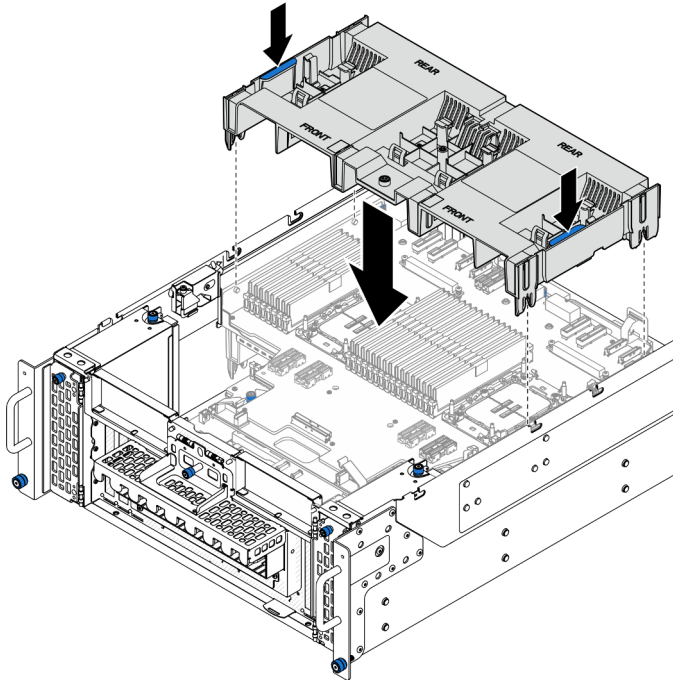
Figura 11. Instalación del deflector de aire de la placa del procesador superior (CPU BD)
