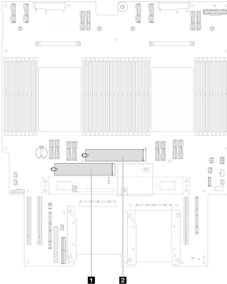
Figura 88. Ranuras de unidad M.2
