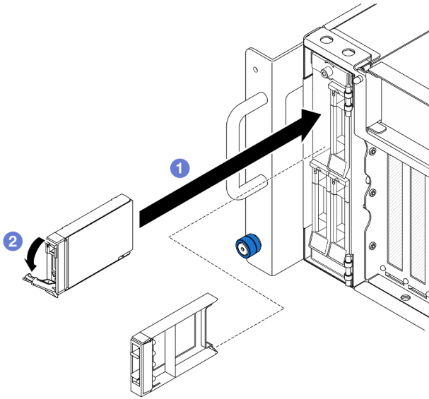
Figura 25. Instalación de una unidad de 2,5 pulgadas
