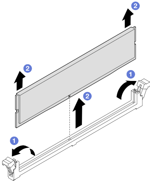
Figura 90. Extracción del módulo de memoria
