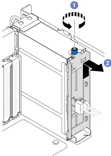
Figura 28. Extracción de una placa posterior de la unidad de 2,5 pulgadas
