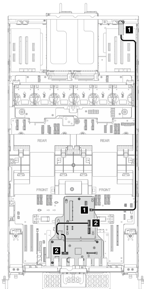
Figura 198. Disposición de los cables del conjunto de puertos Ethernet
