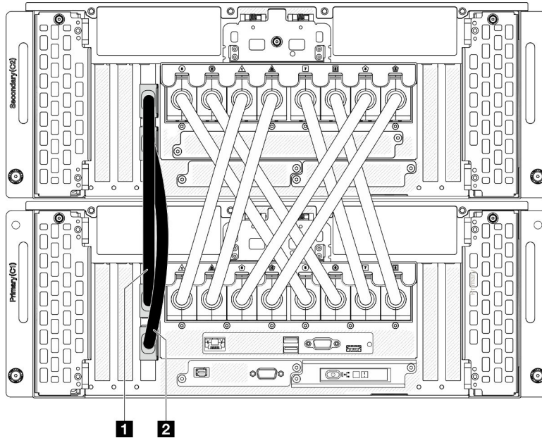
Figura 8. Conexión de los cables de la banda lateral
