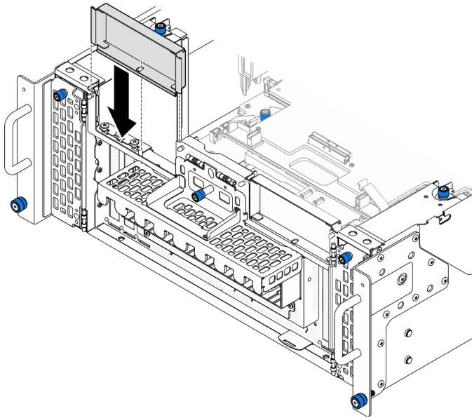
Figura 102. Instalación del relleno de PCIe izquierdo
