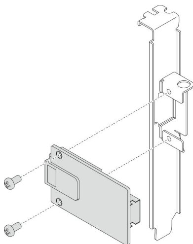
Figura 41. Instalación de la tarjeta del puerto Ethernet
