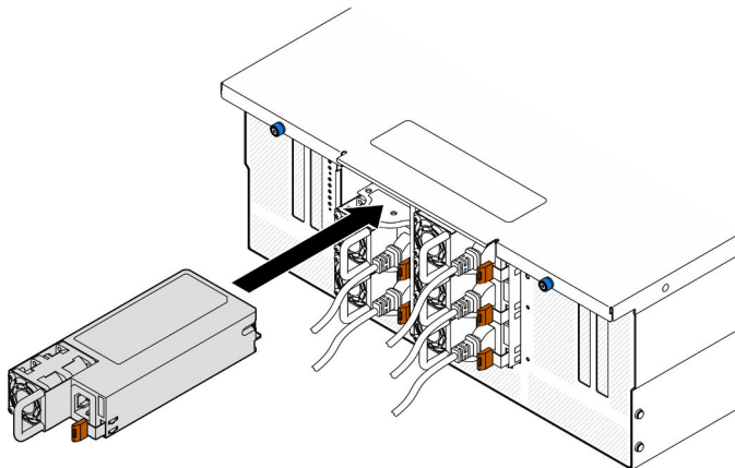
Figura 127. Instalación de una unidad de fuente de alimentación
