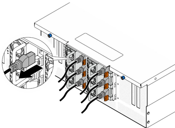
Figura 125. Desconexión del cable de alimentación
