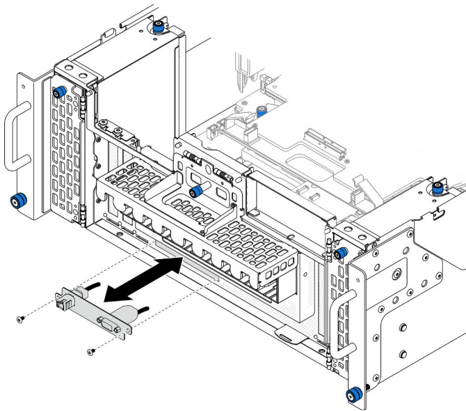
Figura 143. Extracción del conjunto de puertos serie
