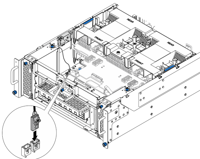
Figura 61. Conexión del conmutador de intrusión
