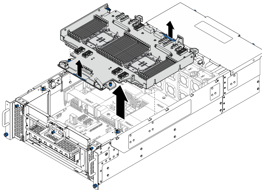
Figura 182. Extracción de la placa del procesador superior (CPU BD)
