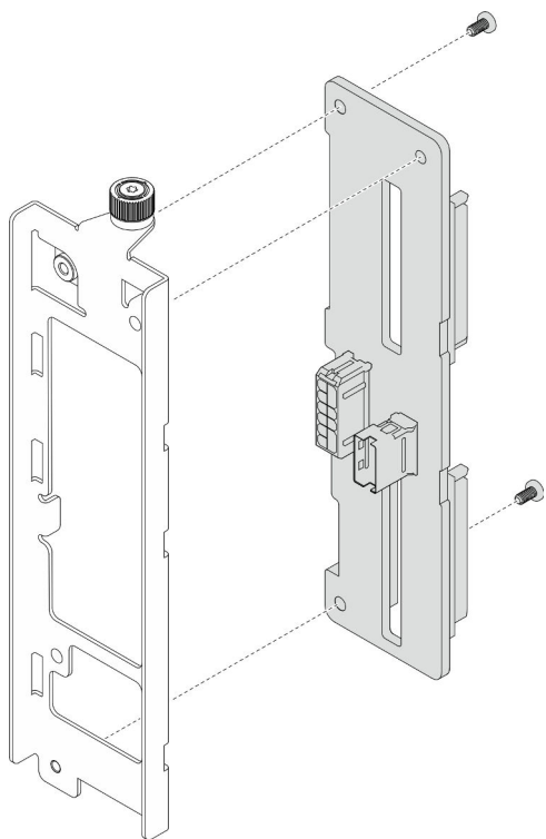
Figura 29. Desensamblaje de la placa posterior de la unidad
