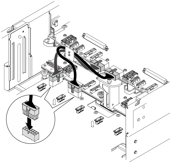
Figura 121. Conexión de los cables de la placa de la distribución de alimentación
