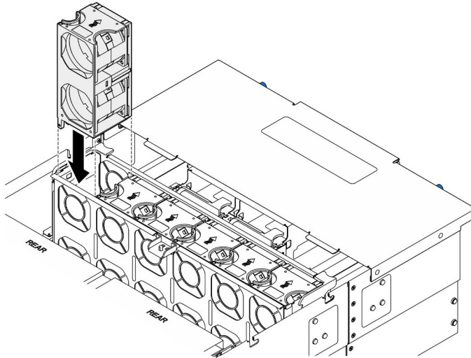
Figura 46. Instalación de un módulo de ventilador
