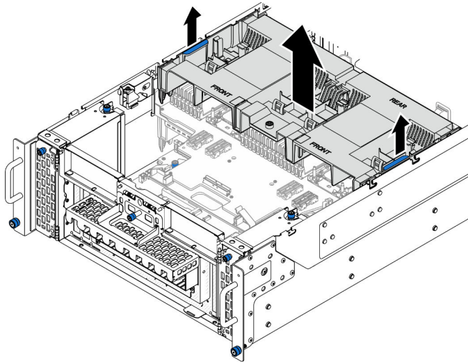
Figura 10. Extracción del deflector de aire de la placa del procesador superior (CPU BD)
