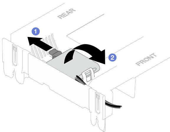
Figura 49. Extracción del módulo de alimentación flash
