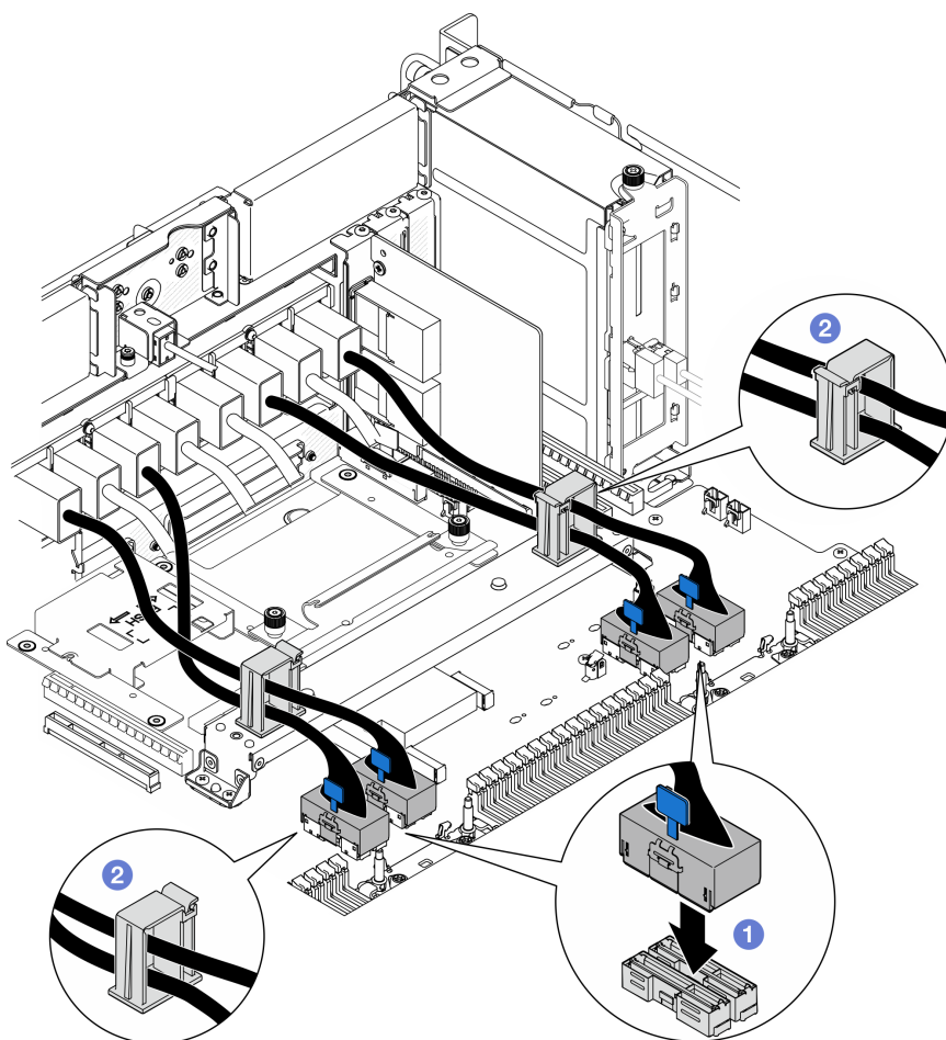
Figura 176. Conexión de los cables del módulo UPI
