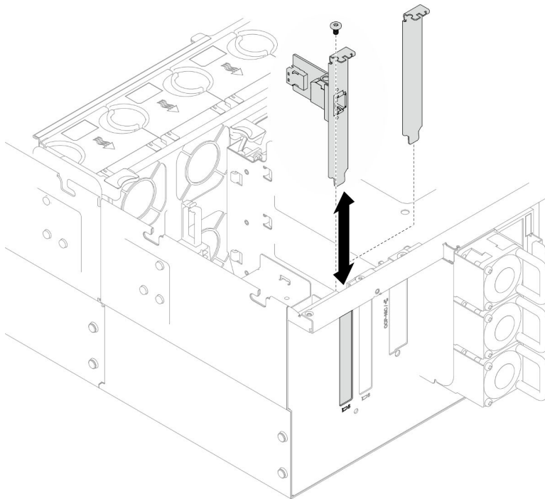
Figura 39. Extracción del conjunto de puertos Ethernet
