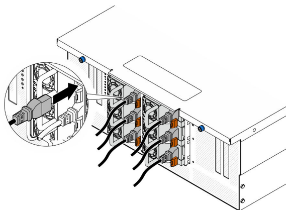
Figura 128. Conexión del cable de alimentación
