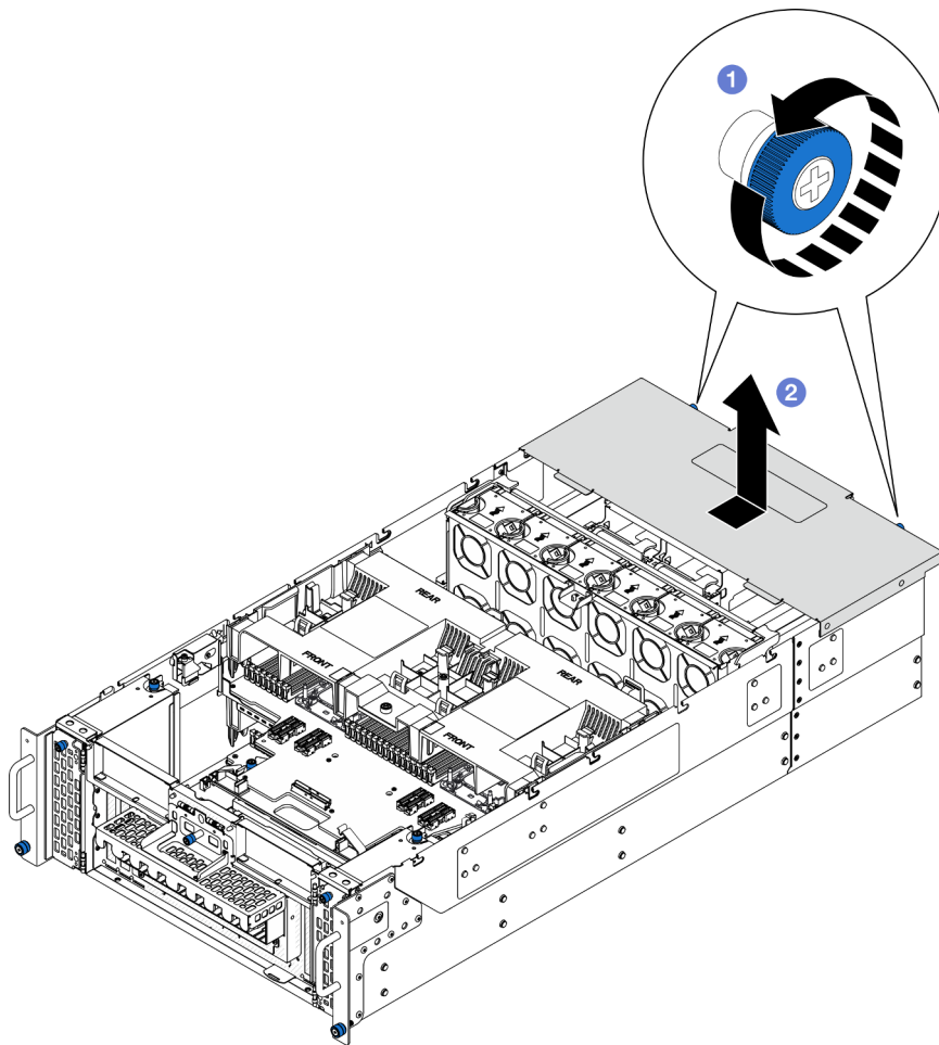
Figura 167. Extracción de la cubierta superior posterior
