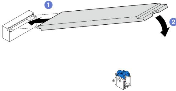
Figura 89. Instalación de una unidad M.2
