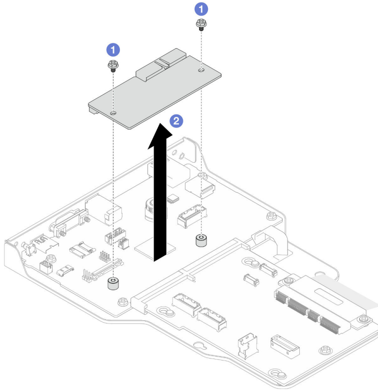
Figura 153. Extracción del firmware y módulo de seguridad de RoT
