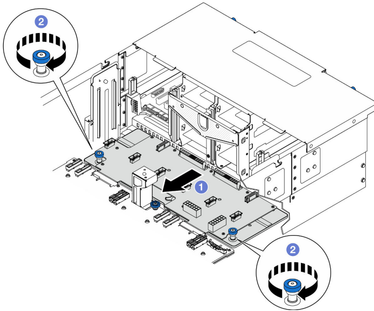
Figura 120. Fijación de la placa de distribución de alimentación.
