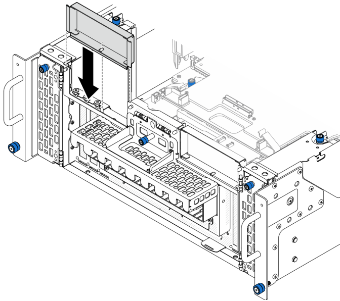
Figura 150. Instalación del relleno de PCIe izquierdo
