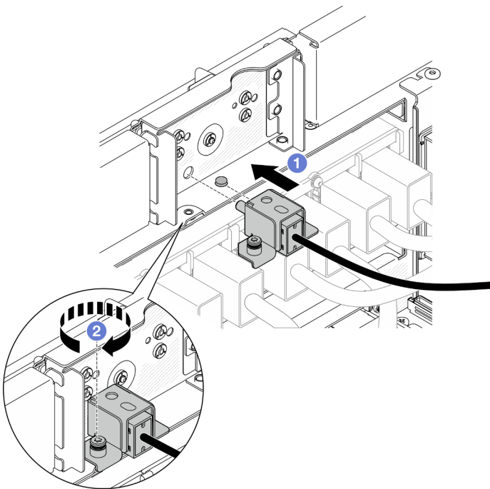
Figura 66. Instalación del conjunto del conmutador de intrusión frontal
