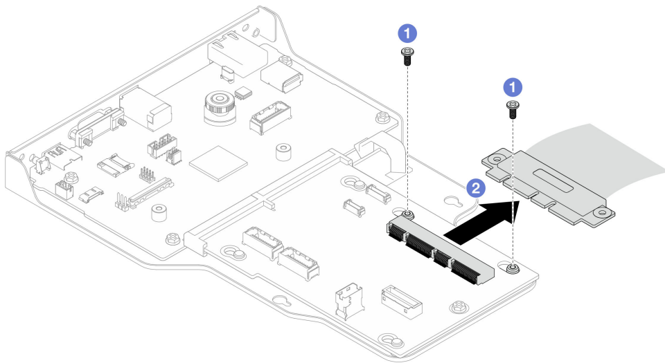
Figura 155. Desconexión del cable SCM
