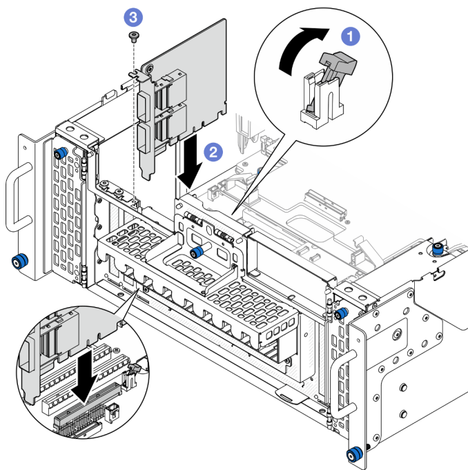
Figura 149. Instalación de la tarjeta de banda lateral
