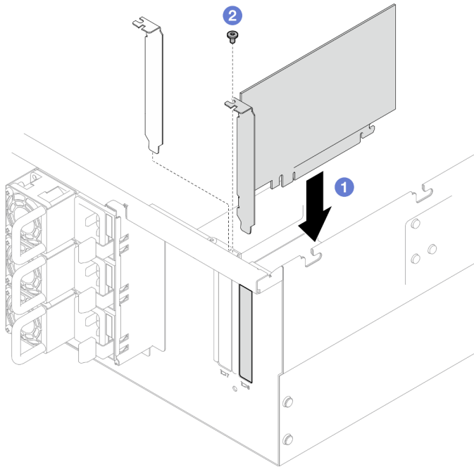
Figura 107. Instalación de un adaptador PCIe
