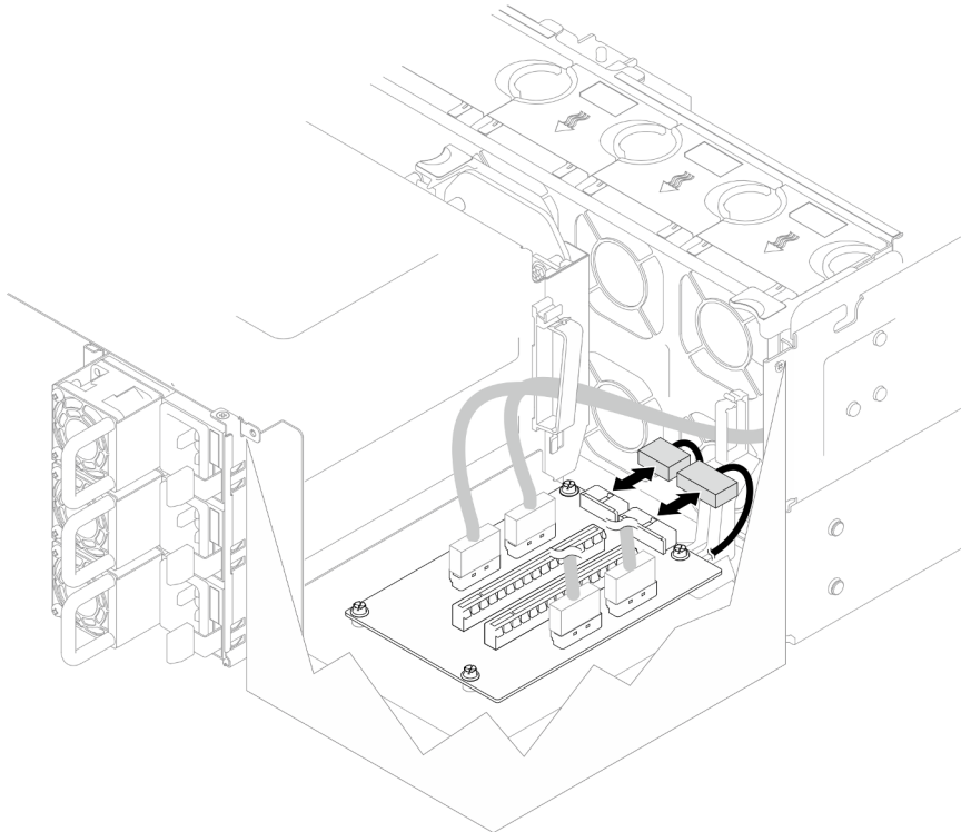
Figura 114. Conexión de los cables de alimentación
