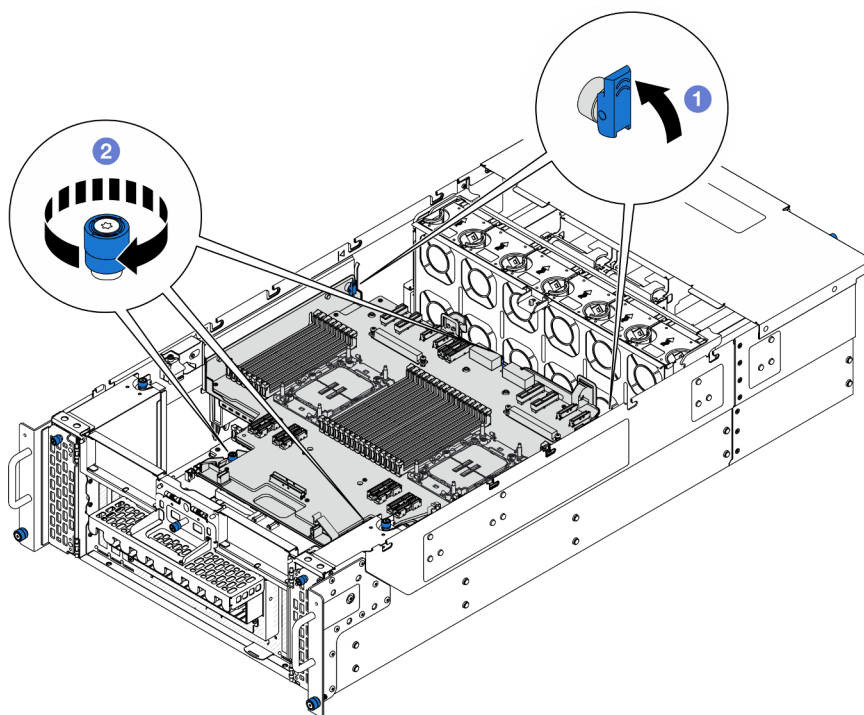
Figura 184. Fijación de la placa del procesador superior (CPU BD)
