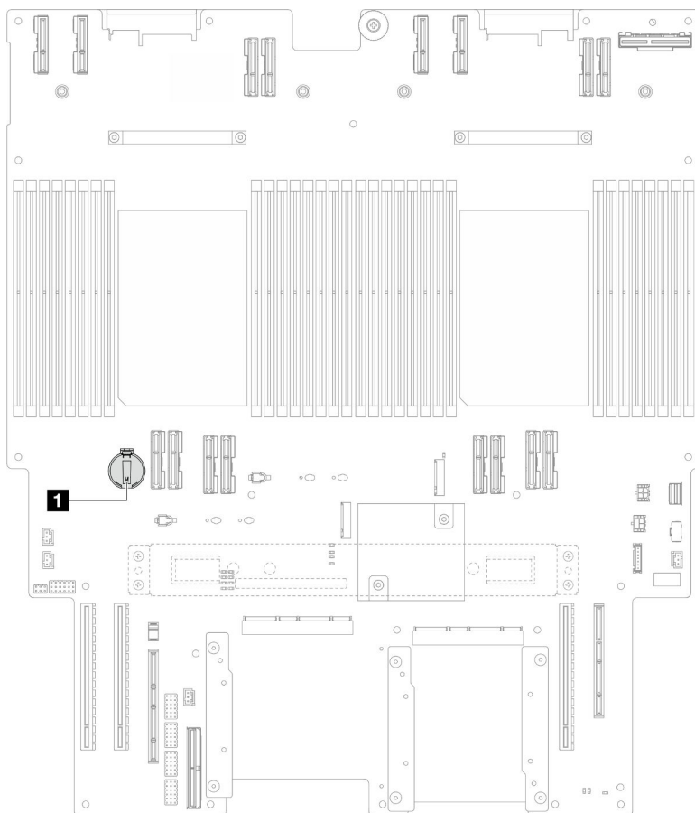
Figura 16. Ubicación de batería CMOS
