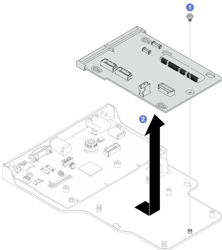
Figura 158. Extracción de la placa de interposición
