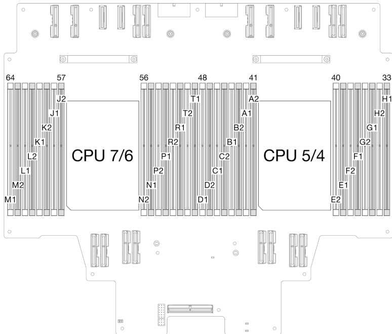
Figura 1. Diseño de los módulos de memoria y procesadores (placa del procesador superior (CPU BD))
