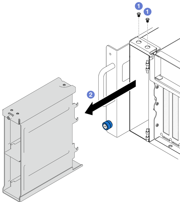
Figura 31. Extracción de un compartimiento de la unidad de 2,5 pulgadas
