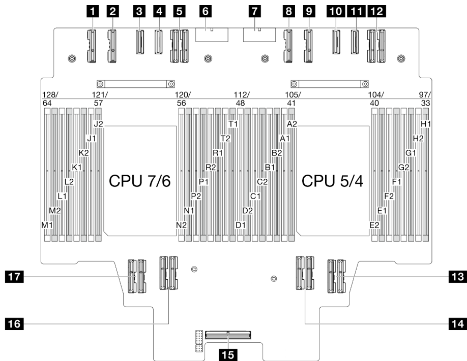
Figura 190. Conectores de la placa del procesador superior (CPU BD)
