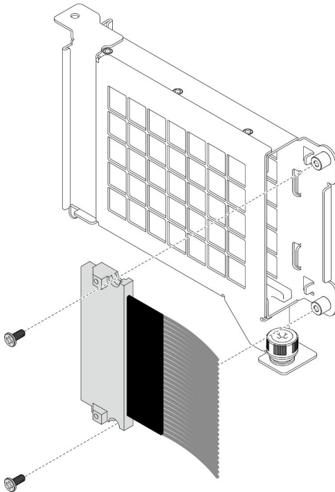
Figura 97. Instalación del cable OCP
