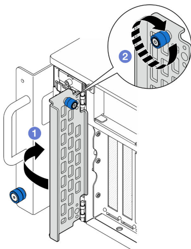
Figura 27. Cierre de la puerta de la unidad
