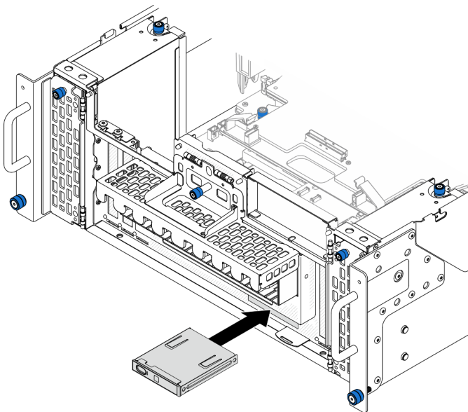
Figura 57. Instalación del panel frontal del operador
