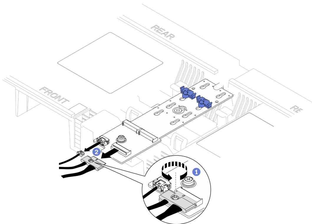
Figura 9. Desconexión del cable del adaptador de arranque M.2
