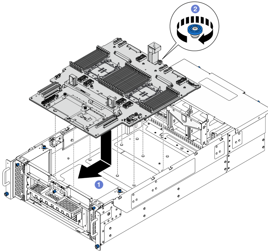
Figura 72. Instalación de la placa del procesador inferior (MB)
