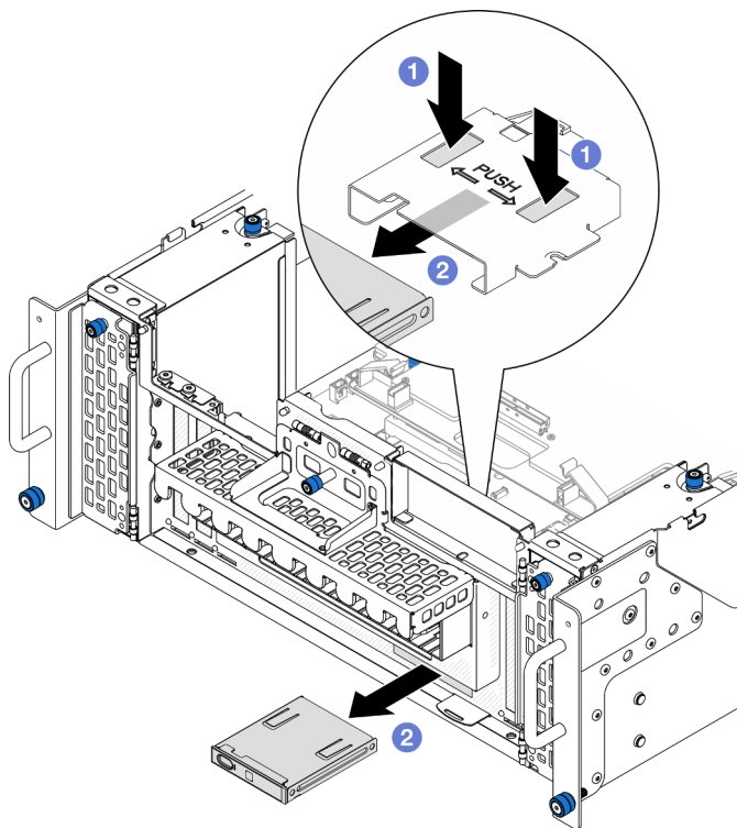
Figura 52. Extracción del panel frontal del operador
