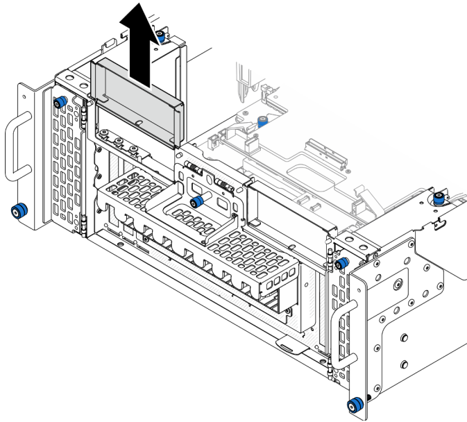
Figura 100. Extracción del relleno de PCIe izquierdo
