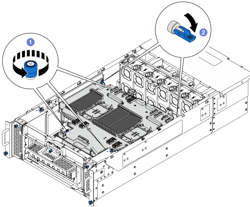
Figura 181. Desenganche de la placa del procesador superior (CPU BD)
