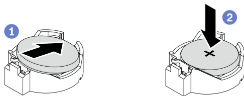
Figura 17. Instalación de la batería CMOS
