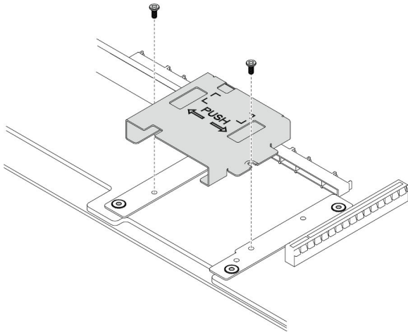
Figura 53. Extracción del compartimiento del panel frontal del operador
