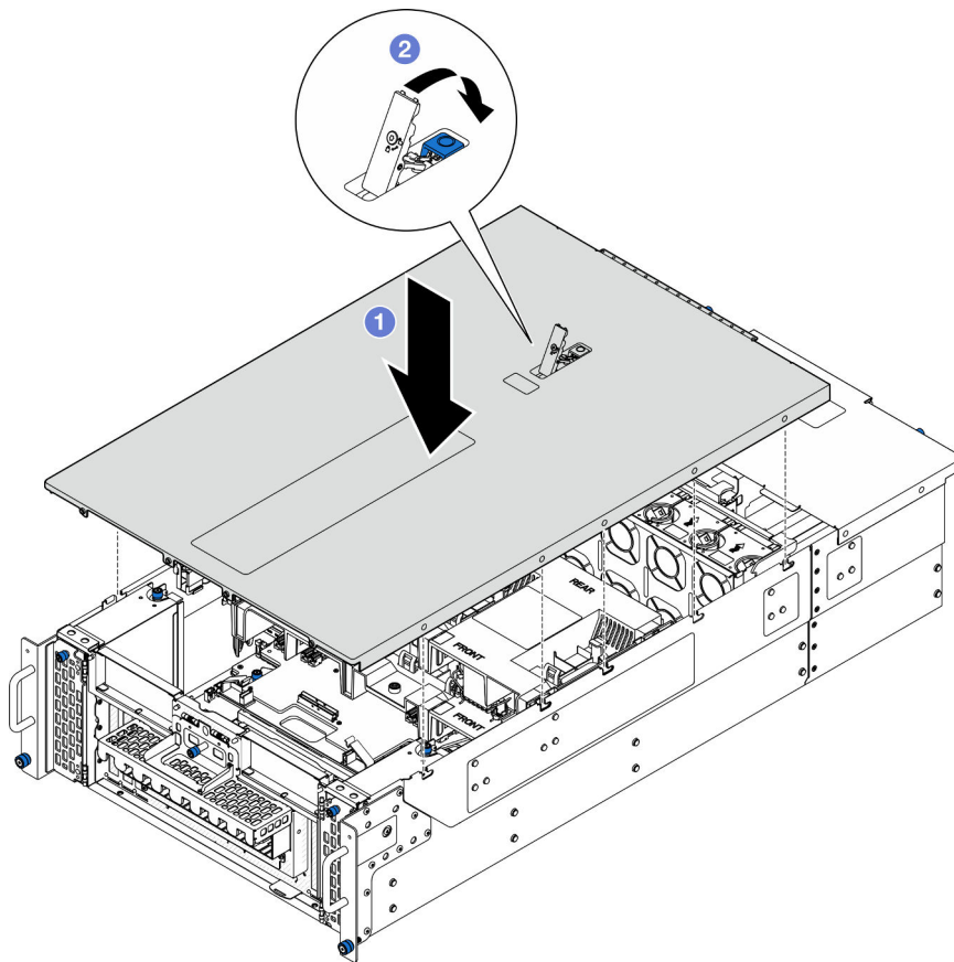
Figura 169. Instalación de la cubierta superior frontal
