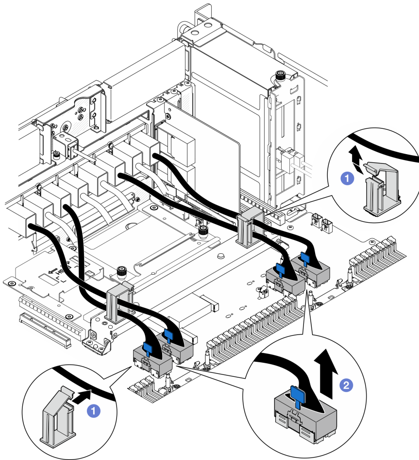
Figura 171. Desconexión de los cables del módulo UPI
