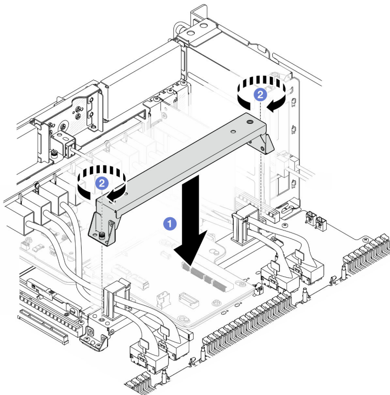
Figura 152. Instalación de la abrazadera de soporte
