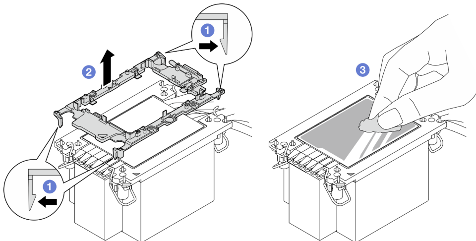
Figura 132. Separación de un transportador de procesador del disipador de calor
