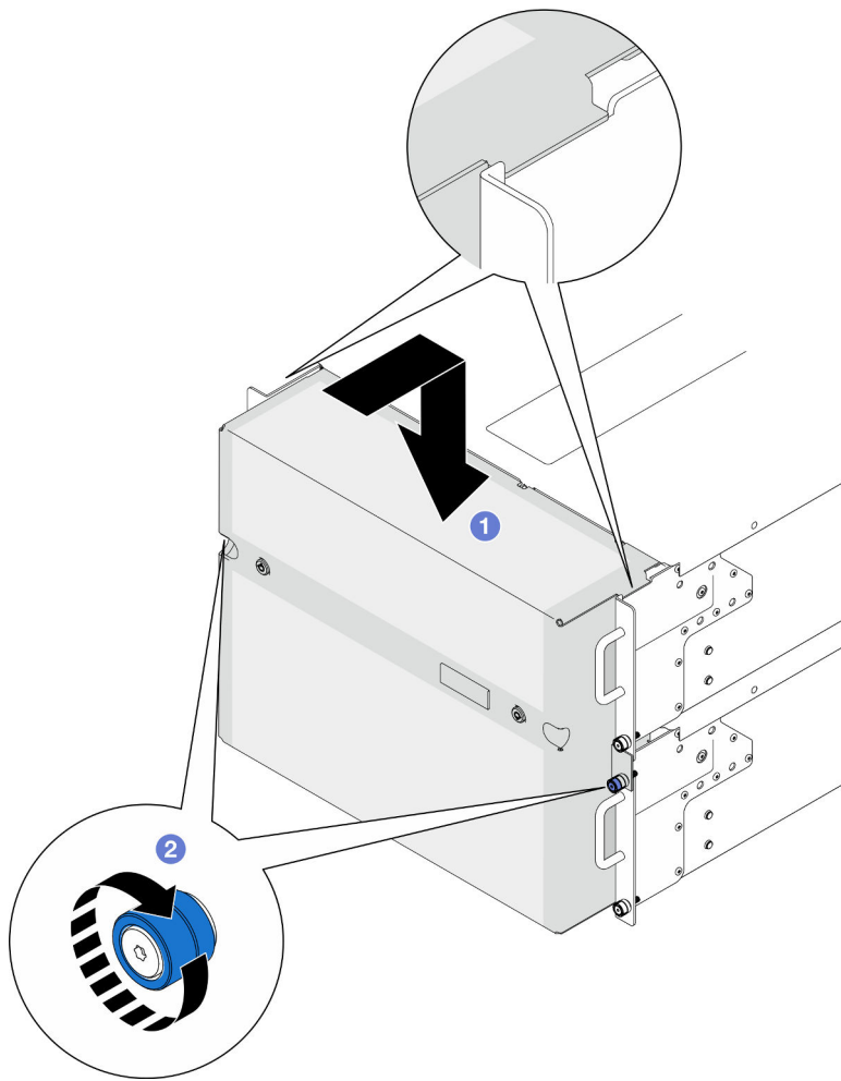
Figura 141. Instalación del marco biselado de seguridad
