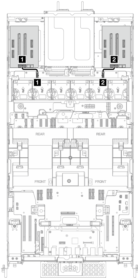
Figura 200. Disposición de los cables de alimentación de la tarjeta de expansión
