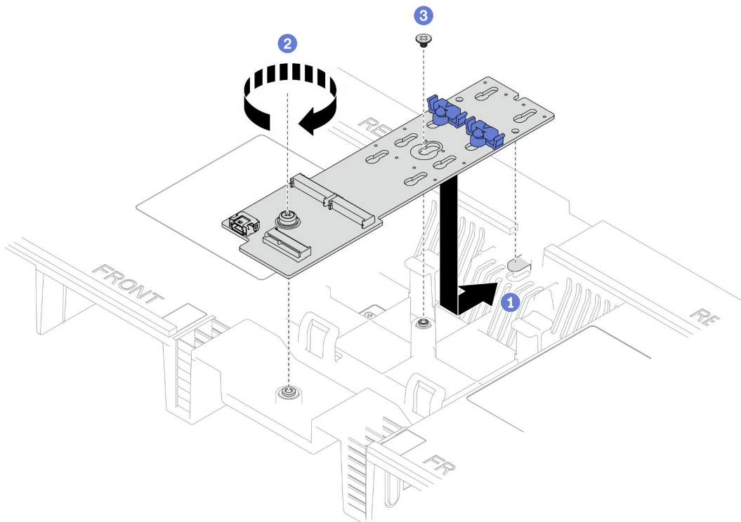
Figura 81. Instalación del adaptador de arranque M.2
