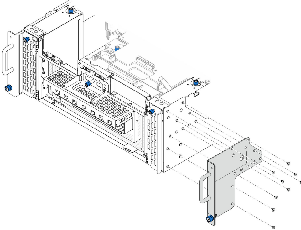
Figura 38. Instalación de la brida EIA
