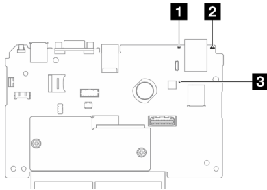
Figura 209. LED de la placa de E/S del sistema
