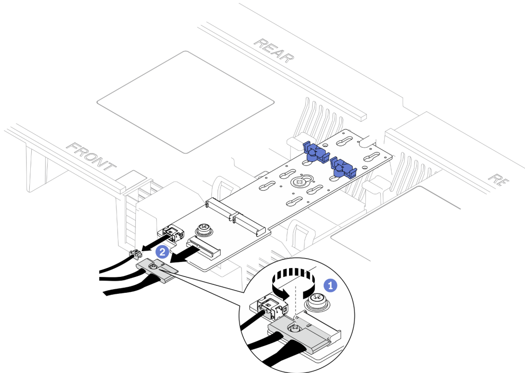
Figura 79. Desconexión del cable del adaptador de arranque M.2
