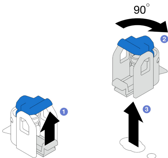
Figura 84. Extracción del elemento de sujeción de M.2
