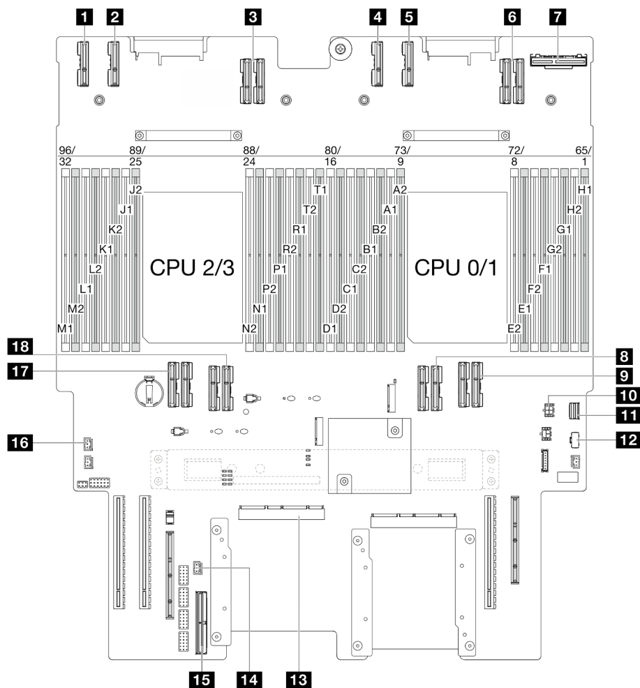
Figura 192. Conectores de la placa del procesador inferior (MB)
