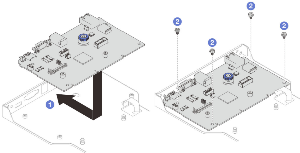
Figura 160. Instalación de la placa de E/S del sistema en la abrazadera
