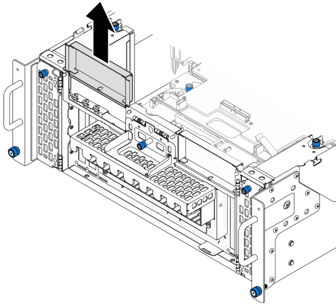
Figura 145. Extracción del relleno de PCIe izquierdo
