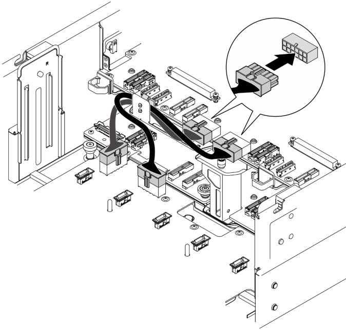
Figura 185. Conexión de los cables de alimentación de la placa del procesador superior (CPU BD)
