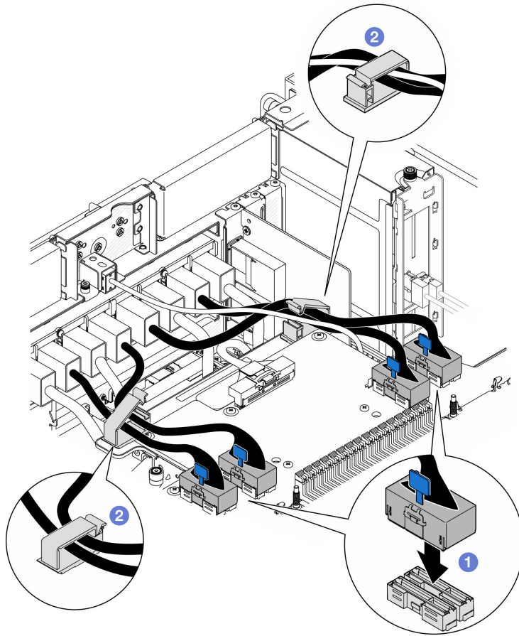
Figura 188. Conexión de los cables del módulo UPI
