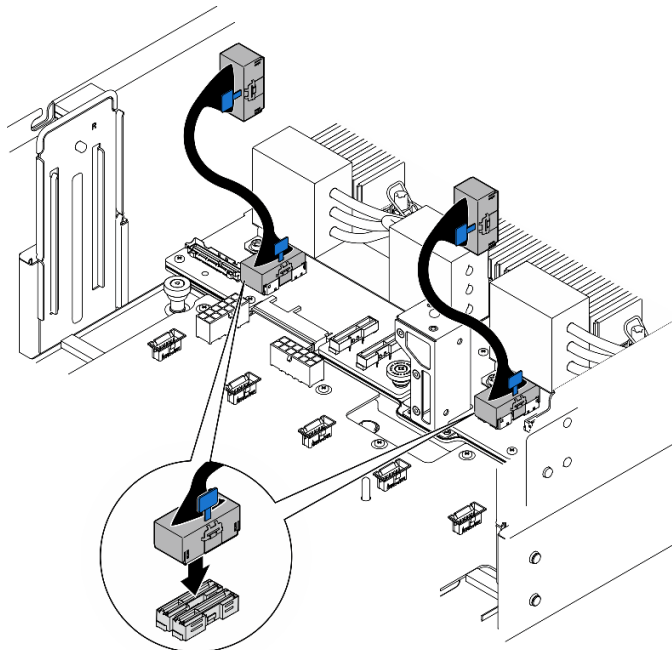
Figura 75. Conexión de los cables de UPI internos
