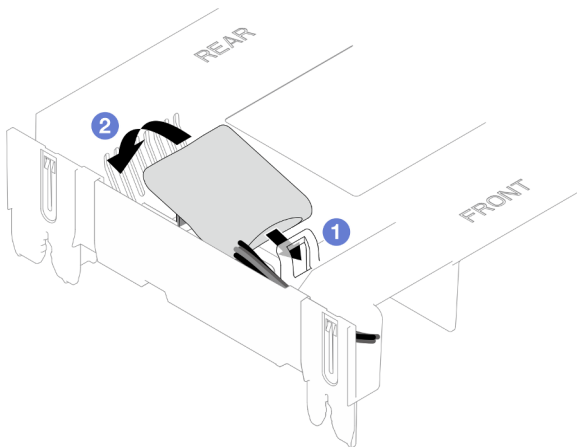
Figura 50. Instalación del módulo de alimentación flash
