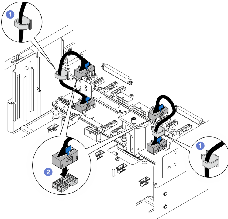
Figura 186. Conexión de los cables de UPI internos
