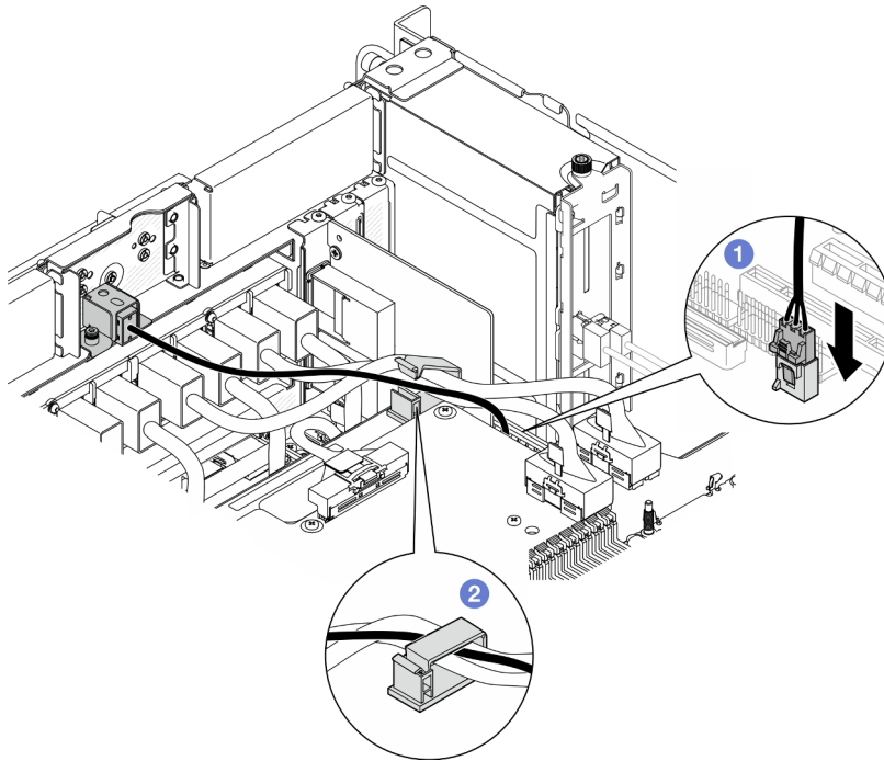
Figura 67. Conexión del conmutador de intrusión
