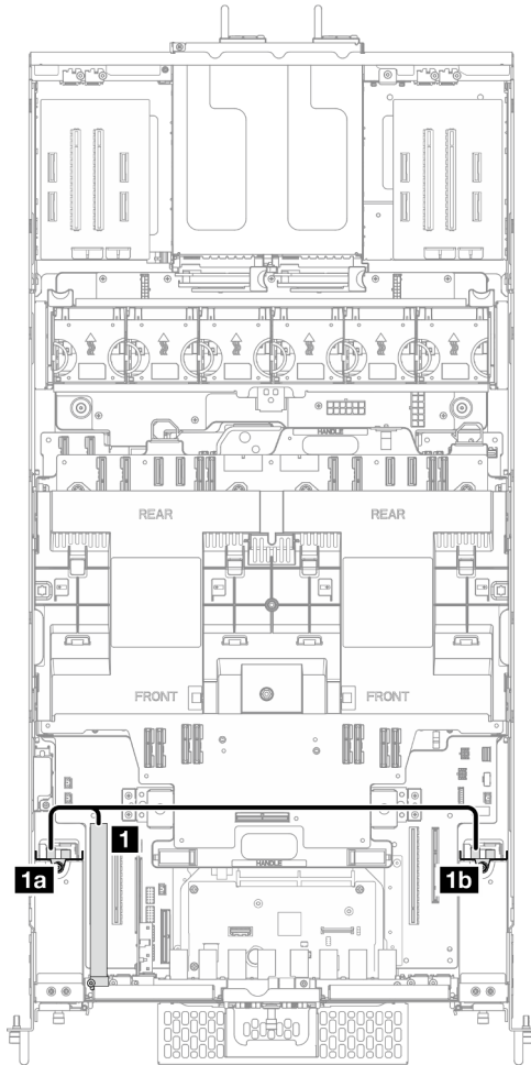
Figura 196. Disposición de los cables de dos placas posteriores de la unidad de 2,5 pulgadas
