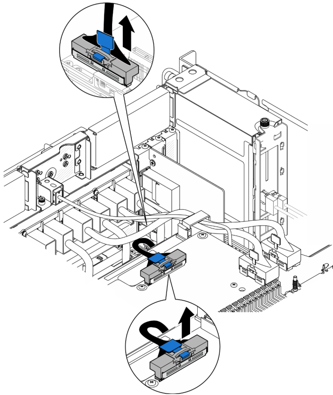
Figura 178. Desconexión del cable de banda lateral interno
