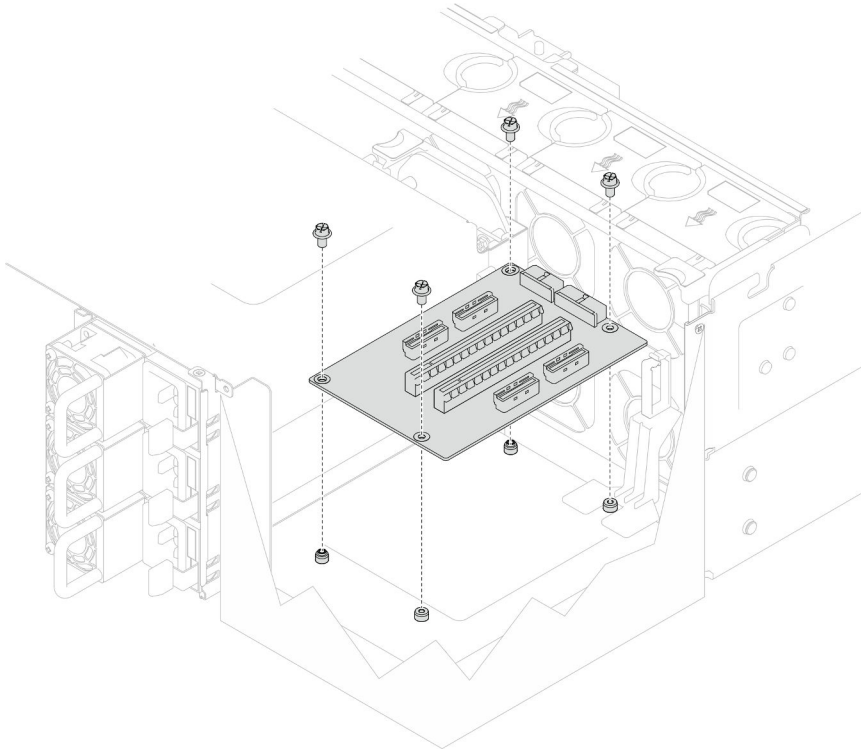
Figura 112. Instalación de la tarjeta de expansión PCIe
