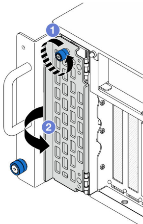
Figura 20. Apertura de la puerta de la unidad
