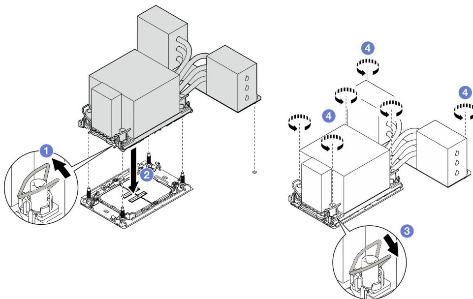
Figura 137. Instalación de un PHM 3U
