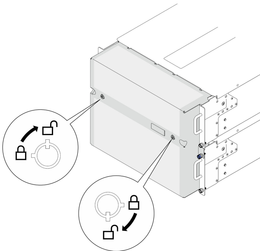
Figura 138. Desbloqueo del marco biselado de seguridad
