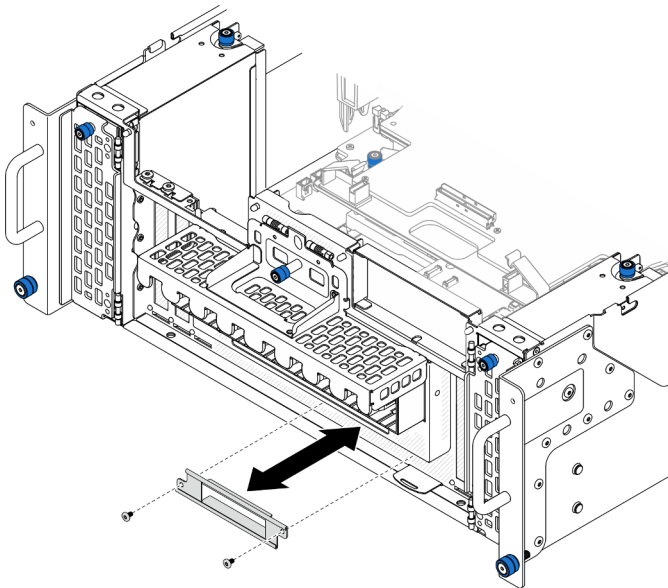
Figura 54. Extracción de la abrazadera del panel frontal del operador
