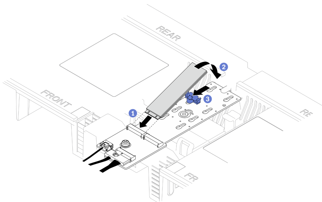
Figura 87. Instalación de una unidad M.2
