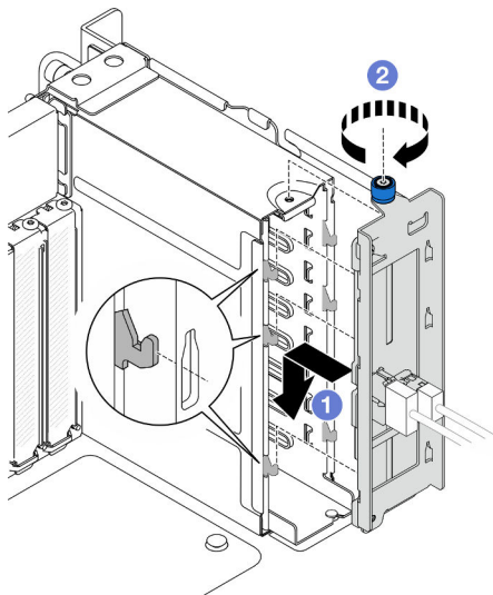
Figura 30. Instalación de una placa posterior de la unidad de 2,5 pulgadas
