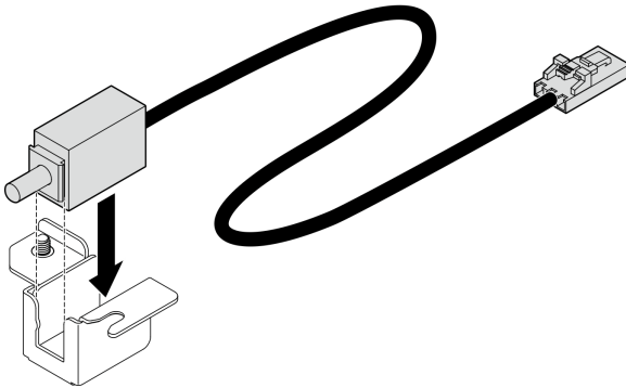
Figura 65. Instalación del conmutador de intrusión
