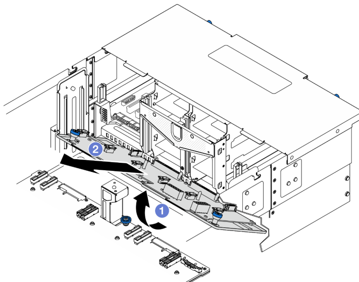
Figura 117. Extracción de la placa de distribución de alimentación
