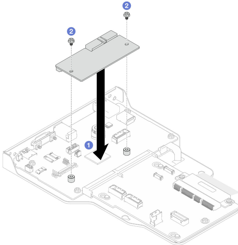
Figura 154. Instalación del firmware y el módulo de seguridad de RoT
