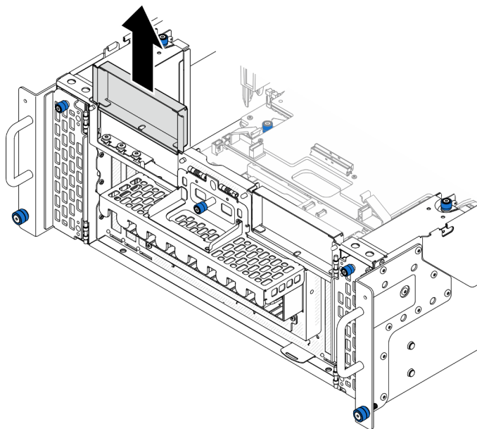
Figura 148. Extracción del relleno de PCIe izquierdo
