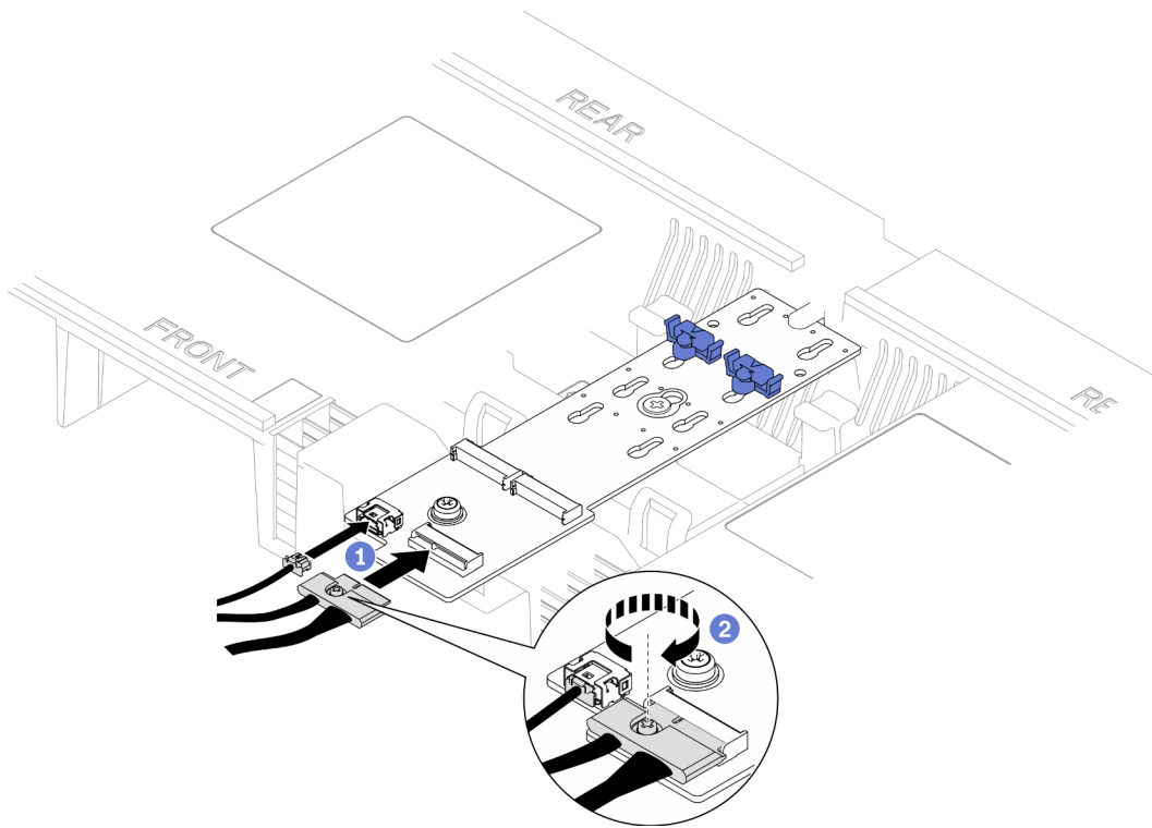
Figura 82. Conexión del cable al adaptador de arranque M.2
