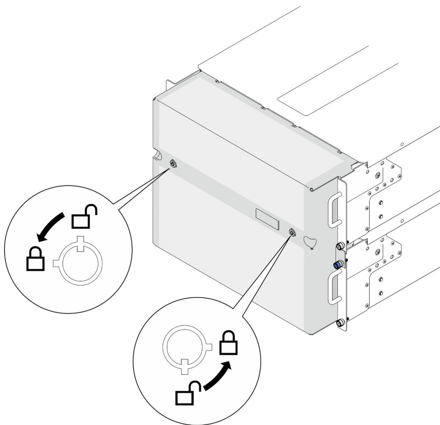
Figura 142. Bloqueo del marco biselado de seguridad
