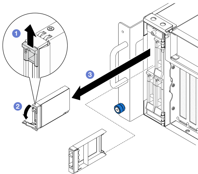
Figura 21. Extracción de una unidad de 2,5 pulgadas
