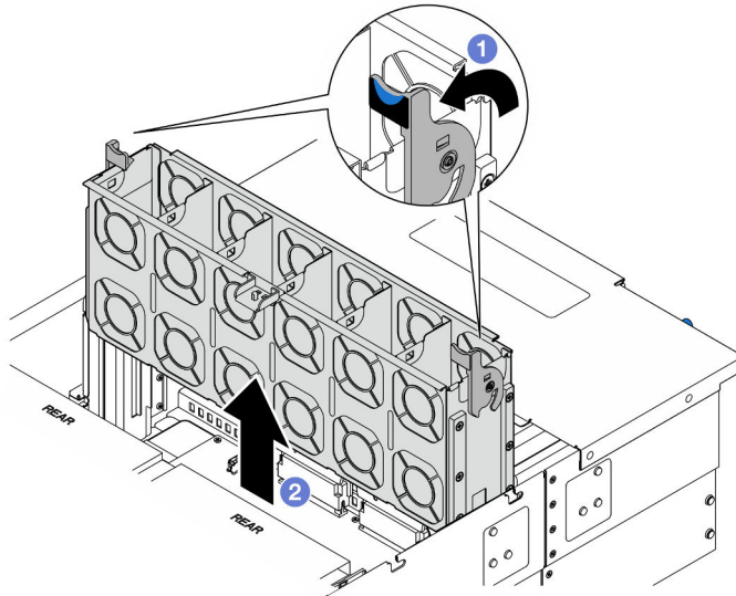
Figura 44. Extracción del compartimiento del ventilador
