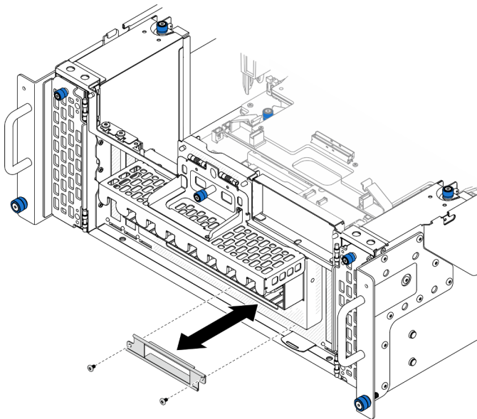
Figura 55. Instalación de la abrazadera del panel frontal del operador
