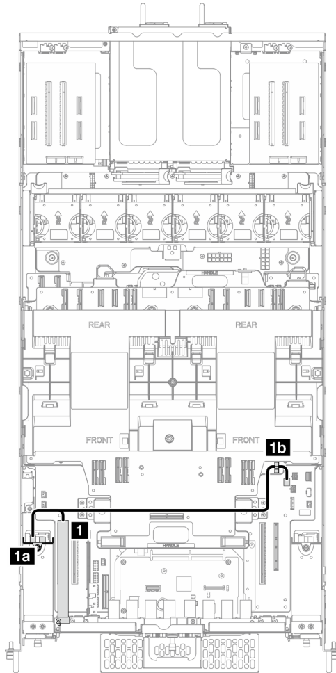
Figura 195. Disposición de los cables de una placa posterior de la unidad de 2,5 pulgadas
