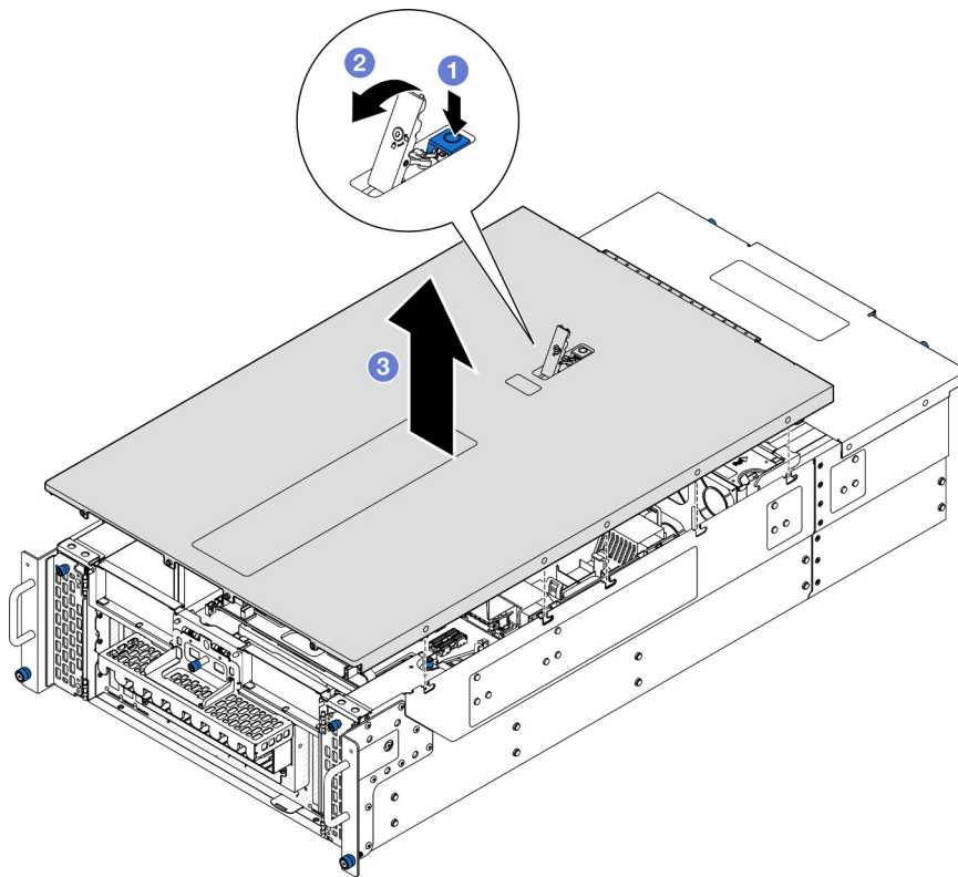
Figura 166. Extracción de la cubierta superior frontal
