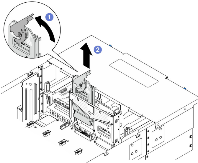
Figura 122. Extracción de la placa de interposición de alimentación
