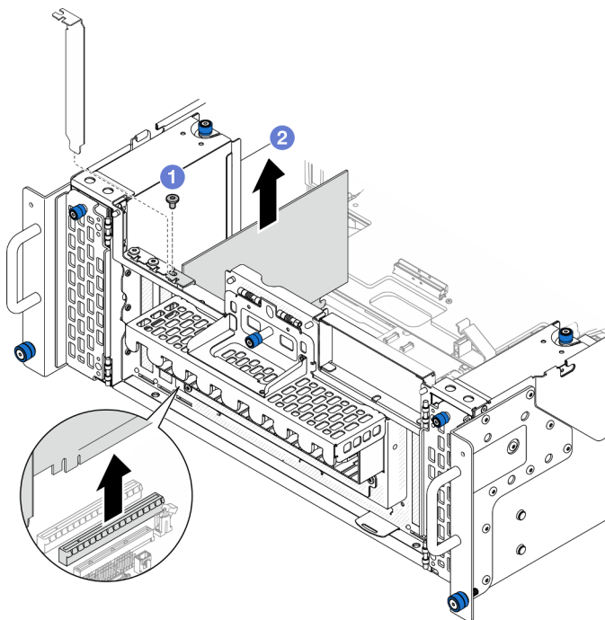
Figura 101. Extracción del adaptador PCIe
