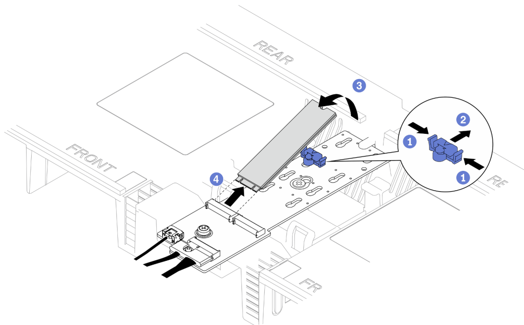
Figura 77. Extracción de la unidad M.2
