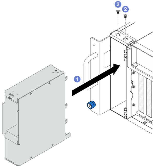
Figura 34. Instalación del compartimiento de la unidad E3.S
