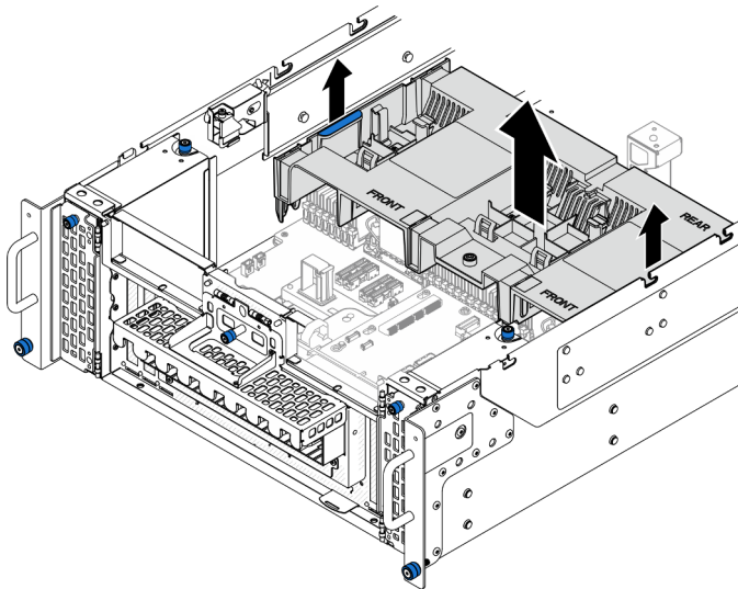
Figura 13. Extracción del deflector de aire de la placa del procesador inferior (MB)
