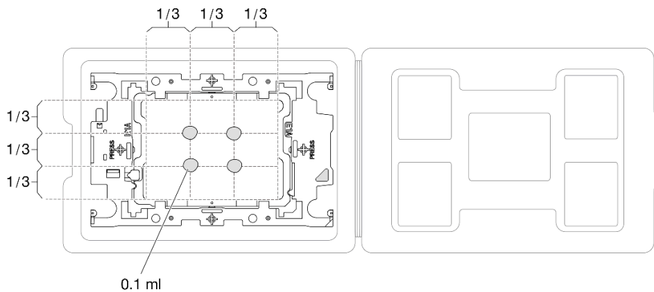
Figura 135. Aplicación de grasa térmica con el procesador en la bandeja de envío
