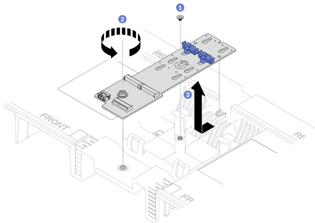
Figura 80. Extracción del adaptador de arranque M.2
