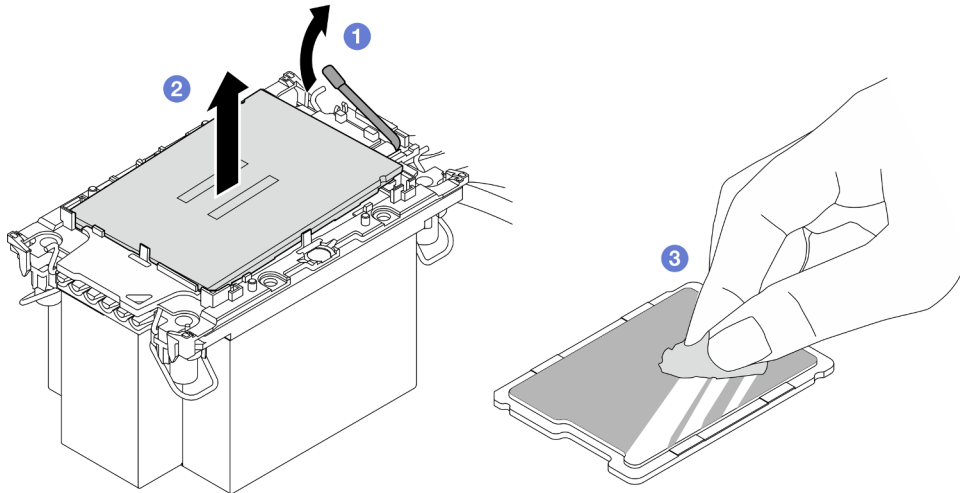
Figura 131. Separación de un procesador del disipador de calor y del transportador
