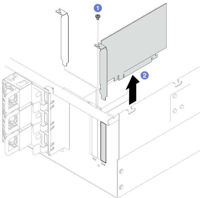
Figura 103. Extracción del adaptador PCIe
