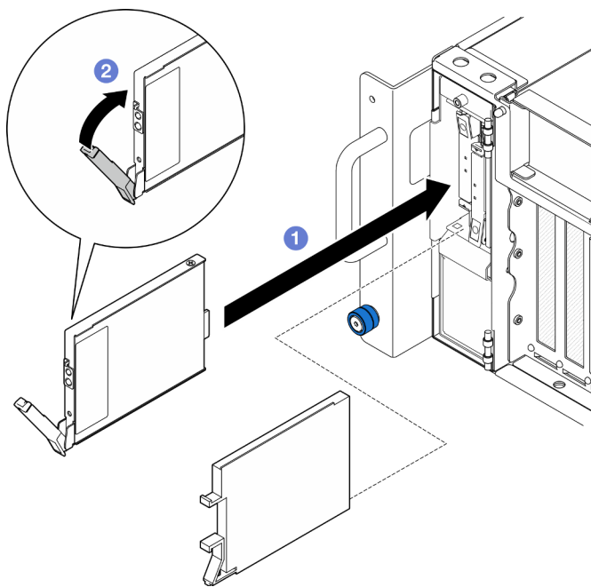
Figura 26. Instalación de una unidad E3.S
