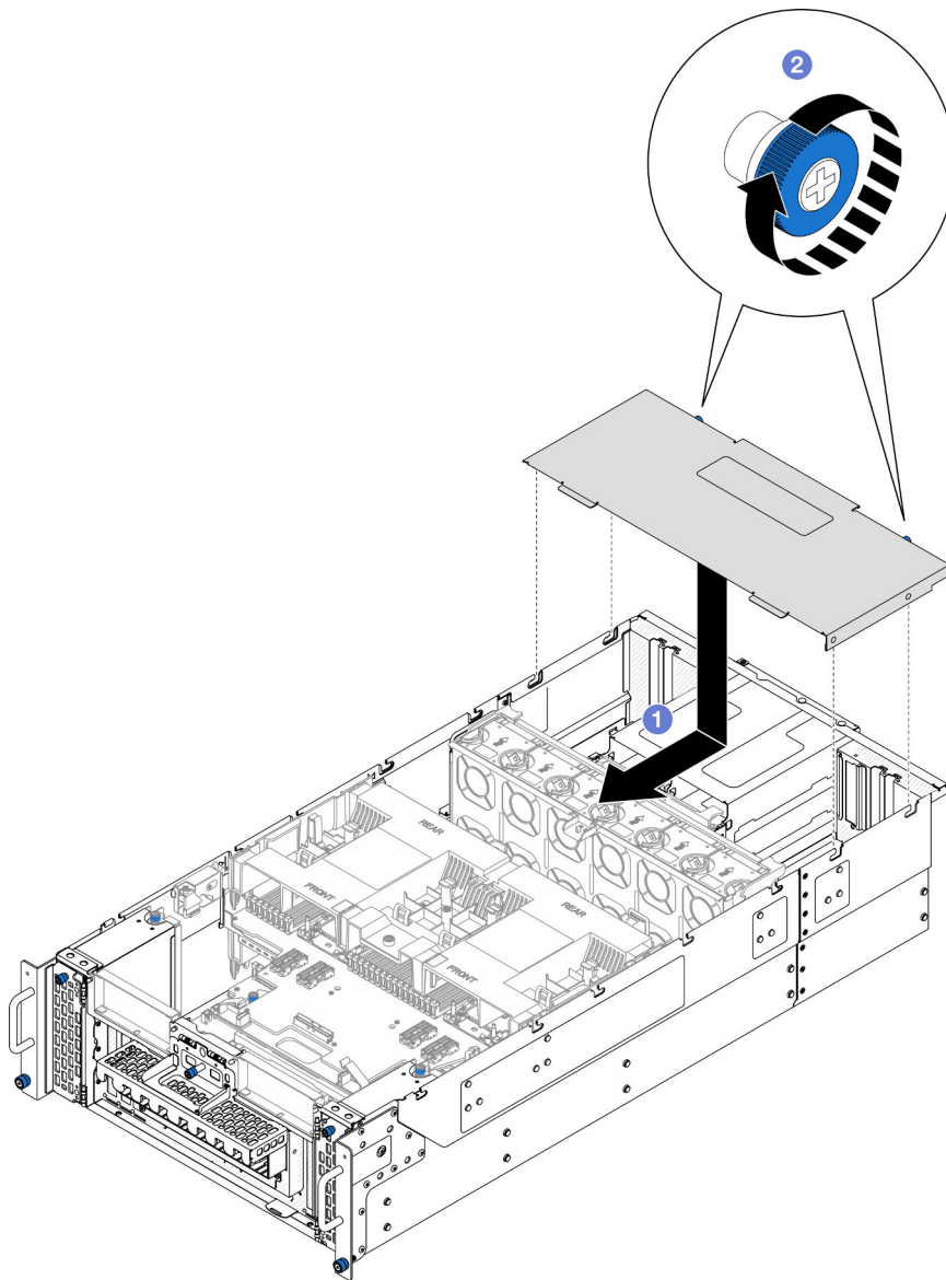
Figura 168. Instalación de la cubierta superior posterior
