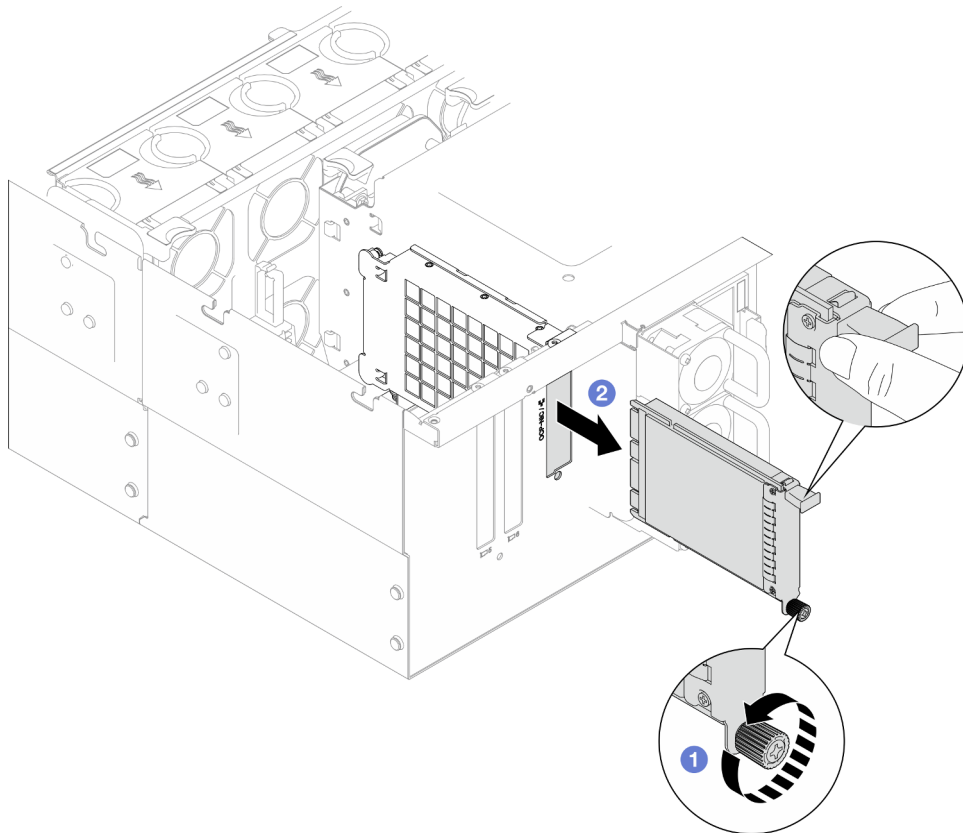
Figura 94. Extracción del módulo OCP
