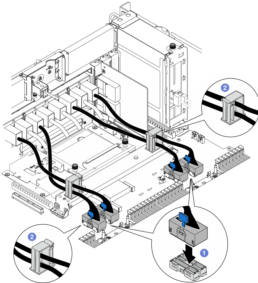
Figura 76. Conexión de los cables del módulo UPI
