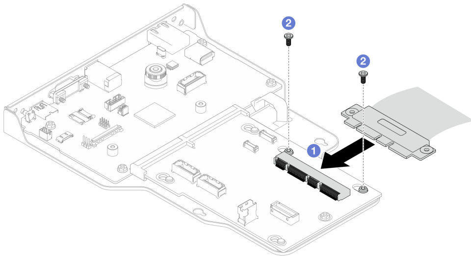
Figura 164. Conexión del cable SCM
