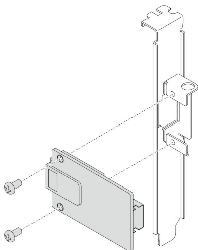
Figura 40. Extracción de la tarjeta del puerto Ethernet
