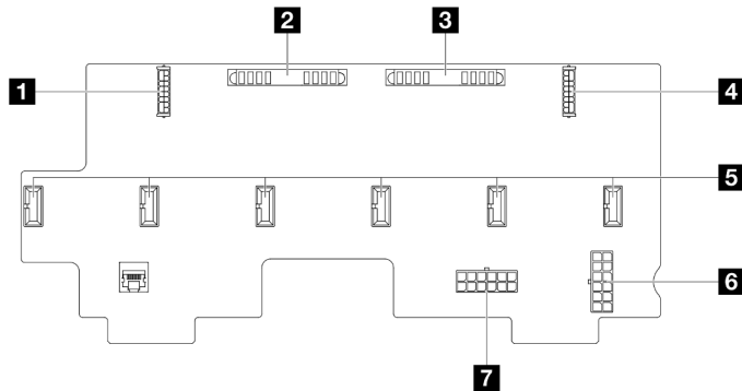
Figura 193. Conectores de placa de distribución de alimentación
