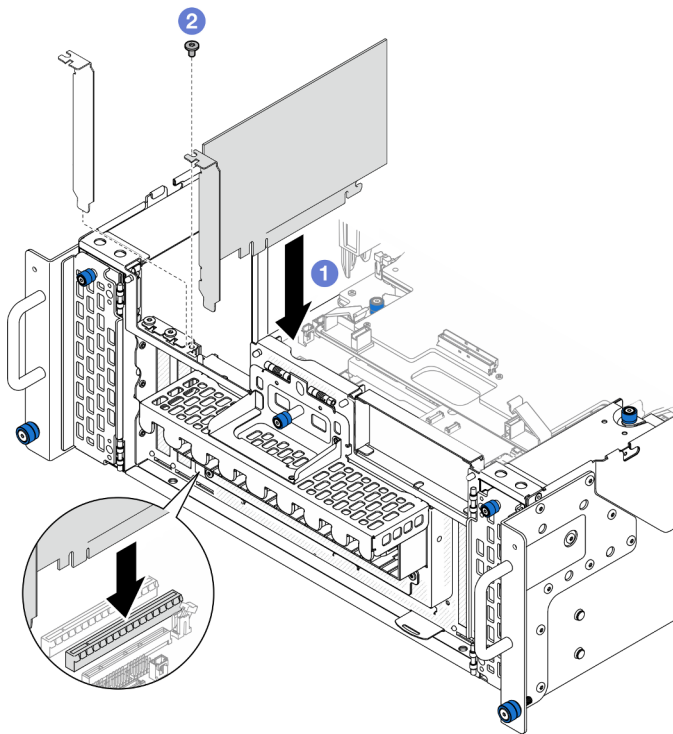
Figura 105. Instalación de un adaptador PCIe
