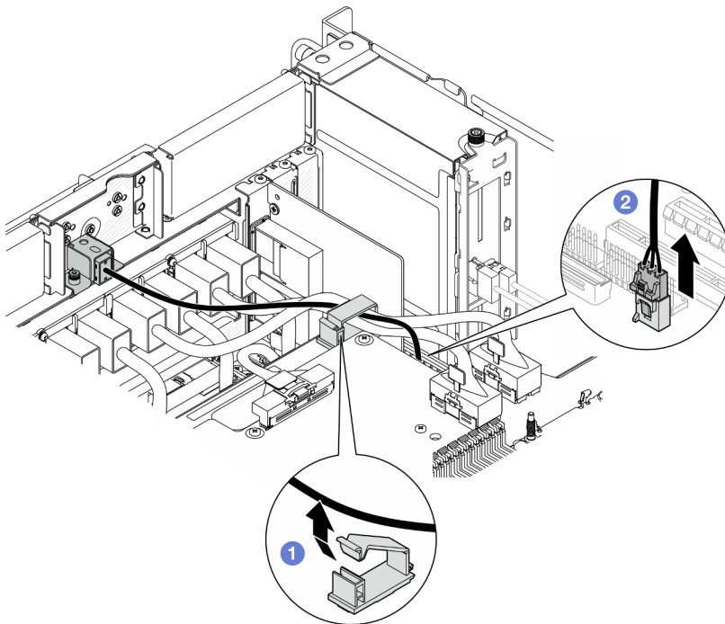
Figura 62. Desconexión del conmutador de intrusión
