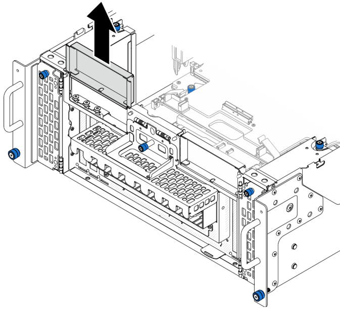
Figura 104. Extracción del relleno de PCIe izquierdo
