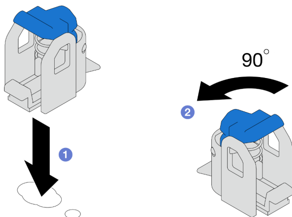
Figura 85. Instalación del elemento de sujeción de M.2
