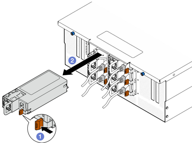
Figura 126. Extracción de la fuente de alimentación
