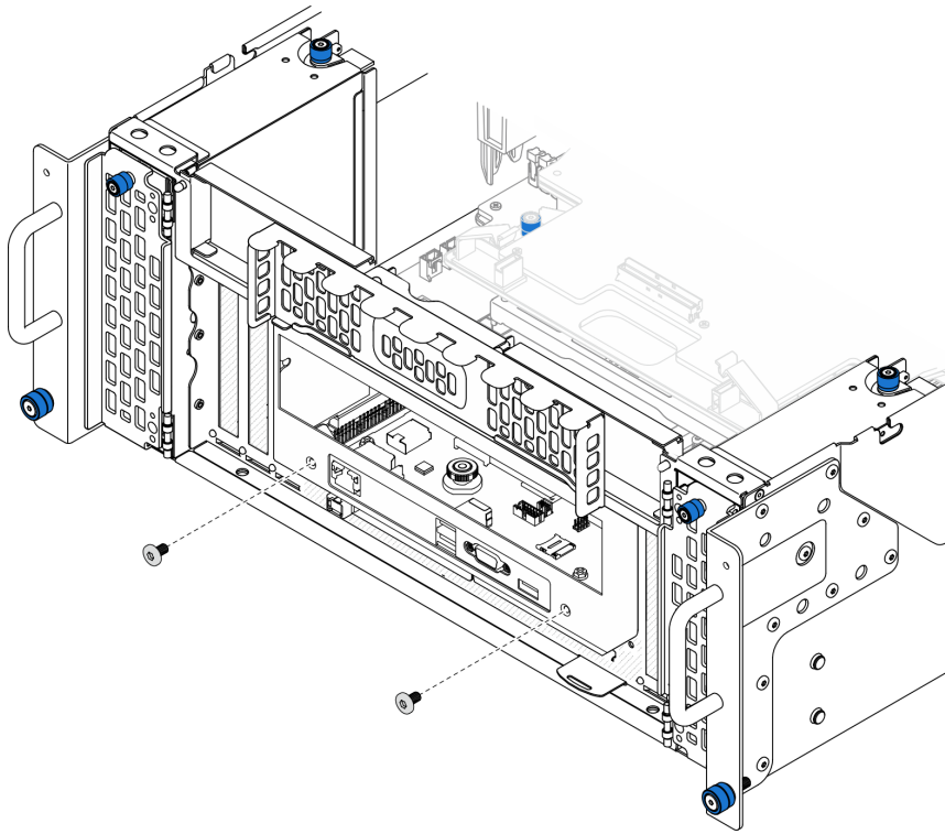
Figura 163. Fijación del conjunto de la placa de E/S y de interposición del sistema
