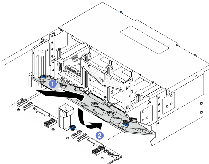
Figura 119. Instalación de la placa de distribución de alimentación
