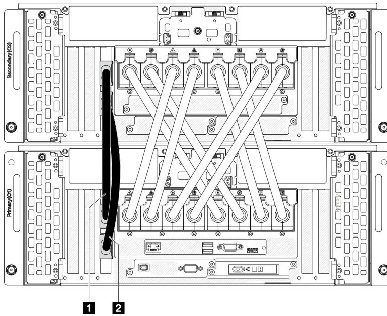
Figura 3. Desconexión de los cables de banda lateral
