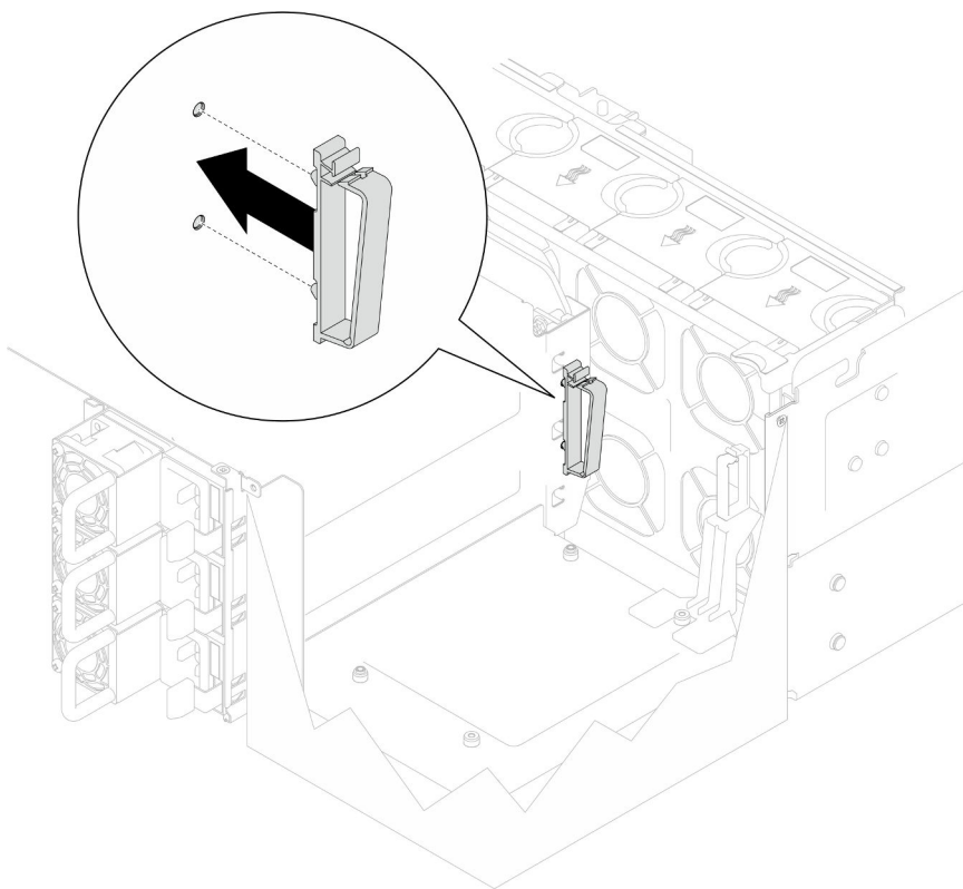
Figura 111. Instalación de la guía de cables
