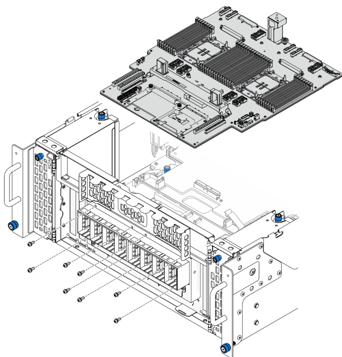
Figura 175. Instalación de los tornillos del módulo UPI
