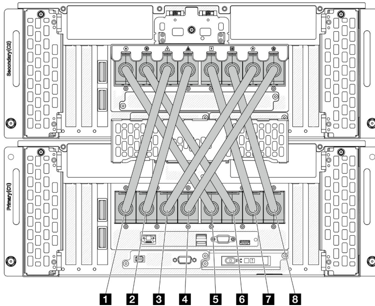
Figura 6. Conexión de los cables de UPI externos
