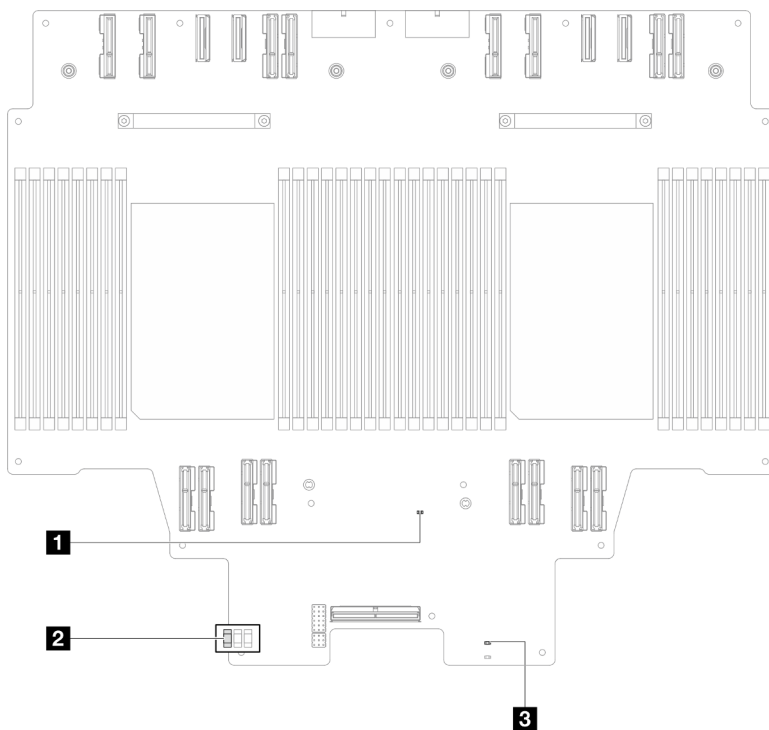
Figura 208. LED de la placa del procesador superior (CPU BD)
