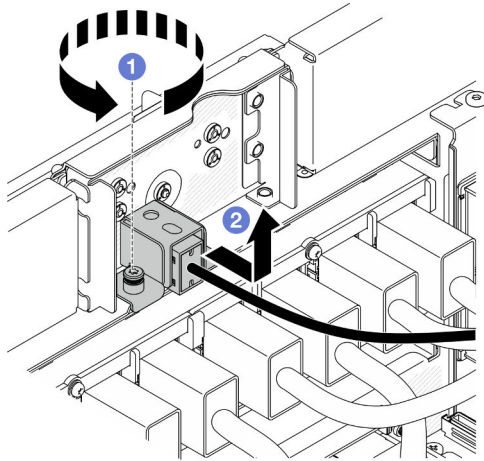
Figura 63. Extracción del conjunto del conmutador de intrusión frontal
