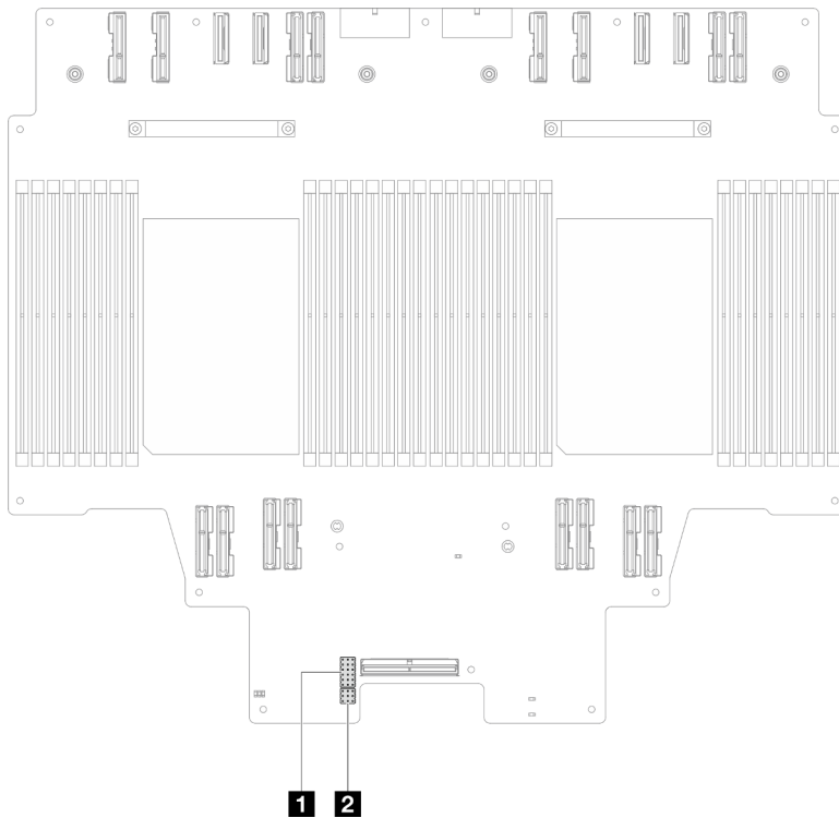
Figura 10. Switch della scheda del processore superiore (CPU BD)
