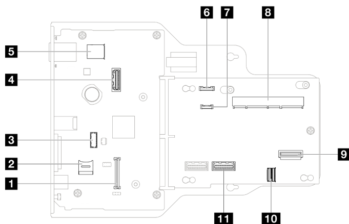
Figura 11. Connettori della scheda I/O di sistema e dell'assieme interposer
