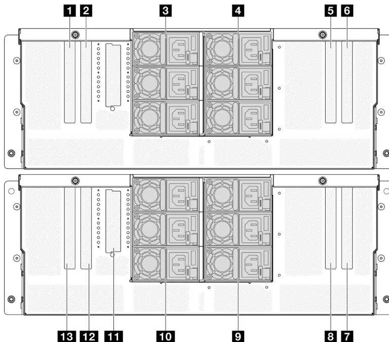
Figura 5. Vista posteriore
