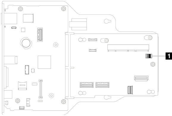
Figura 12. Switch della scheda I/O di sistema e dell'assieme interposer
