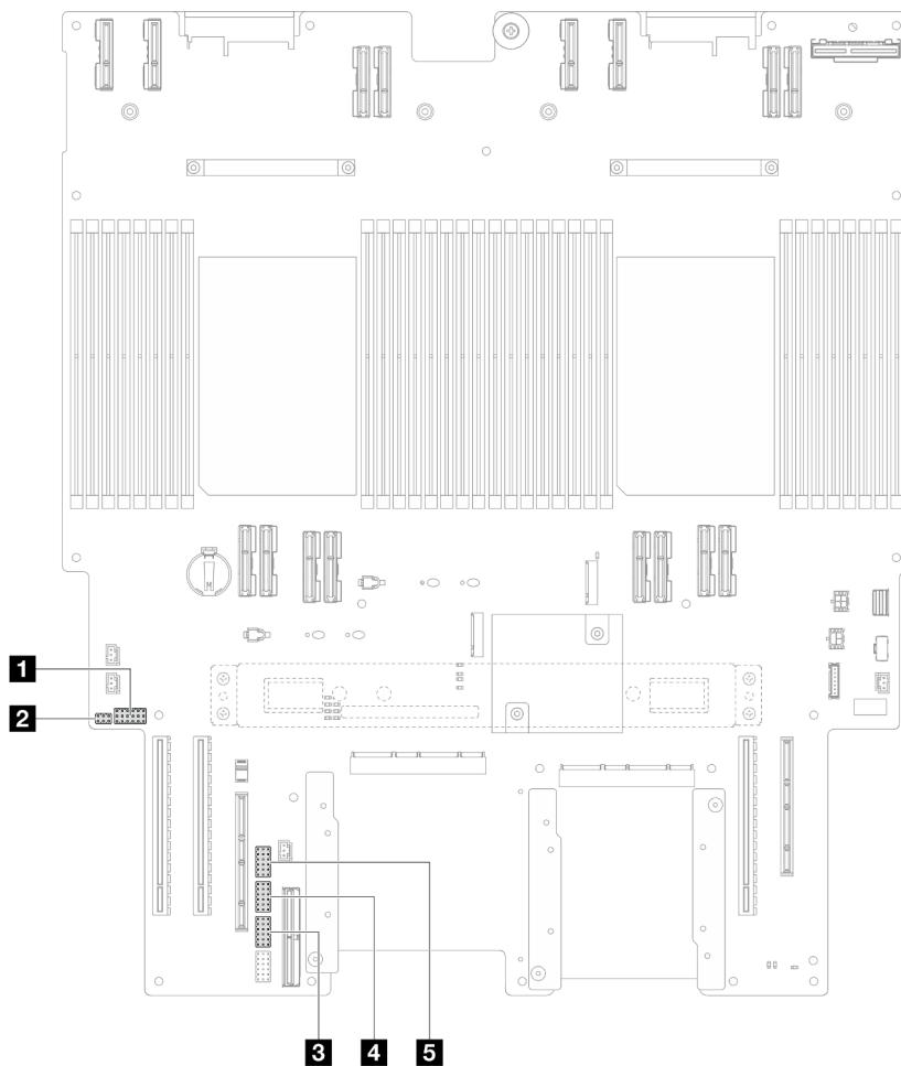
Figura 14. Switch della scheda del processore inferiore (MB)
