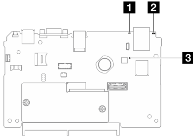
Figura 20. LED della scheda I/O di sistema
