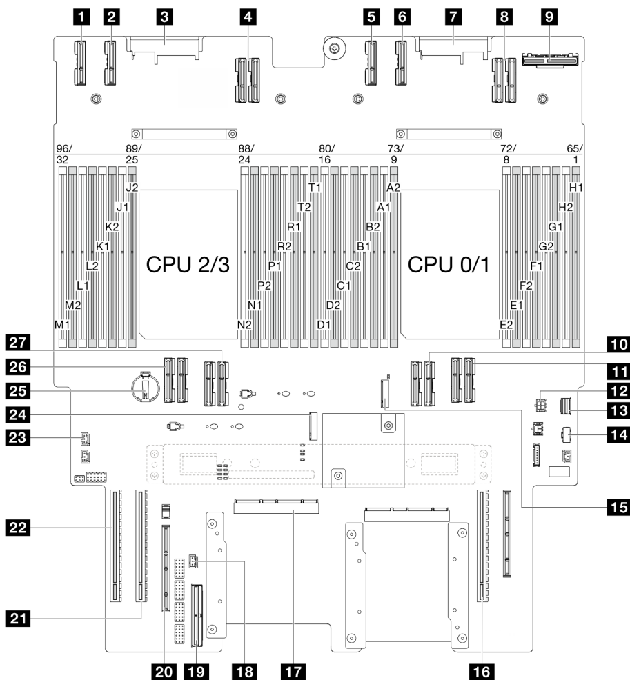
Figura 13. Connettori della scheda del processore inferiore (MB)
