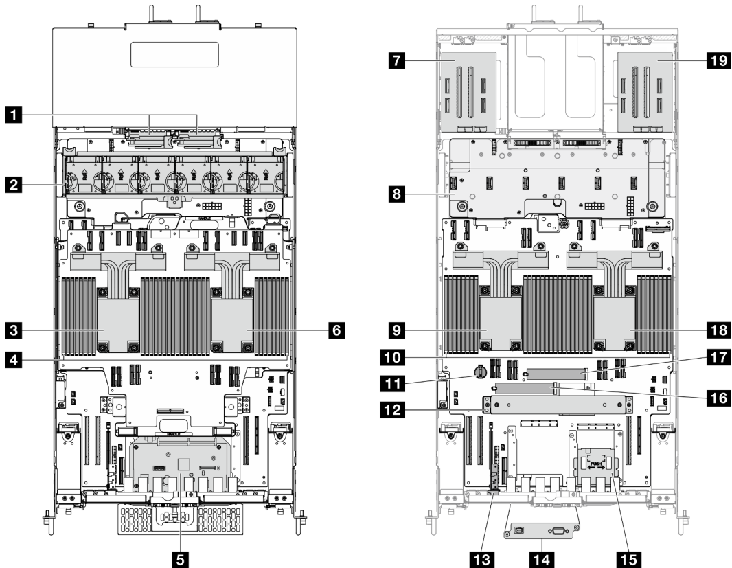
Figura 8. Vista superiore del server
