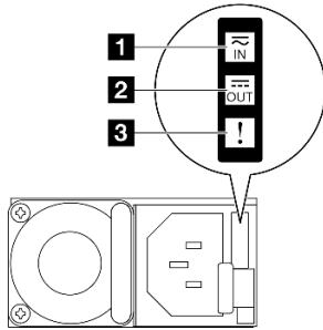
Figura 18. LED dell'alimentatore
