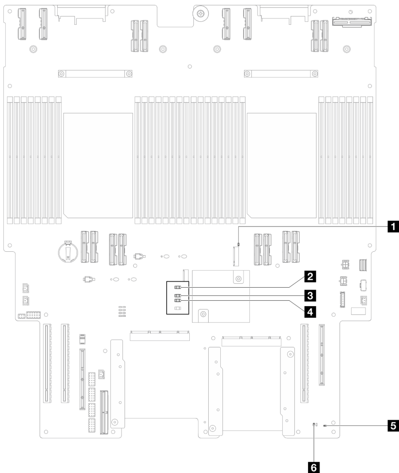
Figura 21. LED della scheda del processore inferiore (MB)
