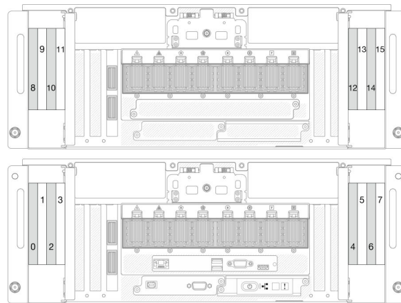
Figura 4. Numeri vani delle unità E3.S
