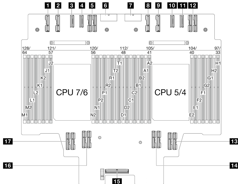
Figura 9. Connettori della scheda del processore superiore (CPU BD)
