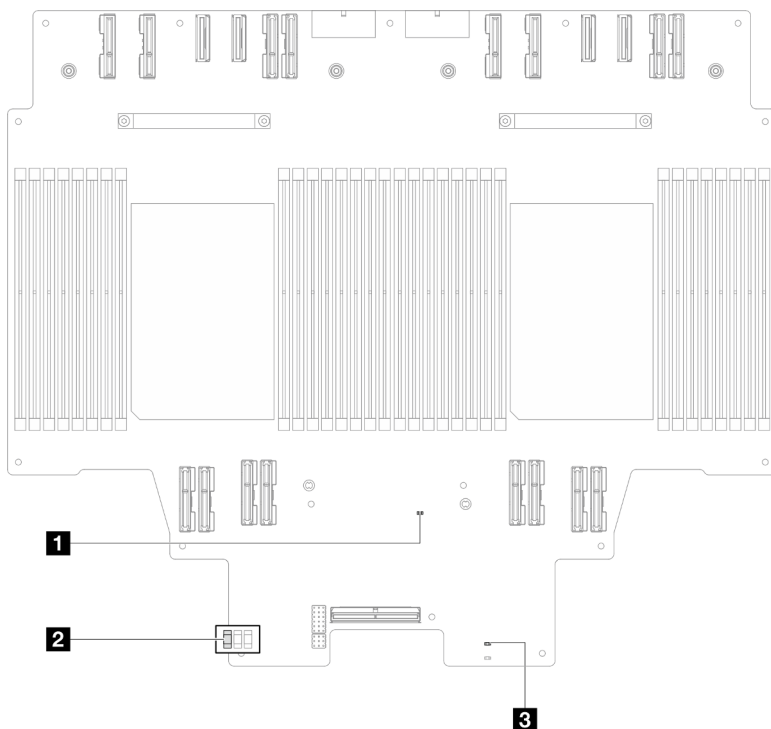
Figura 19. LED della scheda del processore superiore (CPU BD)
