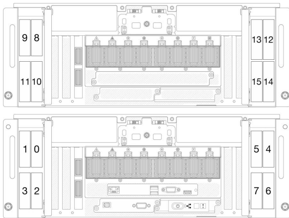
Figura 3. Numerazione del vano dell'unità da 2,5"
