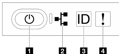
Figura 17. LED del pannello anteriore dell'operatore
