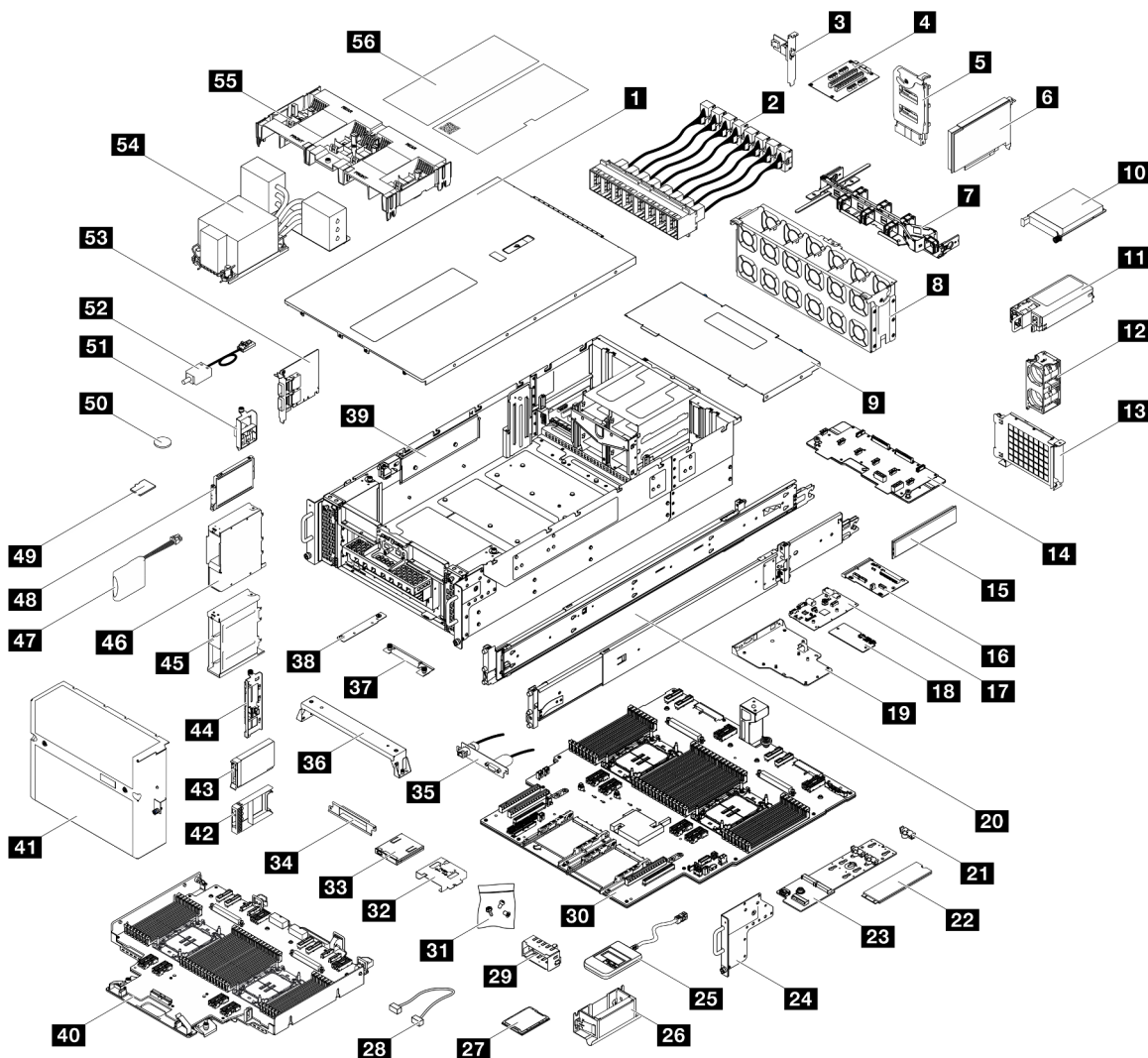
Figura 24. Componenti del server
