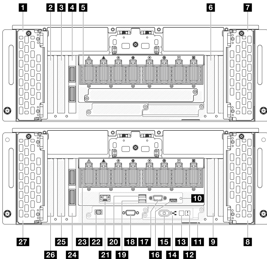
Figura 2. Vista anteriore dello chassis primario
