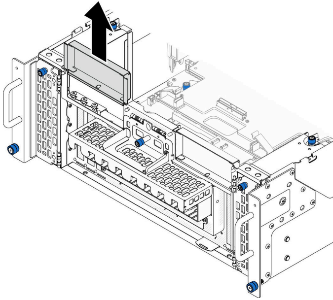
図 148. 左の PCIe フィラーの取り外し
