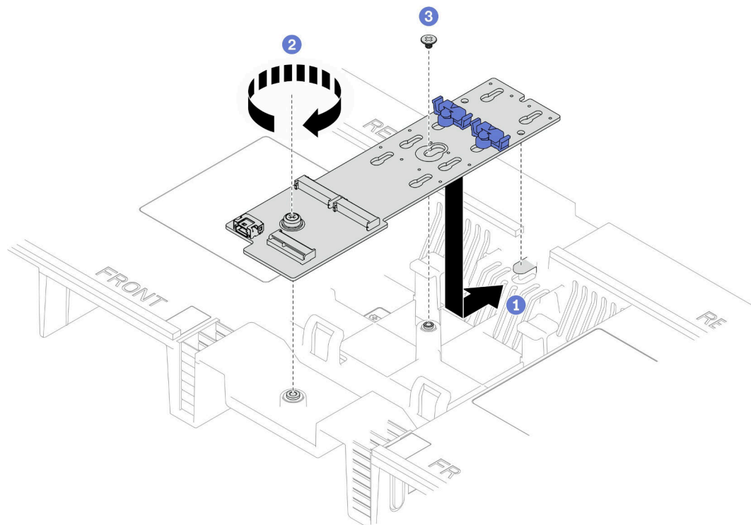
図 81. M.2 ブート・アダプターの取り付け
