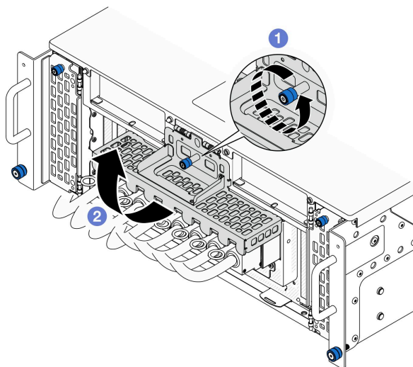
図4. UPIカバーを開く
