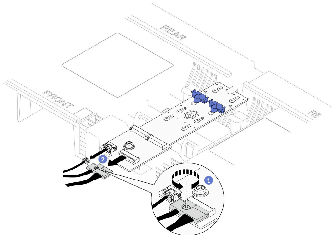
図9. M.2 ブート・アダプターからのケーブルの切り離し
