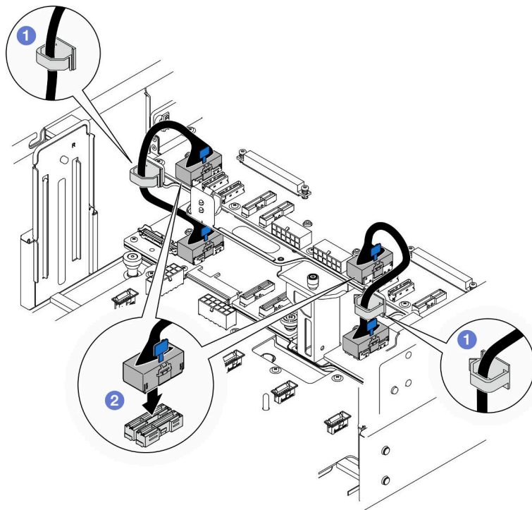
図 186. 内部 UPI ケーブルの接続
