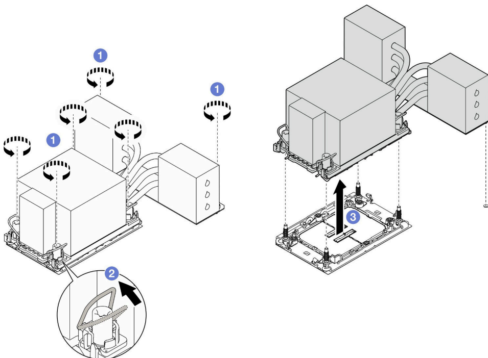
図 130. 3U PHM の取り外し
