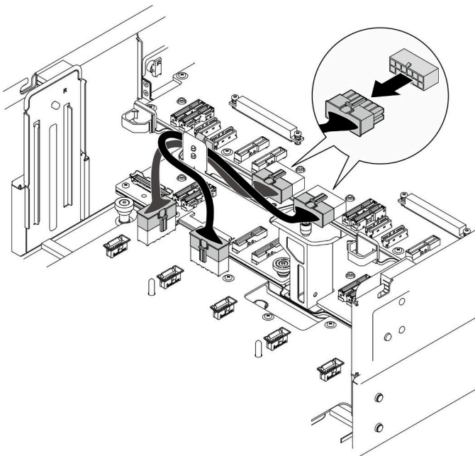
図 180. 上段のプロセッサ・ボード (CPU BD) の電源ケーブルの取り外し
