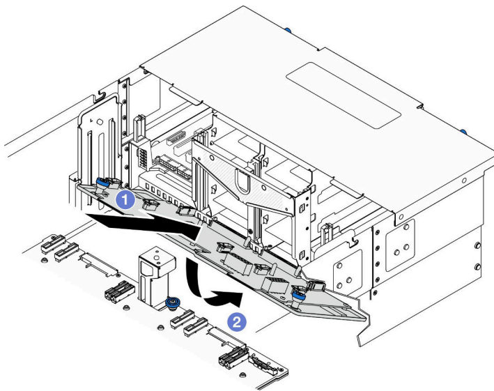
図 119. 分電盤の取り付け
