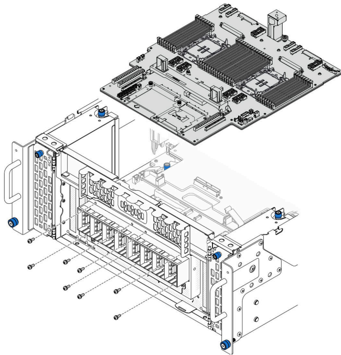
図 172. UPI モジュールのねじの取り外し
