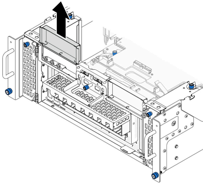
図 145. 左の PCIe フィラーの取り外し
