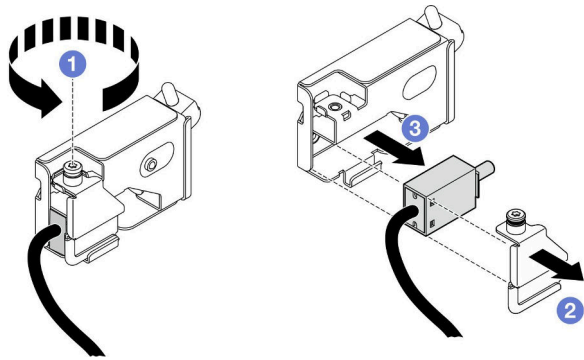
図 59. トップ・カバーの侵入検出スイッチの取り外し
