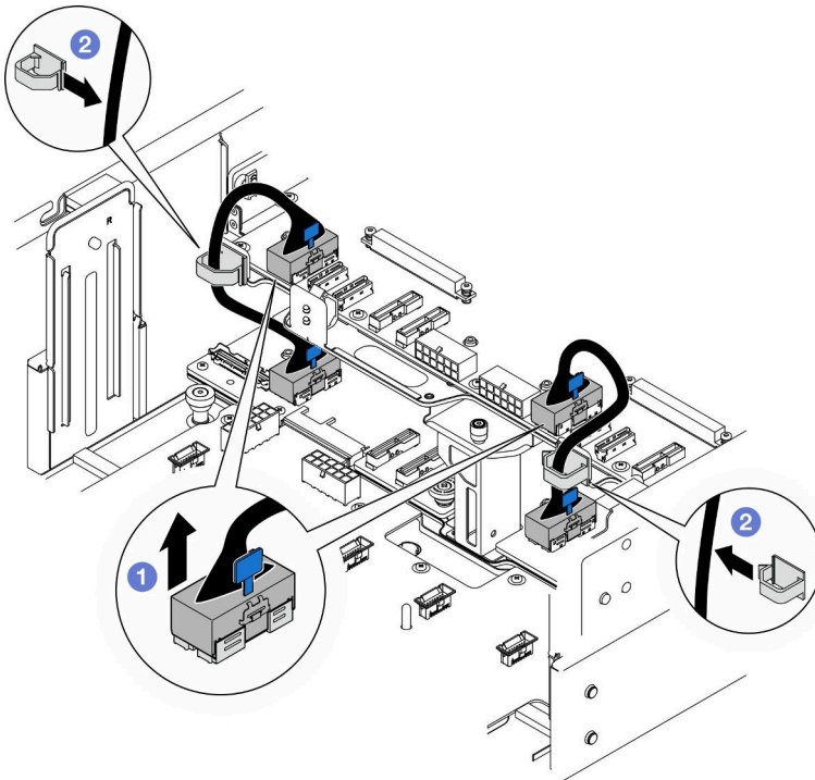
図 179. 内部 UPI ケーブルの取り外し
