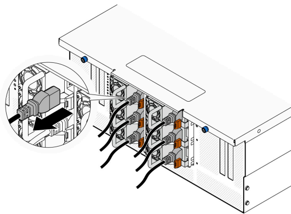
図 125. 電源コードの取り外し
