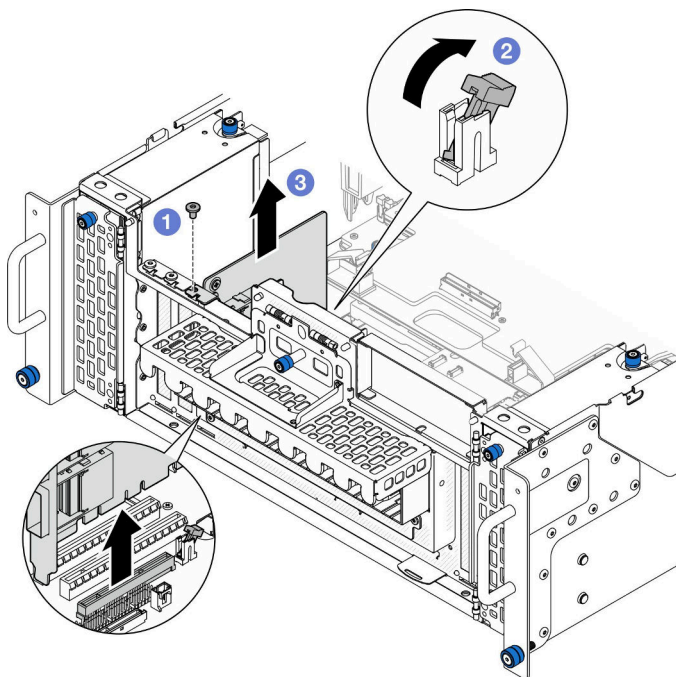
図 146. 側波帯カードの取り外し
