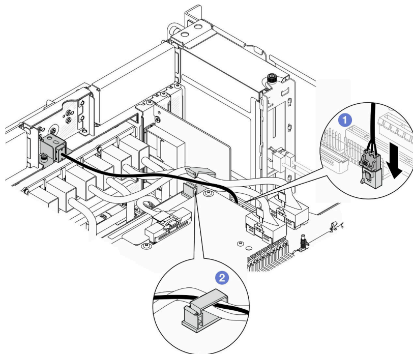
図 67. 侵入検出スイッチの接続
