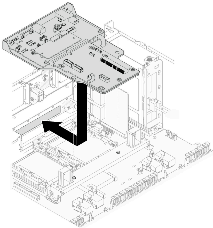
図 162. システム I/O ボードおよび変換コネクタ・アセンブリの取り付け
