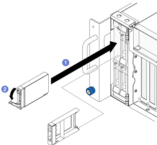
図25. 2.5型ドライブの取り付け
