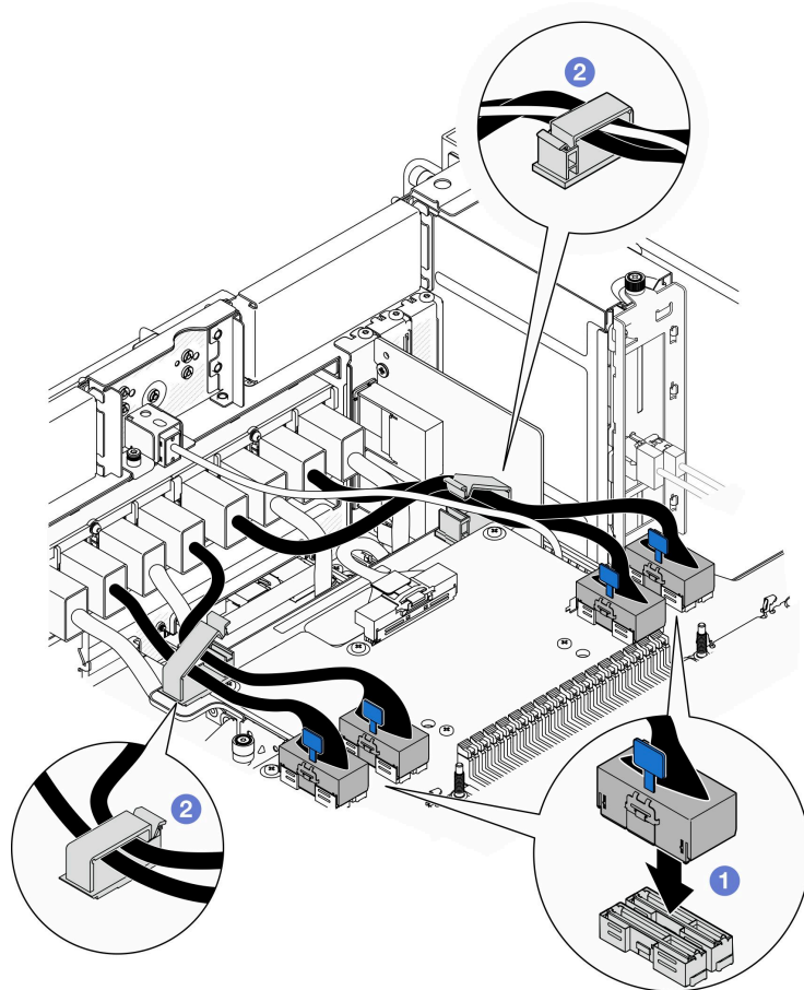
図188. UPI モジュール・ケーブルの接続
