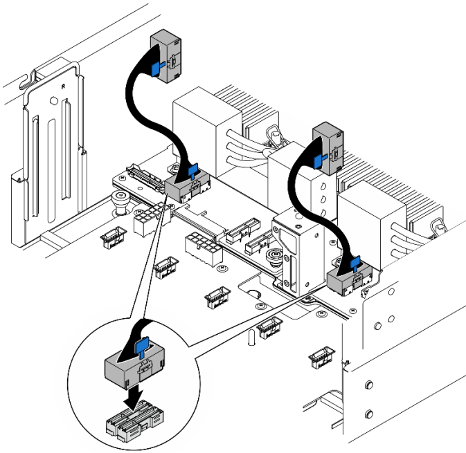
図75. 内部 UPI ケーブルの接続
