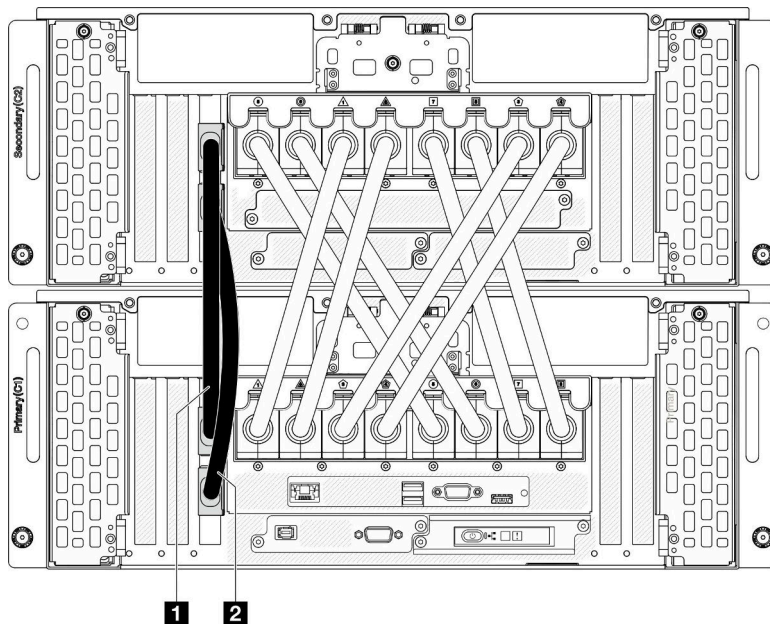
図3. 側波帯ケーブルの切り離し
