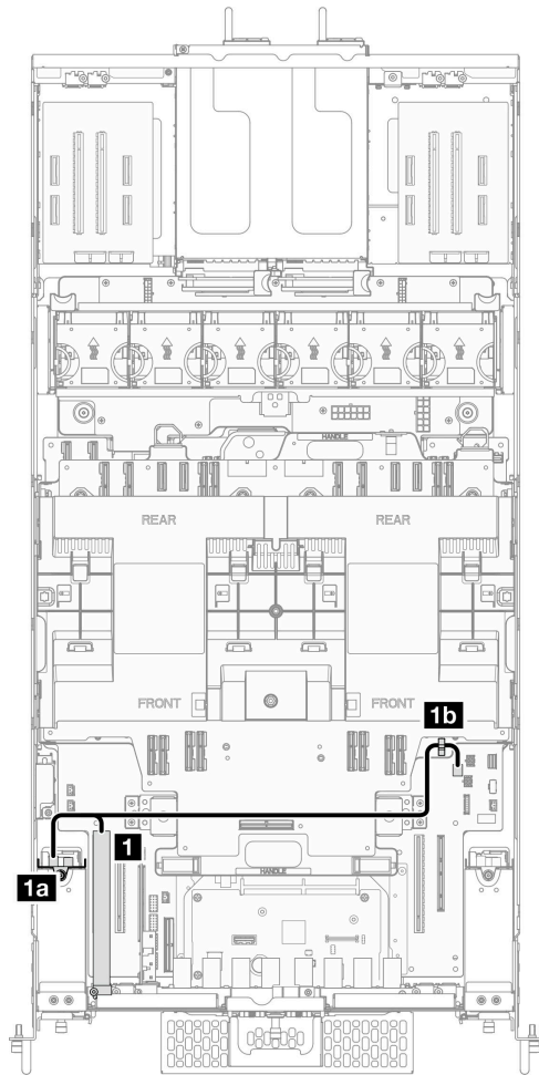
図195. 1つの2.5型ドライブ・バックプレーンのケーブル配線
