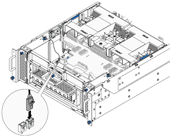
図 61. 侵入検出スイッチの接続
