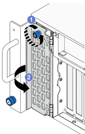
図20. ドライブ・ドアを開く
