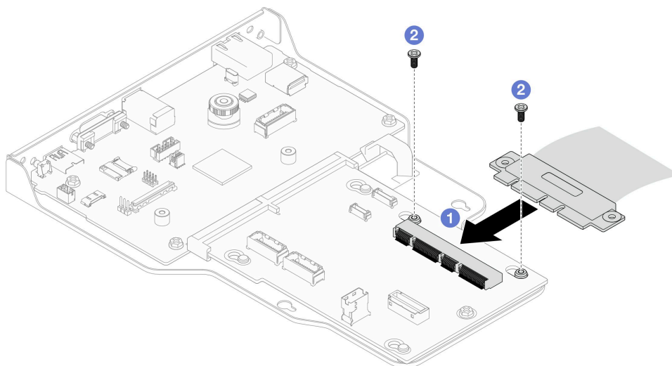
図 164. SCM ケーブルの接続
