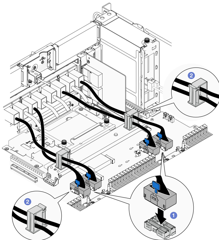
図 76. UPI モジュール・ケーブルの接続
