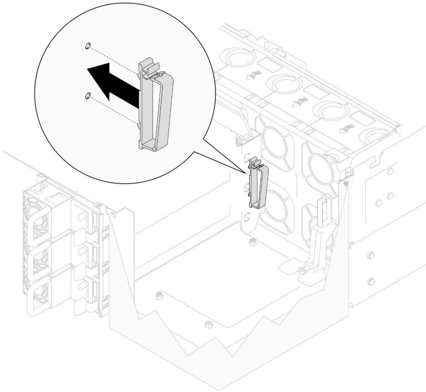
図111. ケーブル・ガイドの取り付け
