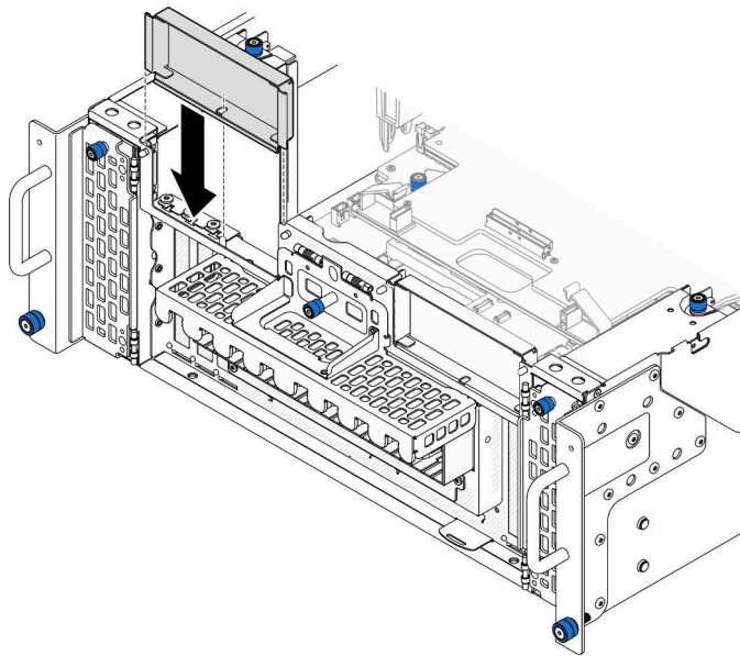
図106. 左の PCIe フィラーの取り付け
