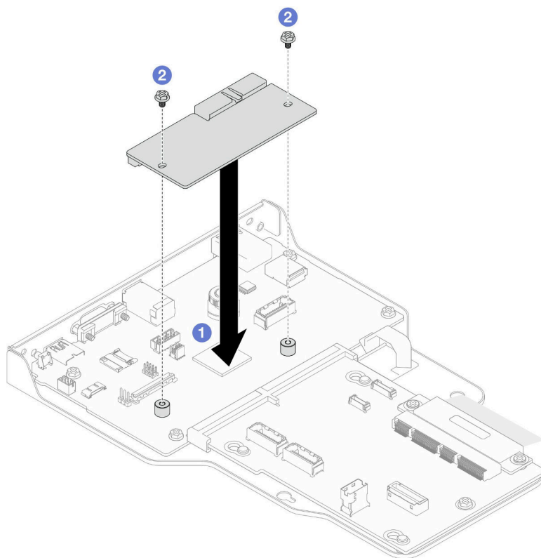
図 154. ファームウェアおよび RoT セキュリティー・モジュールの取り付け
