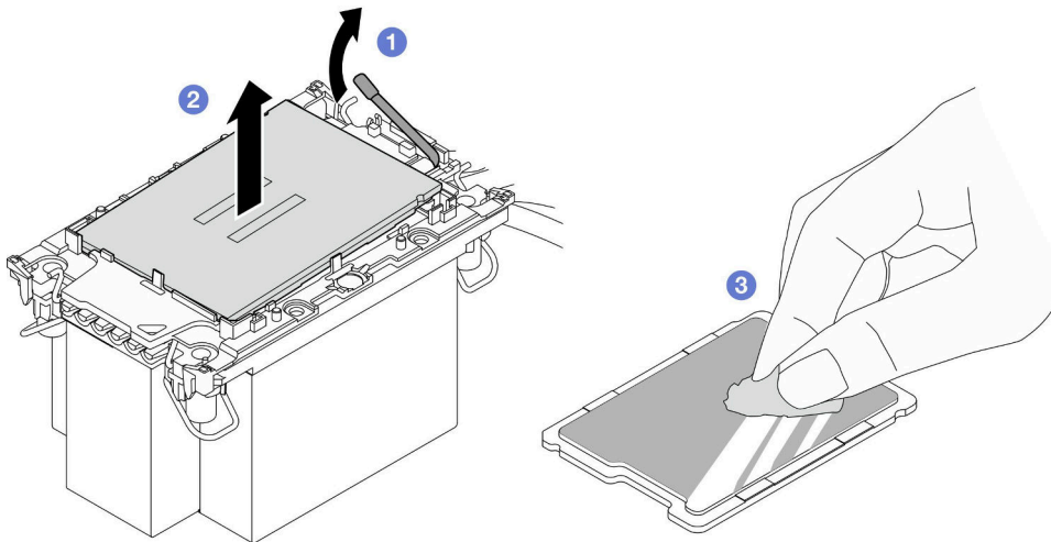
図 131. プロセッサをキャリアとヒートシンクから取り外す
