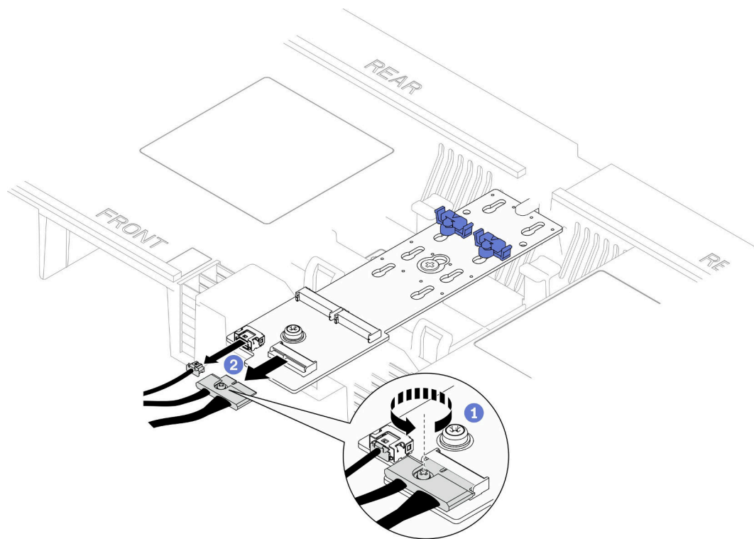
図 79. M.2 ブート・アダプターからのケーブルの切り離し
