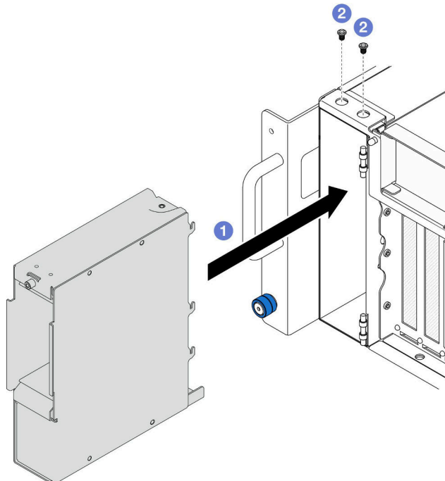
図 34. E3.S ドライブ・ケージの取り付け
