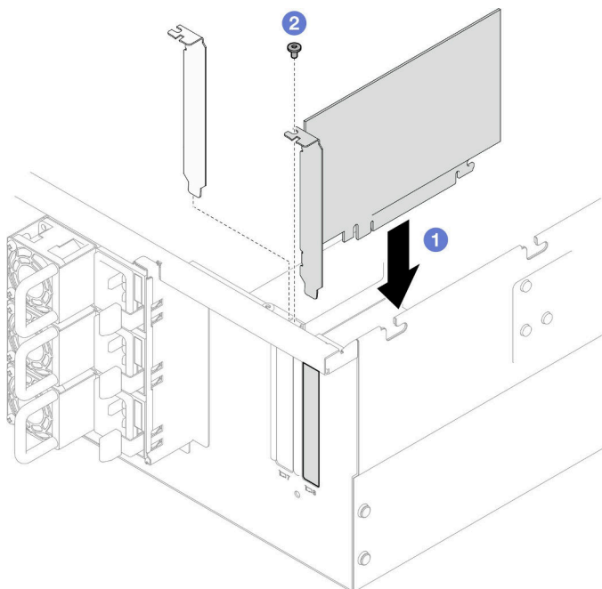
図 107. PCIe アダプターの取り付け
