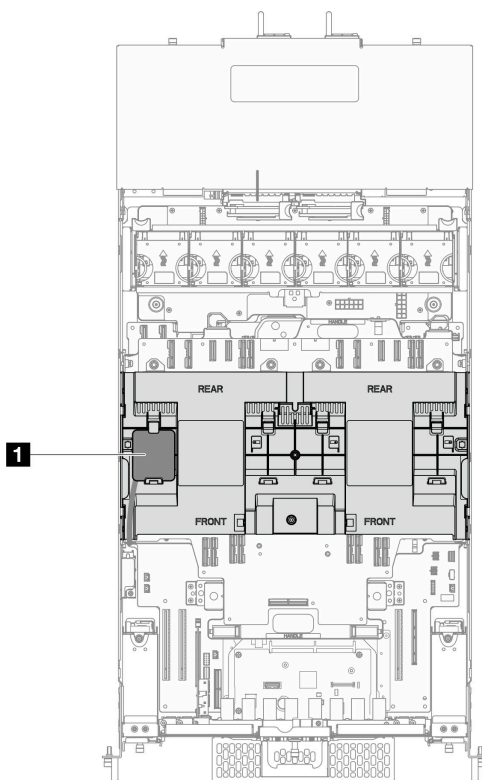
図 47. フラッシュ電源モジュールの位置
