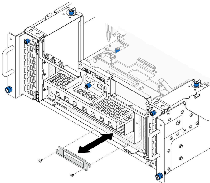
図 55. 前面オペレーター・パネル・ブラケットの取り付け
