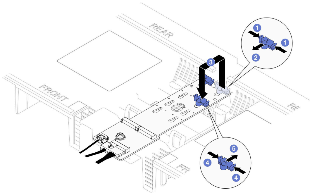
図 83. M.2 保持器具の調整
