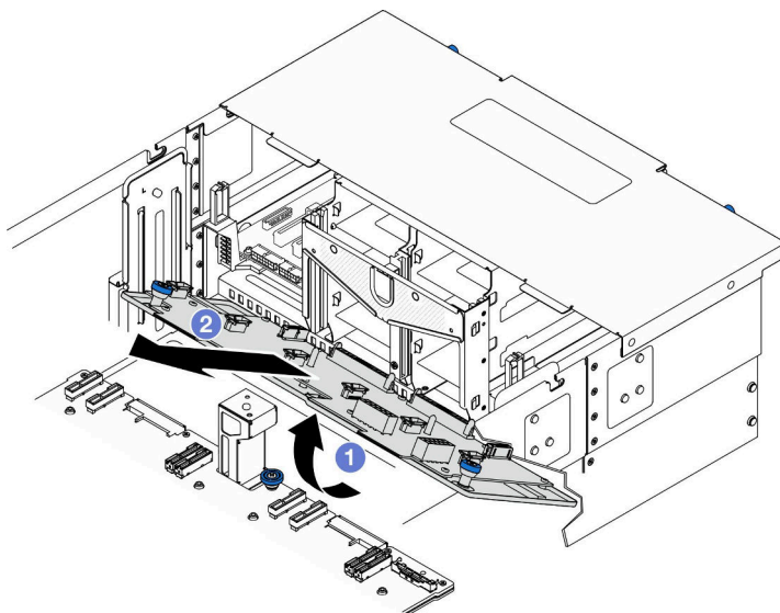
図 117. 分電盤の取り外し
