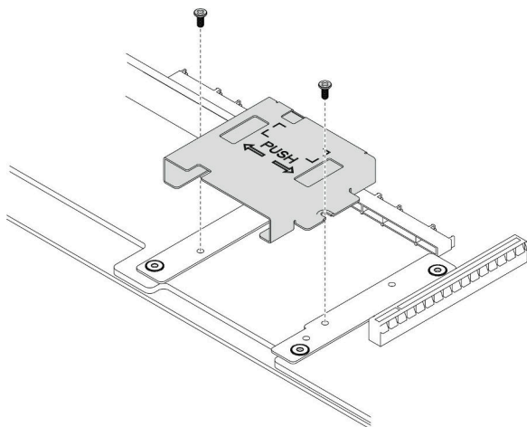
図 56. 前面オペレーター・パネル・ケージの取り付け
