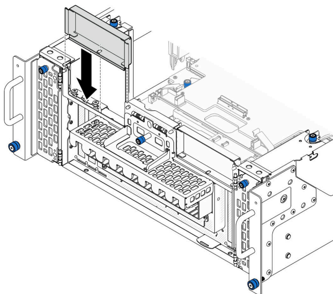
図 102. 左の PCIe フィラーの取り付け
