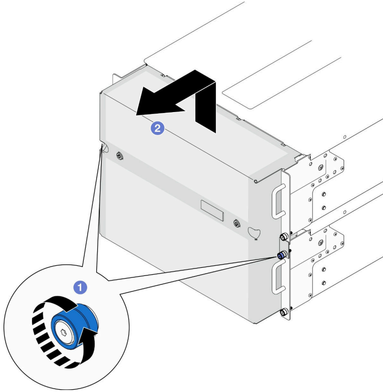
図 139. セキュリティー・ベゼルの取り外し
