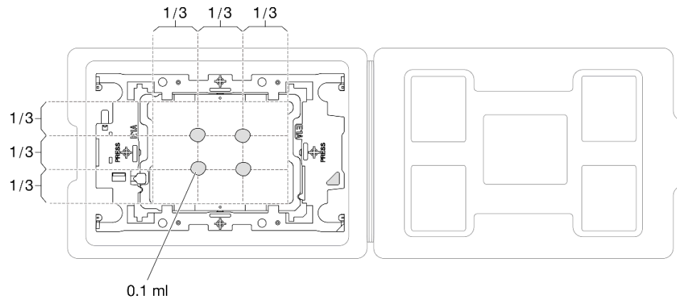
図 135. 配送トレイのプロセッサで熱伝導グリースを塗布する
