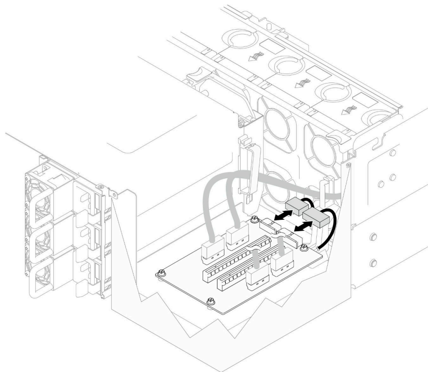
図 114. 電源ケーブルの接続
