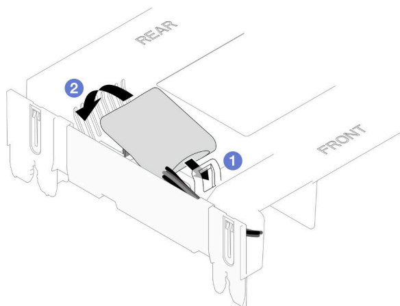
図 50. フラッシュ電源モジュールの取り付け
