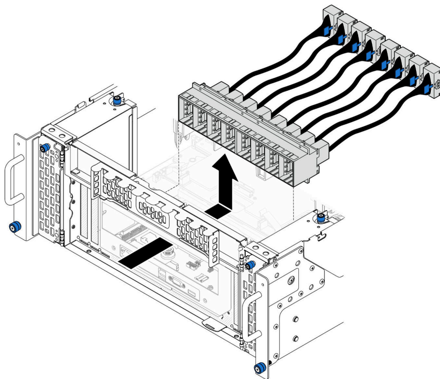
図 173. UPI モジュールの取り外し
