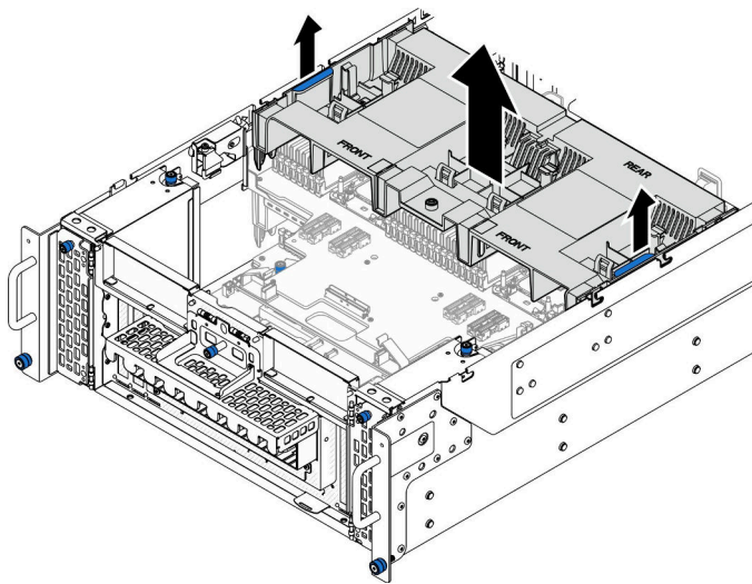
図 10. 上段のプロセッサ・ボード (CPU BD) エアー・バッフルの取り外し
