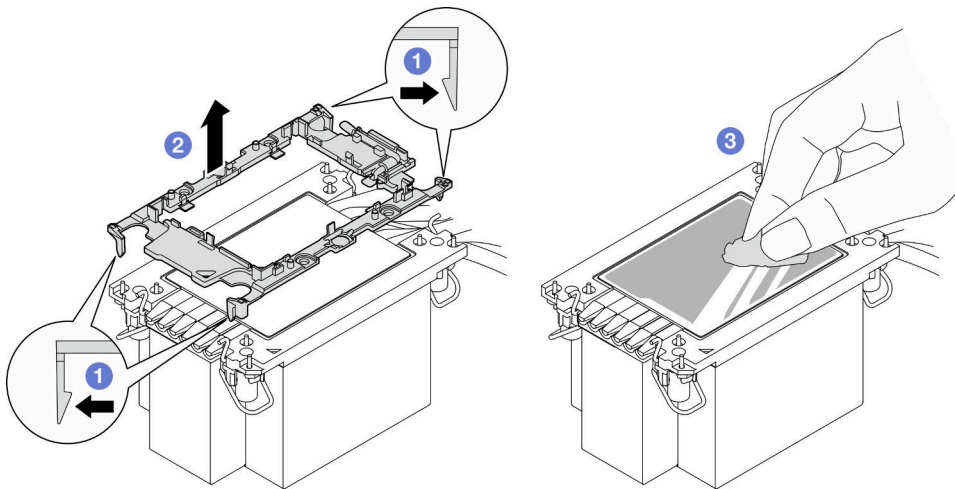
図 132. ヒートシンクからプロセッサ・キャリアを取り外す
