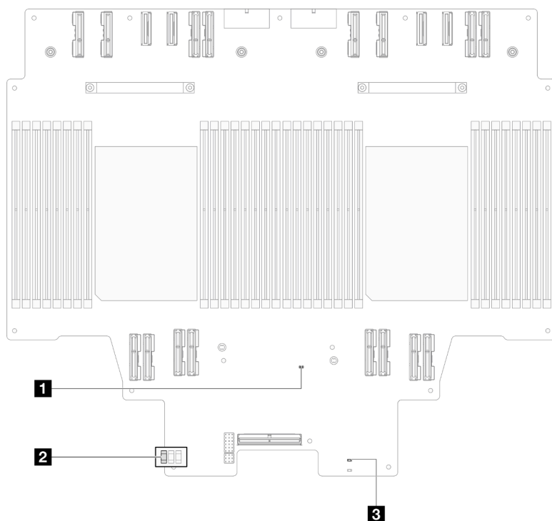
図 208. 上段のプロセッサ・ボード (CPU BD) LED
