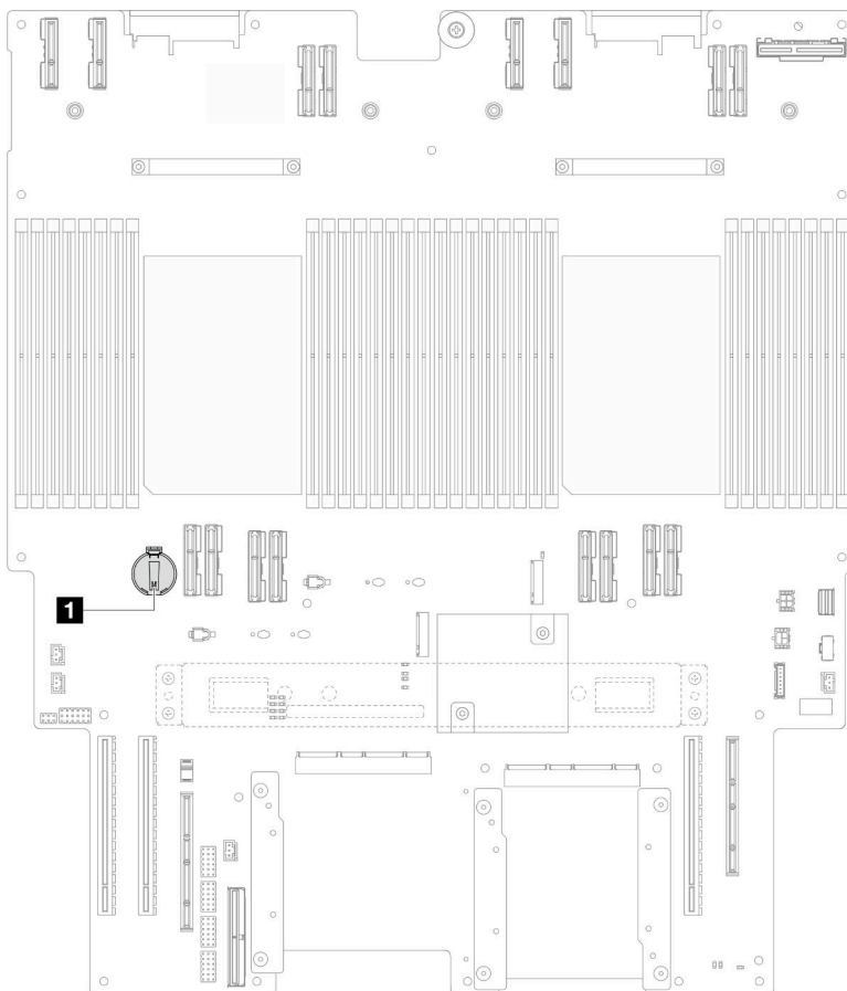
図 15. CMOS バッテリーの位置
