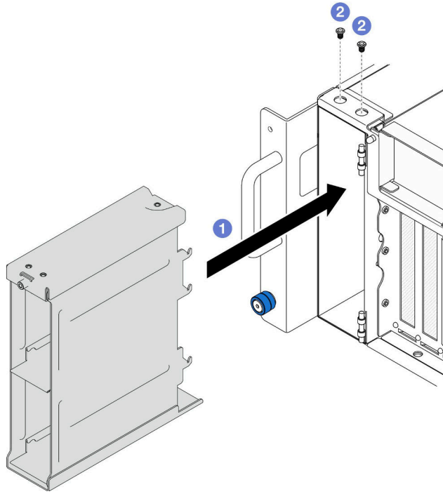
図 33. 2.5 型ドライブ・ケージの取り付け
