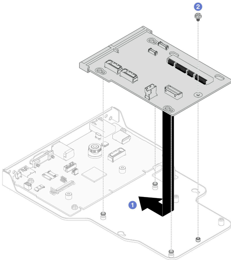
図 161. 変換コネクタ・ボードの取り付け
