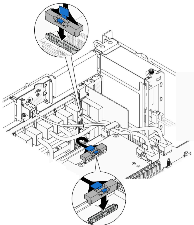
図 187. 内部側波帯ケーブルの接続
