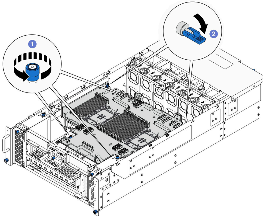
図 181. 上段のプロセッサ・ボード (CPU BD) の取り外し
