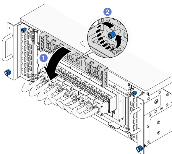
図7. UPI カバーを閉じる
