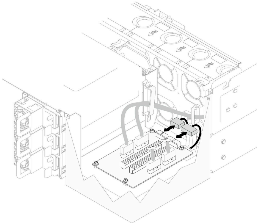
図 108. 電源ケーブルの取り外し
