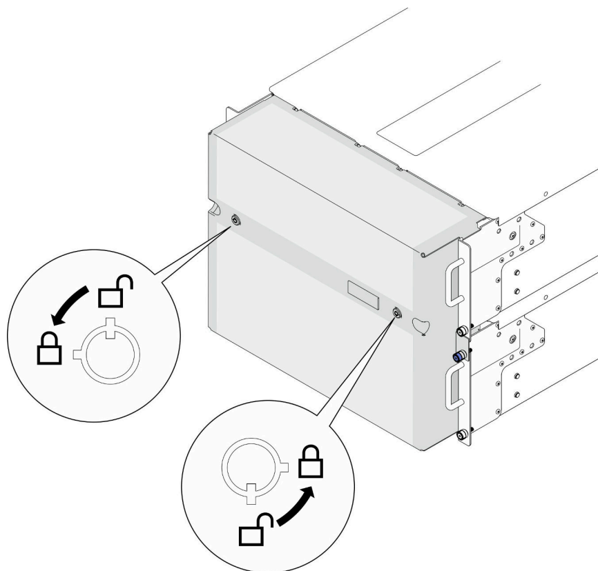
図 142. セキュリティー・ベゼルのロック
