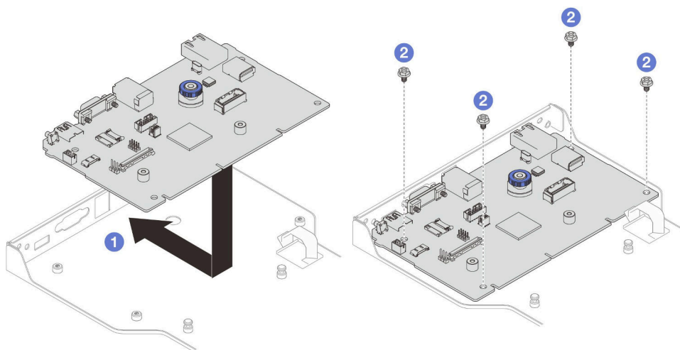
図 160. システム I/O ボードのブラケットへの取り付け
