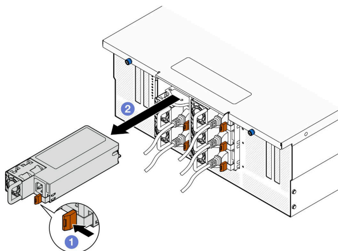
図 126. パワー・サプライの取り外し
