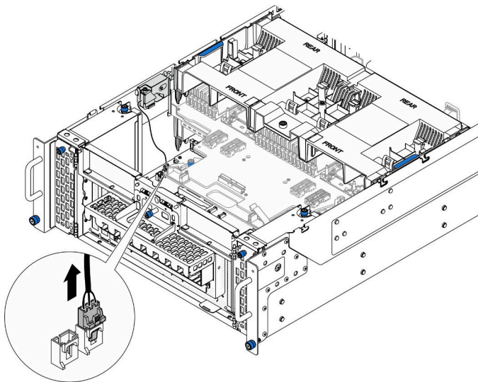
図 58. 侵入検出スイッチの切り離し
