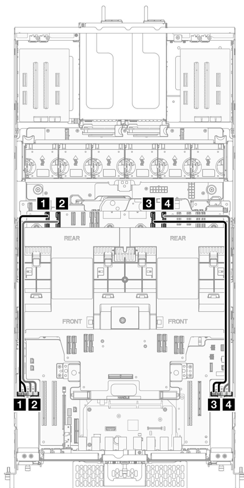
図 197. E3.S ケーブル・アセンブリーのケーブル配線
