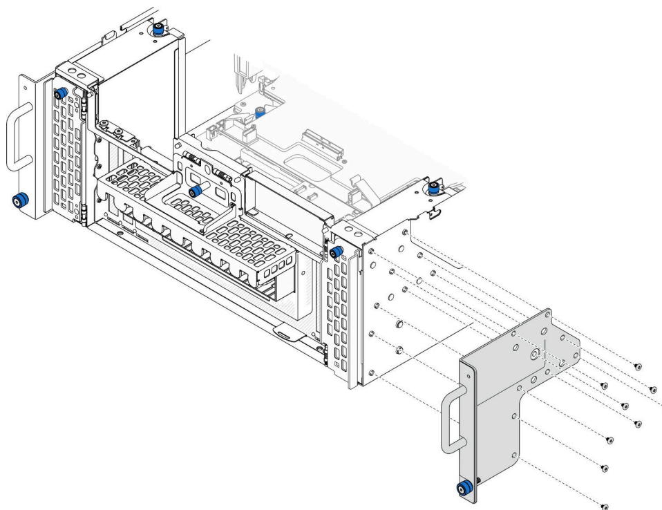
図 37. EIA フランジの取り外し
