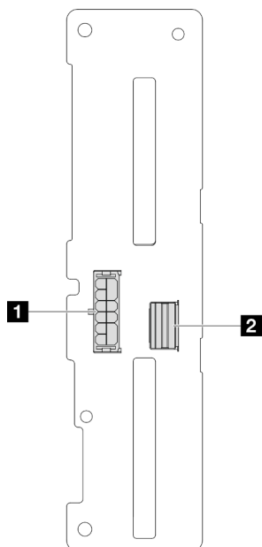
図 189. 2.5 型ドライブ・バックプレーン・コネクタ
