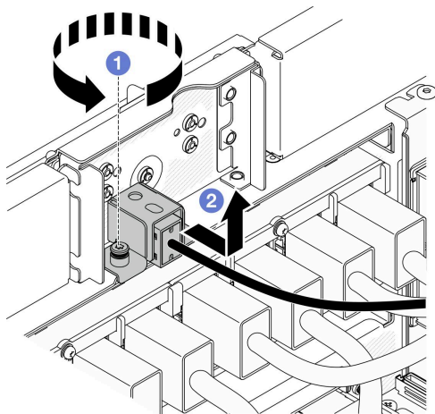
図 63. 前面侵入検出スイッチ・アセンブリーの取り外し
