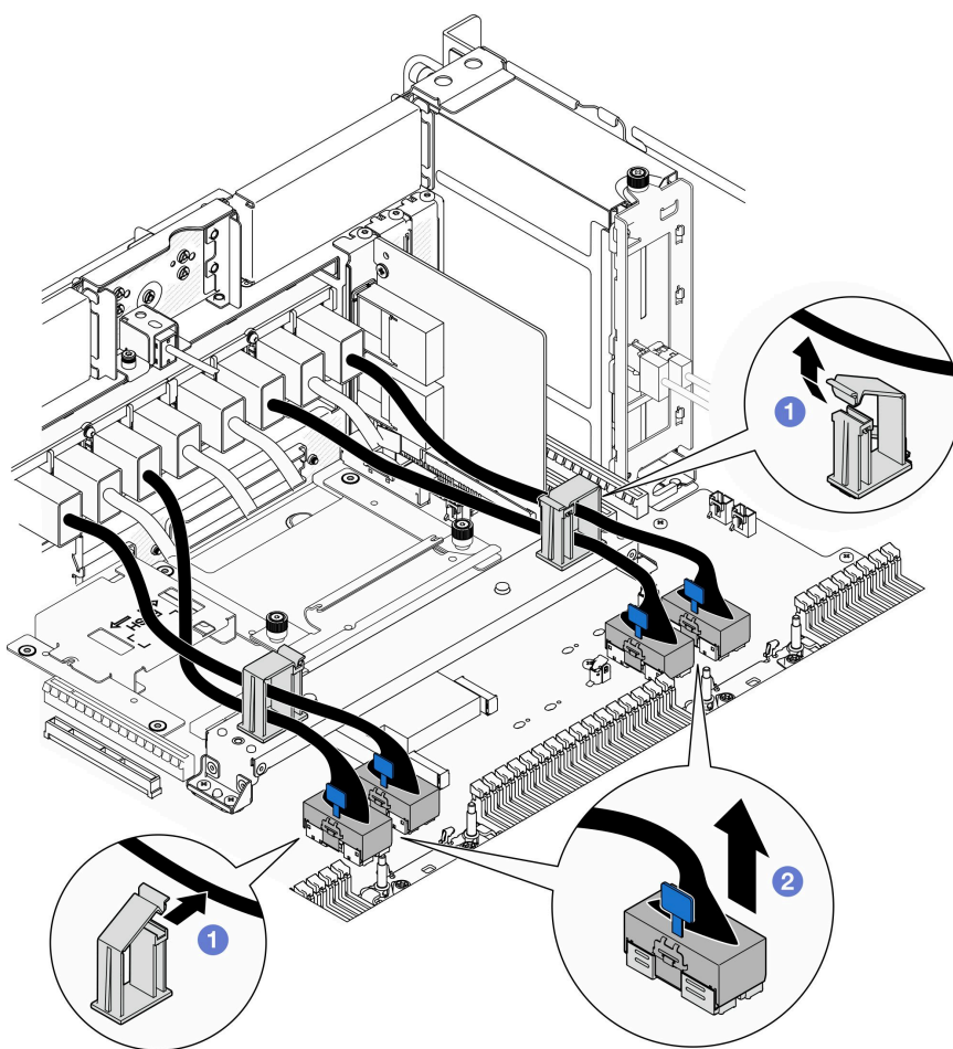
図 171. UPI モジュール・ケーブルの取り外し
