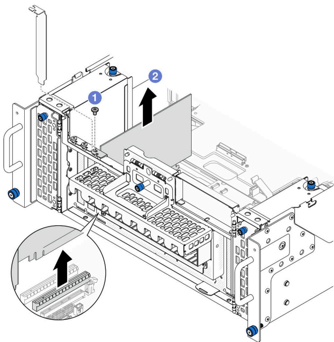
図101. PCIe アダプターの取り外し
