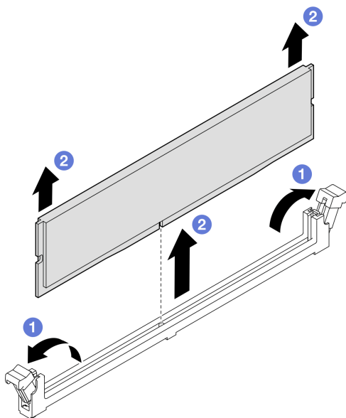
図 90. メモリー・モジュールの取り外し
