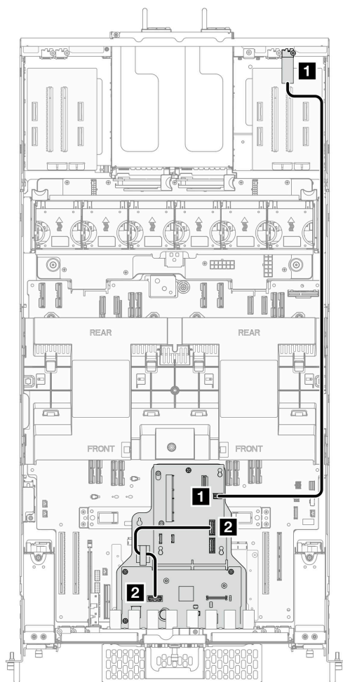
図 198. イーサネット・ポート・アセンブリのケーブル配線
