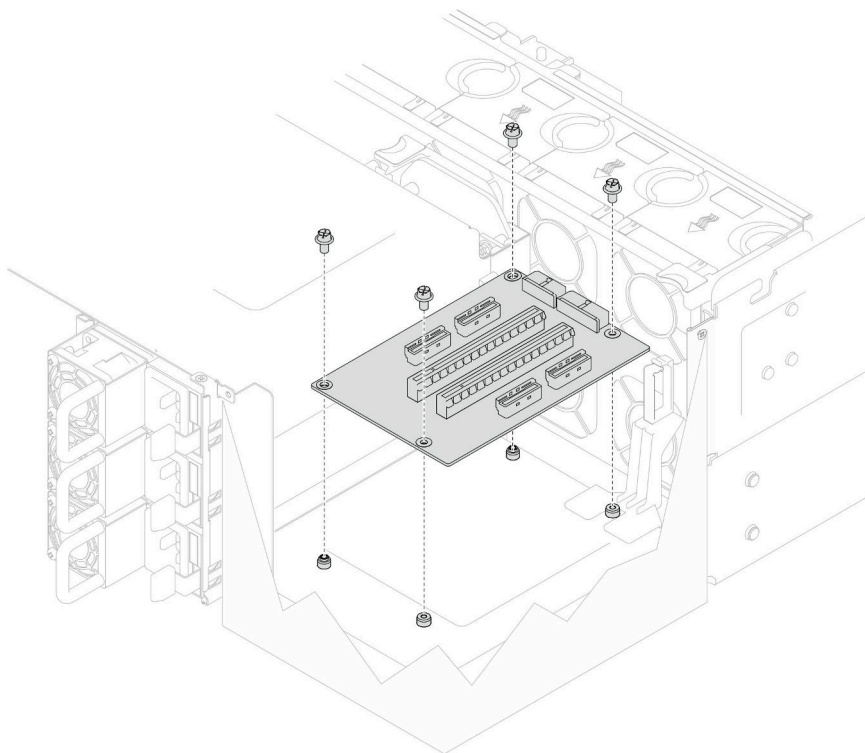
図 110. PCIe ライザー・カードの取り外し
