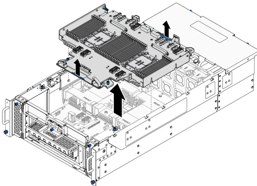
図 182. 上段のプロセッサ・ボード (CPU BD) の取り外し
