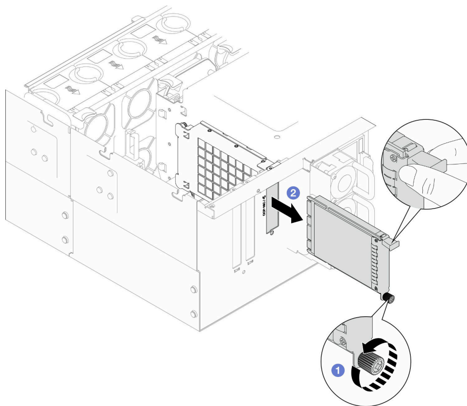
図 94. OCP モジュールの取り外し
