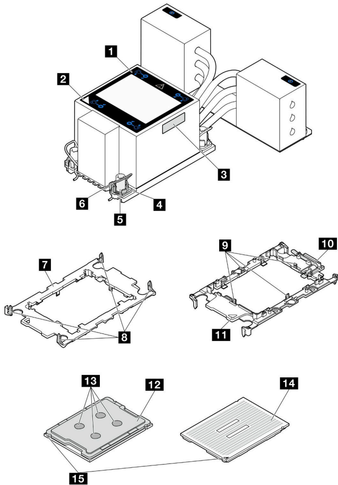
図 129. PHM コンポーネント
