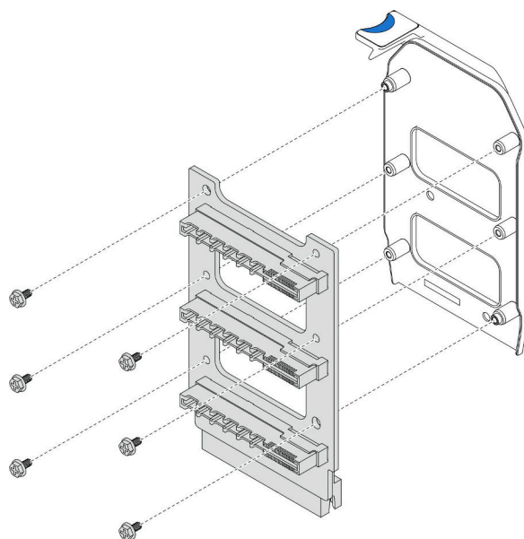
図 123. 電源変換コネクタ・ボードの切り離し
