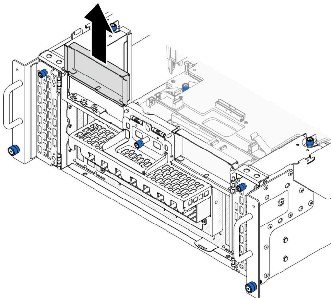
図100. 左の PCIe フィラーの取り外し
