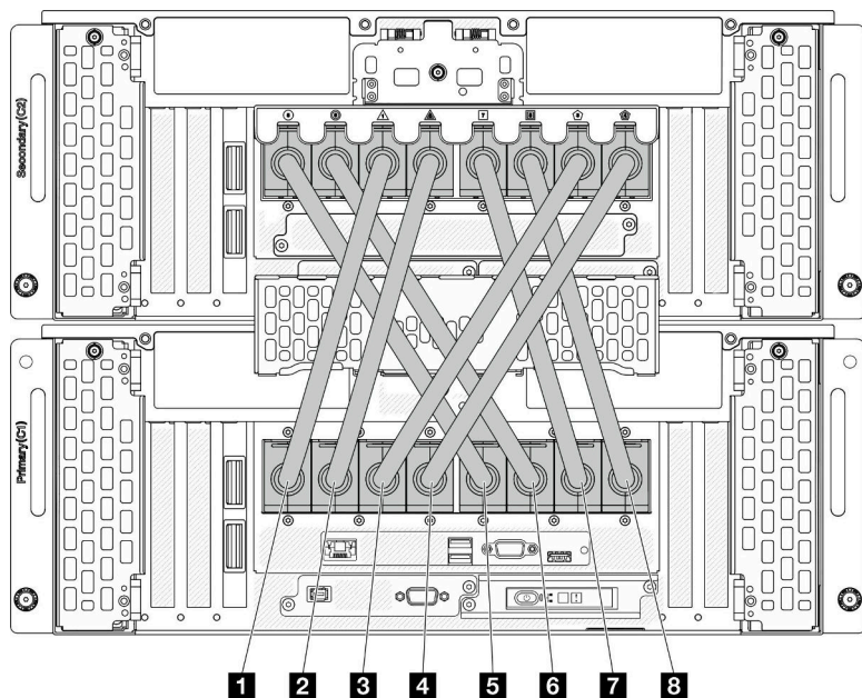
図5. 外部 UPI ケーブルの切り離し
