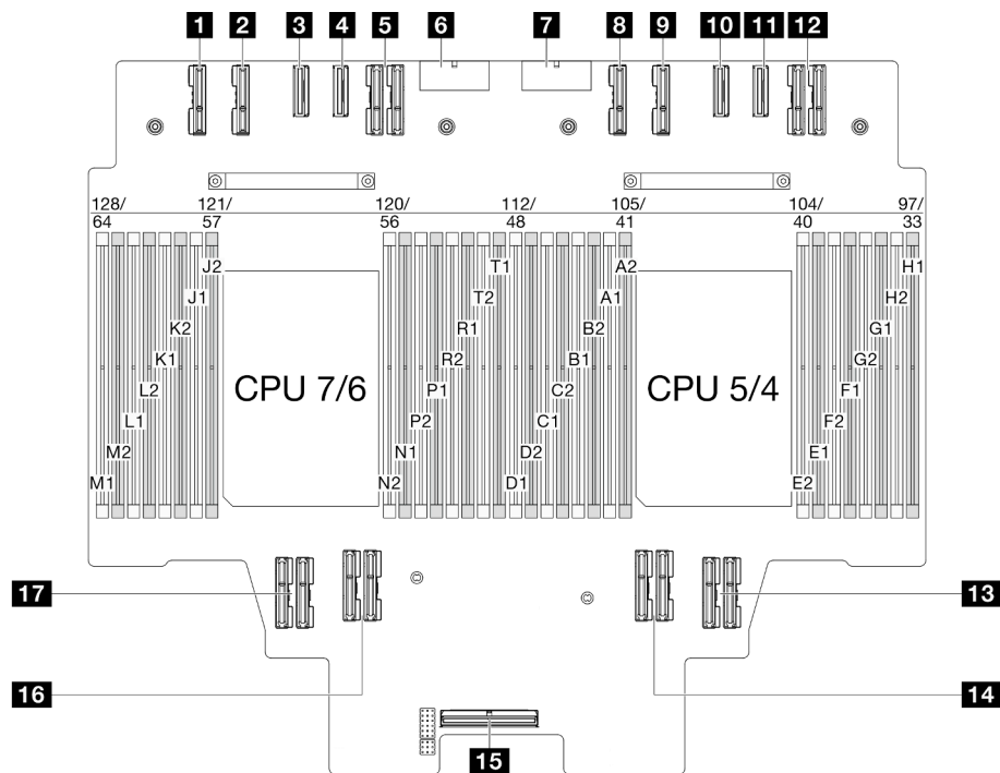
図 190. 上段のプロセッサ・ボード (CPU BD) コネクタ
