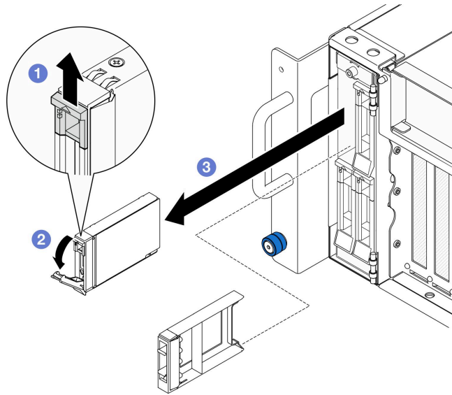
図21. 2.5型ドライブの取り外し
