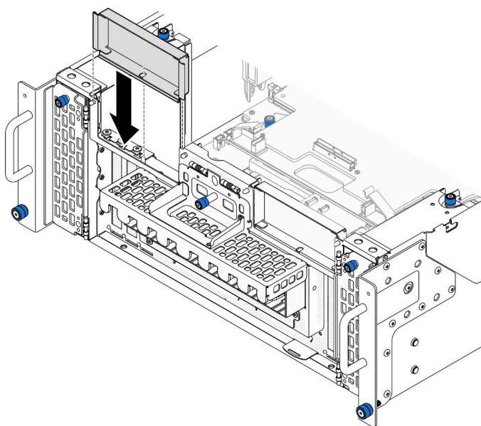
図 147. 左の PCIe フィラーの取り付け
