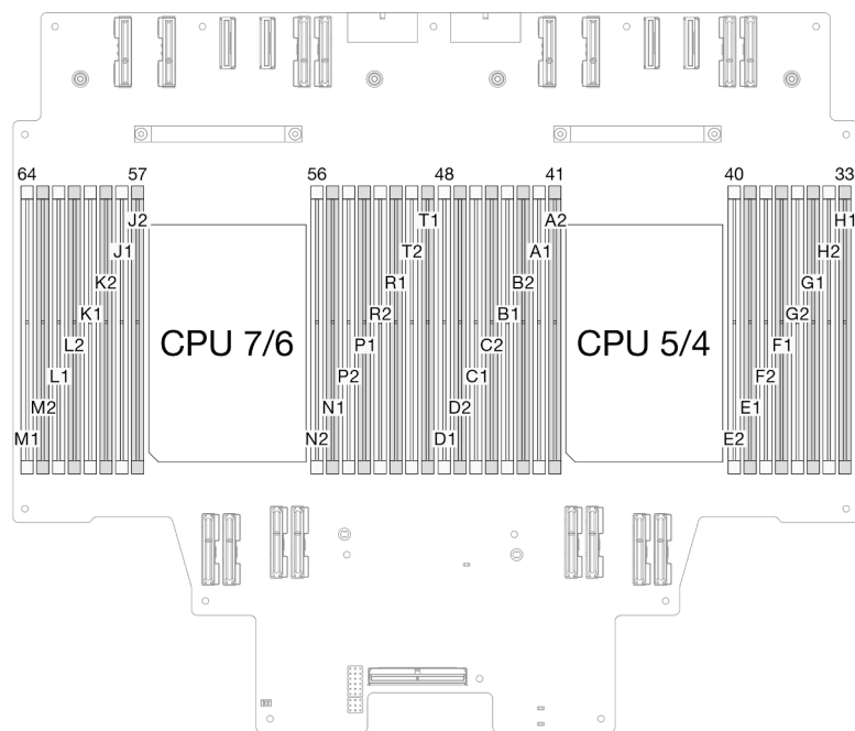
図1. メモリー・モジュールおよびプロセッサのレイアウト (上段のプロセッサ・ボード (CPU BD))
