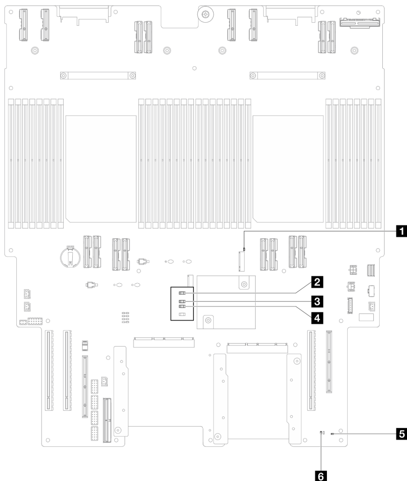
図 210. 下段のプロセッサ・ボード (MB) LED
