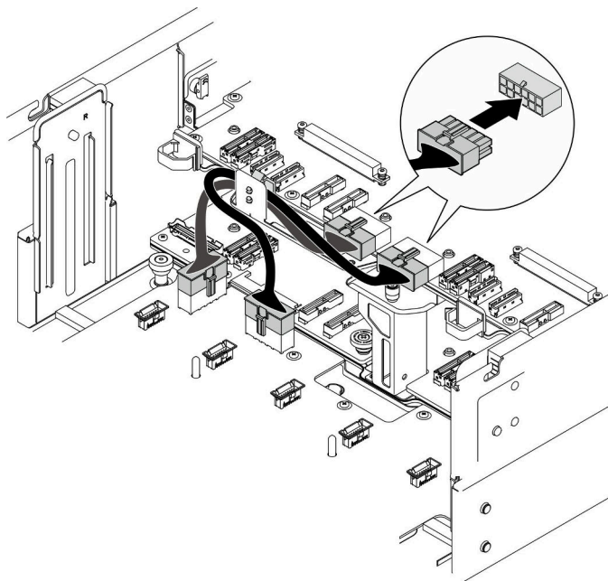
図 185. 上段のプロセッサ・ボード (CPU BD) の電源ケーブルの接続
