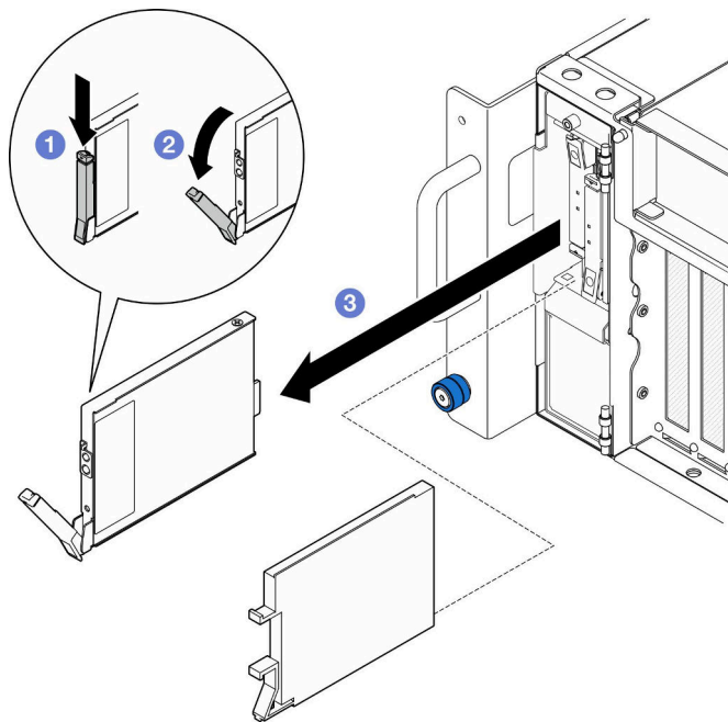
図22. E3.Sドライブの取り外し
