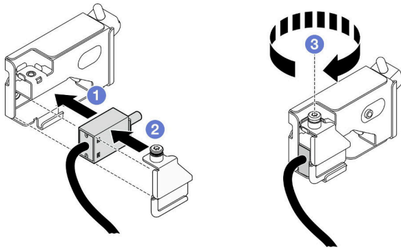
図 60. トップ・カバー侵入検出スイッチの取り付け
