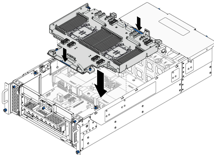
図 183. 上段のプロセッサ・ボード (CPU BD) の取り付け
