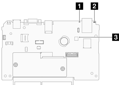
図 209. システム I/O ボード LED
