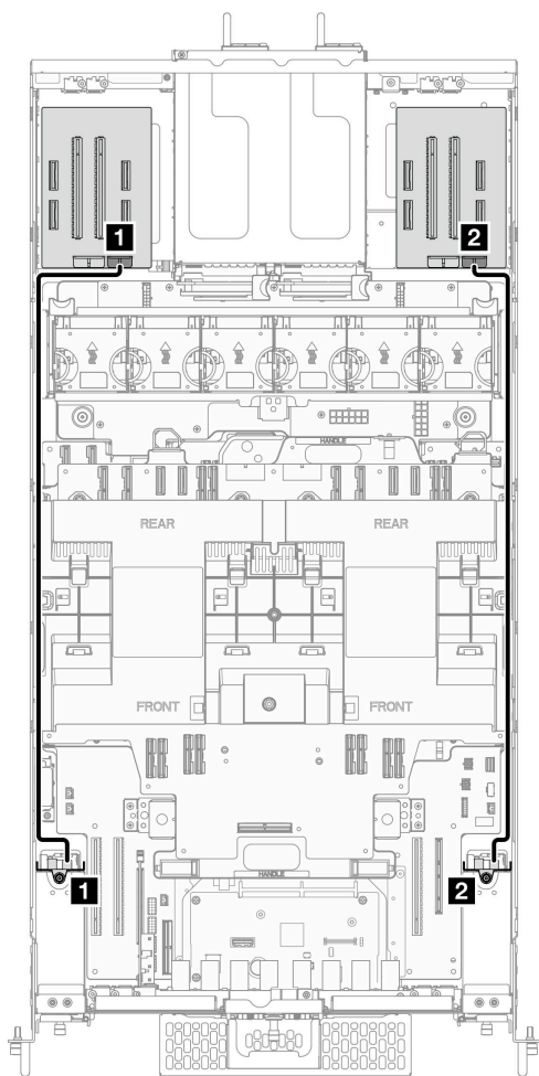
図 194. 2.5 型ドライブ・バックプレーンの電源ケーブルの配線
