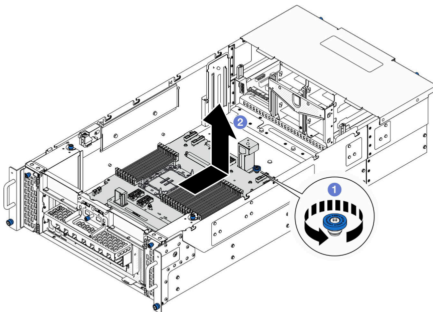
図 71. 下段のプロセッサ・ボード (MB) の取り外し
