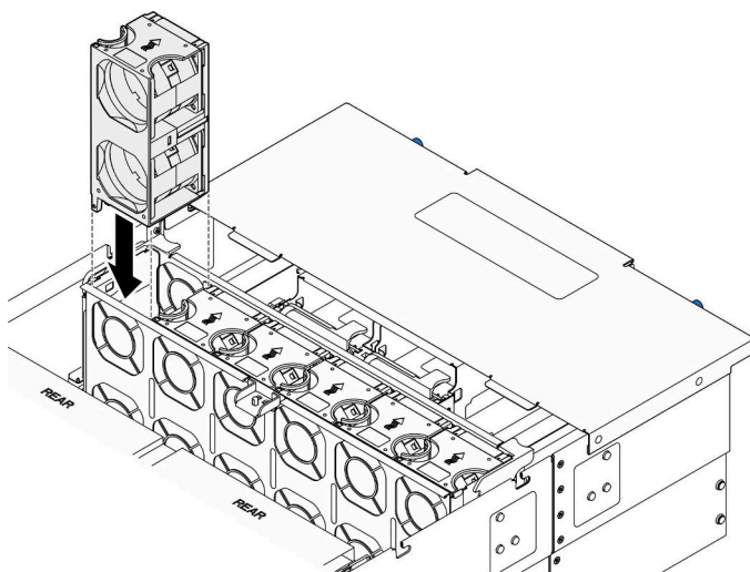
図 46. ファン・モジュールの取り付け
