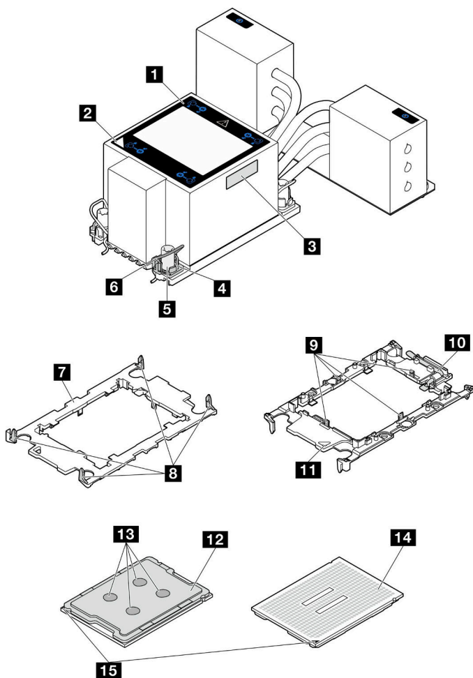
図 133. PHM コンポーネント
