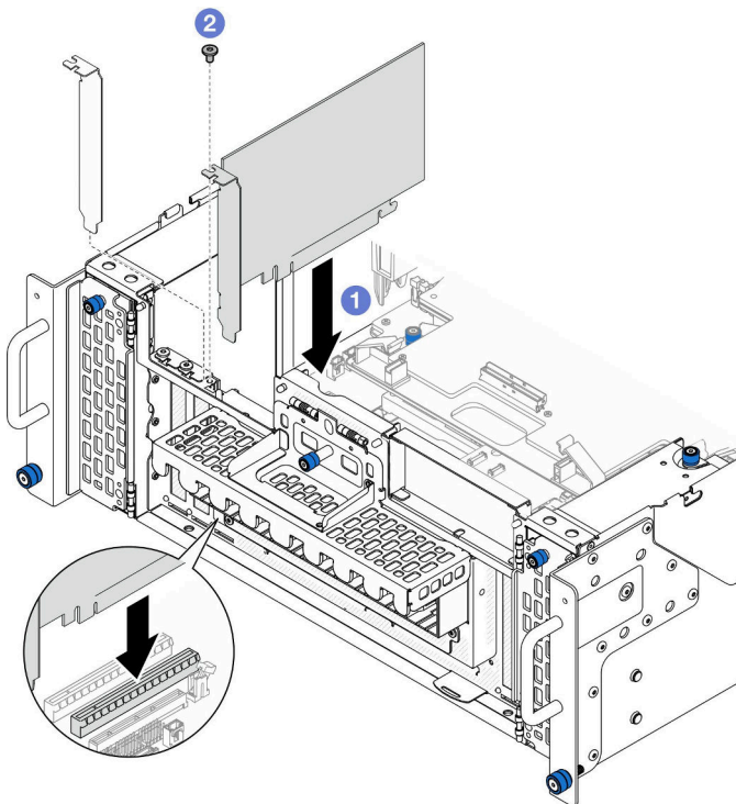
図 105. PCIe アダプターの取り付け
