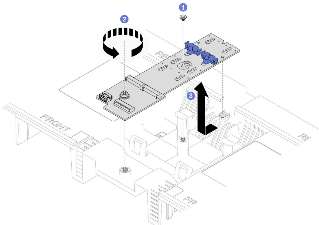
図 80. M.2 ブート・アダプターの取り外し
