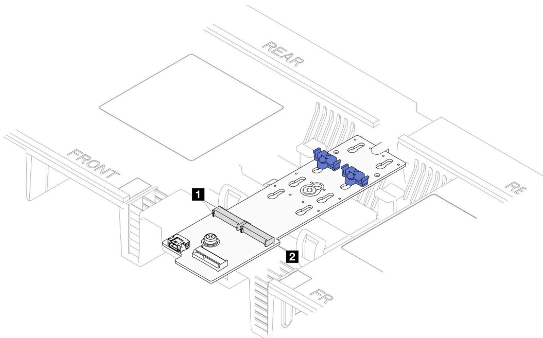
図 86. M.2 ドライブ・スロット
