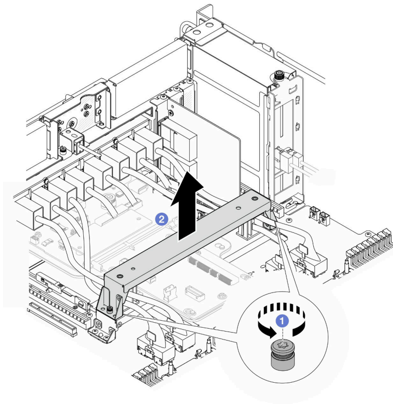
図 151. サポート・ブラケットの取り外し
