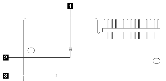
図 211. Firmware and RoT Security Module 上の LED
