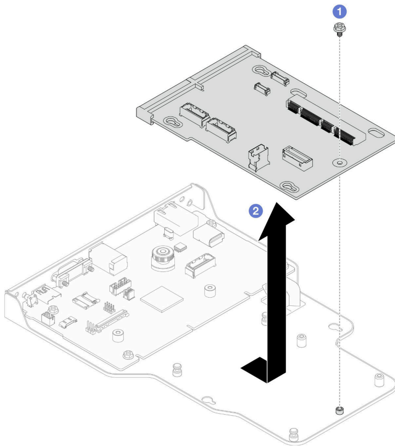
図 158. 変換コネクタ・ボードの取り外し
