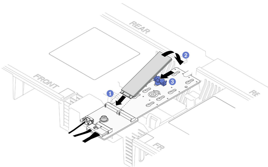
図 87. M.2 ドライブの取り付け
