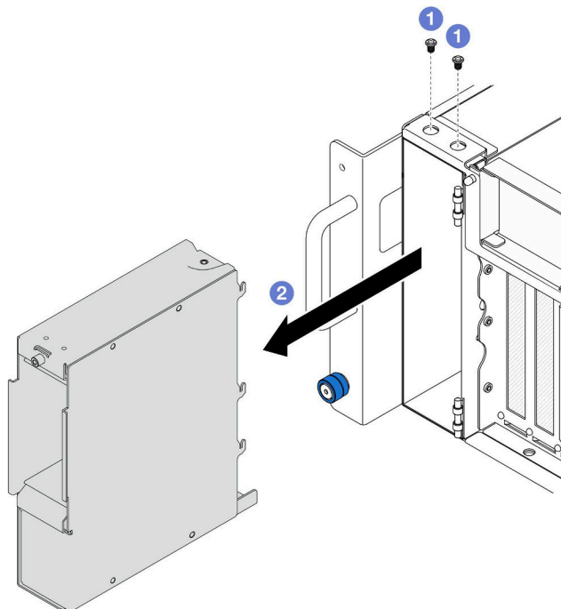
図32. E3.S ドライブ・ケージの取り外し
