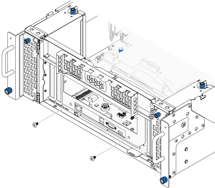
図 156. システム I/O ボードと変換コネクタ・アセンブリを緩める
