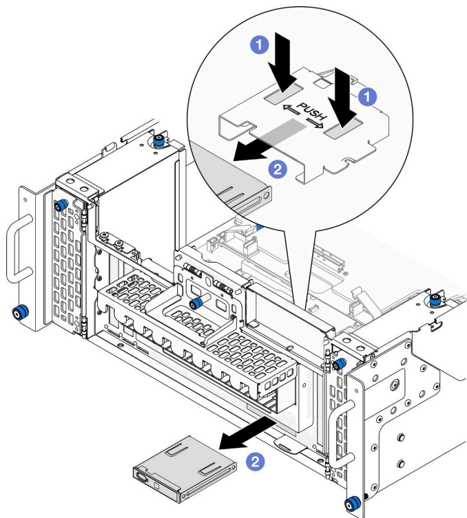
図 52. 前面オペレーター・パネルの取り外し
