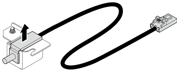
図 64. 侵入検出スイッチの取り外し
