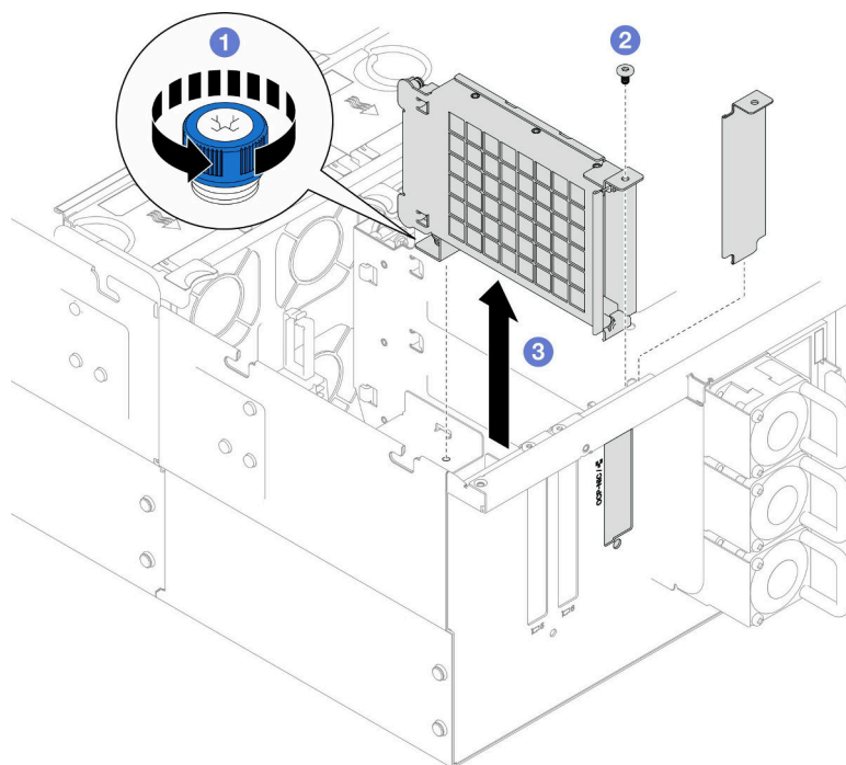
図95. OCP モジュール・ケージの取り外し
