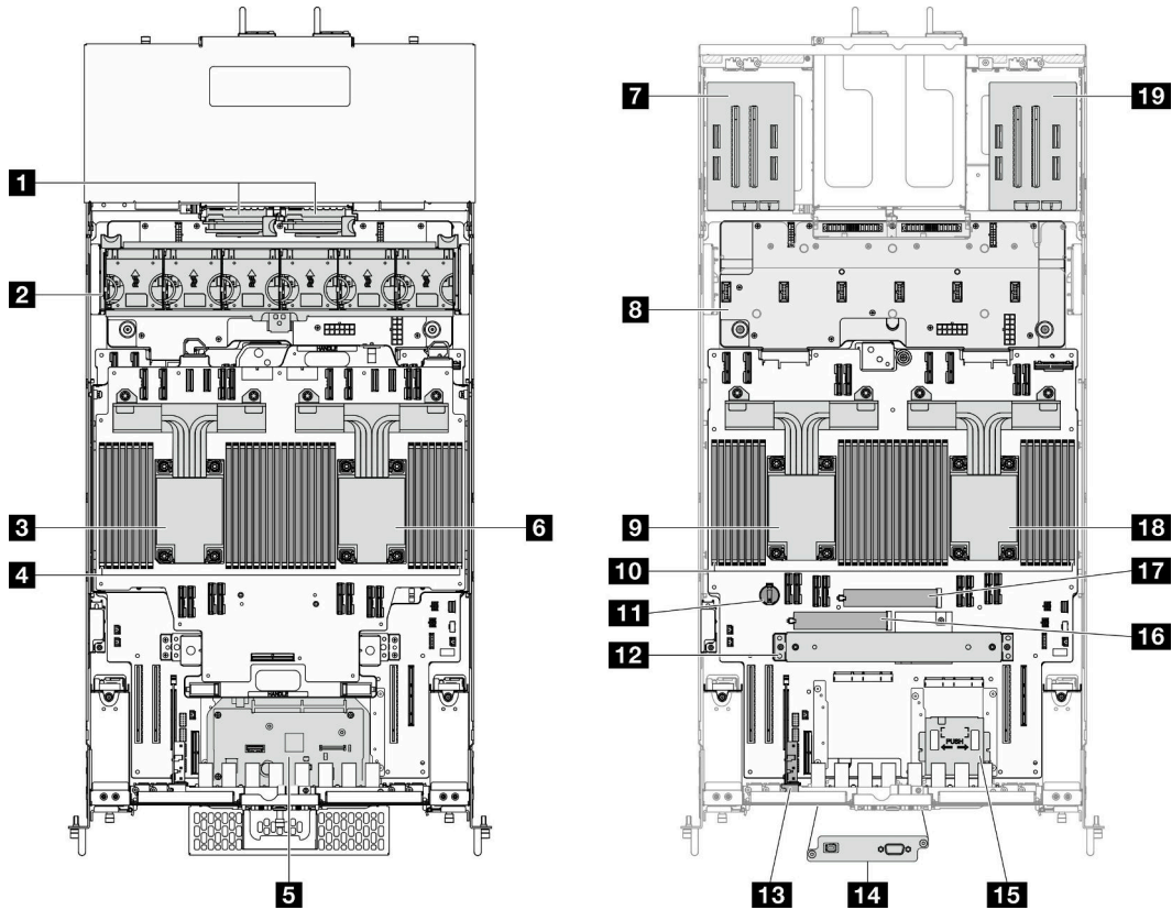
그림 8. 서버 평면도
