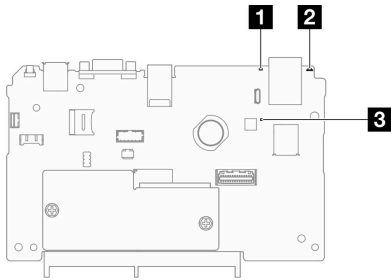
그림 20. 시스템 I/O 보드 LED
