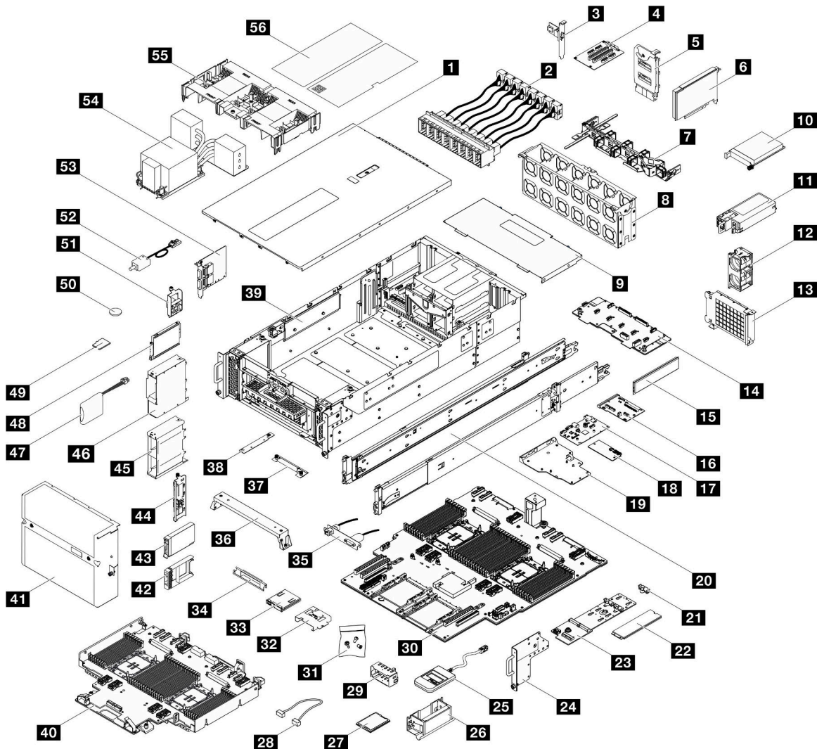
그림 24. 서버 구성 요소
