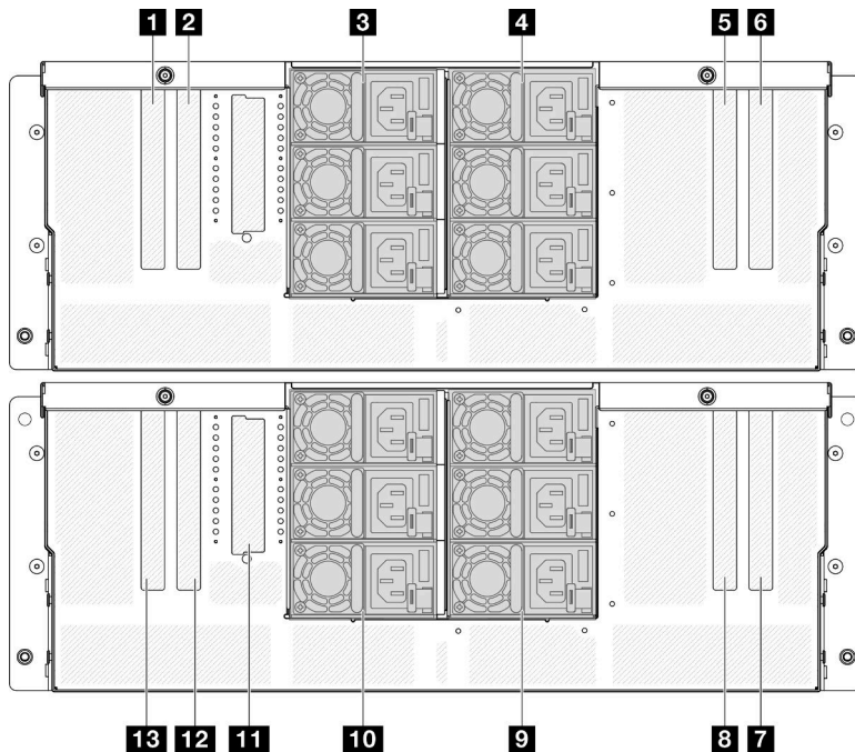
그림 5. 뒷면 보기
