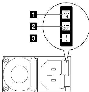
그림 18. 전원 공급 장치 LED
