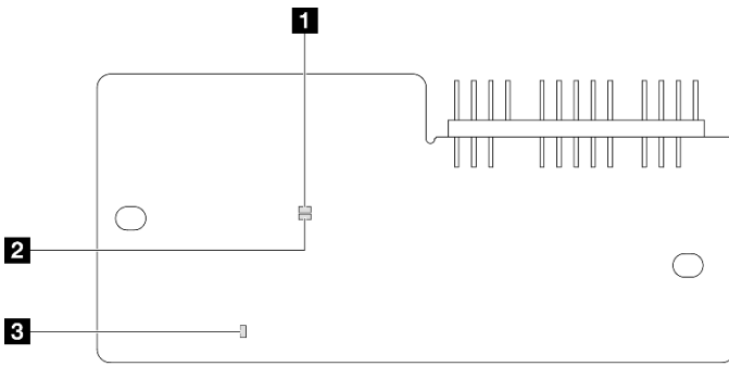
그림 22. Firmware and RoT Security Module의 LED
