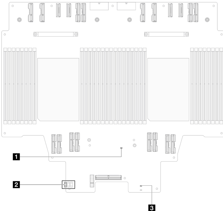
그림 19. 상단 프로세서 보드(CPU BD) LED
