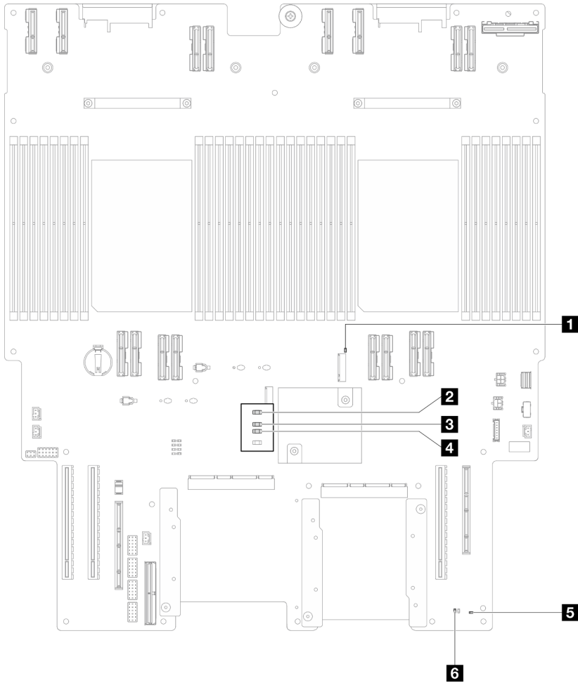
그림 21. 하단 프로세서 보드(MB) LED
