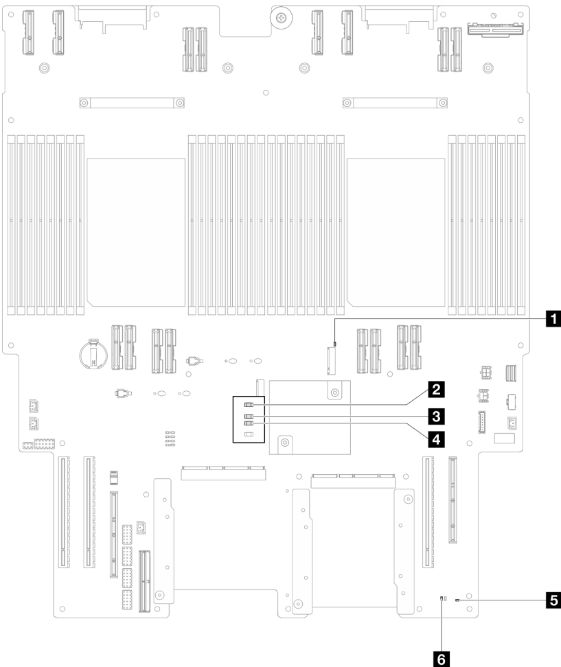
圖例 21. 下方處理器板 (MB) LED
