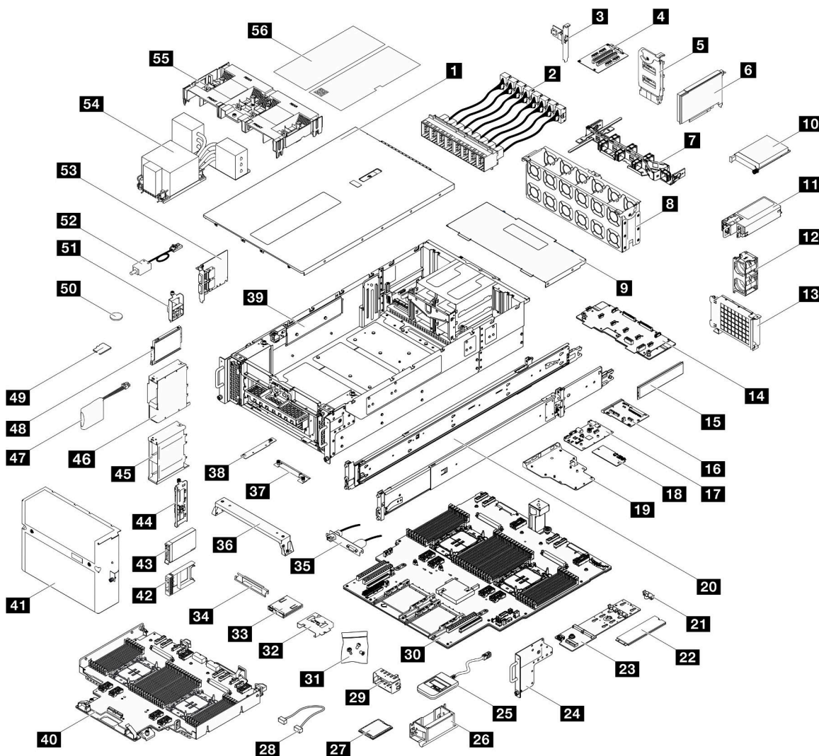
圖例 24. 伺服器元件
