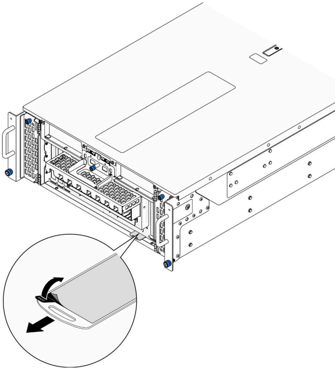
圖例 26. 拉出式資訊標籤上的 Lenovo XClarity Controller 網路存取標籤
