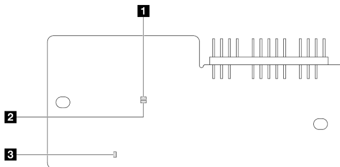
圖例 22. Firmware and RoT Security Module 上的 LED
