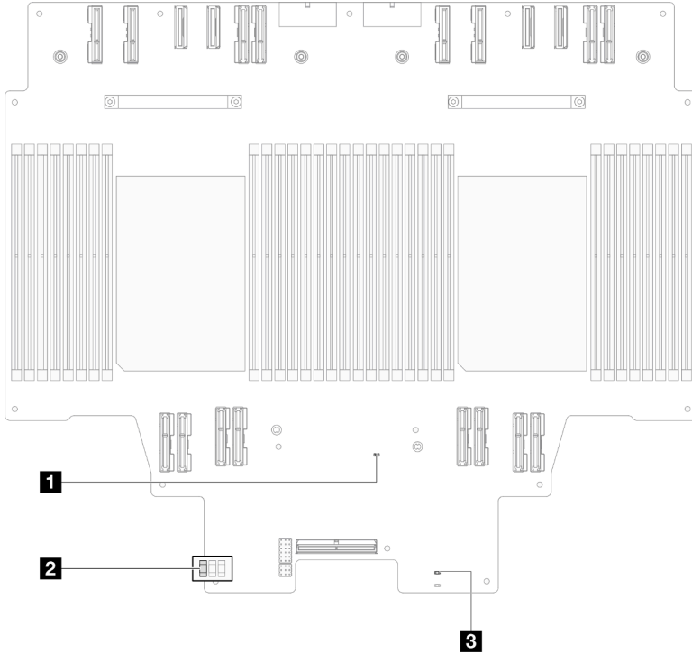
圖例 19. 上方處理器板 (CPU BD) LED
