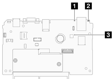
圖例 20. 系統 I/O 板 LED
