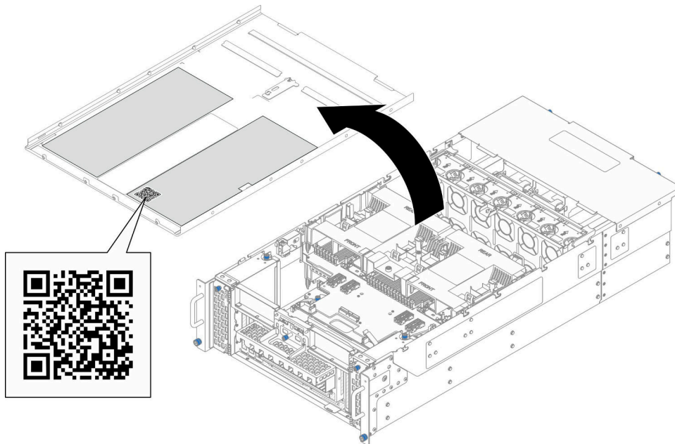
圖例 27. 服務標籤和 QR 代碼
