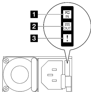
圖例 18. 電源供應器 LED
