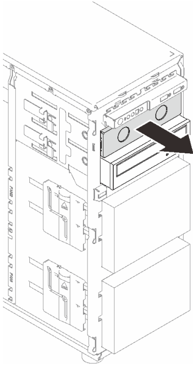
图 49. 从光盘驱动器插槽上卸下 EMI 防护罩
