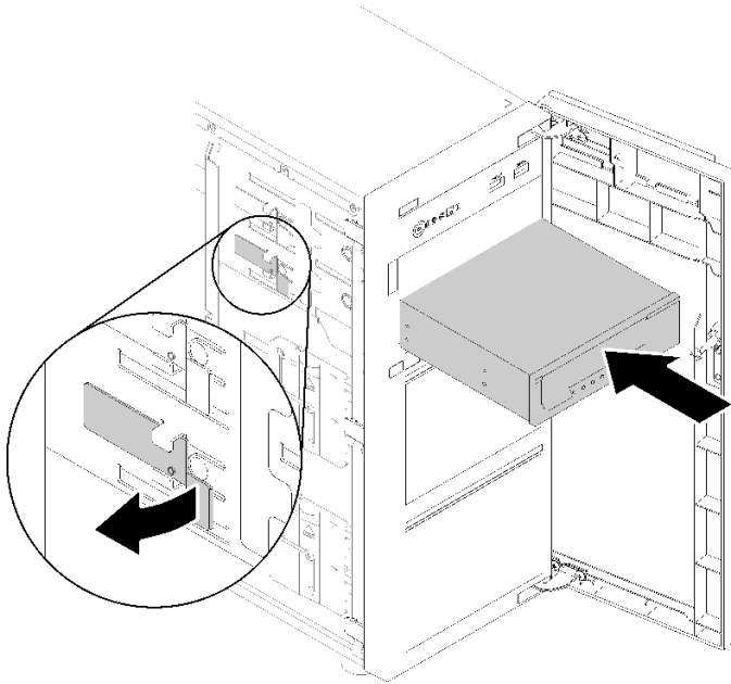
图 51. 安装磁带机
