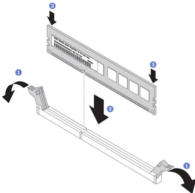
图 37. 安装内存条
