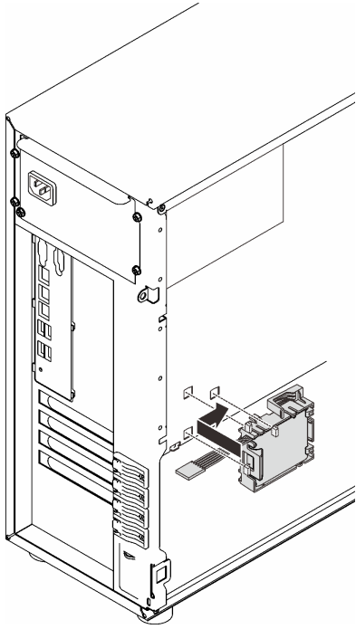
图 41. 将 RAID 快速充电模块和支架组合件安装到机箱上
