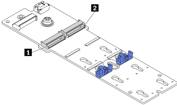
图 38. M.2 硬盘插槽
