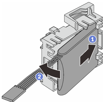
图 40. 将 RAID 快速充电模块安装到支架中
