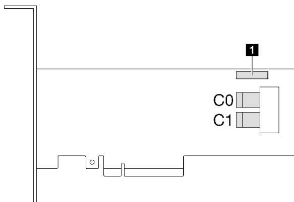
图 13. 9350-8i 接口
