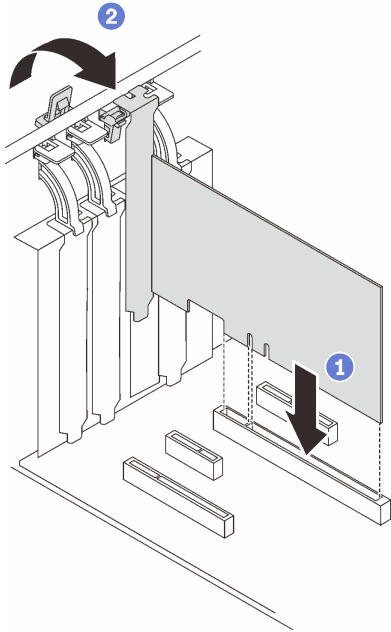
图 42. 安装 PCIe 适配器
