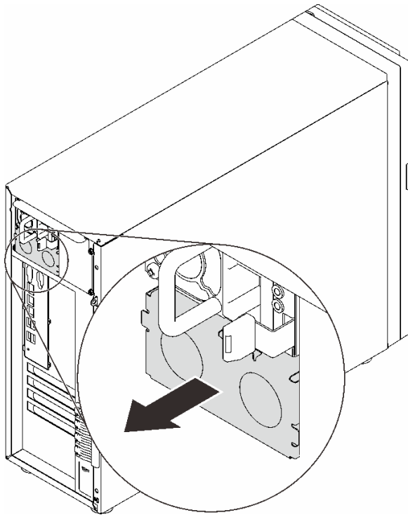
图 29. 卸下热插拔电源模块填充件
