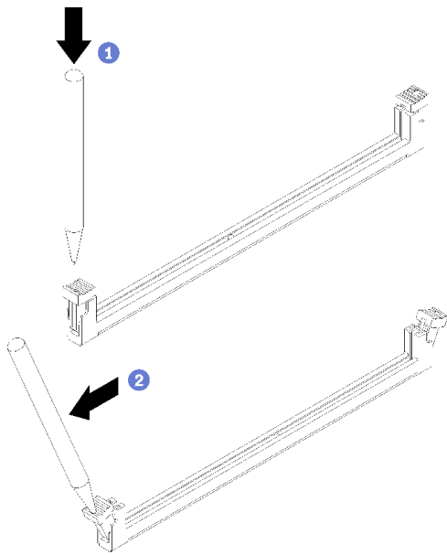
图 36. 打开固定夹
