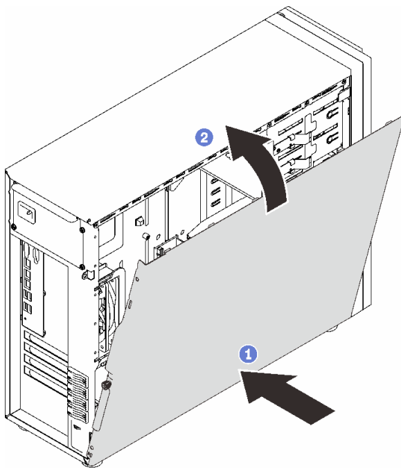
图 52. 将服务器外盖放在机箱上
