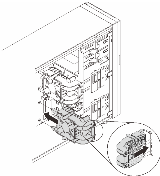
图 34. 安装正面系统风扇
