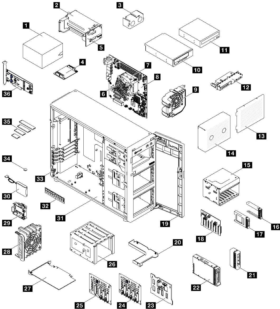
图 23. 服务器组件
