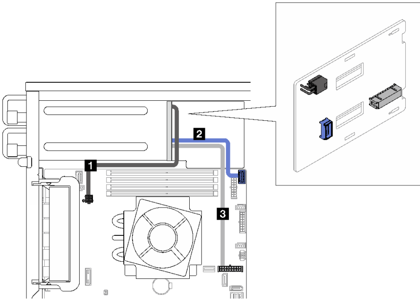
图 22. 冗余电源模块的线缆布放
