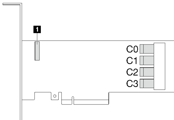
图 14. 9350-16i 接口
