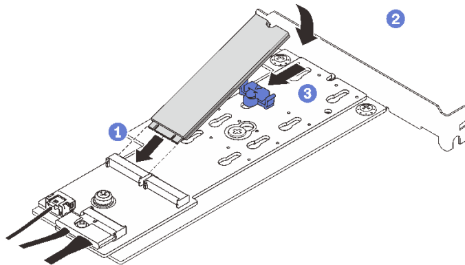
图 39. 安装 M.2 硬盘
