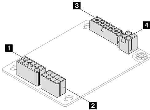
图 11. 固定电源模块的配电板
