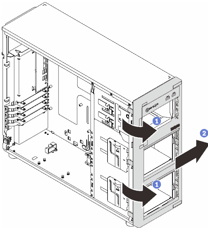
图 27. 卸下前挡板
