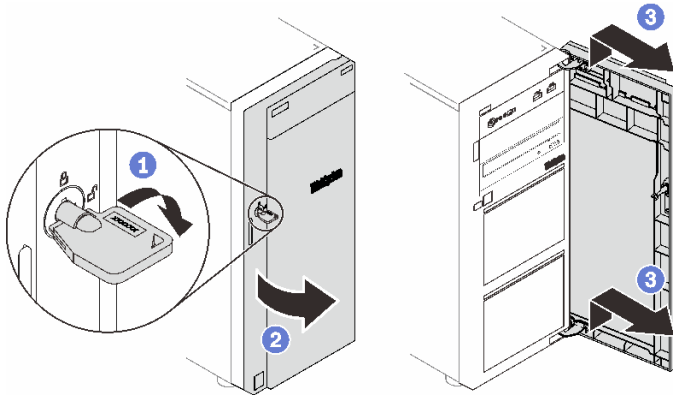
图 26. 卸下前门
