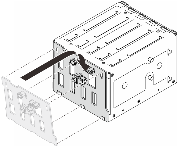
图 32. 安装热插拔硬盘背板
