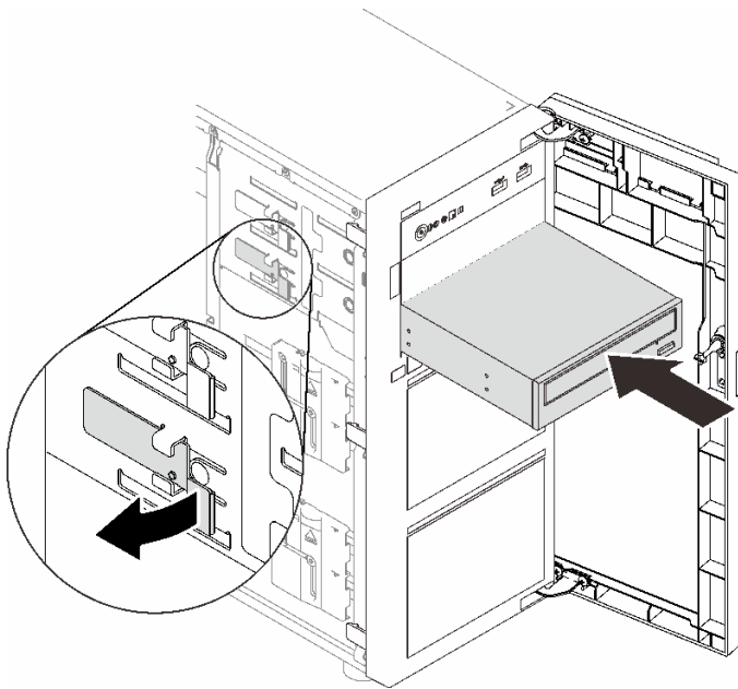
图 50. 安装光盘驱动器
