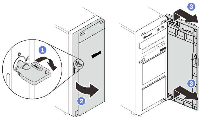
图 18. 前门锁
