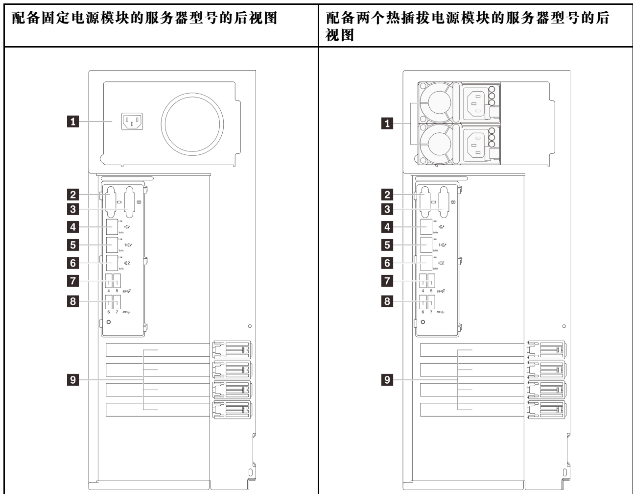
图 6. 后视图
