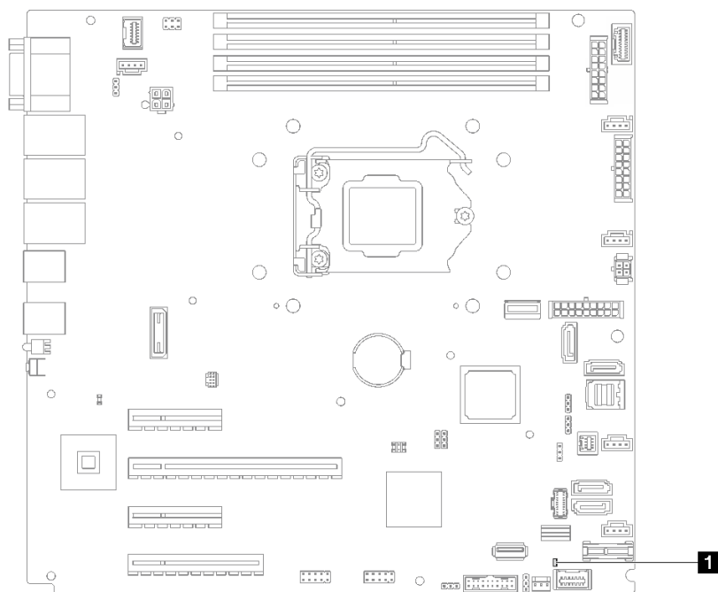
图 9. 主板 LED
