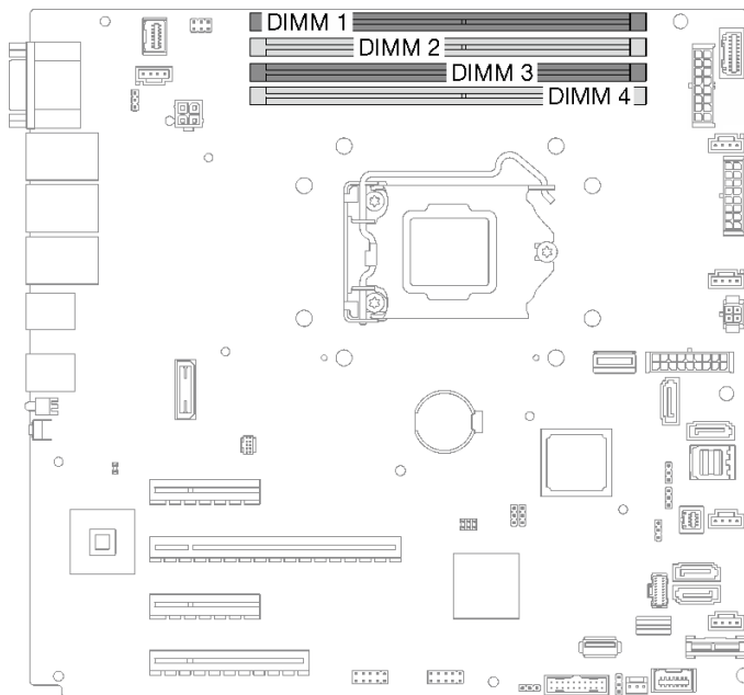
图 24. 主板上的内存条插槽
