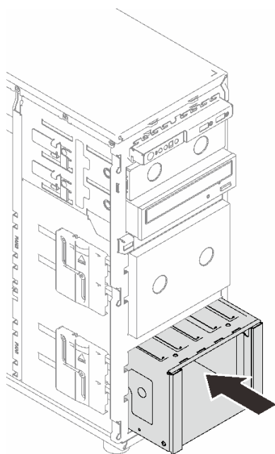
图 31. 安装硬盘仓
