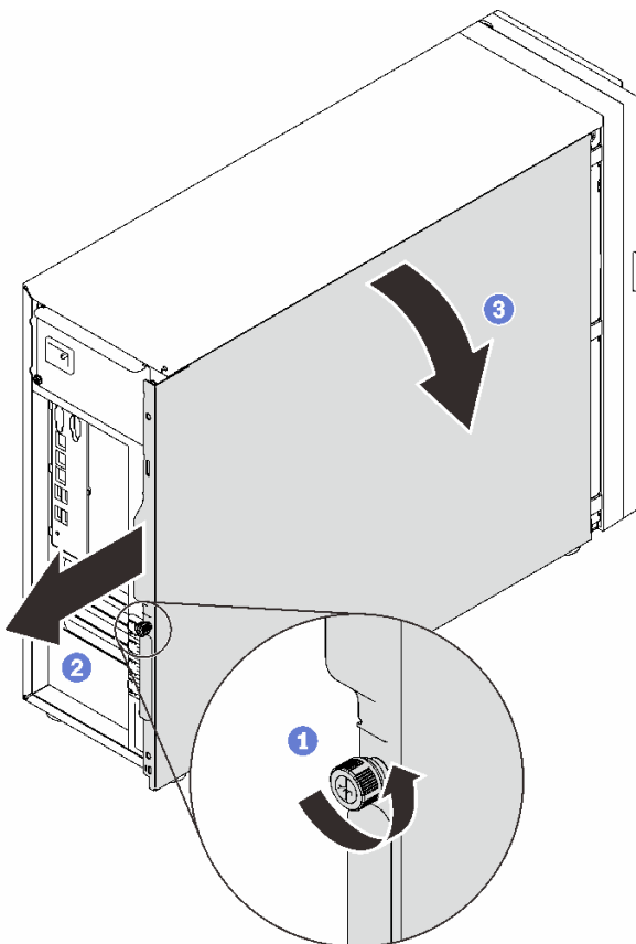
图 25. 卸下服务器外盖
