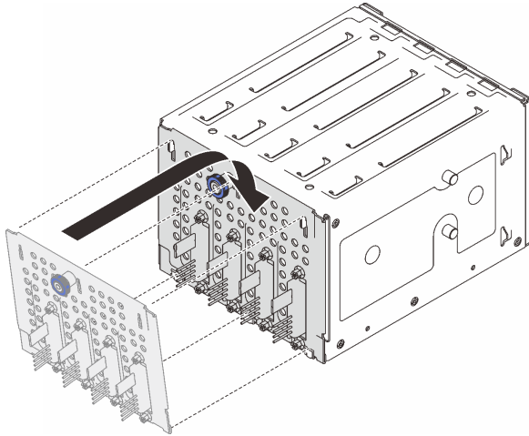
图 33. 安装易插拔硬盘底板
