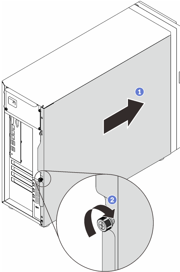
图 53. 将服务器外盖固定到机箱上
