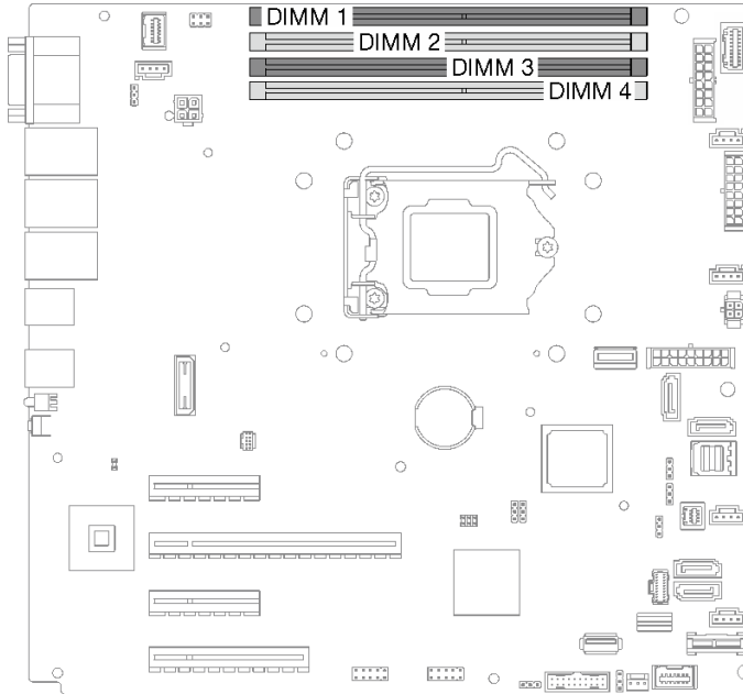
图 35. 主板上的内存条插槽
