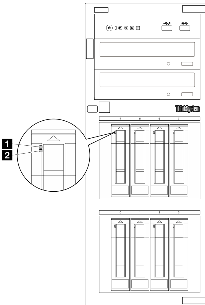
Abbildung 14. Laufwerkanzeigen
