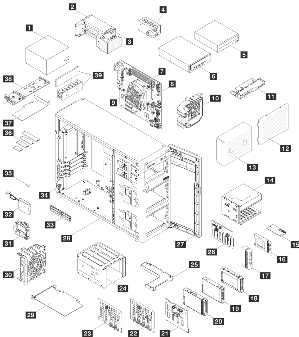
Abbildung 20. Serverkomponenten
