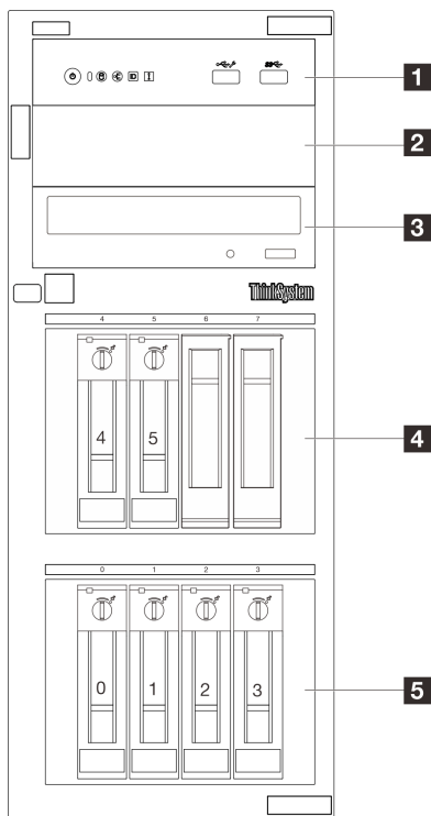
Abbildung 3. Vorderansicht von Servermodellen mit sechs 3,5-Zoll-Simple-Swap-Laufwerkpositionen
