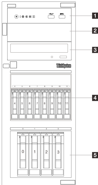
Figure 6. Vue avant des modèles de serveur avec quatre baies d'unités remplaçables à chaud 3,5 pouces + huit baies d'unités remplaçables à chaud 2,5 pouces
