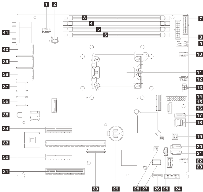
Figure 12. Connecteurs de la carte mère
