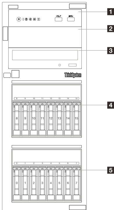
Figure 5. Vue avant des modèles de serveur équipés de seize baies d'unités remplaçables à chaud 2,5 pouces
