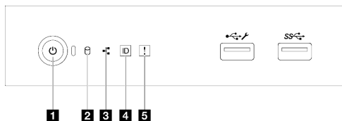
Figure 15. Voyants du module d'E-S avant
