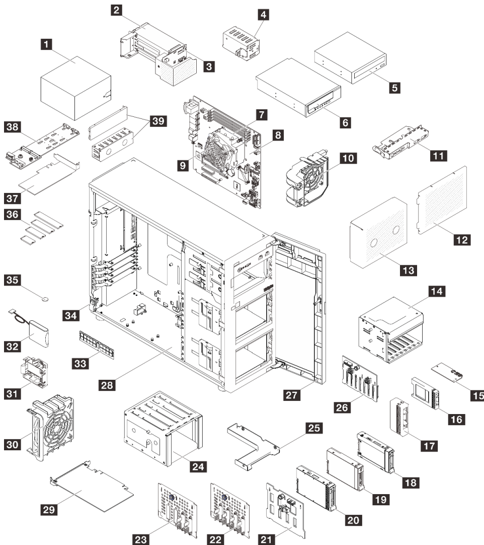
Figure 20. Composants serveur
