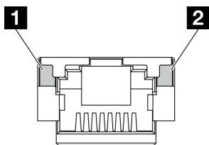
Figure 19. Voyants du port de gestion du système XCC et du port Ethernet
