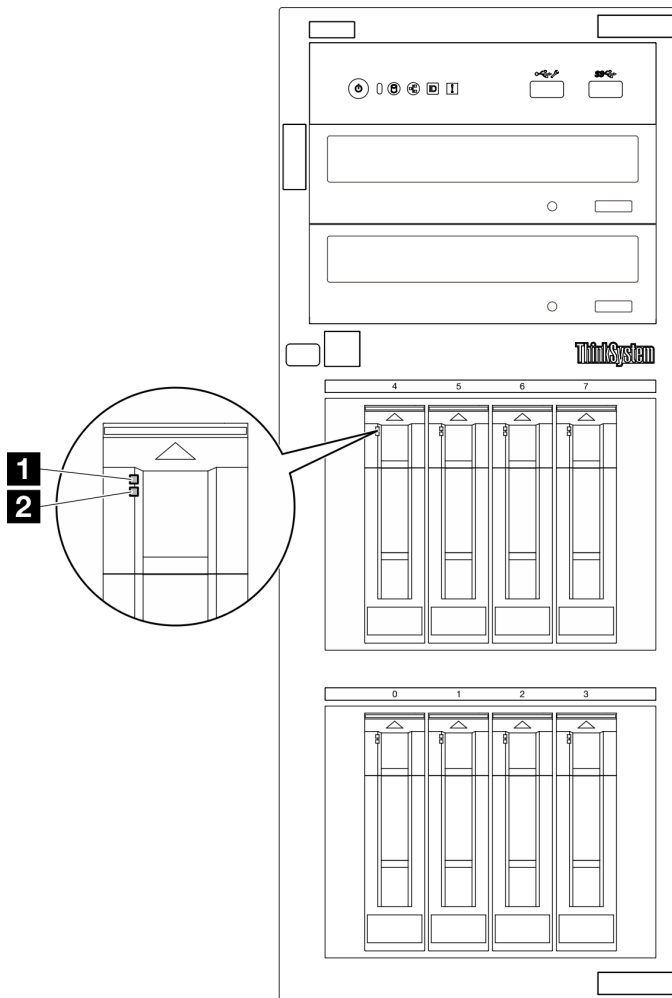
Figure 14. Voyants d'unité
