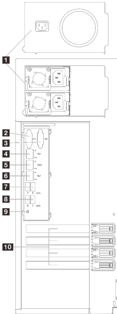
Figure 7. Vue arrière
