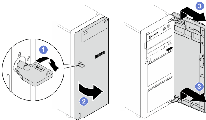
Figure 11. Verrou de la porte avant
