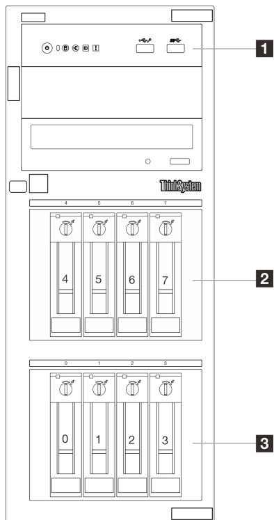
Figure 2. Vue avant des modèles de serveur équipés de huit baies d'unités à remplacement standard 3,5 pouces
