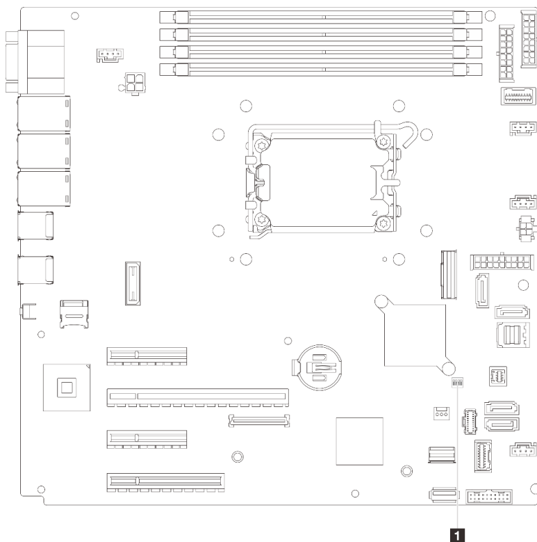
Figure 13. Commutateurs de la carte mère
