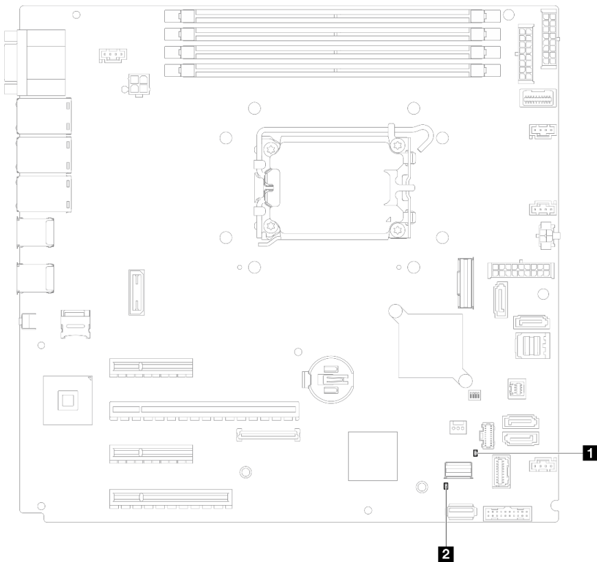
Figure 17. Voyants de la carte mère
