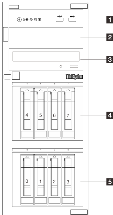
Figure 4. Vue avant des modèles de serveur équipés de huit baies d'unités remplaçables à chaud 3,5 pouces
