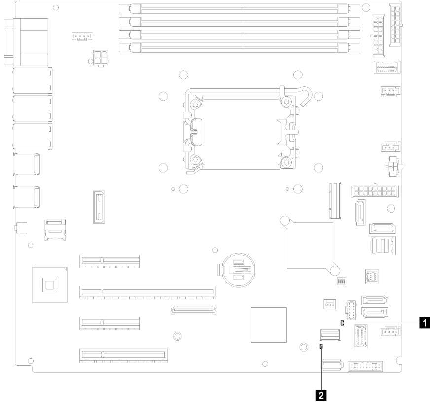
그림 17. 시스템 보드 LED
