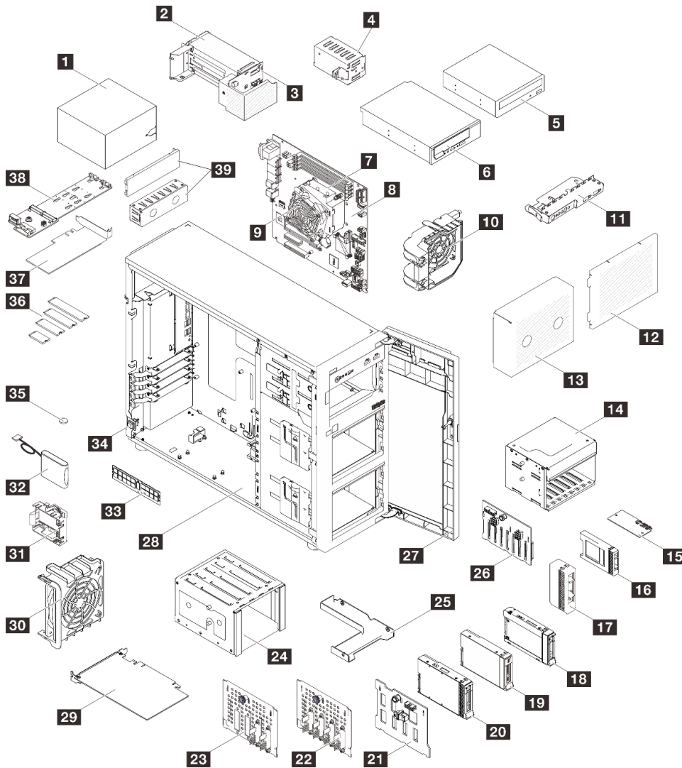
그림 20. 서버 구성 요소
