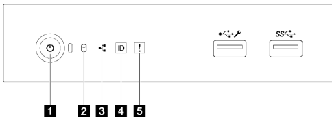
그림 15. 앞면 입/출력 모듈 LED
