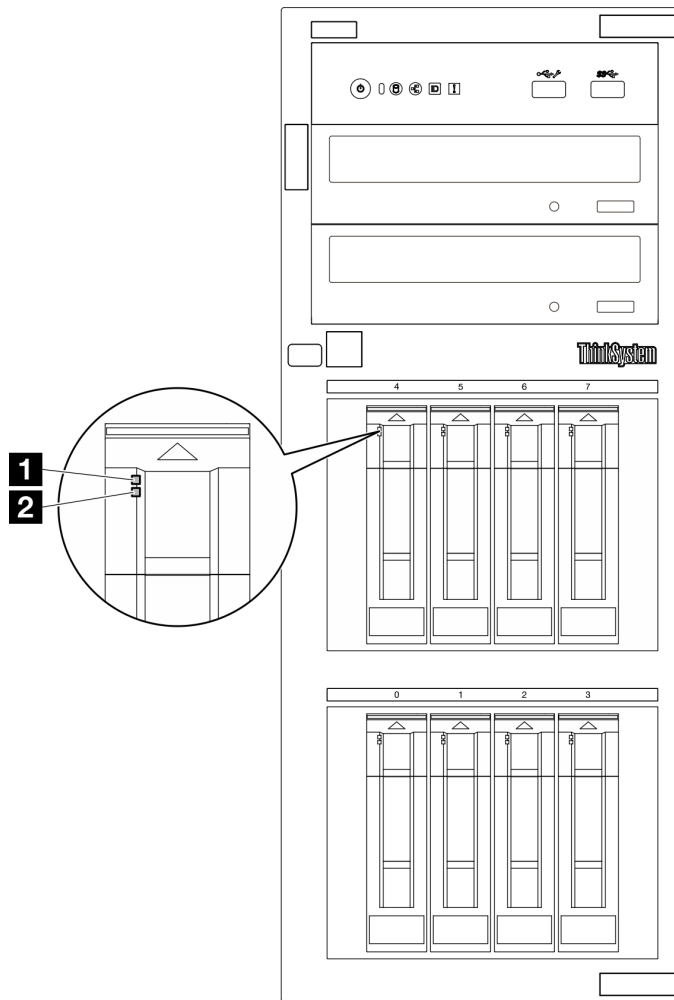
그림 14. 드라이브 LED
