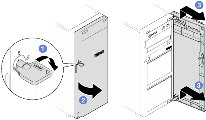
그림 11. 앞면 도어 잠금 장치
