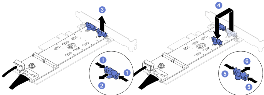
Figura 45. Ajustando o retentor M.2
