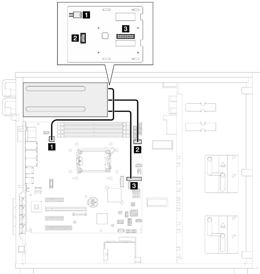
Figura 103. Roteamento de cabos das fontes de alimentação redundantes
