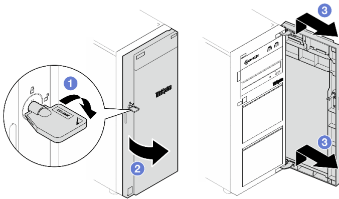
Figura 31. Removendo a porta frontal
