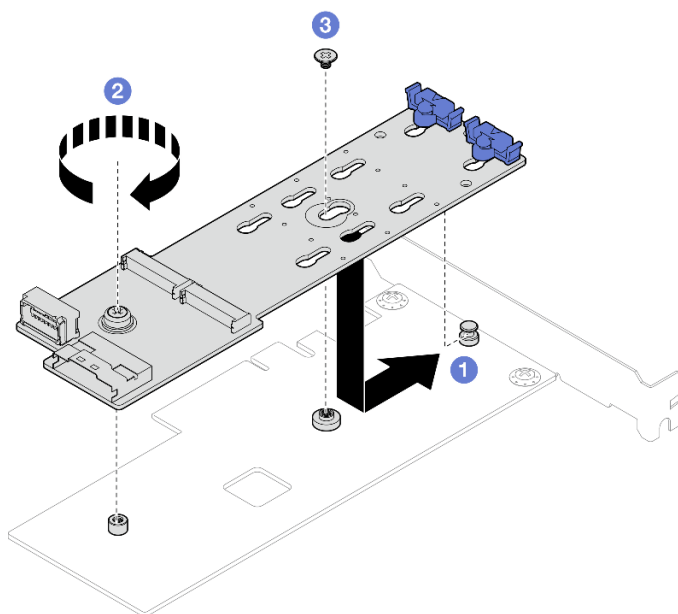
Figura 42. Prendendo o adaptador de inicialização M.2 no adaptador PCIe
