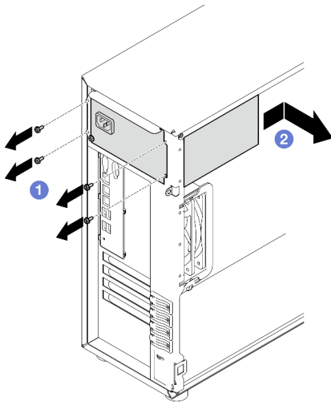
Figura 64. Removendo uma fonte de alimentação fixa
