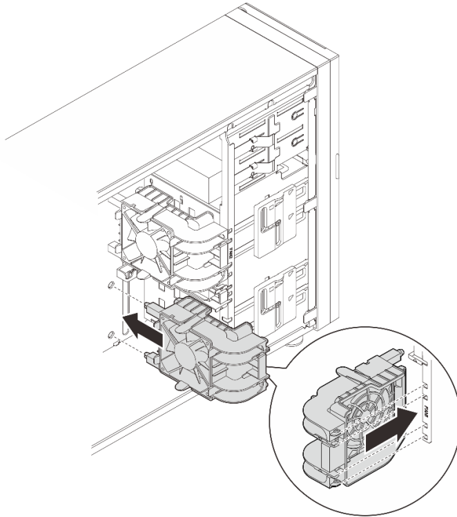
Figura 25. Instalando o ventilador frontal do sistema
