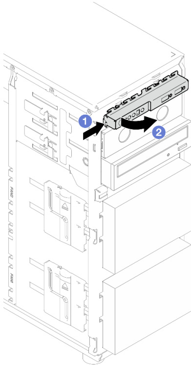
Figura 33. Removendo o módulo de E/S frontal
