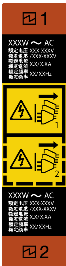
Figura 70. Rótulo da fonte de alimentação hot-swap
