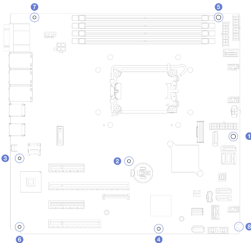
Figura 86. Removendo os parafusos que prendem a placa-mãe.
