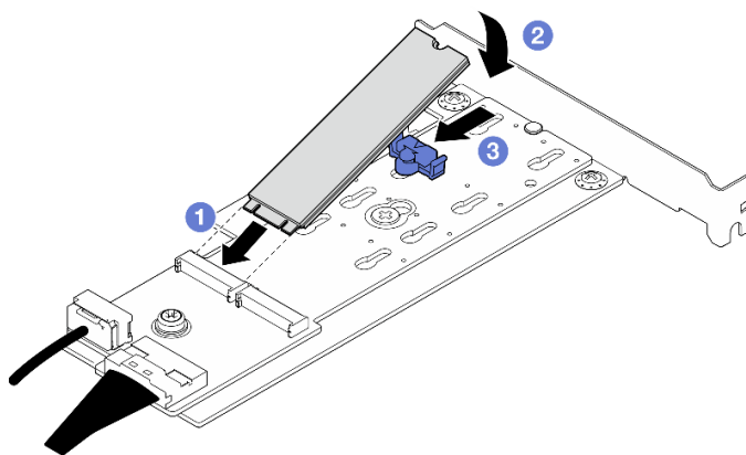
Figura 47. Instalando uma unidade M.2
