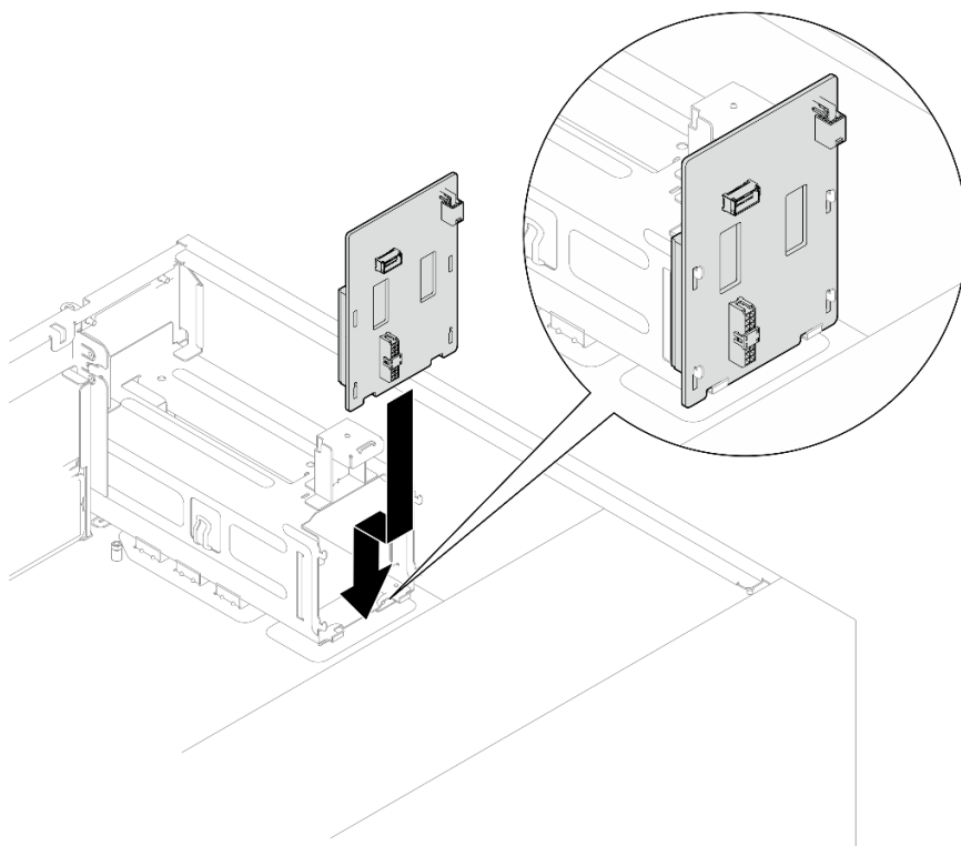
Figura 61. Instalando a placa de distribuição de energia da fonte de alimentação hot-swap
