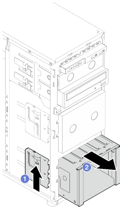
Figura 3. Removendo a gaiola de unidade
