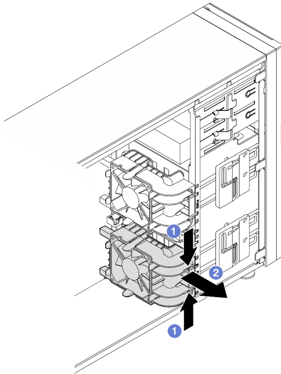
Figura 24. Removendo o ventilador frontal do sistema
