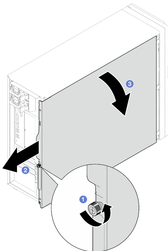
Figura 81. Removendo a tampa do servidor
