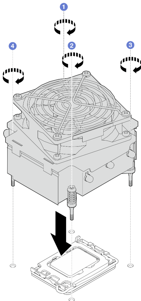
Figura 36. Instalando o módulo de dissipador de calor e de ventilador
