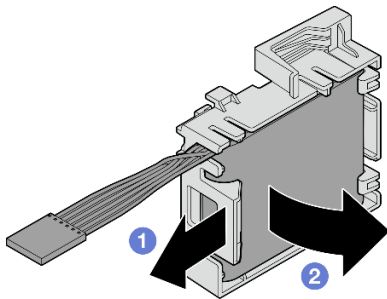
Figura 78. Removendo o módulo de energia flash do RAID do suporte
