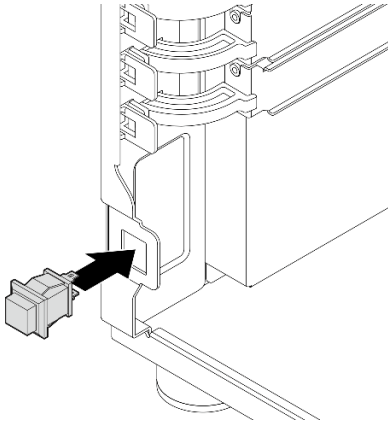
Figura 38. Instalando a chave de intrusão
