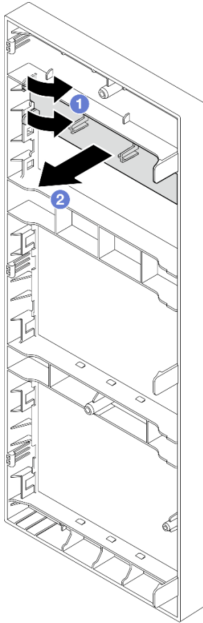
Figura 55. Removendo o preenchimento da unidade óptica do compartimento de unidade óptica
