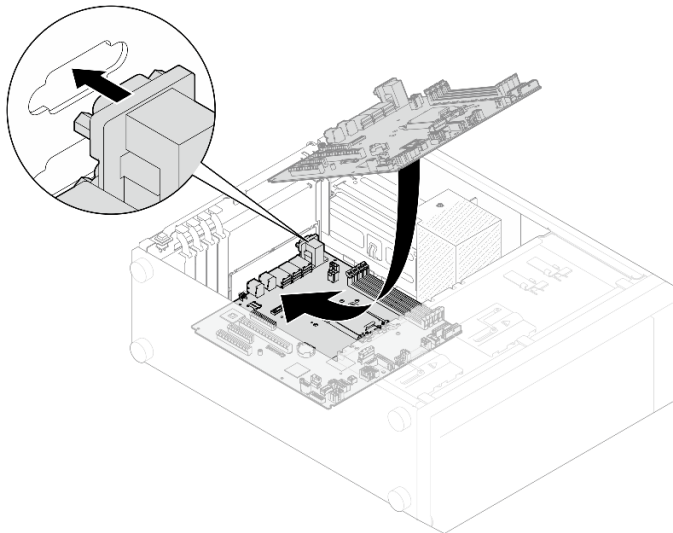
Figura 87. Instalando a placa-mãe
