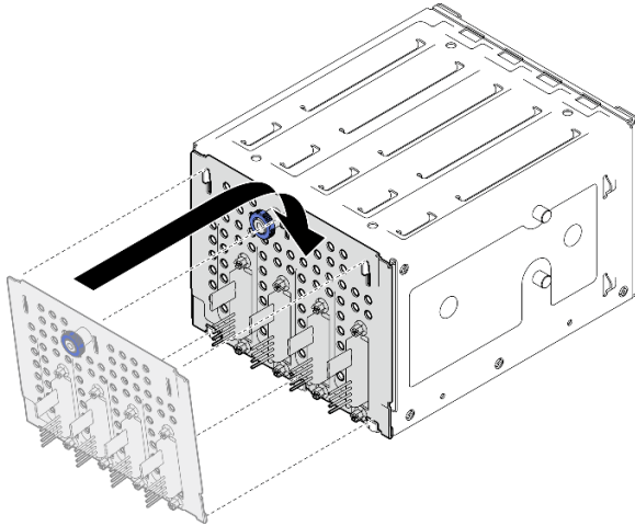
Figura 10. Instalando a placa traseira da unidade simple-swap
