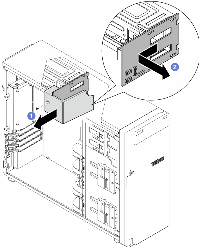
Figura 60. Removendo a placa de distribuição de energia da fonte de alimentação hot-swap
