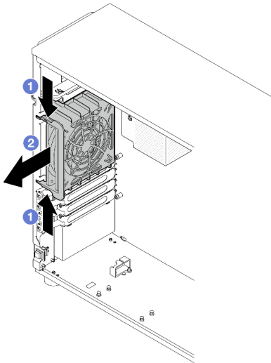
Figura 26. Removendo o ventilador traseiro do sistema
