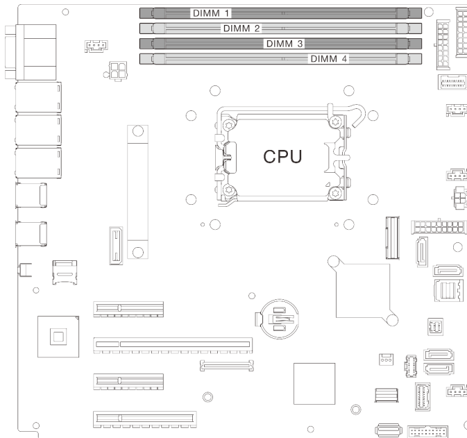
Figura 1. Layout de módulos de memória e processadores
