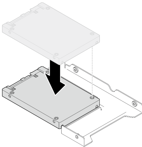
Figura 21. Posicionando a unidade de 2,5 polegadas no adaptador da unidade
