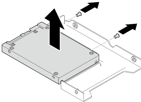
Figura 20. Removendo a unidade de 2,5 polegadas do adaptador de unidade
