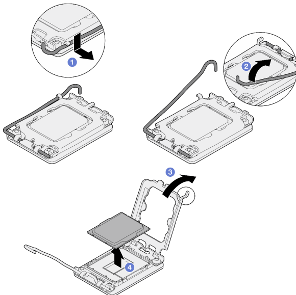
Figura 73. Abrindo o retentor de processador
