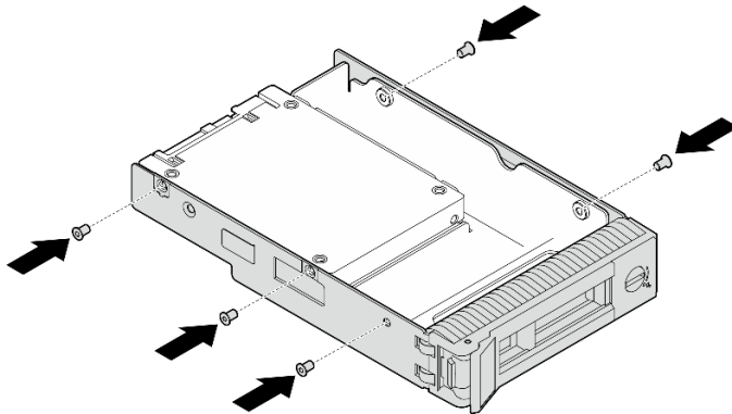
Figura 23. Instalando os parafusos para prender o adaptador de unidade e a unidade na bandeja de unidade
