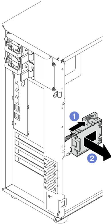
Figura 77. Removendo o módulo de energia flash RAID e o conjunto de suporte do chassi
