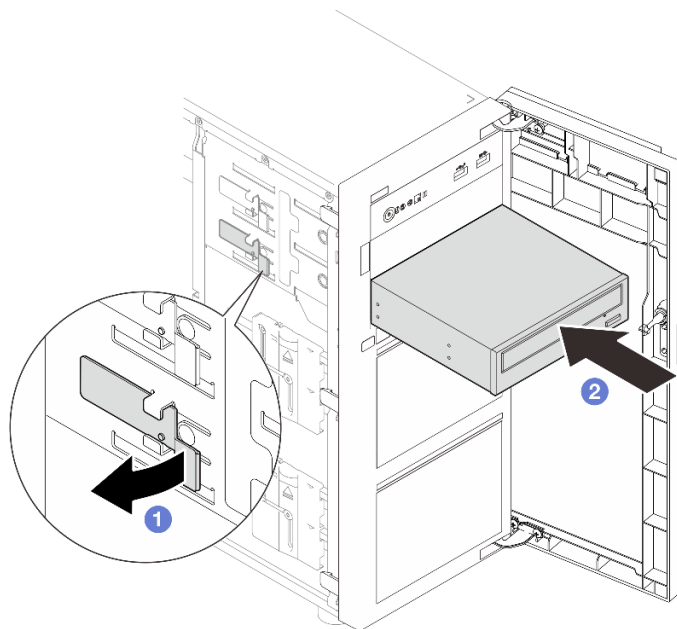
Figura 57. Instalando uma unidade óptica
