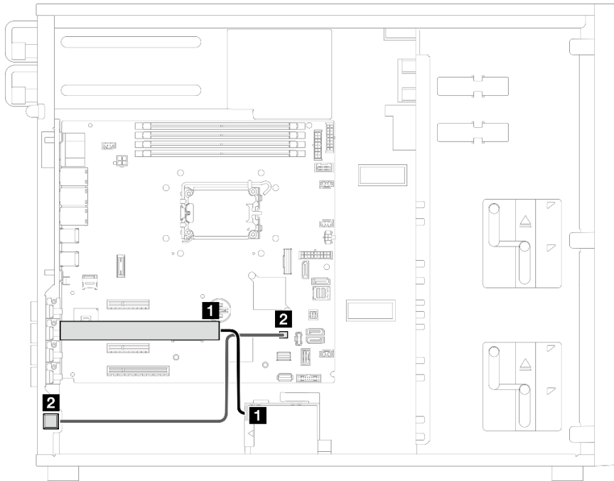
Figura 100. Roteamento de cabos da chave de intrusão e do módulo de energia flash RAID
