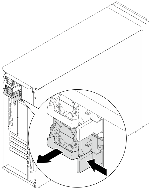
Figura 69. Removendo uma fonte de alimentação hot-swap
