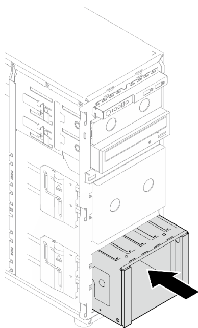
Figura 4. Instalando a gaiola de unidade
