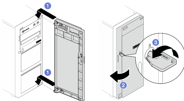
Figura 32. Instalando a porta frontal
