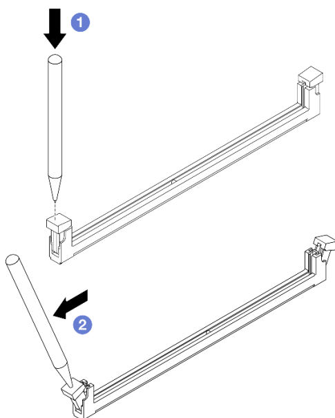
Figura 52. Abrindo as presilhas de retenção
