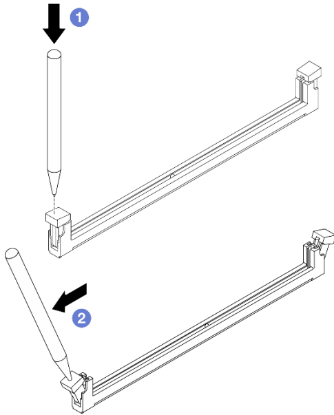
Figura 49. Abrindo as presilhas de retenção
