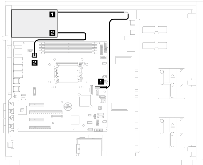
Figura 102. Roteamento de cabos da fonte de alimentação fixa
