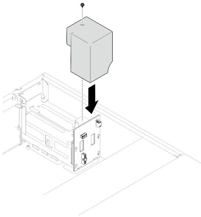
Figura 62. Instalando a tampa da placa de distribuição de energia
