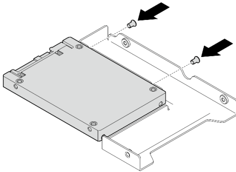
Figura 22. Instalando os parafusos que prendem a unidade ao adaptador da unidade
