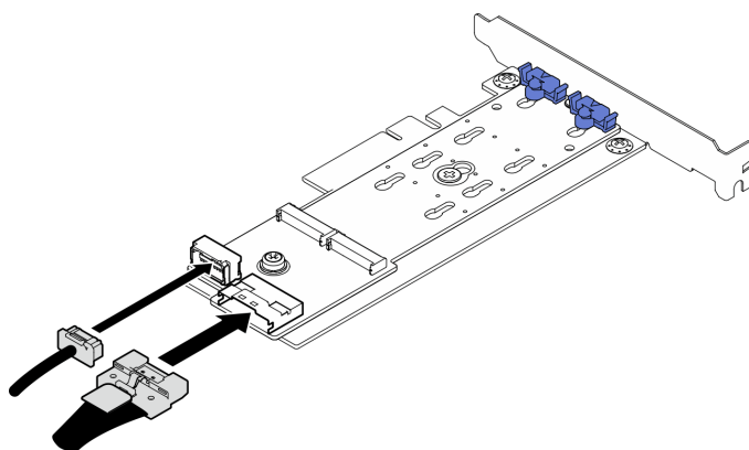
Figura 43. Instalando os cabos de alimentação e de sinal M.2
