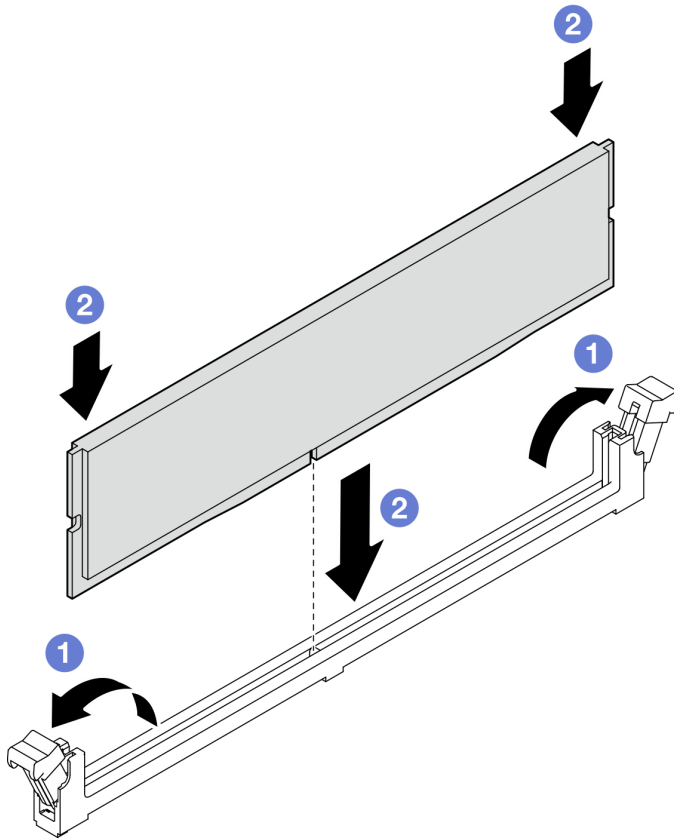
Figura 53. Instalando um módulo de memória
