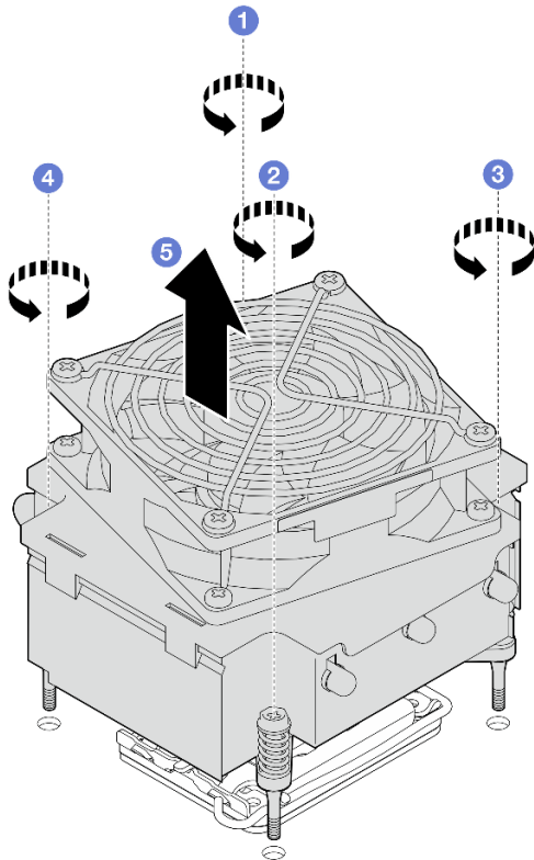
Figura 35. Removendo o módulo de dissipador de calor e de ventilador
