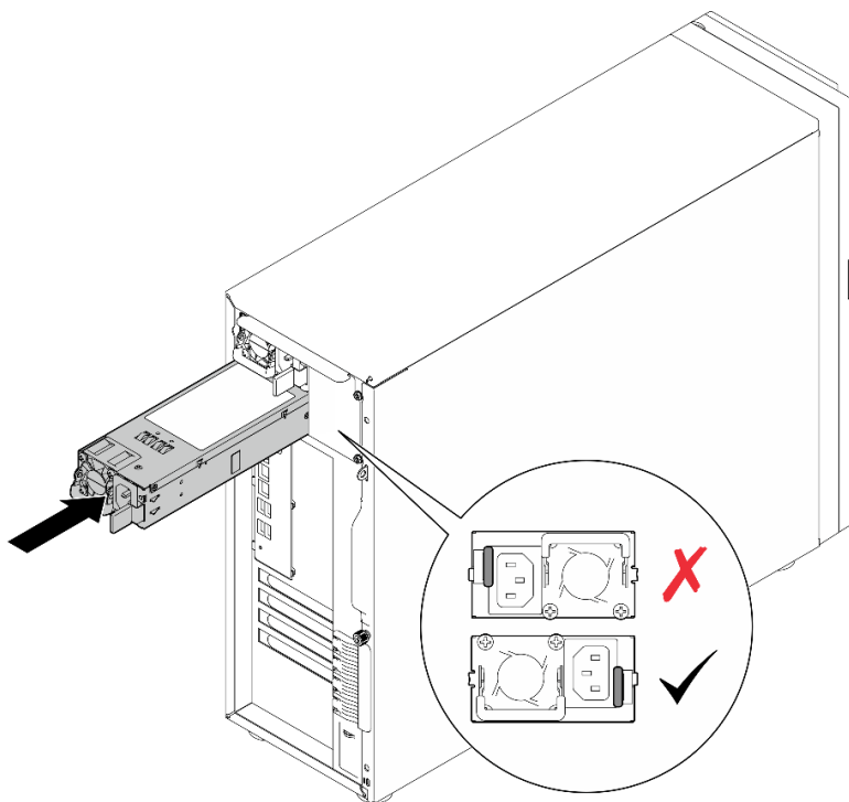
Figura 72. Instalando uma fonte de alimentação hot-swap
