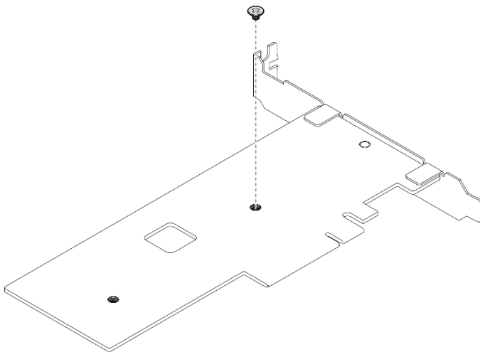
Figura 41. Removendo o parafuso na parte traseira do adaptador PCIe
