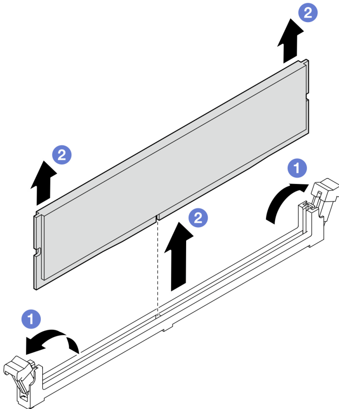
Figura 50. Removendo um módulo de memória
