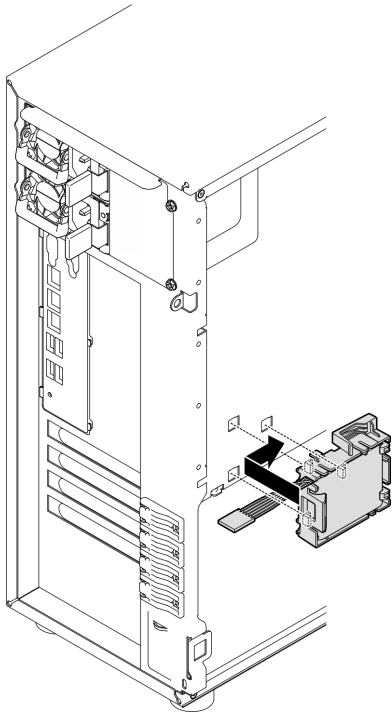
Figura 80. Instalando o módulo de energia flash RAID e o conjunto do suporte no chassi
