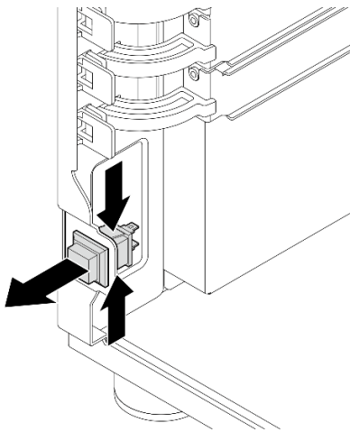
Figura 37. Removendo a chave de intrusão
