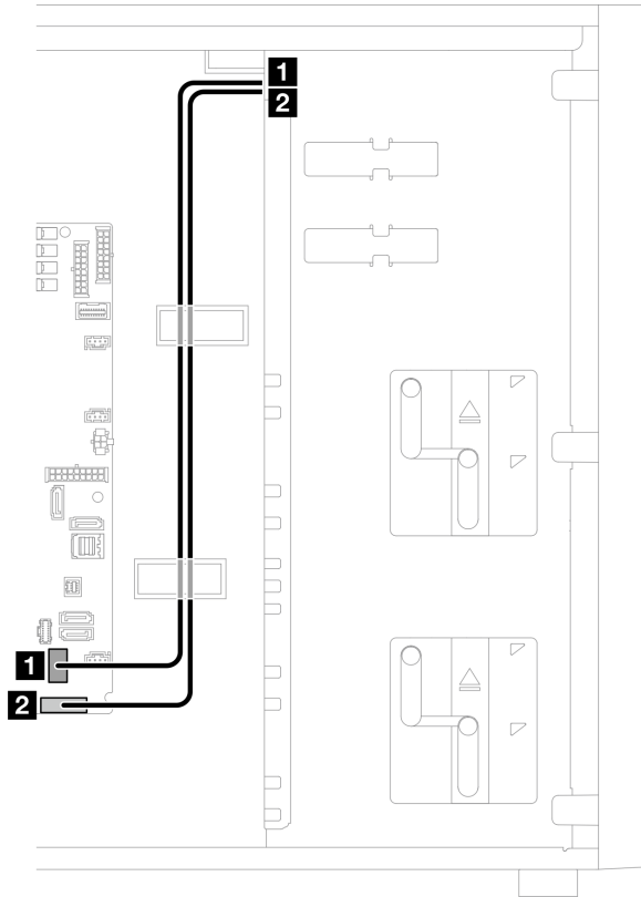
Figura 98. Roteamento de cabos do módulo de E/S frontal
