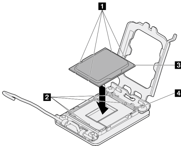
Figura 74. Instalando o processador
