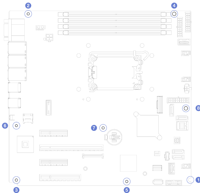
Figura 88. Instalando os parafusos para fixar a placa-mãe
