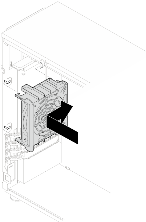
Figura 27. Posicionando o ventilador traseiro do sistema no chassi
