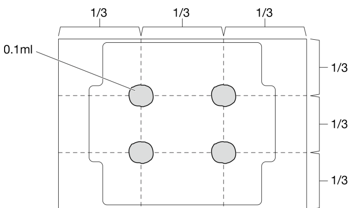
Figura 76. Formato adequado da graxa térmica
