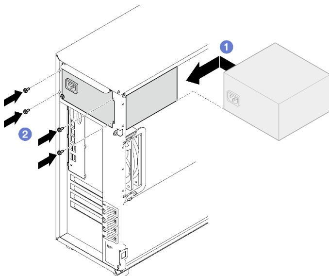
Figura 67. Instalando uma fonte de alimentação fixa
