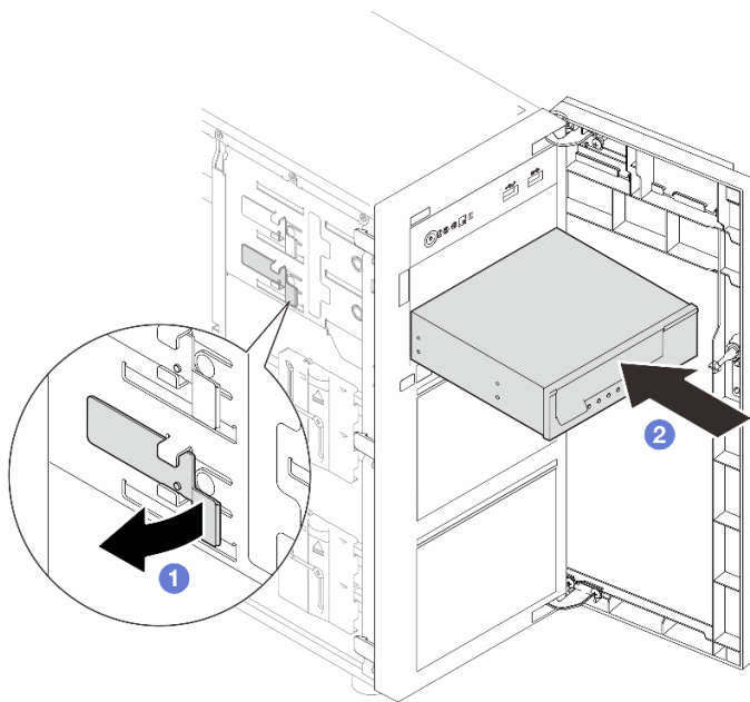
Figura 90. Instalando uma unidade de fita
