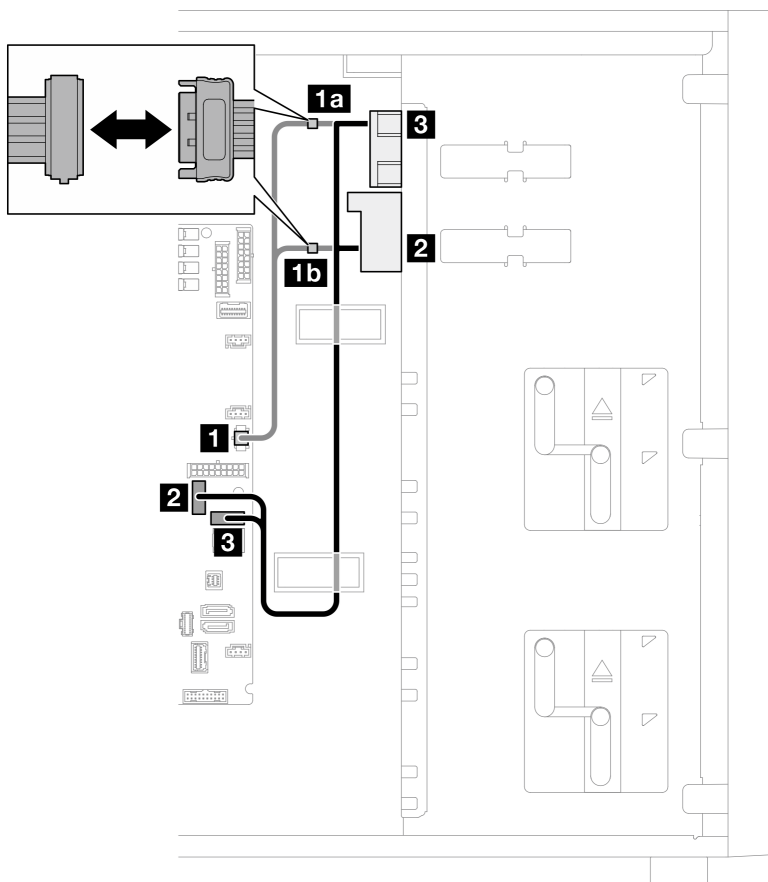
Figura 101. Roteamento dos cabos de unidades de fita/ópticas
