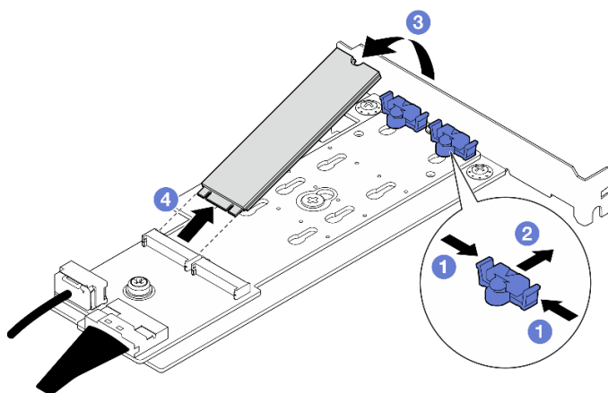
Figura 44. Removendo uma unidade M.2
