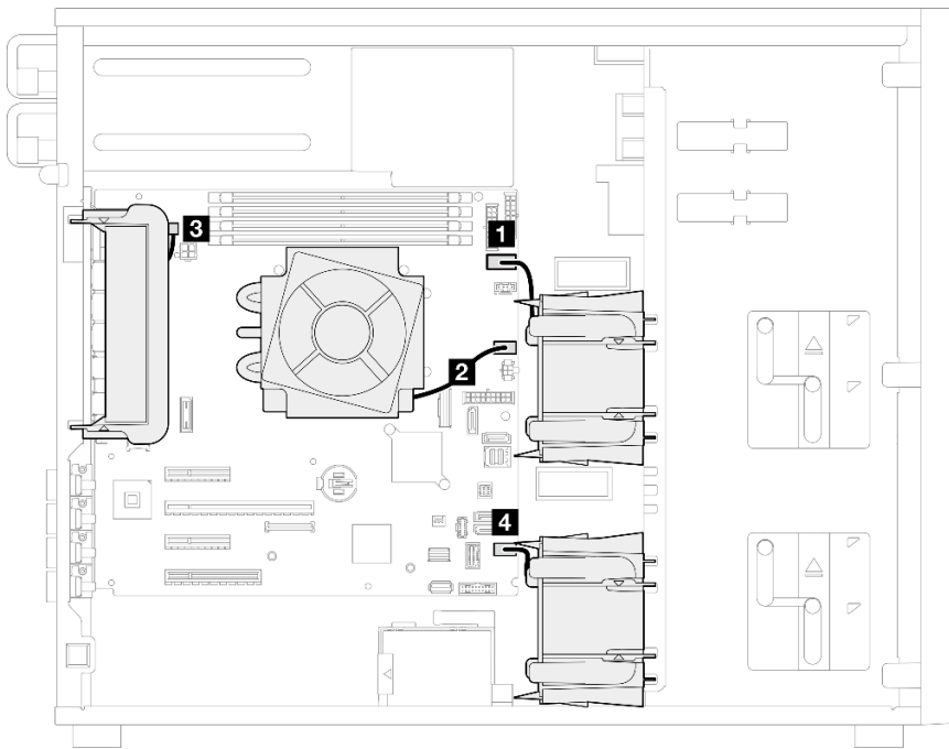
Figura 97. Roteamento do cabo de alimentação do ventilador
