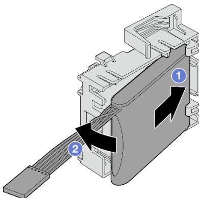
Figura 79. Instalando o módulo de energia flash RAID no suporte
