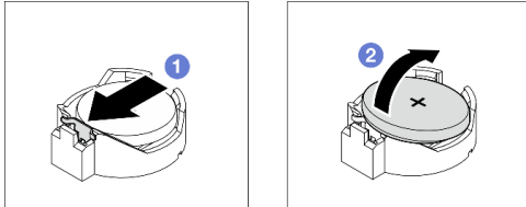
Figura 11. Removendo a bateria CMOS
