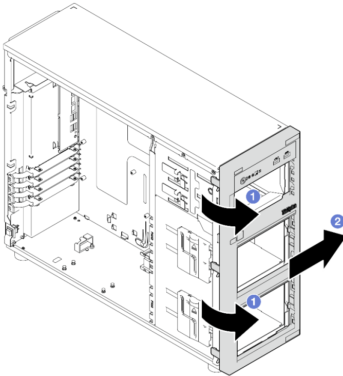
Figura 29. Removendo o painel frontal
