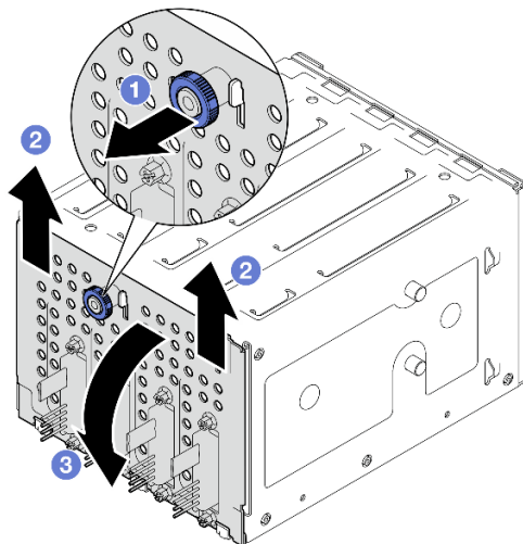
Figura 9. Removendo a placa traseira da unidade simple-swap
