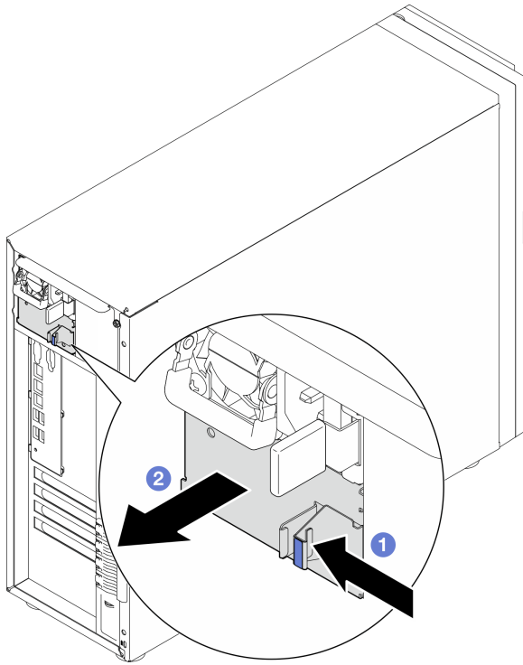
Figura 71. Removendo um preenchimento de fonte de alimentação hot-swap
