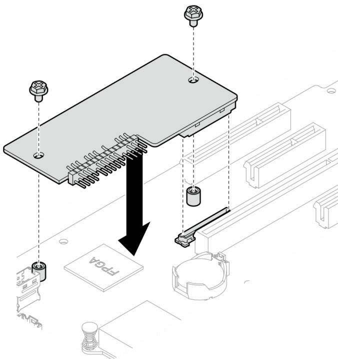
Figura 85. Instalação do firmware e módulo de segurança RoT
