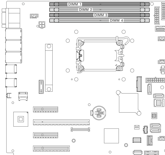
Figura 51. Slots do módulo de memória na placa-mãe
