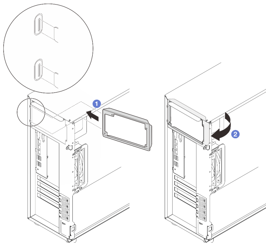
Figura 66. Instalando o suporte da fonte de alimentação fixa
