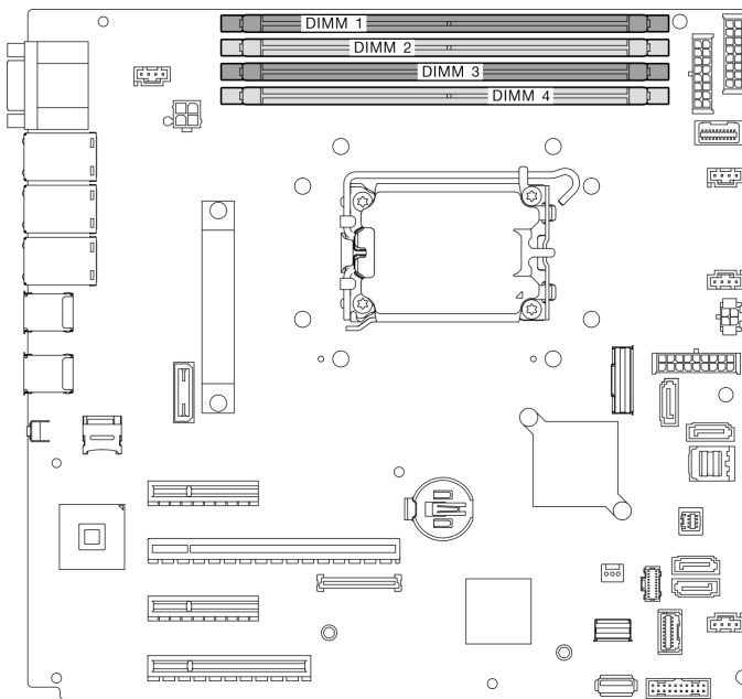
Figura 48. Slots do módulo de memória na placa-mãe
