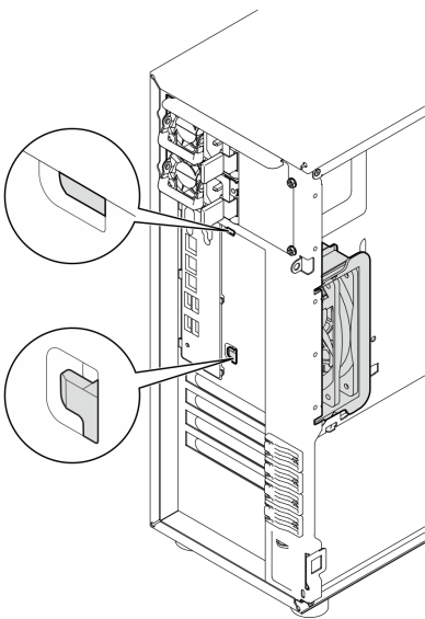
Figura 28. Instalando o ventilador traseiro do sistema
