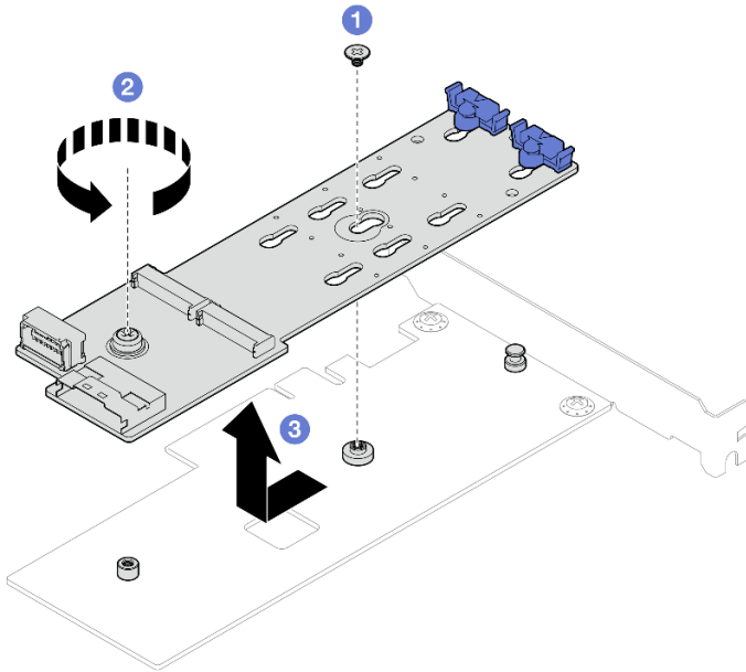
Figura 40. Remoção do adaptador de inicialização M.2
