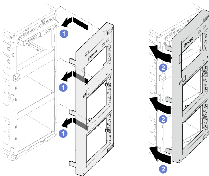
Figura 30. Instalação do painel frontal
