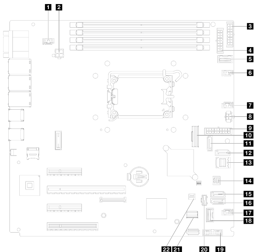
Figura 96. Conectores da Placa-mãe
