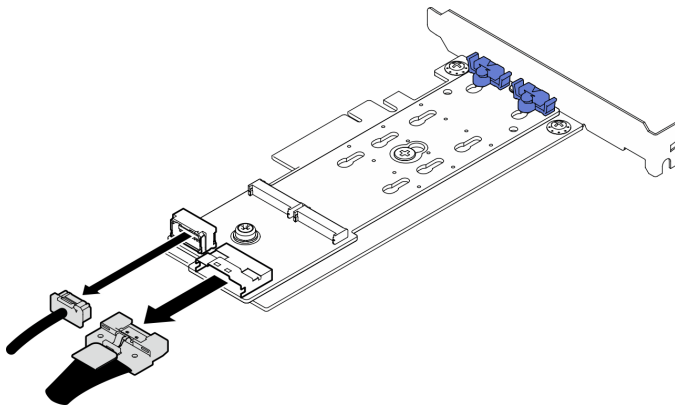
Figura 39. Desconectando os cabos de alimentação e de sinal
