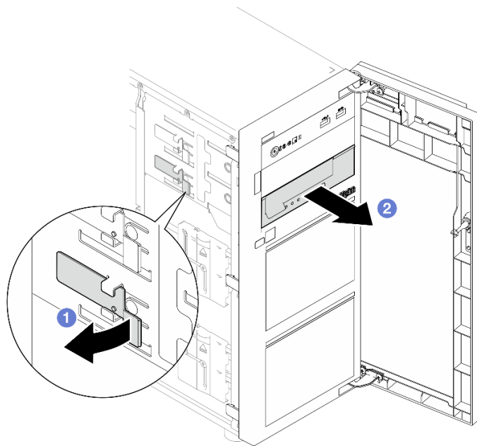
Figura 89. Removendo uma unidade de fita
