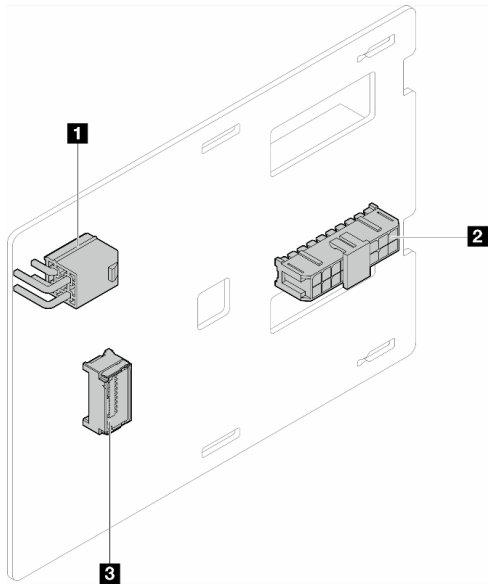
Figura 91. Placa de distribuição de energia para fontes de alimentação hot-swap
