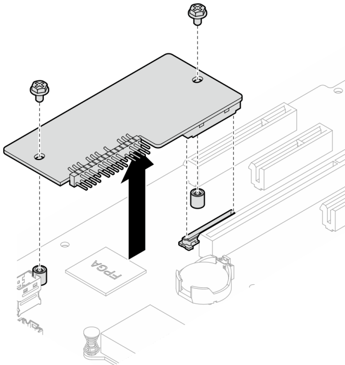
Figura 84. Remoção do firmware e módulo de segurança RoT
