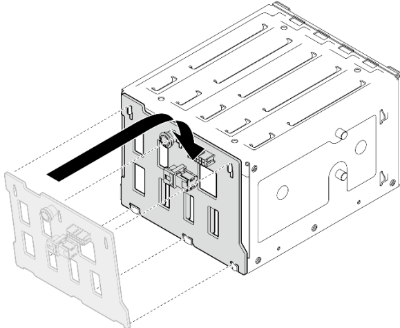
Figura 7. Instalando o backplane da unidade hot-swap
