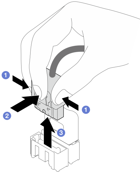
Figura 5. Desconectando o cabo do conector da unidade de disco rígido SATA
