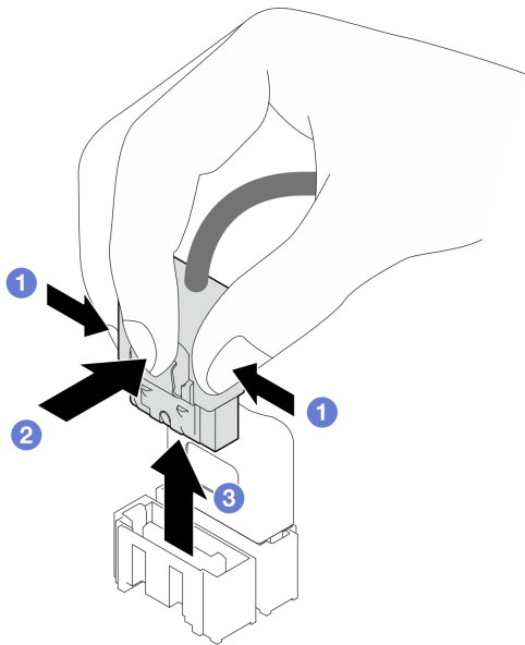
Figura 8. Desconectando o cabo do conector da unidade de disco rígido SATA
