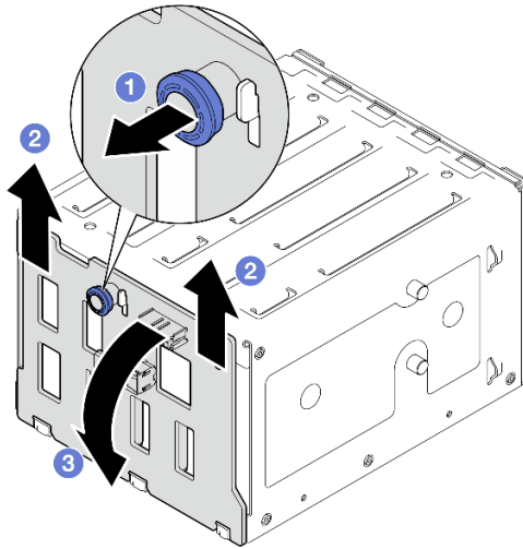
Figura 6. Removendo o backplane da unidade hot-swap
