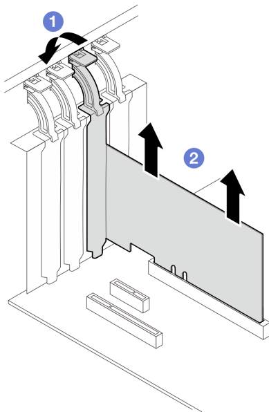
Figura 58. Removendo um adaptador PCIe
