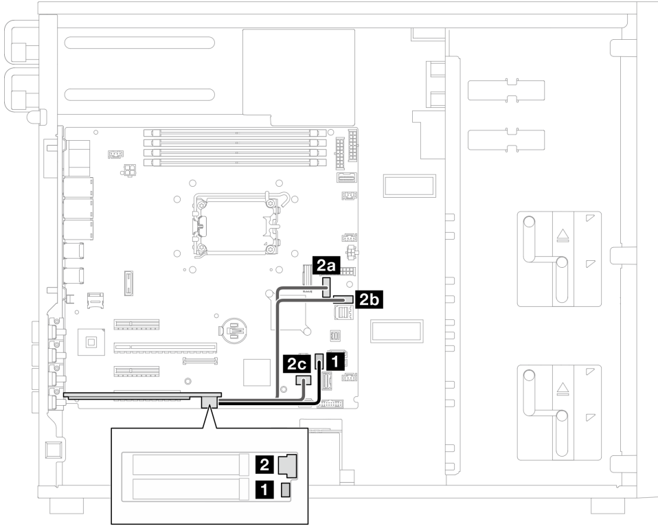
Figura 99. Roteamento de cabos do adaptador M.2
