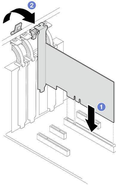
Figura 59. Instalando um adaptador PCIe
