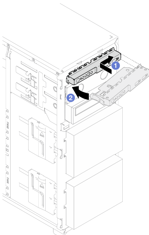
Figura 34. Instalando o módulo de E/S frontal
