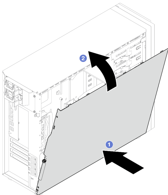
Figura 82. Posicionando a tampa do servidor no chassi
