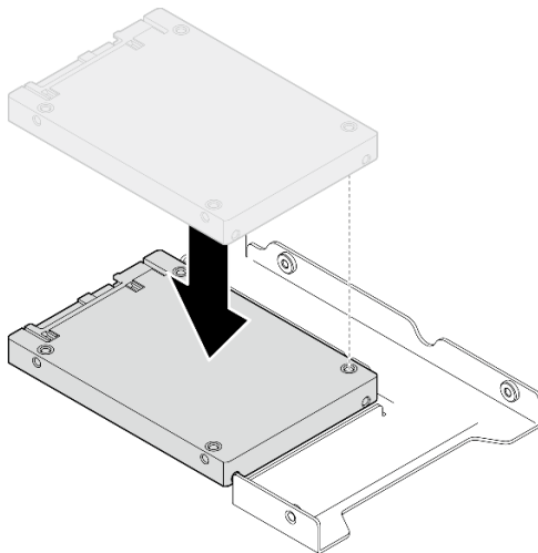
Рис. 21. Размещение 2,5-дюймового диска в адаптере для дисков
