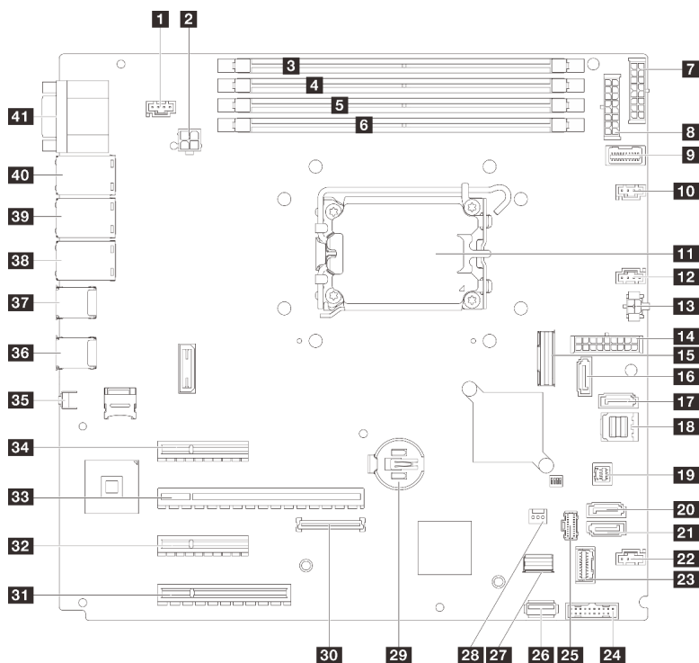
Рис. 106. Разъемы материнской платы
