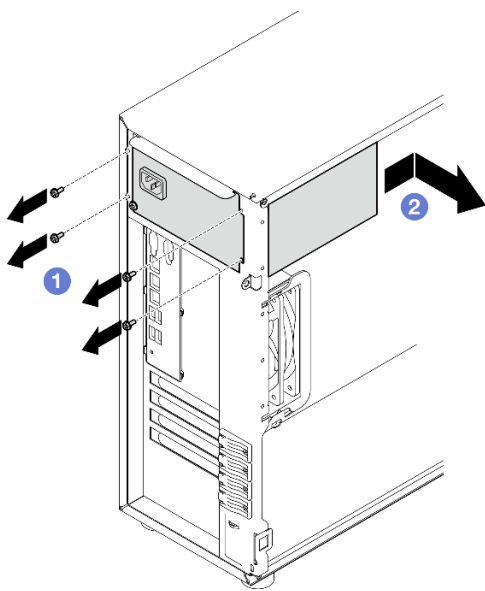
Рис. 64. Снятие стационарного блока питания
