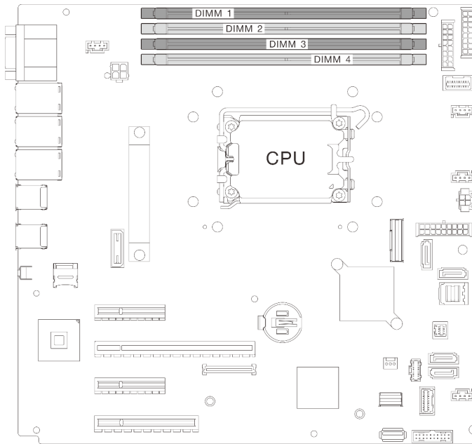
Рис. 1. Расположение модулей памяти и процессоров
