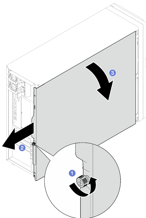
Рис. 81. Снятие кожуха сервера
