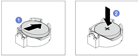
Рис. 12. Установка батарейки CMOS
