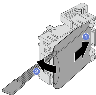
Рис. 79. Установка модуля питания флеш-памяти RAID в скобу
