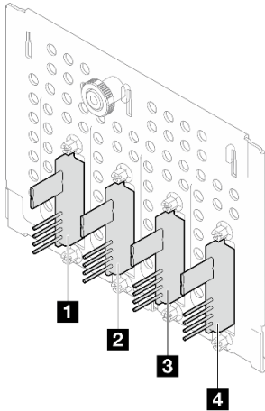
Табл. 4. Задняя панель 3,5-дюймовых дисков с обычной заменой (отсеки 4–7 без дисководов для оптических дисков)
