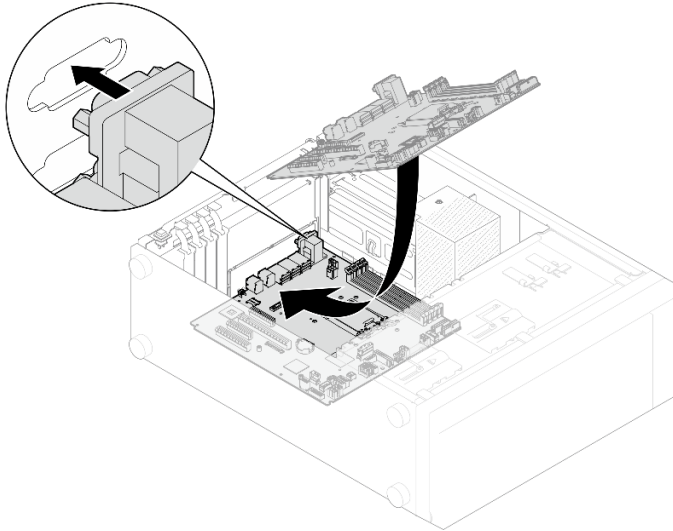
Рис. 87. Установка материнской платы
