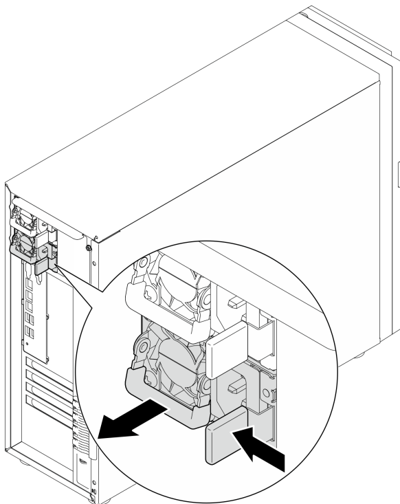
Рис. 69. Снятие оперативно заменяемого блока питания
