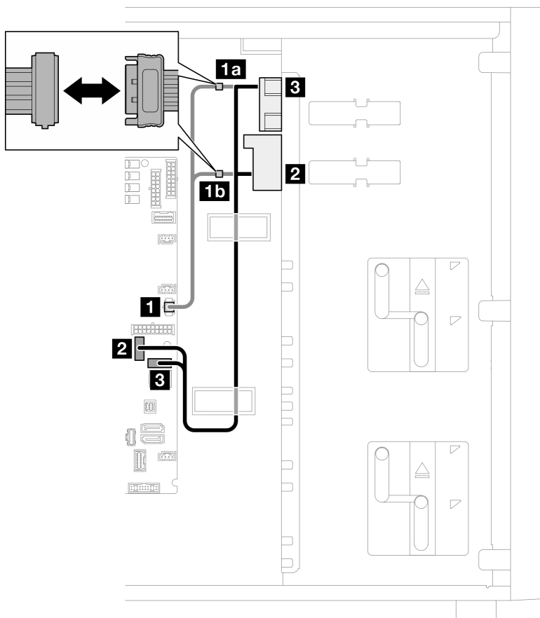
Рис. 101. Прокладка кабелей для дисководов оптических дисков/ленточных накопителей
