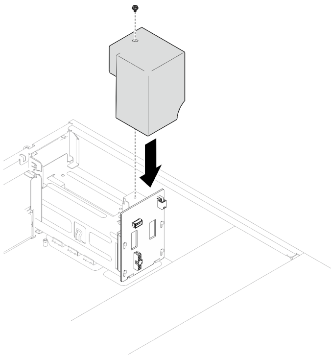
Рис. 62. Установка кожуха распределительного щита
