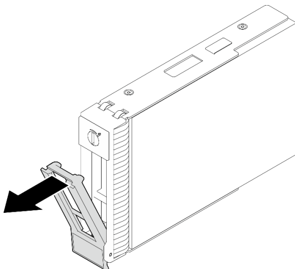
Рис. 17. Снятие диска с обычной заменой
