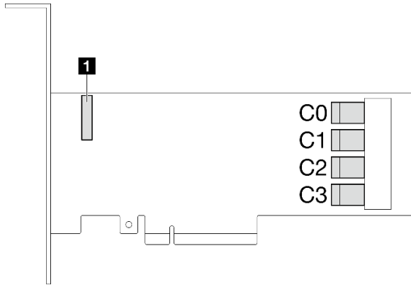
Рис. 95. Разъемы 9350-16i
