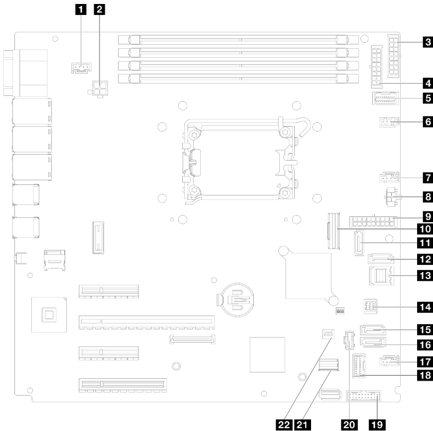
Рис. 96. Разъемы материнской платы
