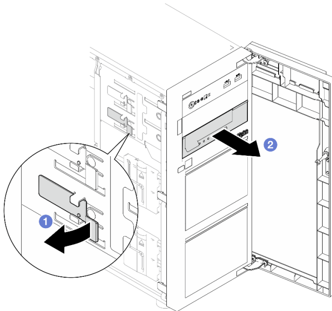
Рис. 89. Удаление ленточного накопителя
