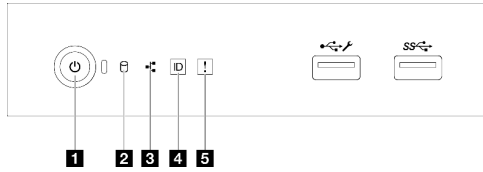
Рис. 108. Светодиодные индикаторы переднего модуля ввода-вывода
