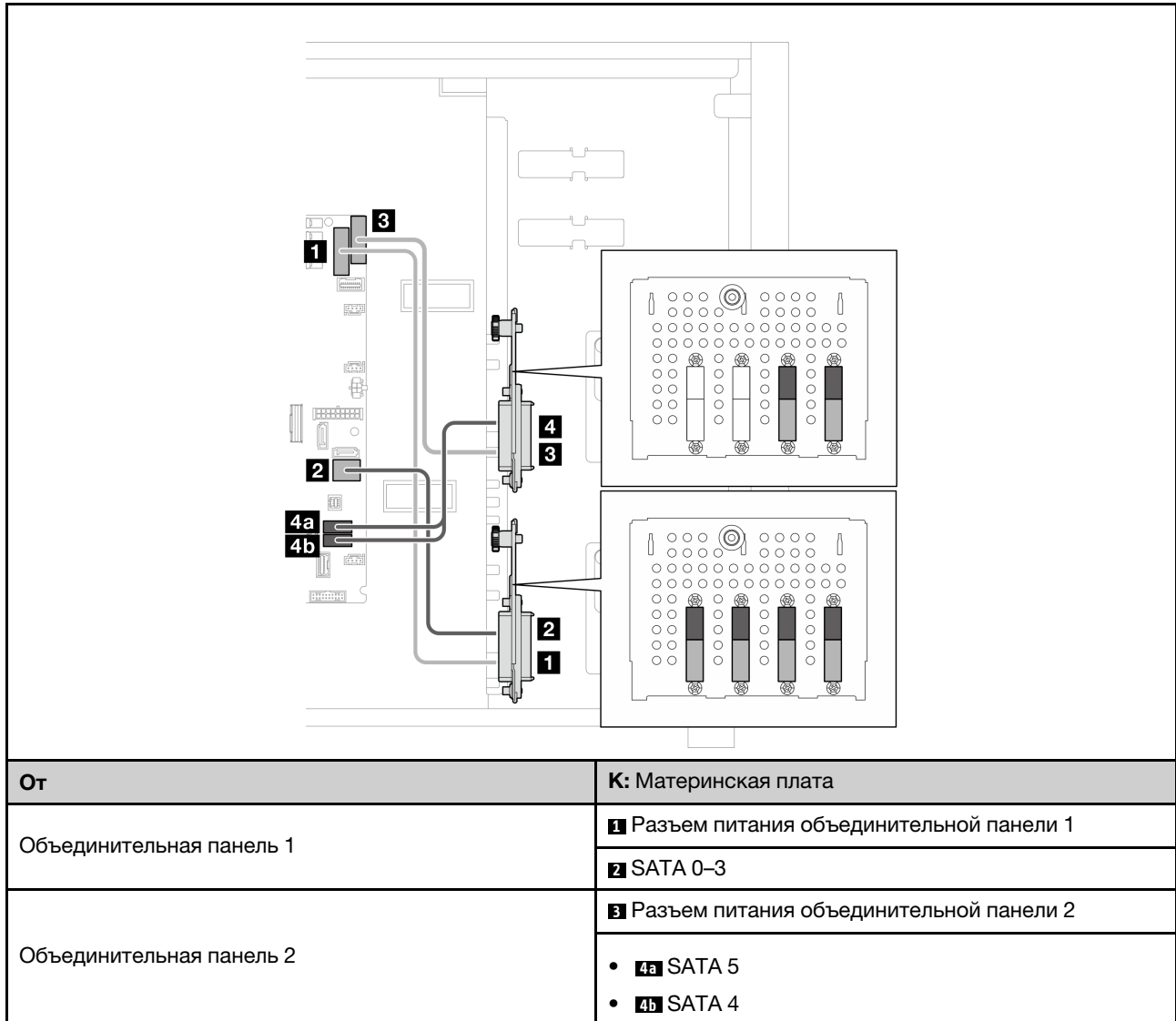
Табл. 14. Прокладка кабелей для шести 3,5-дюймовых дисков с обычной заменой
