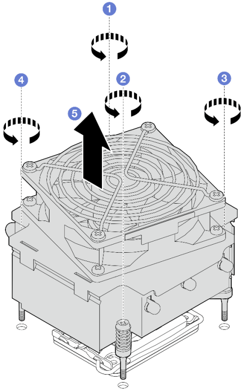
Рис. 35. Снятие модуля радиатора и вентилятора
