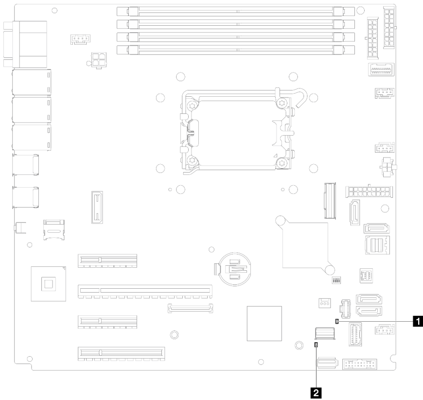
Рис. 110. Светодиодные индикаторы материнской платы
