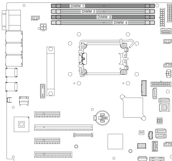
Рис. 51. Гнезда модулей памяти на материнской плате
