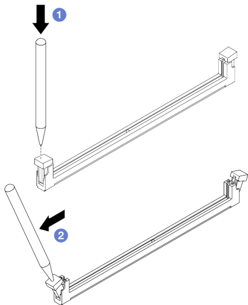
Рис. 49. Открытие фиксирующих защелок
