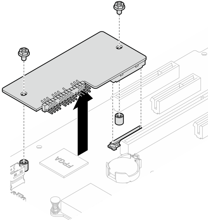
Рис. 84. Снятие модуля безопасности микропрограммы и RoT
