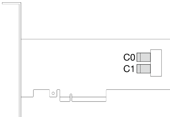
Рис. 94. разъемы 4350/5350-8i
