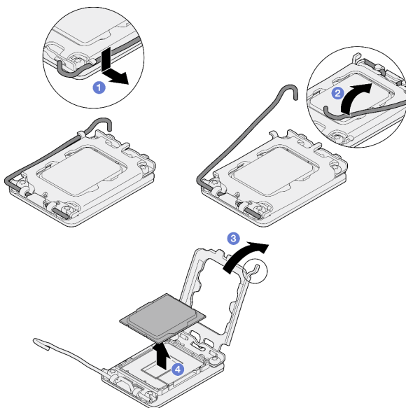
Рис. 73. Открытие фиксатора процессора
