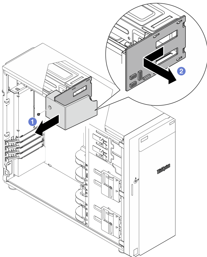
Рис. 60. Снятие платы распределения питания оперативно заменяемого блока питания
