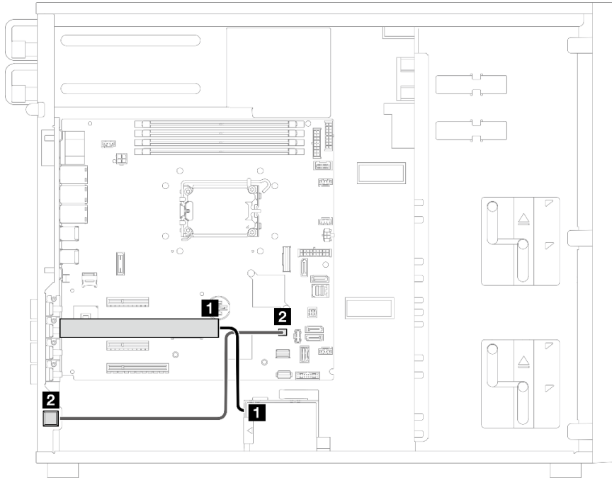
Рис. 100. Прокладка кабелей для датчика вмешательства и модуля питания флэш-памяти RAID
