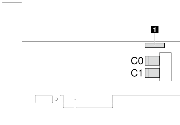
Рис. 92. разъемы 9350-8i
