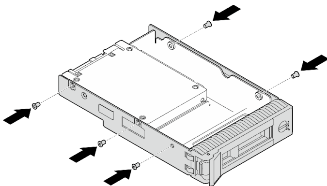
Рис. 23. Установка винтов для фиксации адаптера для дисков и диска в лотке для дисков
