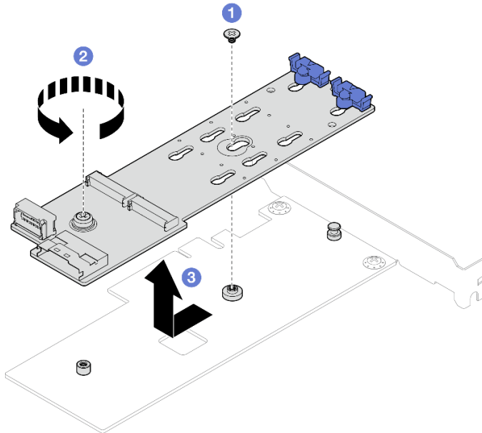
Рис. 40. Снятие адаптера загрузки M.2
