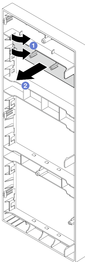
Рис. 55. Снятие заглушки дисководов для оптических дисков с отсека дисководов для оптических дисков
