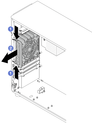
Рис. 26. Снятие заднего вентилятора компьютера
