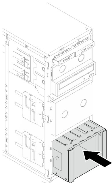
Рис. 4. Установка отсека для дисков
