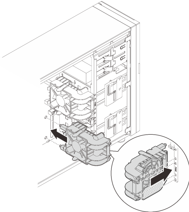
Рис. 25. Установка переднего вентилятора компьютера
