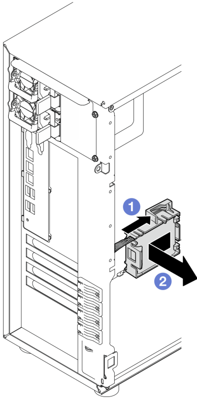
Рис. 77. Снятие модуля питания флеш-памяти RAID и блока скобы с рамы
