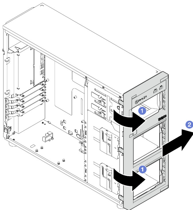
Рис. 29. Снятие лицевой панели
