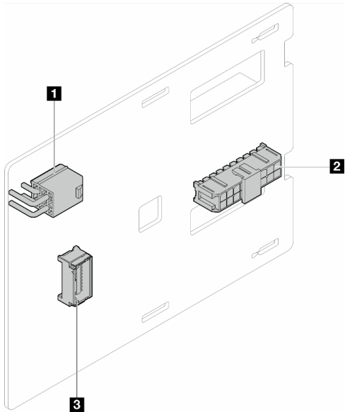
Рис. 91. Плата распределения питания оперативно заменяемых блоков питания
