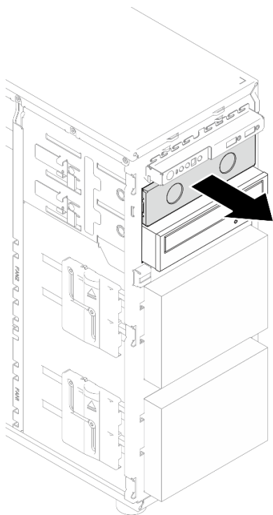
Рис. 56. Снятие крышки заглушки дисководов для оптических дисков с отсека дисководов для оптических дисков
