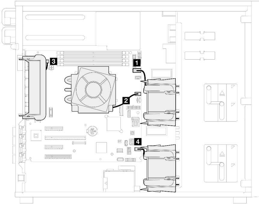
Рис. 97. Прокладка кабелей питания вентиляторов
