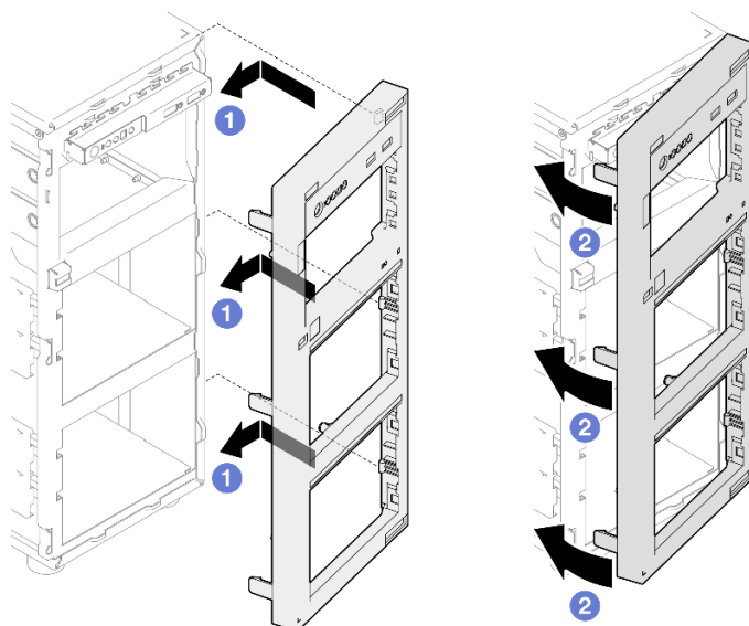
Рис. 30. Установка лицевой панели
