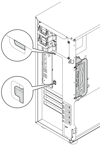
Рис. 28. Установка заднего вентилятора компьютера
