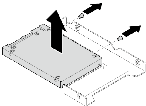
Рис. 20. Снятие 2,5-дюймового диска с адаптера для дисков
