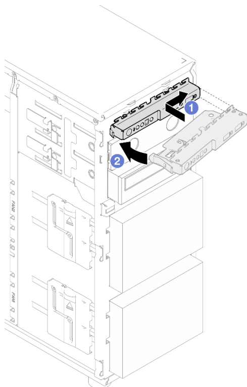
Рис. 34. Установка переднего модуля ввода-вывода
