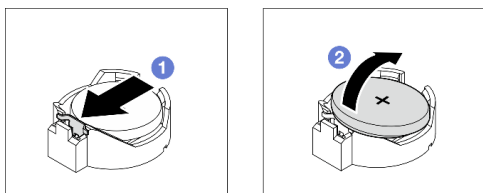
Рис. 11. Снятие батарейки CMOS
