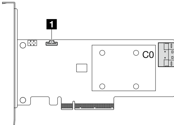
Рис. 93. разъем 940-8i
