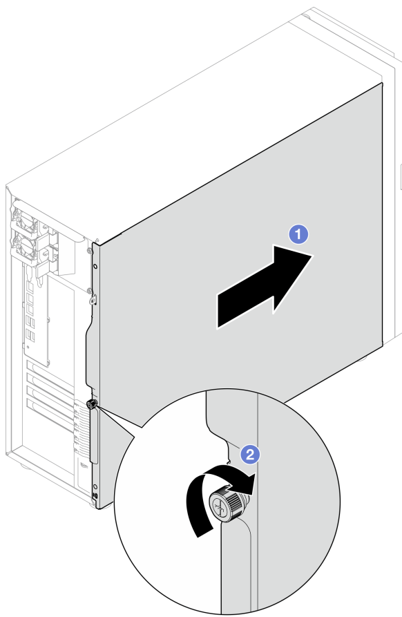
Рис. 83. Фиксация кожуха сервера на раме
