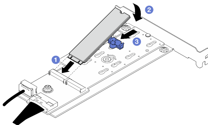
Рис. 47. Установка диска M.2
