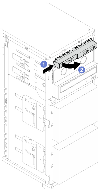
Рис. 33. Снятие переднего модуля ввода-вывода
