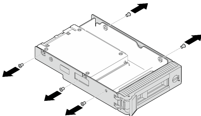
Рис. 19. Снятие винтов, фиксирующих 2,5-дюймовый диск и адаптер диска
