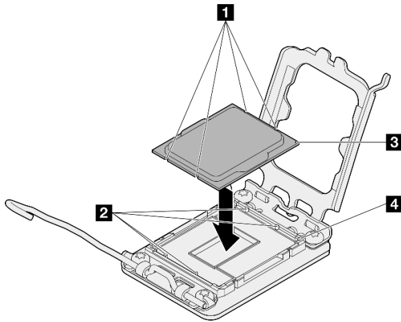
Рис. 74. Установка процессора
