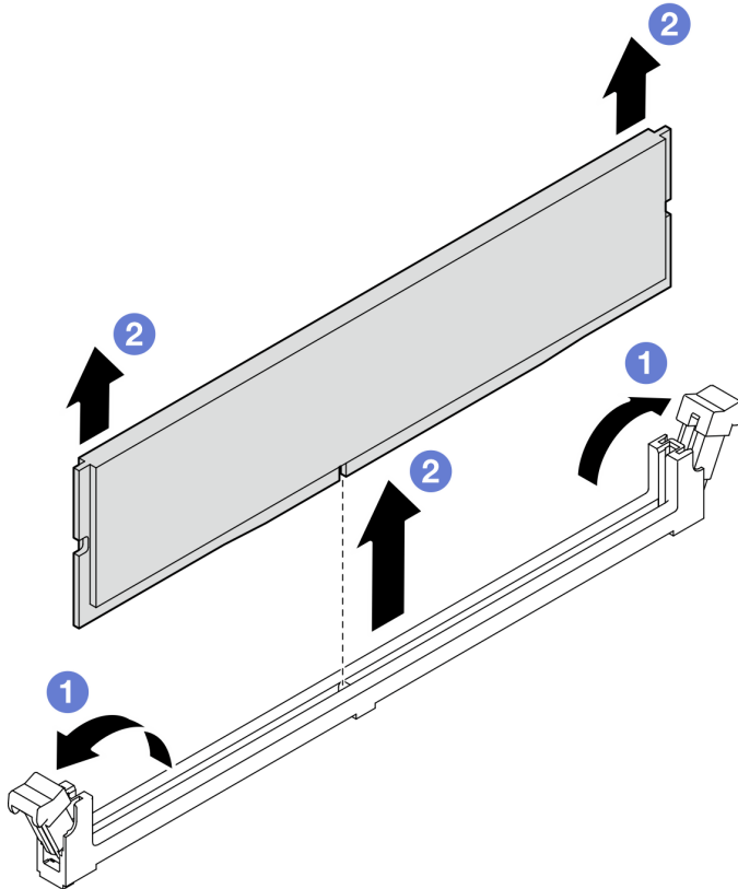
Рис. 50. Снятие модуля памяти
