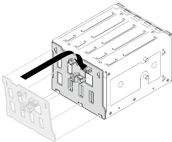
Рис. 7. Установка объединительной панели оперативно заменяемых дисков
