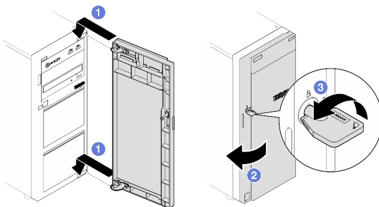
Рис. 32. Установка передней дверцы
