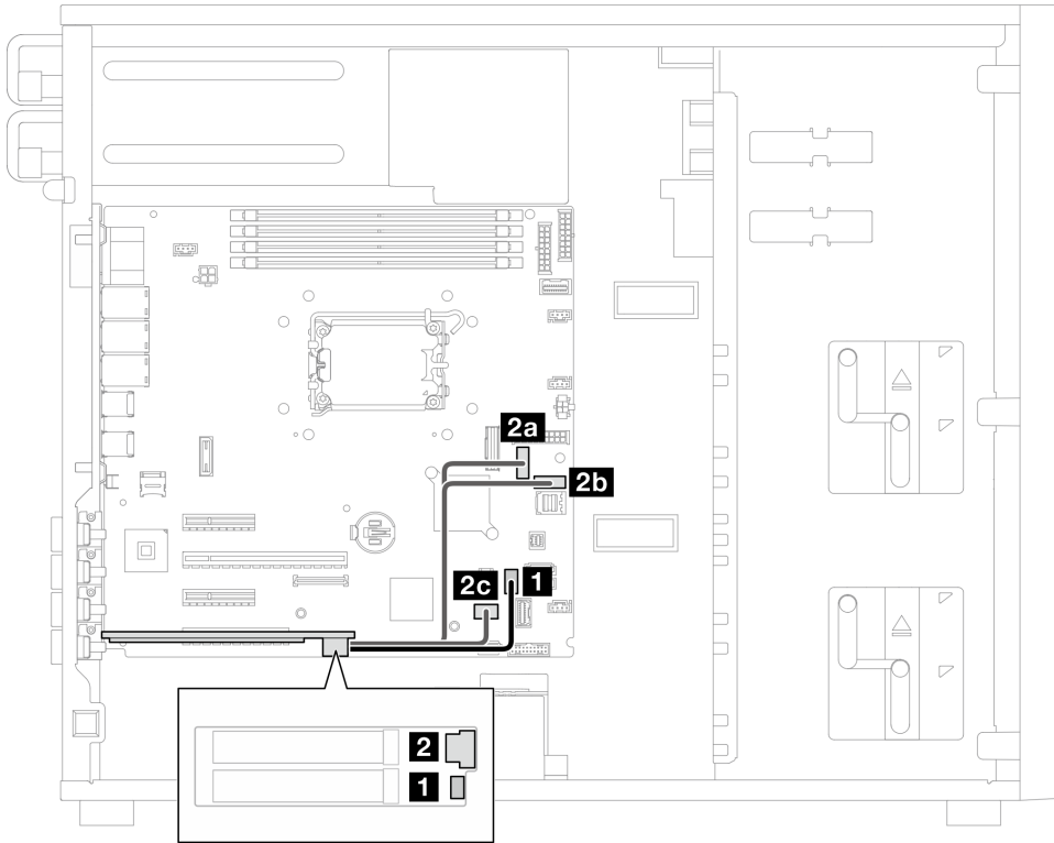
Рис. 99. Прокладка кабелей для адаптера M.2
