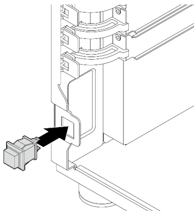
Рис. 38. Установка датчика вмешательства
