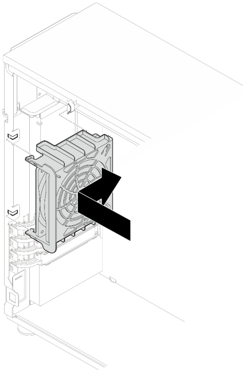
Рис. 27. Вставка заднего вентилятора компьютера в раму
