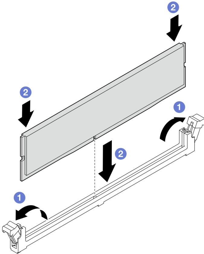
Рис. 53. Установка модуля памяти
