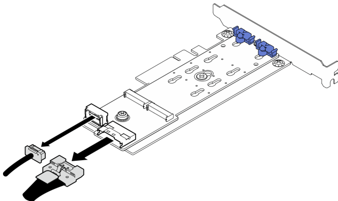
Рис. 39. Отключение кабеля питания и сигнального кабеля
