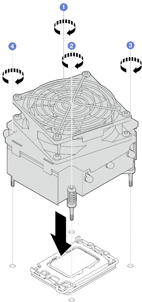
Рис. 36. Установка модуля радиатора и вентилятора
