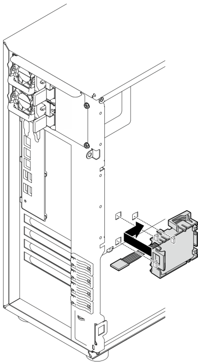
Рис. 80. Установка блока с модулем питания флэш-памяти RAID и скобой на раму
