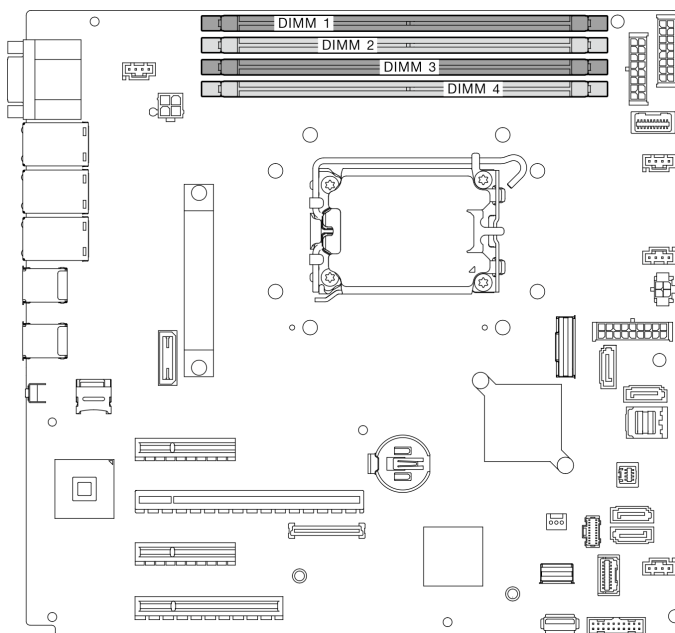
Рис. 48. Гнезда модулей памяти на материнской плате
