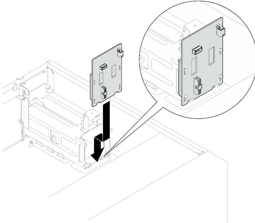
Рис. 61. Установка платы распределения питания оперативно заменяемого блока питания
