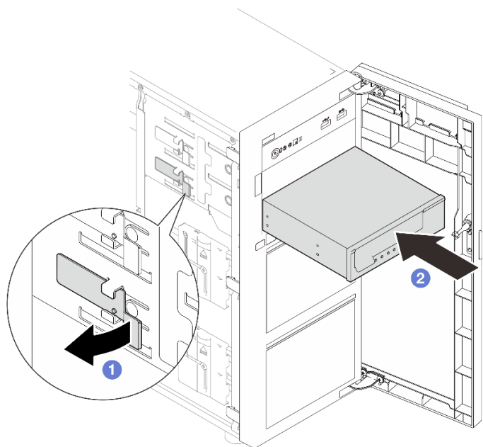
Рис. 90. Установка ленточного накопителя
