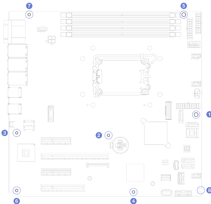
Рис. 86. Снятие винтов, фиксирующих материнскую плату
