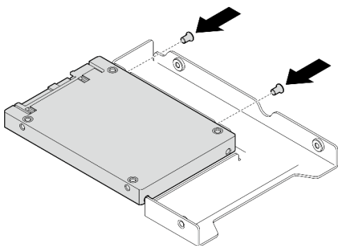
Рис. 22. Установка винтов для фиксации диска в адаптере дисков
