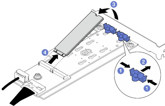
Рис. 44. Снятие диска M.2
