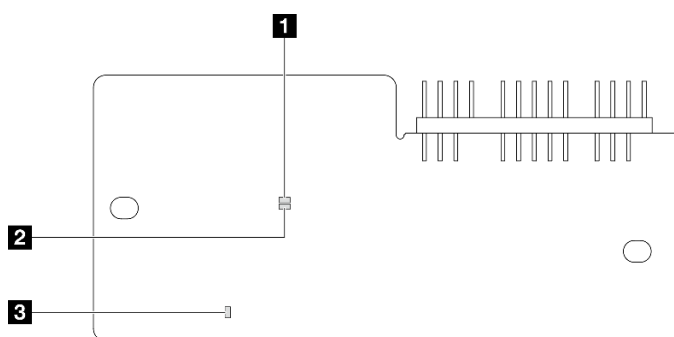
Рис. 111. Светодиодные индикаторы на компоненте «модуль безопасности микропрограммы и RoT»
