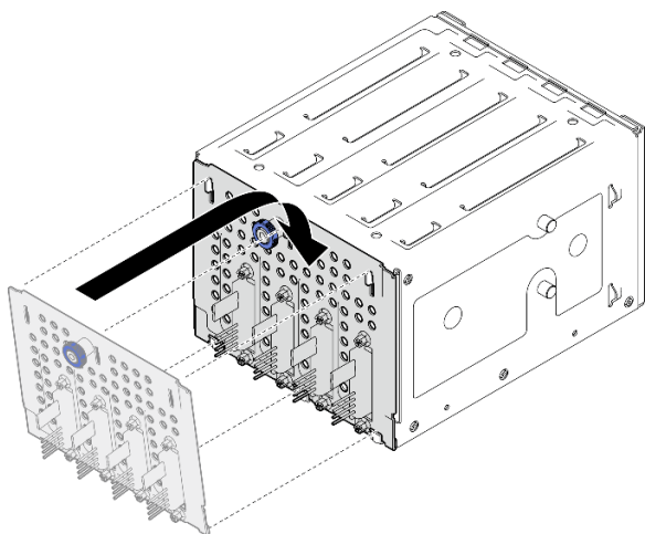
Рис. 10. Установка задней панели дисков с обычной заменой
