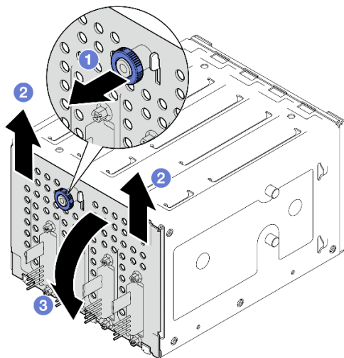
Рис. 9. Снятие задней панели дисков с обычной заменой
