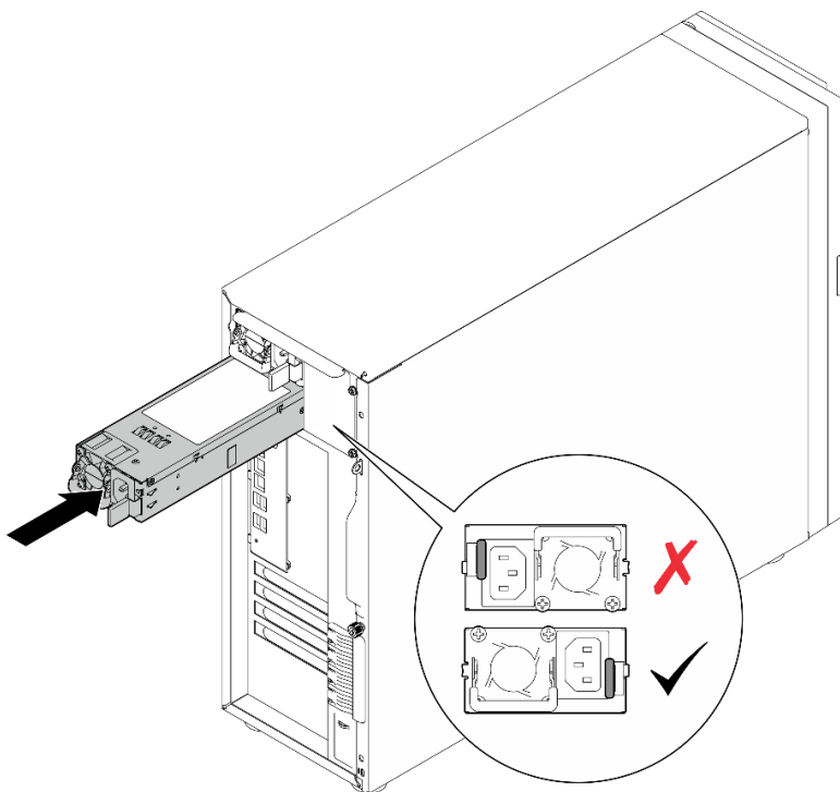
Рис. 72. Установка оперативно заменяемого блока питания
