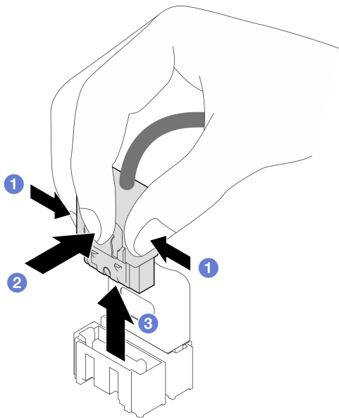
Рис. 2. Отсоединение кабеля от разъема дисководов для жесткого диска SATA
