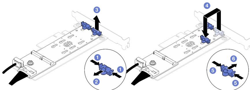
Рис. 45. Регулировка фиксатора M.2
