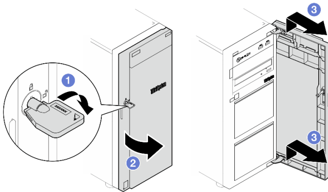
Рис. 31. Снятие передней дверцы
