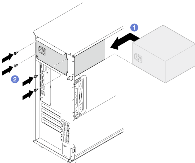
Рис. 67. Установка стационарного блока питания
