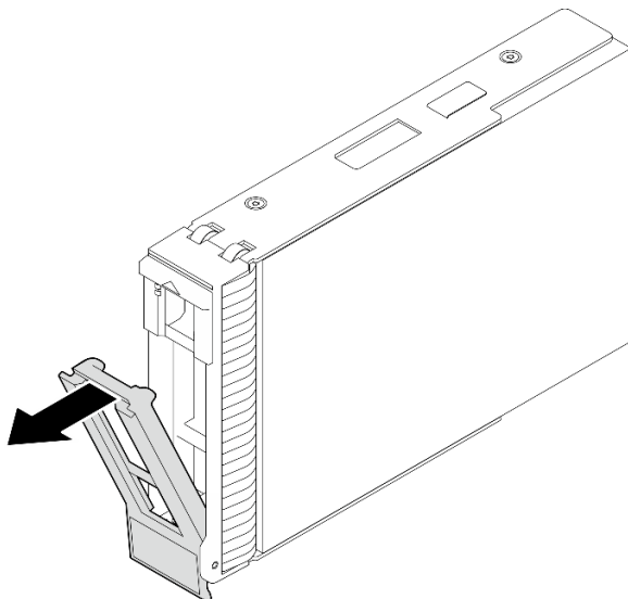
Рис. 14. Извлечение оперативно заменяемого диска из лотка для диска
