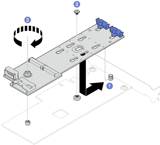
Рис. 42. Фиксация адаптера загрузки M.2 на адаптере PCIe
