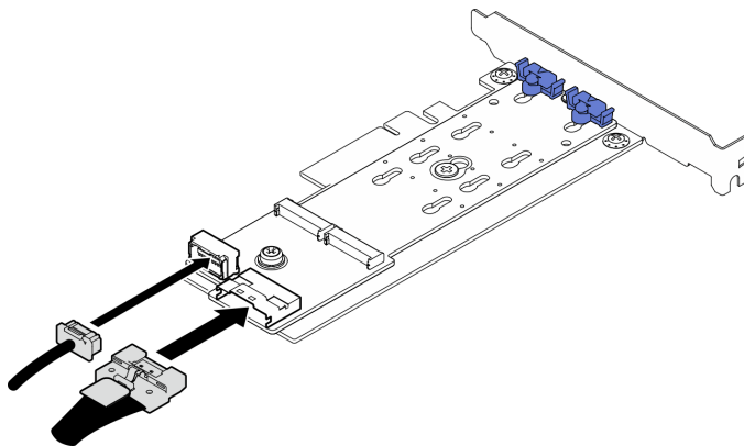
Рис. 43. Установка кабелей питания и сигнальных кабелей M.2
