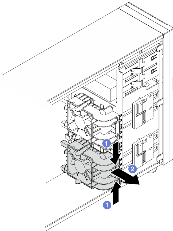
Рис. 24. Снятие переднего вентилятора компьютера
