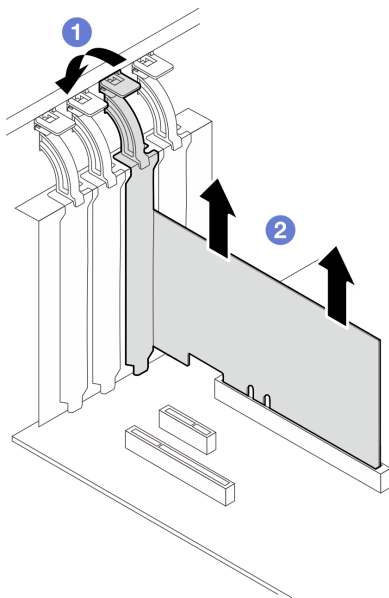
Рис. 58. Снятие адаптера PCIe
