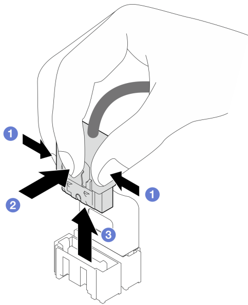
Рис. 5. Отсоединение кабеля от разъема дисководов для жесткого диска SATA
