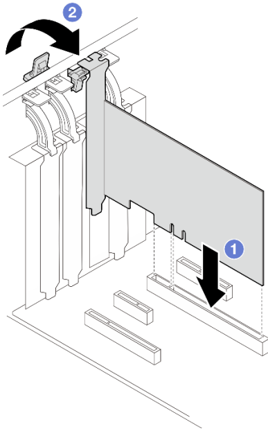
Рис. 59. Установка адаптера PCIe
