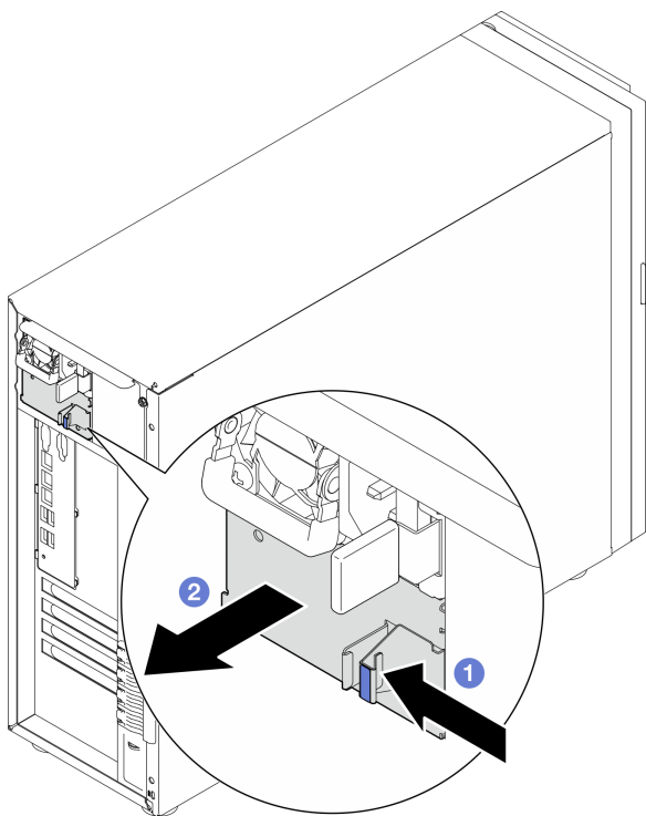
Рис. 71. Снятие заглушки оперативно заменяемого блока питания
