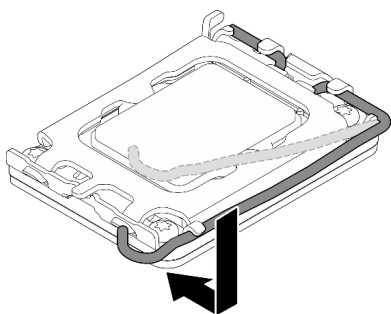
Рис. 75. Закрытие фиксатора процессора
