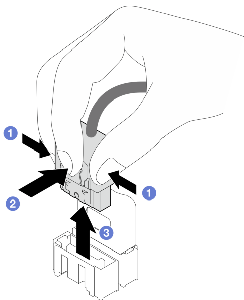
Рис. 8. Отсоединение кабеля от разъема дисководов для жесткого диска SATA
