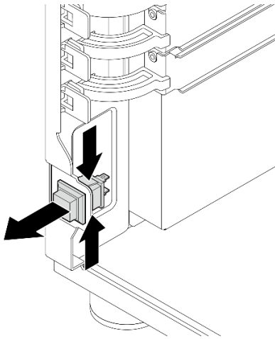
Рис. 37. Снятие датчика вмешательства
