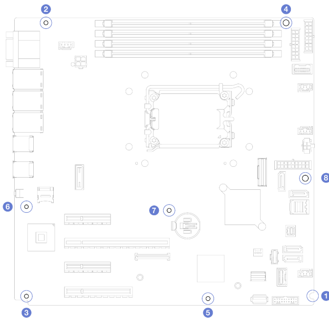
Рис. 88. Затяжка винтов для фиксации материнской платы
