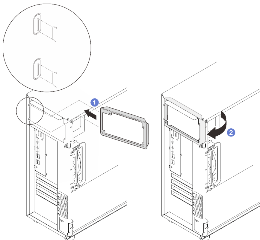
Рис. 66. Установка скобы стационарного блока питания
