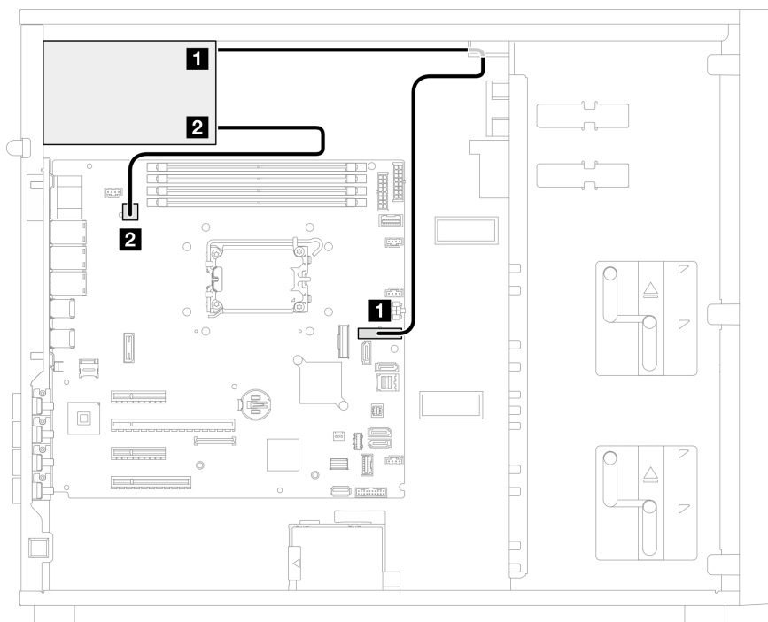
Рис. 102. Прокладка кабелей для стационарного блока питания
