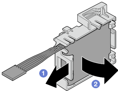
Рис. 78. Снятие модуля питания флеш-памяти RAID со скобы
