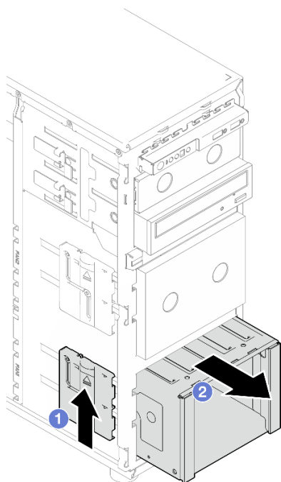
Рис. 3. Снятие отсека для диска
