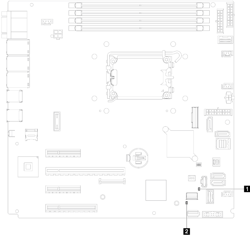
图 17. 主板 LED
