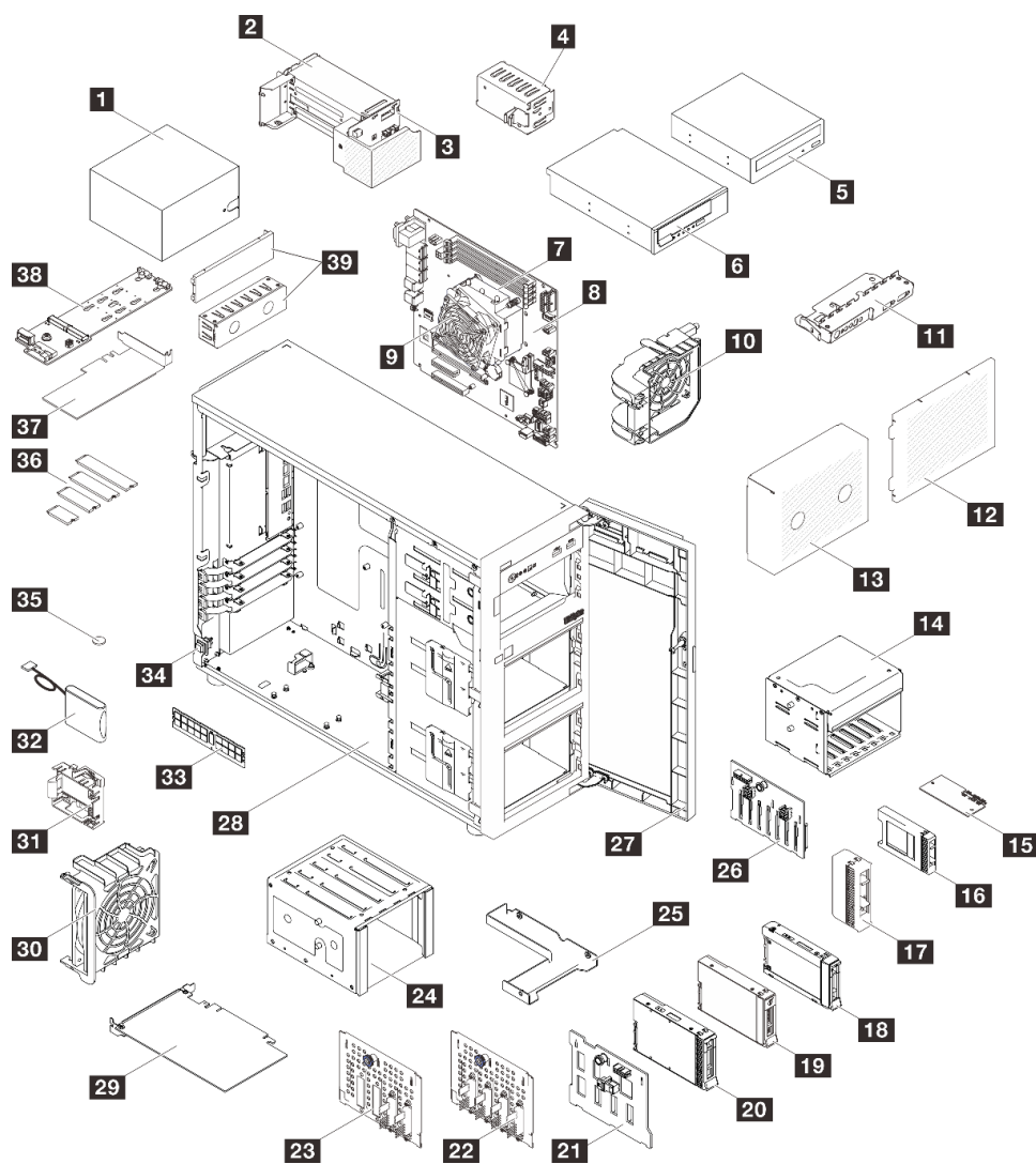
图 20. 服务器组件
