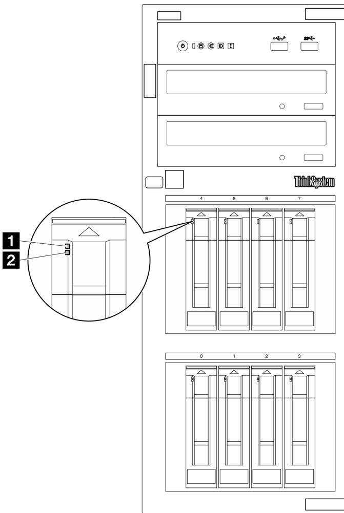
图 14. 硬盘 LED
