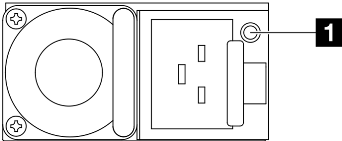
图 16. CRPS 电源模块 LED
