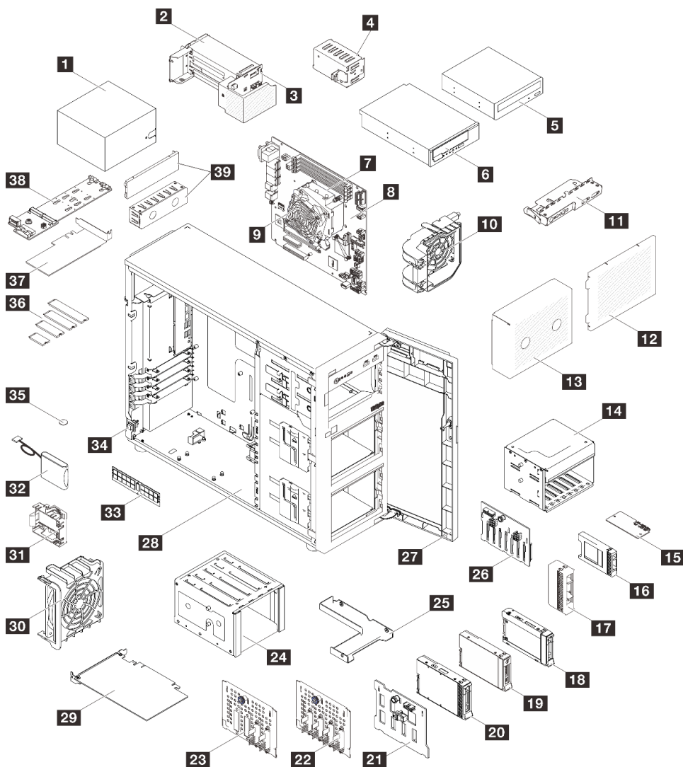
圖例 20. 伺服器元件
