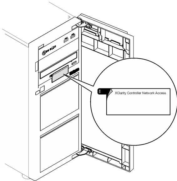
圖例 22. XClarity Controller 網路存取標籤的位置
