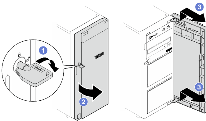
圖例 11. 前門鎖
