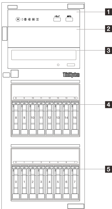
圖例 5. 配備十六個 2.5 吋熱抽換硬碟機槽的伺服器型號正面圖
