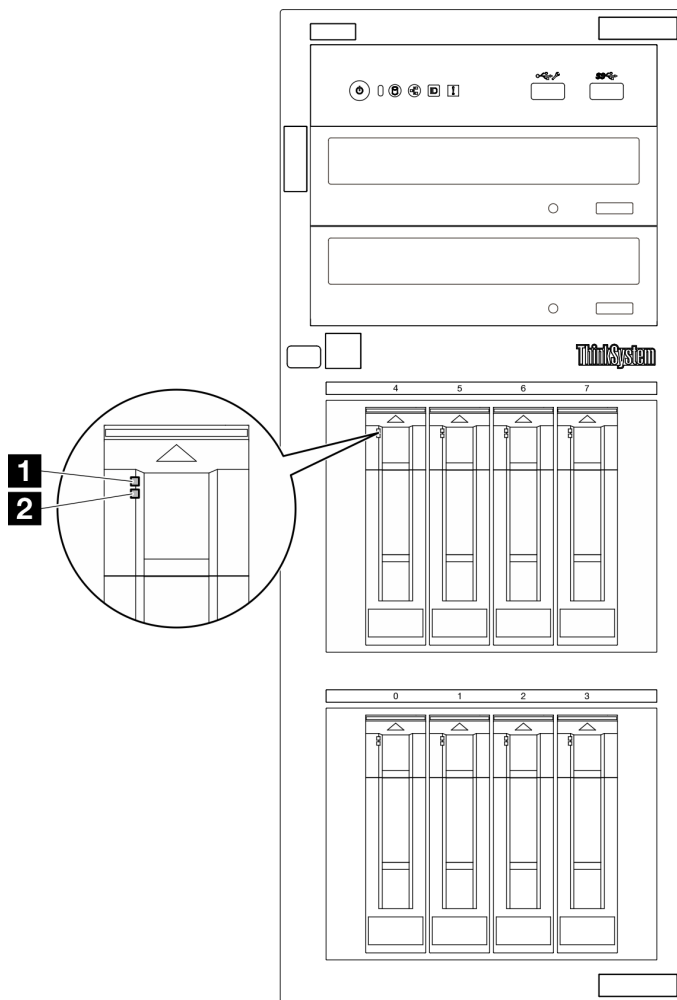
圖例 14. 硬碟 LED
