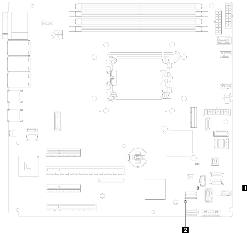
圖例 17. 主機板 LED
