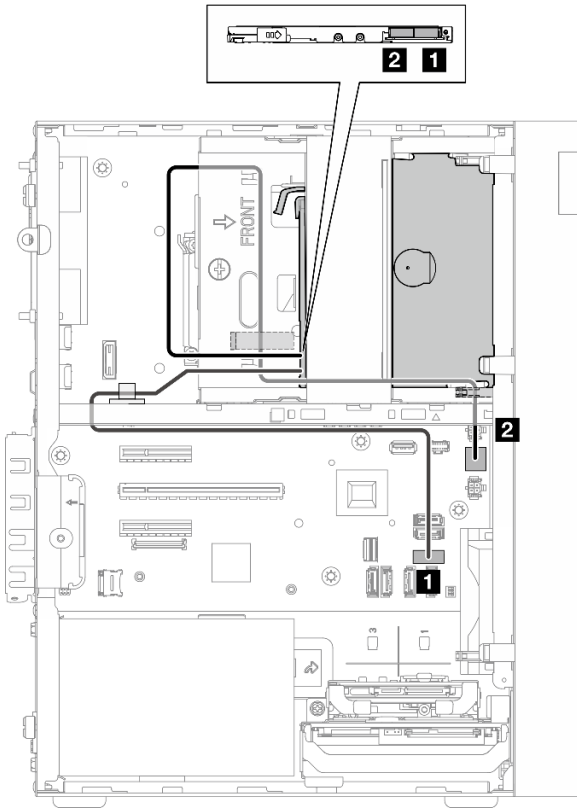
그림 124. 광 디스크 드라이브의 케이블 배선
