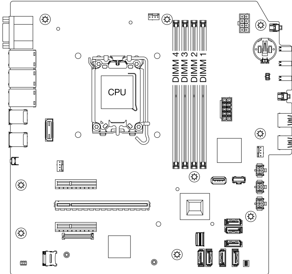
그림 89. 메모리 모듈 및 프로세서 레이아웃
