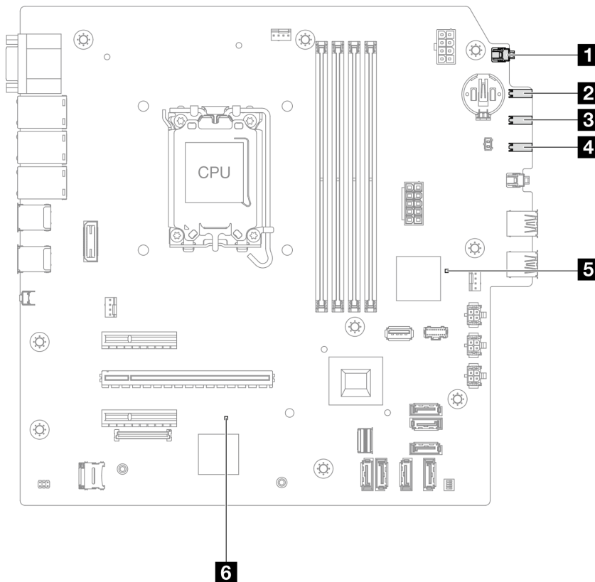
그림 137. 시스템 보드 LED
