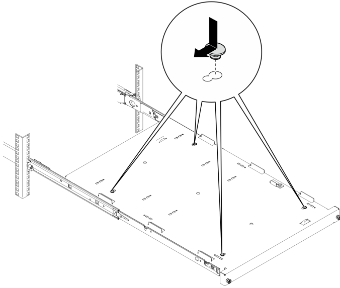
그림 17. 트레이에 고무 안전 패드 설치
