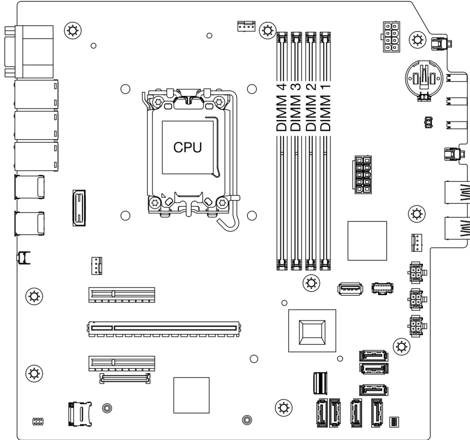
그림 86. 메모리 모듈 및 프로세서 레이아웃
