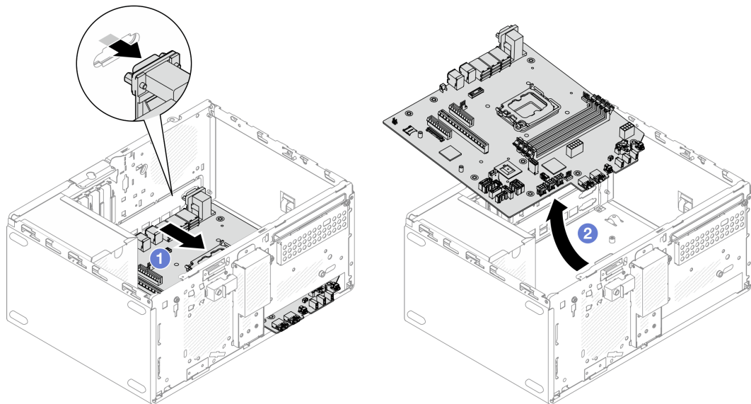
그림 109. 쉼시에서 시스템 보드 제거
