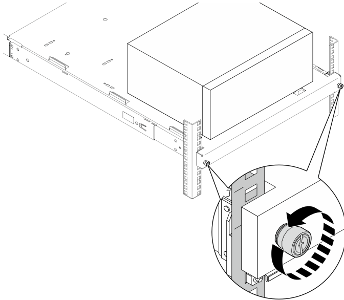
그림 14. 랙 캐비닛 앞면에서 나사 제거
