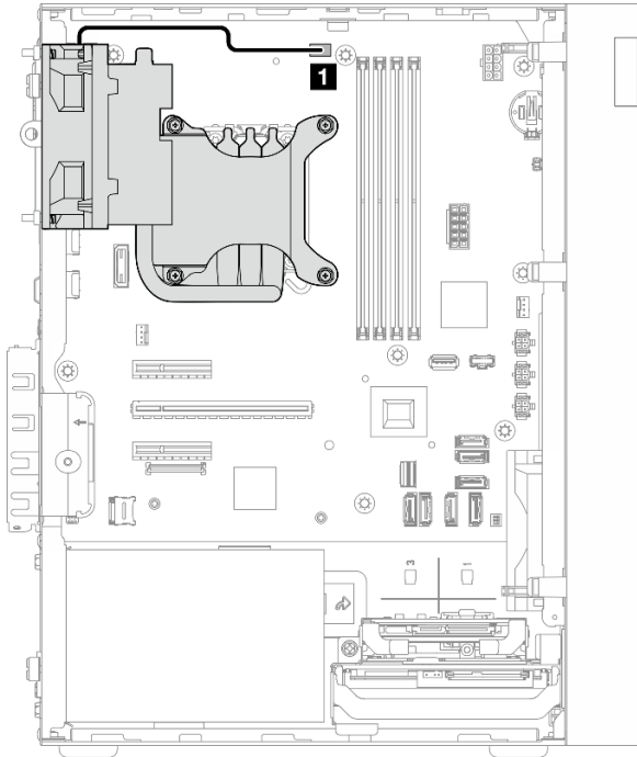
그림 132. 95W TDP가 장착된 프로세서용 방열판 및 팬 모듈의 케이블 배선
