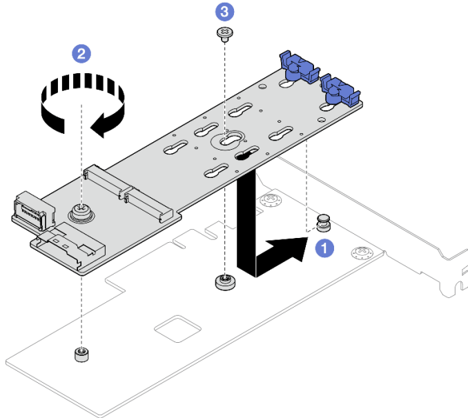
그림 80. PCIe 어댑터에 M.2 부트 어댑터 고정
