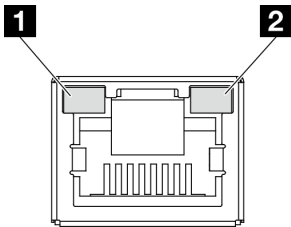
그림 138. XCC 시스템 관리 포트(10/100/1000Mbps RJ-45) LED
