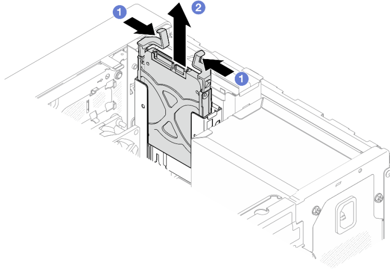
그림 25. 드라이브 베이 1에서 드라이브 어셈블리 제거
