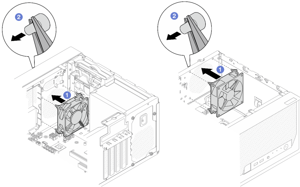
그림 64. 앞면 팬 또는 뒷면 팬 설치
