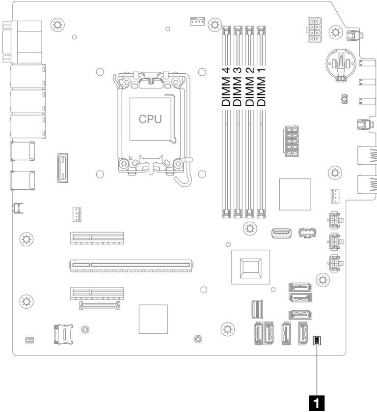
그림 8. 시스템 보드 스위치
