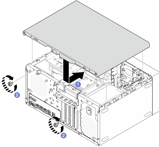
그림 117. 서버 덮개 설치
