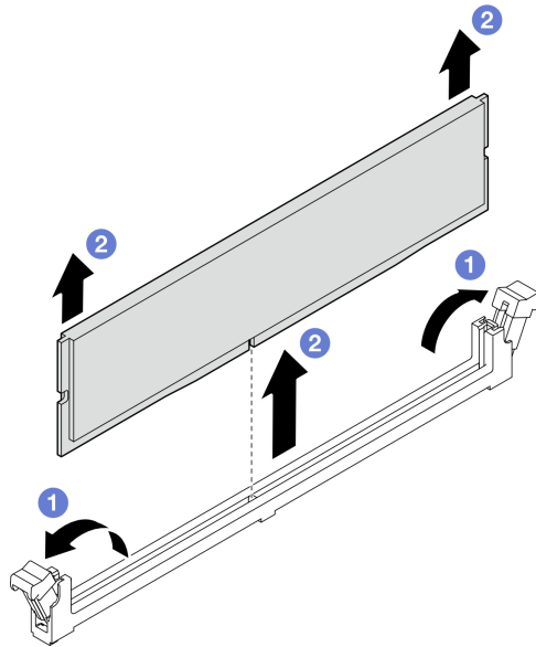
그림 88. 메모리 모듈 제거
