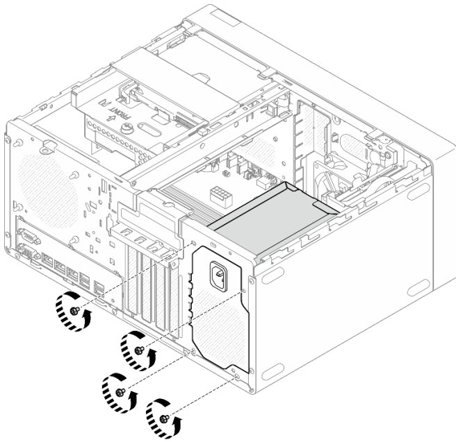
그림 96. 쉐시에 전원 공급 장치를 고정하는 나사 제거
