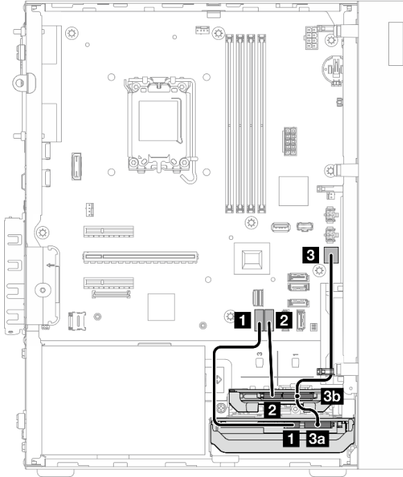
그림 121. 드라이브 베이 0 및 베이 1의 케이블 배선
