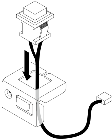
그림 75. 침입 스위치 조립
