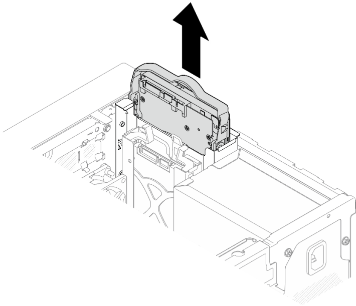
그림 24. 드라이브 베이 0에서 드라이브 어셈블리 제거
