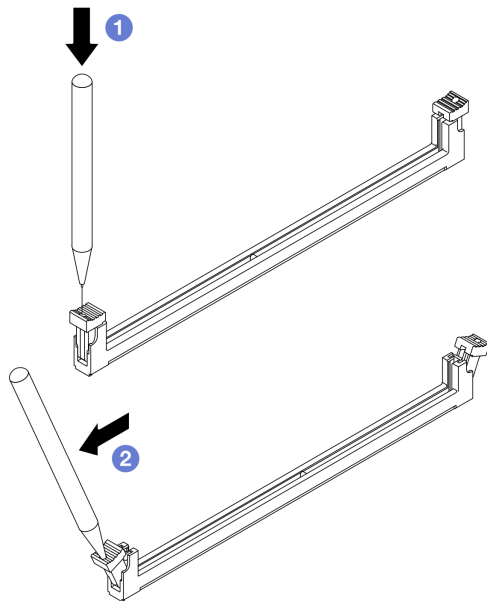
그림 90. 고정 클립 열기
