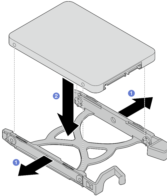
그림 30. 고정장치에 2.5인치 드라이브 설치
