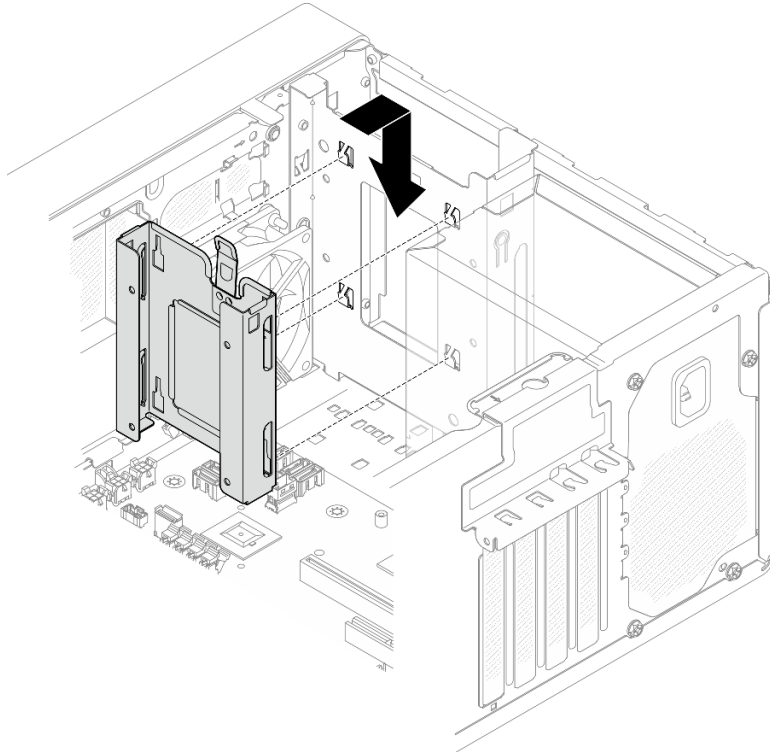
그림 38. 드라이브 베이 1 케이지 설치
