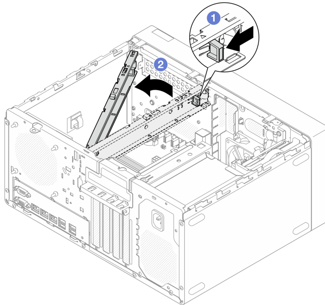
그림 115. 케이스 바 제거
