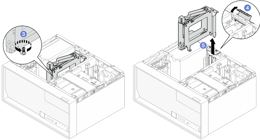
그림 50. PCIe 슬롯 3에서 3.5인치 드라이브 케이스 제거
