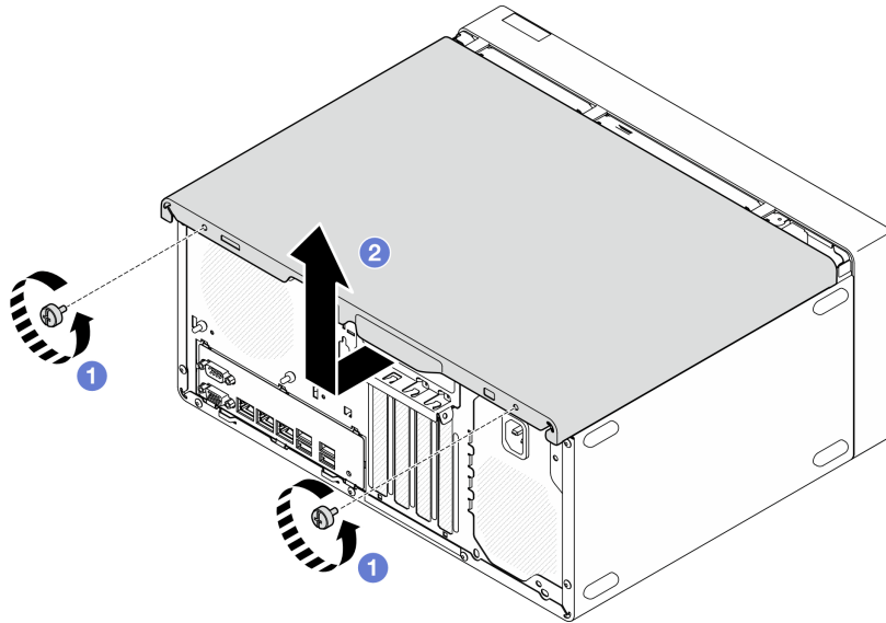
그림 114. 서버 덮개 제거
