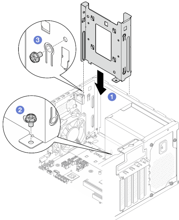
그림 36. 베이 0에 드라이브 케이지 설치
