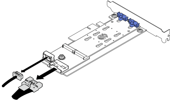
그림 77. 전원 및 신호 케이블 분리
