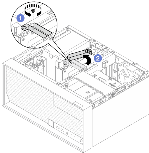
그림 49. 드라이브 케이징 3의 래치 해제
