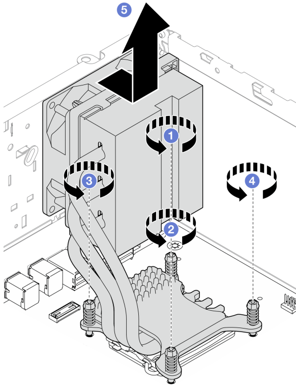
그림 70. 95W TDP가 장착된 프로세서용 방열판 및 팬 모듈의 나사 풀기
