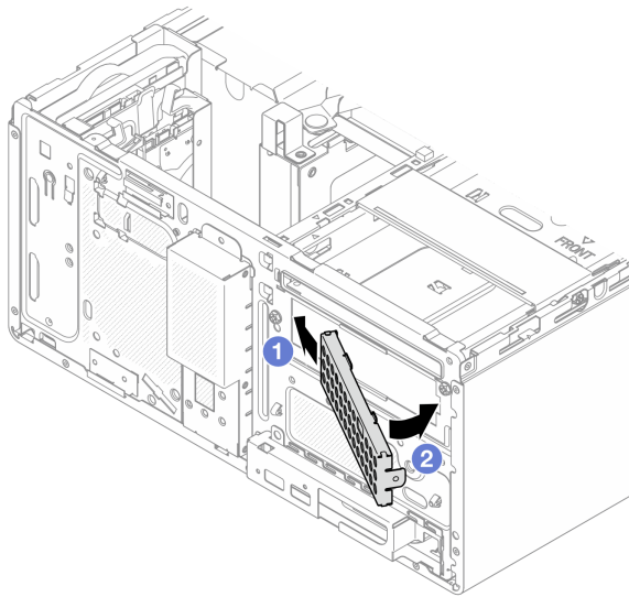
그림 44. EMI 실딩 설치
