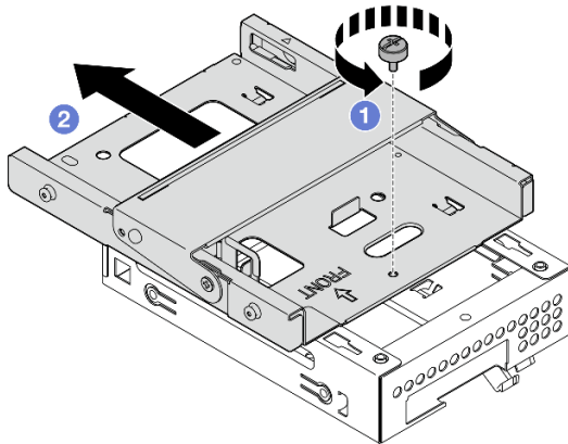
그림 43. 광 드라이브 케이스에 3.5인치 드라이브 케이스 제거
