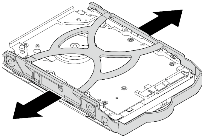
그림 26. 고정장치에서 3.5인치 드라이브 제거
