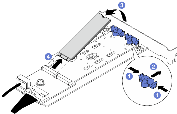
그림 82. M.2 드라이브 제거
