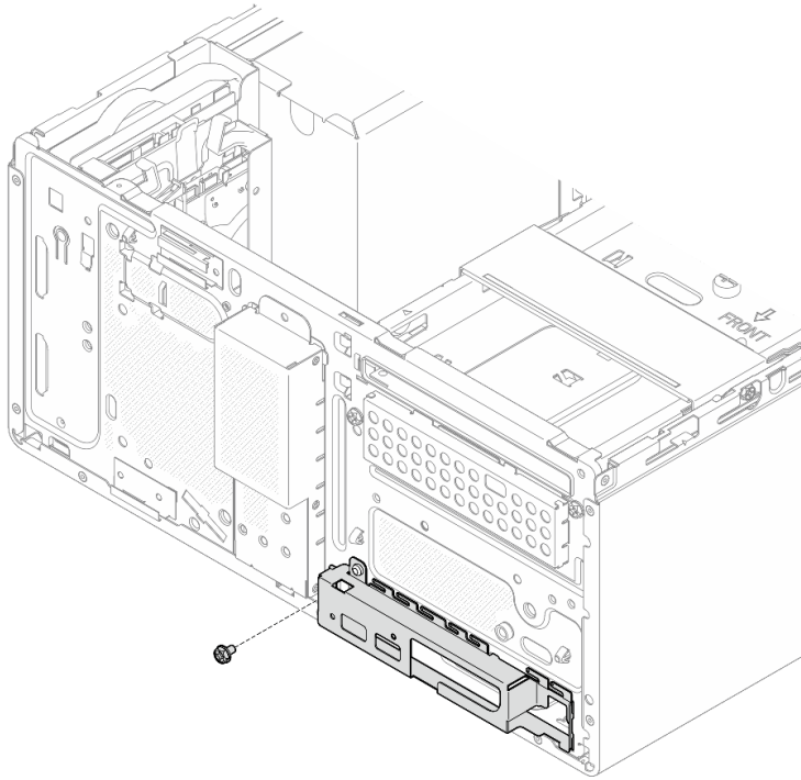
그림 139. 앞면 I/O 브래킷을 새시에 고정하는 나사를 제거합니다
