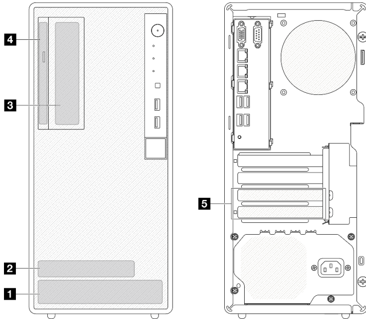
그림 23. 드라이브 베이 위치
