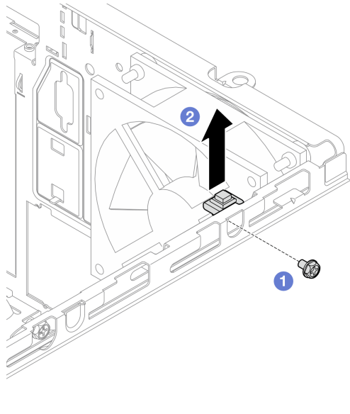
그림 74. 침입 스위치 제거
