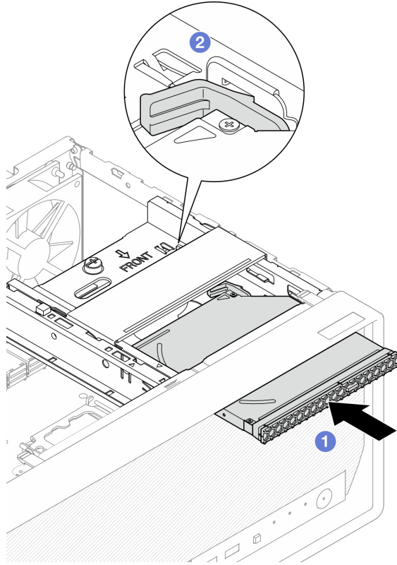
그림 60. 광 드라이브 설치
