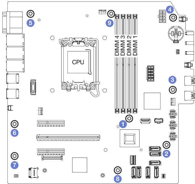
그림 108. 시스템 보드 나사 제거 순서
