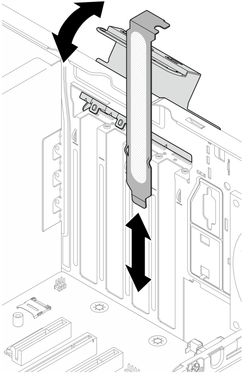
그림 93. PCIe 어댑터 브래킷 설치
