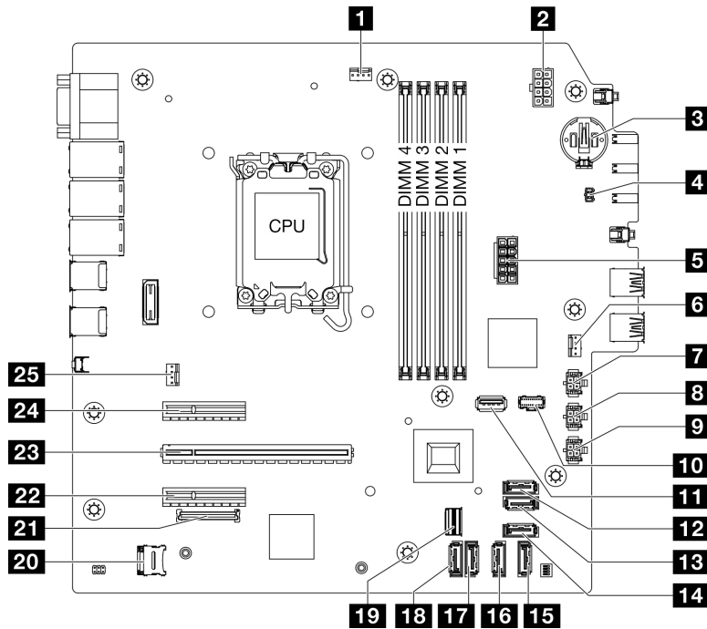
그림 7. 시스템 보드 커넥터
