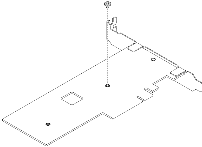
그림 79. PCIe 어댑터 뒷면의 나사 제거
