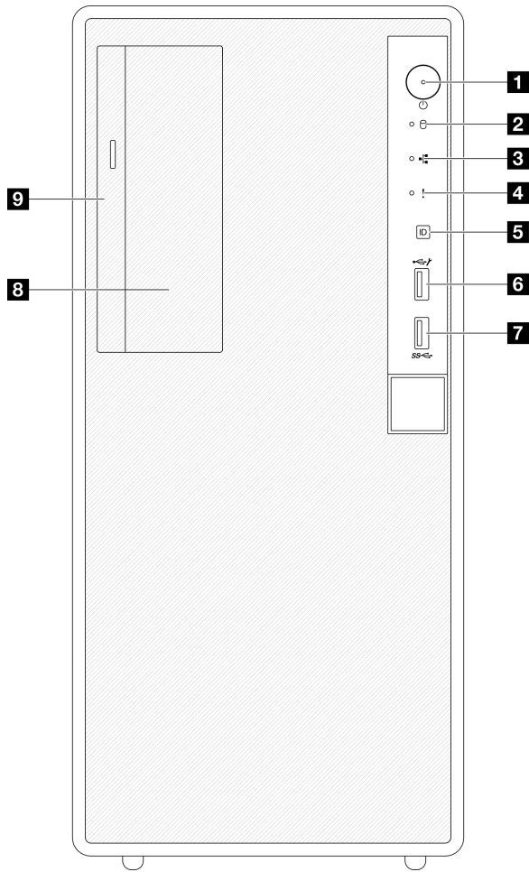
그림 2. 서버 구성 요소의 앞면 보기
