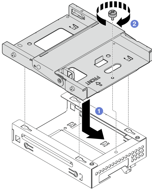
그림 45. 광 드라이브 케이스에 3.5인치 드라이브 케이스 설치
