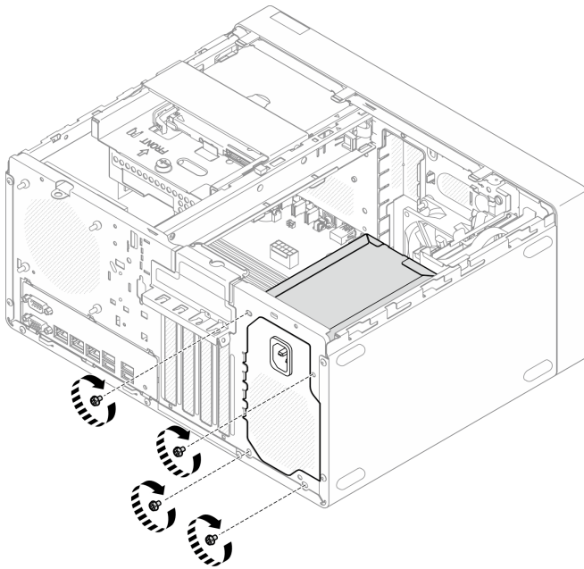
그림 99. 새시에 전원 공급 장치 고정
