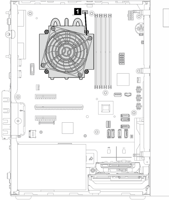
그림 131. 95W 미만의 TDP가 장착된 프로세서용 방열판 및 팬 모듈의 케이블 배선
