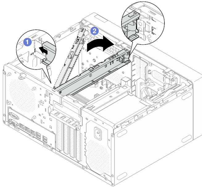
그림 116. 케이지 바 설치
