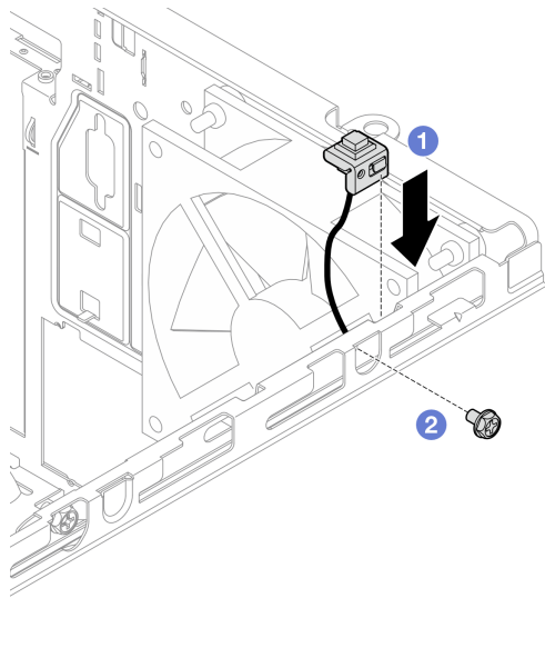
그림 76. 침입 스위치 설치
