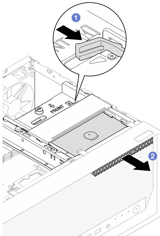
그림 53. 광 드라이브 제거
