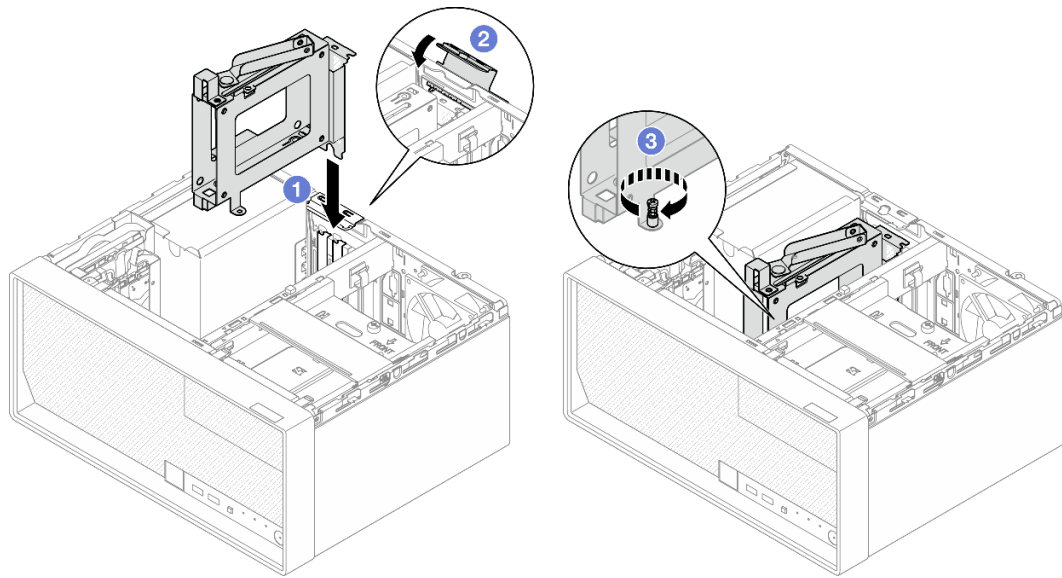
그림 51. PCIe 슬롯 3에 드라이브 케이스 설치
