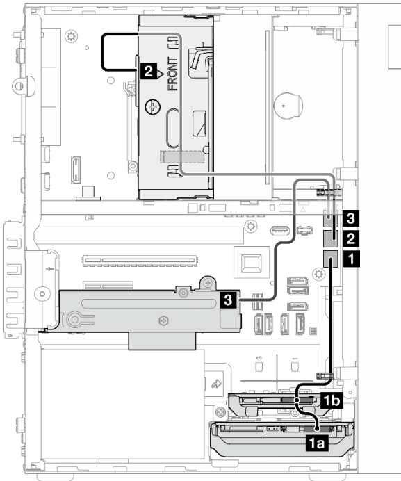
그림 127. 전원 케이블 배선
