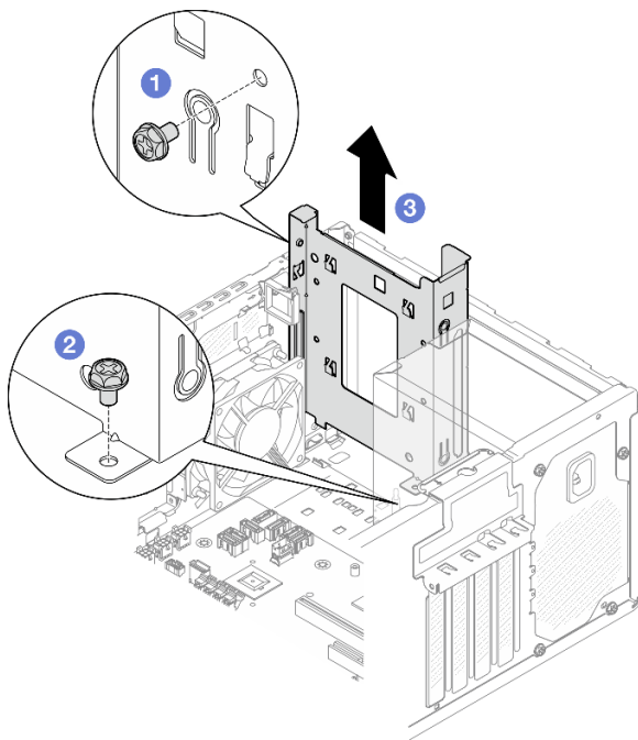
그림 35. 드라이브 베이 0에서 드라이브 캐이지 제거
