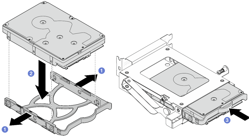
그림 48. 드라이브 케이스에 3.5인치 드라이브 설치
