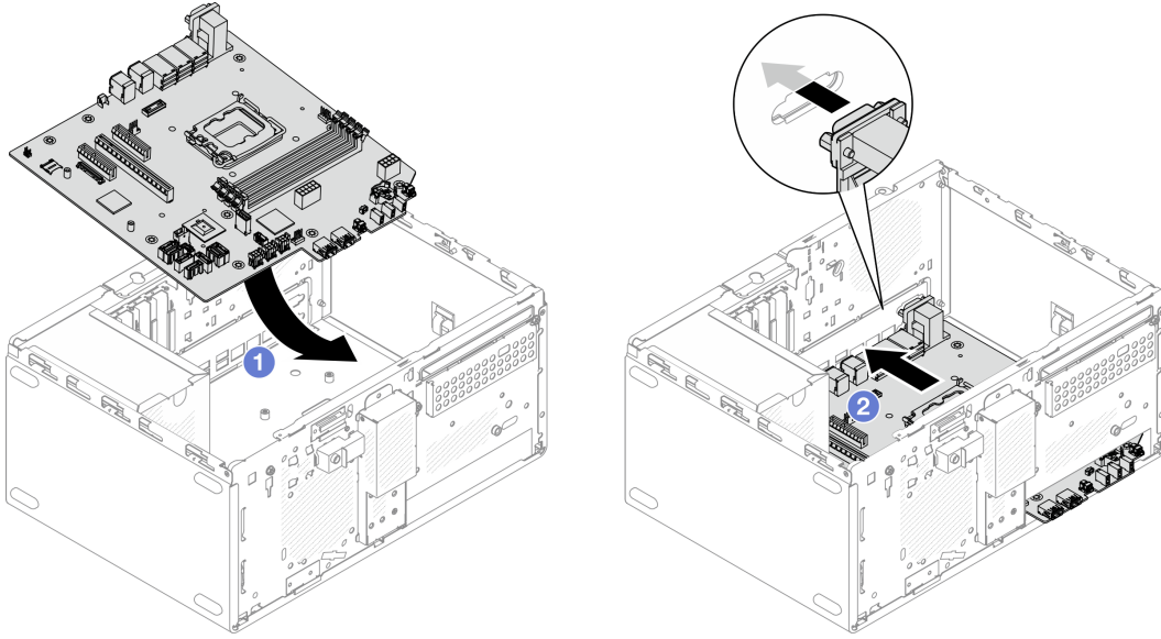
그림 110. 새시에 시스템 보드 설치
