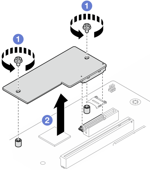
그림 104. 펌웨어 및 RoT 보안 모듈 제거
