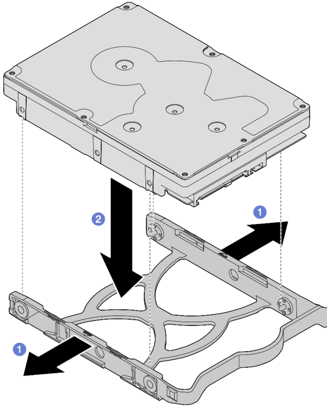
그림 29. 고정장치에 3.5인치 드라이브 설치
