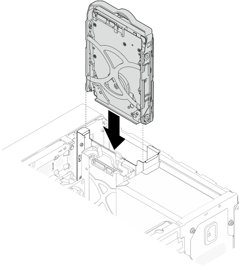
그림 31. 드라이브 베이 0에 3.5인치 드라이브 어셈블리 설치
