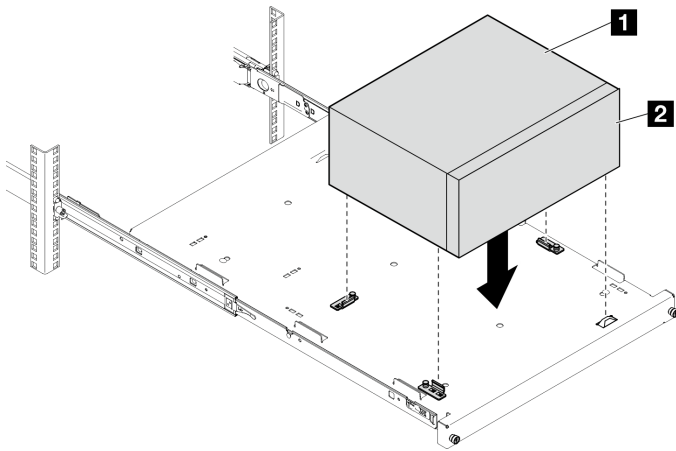
그림 18. 트레이에 서버 설치
