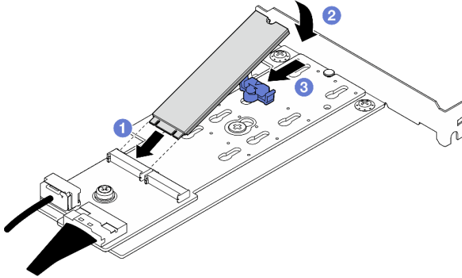
그림 85. M.2 드라이브 설치
