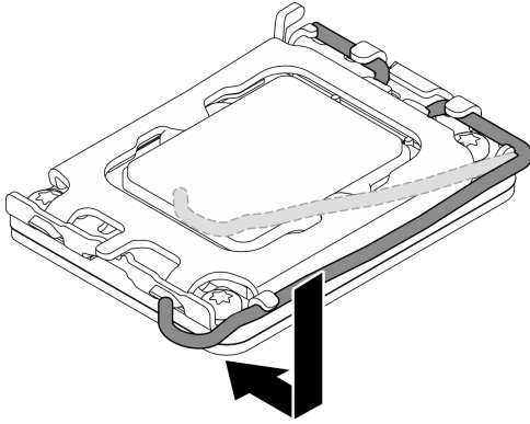
그림 103. 프로세서 고정장치 닫기
