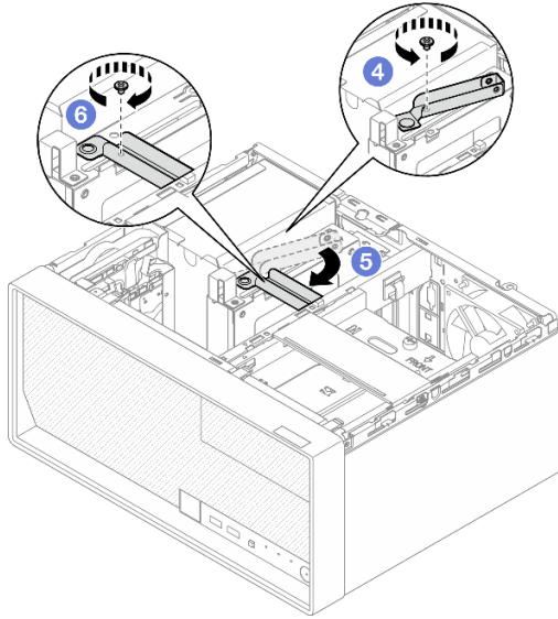
그림 52. PCIe 슬롯 3에 드라이브 케이지 고정
