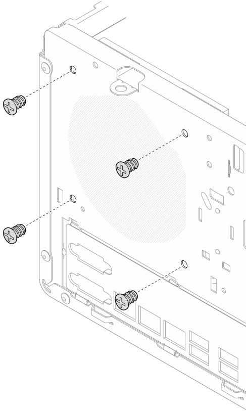
그림 68. 방열판 팬을 새시에 고정하는 나사 4개 제거
