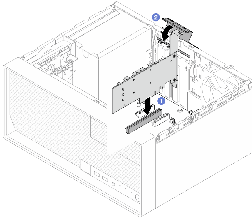
그림 95. PCIe 어댑터 설치
