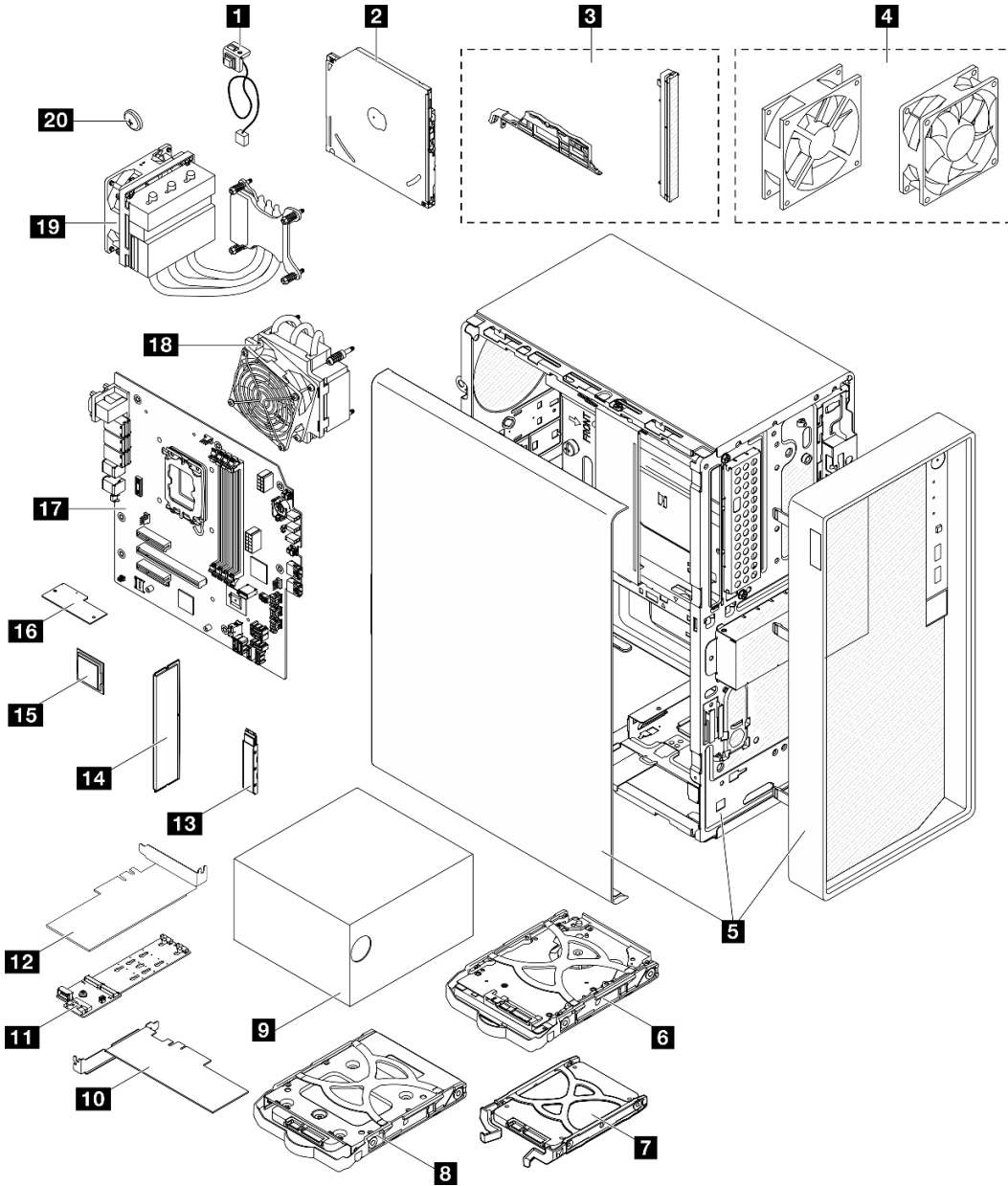
그림 9. 서버 구성 요소
