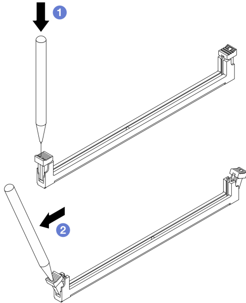
그림 87. 고정 클립 열기
