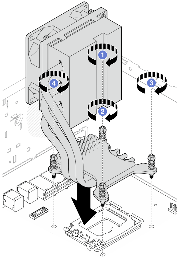
그림 72. 95W TDP가 장착된 프로세서용 방열판 및 팬 모듈의 나사 조이기
