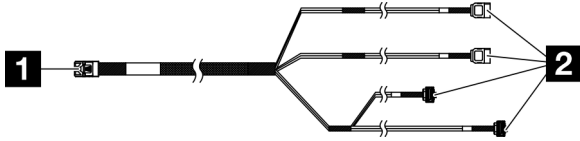
그림 126. Mini SAS HD X4 Vertical to VT SATA 7P x2 + RA SATA 7P x2 cable
