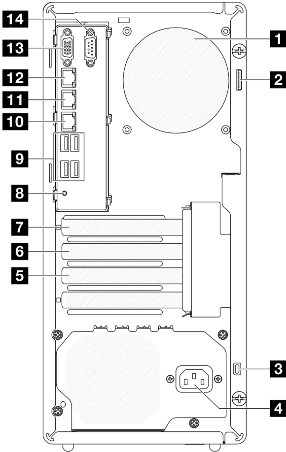
그림 3. 뒷면 보기
