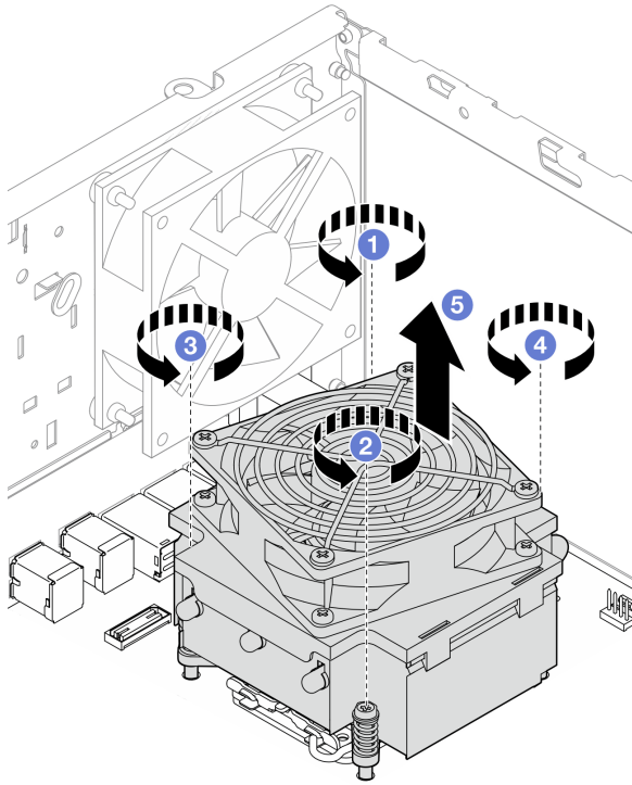
그림 69. 95W 미만의 TDP가 장착된 프로세서용 방열판 및 팬 모듈의 나사 풀기
