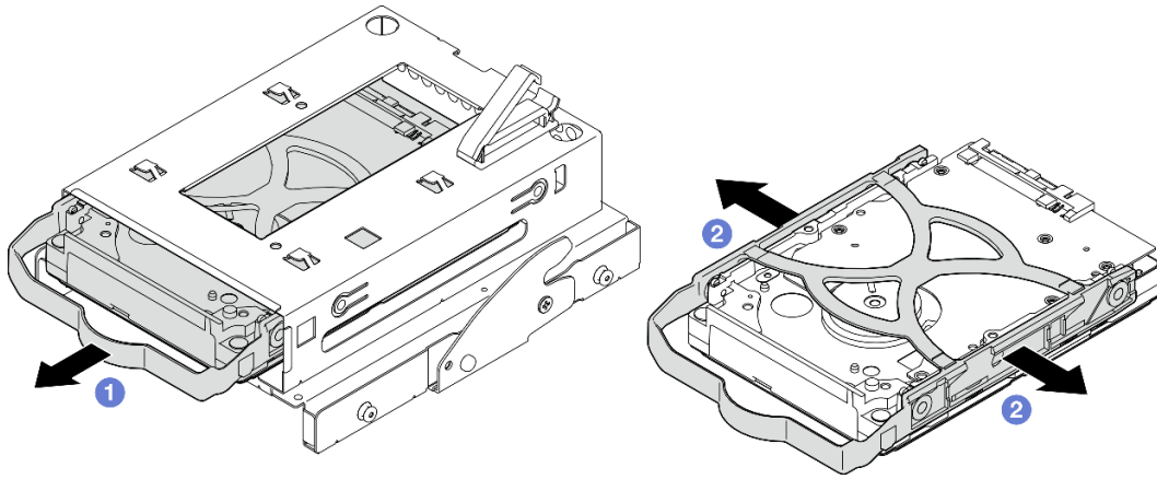
그림 39. 3.5인치 드라이브 어셈블리 제거
