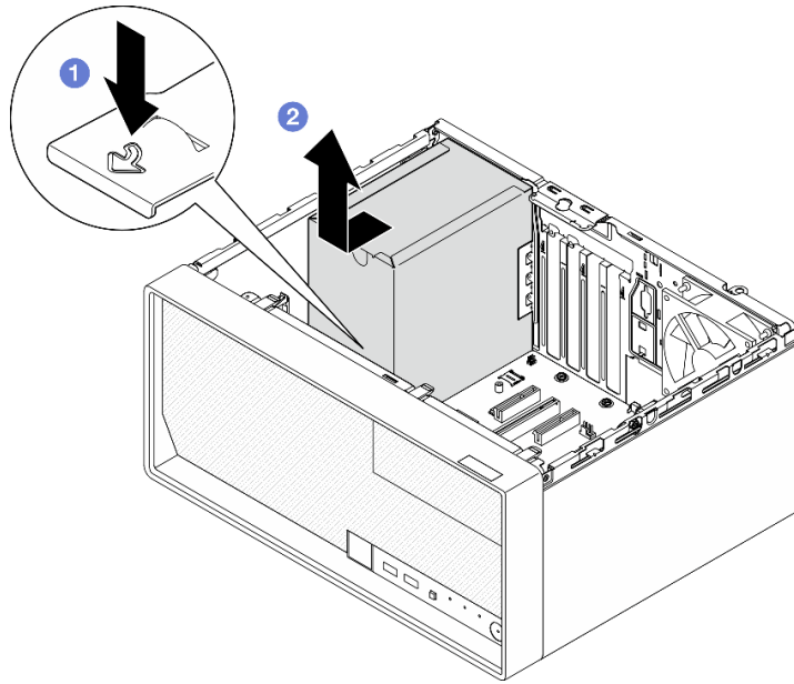
그림 97. 전원 공급 장치 제거
