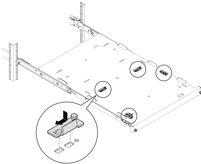
그림 16. 트레이에 브래킷 설치
