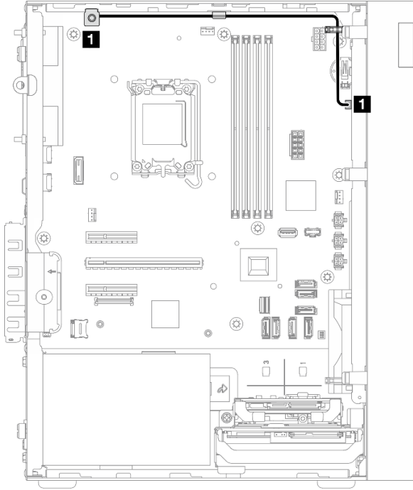
그림 133. 침입 스위치의 케이블 배선
