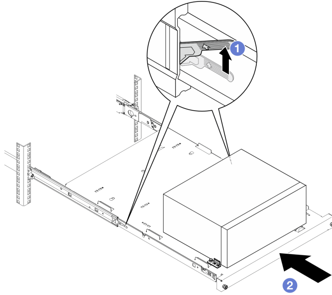
그림 19. 랙 캐비닛에 서버 설치
