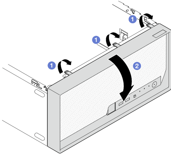
그림 34. 앞면 베젤 제거
