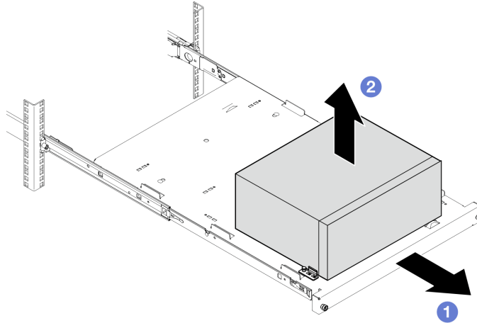
그림 15. 레일에서 서버 제거
