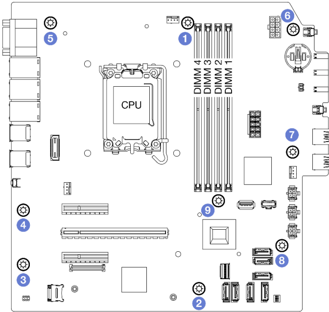
그림 111. 새시에 시스템 보드 설치
