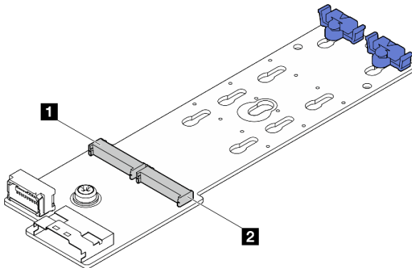
그림 84. M.2 드라이브 슬롯
