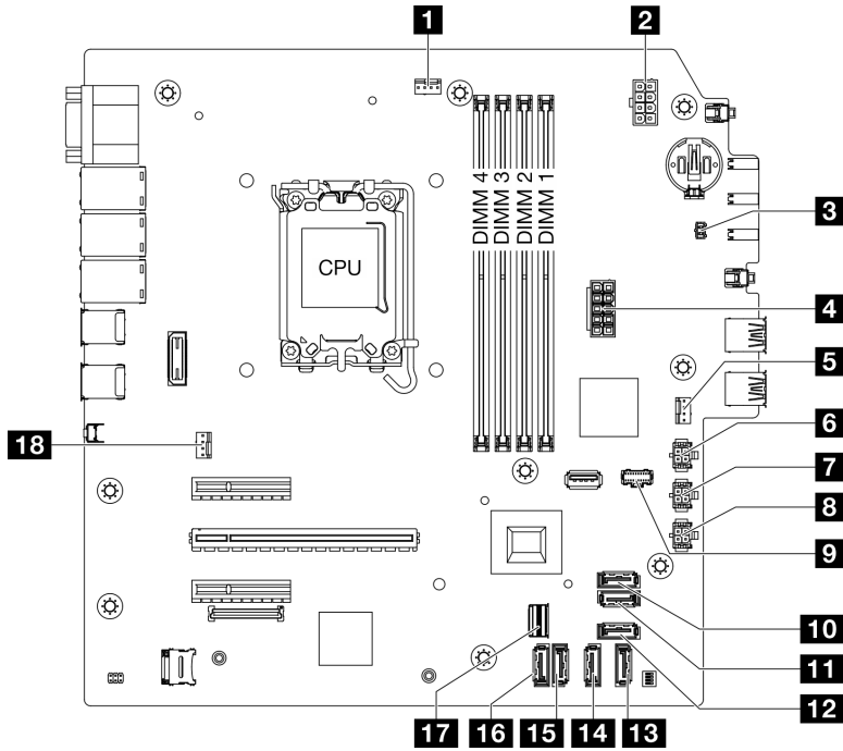
그림 120. 시스템 보드 커넥터
