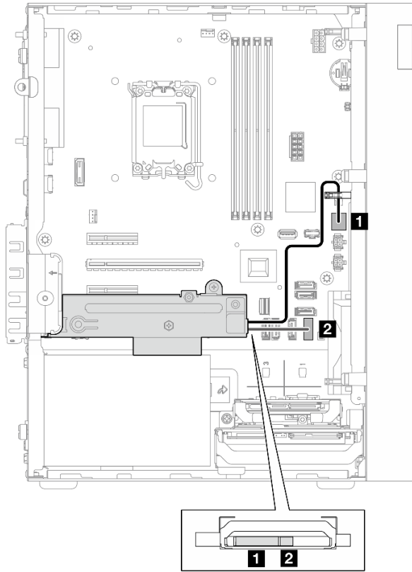
그림 123. 드라이브 베이 3의 케이블 배선
