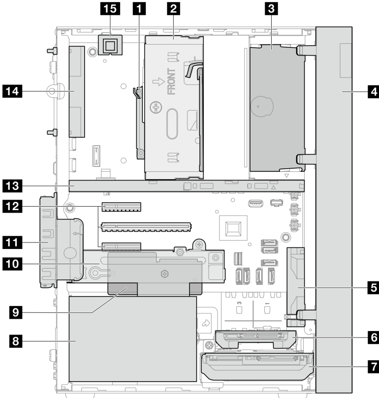
그림 4. 측면 보기
