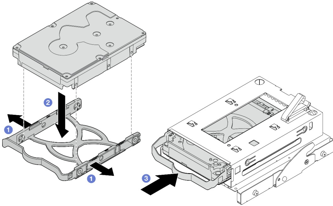
그림 41. 드라이브 케이스에 3.5인치 드라이브 설치
