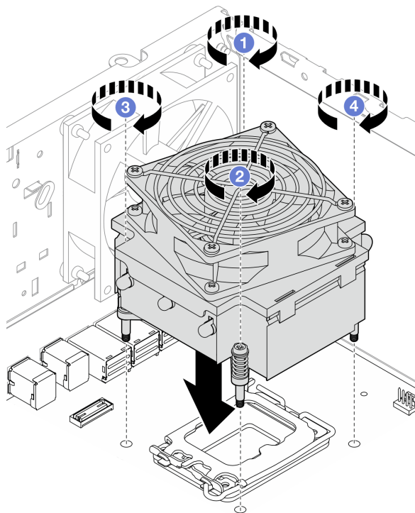
그림 71. 95W 미만의 TDP가 장착된 프로세서용 방열판 및 팬 모듈의 나사 조이기
