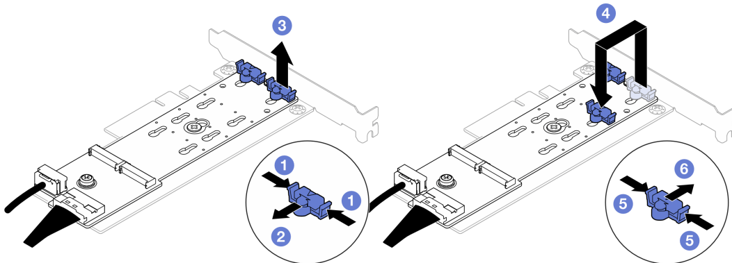
그림 83. M.2 고정장치 조정
