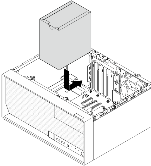
그림 98. 새시에 전원 공급 장치 설치
