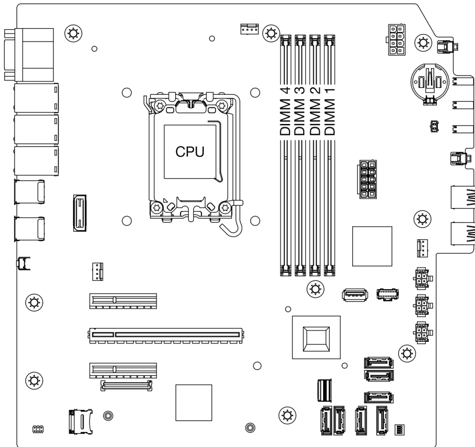
그림 13. 메모리 모듈 및 프로세서 레이아웃
