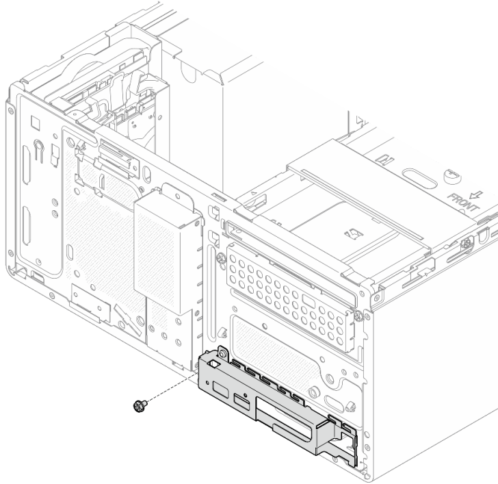
그림 106. 앞면 I/O 브래킷을 새시에 고정하는 나사를 제거합니다
