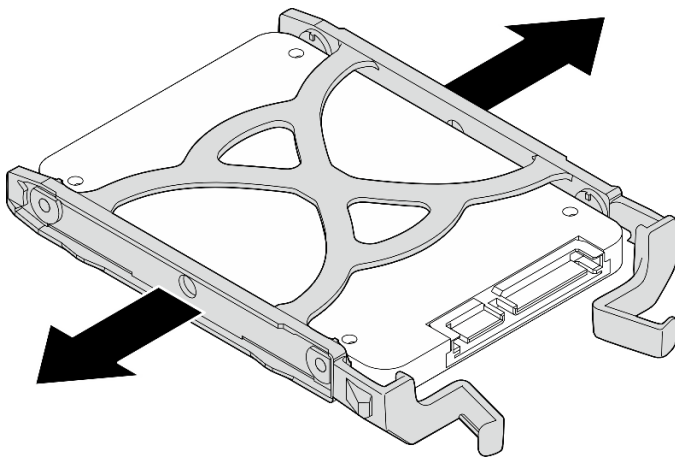
그림 27. 고정장치에서 2.5인치 드라이브 제거
