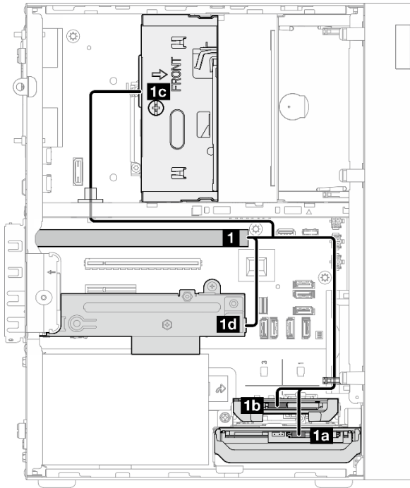
그림 128. 신호 케이블 배선
