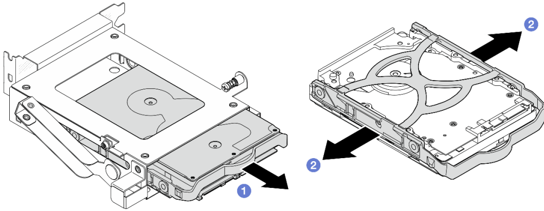
그림 46. 3.5인치 드라이브 어셈블리 제거
