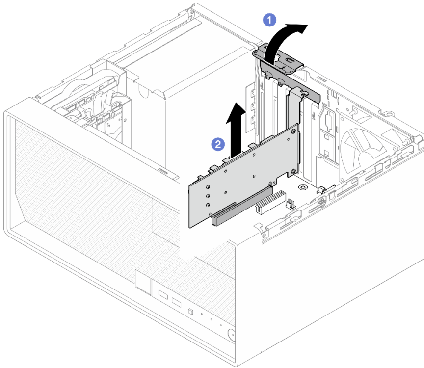
그림 92. PCIe 어댑터 제거
