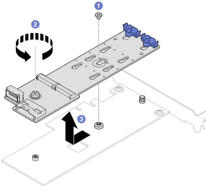
그림 78. M.2 부트 어댑터 제거
