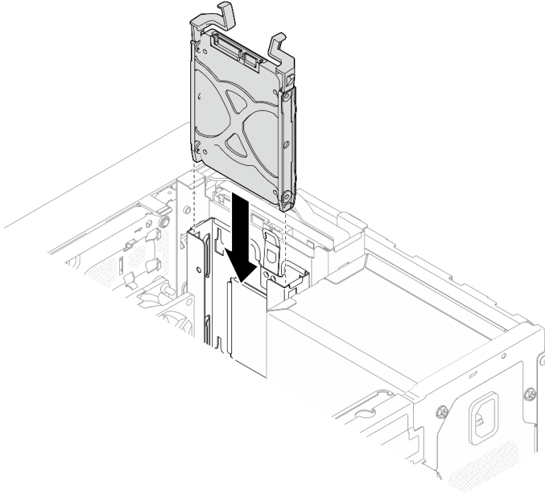
그림 32. 드라이브 베이 1에 2.5인치 드라이브 어셈블리 설치
