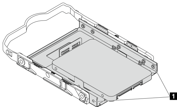
그림 42. 고정장치의 드라이브 나사 구멍 배치
