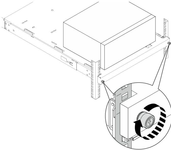
그림 20. 나사로 트레이 고정
