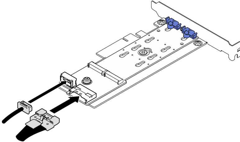
그림 81. M.2 전원 및 신호 케이블 설치
