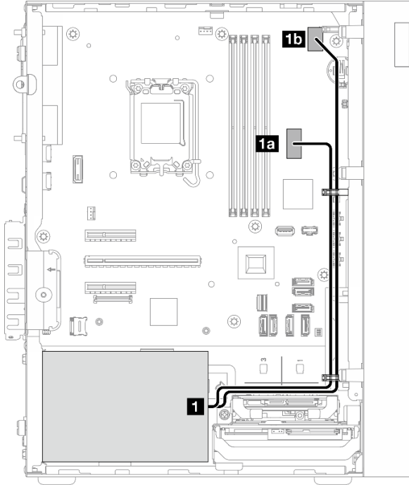
그림 129. PSU의 케이블 배선
