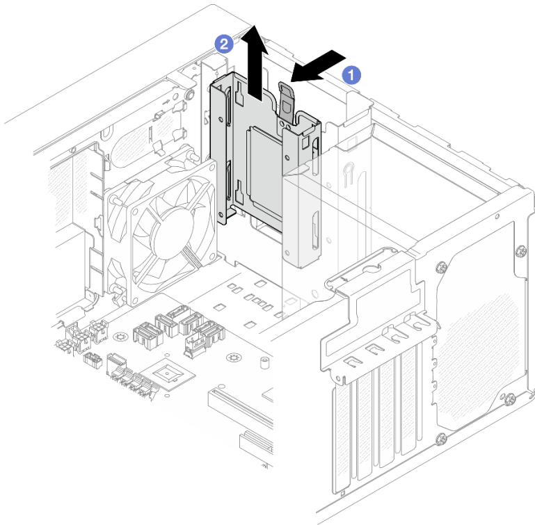
그림 33. 드라이브 베이 1에서 드라이브 케이스 제거
