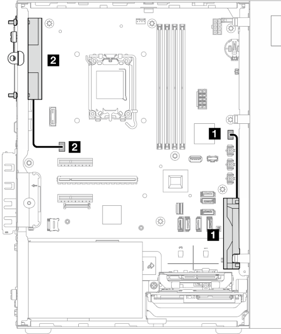
그림 130. 앞면 팬 및 뒷면 팬의 케이블 배선
