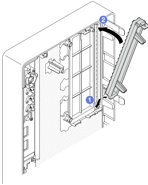
그림 56. 광 드라이브 베이 실드 설치
