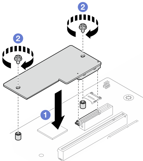
그림 105. 펌웨어 및 RoT 보안 모듈 설치
