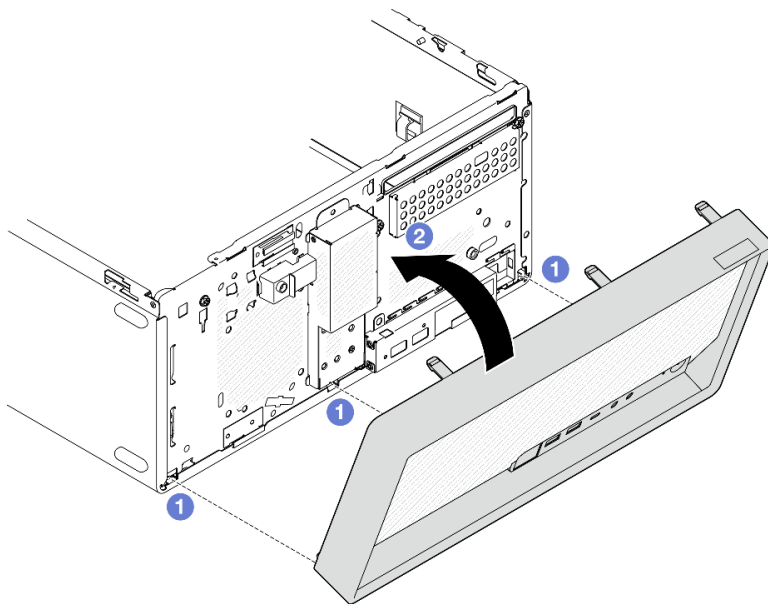
그림 37. 앞면 베젤 설치
