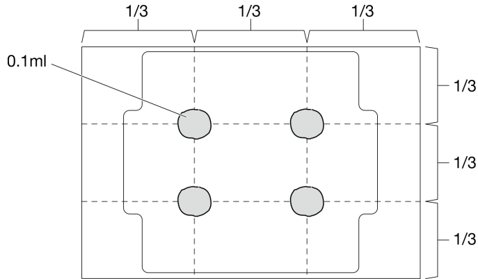
그림 101. 열 그리스의 적절한 형태
