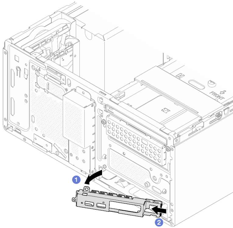
그림 140. 새시에서 앞면 I/O 브래킷 제거
