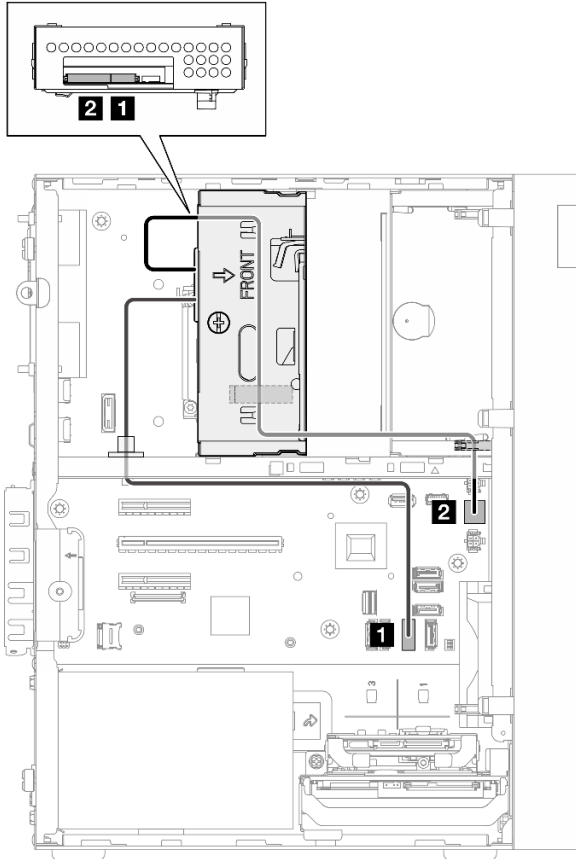
그림 122. 드라이브 베이 2의 케이블 배선
