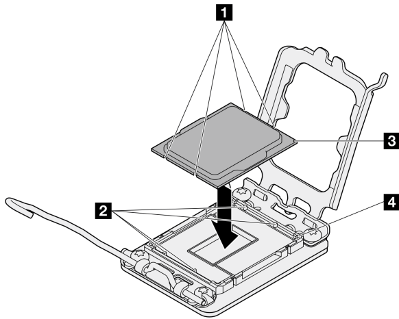
그림 102. 프로세서 설치
