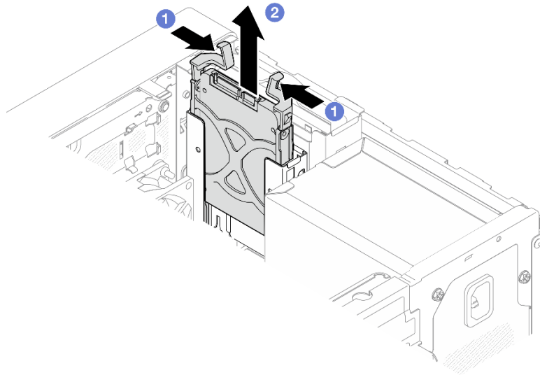
Рис. 13. Извлечение блока диска из отсека для диска 1
