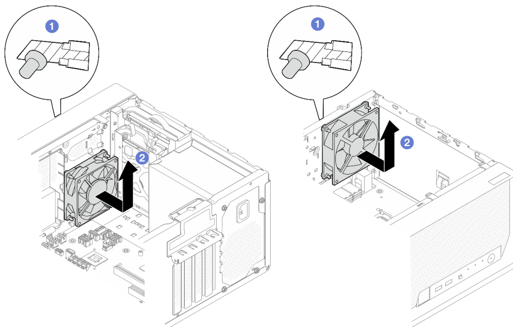
Рис. 51. Снятие переднего или заднего вентилятора
