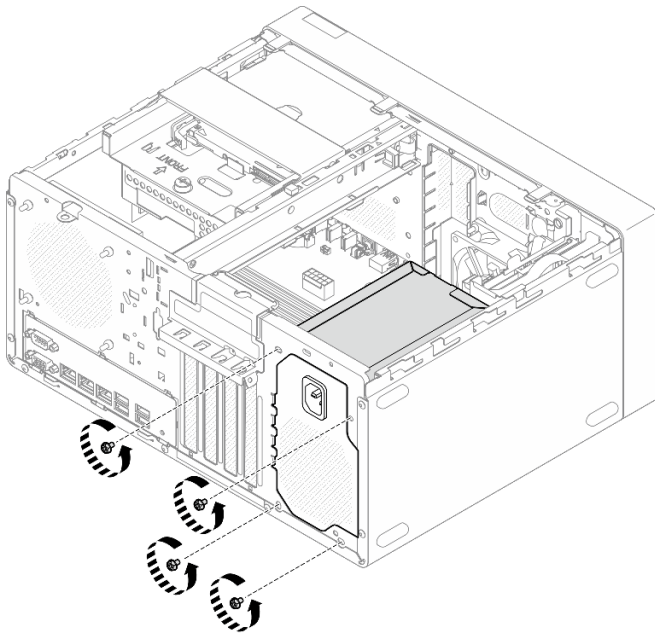
Рис. 84. Снятие винтов, фиксирующих модуль блока питания на раме
