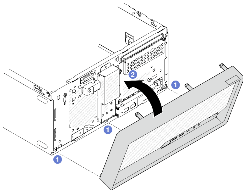
Рис. 25. Установка лицевой панели
