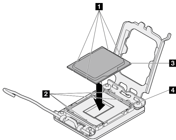
Рис. 90. Установка процессора
