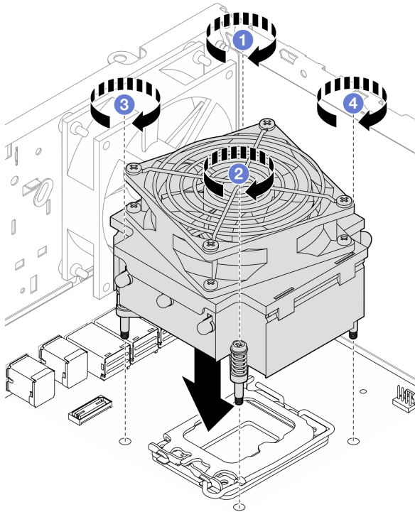
Рис. 59. Затягивание винтов на модуле радиатора и вентилятора для процессора с величиной отвода тепловой мощности менее 95 Вт
