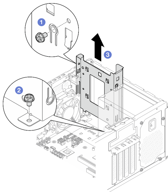
Рис. 23. Извлечение отсека для диска из отсека 0
