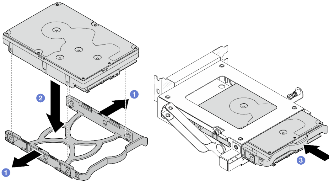
Рис. 36. Установка 3,5-дюймового диска в отсек для диска
