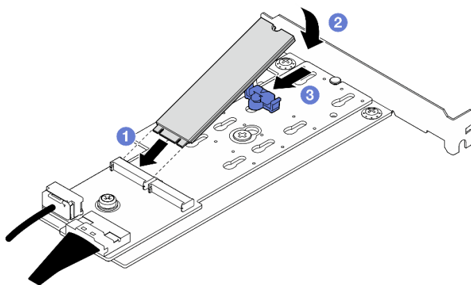
Рис. 73. Установка диска M.2
