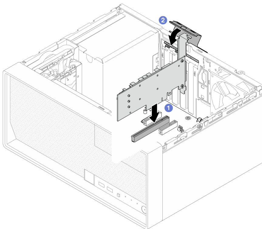
Рис. 83. Установка адаптера PCIe
