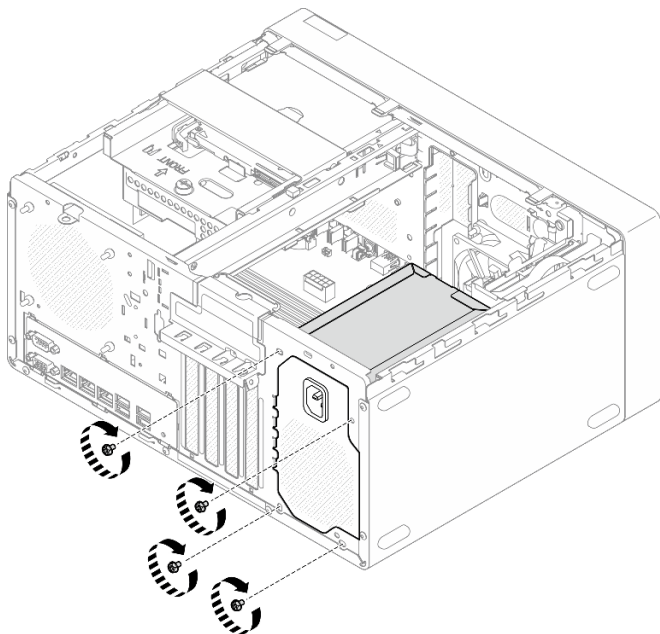
Рис. 87. Фиксация модуля блока питания на раме
