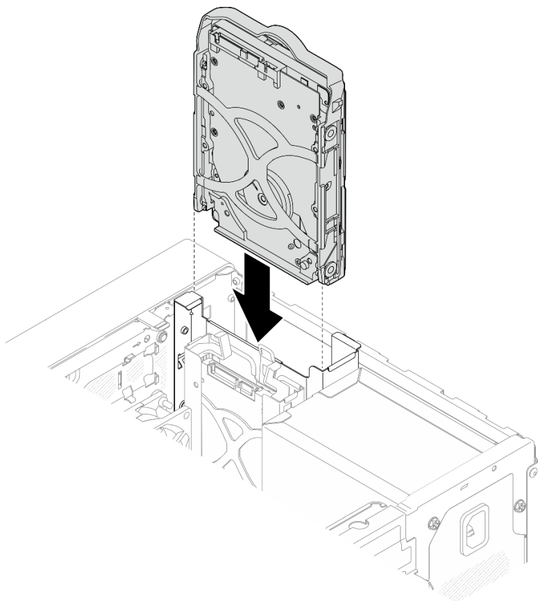
Рис. 19. Установка блока 3,5-дюймового диска в отсек для диска 0
