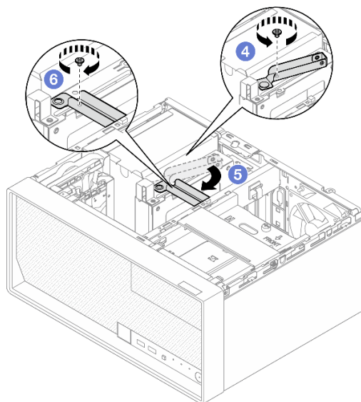
Рис. 40. Фиксация отсека для диска в гнезде PCIe 3
