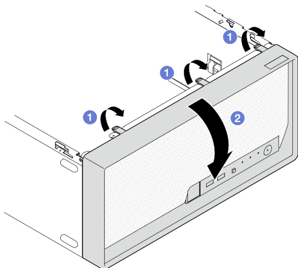
Рис. 22. Снятие лицевой панели
