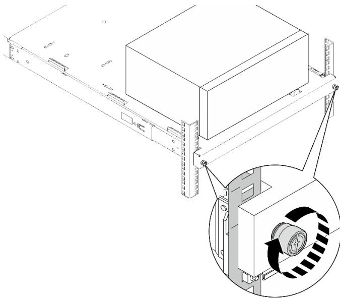
Рис. 8. Фиксация лотка винтами
