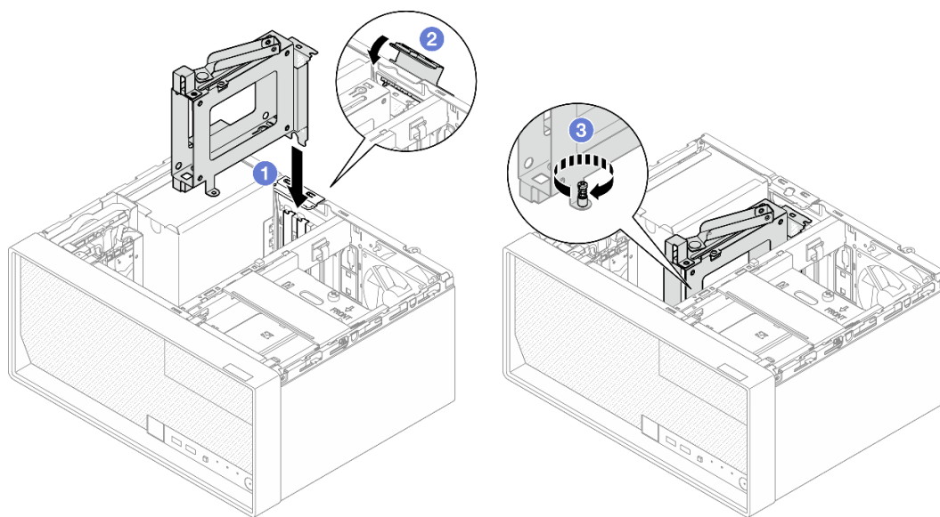
Рис. 39. Установка отсека для диска в гнездо PCIe 3
