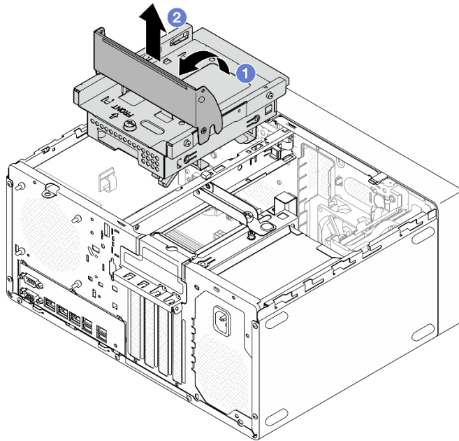
Рис. 49. Снятие отсека дисководов для оптических дисков
