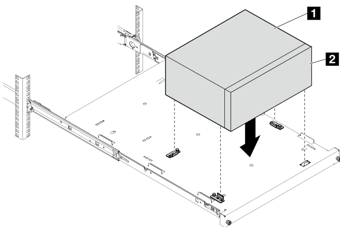
Рис. 6. Установка сервера на лоток
