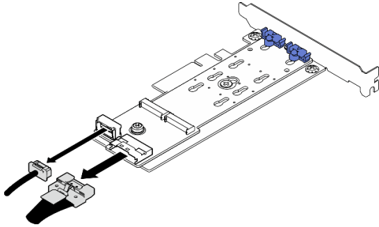
Рис. 65. Отключение кабеля питания и сигнального кабеля
