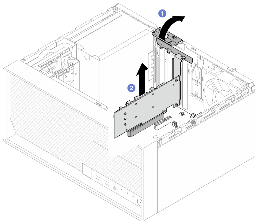
Рис. 80. Снятие адаптера PCIe
