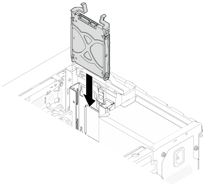
Рис. 20. Установка блока 2,5-дюймового диска в отсек для диска 1
