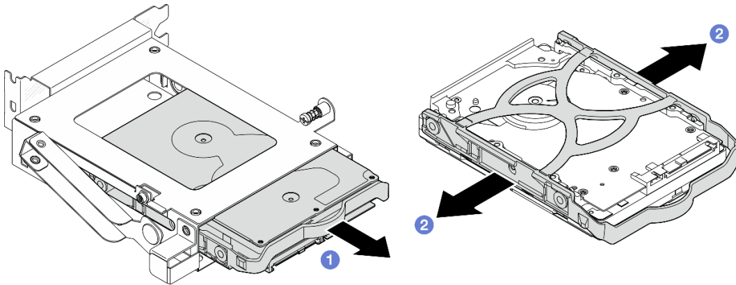
Рис. 34. Снятие блока 3,5-дюймового диска
