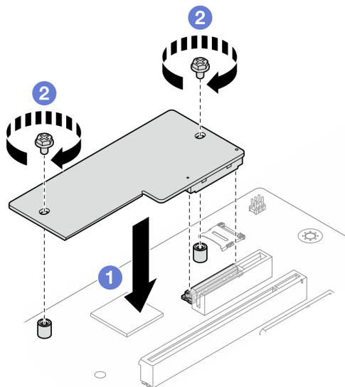
Рис. 93. Установка Модуль безопасности микропрограммы и RoT
