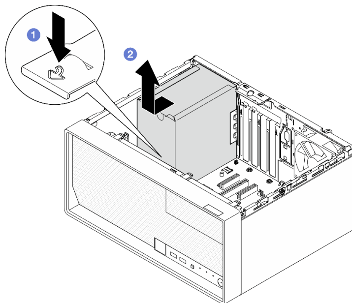
Рис. 85. Снятие блока питания
