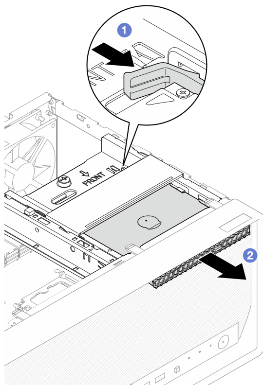
Рис. 41. Снятие дисководов для оптических дисков
