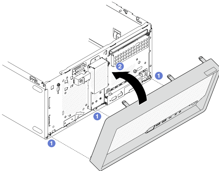
Рис. 55. Установка лицевой панели
