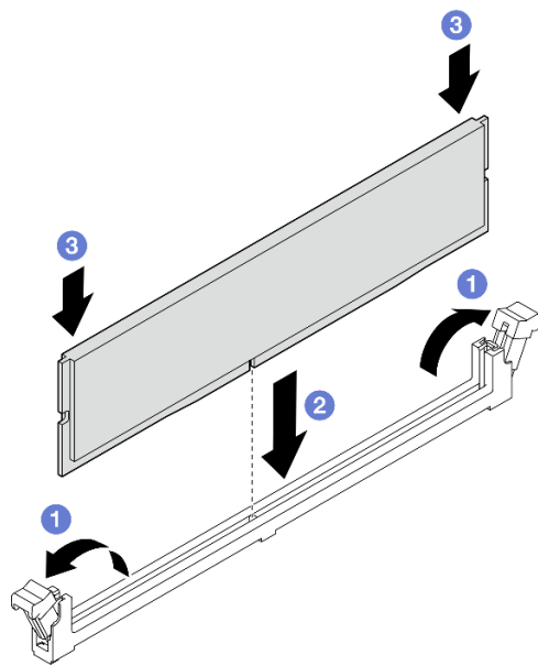
Рис. 79. Установка модуля памяти
