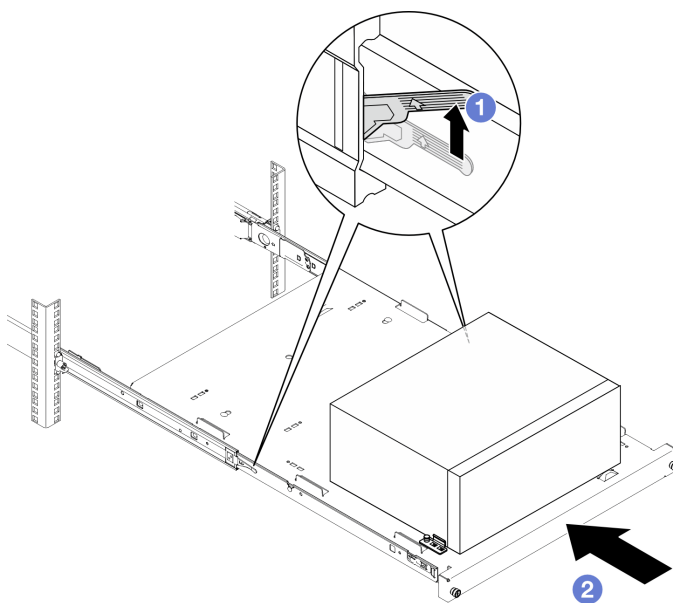
Рис. 7. Установка сервера в стойку
