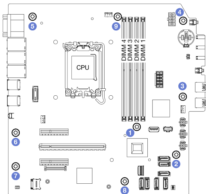
Рис. 96. Последовательность снятия винтов с материнской платы
