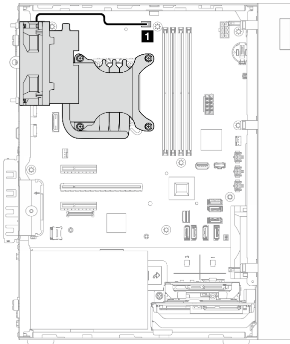
Рис. 120. Прокладка кабеля для модуля радиатора и вентилятора процессора с величиной отвода тепловой мощности 95 Вт
