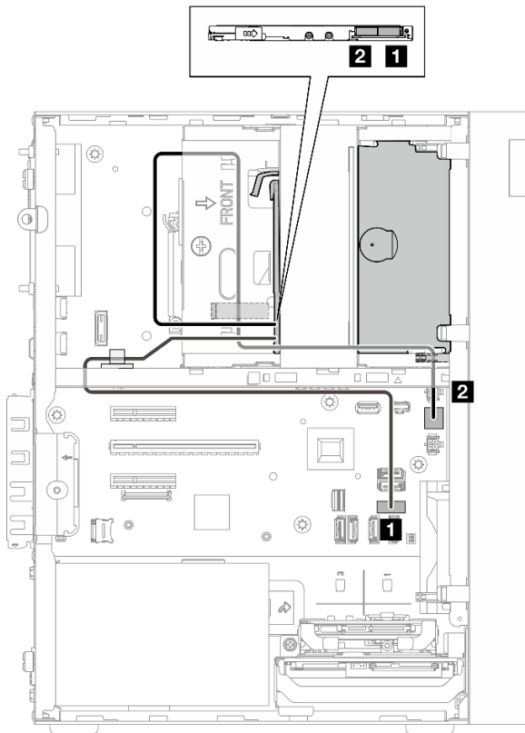
Рис. 112. Прокладка кабелей для дисководов для оптических дисков
