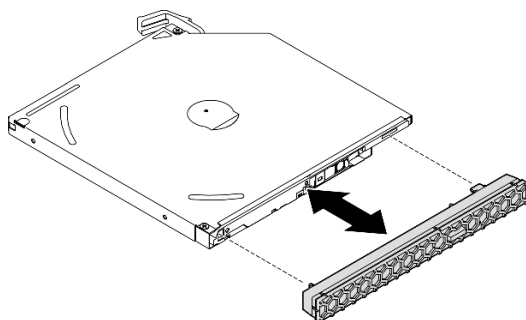
Рис. 47. Установка панели дисководов для оптических дисков
