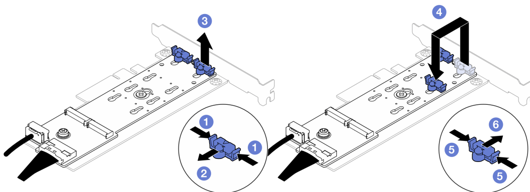
Рис. 71. Регулировка фиксатора M.2
