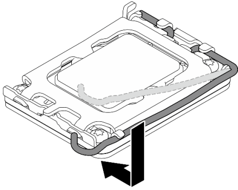
Рис. 91. Закрытие фиксатора процессора
