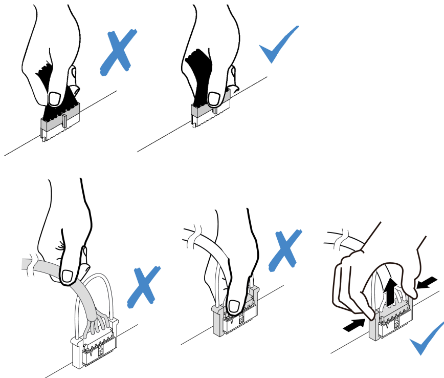
Рис. 107. Нажатие на язычки с двух сторон с целью отсоединения разъема
