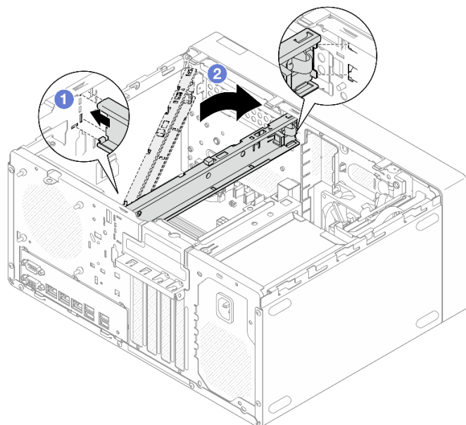
Рис. 104. Установка планки для отсека
