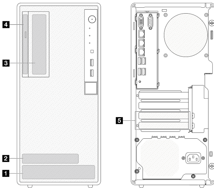
Рис. 11. Расположение отсеков для дисков
