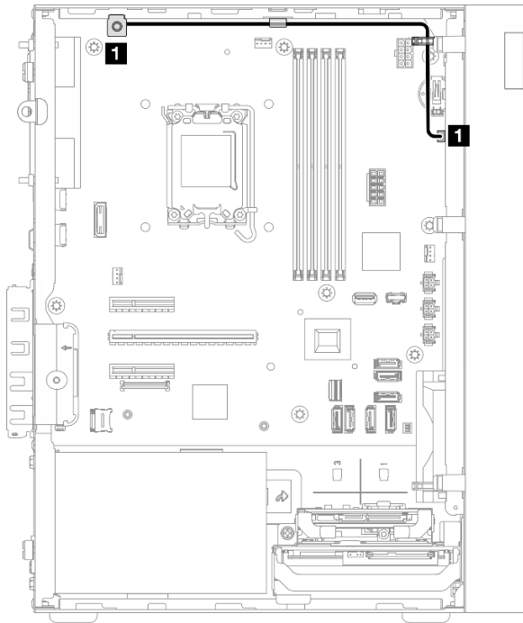
Рис. 121. Прокладка кабеля для датчика вмешательства
