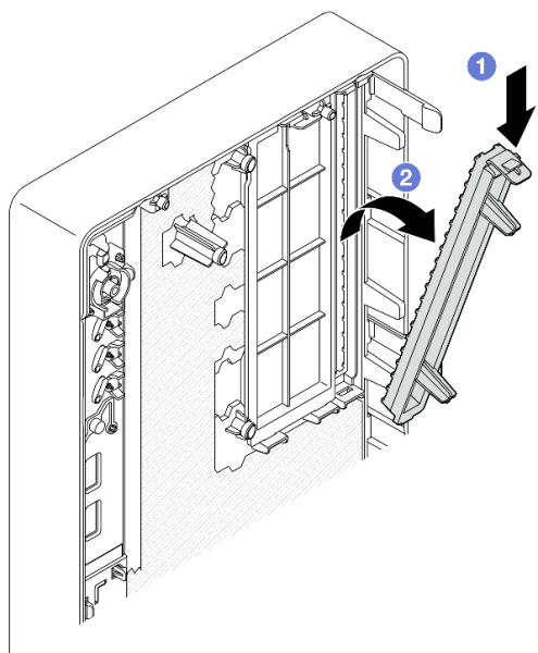
Рис. 45. Снятие защитного экрана отсека дисководов для оптических дисков
