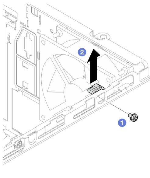
Рис. 62. Снятие датчика вмешательства
