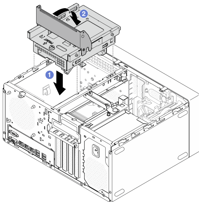
Рис. 50. Установка отсека дисководов для оптических дисков
