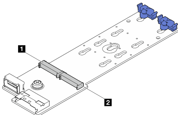
Рис. 72. Гнезда для диска M.2
