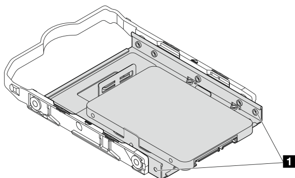
Рис. 30. Размещение отверстий для винтов диска на фиксаторе
