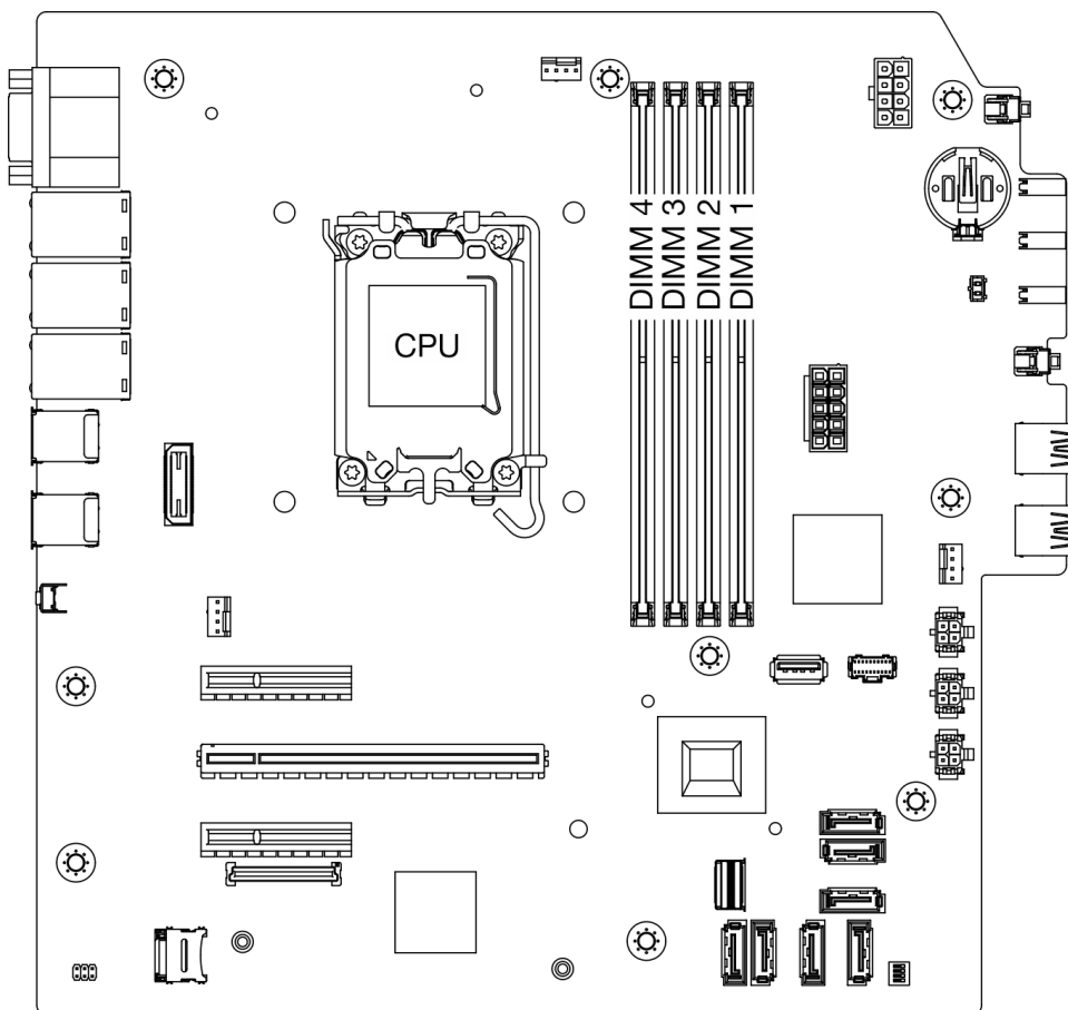
Рис. 1. Расположение модулей памяти и процессоров
