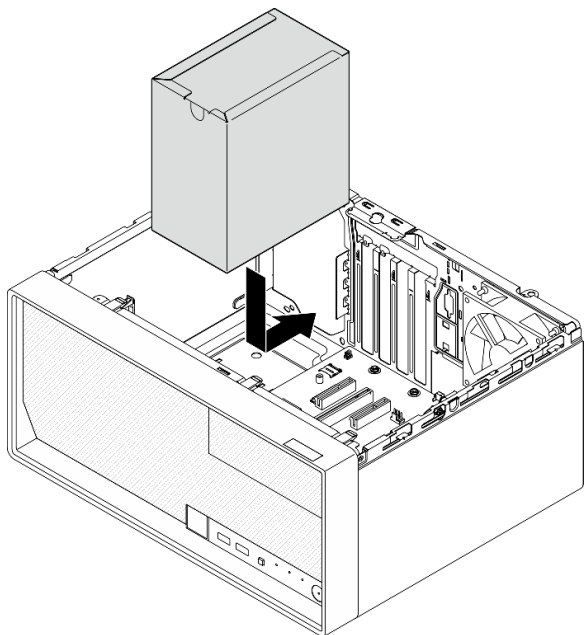
Рис. 86. Установка модуля блока питания в раму
