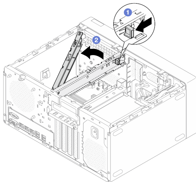
Рис. 103. Снятие планки для отсека
