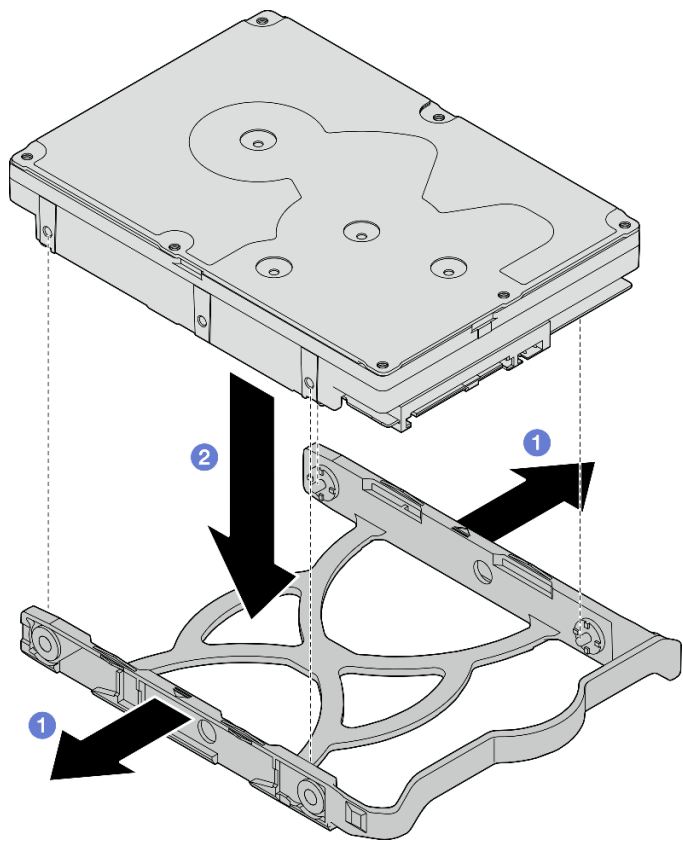
Рис. 17. Установка 3,5-дюймового диска в фиксатор
