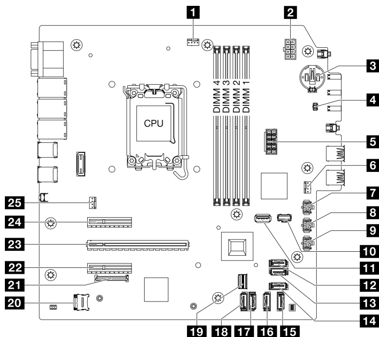
Рис. 124. Разъемы материнской платы
