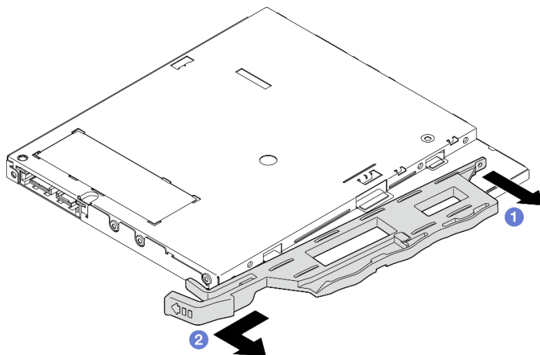
Рис. 42. Снятие фиксатора дисководов для оптических дисков
