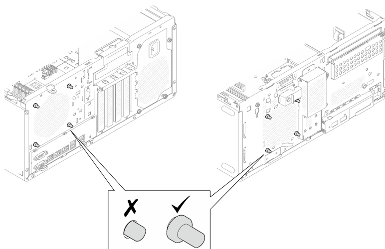
Рис. 53. Установка резиновых креплений переднего и заднего вентиляторов
