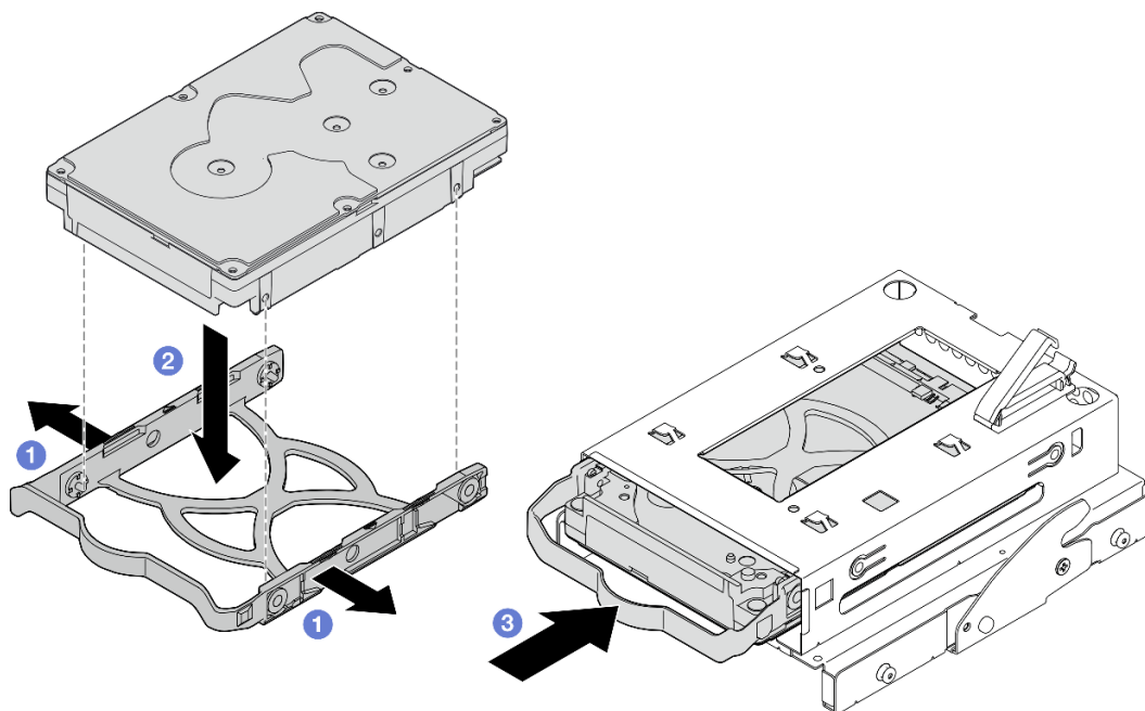
Рис. 29. Установка 3,5-дюймового диска в отсек для диска
