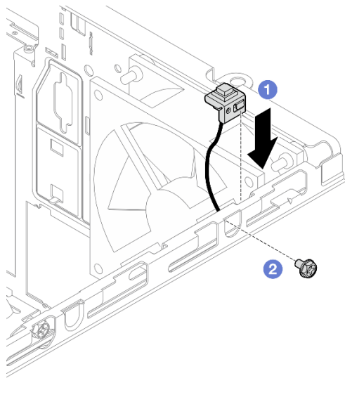
Рис. 64. Установка датчика вмешательства
