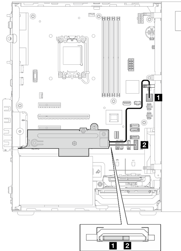
Рис. 111. Прокладка кабелей для отсека для дисков 3
