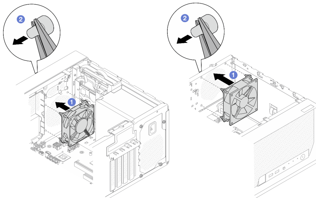
Рис. 52. Установка переднего или заднего вентилятора
