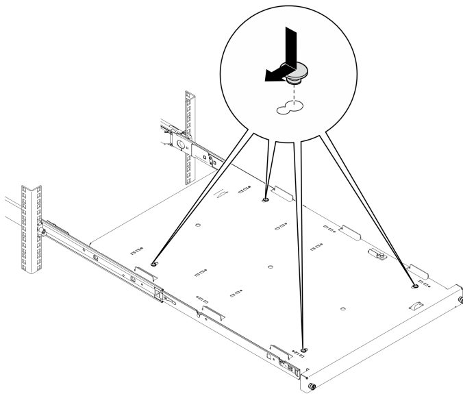
Рис. 5. Установка на лоток резиновых защитных подкладок
