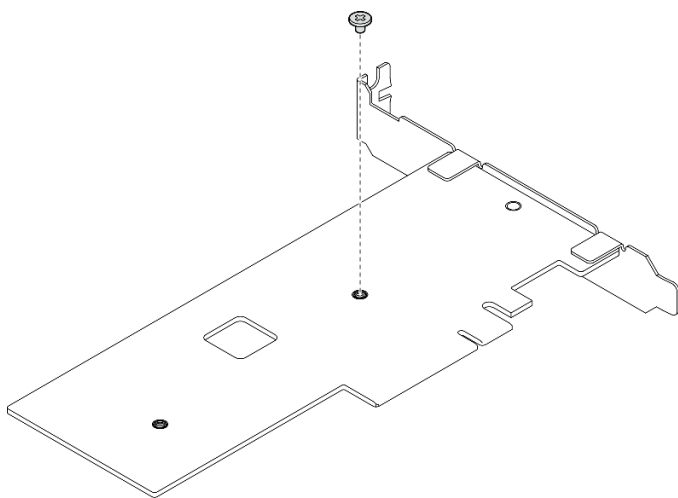
Рис. 67. Удаление винта в задней части адаптера PCIe
