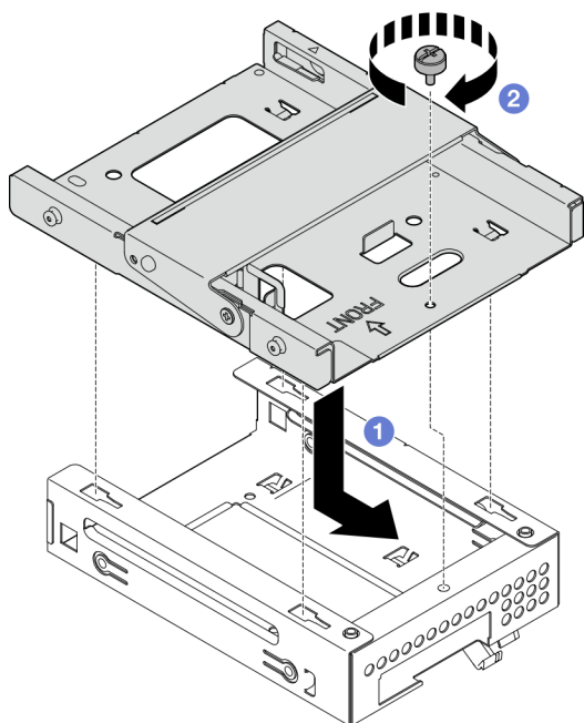
Рис. 33. Установка отсека для 3,5-дюймового диска в отсек дисковод для оптических дисков
