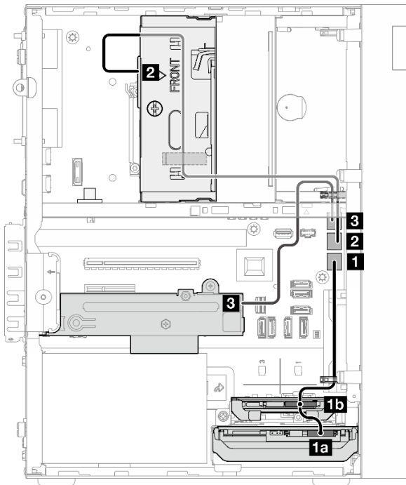
Рис. 115. Прокладка кабелей питания
