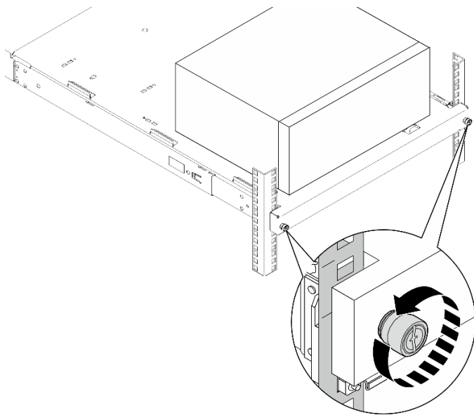
Рис. 2. Снятие винтов на передней панели стойки
