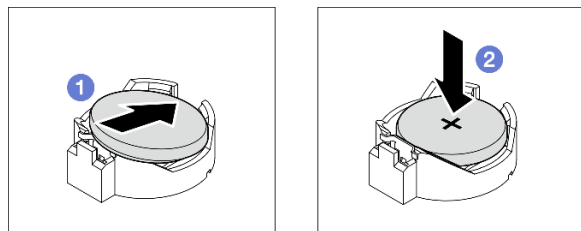
Рис. 10. Установка батарейки CMOS
