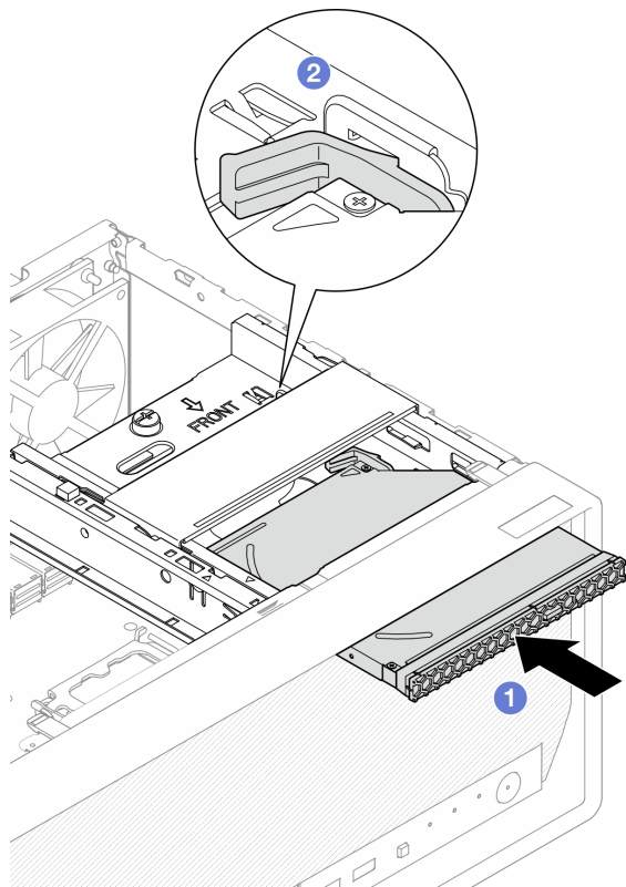
Рис. 48. Установка дисководов для оптических дисков
