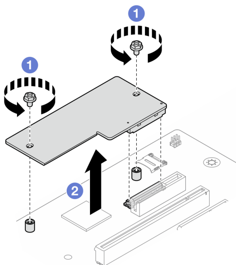
Рис. 92. Снятие Модуль безопасности микропрограммы и RoT
