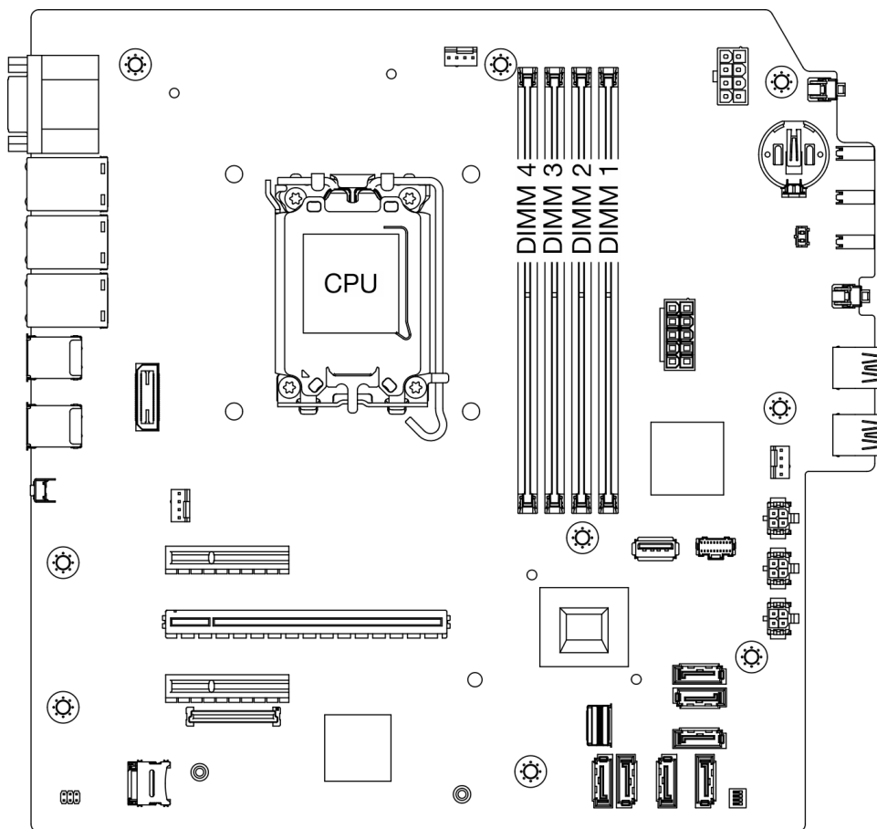
Рис. 77. Расположение модулей памяти и процессоров
