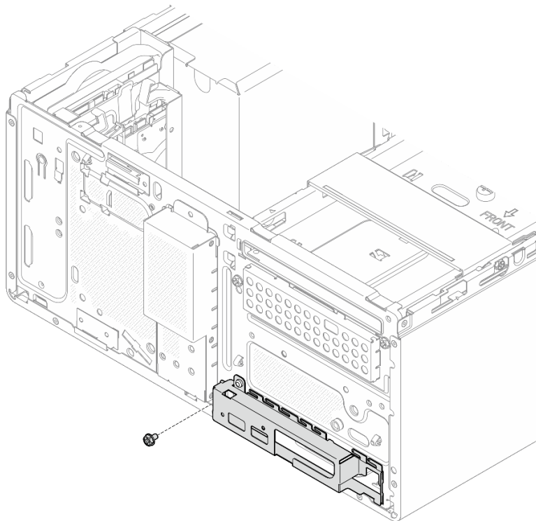
Рис. 101. Фиксация передней скобы ввода-вывода на раме
