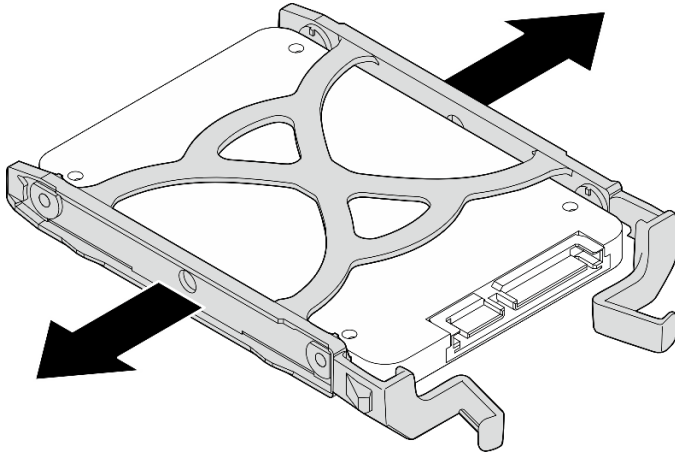
Рис. 15. Снятие 2,5-дюймового диска с фиксатора
