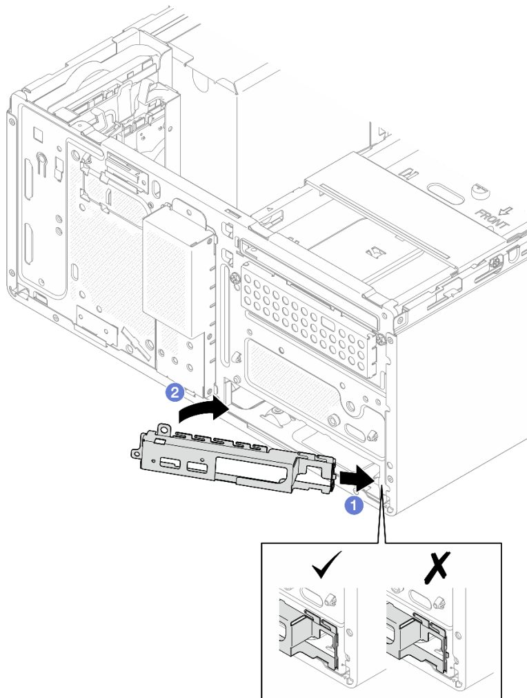
Рис. 100. Установка передней скобы ввода-вывода на раму
