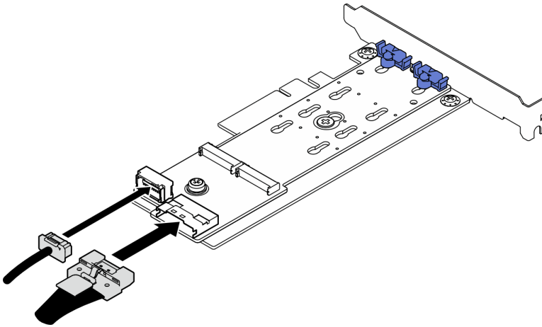
Рис. 69. Установка кабелей питания и сигнальных кабелей M.2
