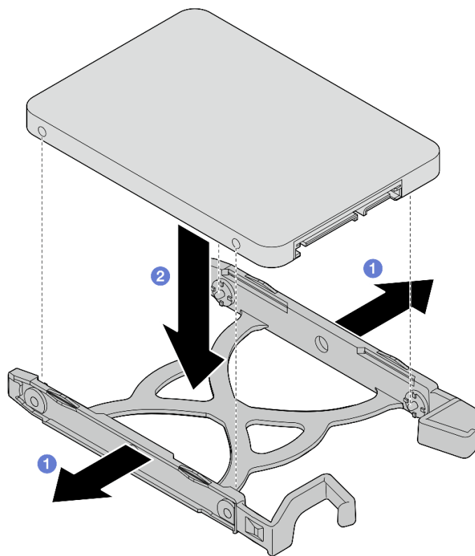
Рис. 18. Установка 2,5-дюймового диска в фиксатор
