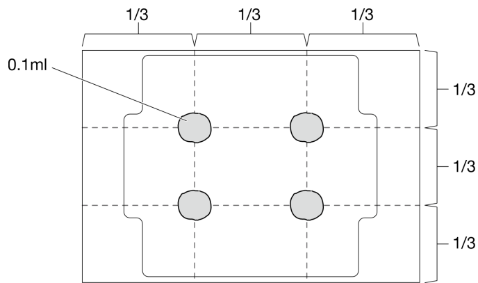
Рис. 89. Надлежащая форма термопасты
