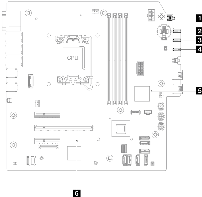
Рис. 126. Светодиодные индикаторы материнской платы
