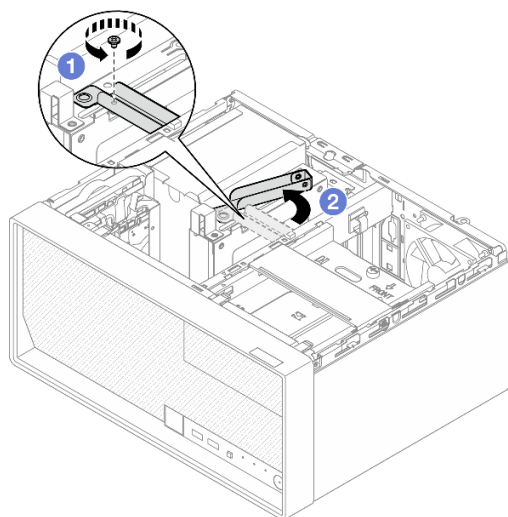
Рис. 37. Разблокировка защелки отсека для диска 3
