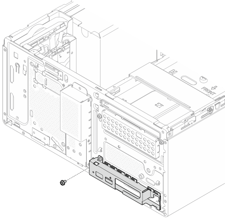
Рис. 94. Снятие винта, фиксирующего переднюю скобу ввода-вывода на раме
