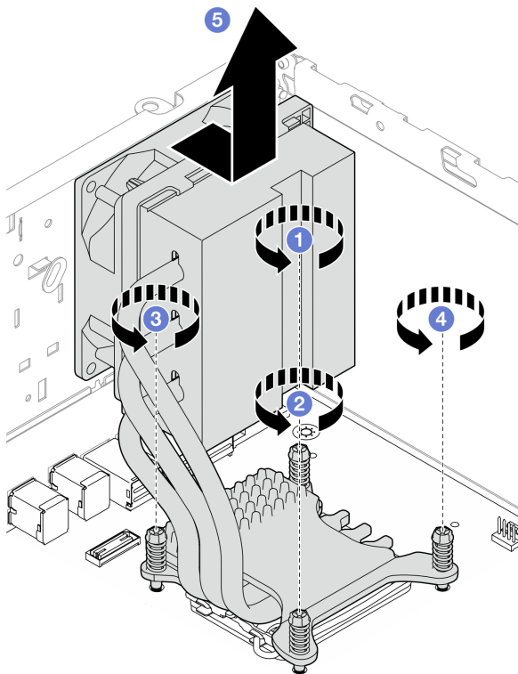
Рис. 58. Ослабление винтов на модуле радиатора и вентилятора для процессора с величиной отвода тепловой мощности 95 Вт
