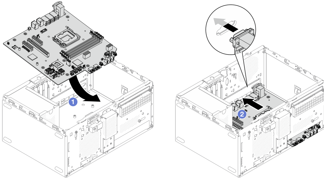
Рис. 98. Установка материнской платы в раму
