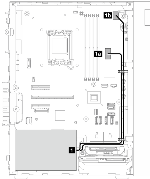
Рис. 117. Прокладка кабелей для модуля блока питания
