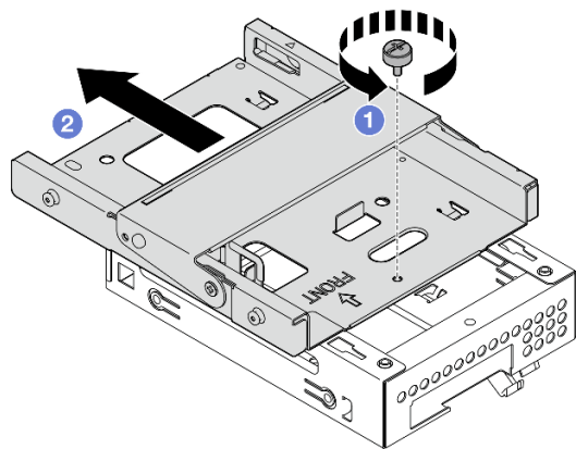
Рис. 31. Снятие отсека для 3,5-дюймового диска с отсека дисководов для оптических дисков
