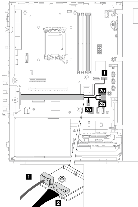
Рис. 113. Прокладка кабелей для адаптера загрузки M.2
