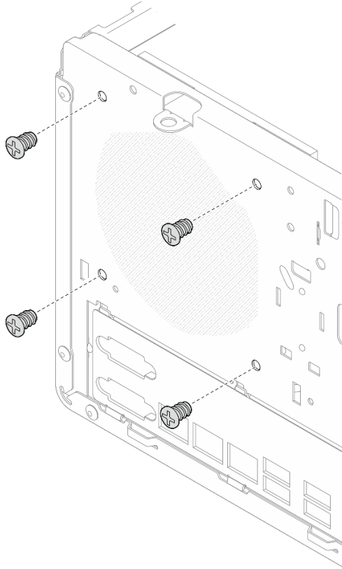
Рис. 56. Снятие четырех винтов, которыми вентилятор радиатора крепится к раме
