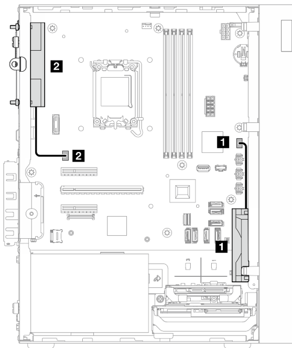
Рис. 118. Прокладка кабелей для переднего и заднего вентиляторов
