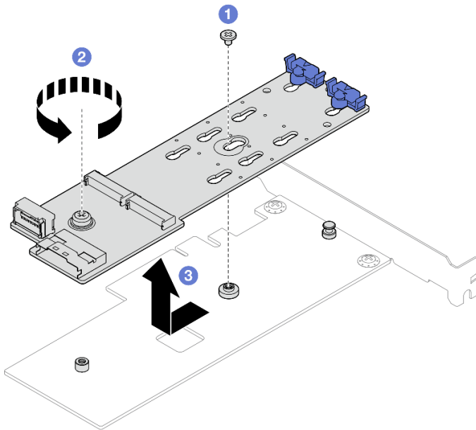
Рис. 66. Снятие адаптера загрузки M.2
