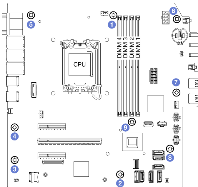
Рис. 99. Установка материнской платы в раму
