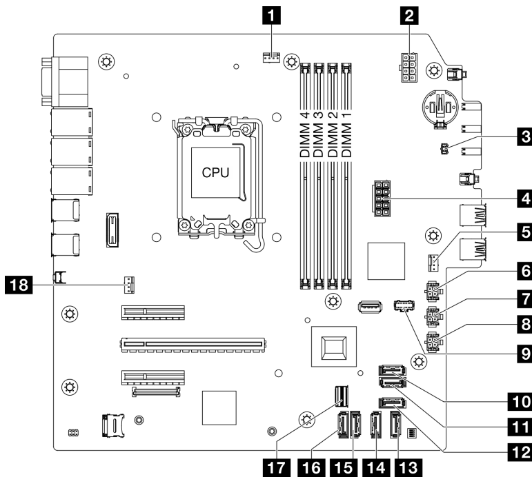
Рис. 108. Разъемы материнской платы
