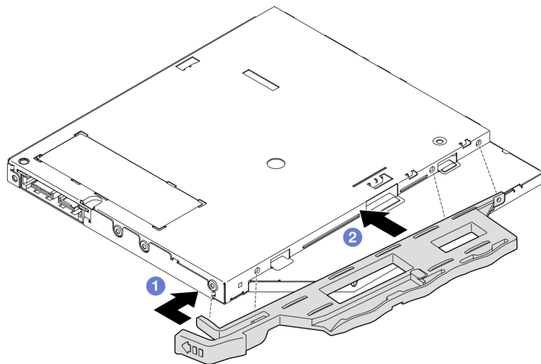
Рис. 46. Установка фиксатора на дисковод для оптических дисков
