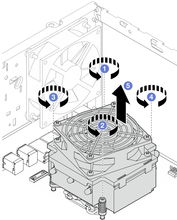
Рис. 57. Ослабление винтов на модуле радиатора и вентилятора для процессора с величиной отвода тепловой мощности менее 95 Вт
