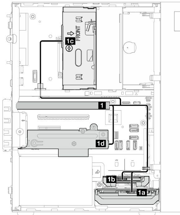
Рис. 116. Прокладка сигнальных кабелей
