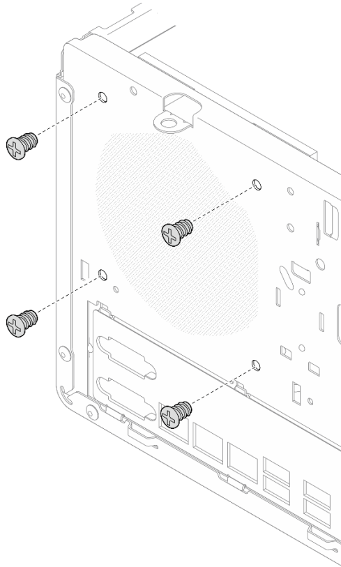
Рис. 61. Установка вентилятора радиатора с задней стороны рамы
