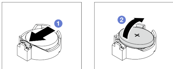
Рис. 9. Извлечение батарейки CMOS
