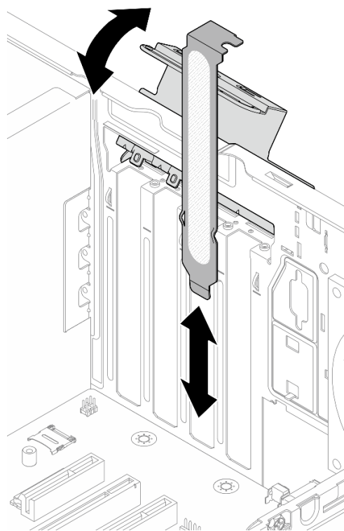
Рис. 82. Снятие скобы адаптера PCIe
