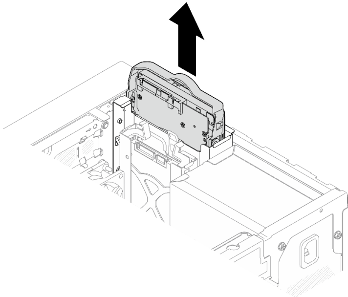
Рис. 12. Снятие блока диска с отсека для диска 0
