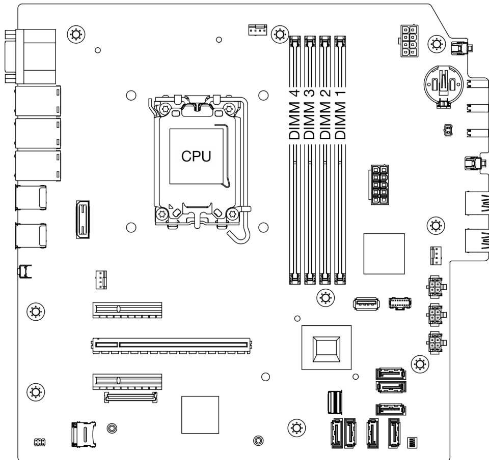
Рис. 74. Расположение модулей памяти и процессоров
