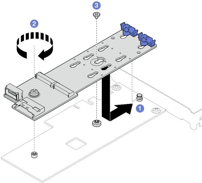
Рис. 68. Фиксация адаптера загрузки M.2 на адаптере PCIe
