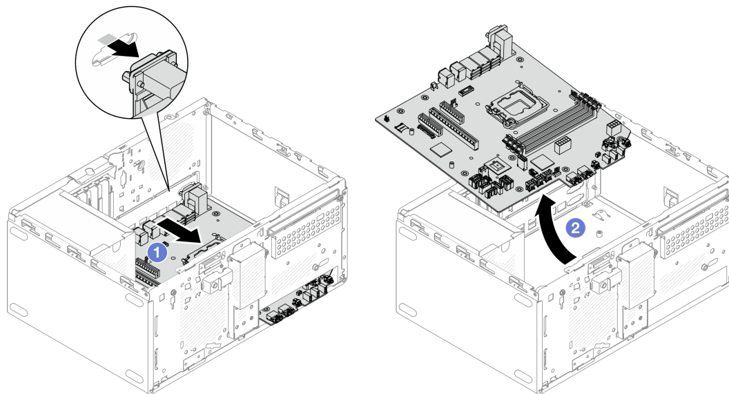
Рис. 97. Снятие материнской платы с рамы
