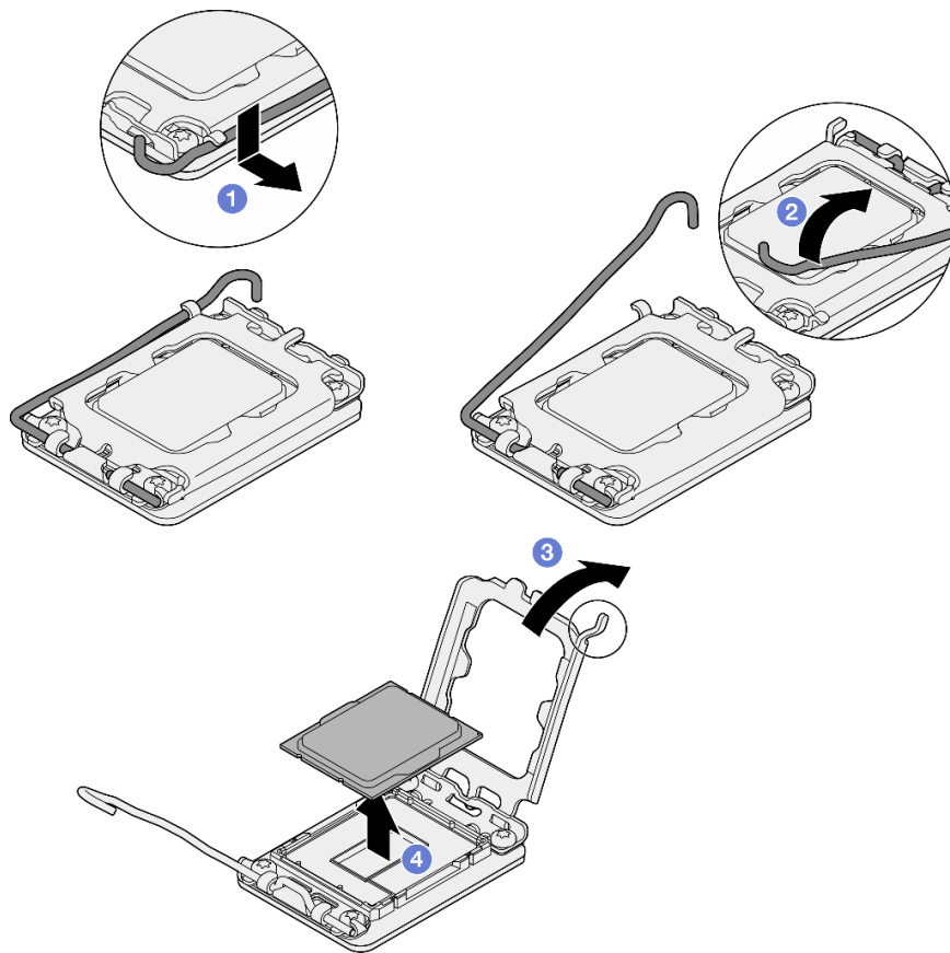
Рис. 88. Снятие процессора
