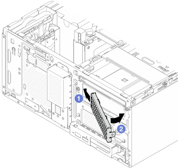
Рис. 32. Установка экрана защиты от электромагнитных помех
