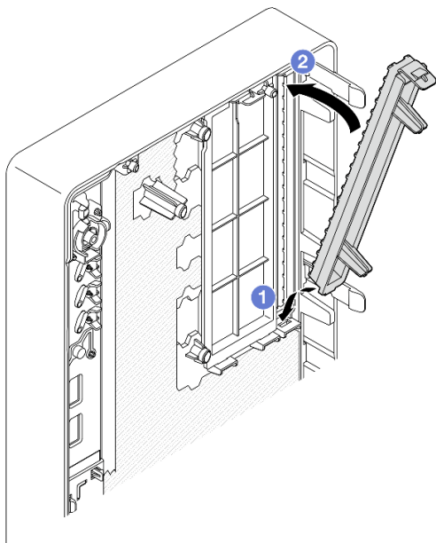
Рис. 44. Установка защитного экрана отсека дисковода для оптических дисков
