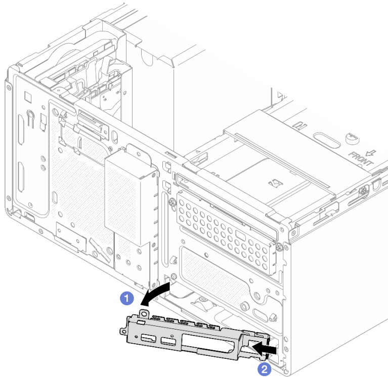
Рис. 95. Снятие передней скобы ввода-вывода с рамы
