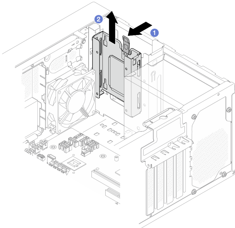
Рис. 21. Извлечение отсека для диска из отсека 1
