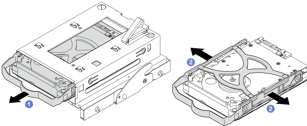
Рис. 27. Снятие блока 3,5-дюймового диска
