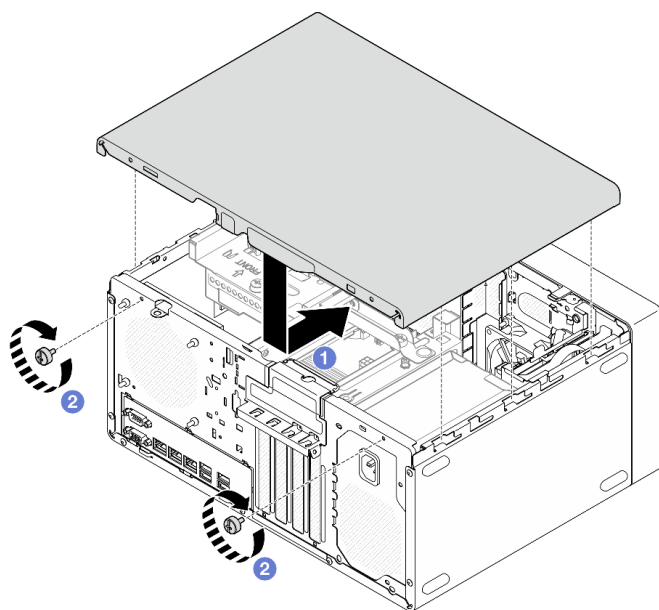
Рис. 105. Установка кожуха сервера
