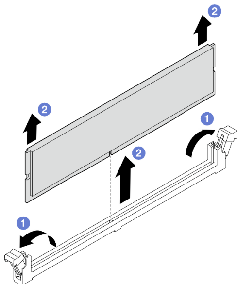
Рис. 76. Снятие модуля памяти
