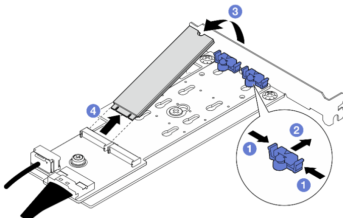
Рис. 70. Снятие диска M.2
