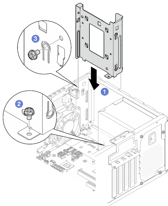
Рис. 24. Установка отсека для диска в отсек 0
