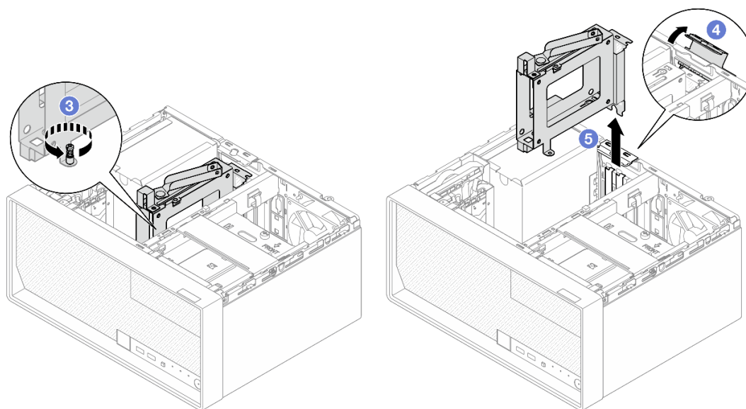
Рис. 38. Извлечение отсека для 3,5-дюймовых дисков из разъема PCIe 3
