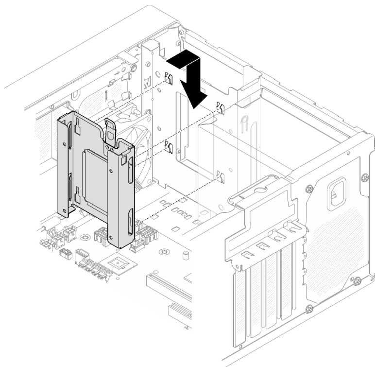
Рис. 26. Установка отсека для диска в отсек 1
