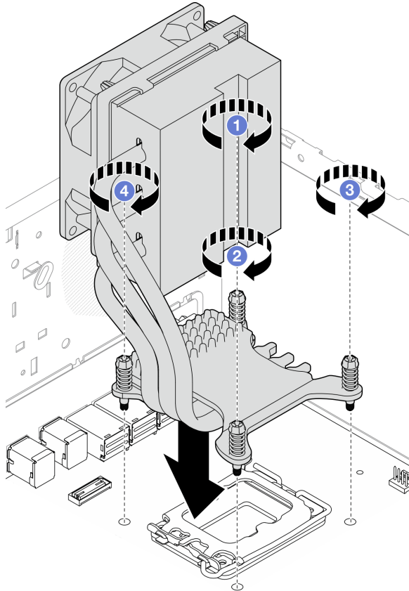
Рис. 60. Затягивание винтов на модуле радиатора и вентилятора для процессора с величиной отвода тепловой мощности 95 Вт
