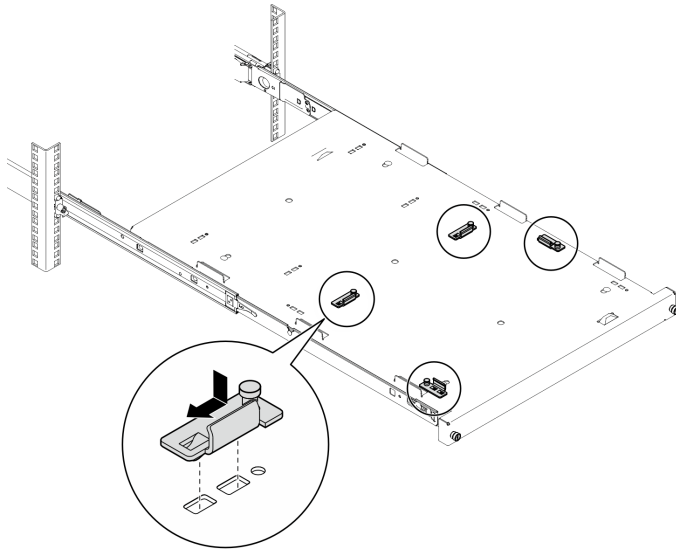
Рис. 4. Установка скоб на лоток
