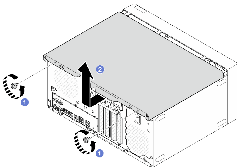
Рис. 102. Снятие кожуха сервера
