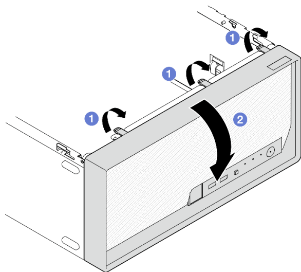
Рис. 54. Снятие лицевой панели
