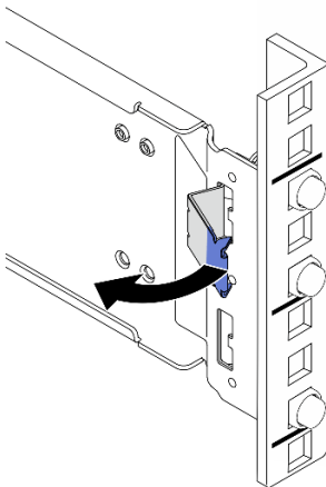
Figure 10. Dégager la glissière à partir de la bride de montage arrière
