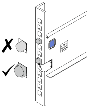
Figure 4. Broches dans les orifices carrés de bride de montage
