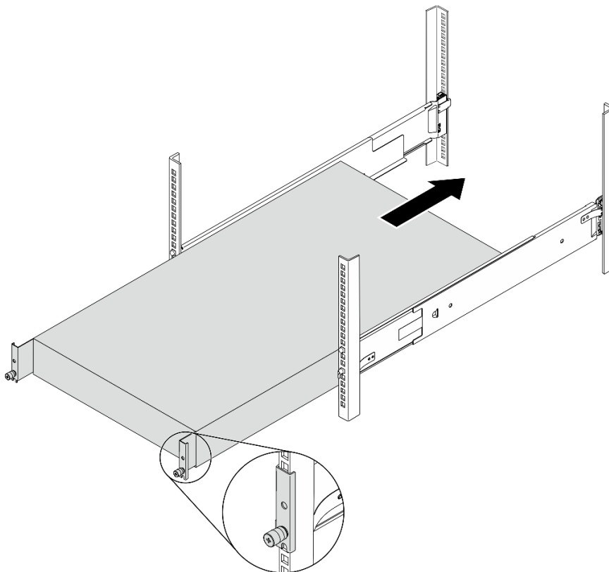
Figure 7. Installation du boîtier 2U à quatre nœuds dans les glissières
