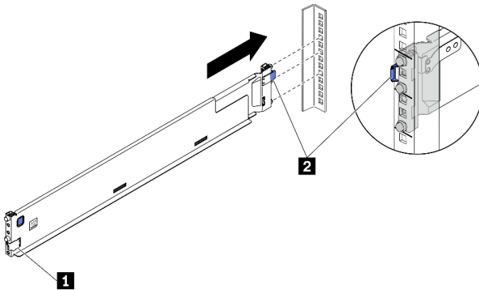
Figure 2. Installation de l'extrémité arrière de la glissière
