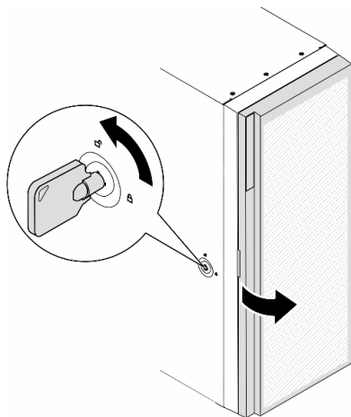
Figure 9. Verrouillage de la porte de sécurité et du carter du serveur
