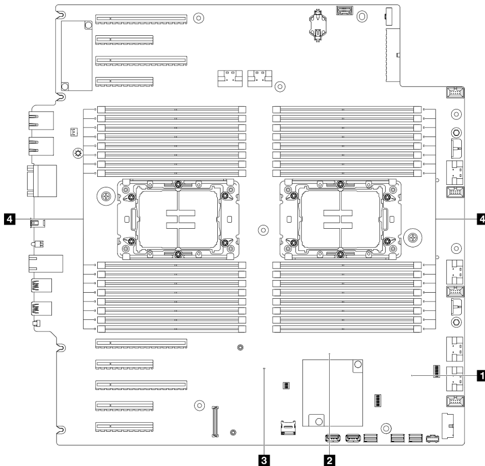
Figure 13. Voyants de la carte mère
