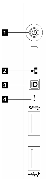
Figure 11. Voyants du panneau opérateur avant
