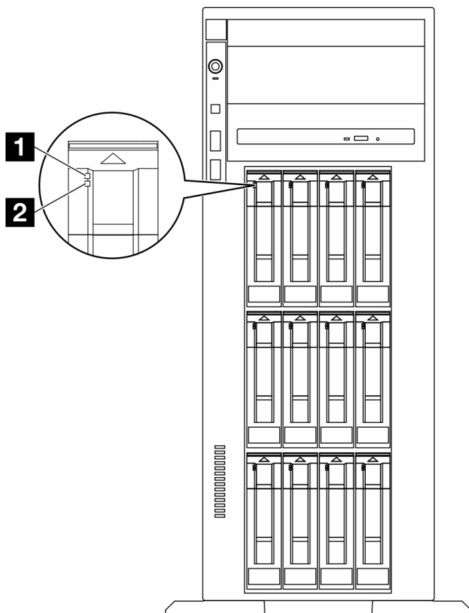
Figure 10. Voyants d'unité
