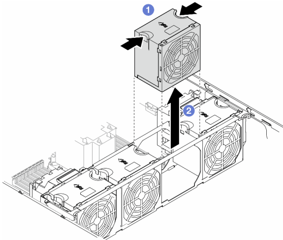
図 30. ファン・モジュールの取り外し
