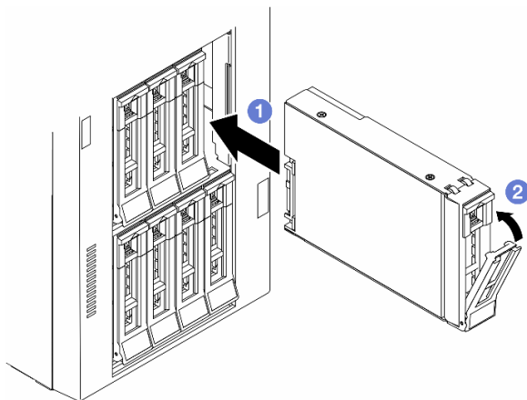
図 27. ホット・スワップ・ドライブの取り付け
