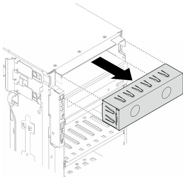
図 79. ドライブ・フィラー・カバーの取り外し
