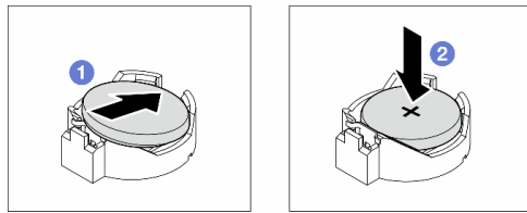
図 21. CMOS バッテリーの取り付け
