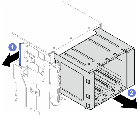
図 28. 拡張ドライブ・ケージの取り外し
