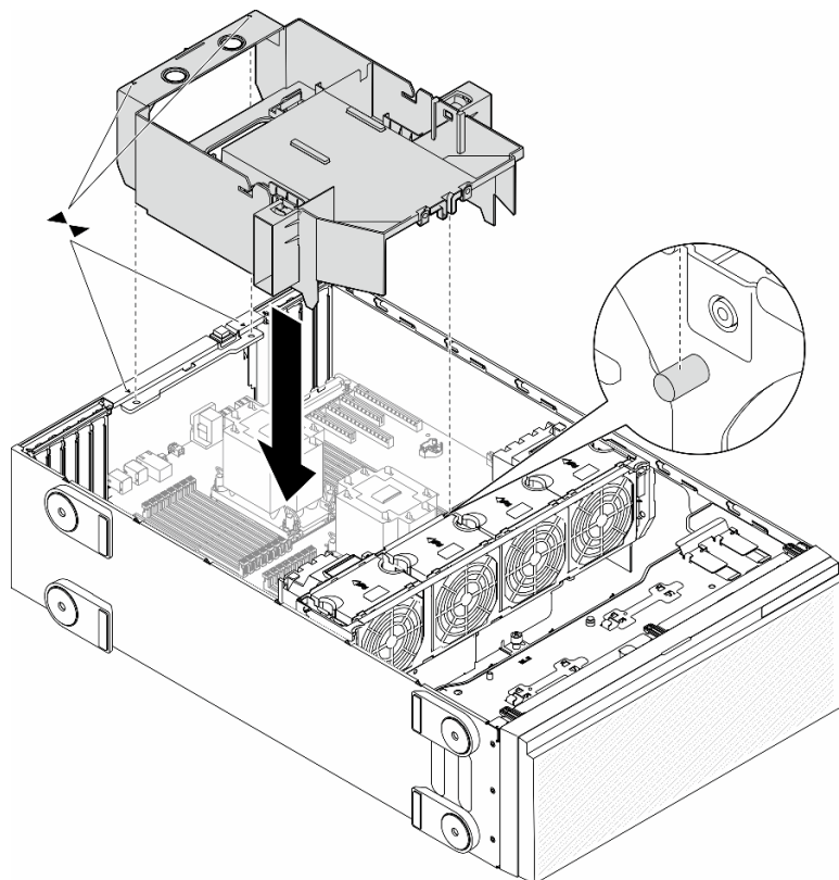
図19. エアー・バッフルの取り付け
