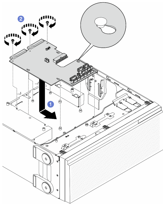
図98. 分電盤の取り付け
