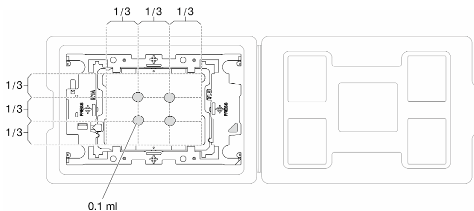
図 113. 配送トレイのプロセッサで熱伝導グリースを塗布する
