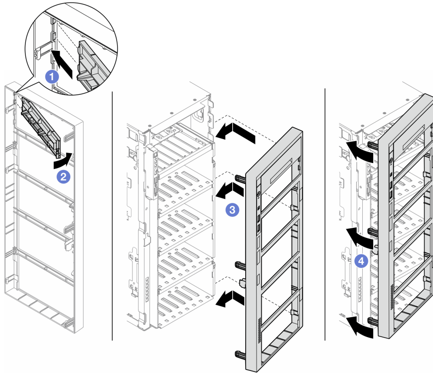
図76. ドライブ・ベイ・フィラー・カバーおよび前面ベゼルの取り付け
