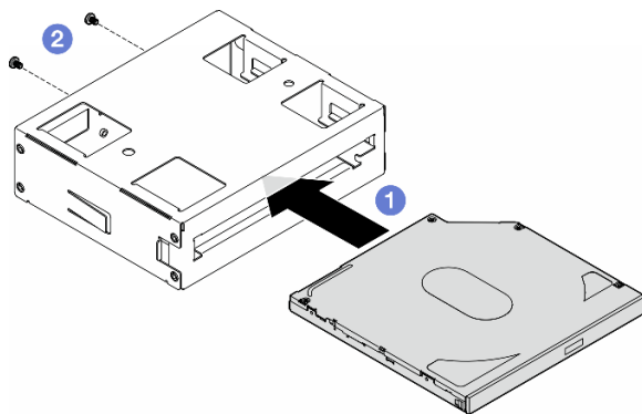
図89. 光学式スリム・ドライブのドライブ・ベイ・アダプターへの取り付け
