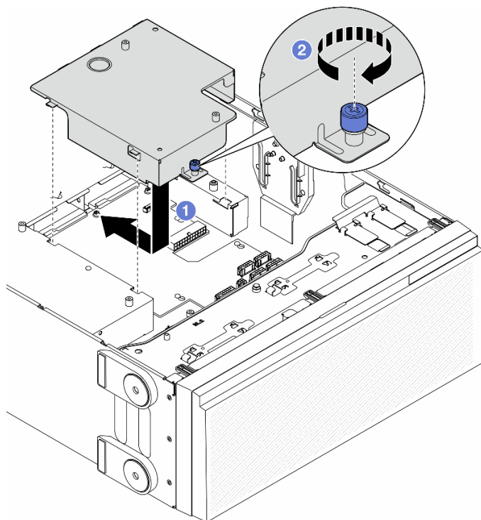
図 100. 分電盤カバーの取り付け
