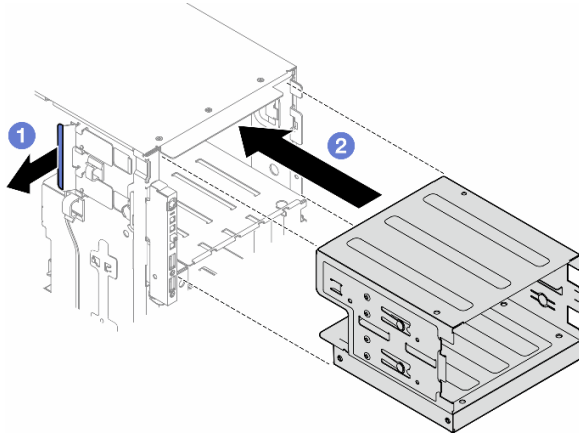
図 73. 光学式ドライブ・ケージの取り付け
