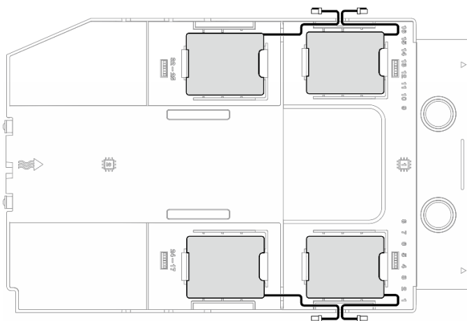
図 38. フラッシュ電源モジュールのケーブル配線
