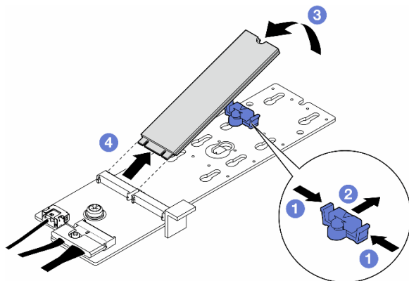
図 58. M.2 ドライブの取り外し
