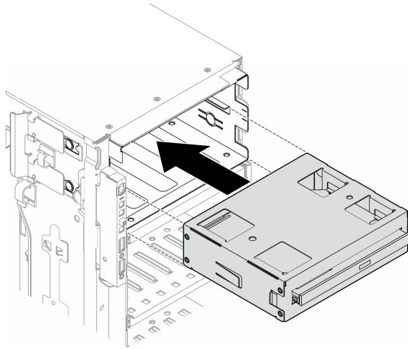
図90. 光学式ドライブ・ケージ・アセンブリーの取り付け
