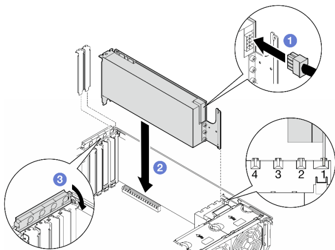
図 96. FL GPU アダプターの取り付け
