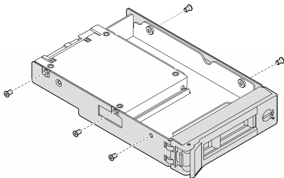
図 26. 2.5 型ドライブおよびドライブ・アダプターを固定するねじの取り付け
