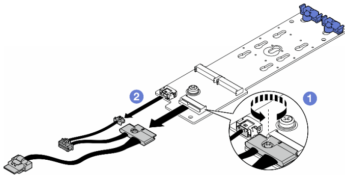
図 59. M.2 信号ケーブルの取り外し
