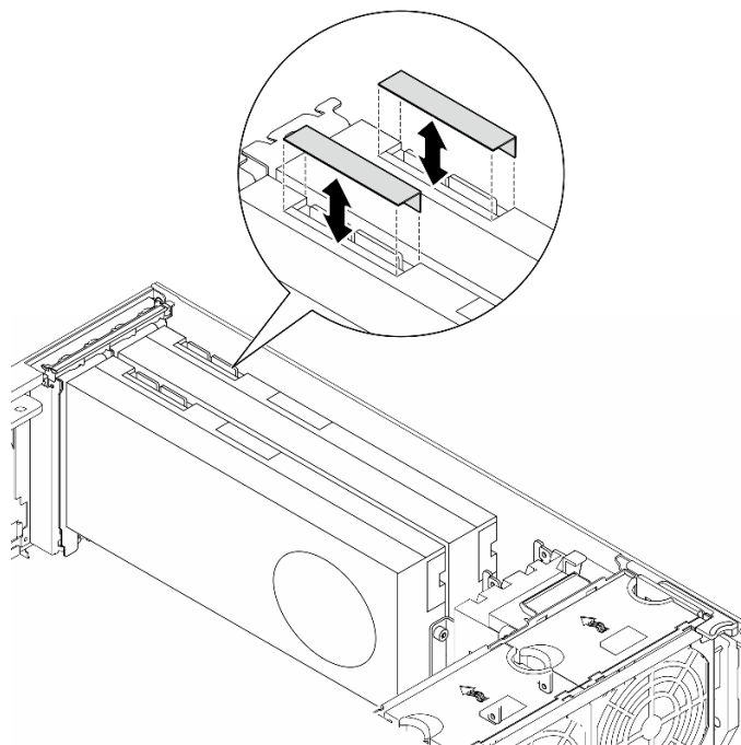
図 70. NVLink カバーの取り外し
