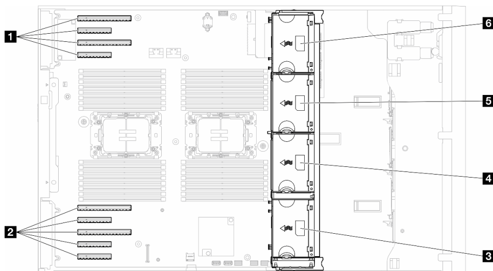
図 33. ファン・スロットの位置
