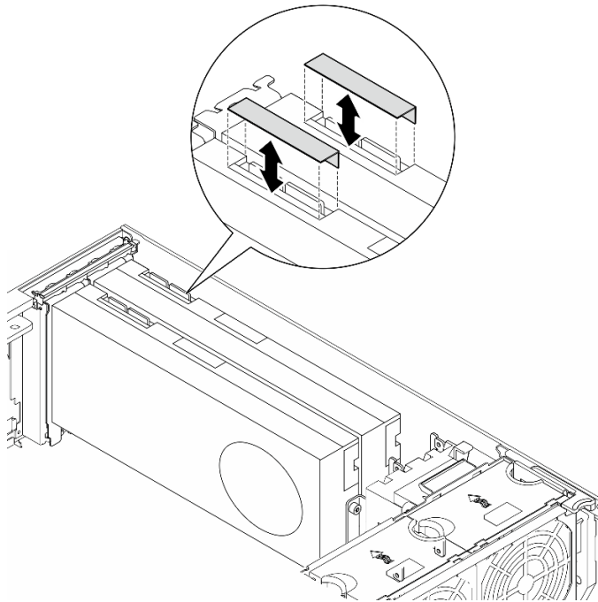
図 69. NVLink カバーの取り付け
