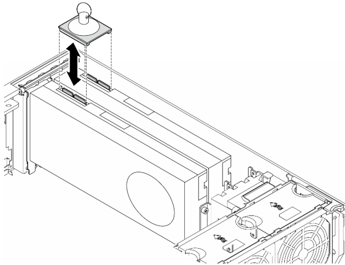
図 68. NVLink ブリッジの取り外し
