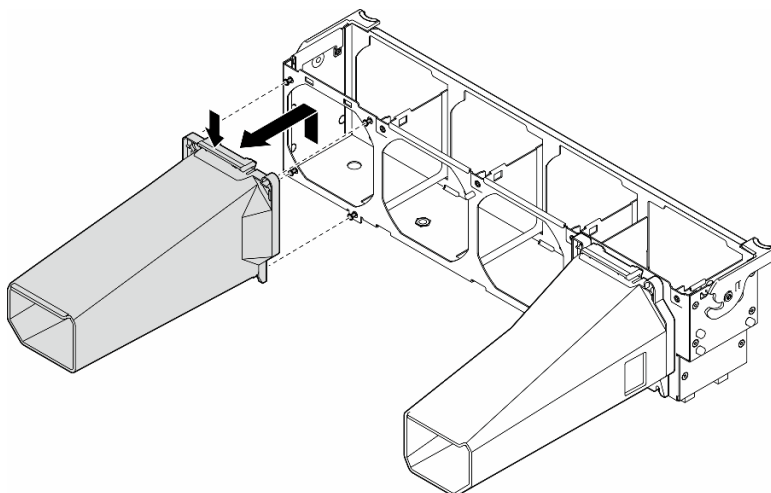
図 16. A2/L4 エアー・ダクトの取り外し
