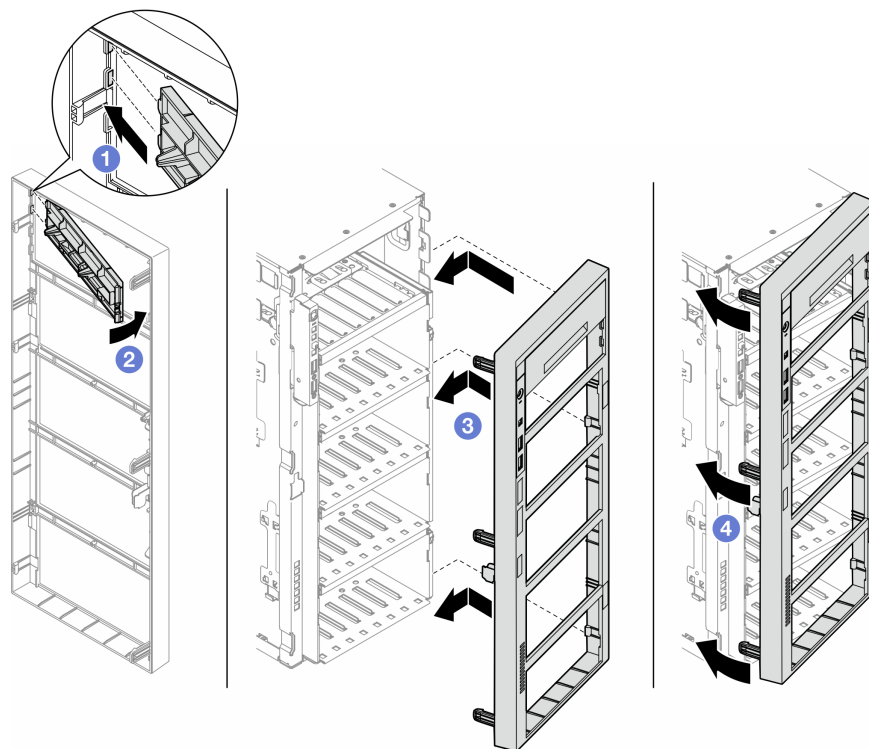
図 86. ドライブ・ベイ・フィラー・カバーおよび前面ベゼルの取り付け
