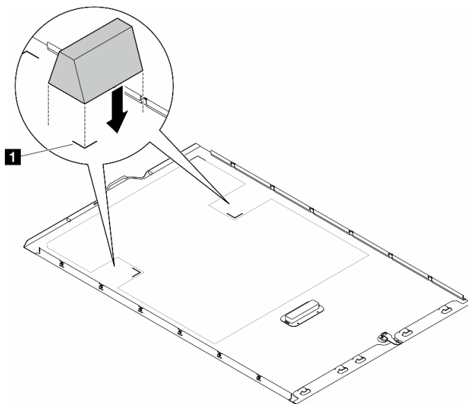
図 128. T4 フィラーの取り付け
