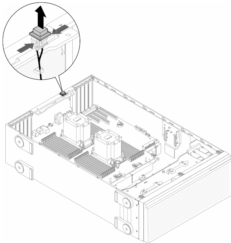
図 56. 侵入検出スイッチの取り外し
