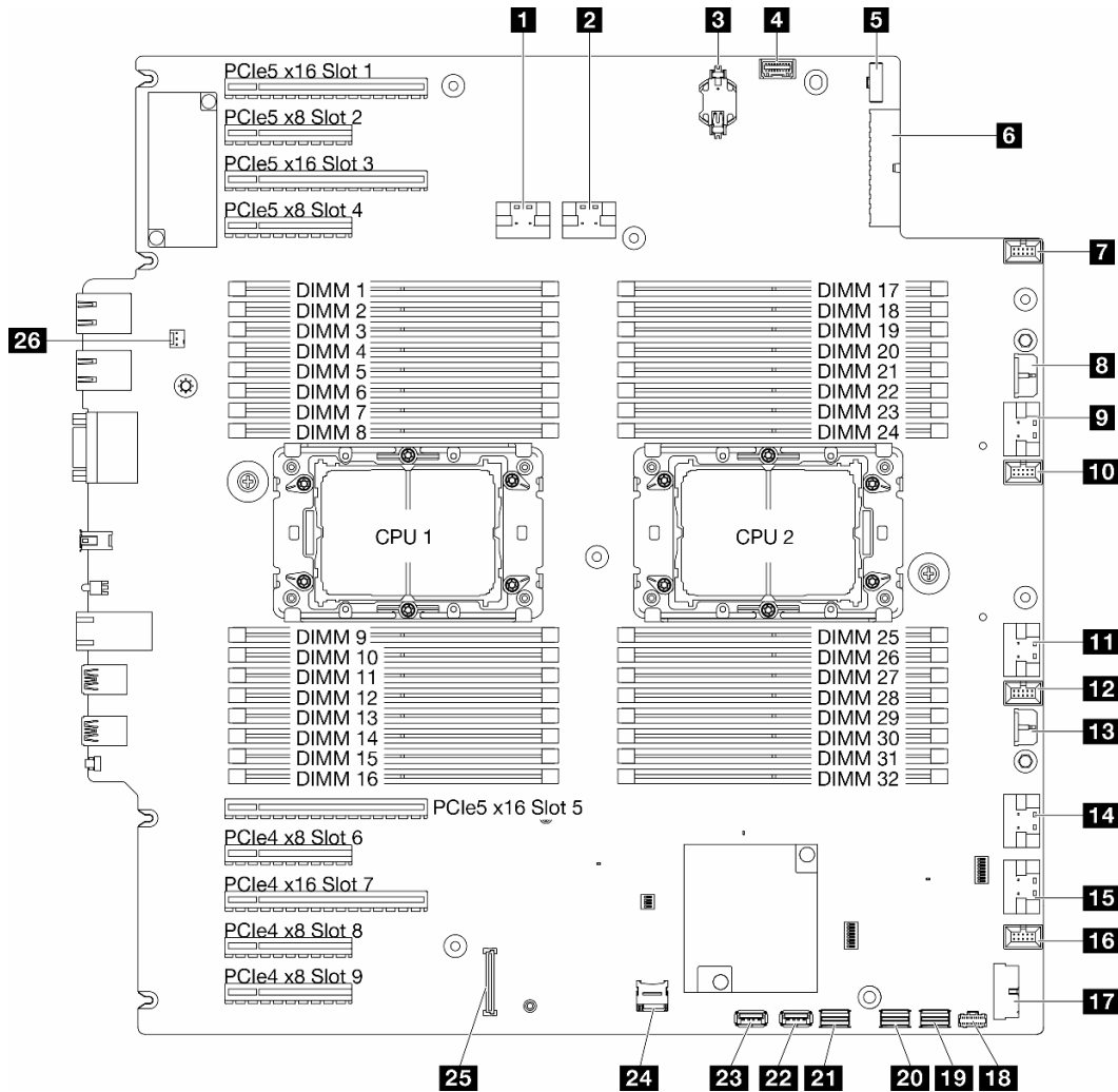
図 145. システム・ボード・コネクタ
