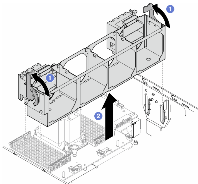
図 31. ファン・ケージ・アセンブリーの取り外し
