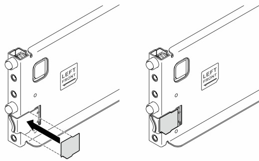
図9. 左側のラッチ・カバーの貼り付け
