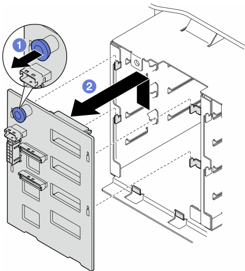
図 14. 3.5 型ドライブ・バックプレーンの取り外し
