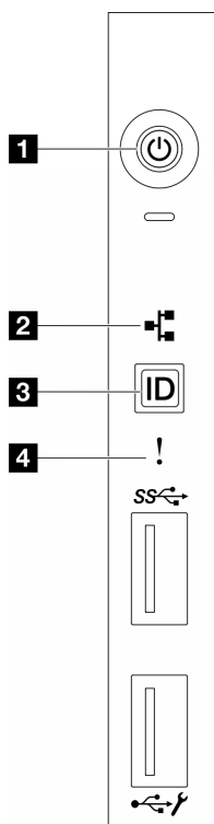
図 147. 前面オペレーター・パネル LED
