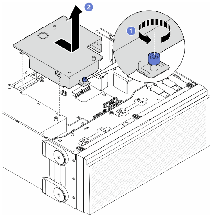
図 99. 分電盤カバーの取り外し
