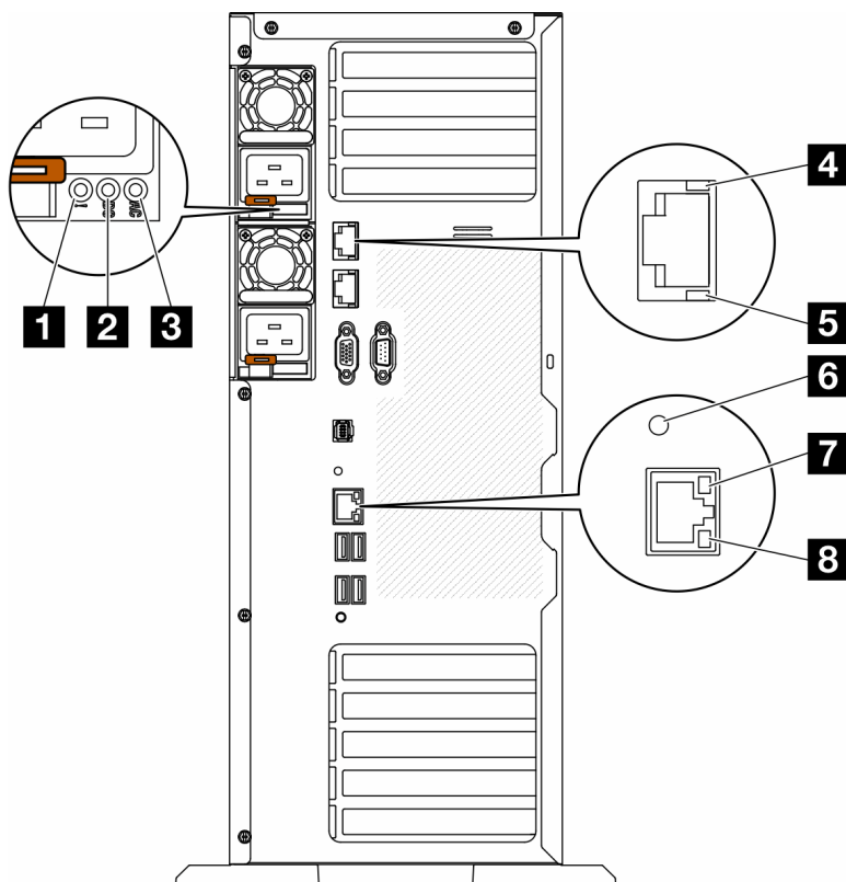
図 148. サーバーの背面システム LED
