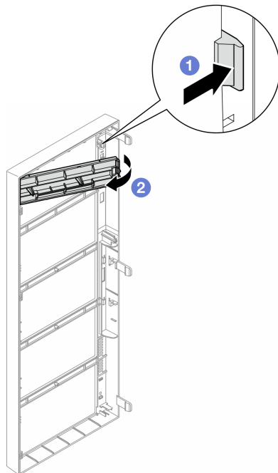
図 87. ドライブ・フィルター・カバーの取り外し
