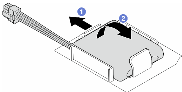
図36. フラッシュ電源モジュールの取り外し
