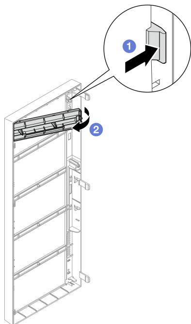
図 78. ドライブ・フィラー・カバーの取り外し
