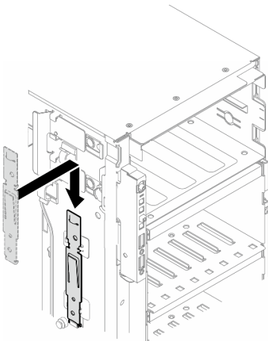
図77. ドライブ保持具の取り付け
