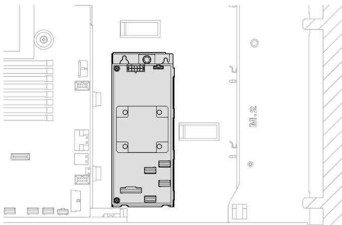
図 53. 内部 CFF アダプターの位置
