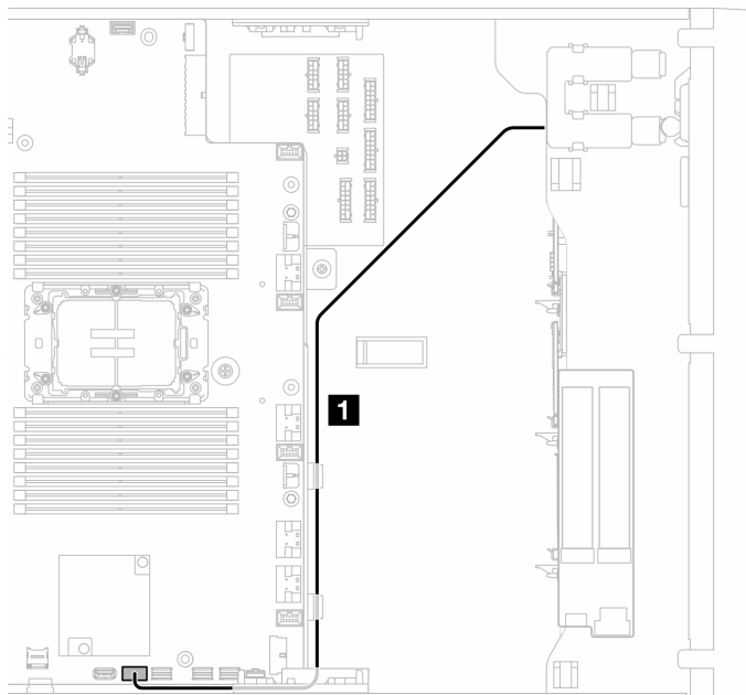
図 141. 光学式ドライブのケーブル配線
