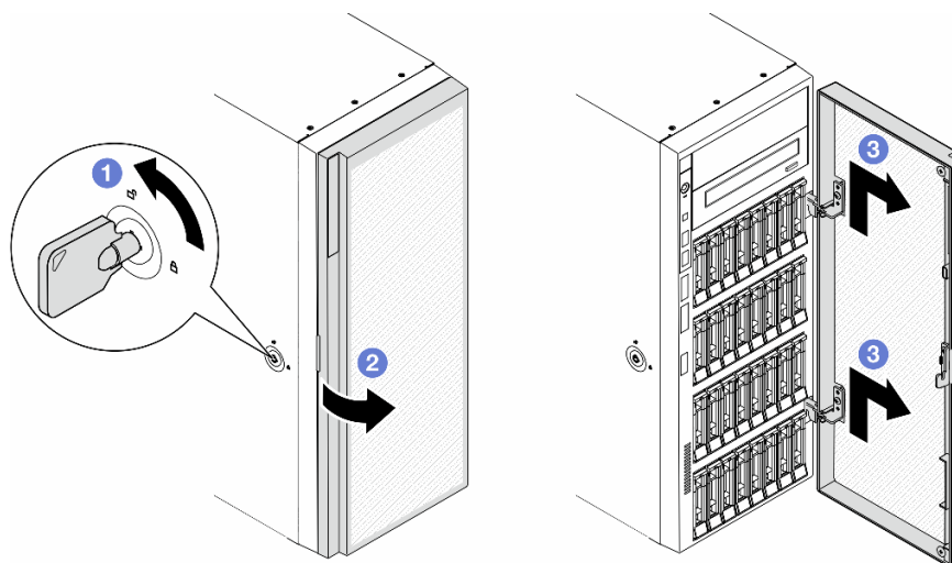
図118. セキュリティー・ドアの取り外し
