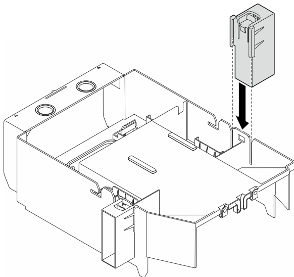
図 49. FL GPU フィラーの取り付け
