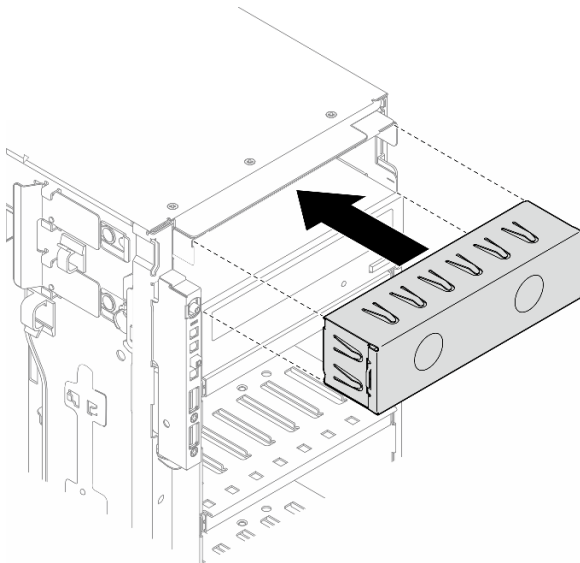
図75. ドライブ・ベイ・フィラーの取り付け
