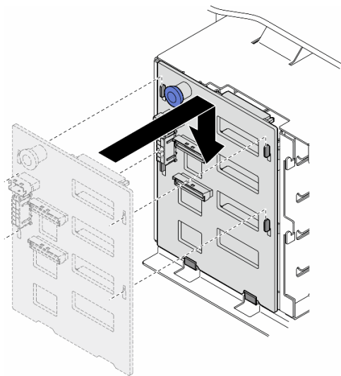
図 15. 3.5 型ドライブ・バックプレーンの取り付け
