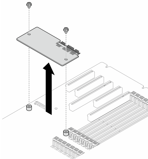
図116. ファームウェアおよびRoTセキュリティー・モジュールの取り外し
