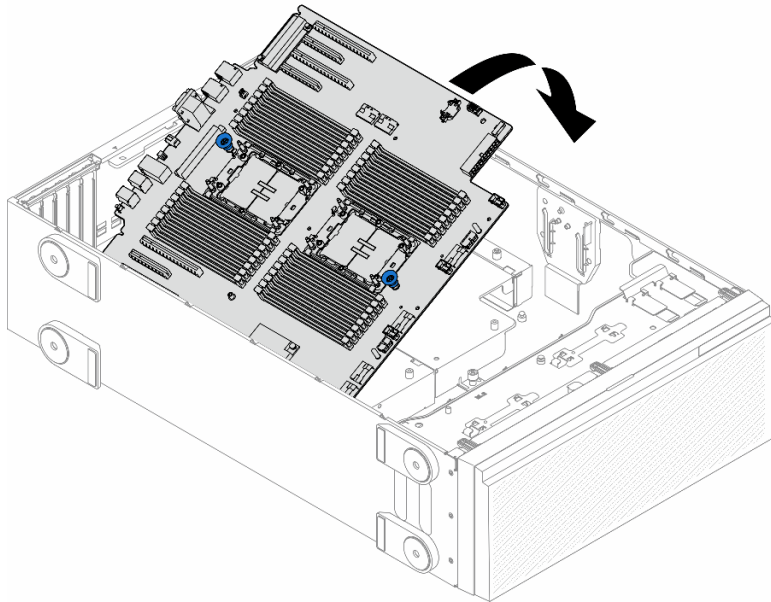
図 123. システム・ボードの取り付け
