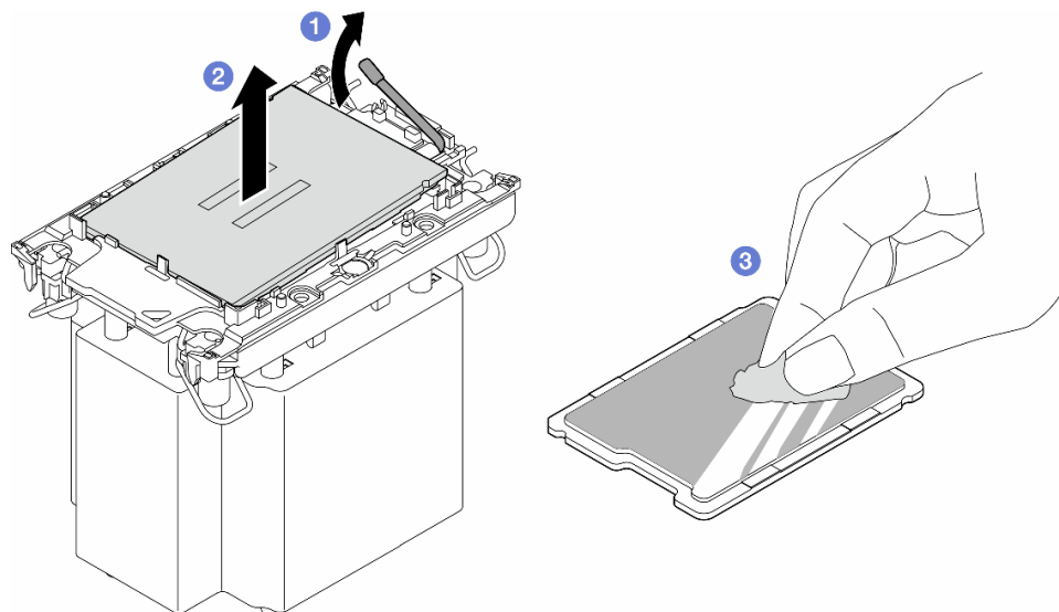
図 108. プロセッサをキャリアとヒートシンクから取り外す
