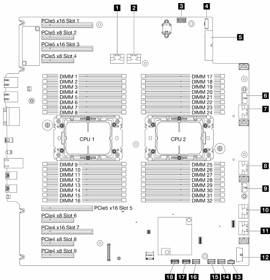
図 131. システム・ボード・コネクタ
