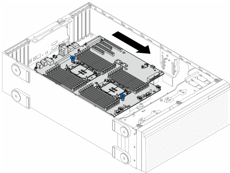
図 121. システム・ボードのシャーシからの取り外し
