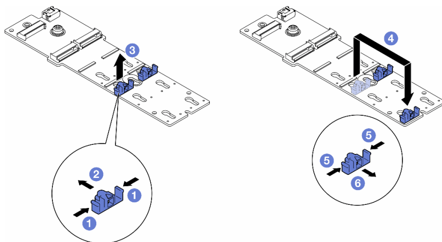
図 63. M.2 保持具の調整
