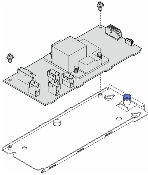
図 54. 内部 CFF アダプターのトレイへの取り付け
