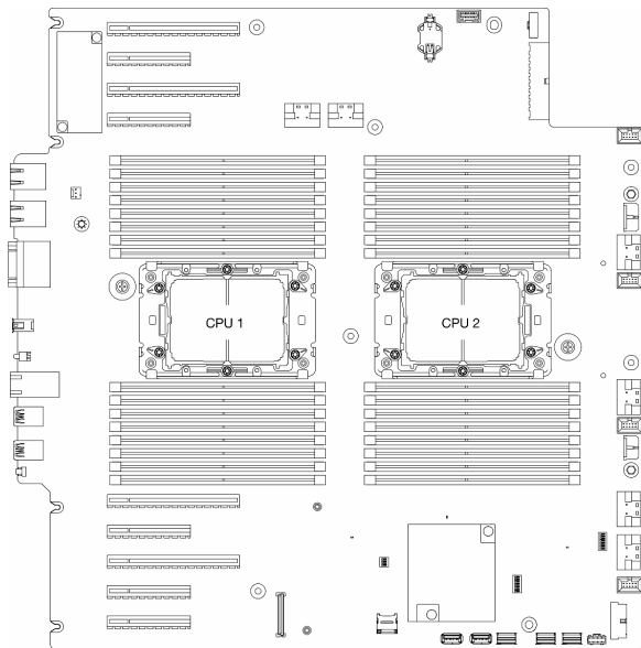
図 105. システム・ボード上のプロセッサの位置
