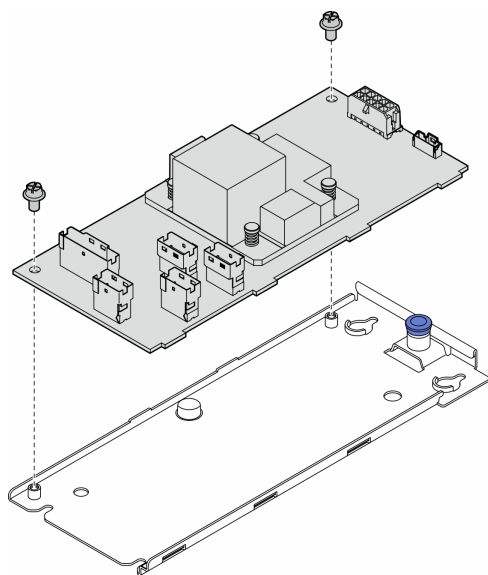
図 52. 内部 CFF アダプターのトレイからの取り外し
