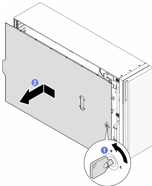
図 129. サーバー・カバーの取り外し
