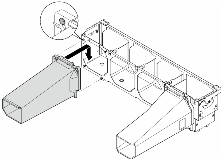
図 17. A2/L4 エアー・ダクトの取り付け
