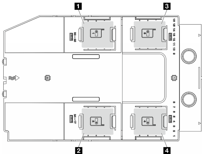
図 37. フラッシュ電源モジュール・スロットの位置
