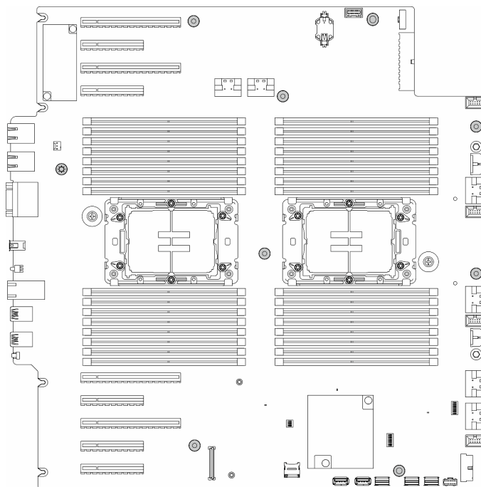
図 125. システム・ボードのねじの取り付け
