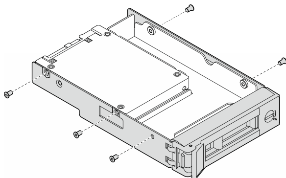
図23. 2.5型ドライブおよびドライブ・アダプターを固定しているねじの取り外し
