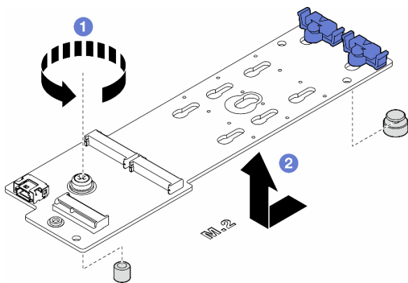
図 60. M.2 ブート・アダプターの取り外し
