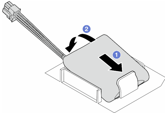
図 39. フラッシュ電源モジュールの取り付け
