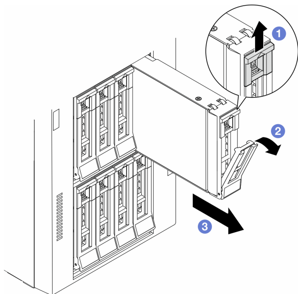
図22. トレイ・ハンドルを開く
