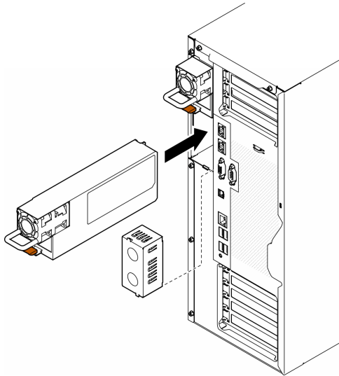
図104. パワー・サプライ・ユニットまたは PSU フィラーの取り付け
