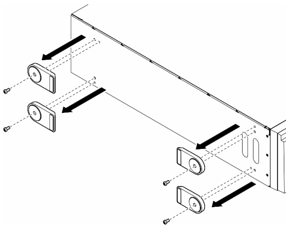
図41. 脚部スタンドの取り外し
