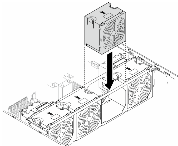
図34. ファン・モジュールの取り付け
