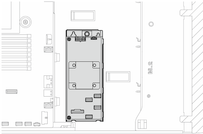
図 50. 内部 CFF アダプターの位置
