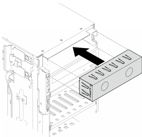
図 85. ドライブ・ベイ・フィラーの取り付け
