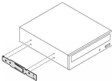
図 81. 光学式ドライブ保持具の取り付け
