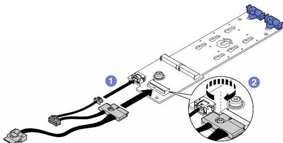
図 62. M.2 信号ケーブルの取り付け
