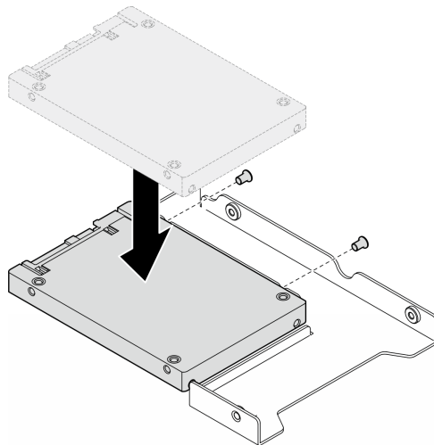
図 25. 2.5 型ドライブのドライブ・アダプターへの取り付け
