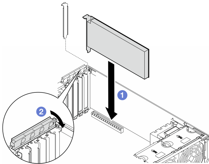
図94. HL PCIe アダプターの取り付け
