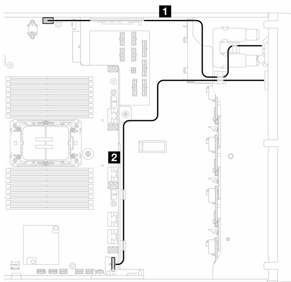
図 139. 前面入出力モジュールのケーブル配線
