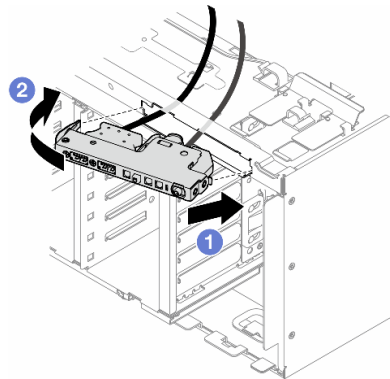
図 47. 前面出入力モジュールの取り付け
