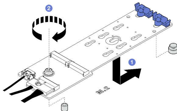
図61. M.2 ブート・アダプターの取り付け
