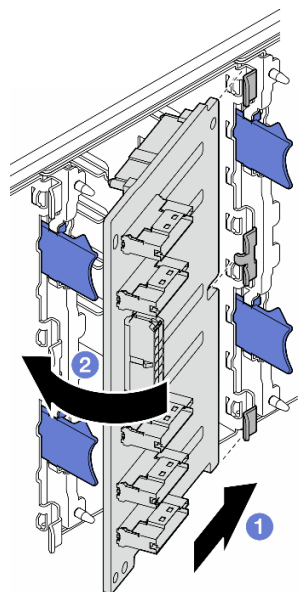
図13. 2.5型ドライブ・バックプレーンの取り付け
