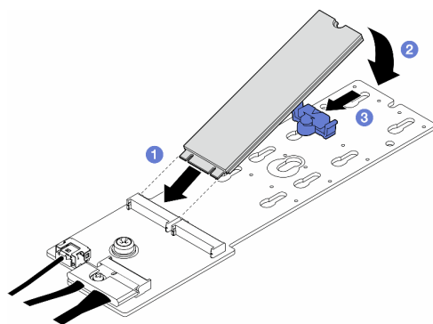
図 65. M.2 ドライブの取り付け
