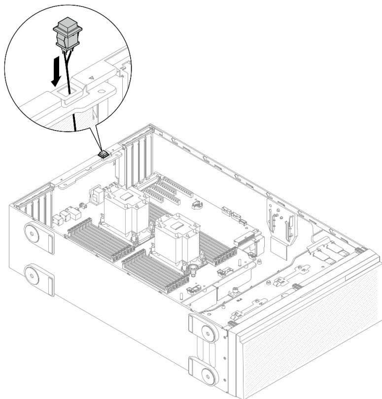
図 57. 侵入検出スイッチの取り付け
