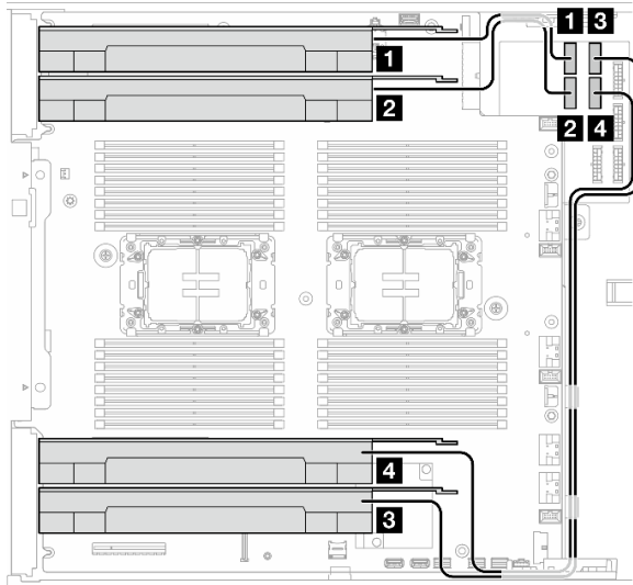
図 138. GPU のケーブル配線
