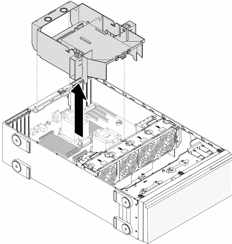
図 18. エアール・バッフルの取り外し
