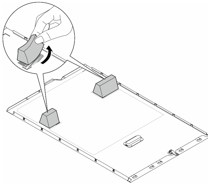
図 126. T4 フィラーの取り外し
