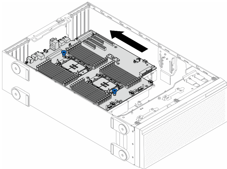
図 124. システム・ボードのシャーシへの取り付け
