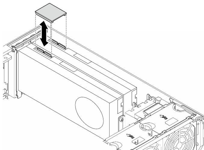
図 71. NVLink ブリッジの取り付け
