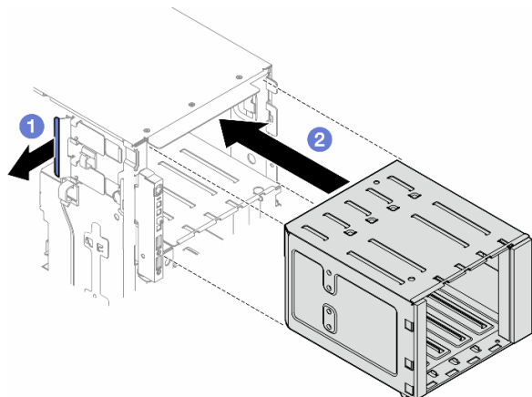
図 29. 拡張ドライブ・ケージの取り付け
