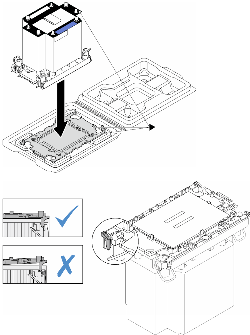
図 114. 配送用トレイのプロセッサーで PHM を取り付けます。
