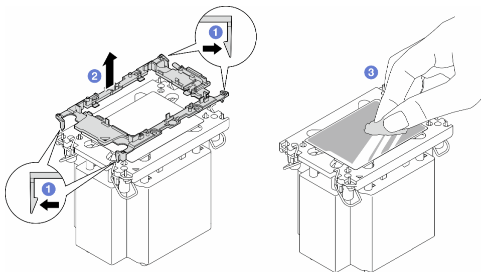
図 109. ヒートシンクからプロセッサ・キャリアを取り外す
