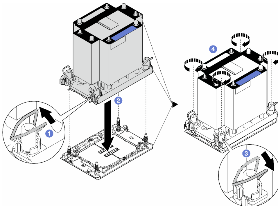
図 115. 標準 PHM の取り付け
