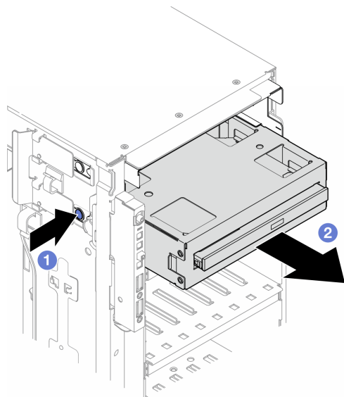
図 83. 5.25 型ドライブ・ベイ・アダプター・アセンブリーの取り外し
