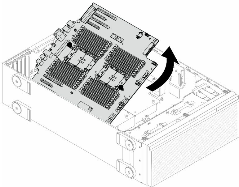
図 122. システム・ボードの取り外し
