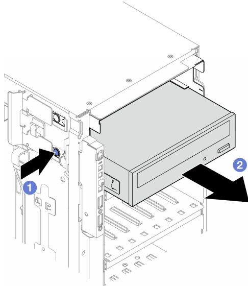
図74. 光学式ドライブの取り外し
