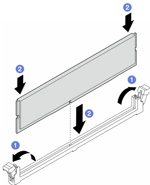
図 67. メモリー・モジュールの取り付け
