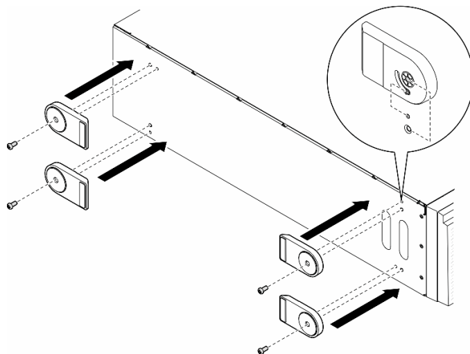
図 42. 脚部スタンドの取り付け
