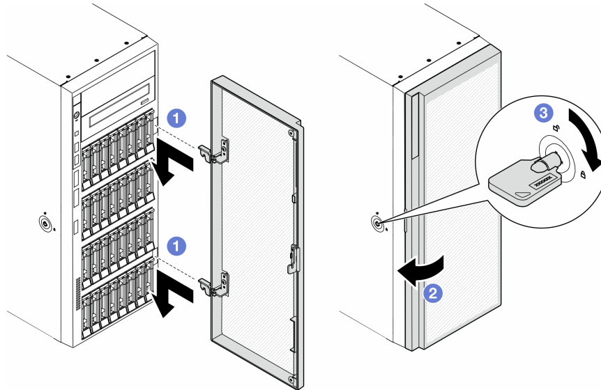
図 119. セキュリティー・ドアの取り付け
