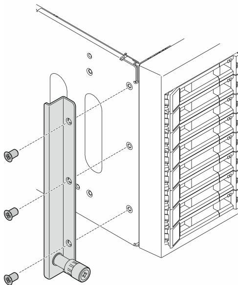
図4. 左側の EIA ブラケットの取り外し
