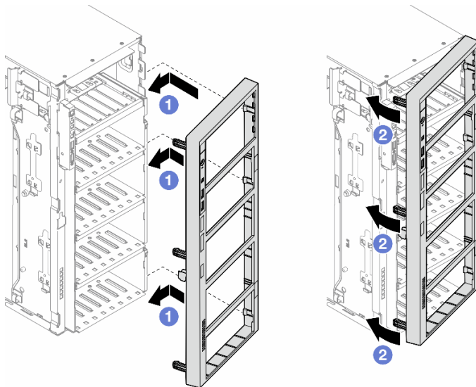
図 45. 前面ベゼルの取り付け
