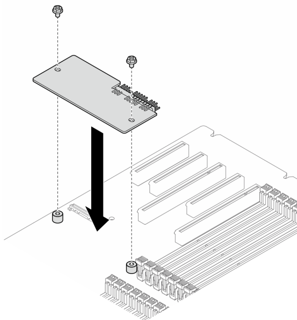
図117. ファームウェアおよびRoTセキュリティー・モジュールの取り付け
