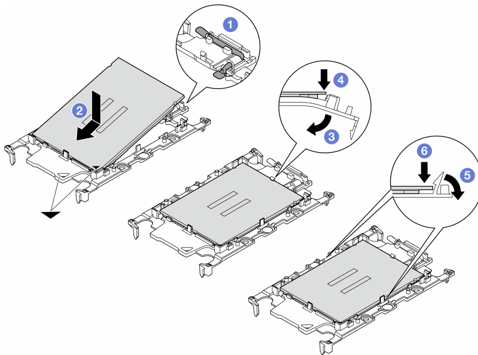
図 112. プロセッサ・キャリアの取り付け
