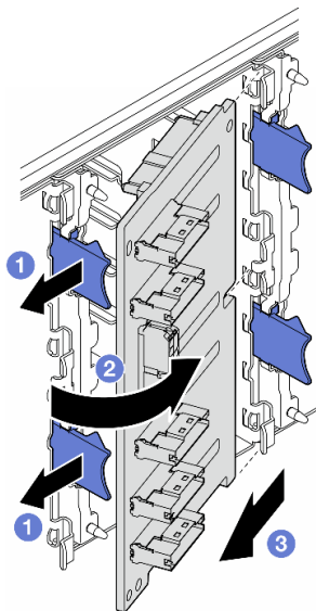
図 12. 2.5 型ドライブ・バックプレーンの取り外し
