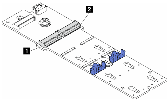
図 64. M.2 アダプター上の M.2 ドライブ・スロット
