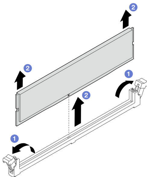
図 66. メモリー・モジュールの取り外し
