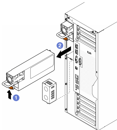
図 102. パワー・サプライ・ユニットまたは PSU フィラーの取り外し
