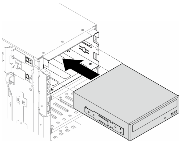
図 82. 光学式ドライブ・ケージの取り付け
