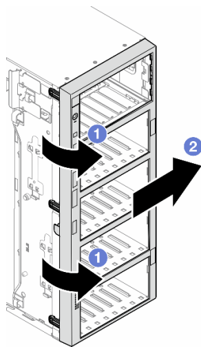
図 44. 前面ベゼルの取り外し
