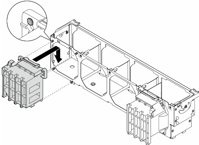
図 92. FL PCIe アダプター・ホルダーの取り付け
