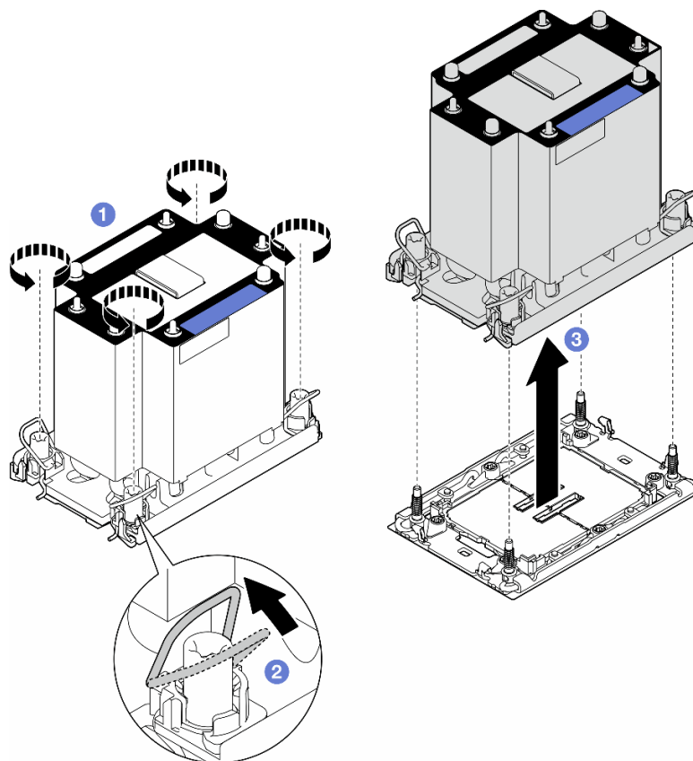
図 107. PHM の取り外し
