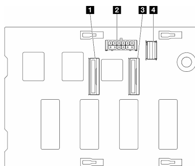
図 135. 3.5 型 SAS/SATA/NVMe および NVMe 4 ベイ・バックプレーン・コネクタ
