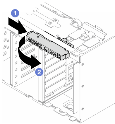
図 46. 前面 I/O モジュールの取り外し
