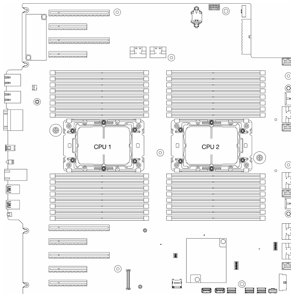
図110. システム・ボード上のプロセッサの位置
