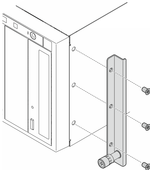
図7. 右側の EIA ブラケットの取り付け
