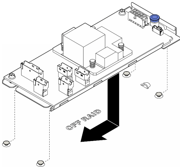
図 55. 内蔵 CFF アダプターの取り付け
