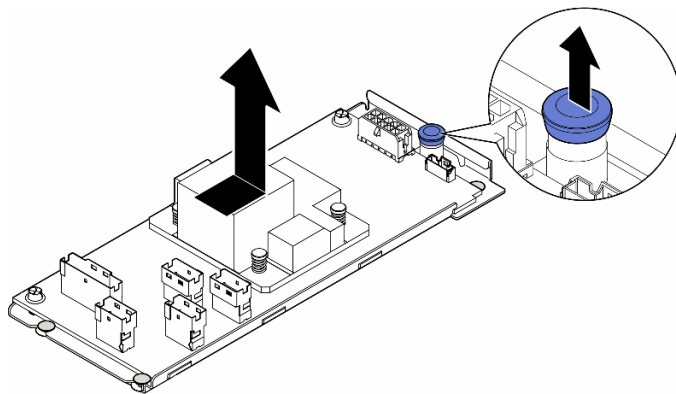
図 51. 内部 CFF アダプターの取り外し
