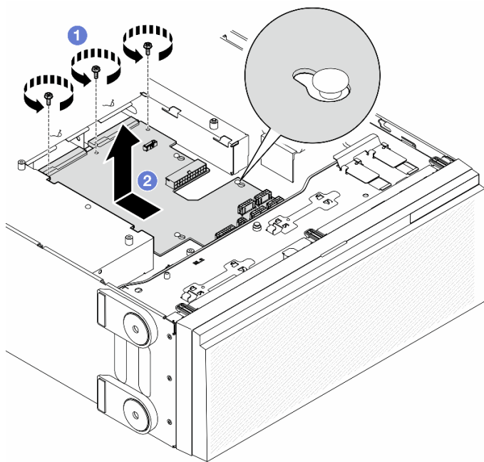
図97. 分電盤の取り外し
