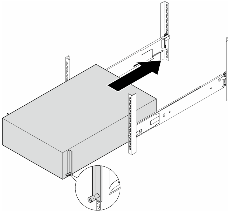
図 11. サーバーをラックに取り付ける
