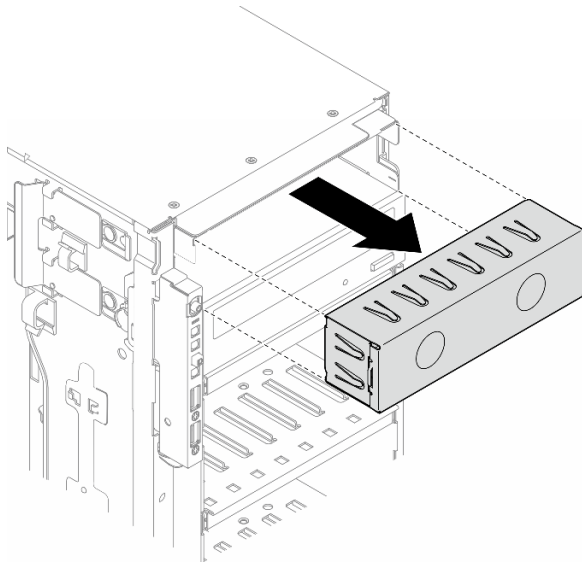
図88. ドライブ・フィラー・カバーの取り外し
