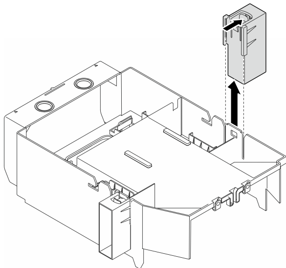
図 48. FL GPU フィラーの取り外し
