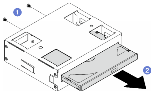
図 84. 光学式スリム・ドライブのドライブ・ベイ・アダプターからの取り外し
