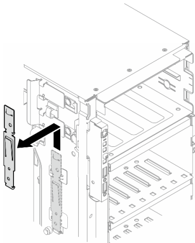
図 80. ドライブ保持具の取り外し
