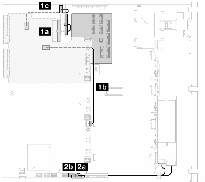
図 140. 分電盤および M.2 アダプターのケーブル配線
