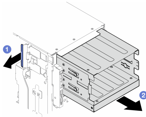
図 72. 光学式ドライブ・ケージの取り外し
