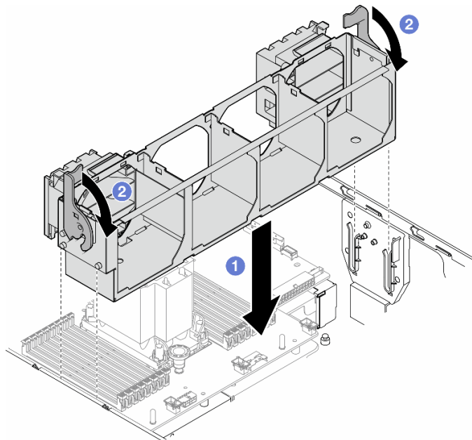
図32. ファン・ケージ・アセンブリーの取り付け
