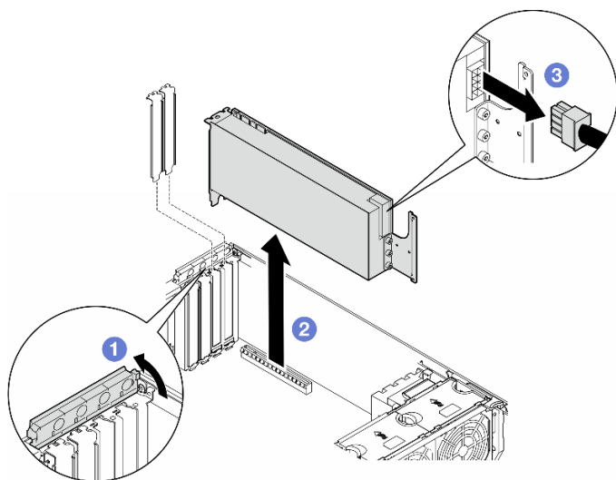
図 95. FL GPU アダプターの取り外し
