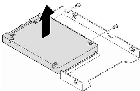
図 24. 2.5 型ドライブのドライブ・アダプターからの取り外し
