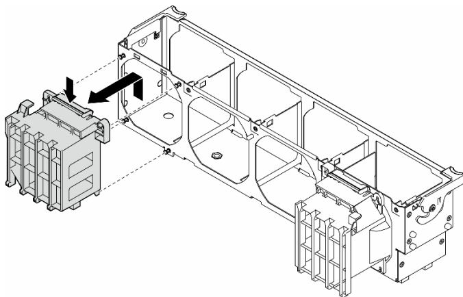
図 91. PCIe アダプター・ホルダーの取り外し
