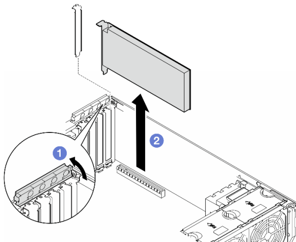
図 93. PCIe アダプターの取り外し
