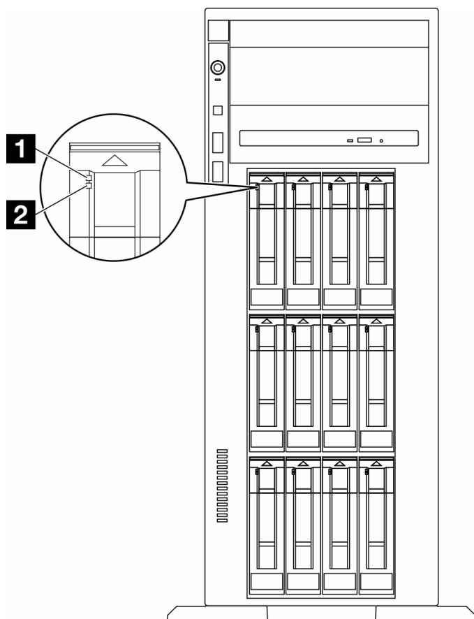
図10. ドライブ LED
