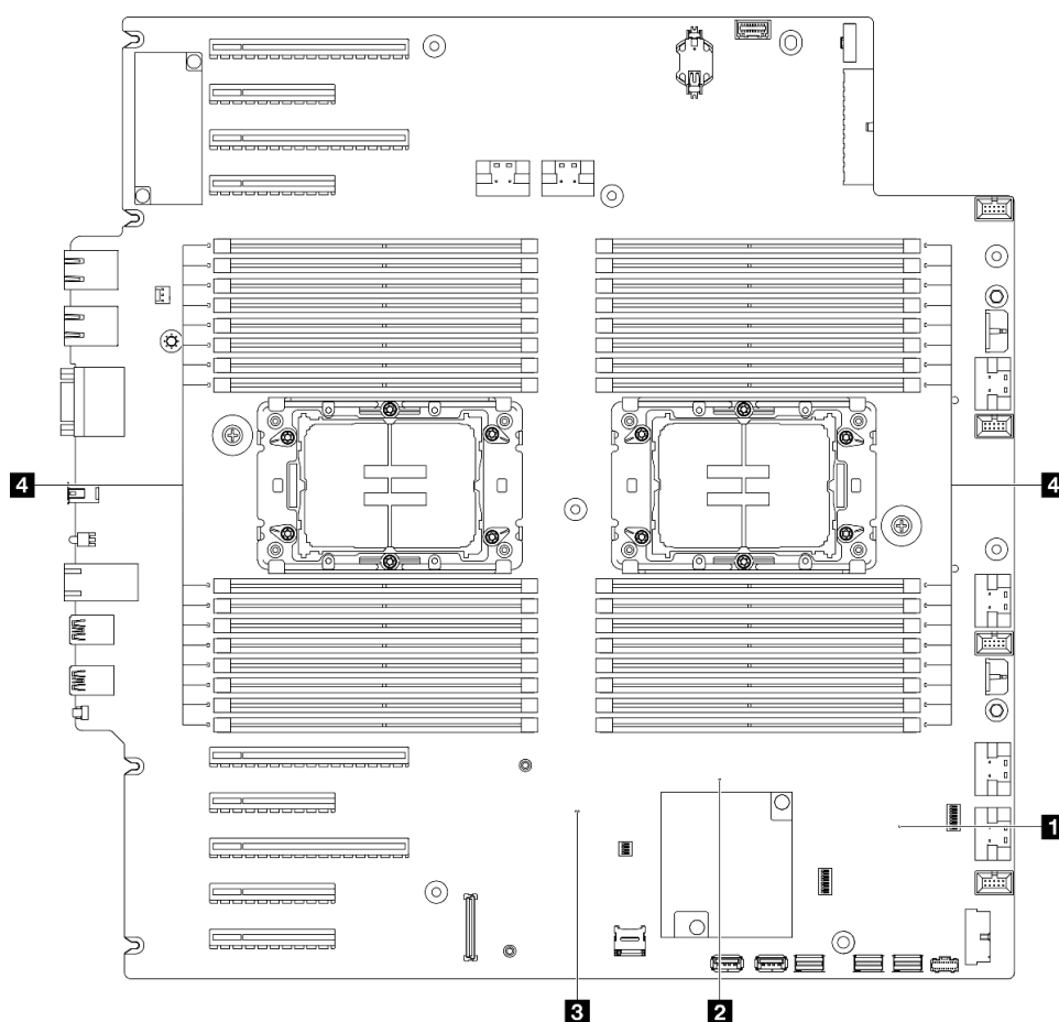
図 13. システム・ボード LED
