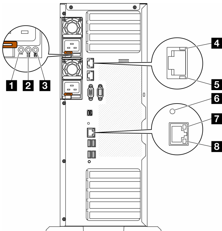
図 12. サーバーの背面システム LED
