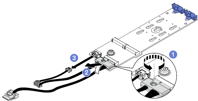
图 66. 从 ThinkSystem M.2 SATA/NVMe 2-Bay Enablement Kit 或 ThinkSystem M.2 NVMe 2-Bay RAID Enablement Kit 上拔下 M.2 线缆
