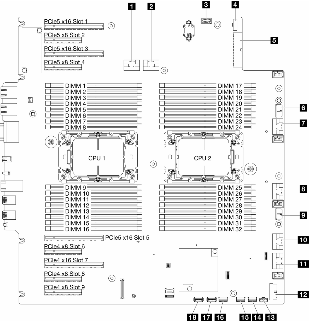
图 144. 主板接口
