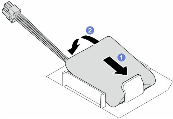
图 46. 安装快速充电模块
