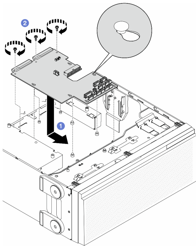
图 112. 安装配电板
