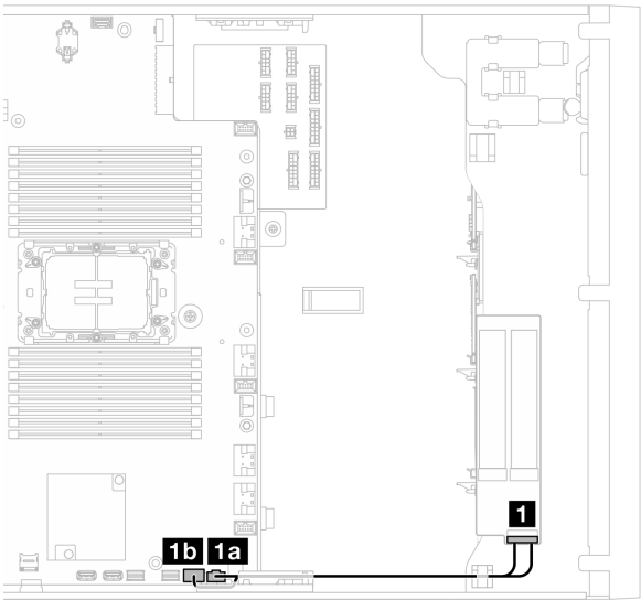
图 156. ThinkSystem M.2 NVMe 2-Bay RAID Enablement Kit 线缆布放
