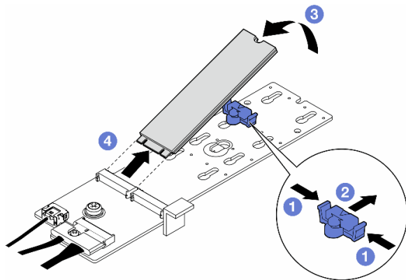
图 65. 卸下 M.2 硬盘
