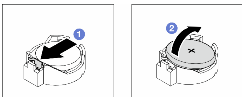
图 27. 卸下 CMOS 电池
