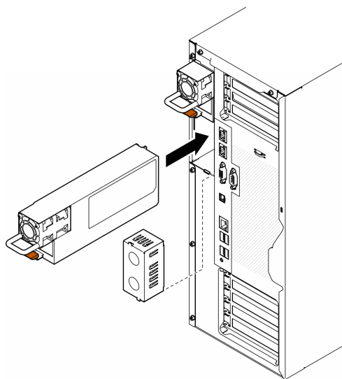
图 117. 安装电源模块单元或 PSU 填充件
