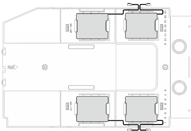
图 45. 快速充电模块线缆布放
