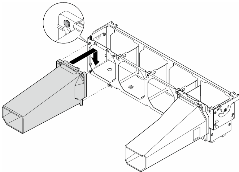
图 24. 安装 A2/L4 GPU 导风管
