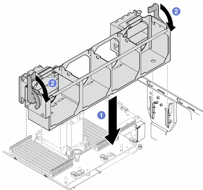
图 39. 安装风扇架组合件
