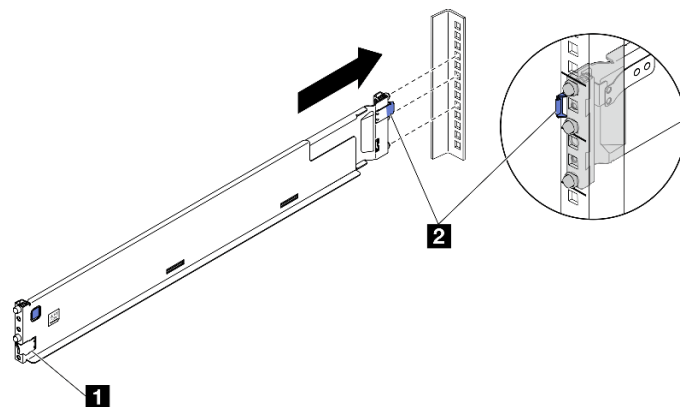
图 14. 安装导轨后端
