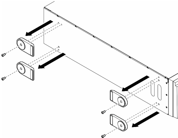
图 48. 卸下支脚
