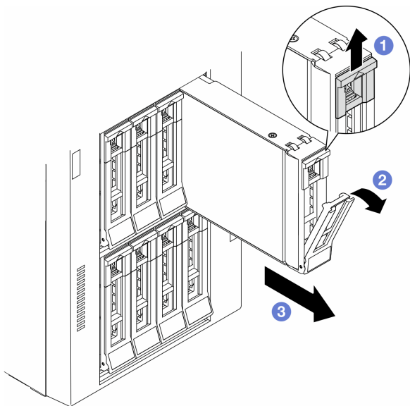
图 29. 打开托盘手柄
