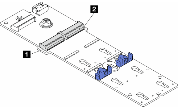
图 73. M.2 适配器上的 M.2 硬盘插槽
