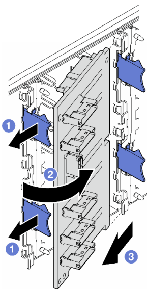
图 19. 卸下 2.5 英寸硬盘背板
