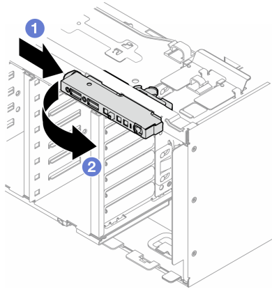
图 53. 卸下正面 I/O 模块
