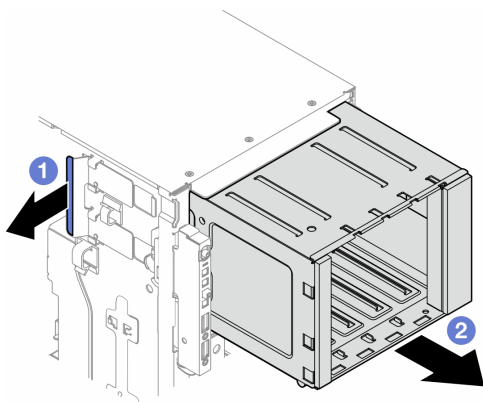
图 35. 卸下扩展硬盘仓
