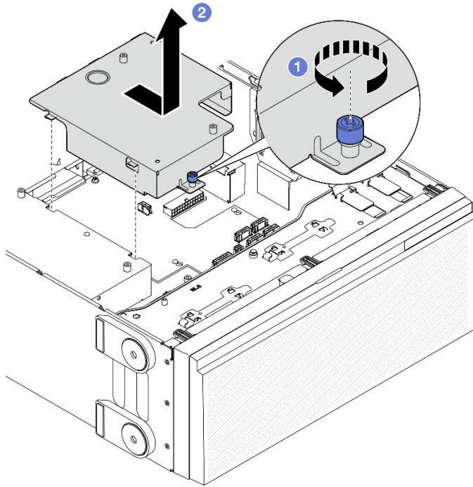
图 110. 卸下配电板外盖
