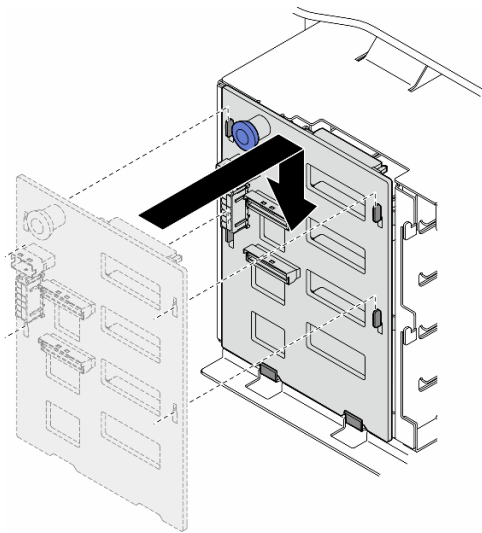
图 22. 安装 3.5 英寸硬盘背板
