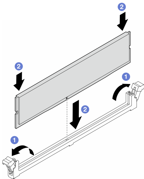
图 78. 安装内存条
