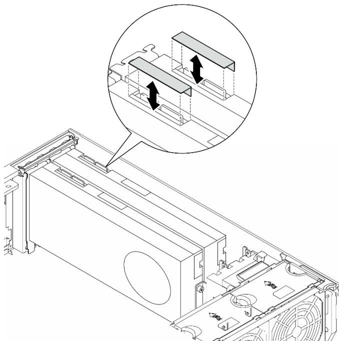
图 83. 卸下 NVLink 盖
