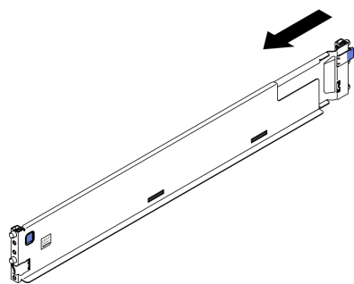
图 13. 缩短导轨
