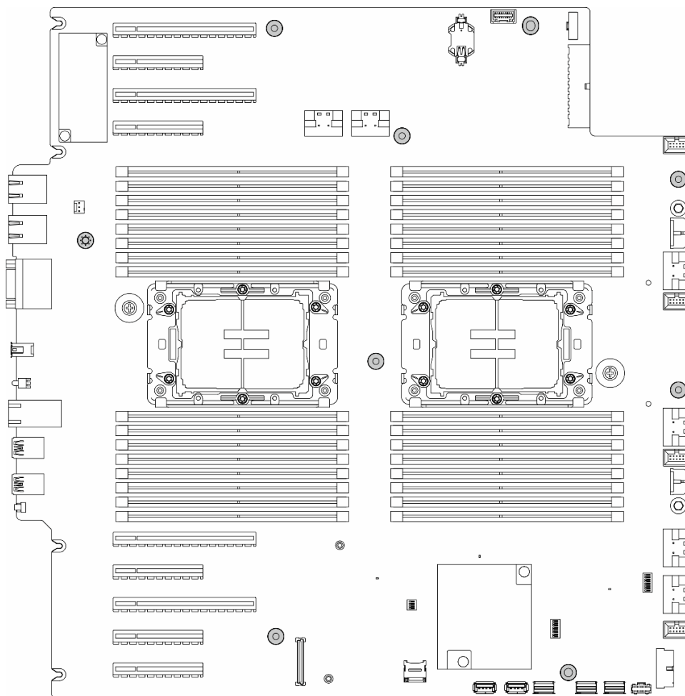
图 138. 安装主板螺钉
