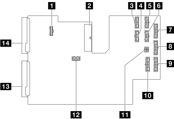
图 145. 配电板上的接口
