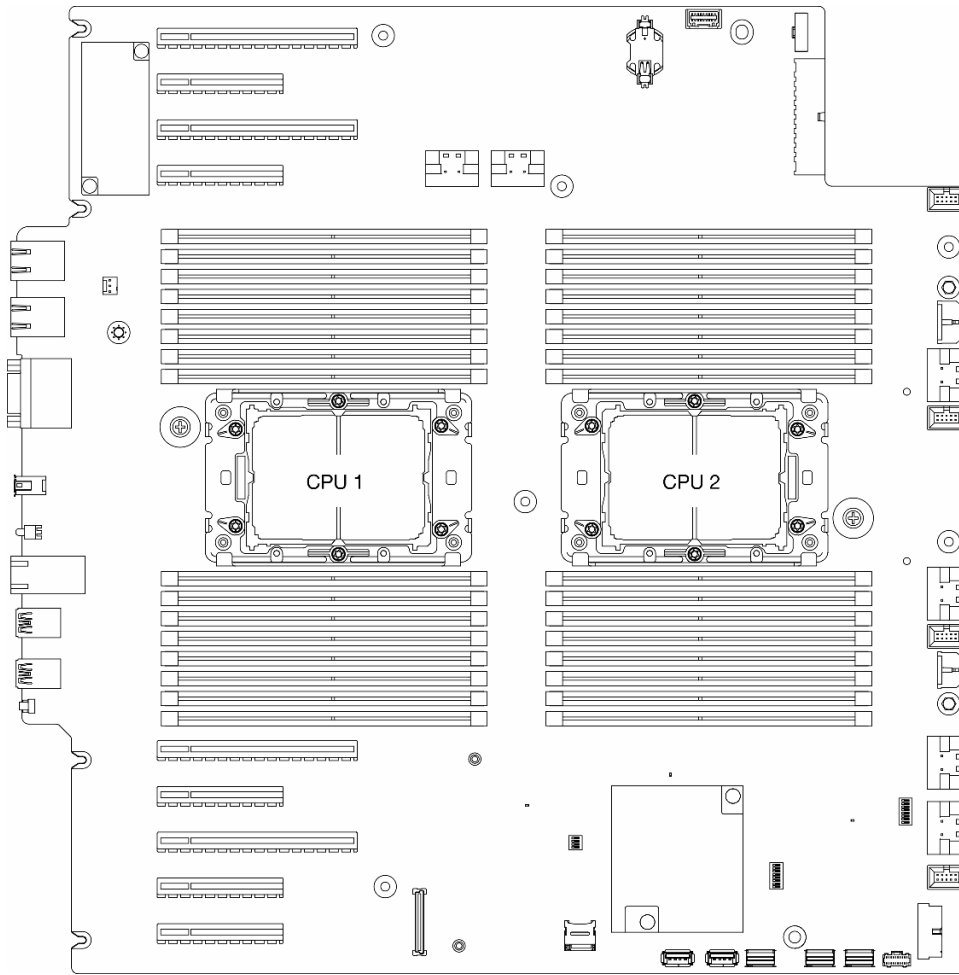
图 118. 主板上的处理器位置
