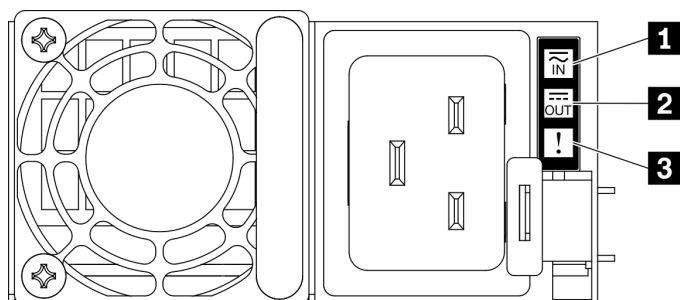
图 165. 电源模块 LED
