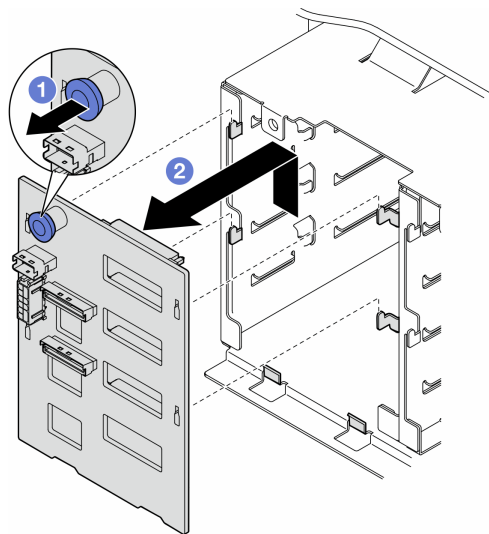
图 21. 卸下 3.5 英寸硬盘背板
