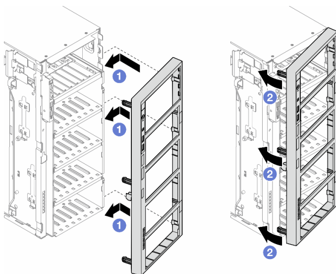
图 52. 安装前挡板
