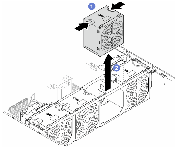
图 37. 卸下风扇模块
