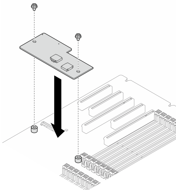
图 132. 安装固件和 RoT 安全模块
