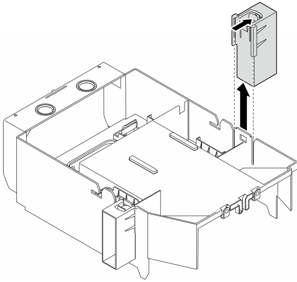
图 55. 卸下 FL GPU 填充件
