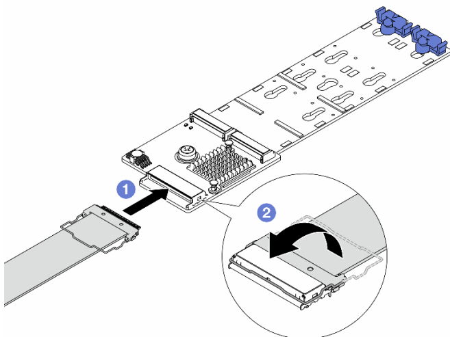
图 71. 将 M.2 线缆连接到 ThinkSystem M.2 NVMe 2-Bay RAID Enablement Kit
