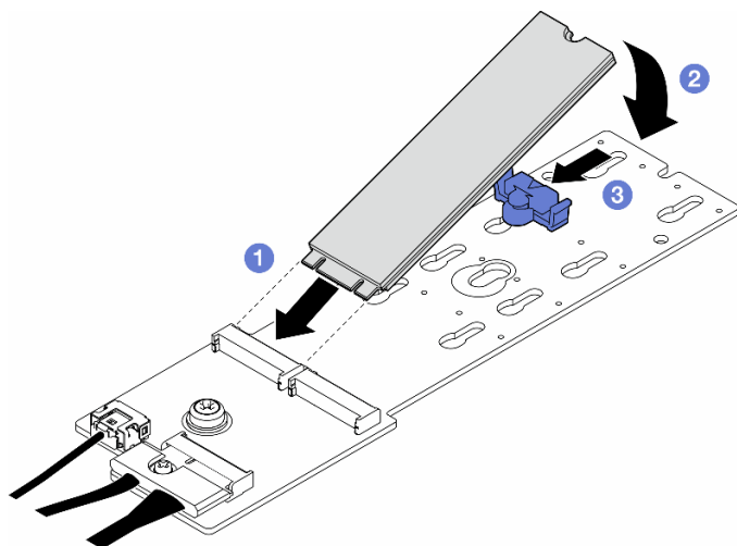
图 74. 安装 M.2 硬盘
