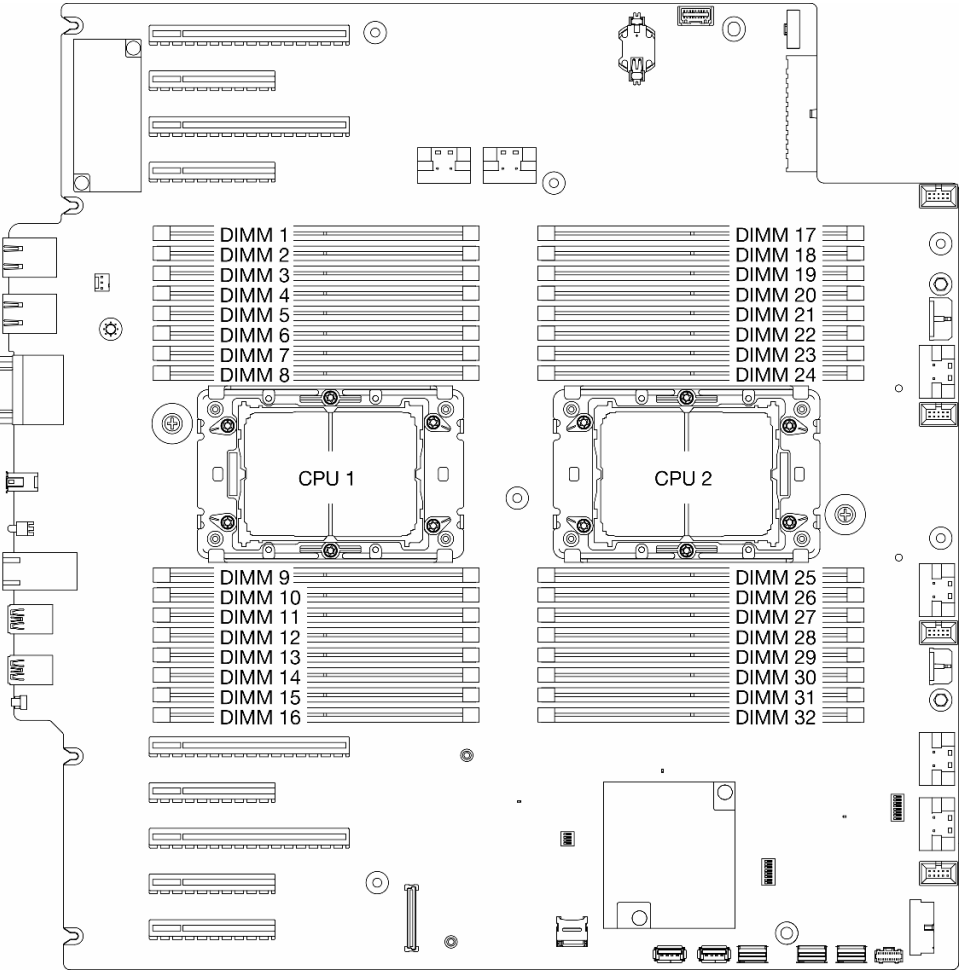
图 1. 内存条和处理器布局
