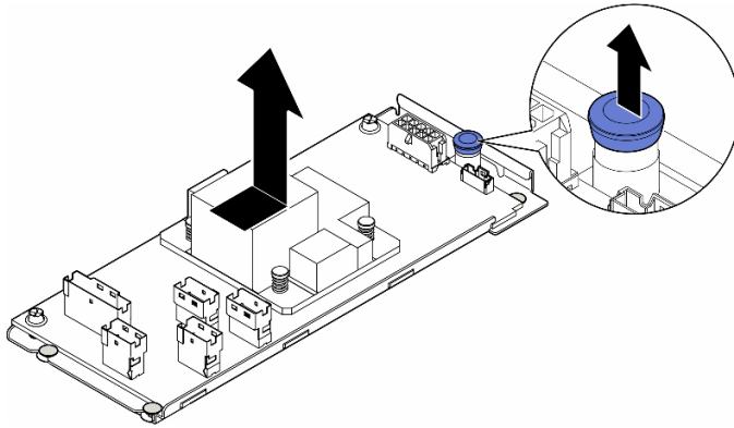
图 58. 卸下内部 CFF 适配器
