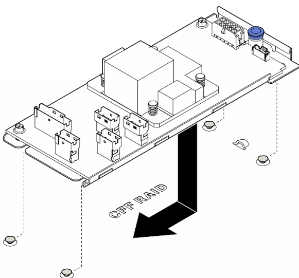
图 62. 安装内部 CFF 适配器
