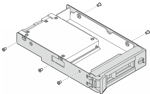
图 33. 安装用于固定 2.5 英寸硬盘和硬盘适配器的螺钉
