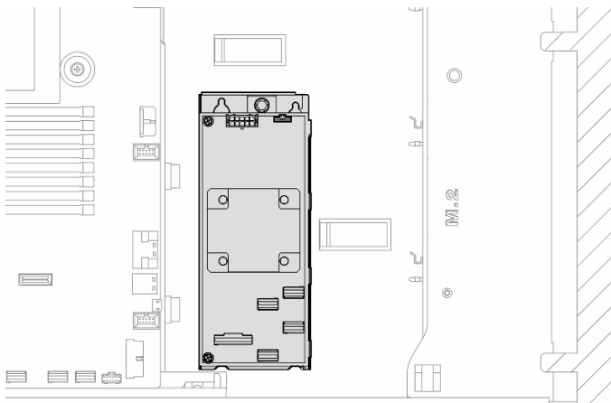
图 60. 内部 CFF 适配器的位置
