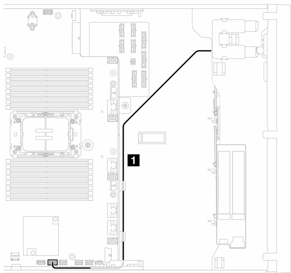
图 157. 光盘驱动器的线缆布放
