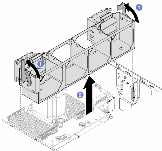
图 38. 卸下风扇架组合件
