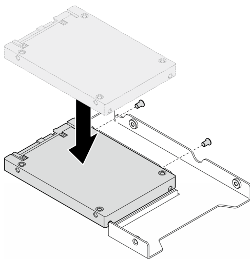
图 32. 将 2.5 英寸硬盘安装到硬盘适配器中
