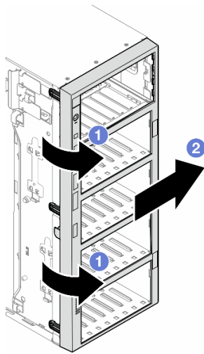
图 51. 卸下前挡板
