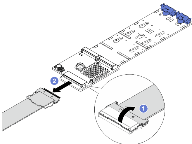
图 67. 从 ThinkSystem M.2 NVMe 2-Bay RAID Enablement Kit 上断开 M.2 线缆
