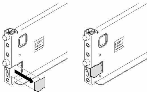
图 7. 卸下左滑锁盖
