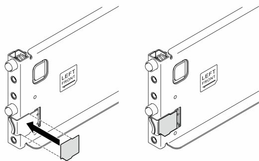
图 11. 安装左滑锁盖
