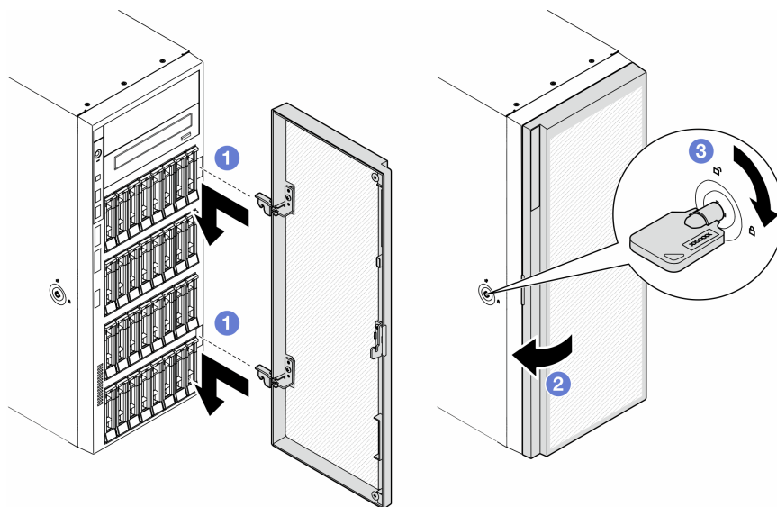
图 130. 安装安全门
