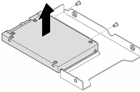
图 31. 从硬盘适配器上卸下 2.5 英寸硬盘
