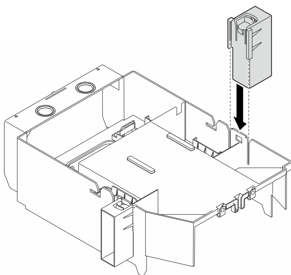
图 56. 安装 FL GPU 填充件
