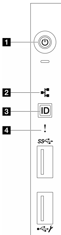
图 163. 正面操作员面板 LED
