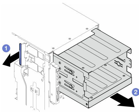
图 85. 卸下光盘驱动器仓
