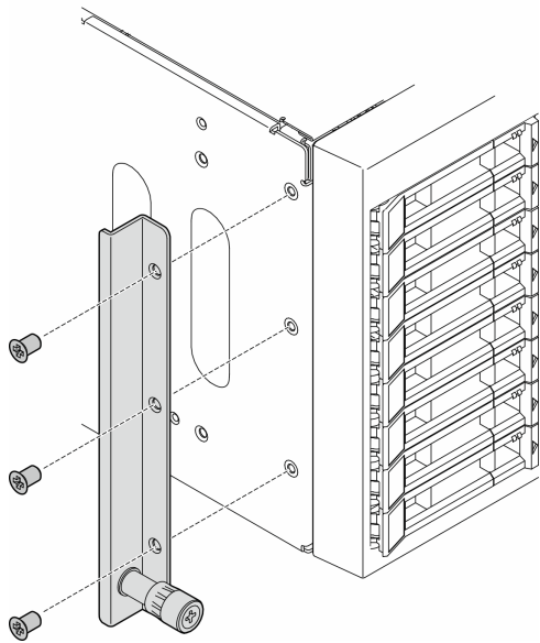
图 10. 安装左侧 EIA 支架
