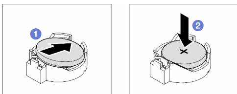
图 28. 安装 CMOS 电池
