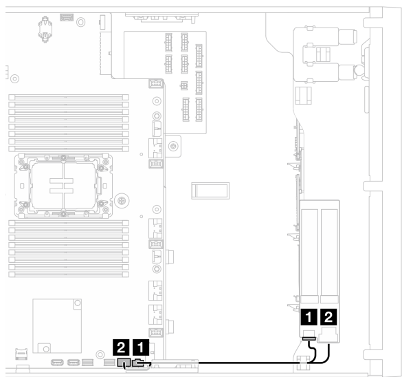
图 154. ThinkSystem M.2 SATA/NVMe 2-Bay Enablement Kit 线缆布放
