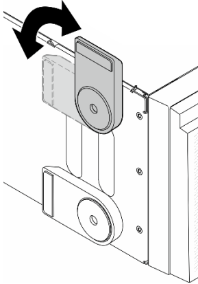
图 47. 调整支脚
