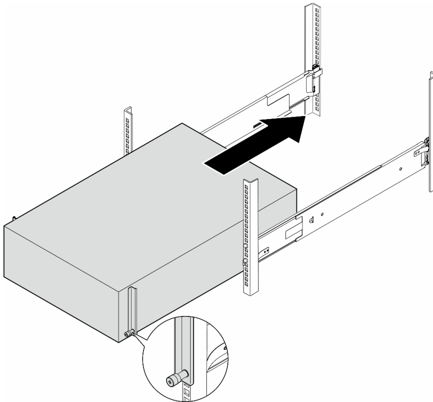
图 18. 将服务器安装到导轨上
