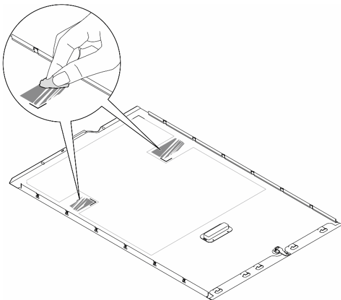
图 140. 清洁表面
