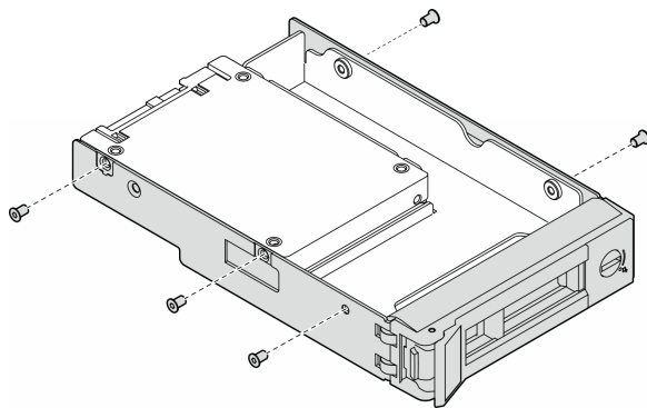
图 30. 卸下固定 2.5 英寸硬盘和硬盘适配器的螺钉
