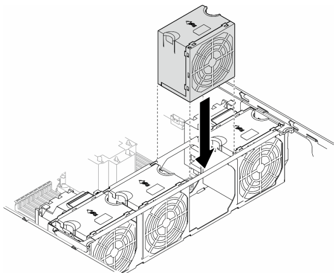
图 41. 安装风扇模块
