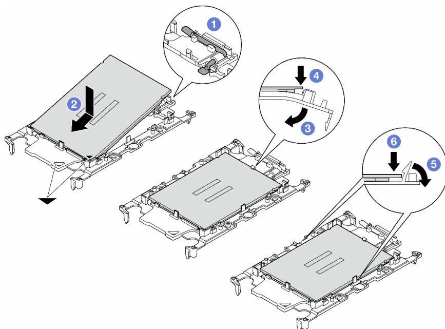
图 125. 安装处理器支架
