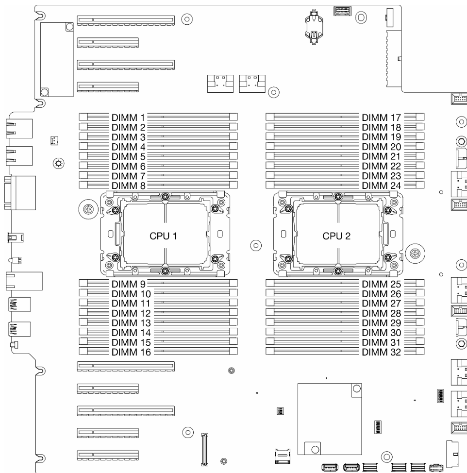
图 77. 内存条和处理器布局
