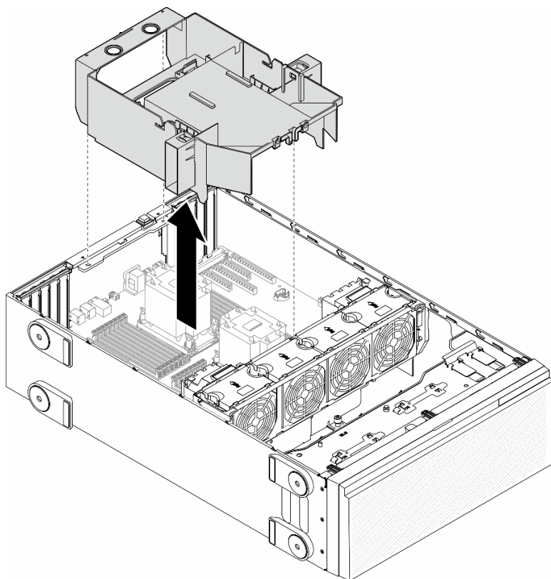
图 25. 卸下导风罩
