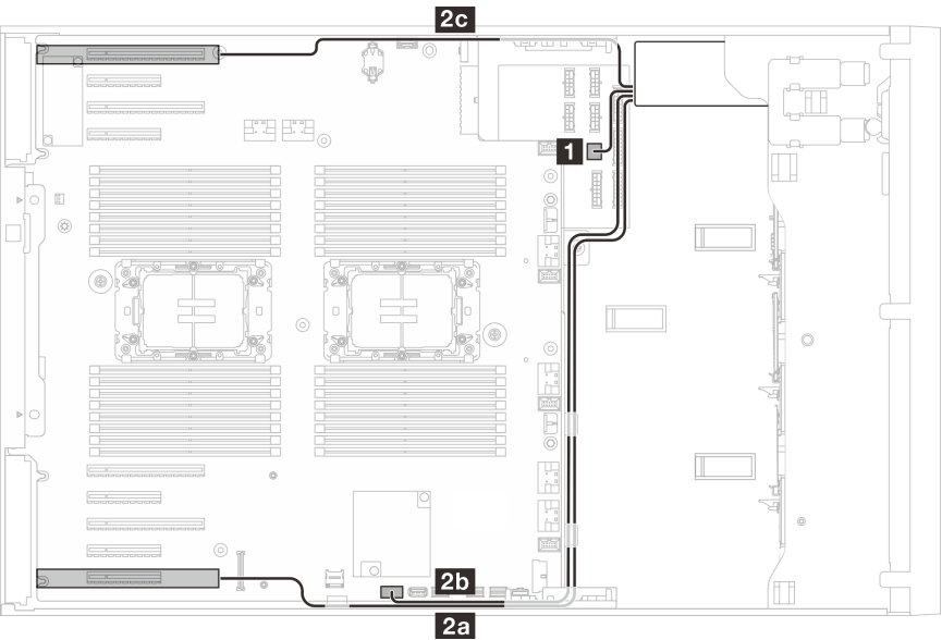
图 158. SAS/USB 磁带机的线缆布放
