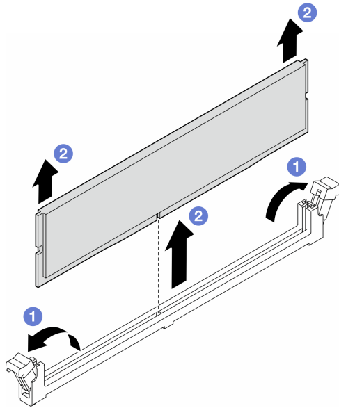
图 76. 卸下内存条
