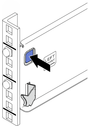
图 5. 从正面安装凸缘上松开导轨
