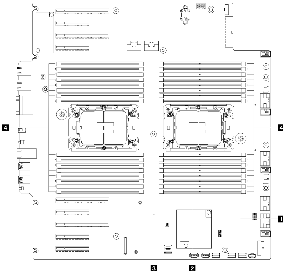
图 167. 主板 LED
