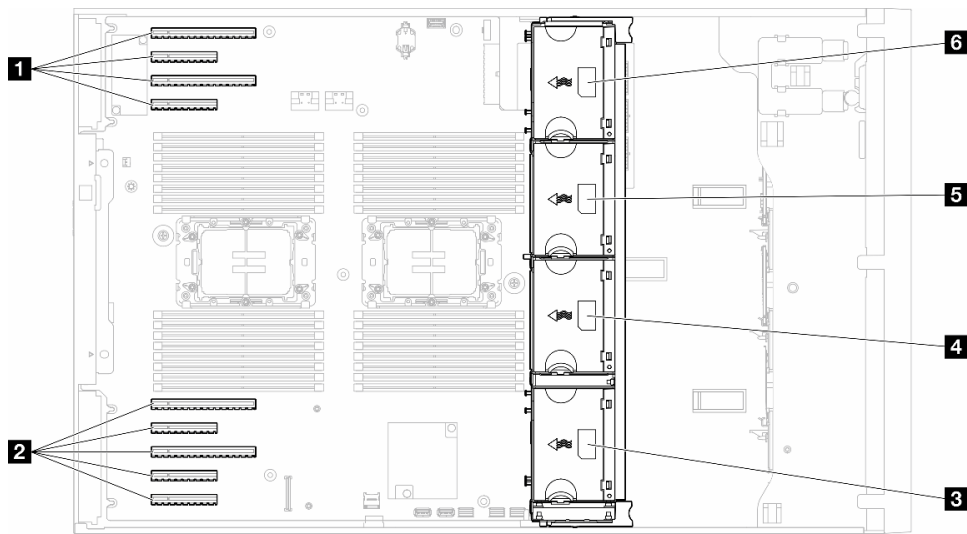
图 40. 风扇插槽位置
