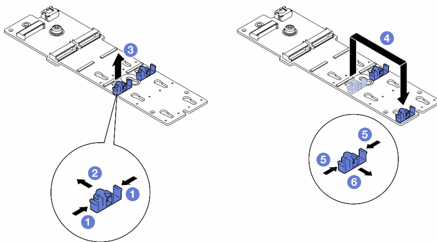
图 72. 调整 M.2 固定器
