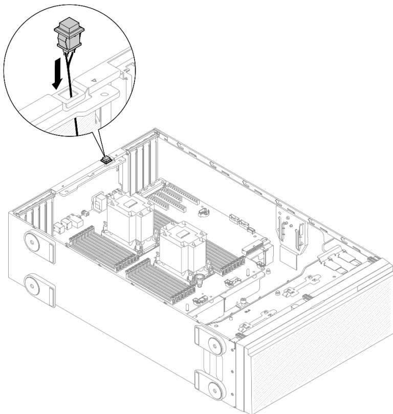
图 64. 安装入侵感应开关
