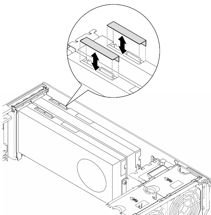
图 82. 安装 NVLink 盖
