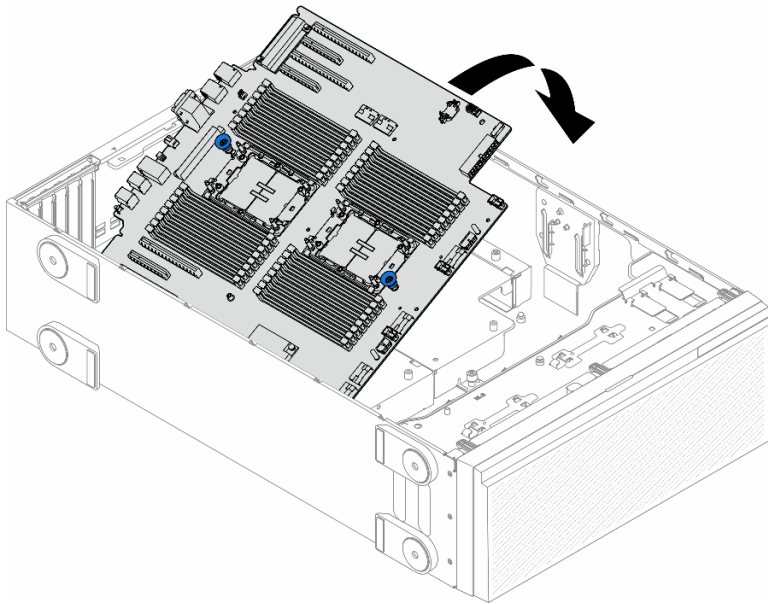
图 136. 安装主板
