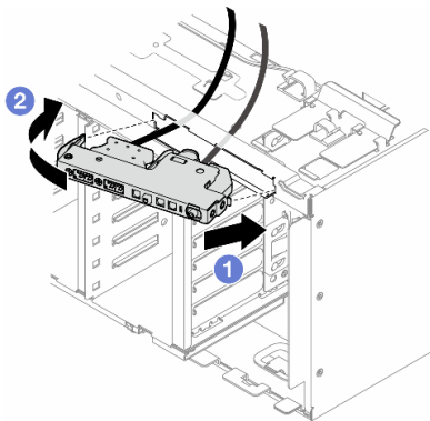
图 54. 安装正面 I/O 模块
