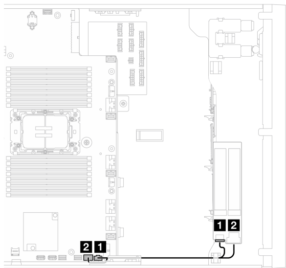
图 155. ThinkSystem M.2 NVMe 2-Bay RAID Enablement Kit 线缆布放
