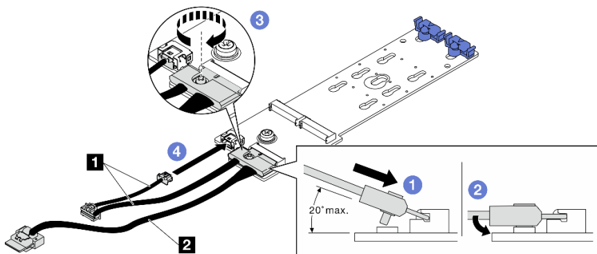
图 70. 将 M.2 线缆连接到 ThinkSystem M.2 SATA/NVMe 2-Bay Enablement Kit 或 ThinkSystem M.2 NVMe 2-Bay RAID Enablement Kit
