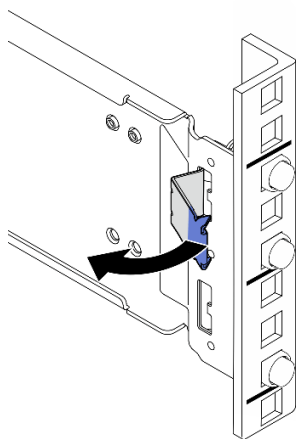
图 6. 从背面安装凸缘上松开导轨
