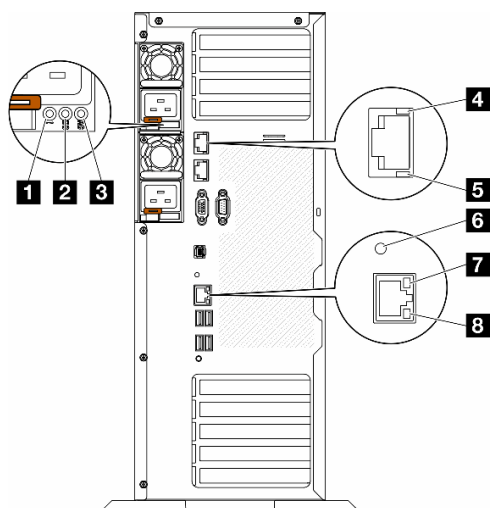
图 164. 服务器的背面系统 LED
