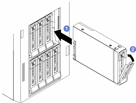
图 34. 安装热插拔硬盘
