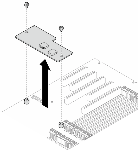
图 131. 卸下固件和 RoT 安全模块
