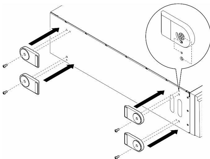
图 49. 安装支脚
