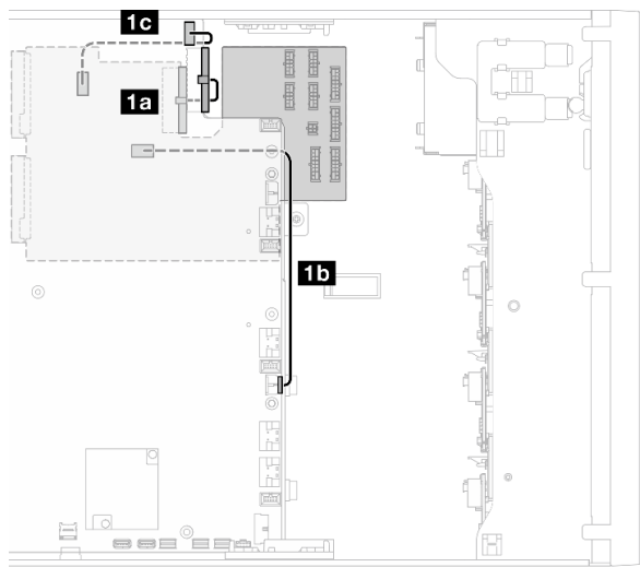
图 153. 配电板的线缆布放
