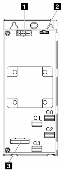
图 146. 内部 CFF RAID 适配器上的接口
