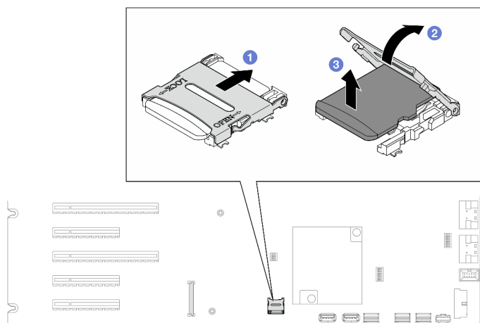
图 79. 卸下 MicroSD 卡
