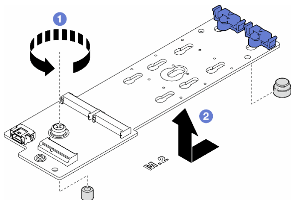
图 68. 卸下 M.2 引导适配器
