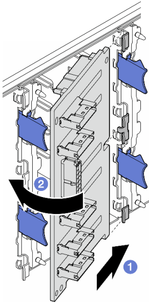
图 20. 安装 2.5 英寸硬盘背板
