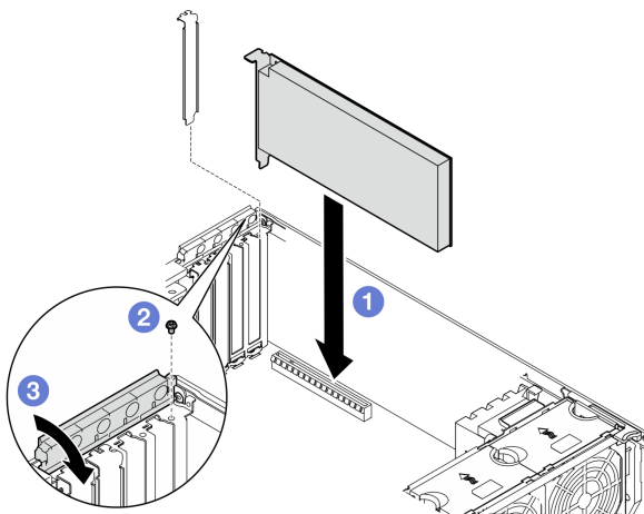
图 107. 安装 HL PCIe 适配器
