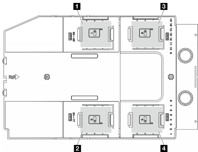
图 42. 快速充电模块插槽的位置
