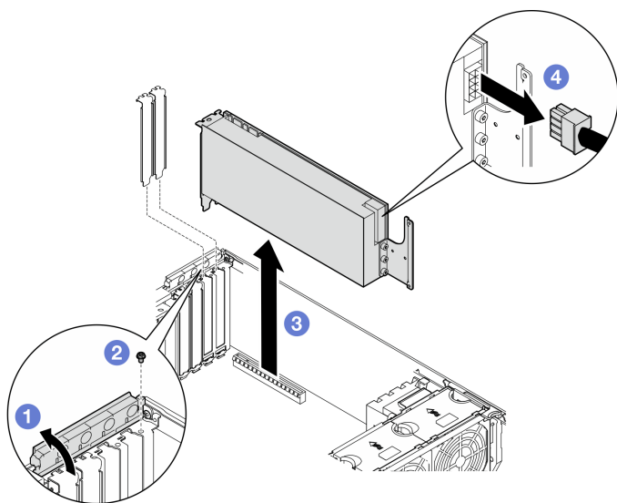
图 108. 卸下 FL GPU 适配器
