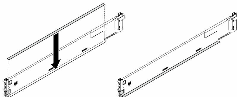
图 12. 贴附左侧导轨覆盖条
