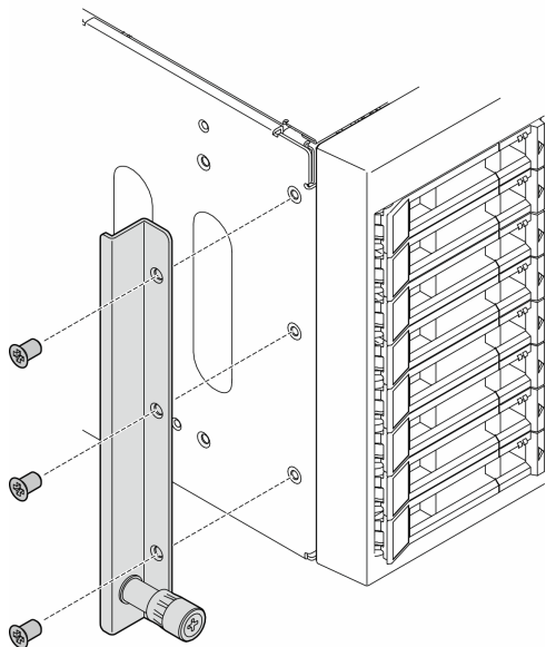
图 4. 卸下左侧 EIA 支架
