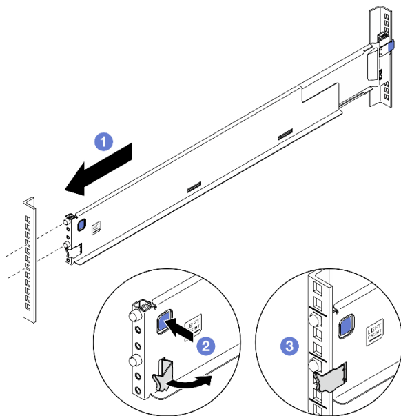
图 15. 安装导轨前端
