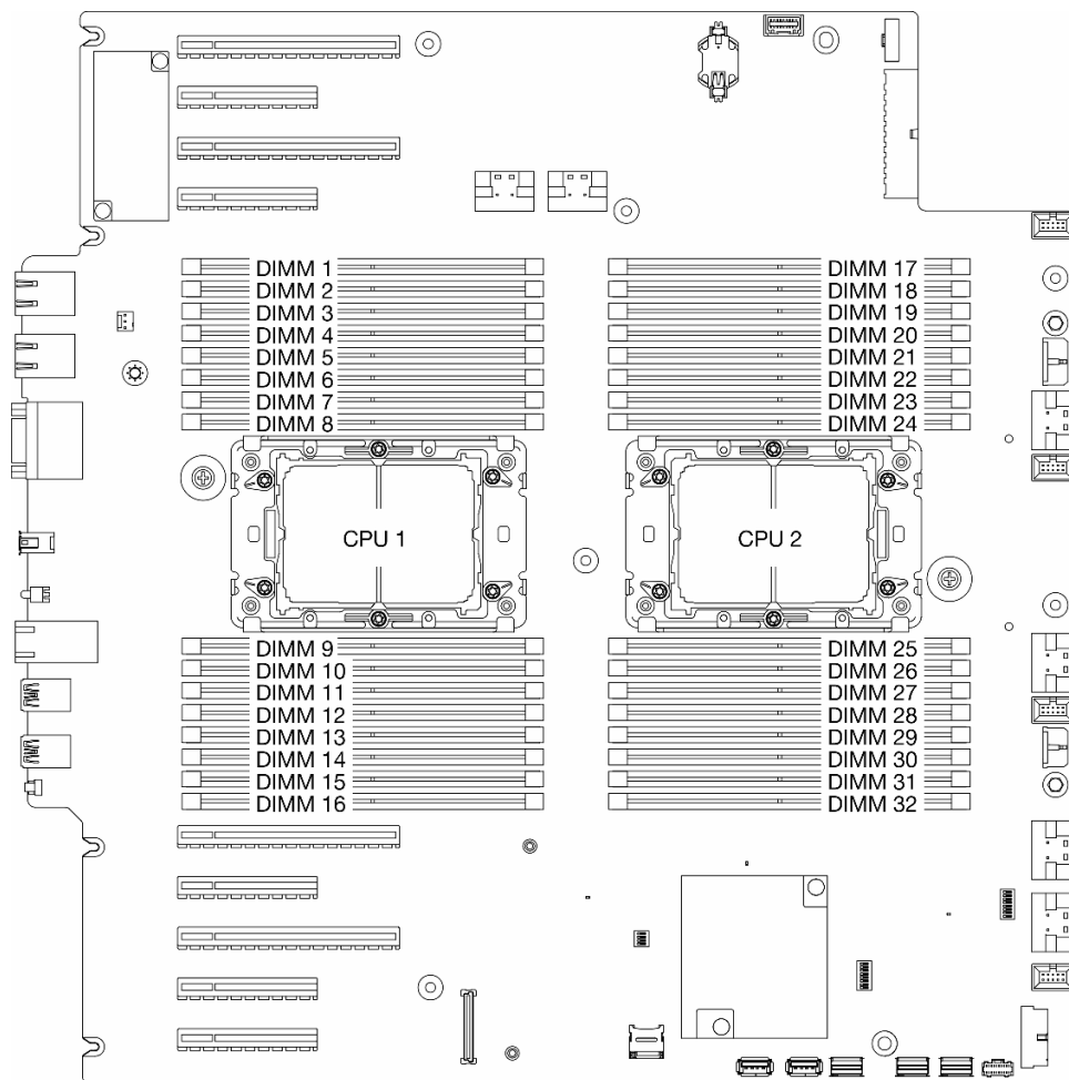
图 75. 内存条和处理器布局
