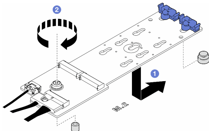
图 69. 安装 M.2 引导适配器
