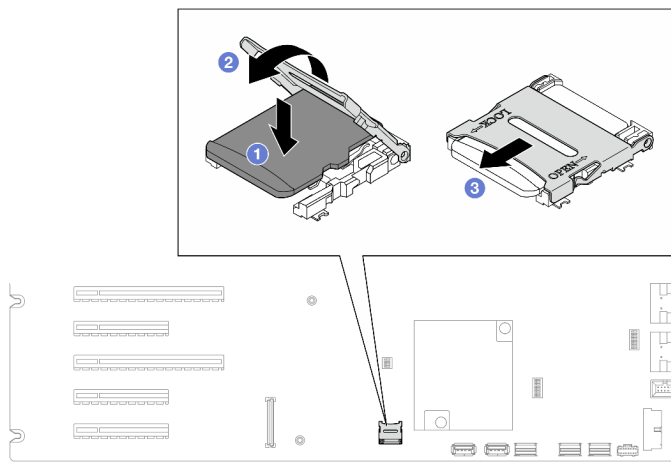
图 80. 安装 MicroSD 卡
