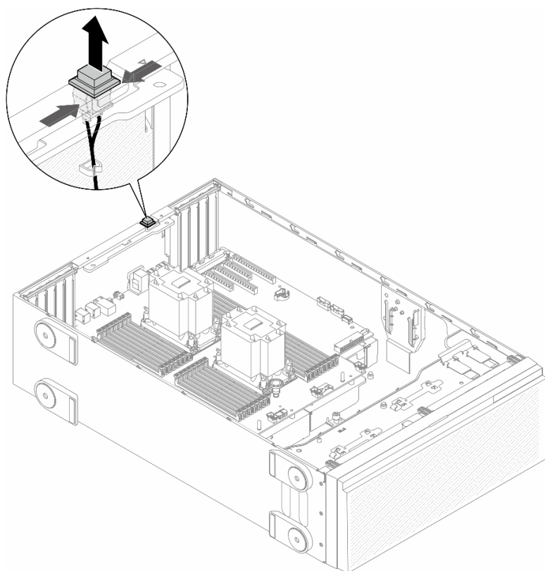
图 63. 卸下入侵感应开关
