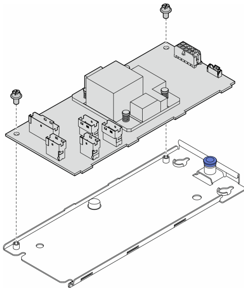
图 59. 将内部 CFF 适配器从其托盘上卸下
