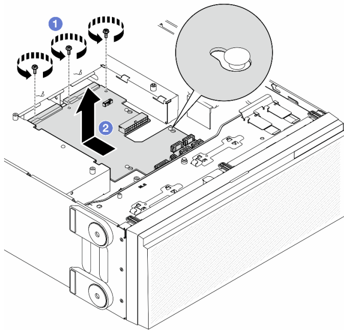
图 111. 卸下配电板
