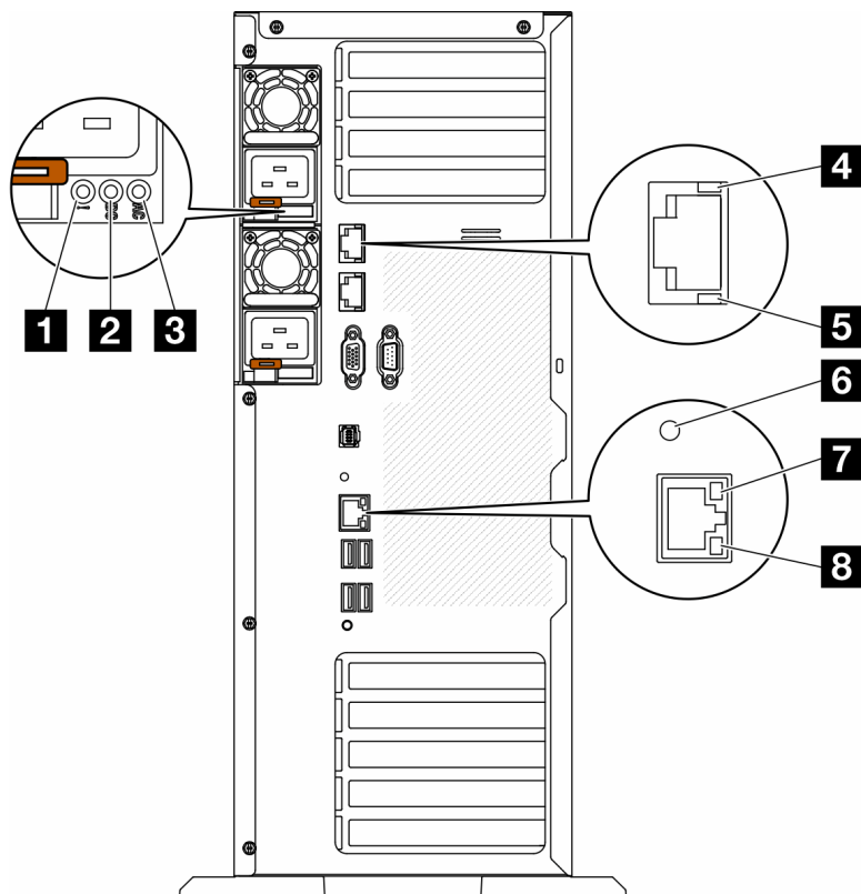
图 12. 服务器的背面系统 LED
