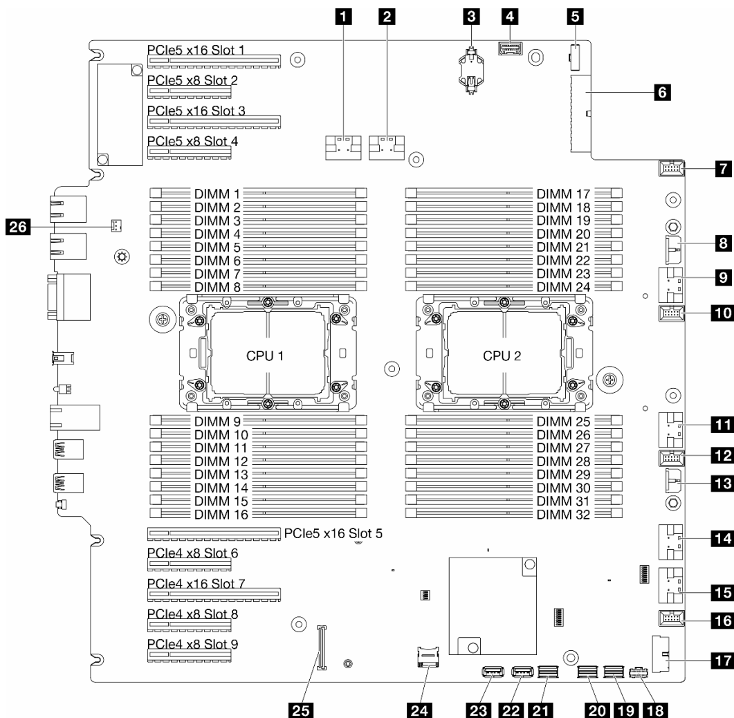
图 7. 主板接口
