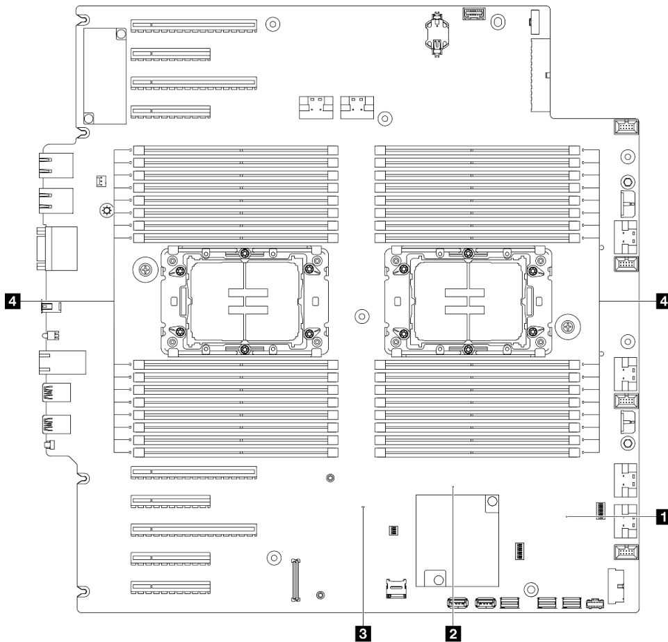
图 13. 主板 LED
