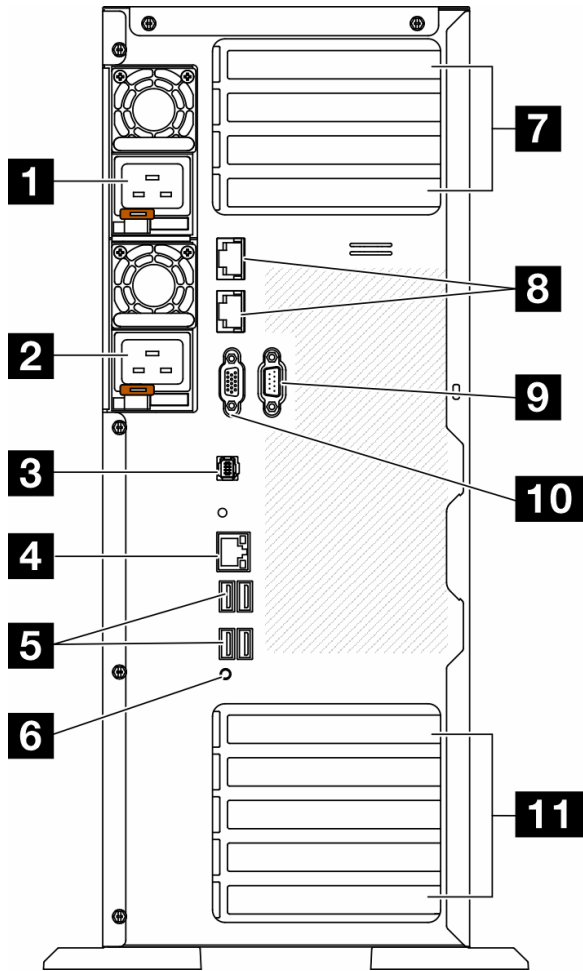
图 5. 后视图
