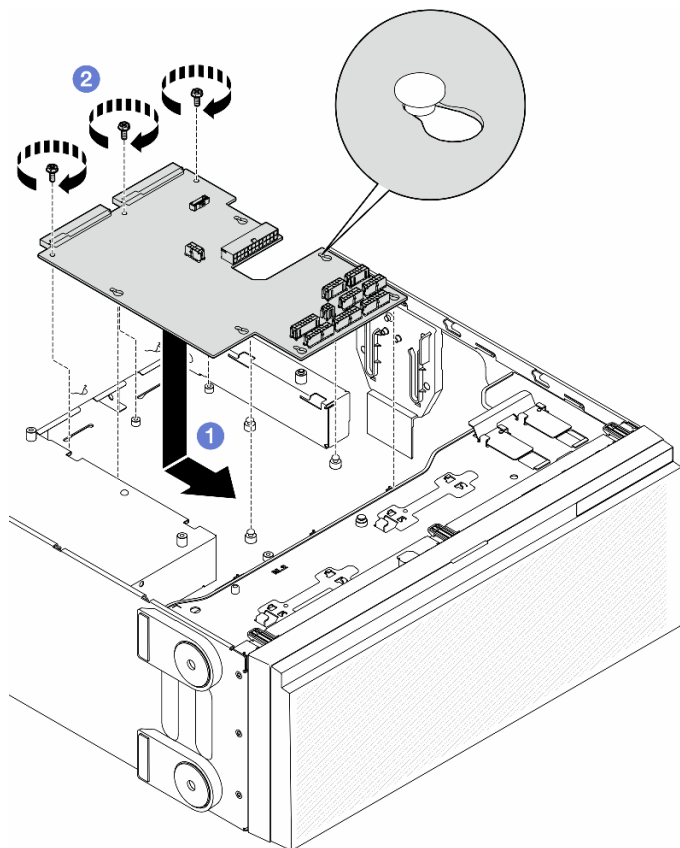
圖例 98. 安裝電源配送板
