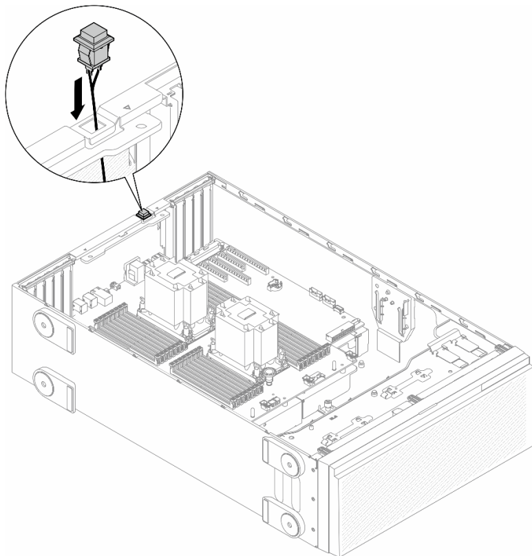
圖例 57. 安裝入侵開關
