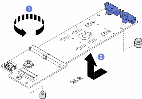
圖例 60. 卸下 M.2 開機配接卡
