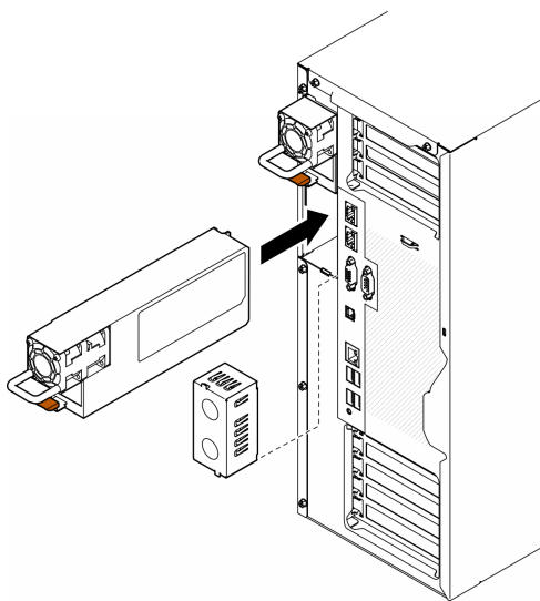
圖例 104. 安裝電源供應器或 PSU 填充板
