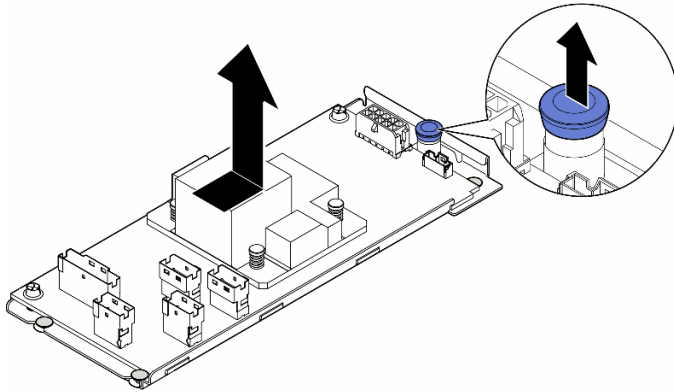
圖例 51. 卸下內部 CFF 配接卡
