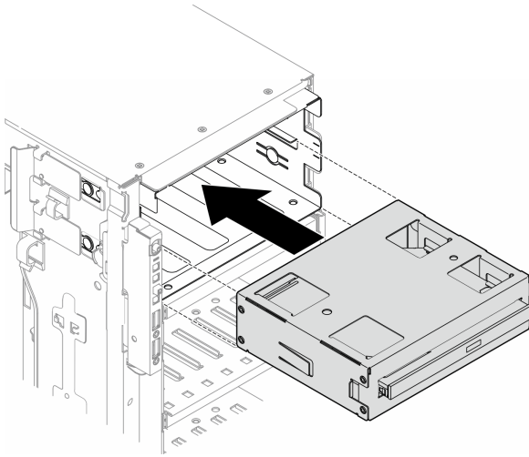
圖例 90. 安裝光碟機組件
