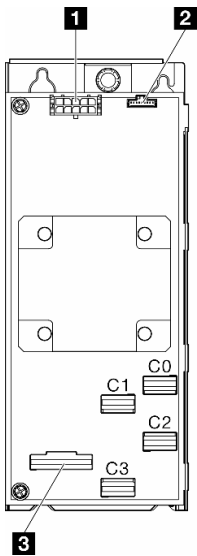
圖例 133. 內部 CFF RAID 配接卡上的接頭
