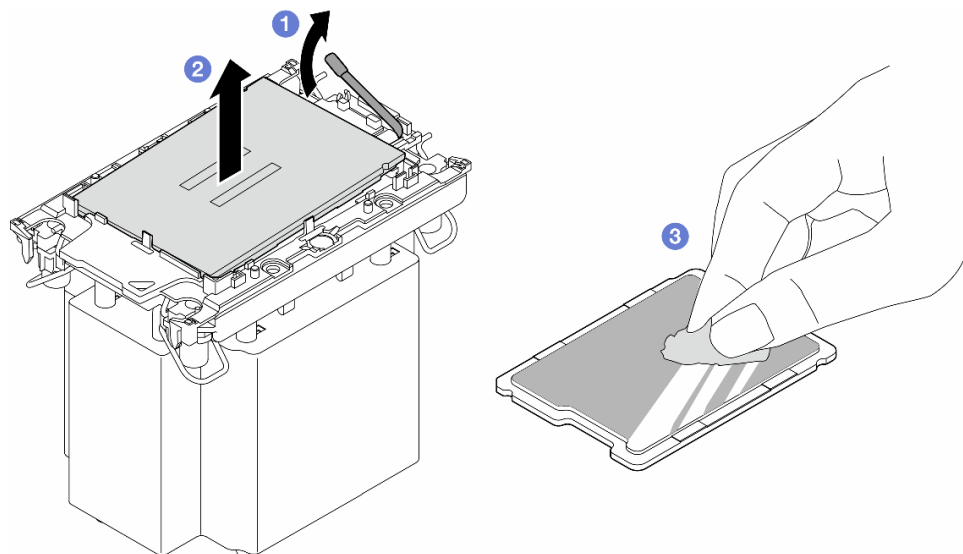
圖例 108. 將處理器與散熱槽和支架分開
