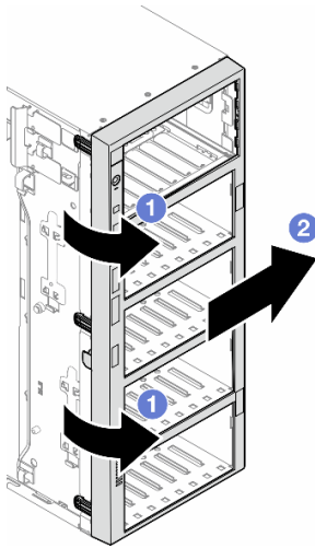
圖例 44. 卸下前方擋板
