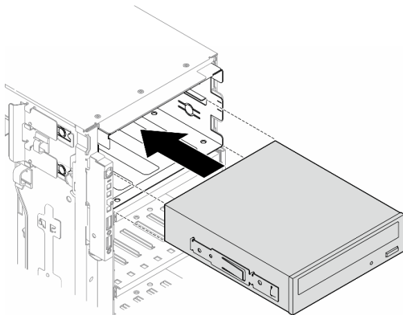
圖例 82. 安裝光碟機
