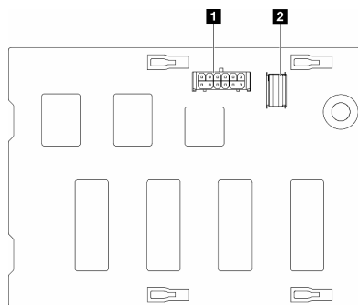
圖例 134. 3.5 吋 SAS/SATA 4 機槽背板接頭
