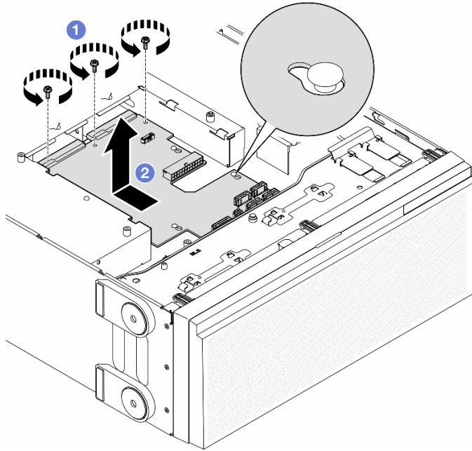
圖例 97. 卸下電源配送板
