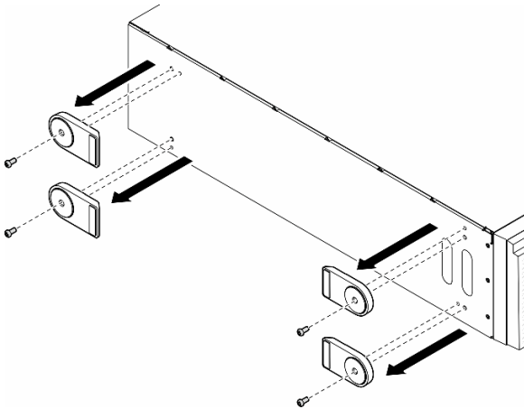
圖例 41. 卸下腳架
