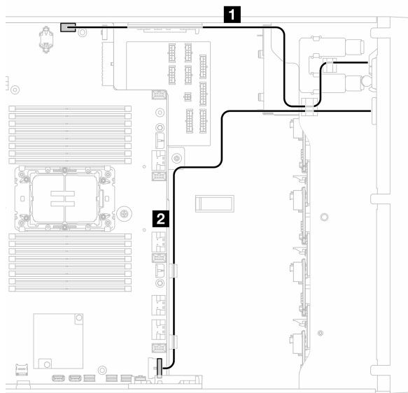
圖例 139. 正面 I/O 模組的纜線佈線
