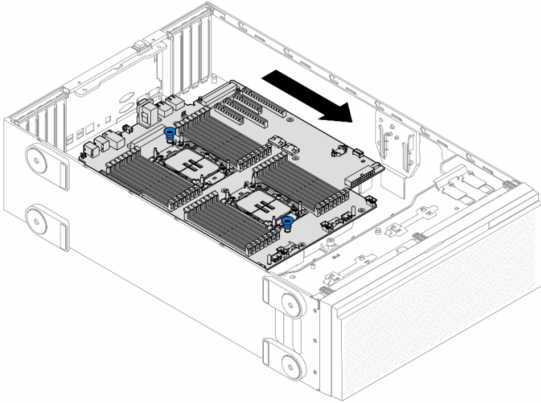
圖例 121. 將主機板脫離機箱
