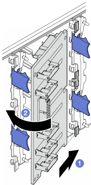
圖例 13. 安裝 2.5 吋硬碟背板
