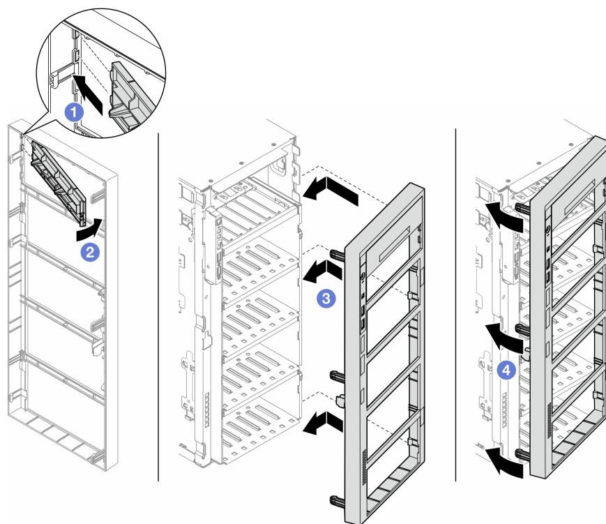
圖例 76. 依序安裝機槽填充板蓋板和前方擋板
