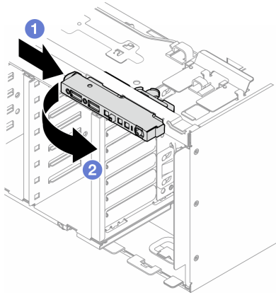
圖例 46. 卸下正面 I/O 模組
