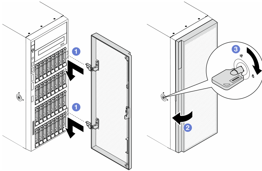
圖例 119. 安裝安全門
