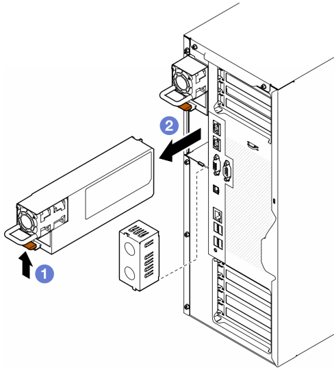
圖例 102. 卸下電源供應器或 PSU 填充板
