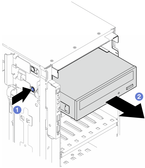
圖例 74. 卸下光碟機
