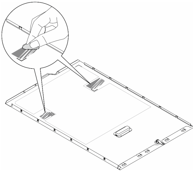
圖例 127. 清潔表面
