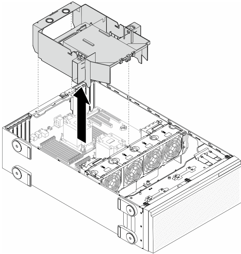
圖例 18. 卸下空氣擋板
