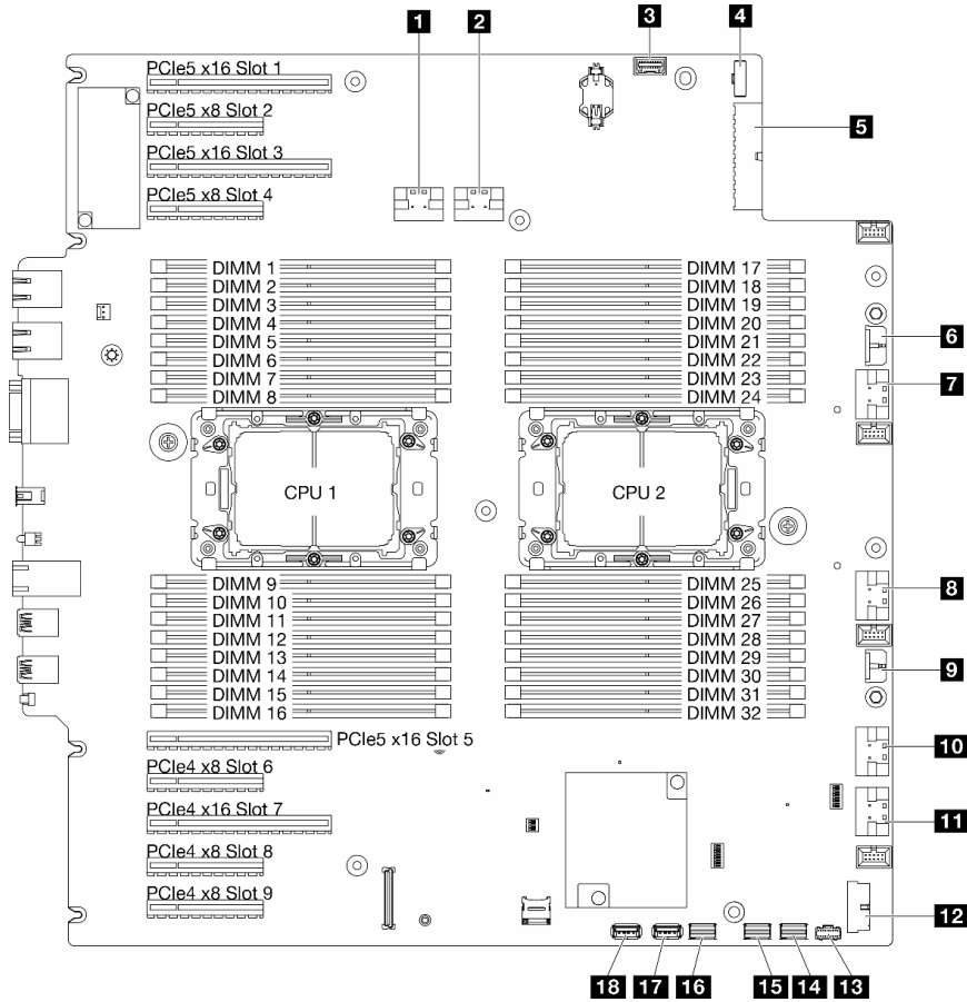
圖例 131. 主機板接頭
