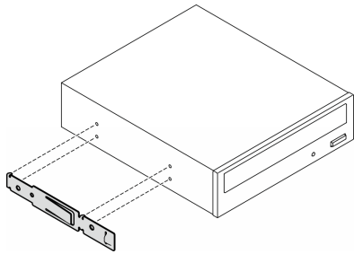
圖例 81. 安裝光碟機固定器
