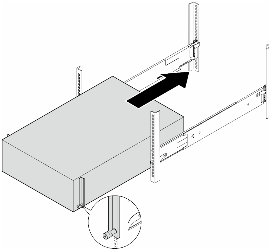
圖例 11. 將伺服器安裝到滑軌
