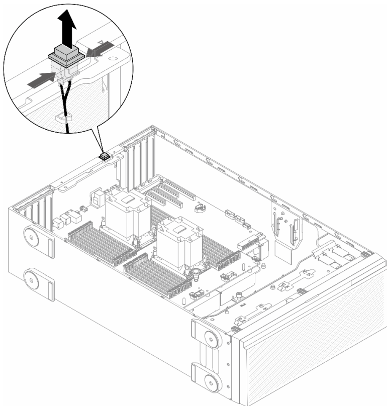
圖例 56. 卸下入侵開關
