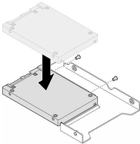
圖例 25. 將 2.5 吋硬碟安裝到硬碟配接器中
