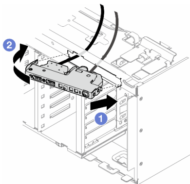
圖例 47. 安裝正面 I/O 模組
