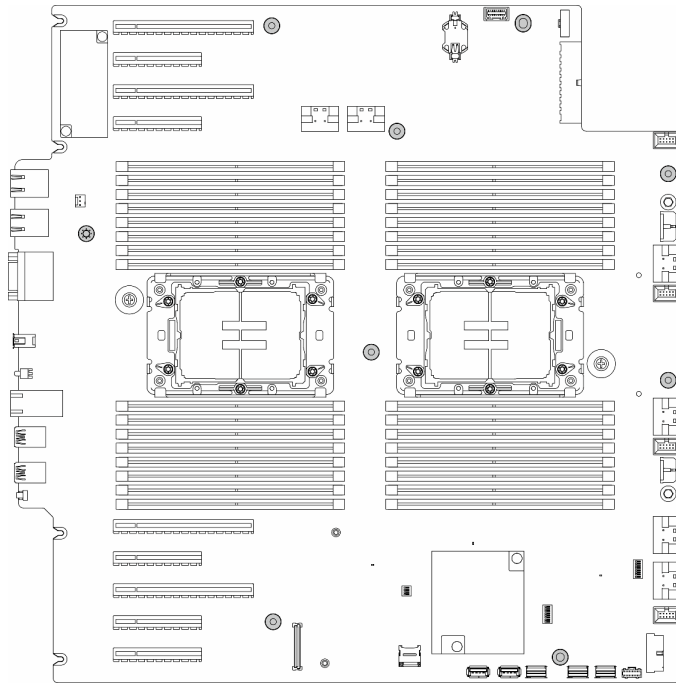
圖例 125. 安裝主機板螺絲
