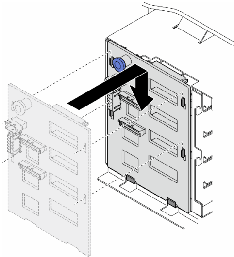
圖例 15. 安裝 3.5 吋硬碟背板
