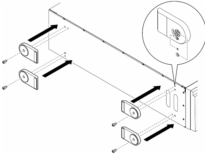
圖例 42. 安裝腳架
