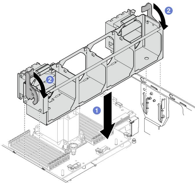
圖例 32. 安裝風扇機盒組件
