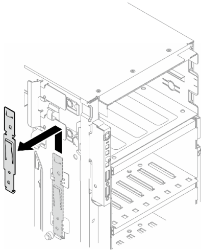
圖例 80. 卸下硬碟固定器
