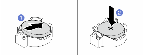
圖例 21. 安裝 CMOS 電池
