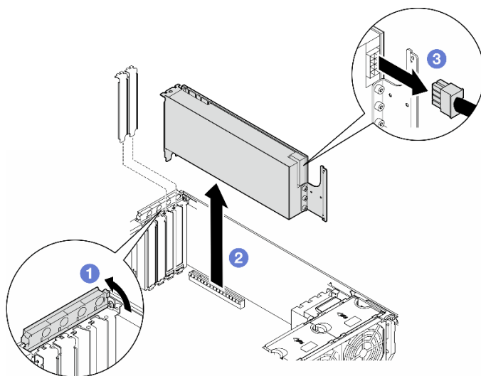
圖例 95. 卸下 FL GPU 配接卡
