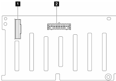
圖例 136. 2.5 吋 SAS/SATA 8 機槽磁碟機背板接頭
