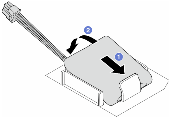
圖例 39. 安裝快閃記憶體電源模組
