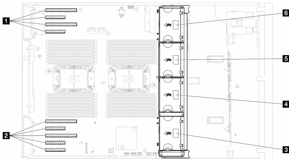
圖例 33. 風扇插槽位置
