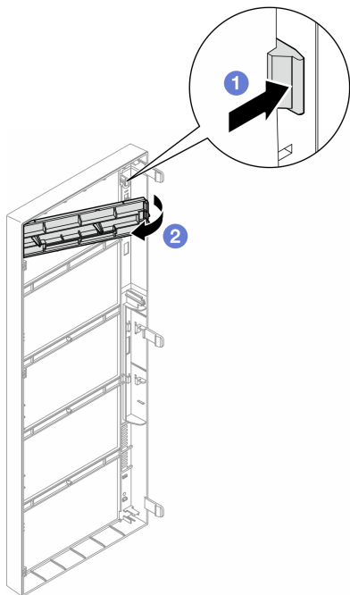
圖例 87. 卸下機槽填充板蓋板
