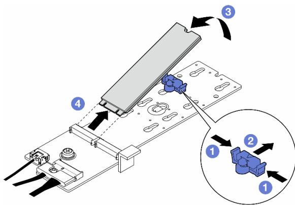
圖例 58. 卸下 M.2 硬碟
