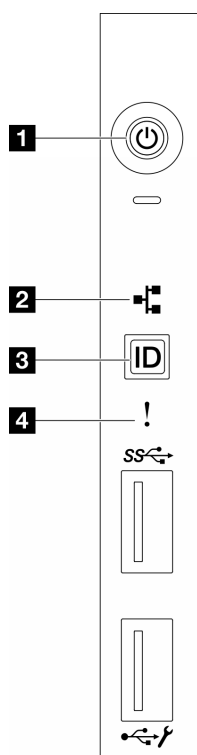
圖例 147. 前方操作面板 LED
