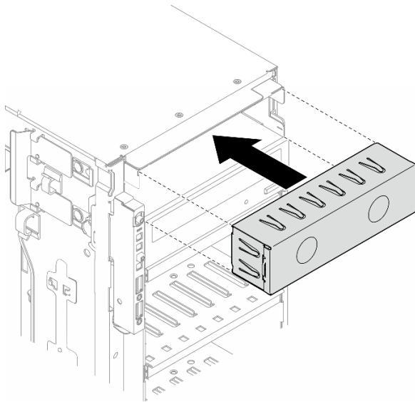
圖例 75. 安裝機槽填充板
