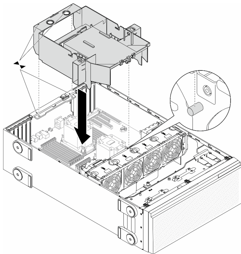
圖例 19. 安裝空氣擋板
