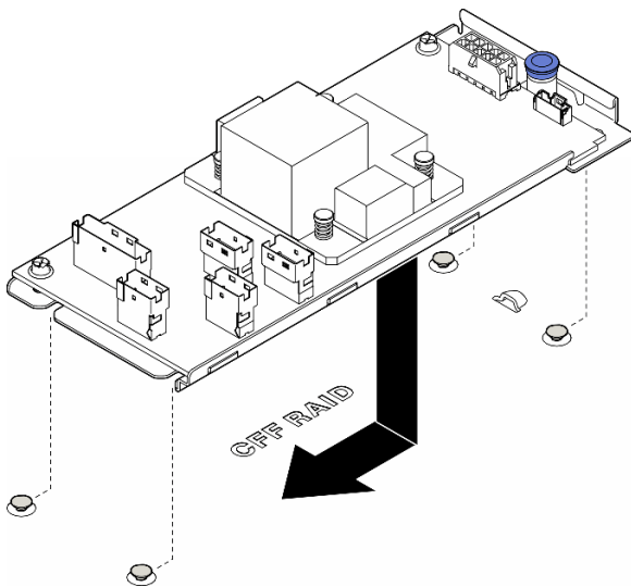
圖例 55. 安裝內部 CFF 配接卡
