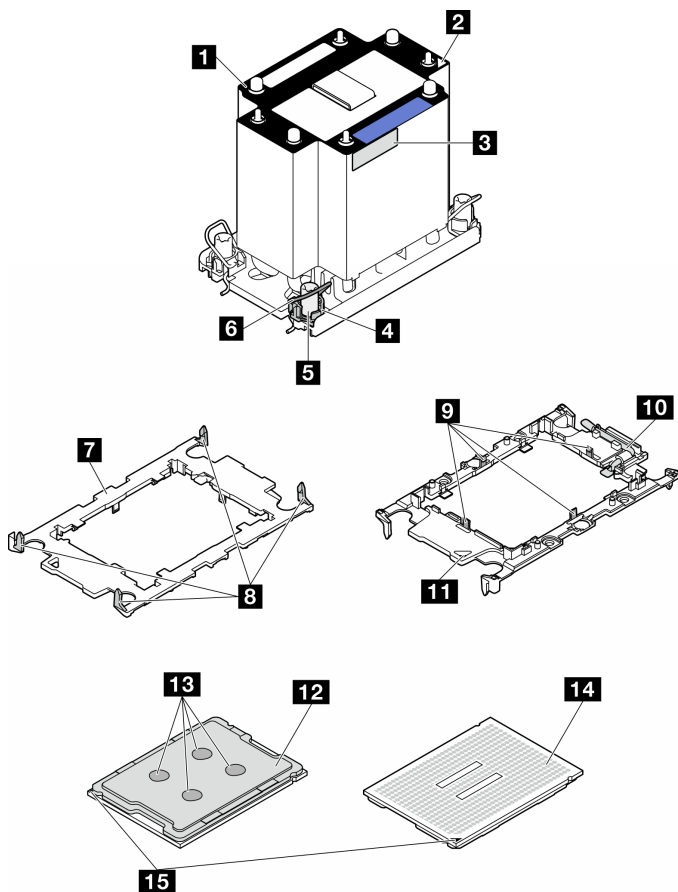
圖例 111. PHM 元件
