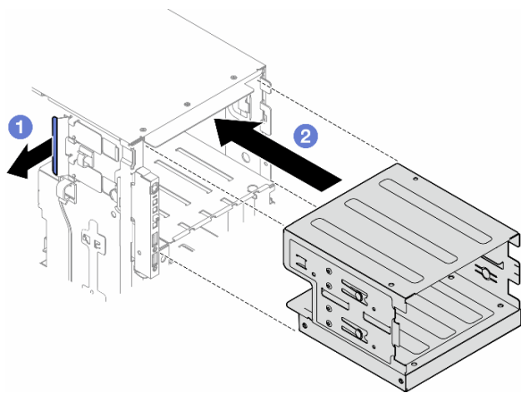
圖例 73. 安裝光碟機機盒
