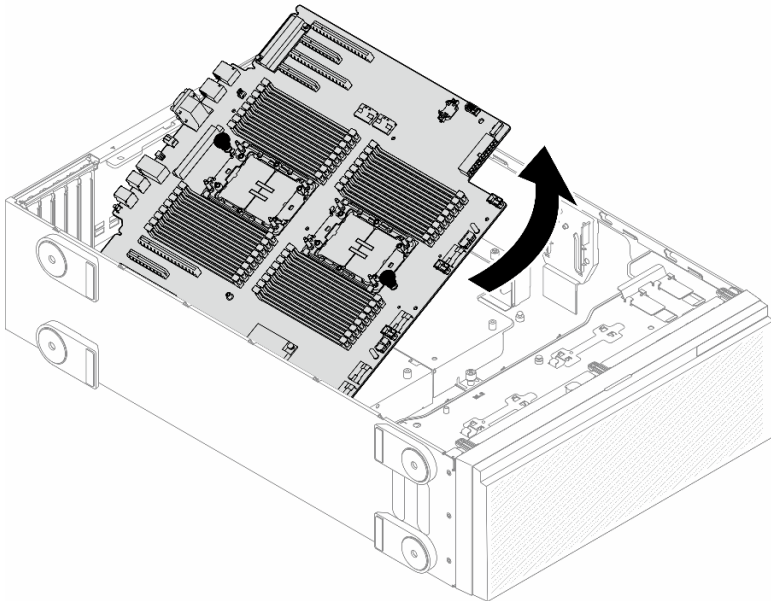
圖例 122. 卸下主機板
