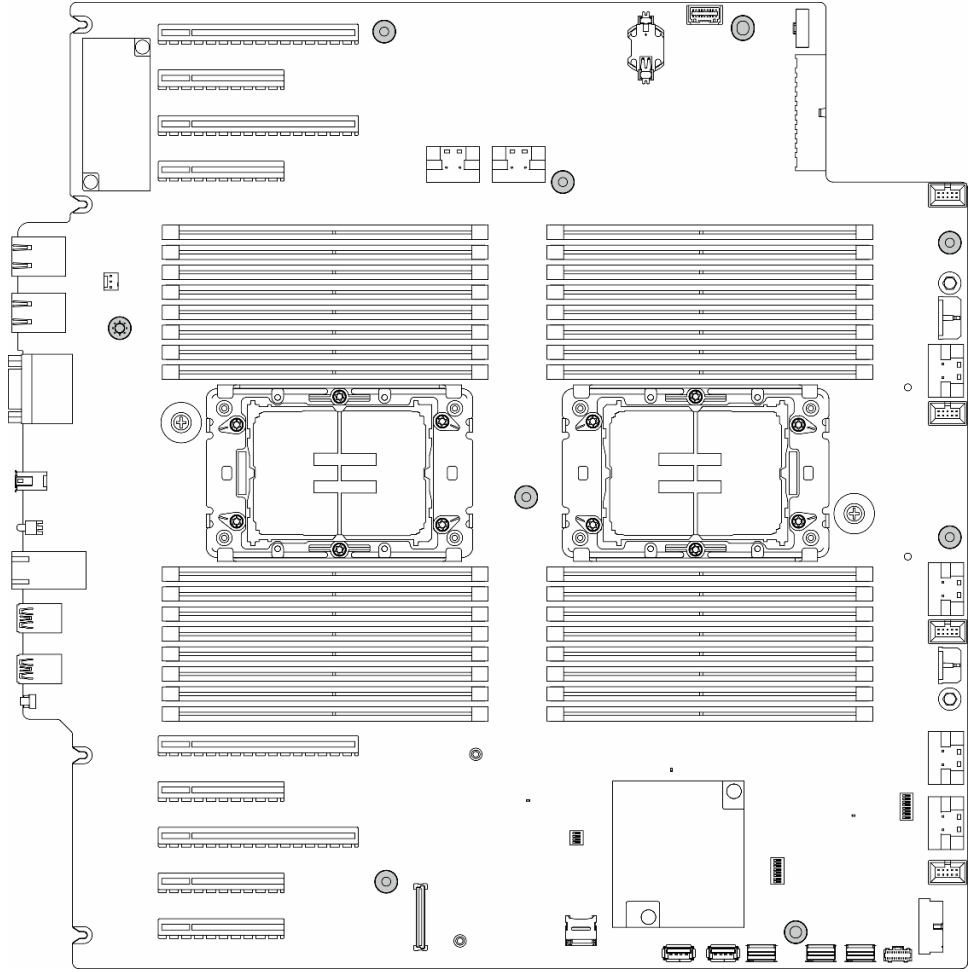
圖例 120. 卸下主機板螺絲
