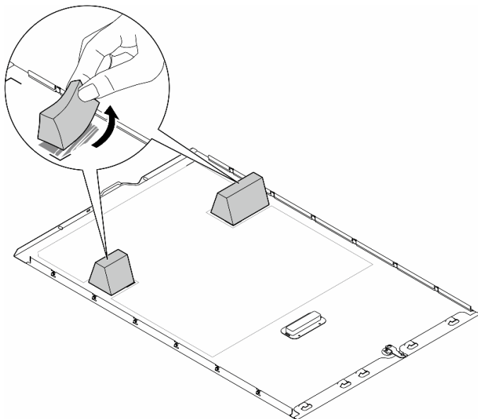
圖例 126. 卸下 T4 填充板
