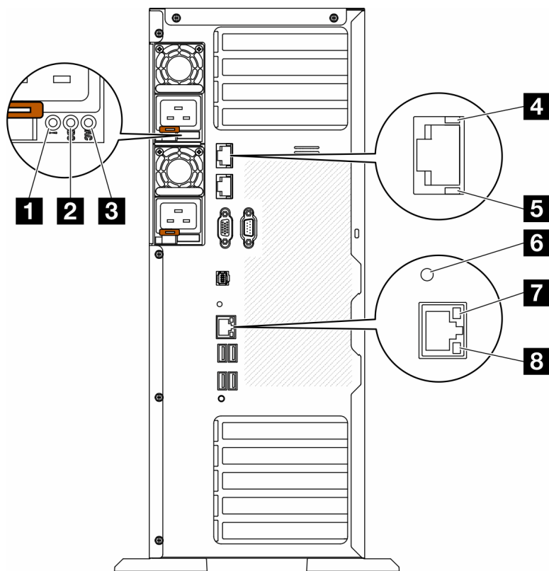
圖例 148. 伺服器的背面系統 LED
