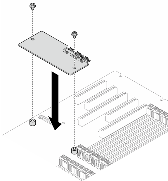
圖例 117. 安裝韌體和 RoT 安全模組
