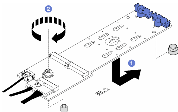
圖例 61. 安裝 M.2 開機配接卡
