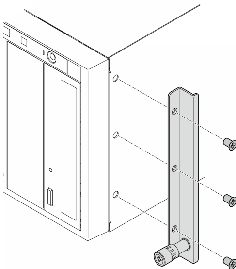
圖例 7. 安裝右邊 EIA 托架
