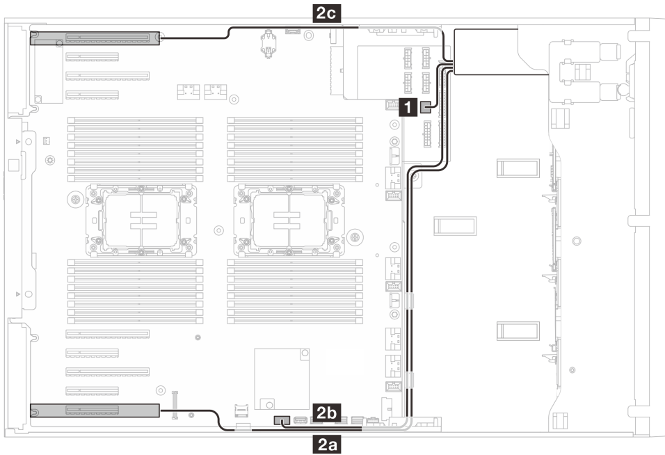
圖例 142. SAS/USB 磁帶機的纜線佈線
