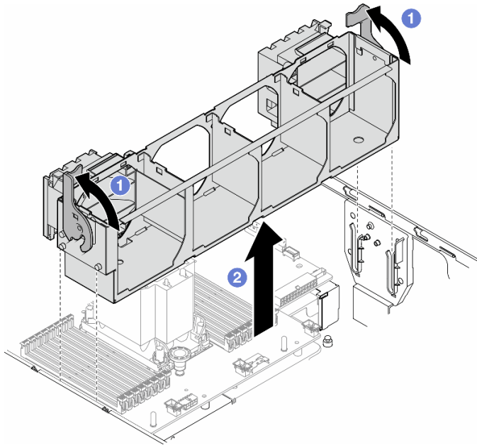
圖例 31. 卸下風扇機盒組件
