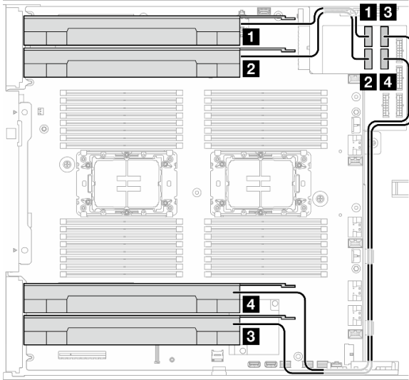
圖例 138. GPU 的纜線佈線
