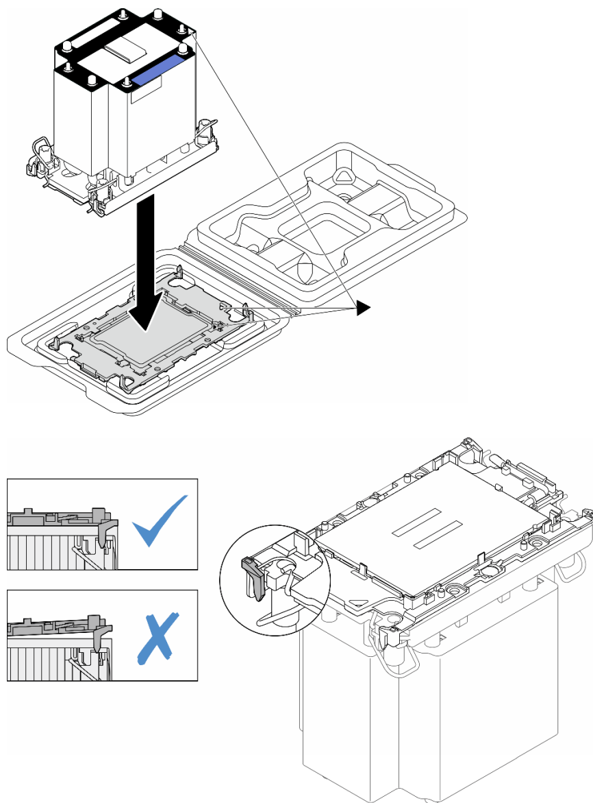
圖例 114. 將 PHM 和處理器裝到運送匣中
