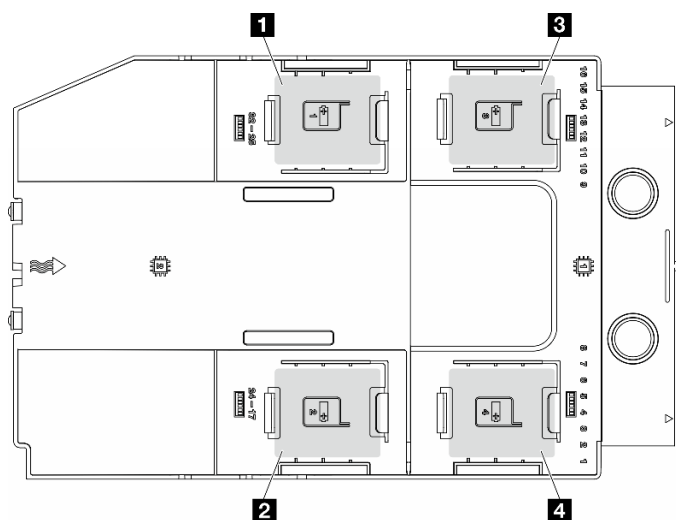
圖例 35. 快閃記憶體電源模組插槽的位置
