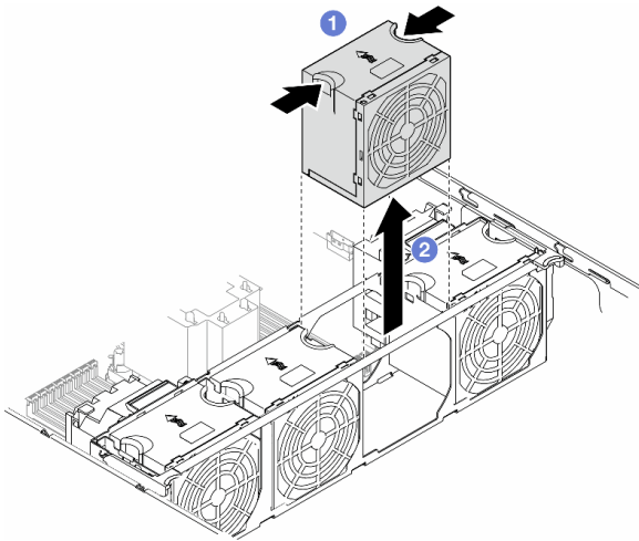
圖例 30. 卸下風扇模組
