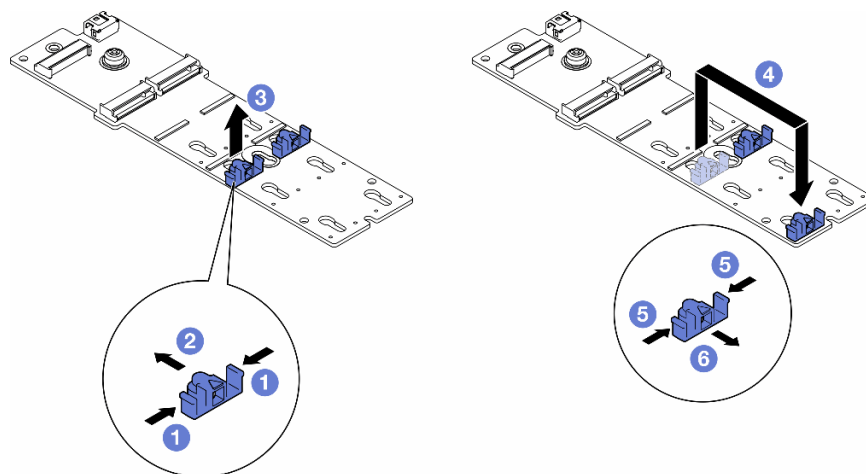
圖例 63. 調整 M.2 固定器
