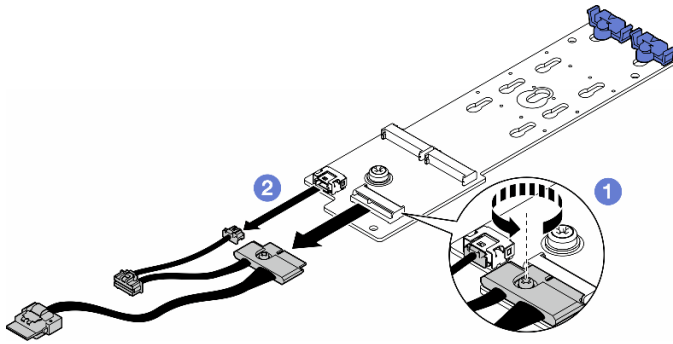
圖例 59. 卸下 M.2 信號線
