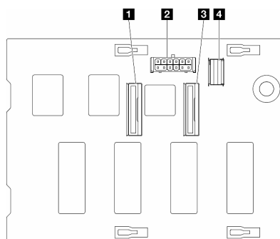
圖例 135. 3.5 吋 SAS/SATA/NVMe 和 NVMe 4 機槽背板接頭
