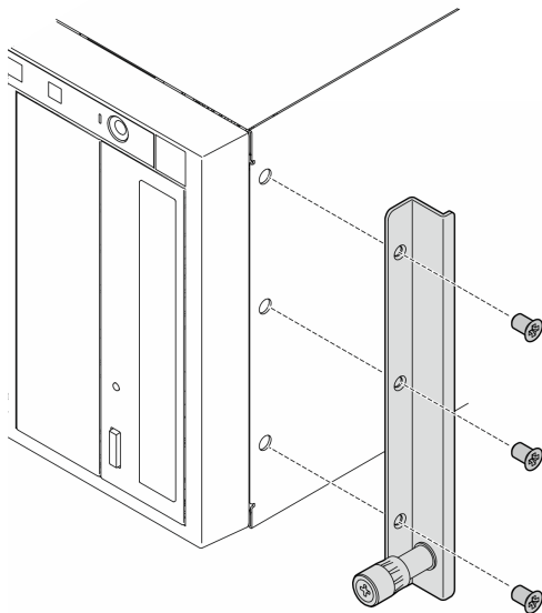
圖例 3. 卸下右邊 EIA 托架
