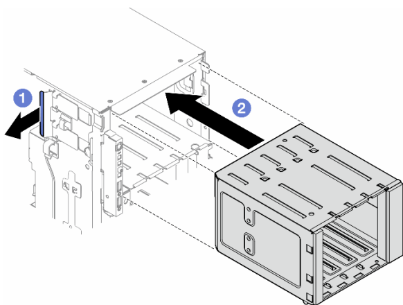
圖例 29. 安裝擴充框架
