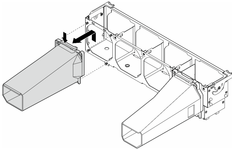
圖例 16. 卸下 A2/L4 GPU 空氣導管
