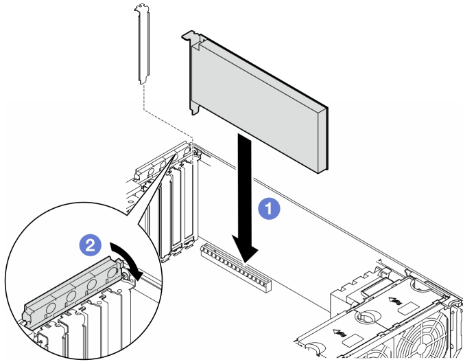
圖例 94. 安裝 HL PCIe 配接卡
