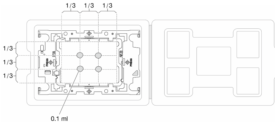
圖例 113. 運送匣中的處理器塗上散熱膏
