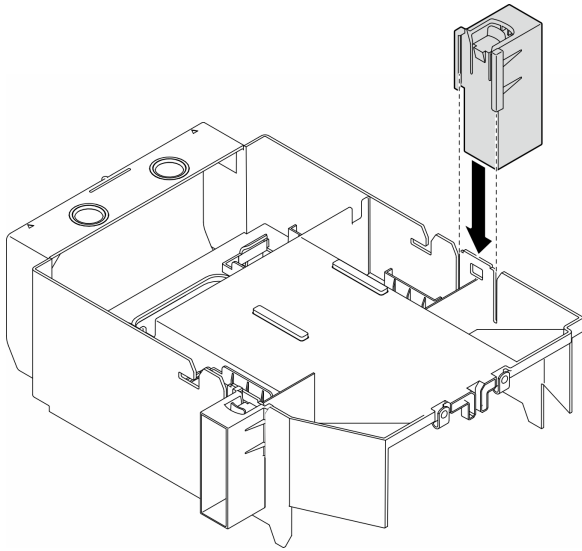
圖例 49. 安裝 FL GPU 填充板
