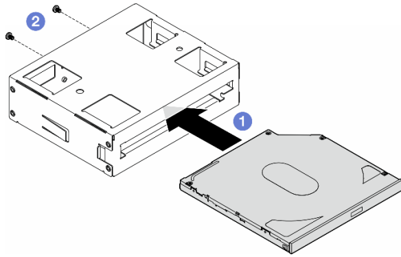
圖例 89. 將 Slim 光碟機安裝到機槽配接器
