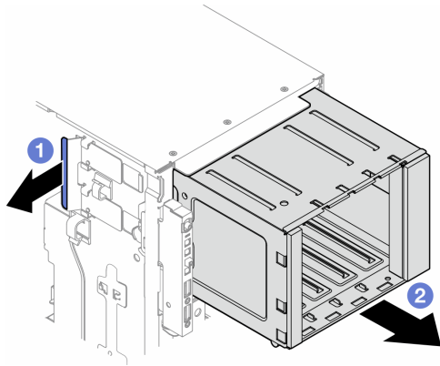
圖例 28. 卸下擴充框架
