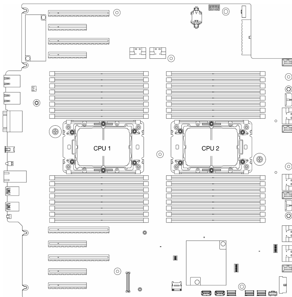
圖例 110. 主機板上的處理器位置
