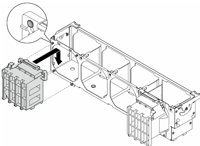
圖例 92. 安裝 FL PCIe 配接卡匣
