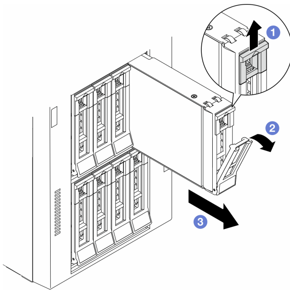
圖例 22. 打開匣把手
