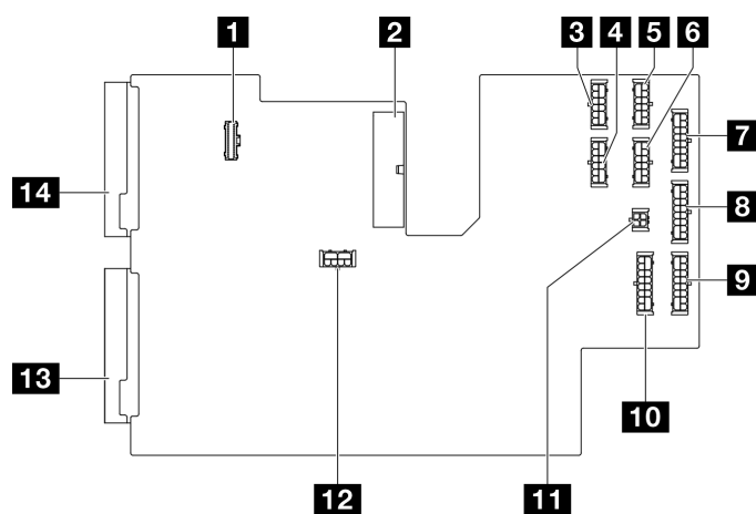
圖例 132. 電源配送板上的接頭
