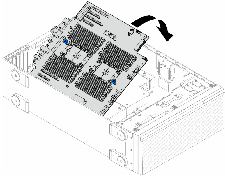
圖例 123. 安裝主機板
