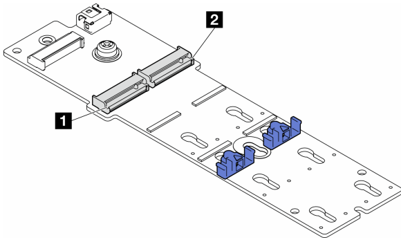
圖例 64. M.2 配接卡上的 M.2 硬碟插槽
