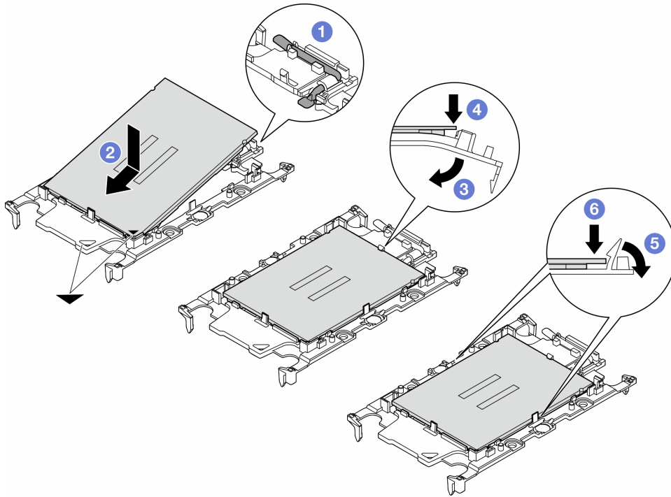
圖例 112. 安裝處理器支架
