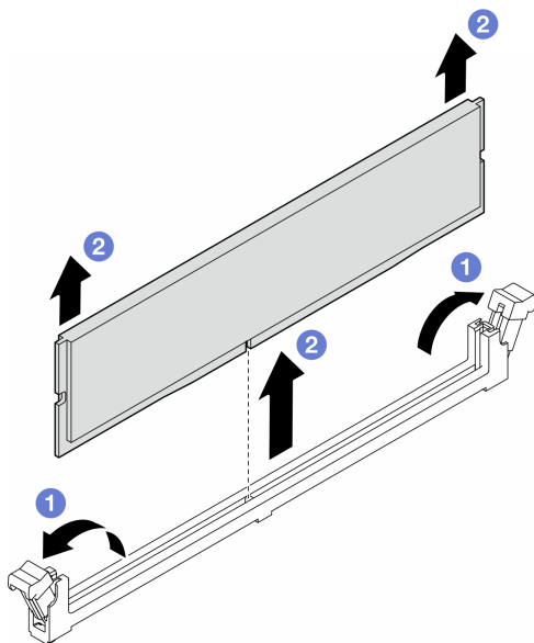
圖例 66. 卸下記憶體模組
