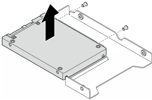
圖例 24. 從硬碟配接器卸下 2.5 吋硬碟
