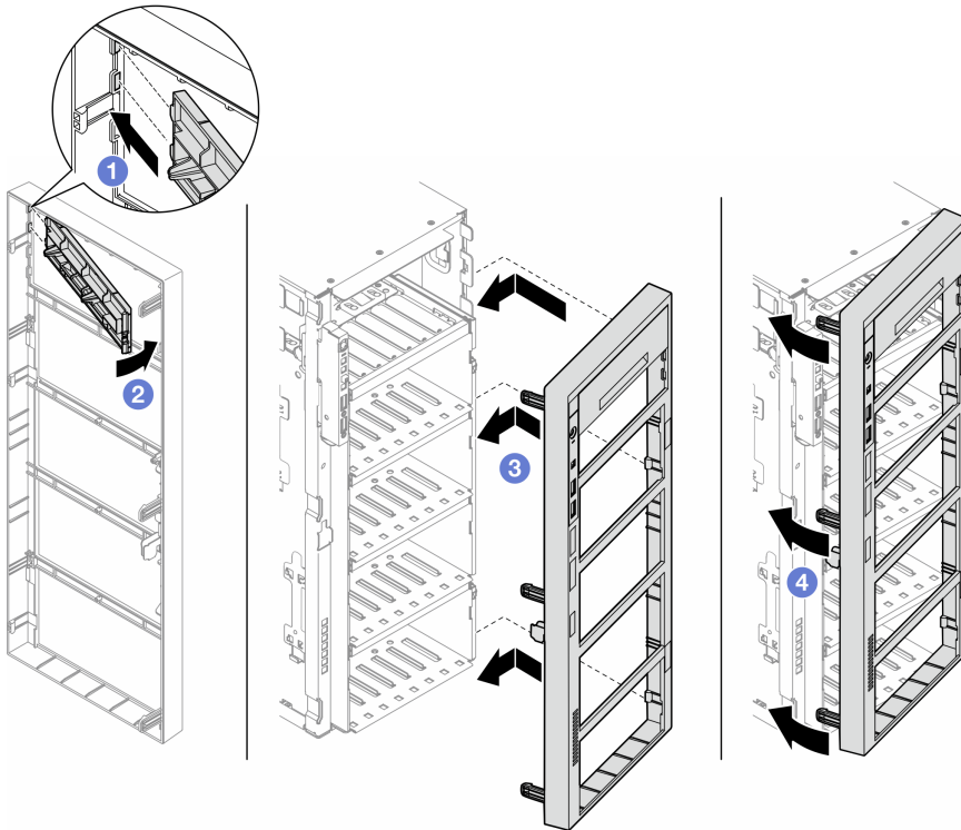
圖例 86. 依序安裝機槽填充板蓋板和前方擋板
