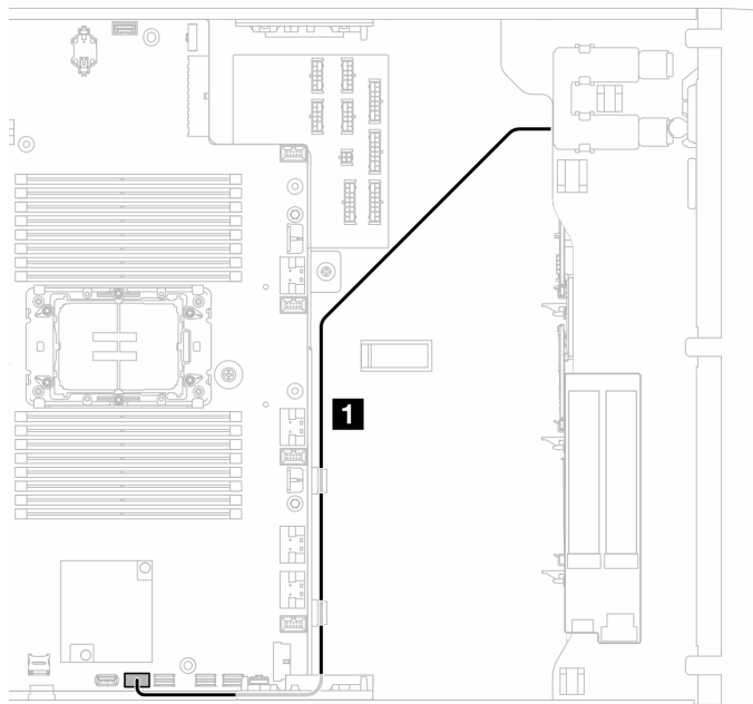
圖例 141. 光碟機纜線佈線
