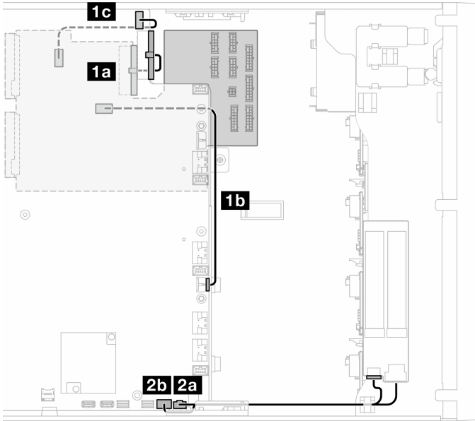
圖例 140. 電源配送板和 M.2 配接卡的纜線佈線
