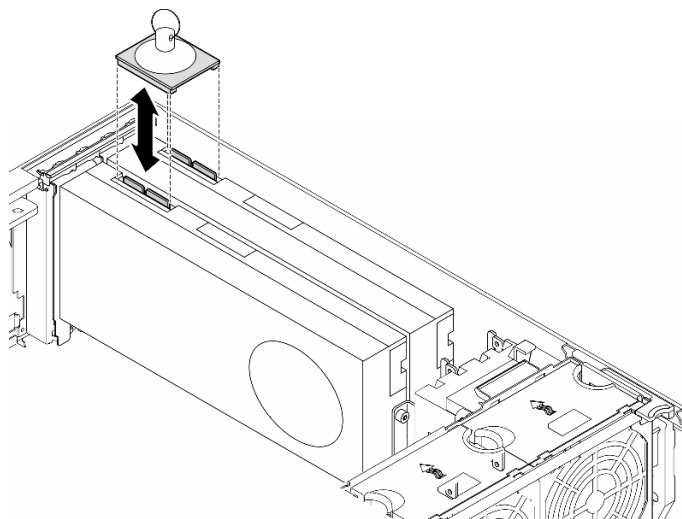
圖例 68. 卸下 NVLink 橋接器
