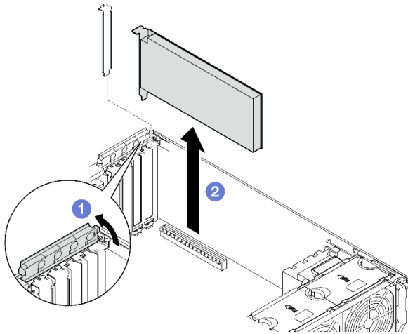
圖例 93. 卸下 PCIe 配接卡
