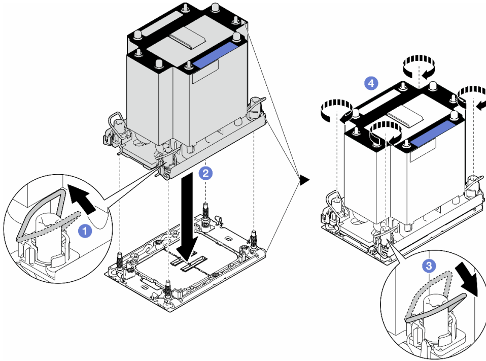
圖例 115. 安裝標準 PHM
