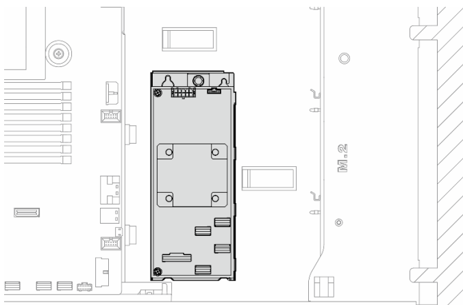
圖例 50. 內部 CFF 配接卡的位置
