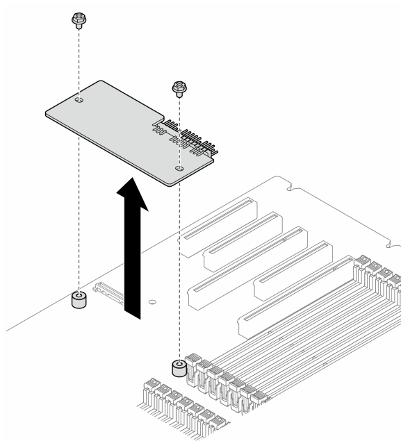
圖例 116. 卸下韌體和 RoT 安全模組
