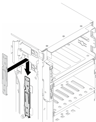
圖例 77. 安裝光碟機或磁帶機的固定器
