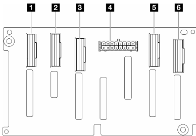
圖例 137. 2.5 吋 SAS/SATA/NVMe 和 NVMe 8 機槽背板接頭
