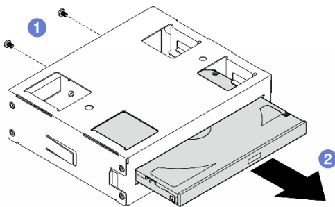
圖例 84. 將 Slim 光碟機從其機槽配接器卸下
