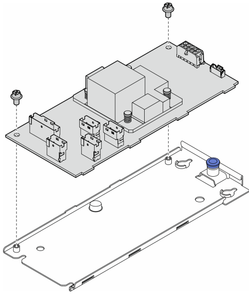
圖例 54. 將內部 CFF 配接卡安裝在其匣上
