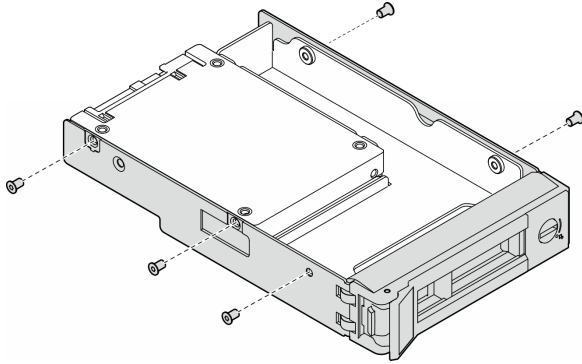
圖例 23. 卸下固定 2.5 吋硬碟和硬碟配接器的螺絲
