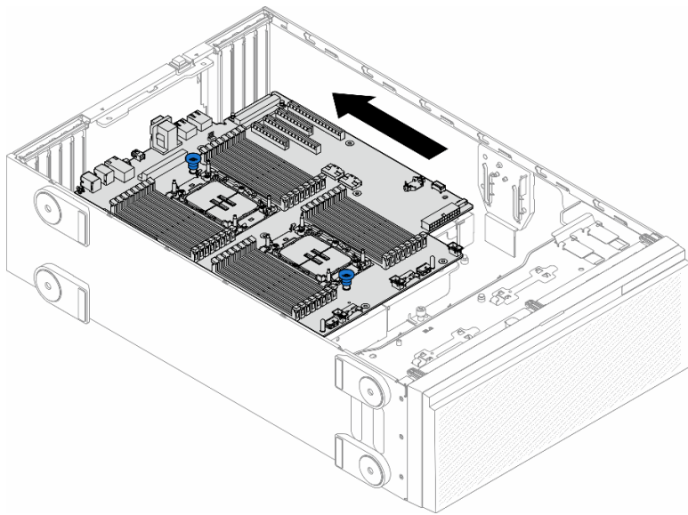
圖例 124. 將主機板嚙合到機箱
