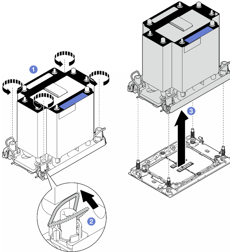
圖例 107. 卸下 PHM
