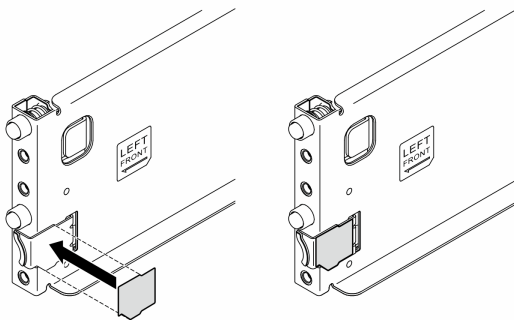
圖例 9. 裝上左邊門鎖蓋板
