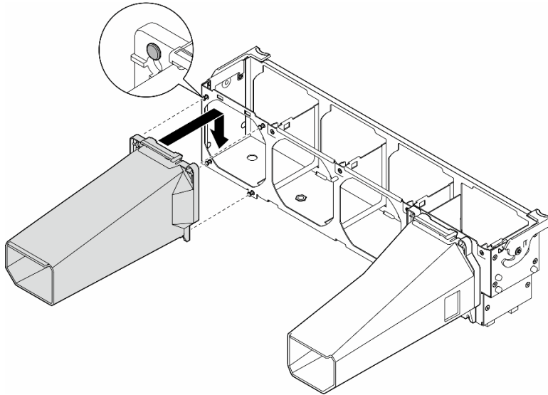
圖例 17. 安裝 A2/L4 GPU 空氣導管
