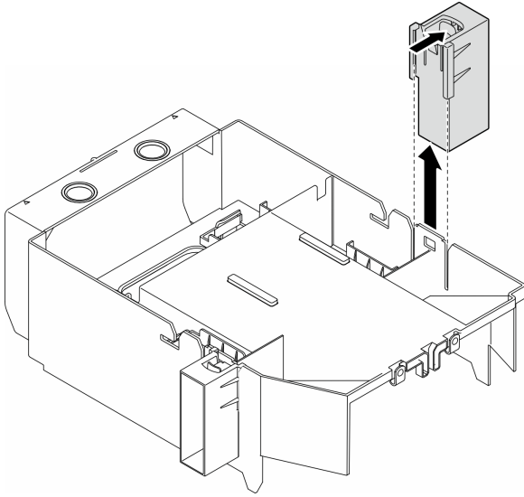
圖例 48. 卸下 FL GPU 填充板
