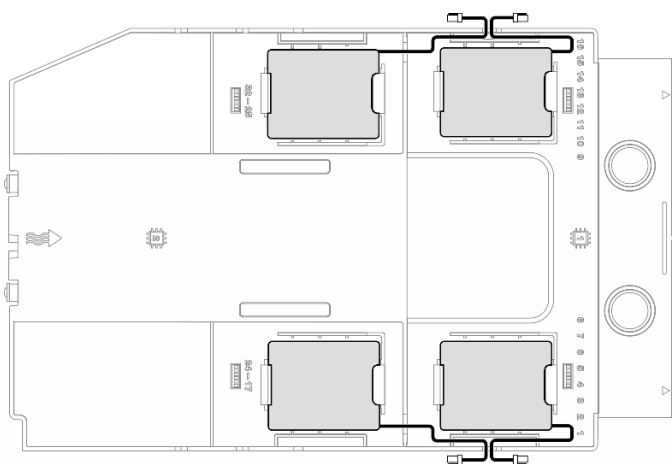
圖例 38. 快閃記憶體電源模組纜線佈線
