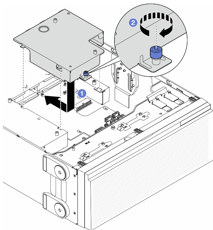
圖例 100. 安裝電源配送板蓋板
