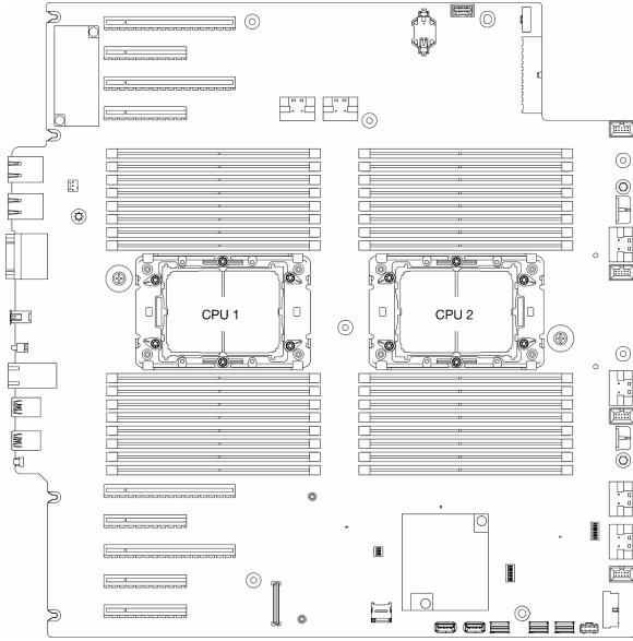
圖例 105. 主機板上的處理器位置
