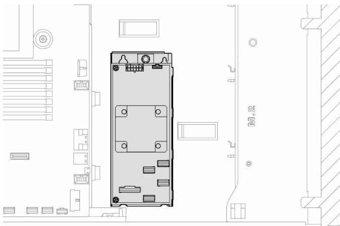
圖例 53. 內部 CFF 配接卡的位置
