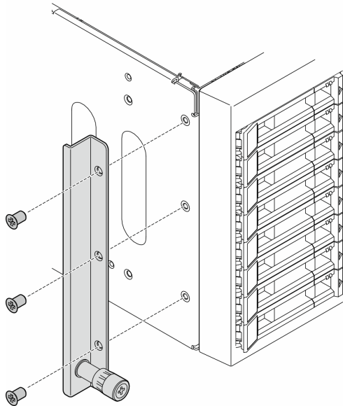
圖例 8. 安裝左邊 EIA 托架
