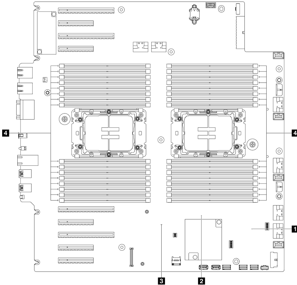
圖例 149. 主機板 LED
