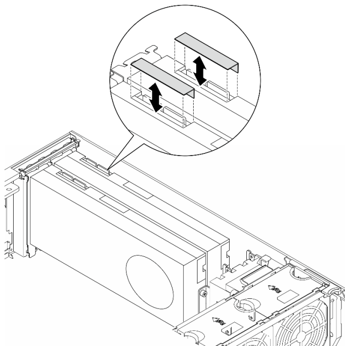
圖例 69. 安裝 NVLink 蓋板
