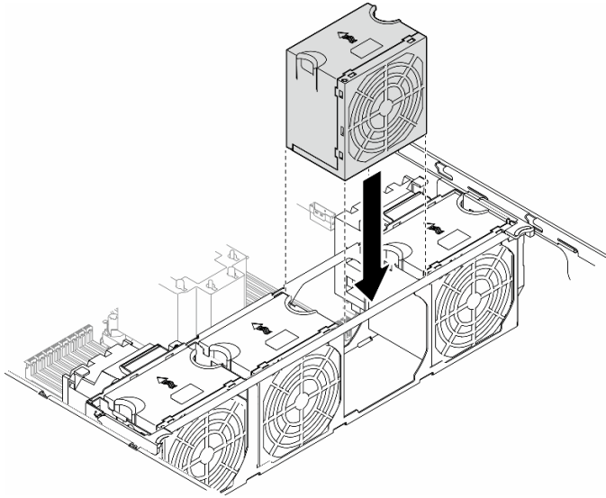
圖例 34. 安裝風扇模組
