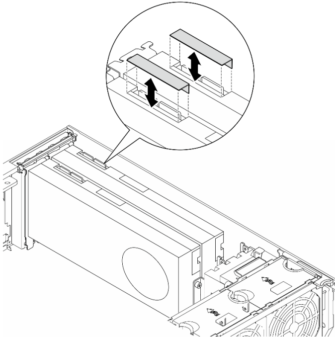
圖例 70. 卸下 NVLink 蓋板
