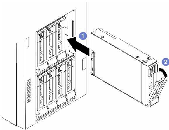
圖例 27. 安裝熱抽換硬碟
