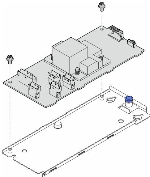
圖例 52. 將內部 CFF 配接卡從匣上卸下
