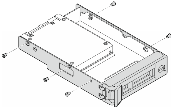
圖例 26. 安裝固定 2.5 吋硬碟和硬碟配接器的螺絲
