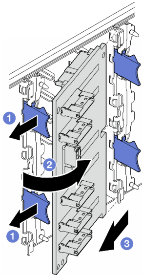
圖例 12. 卸下 2.5 吋硬碟背板
