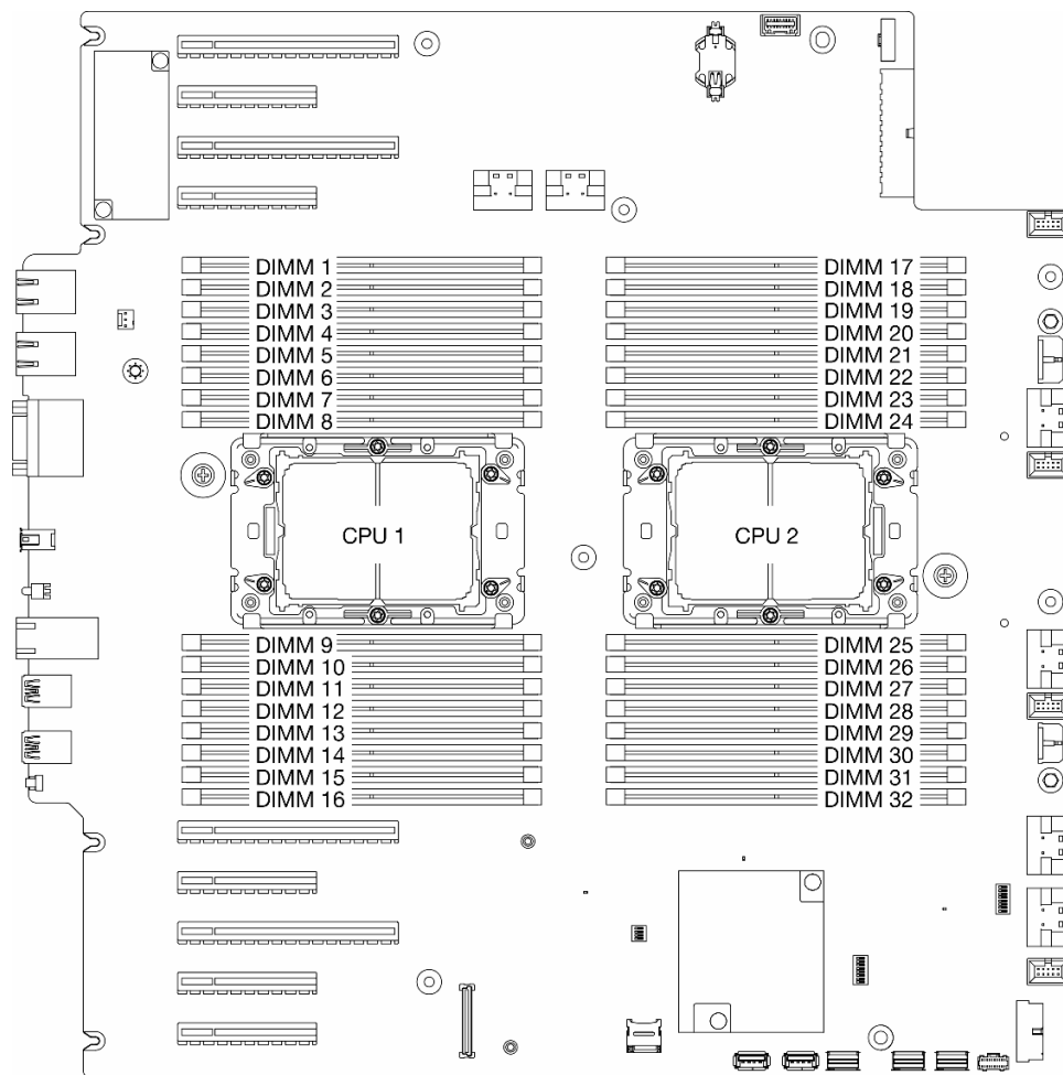
圖例 1. 記憶體模組和處理器佈置
