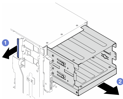
圖例 72. 卸下光碟機機盒
