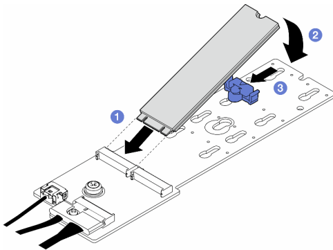
圖例 65. 安裝 M.2 硬碟
