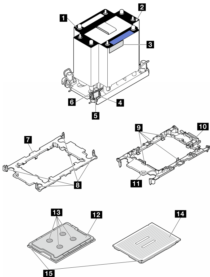
圖例 106. PHM 元件
