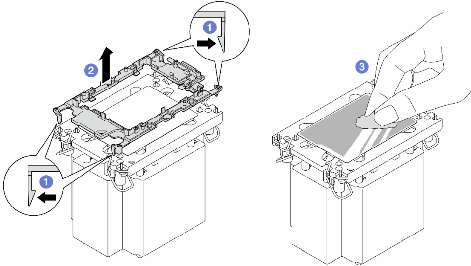
圖例 109. 將處理器支架與散熱槽分開
