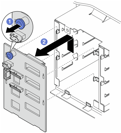
圖例 14. 卸下 3.5 吋硬碟背板
