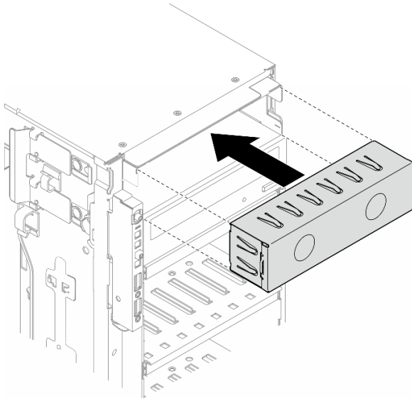
圖例 85. 安裝機槽填充板
