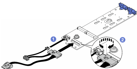
圖例 62. 安裝 M.2 信號線
