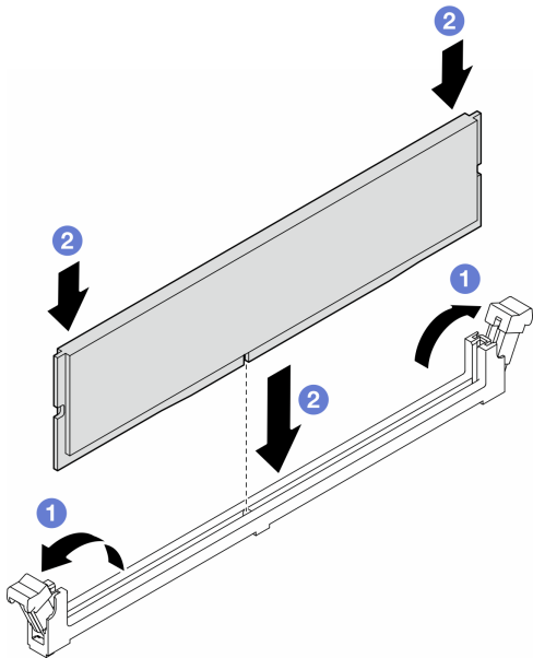
圖例 67. 安裝記憶體模組
