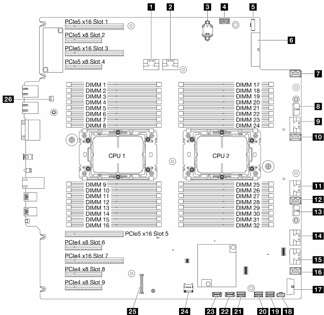
圖例 145. 主機板接頭
