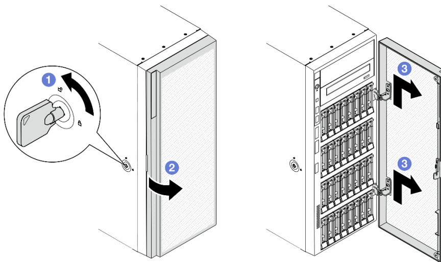
圖例 118. 卸下安全門
