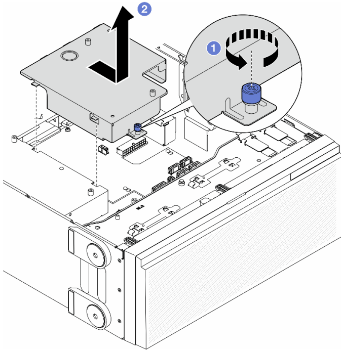
圖例 99. 卸下電源配送板蓋板
