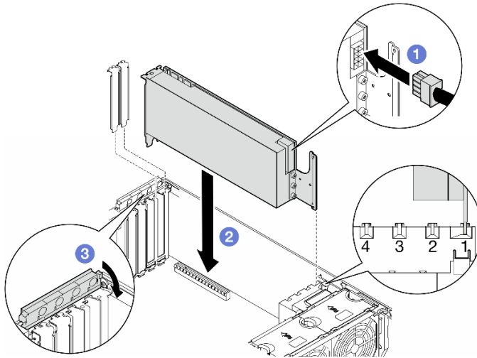
圖例 96. 安裝 FL GPU 配接卡
