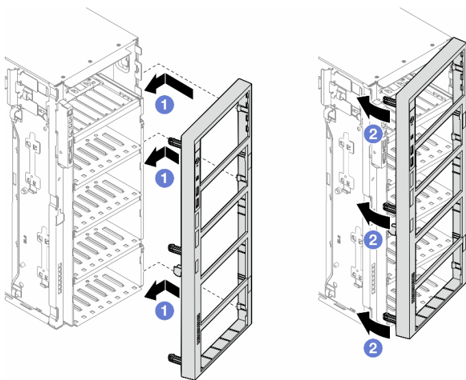
圖例 45. 安裝前方擋板
