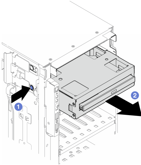
圖例 83. 卸下 5.25 吋機槽配接器組件
