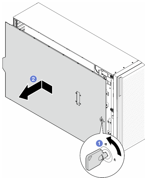
圖例 129. 卸下伺服器蓋板
