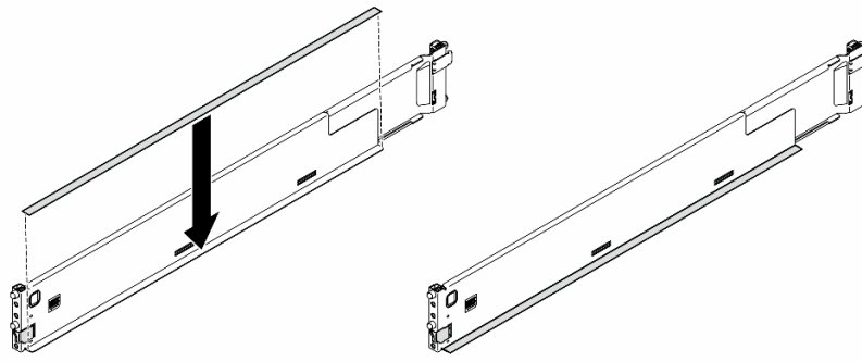
圖例 10. 裝上左邊滑軌蓋板條
