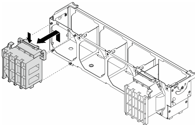
圖例 91. 卸下 PCIe 配接卡匣
