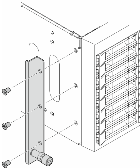
圖例 4. 卸下左邊 EIA 托架
