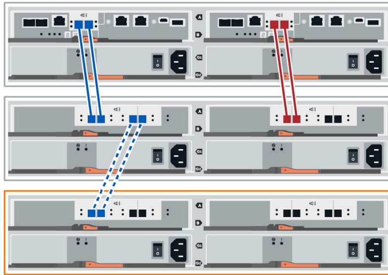
Figura 12. Diagrama de pila única (modelos de 2U)
