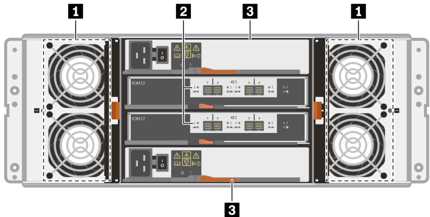
Figura 10. Vista posterior de DE600S (4U)
