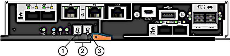
Figura 61. Pantalla de siete segmentos
